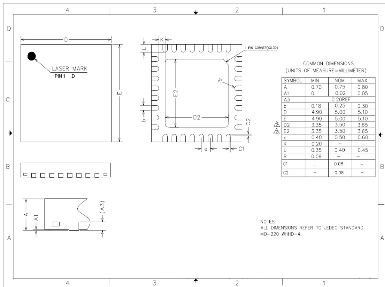
图 5-5 QFN32(5mmx5mm)封装尺寸
