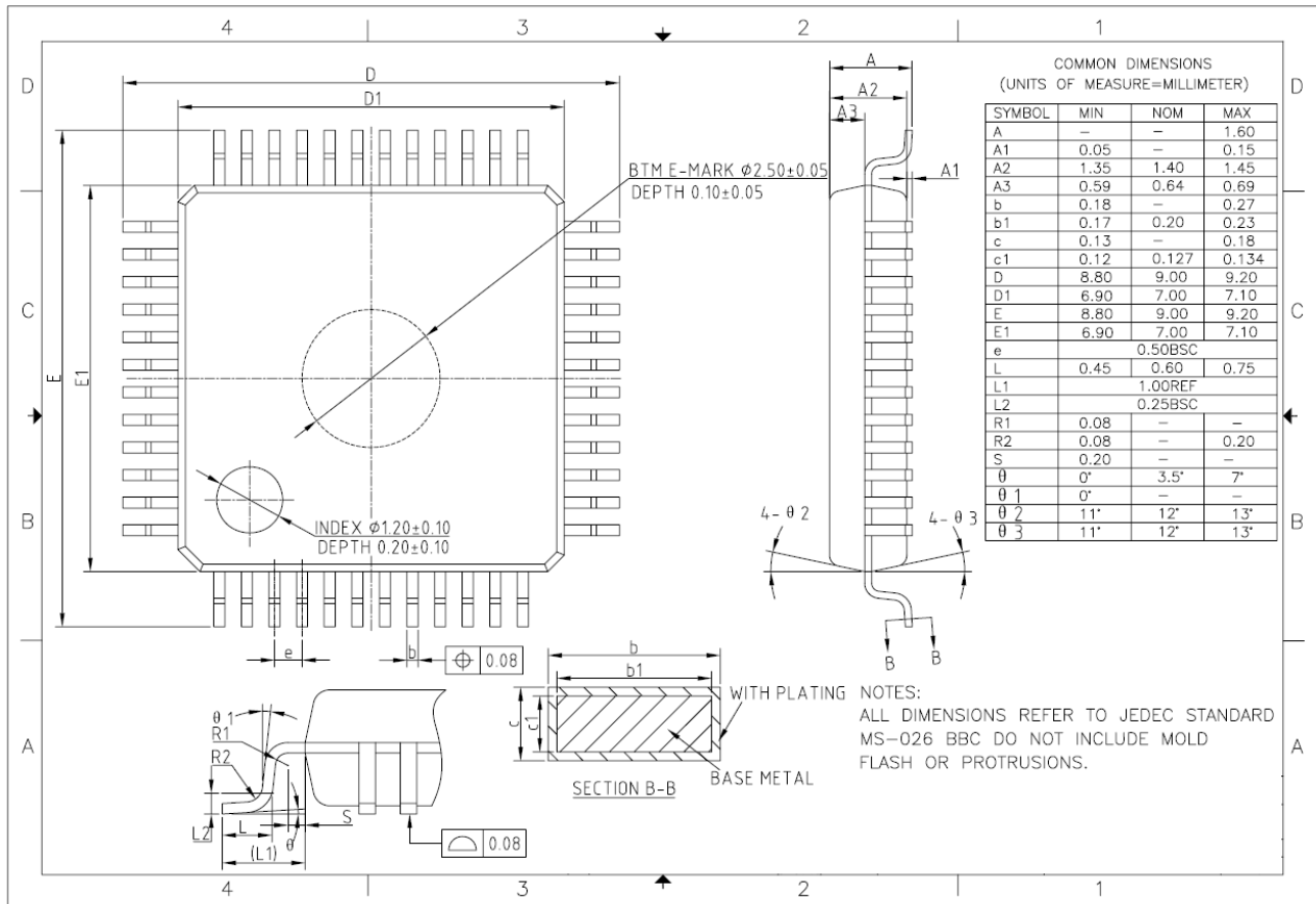
图 5-1 LQFP48 封装尺寸
