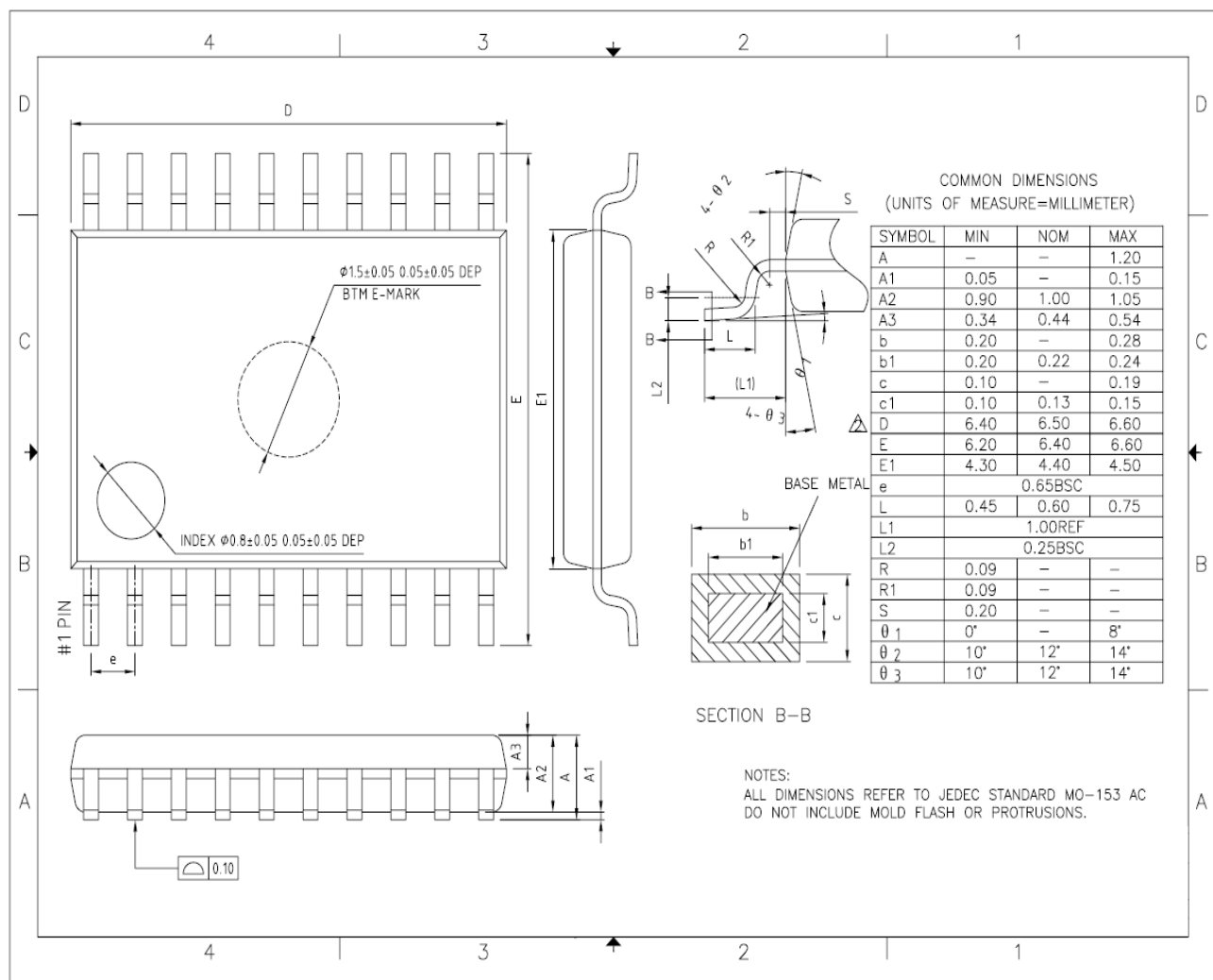
图 5-11 TSOP20 封装尺寸
