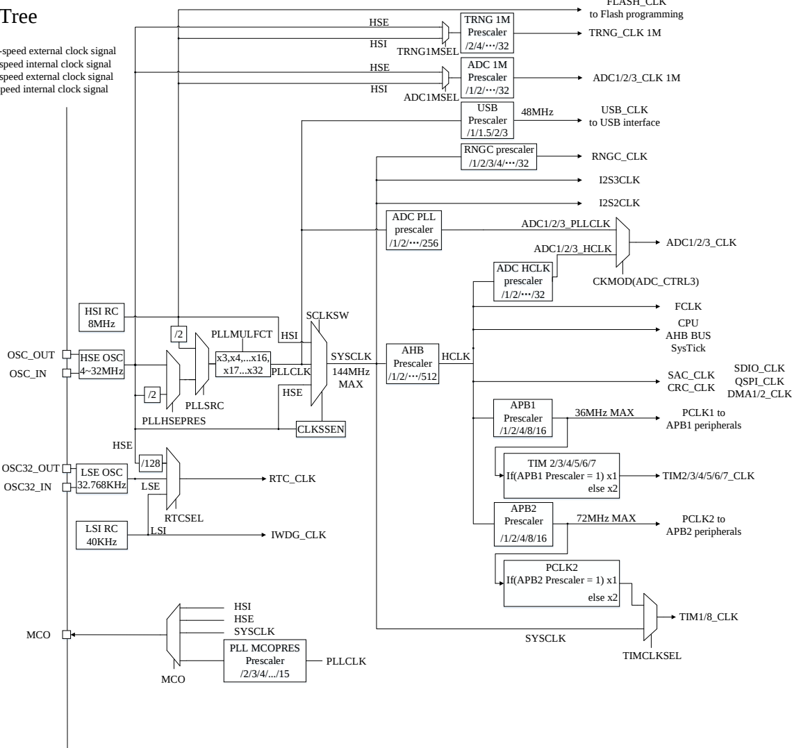
图 2-2 时钟树
