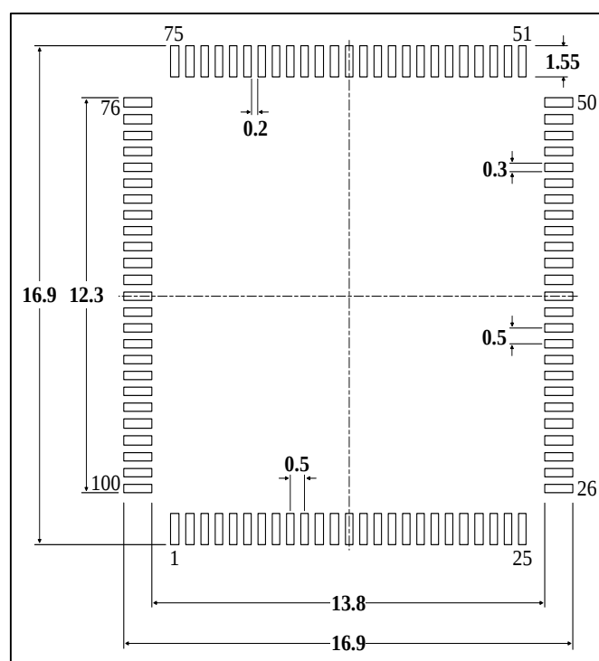
图 5-6 LQFP100封装焊盘建议 (1)
