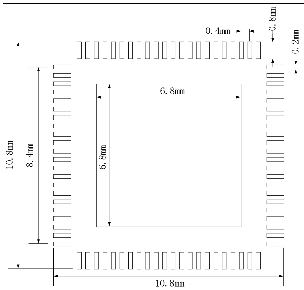
图 5-6 QFN88封装焊盘建议 (1)
