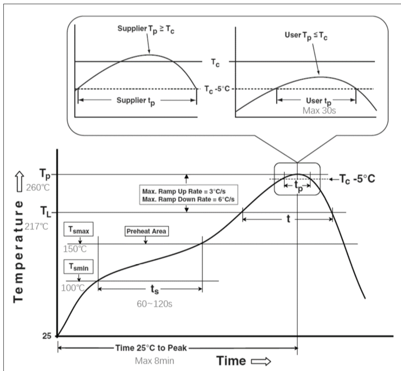
图 4-25 SMT焊接温度特性曲线图
