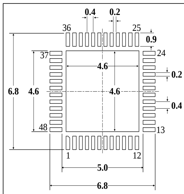
图 5-2 QFN48封装焊盘建议 (1)
