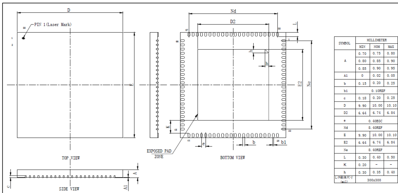
图 5-6 QFN88封装焊盘建议 (1)
