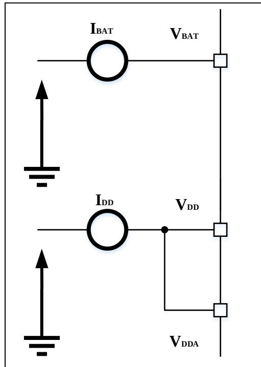
图 4-4 电流消耗测量方案
