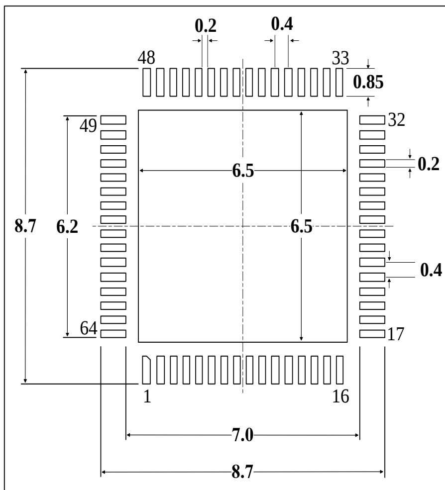
图 5-4 QFN64封装焊盘建议 (1)
