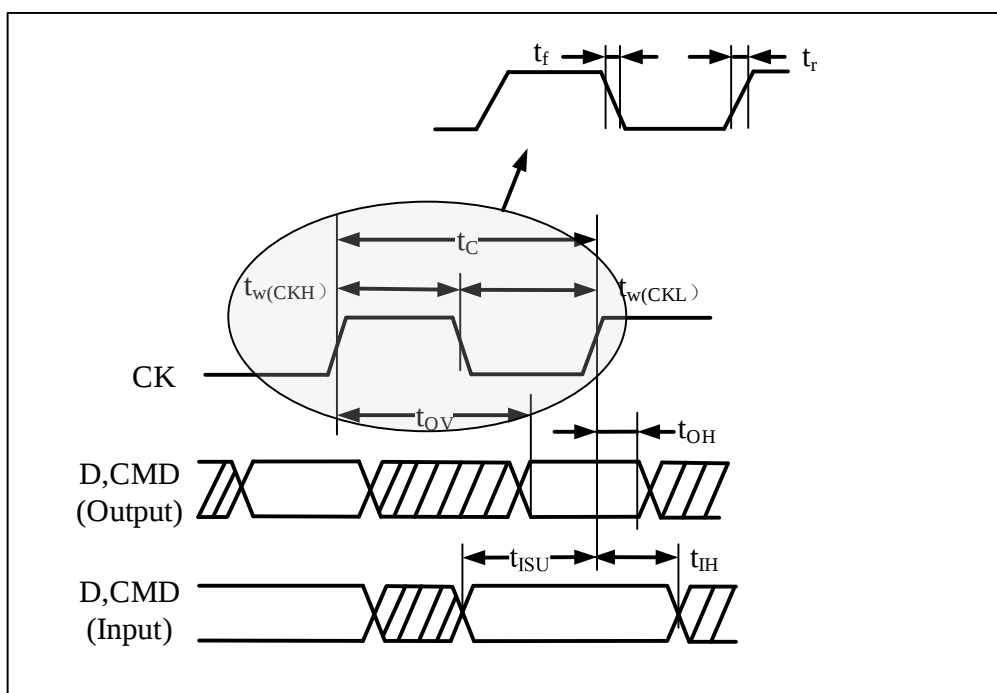
图 4-18 SDIO高速模式
