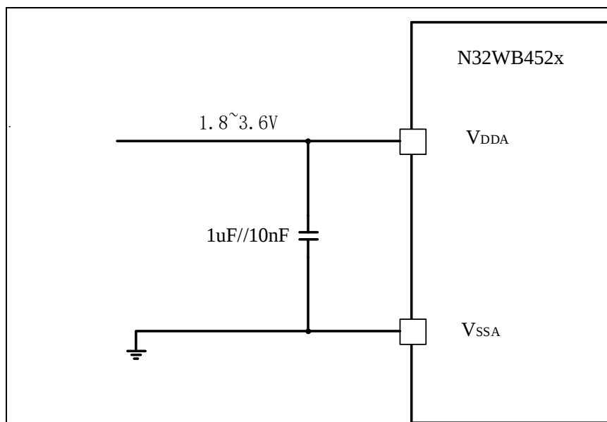
图 4-24 供电电源和参考电源去藕线路
