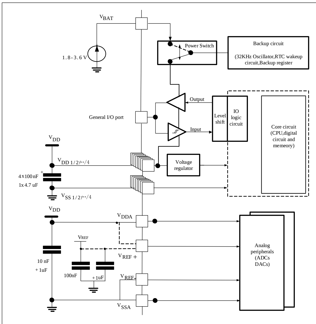
图 4-3 供电方案(非蓝牙部分)
