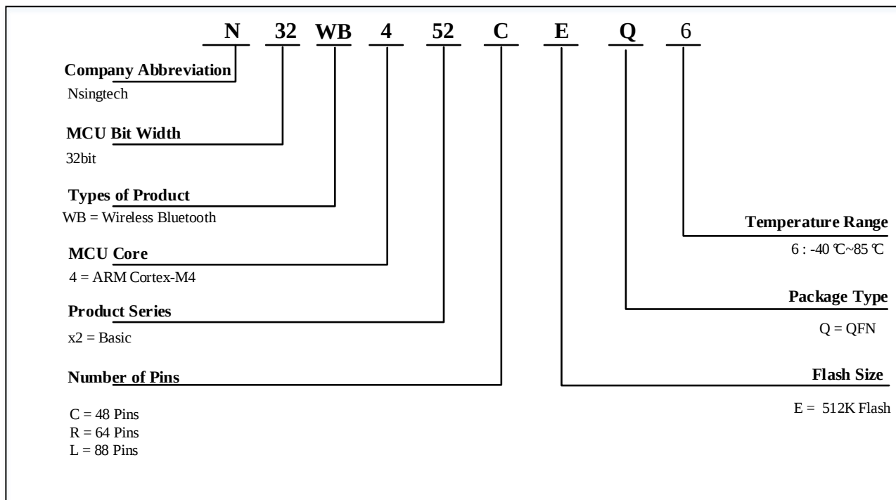
图 6-1 N32WB452系列订货代码信息图示
