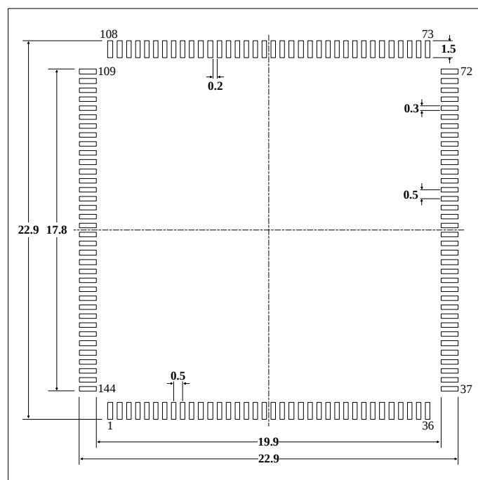
图 5-8 LQFP144 封装焊盘建议 (1)
