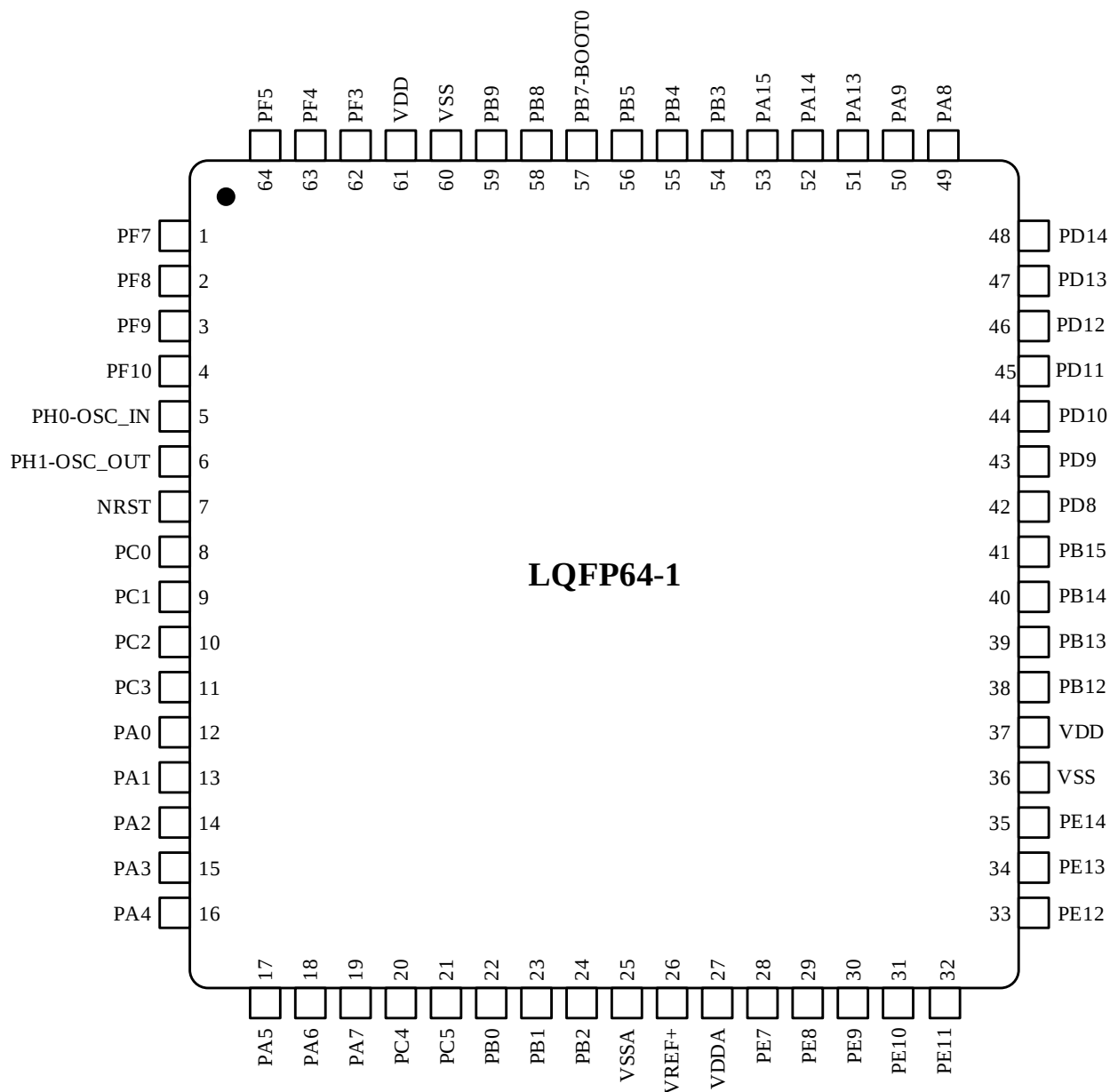
图 3-1 LQFP64-1 引脚分布
