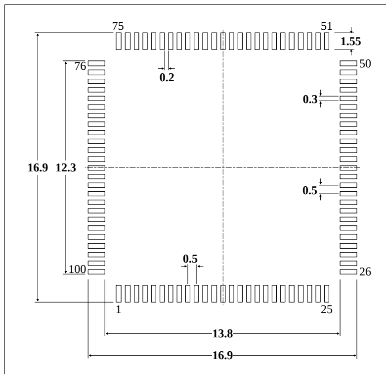
图 5-6 LQFP100 封装焊盘建议 (1)
