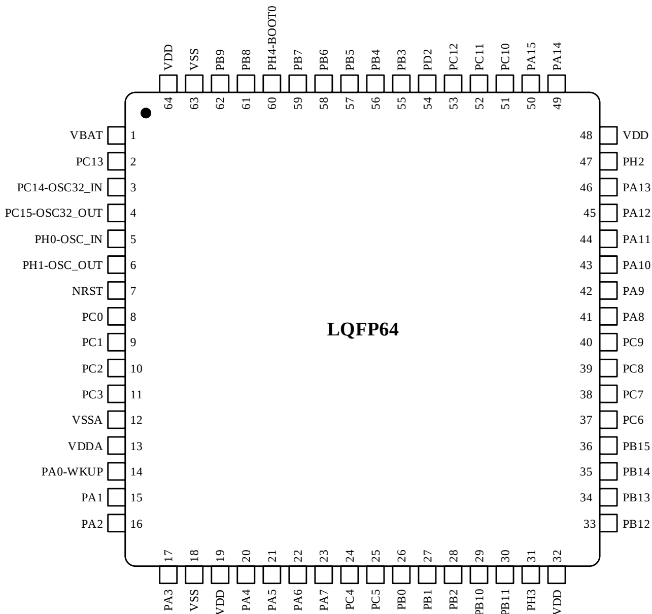
图 3-2 LQFP64 引脚分布
