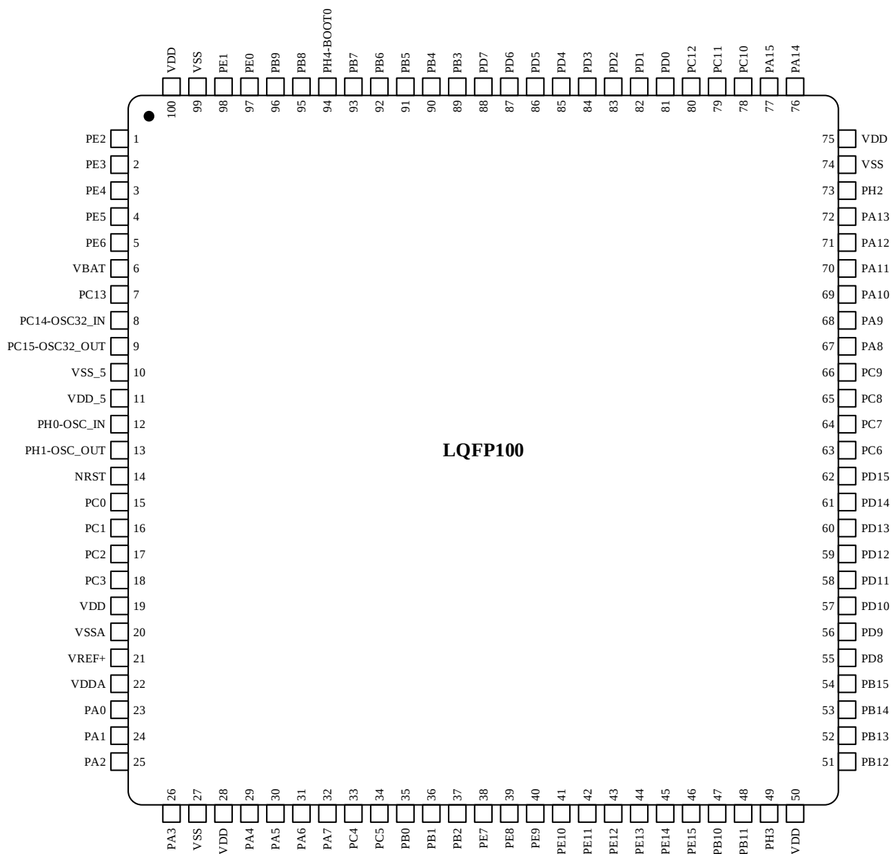
图 3-3 LQFP100 引脚分布
