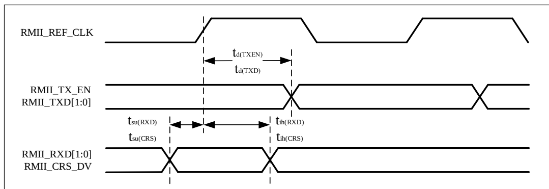
图 4-37 以太网RMII时序图
