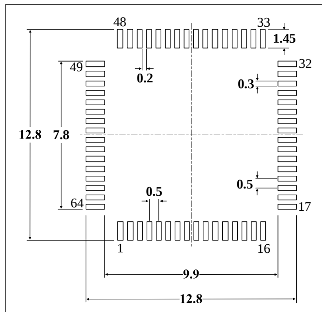
图 5-4 LQFP64 封装焊盘建议 (1)
