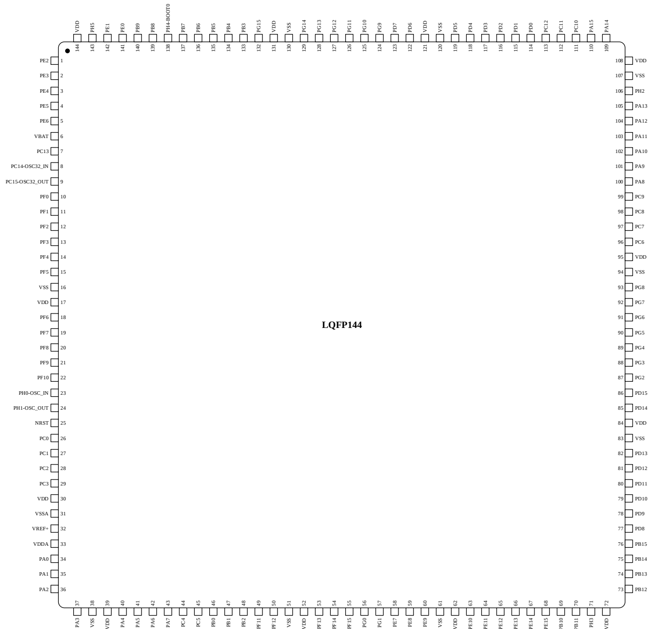
图 3-4 LQFP144 引脚分布
