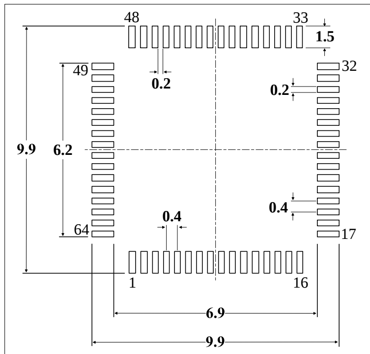
图 5-2 LQFP64-1 封装焊盘建议 (1)
