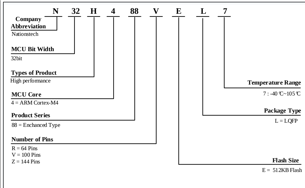
图 7-1 N32H488 系列订货代码信息图示
