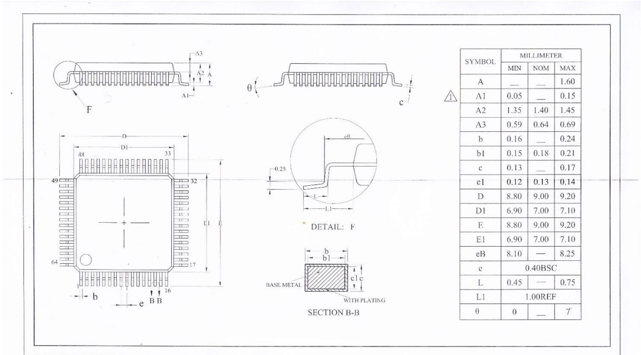
图 5-1 LQFP64-1 封装尺寸
