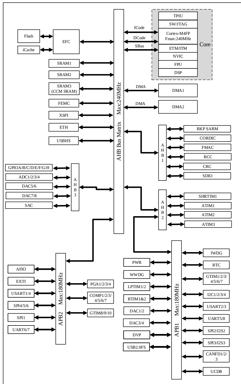
图 1-1 N32H488 系列框图
