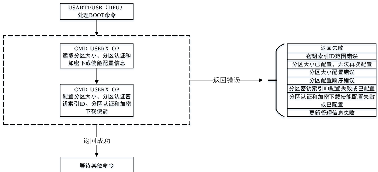
图 3-4 分区操作命令控制流程图
