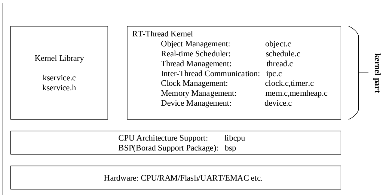
图 1-2 RT_Thread 内核及底层结构
