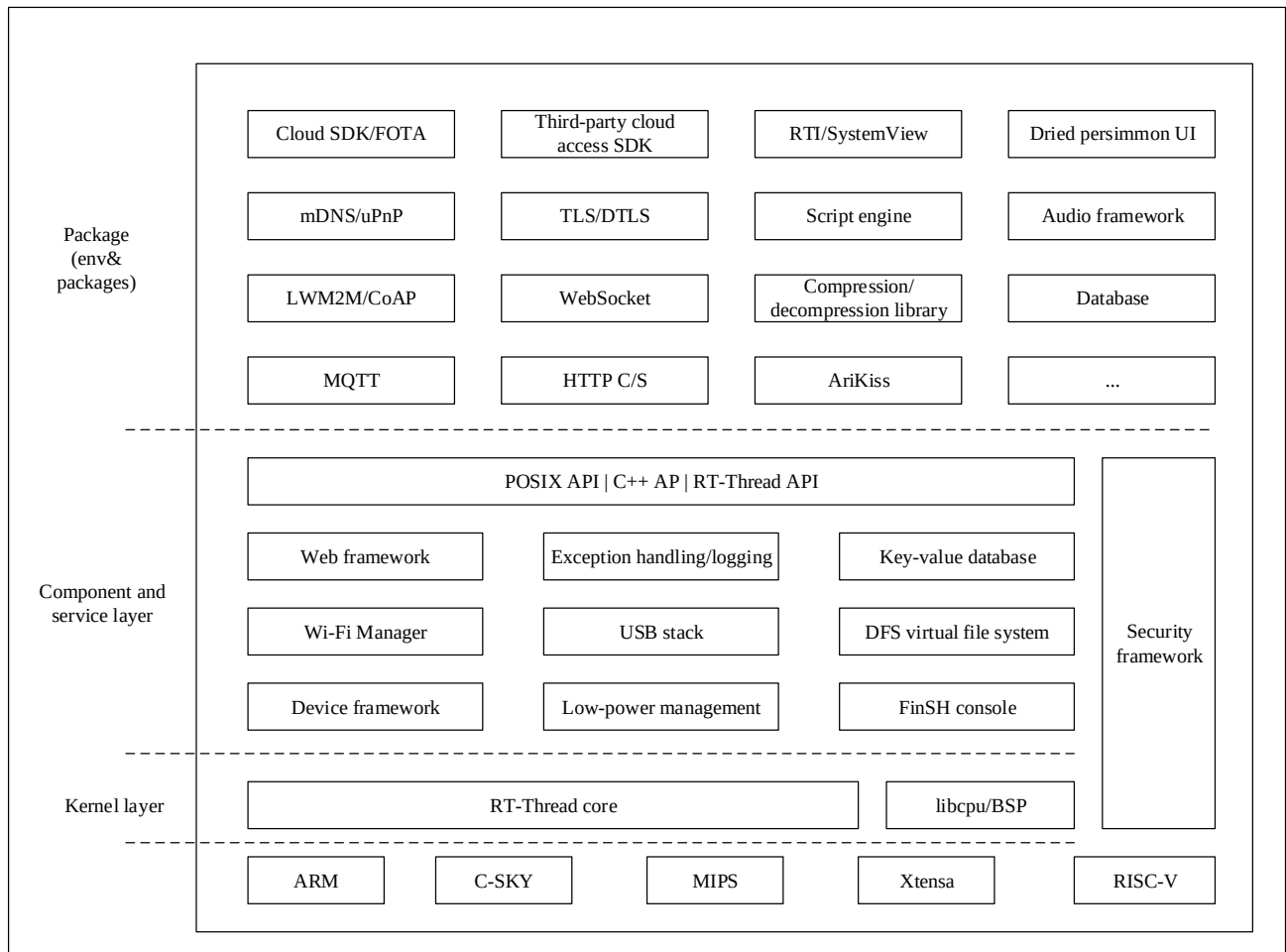
图 1-1 RT_Thread 软件框架图
