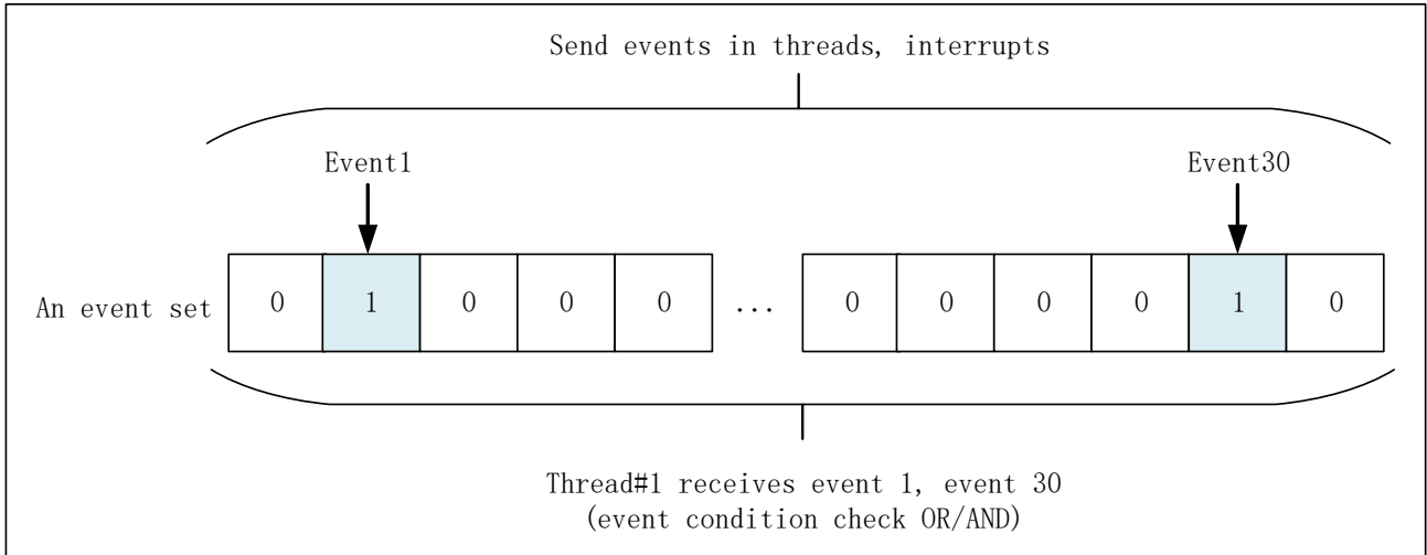
图 2-7 事件工作示意图
