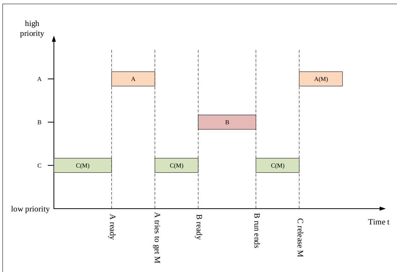
图 2-3 优先级反转 (M 为信号量)
