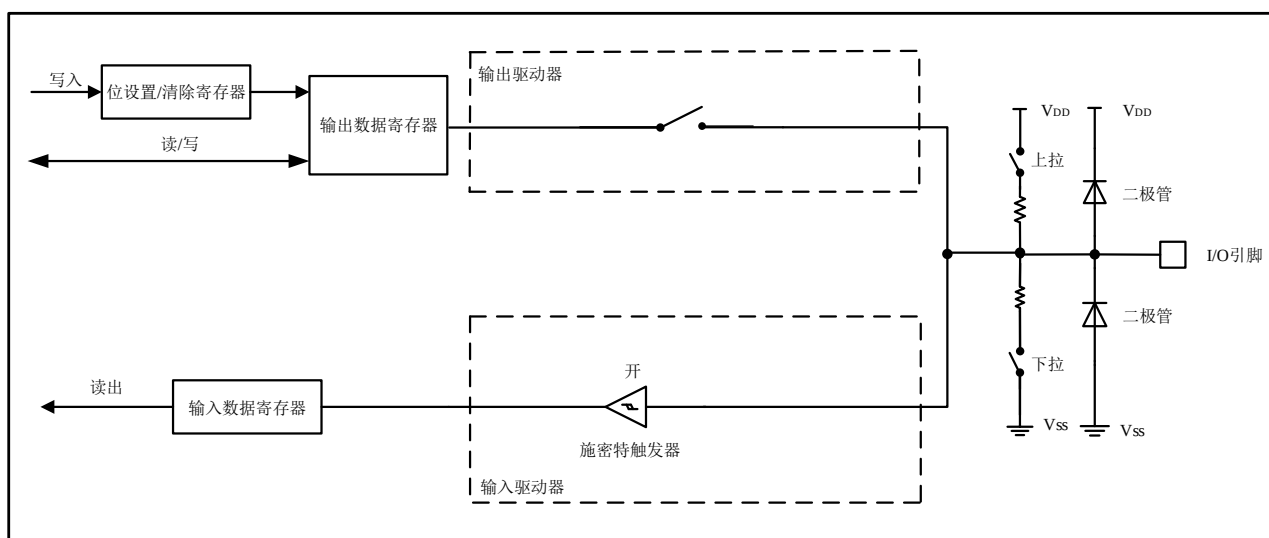
图 5-2 输入浮空/上拉/下拉配置
