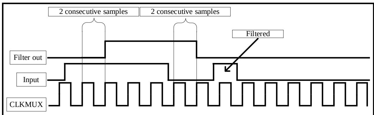
图 12-2 抖动滤波器时序图
