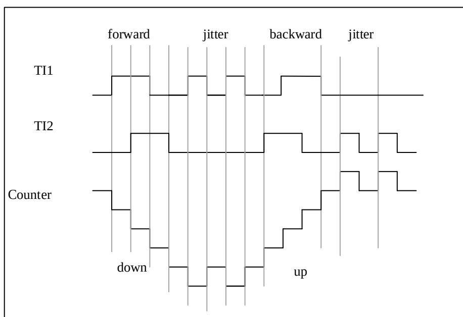
图 9-34 IC1FP1 反相的编码器接口模式实例
