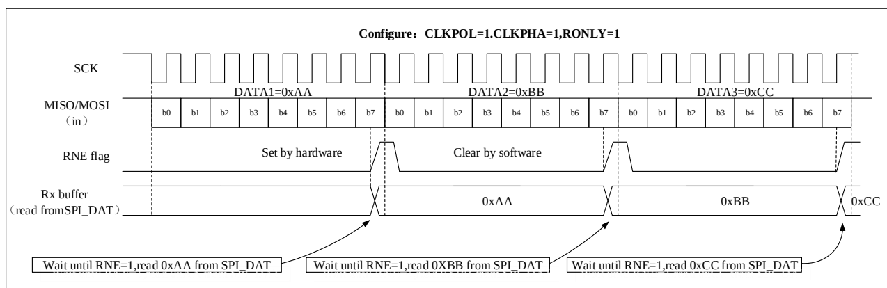
图 20-7 只接收模式（BIDIRMODE=0 并且 RONLY=1）下连续传输时，RNE 变化示意图
