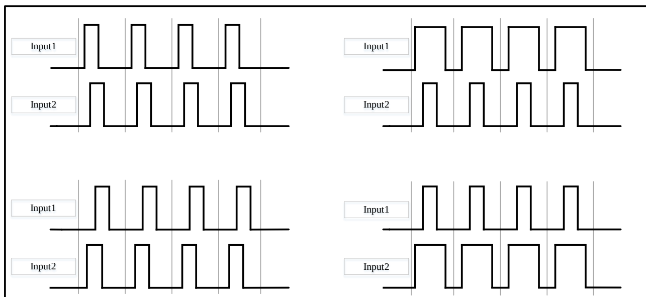
图 12-9 非正交编码器非正常工作 Input1、Input2 波形
