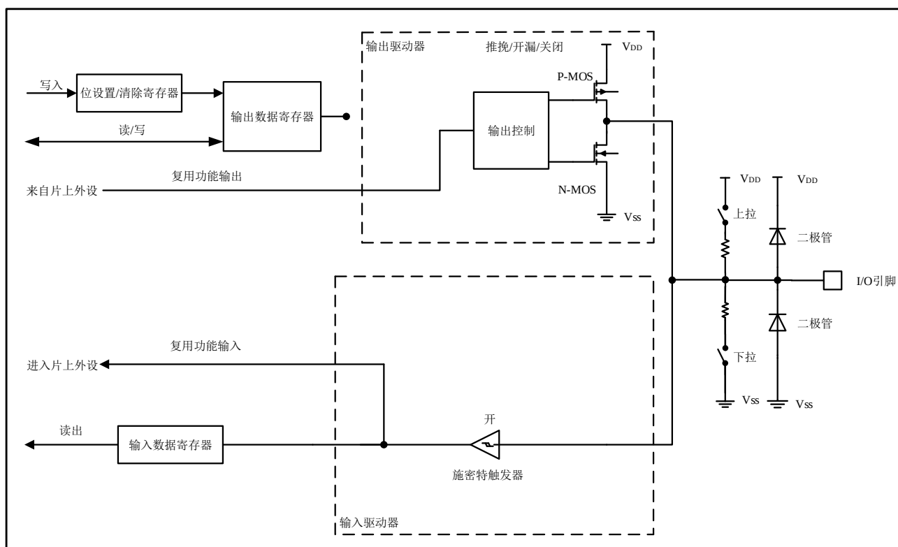
图 5-4 复用功能配置
