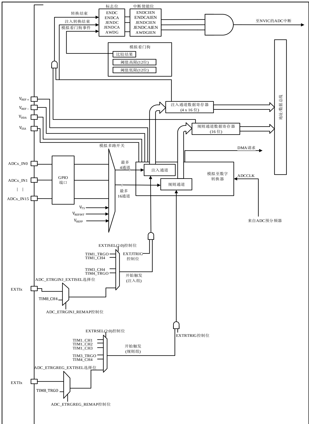
图 15-1 ADC 框图
