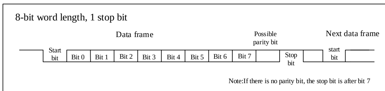
图 19-2 帧格式
