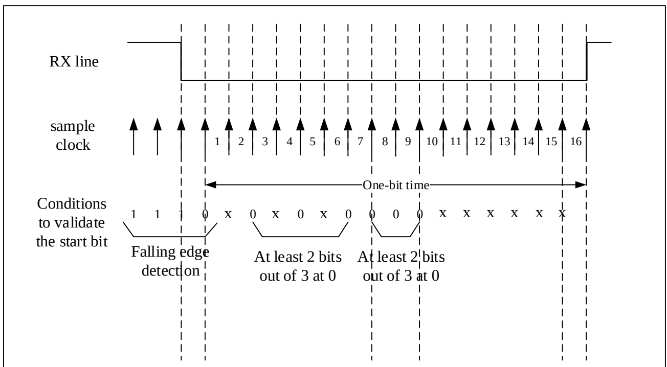
图 18-7 起始位检测
