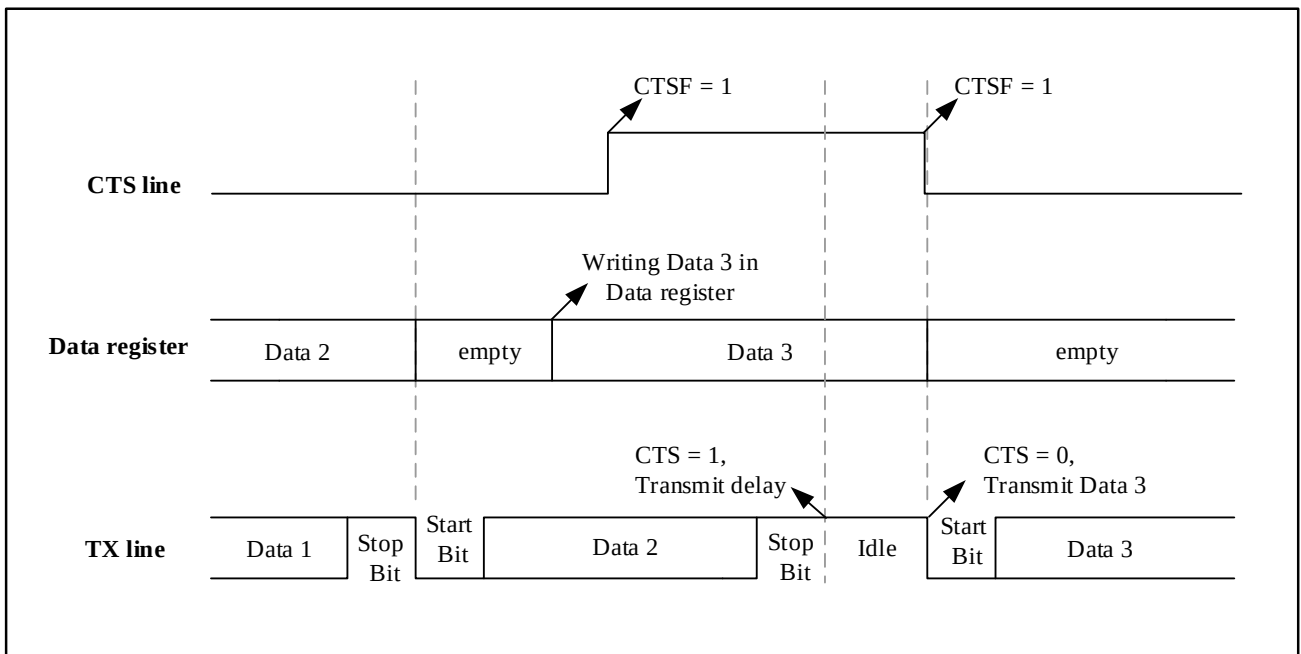
图 19-9 CTS 流控制
