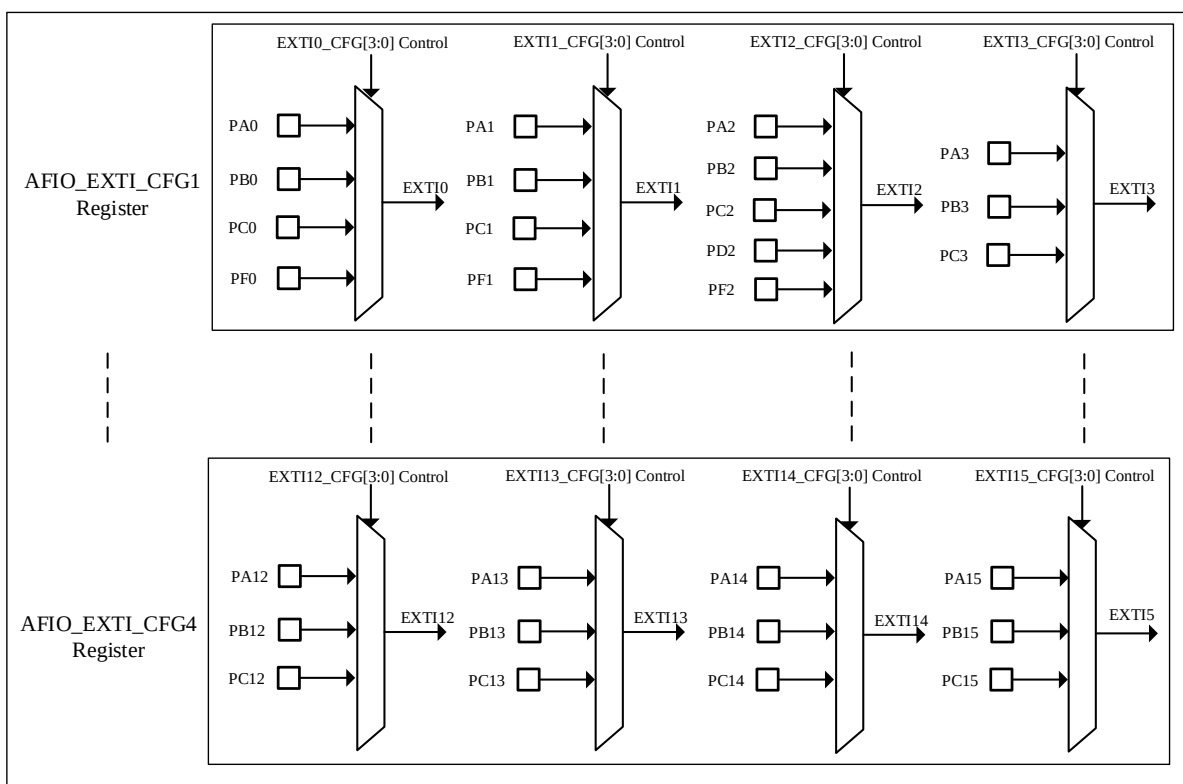
图 6-2 外部中断通用 I/O 映射
