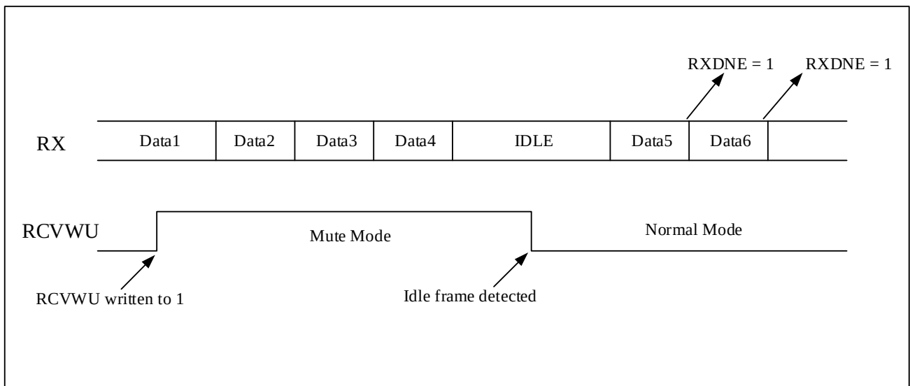
图 18-13 静默模式下的空闲总线检测
