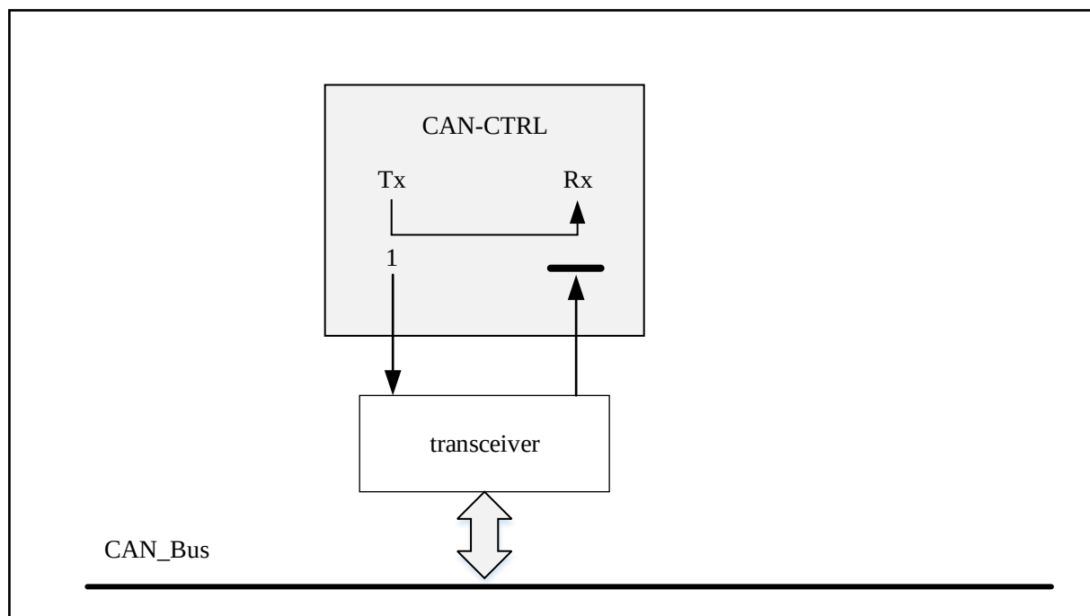
图 25-6 回环静默模式
