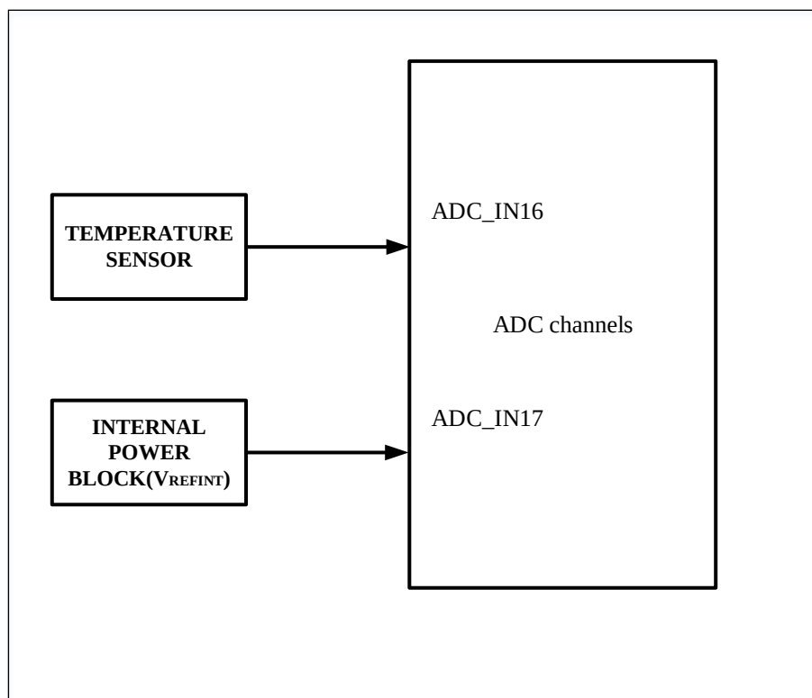
图 15-5 温度传感器和 V REFINT 通道框图
