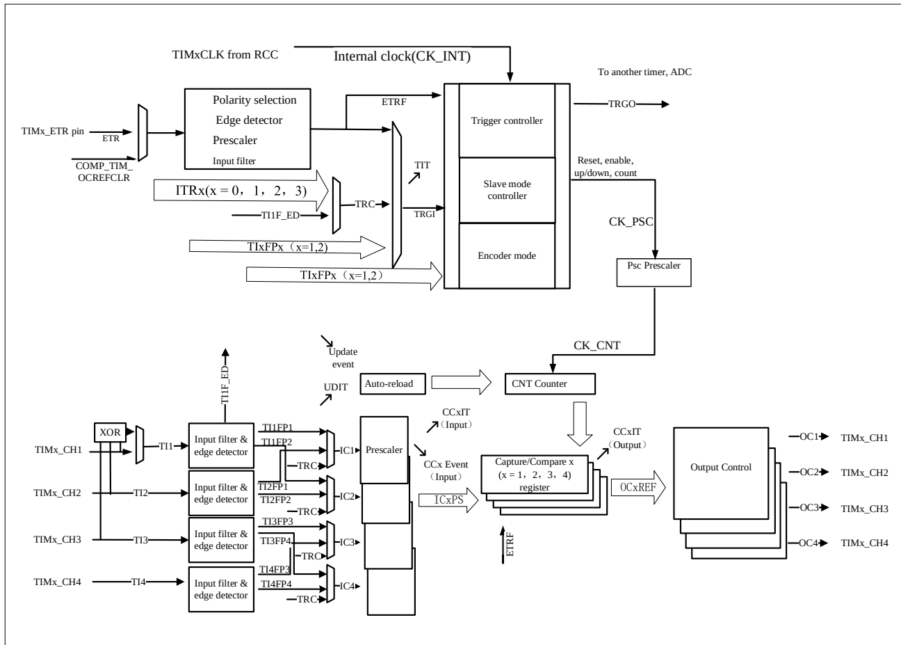
图 10-1 TIMx (x=3 and 4) 框图
