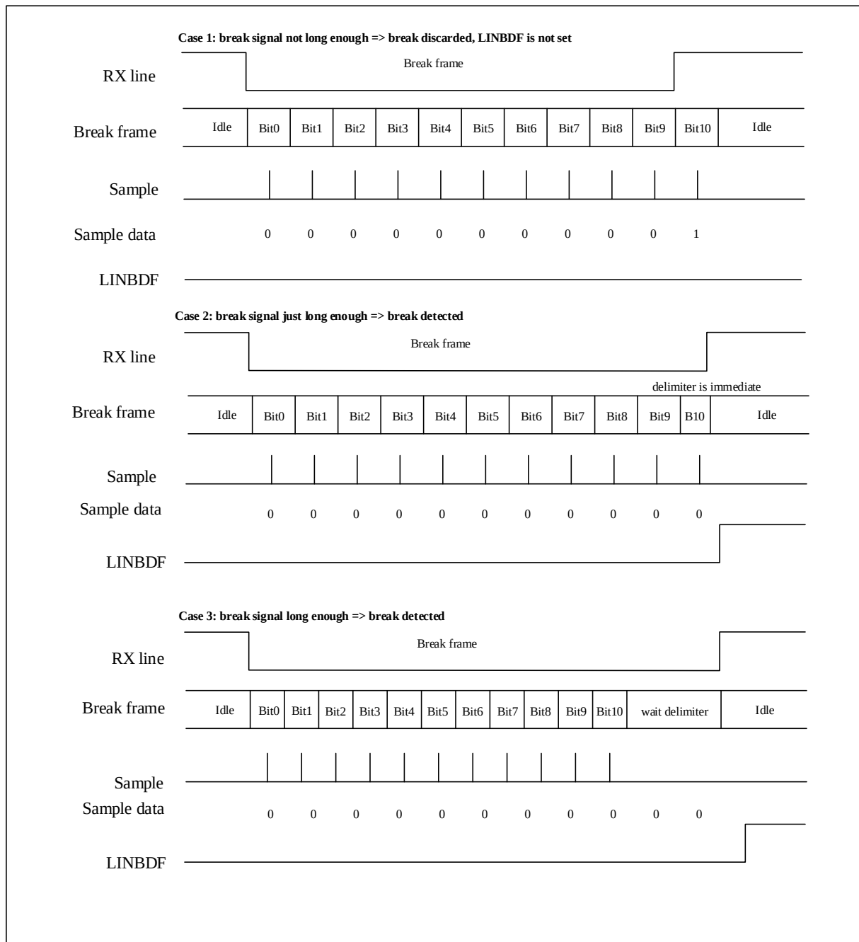
图 18-21 LIN 模式下的断开检测（11 位断开帧长度-设置了 LINBDL 位）
