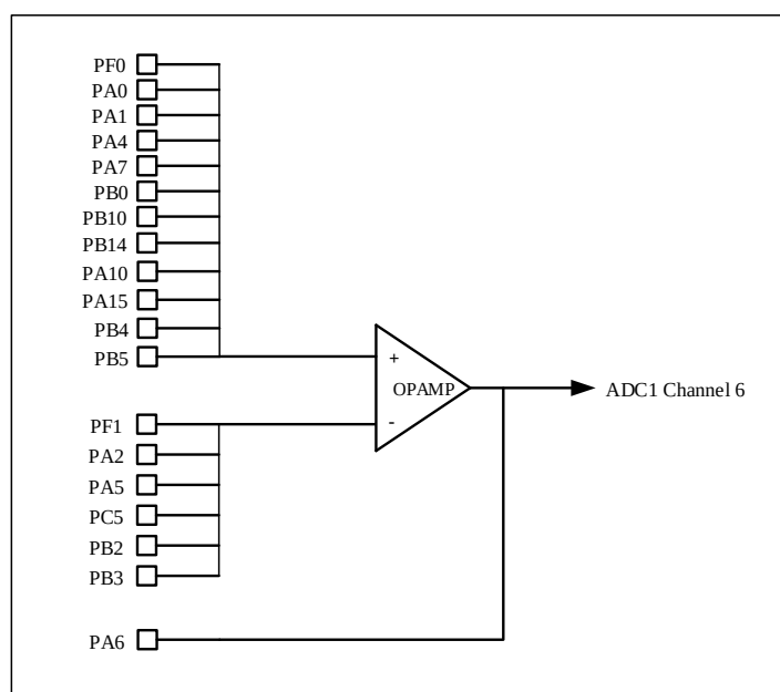
图 22-1 OPAMP 连接图框图
