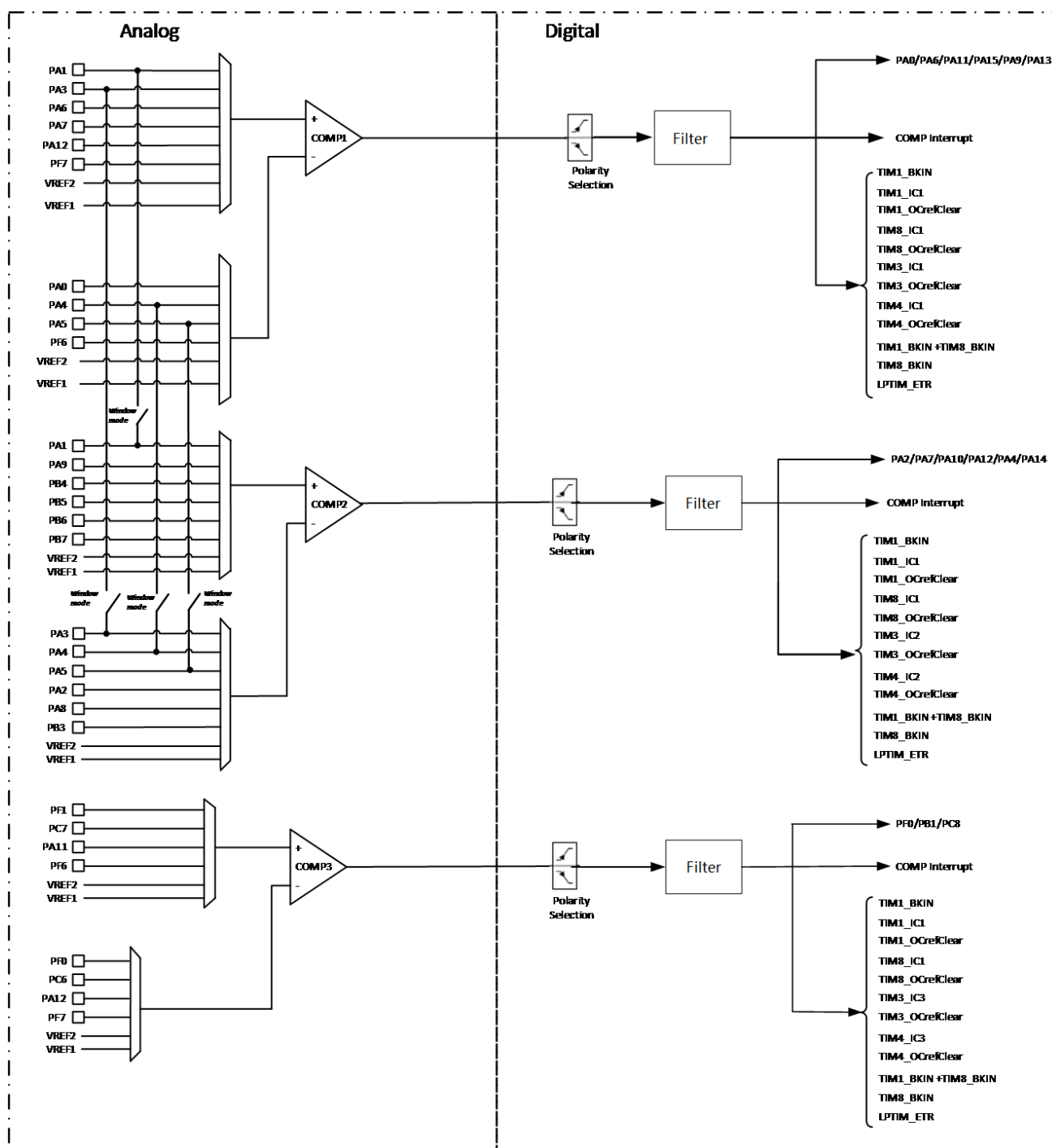
图 16-1 比较器 1/2/3 系统连接图
