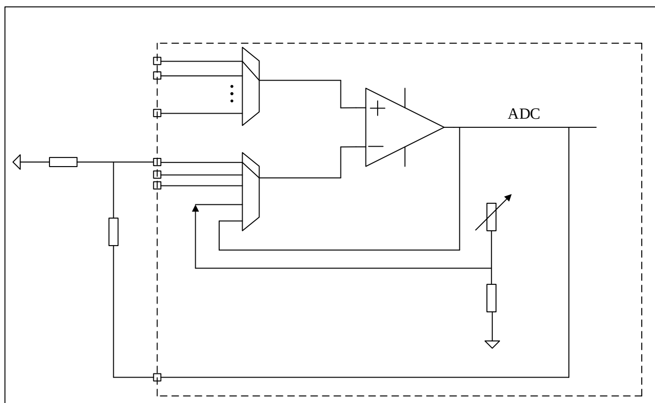
图 22-2 OPAMP 外部放大模式
