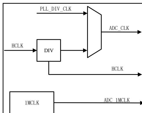
图 15-2 ADC 时钟
