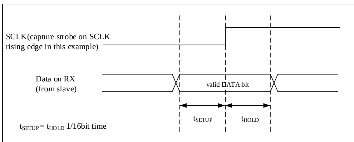
图 18-18 RX 数据采样/保持时间
