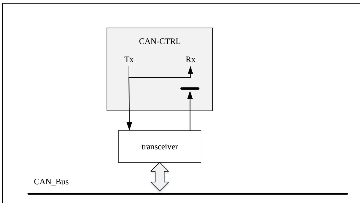
图 25-4 回环模式
