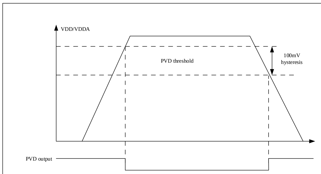
图 3-3 PVD 阈值图
