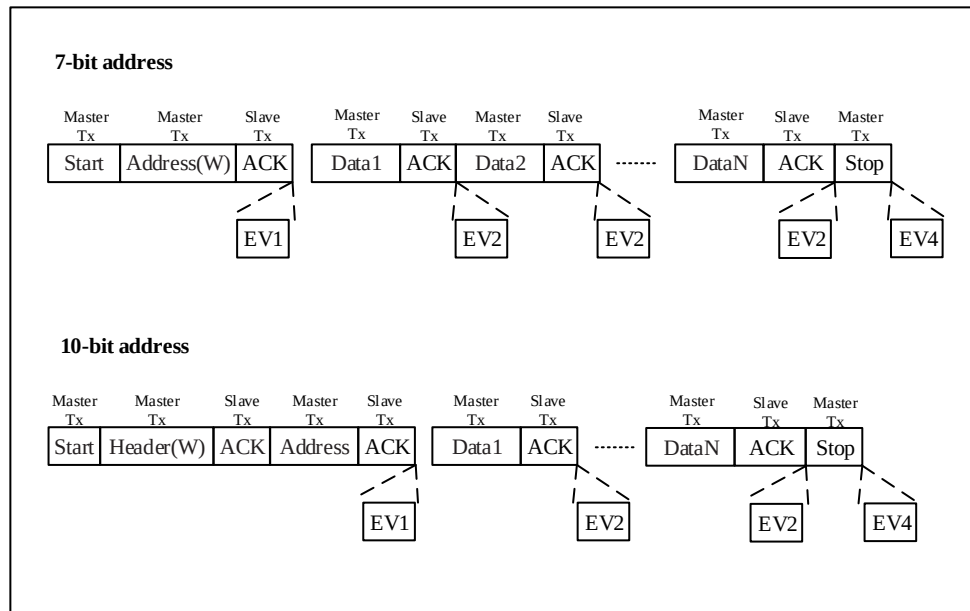
图 17-4 从机接收器传送序列
