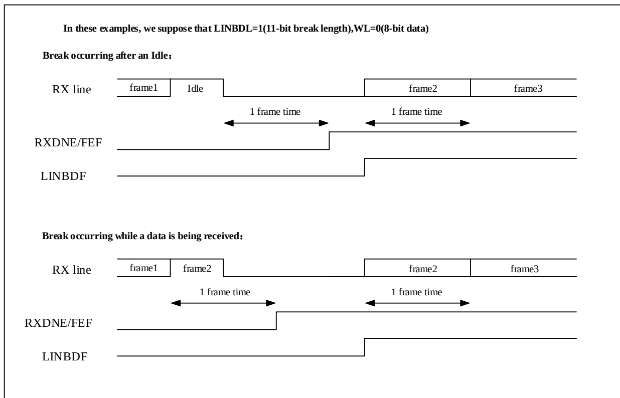
图 18-22 LIN 模式下的断开检测与帧错误的检测
