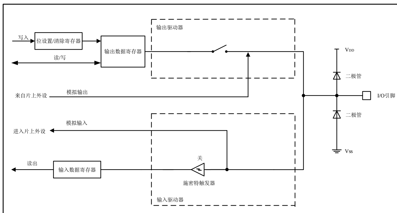
图 5-5 高阻抗的模拟输入配置
