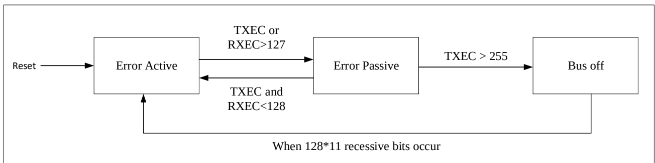
图 25-14 CAN 错误状态框图
