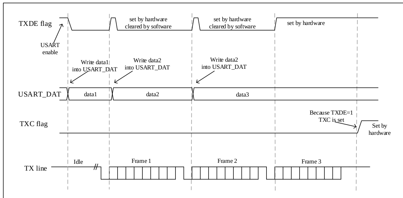
图 18-6 发送时 TXC/TXDE 的变化情况
