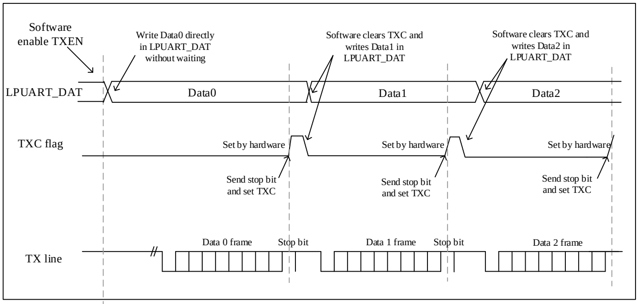
图 19-3 发送时 TXC 的变化情况
