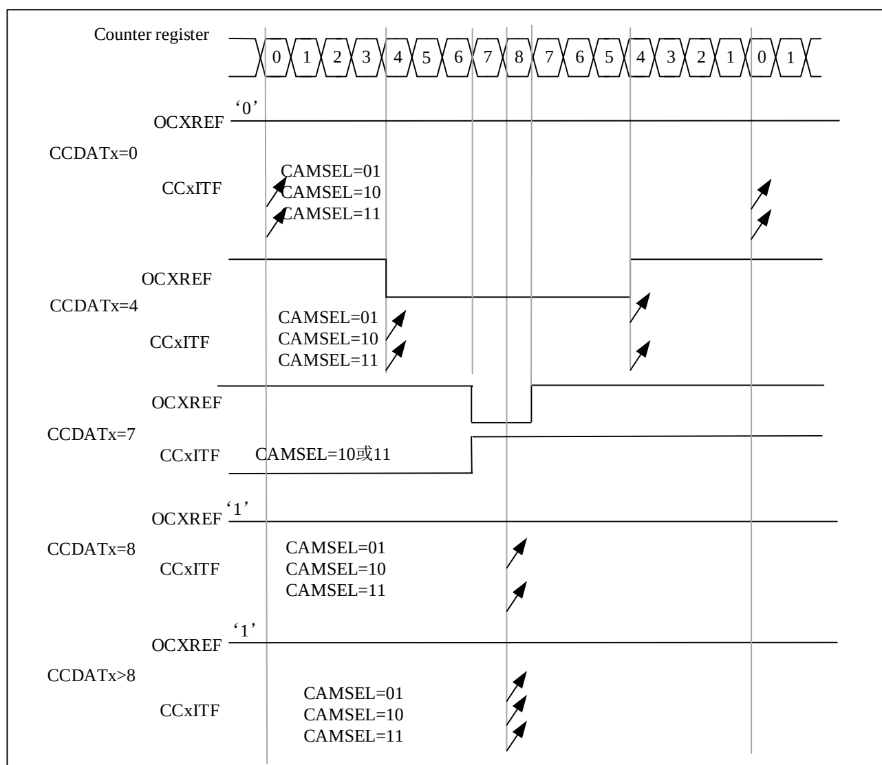
图 10-18 中央对齐的 PWM 波形 (AR=8)
