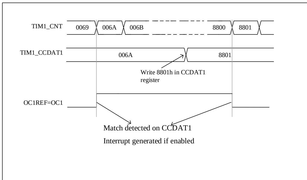
图 10-17 输出比较模式，开启 OC1
