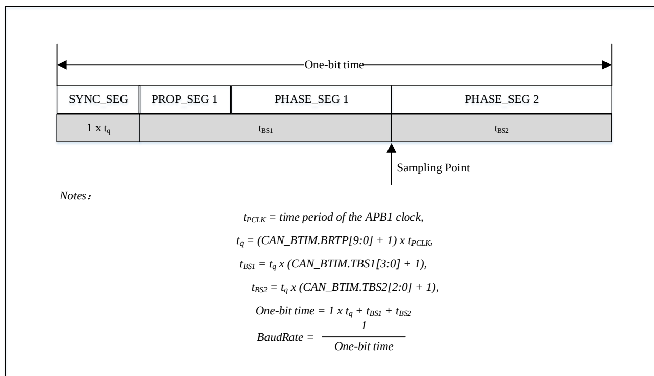
图 25-11 位时序
