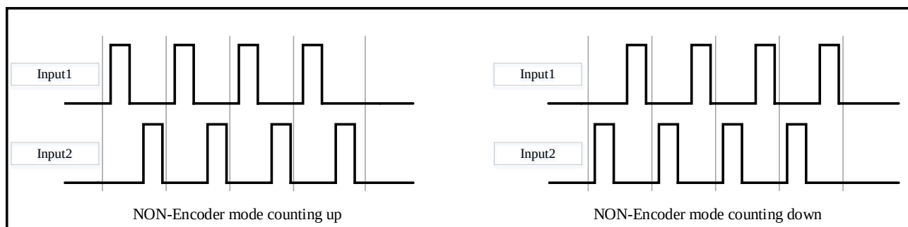
图 12-8 非正交编码器正常工作 Input1、Input2 波形
