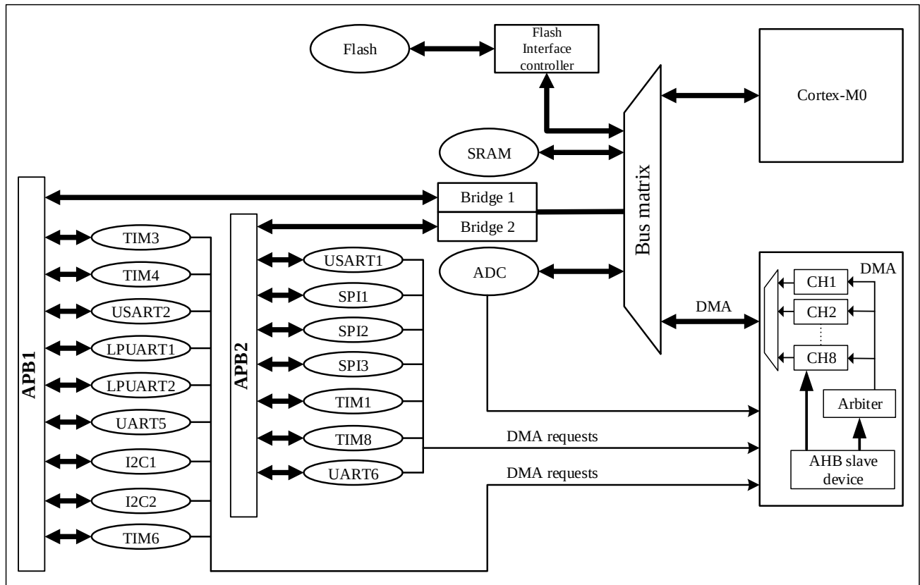
图 7-1 DMA 框图
