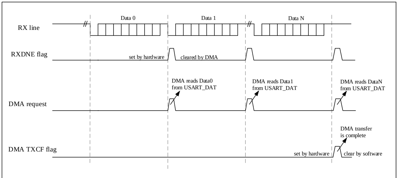
图 18-9 DMA 接收
