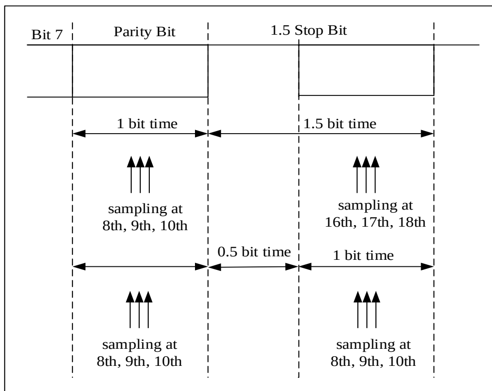
图 18-24 使用 1.5 停止位检测奇偶检验错误
