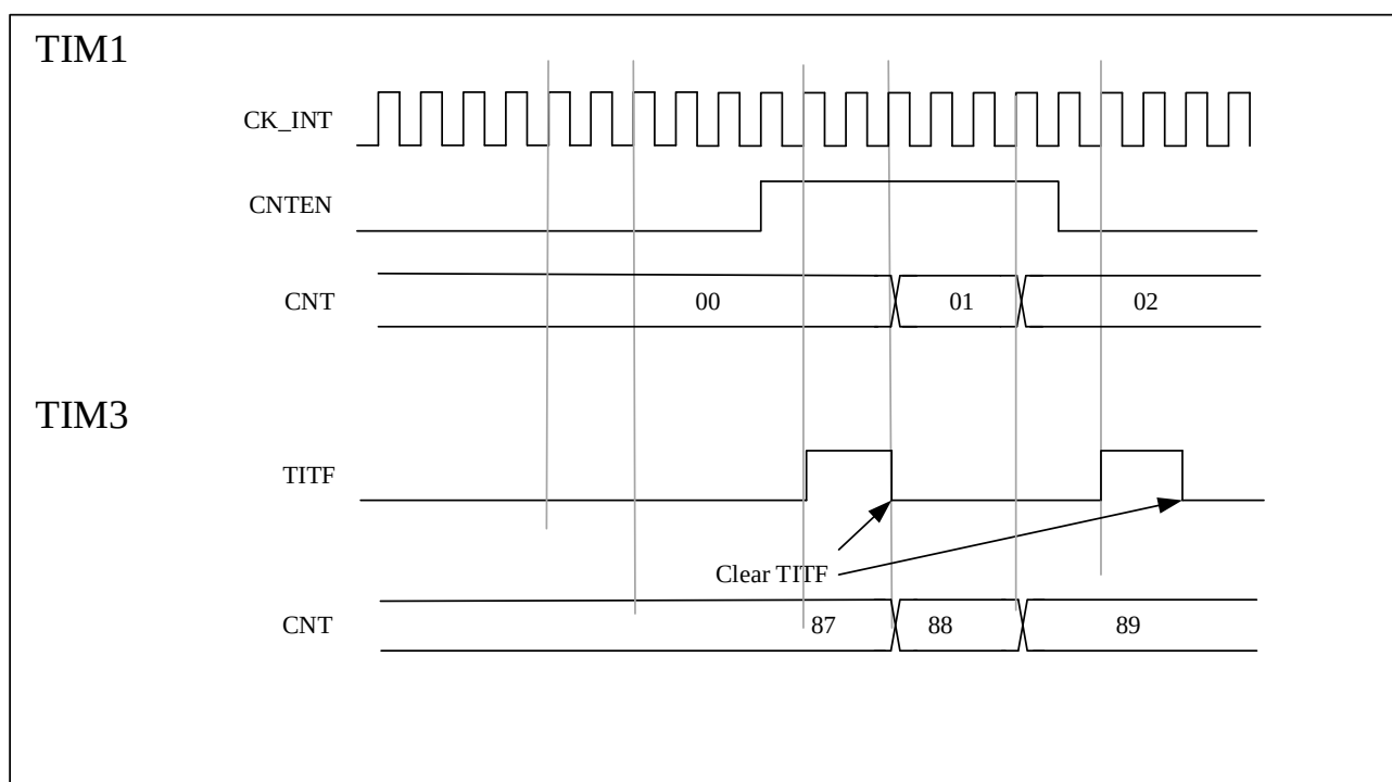
图 10-24 定时器 3 由定时器 1 的使能门控
