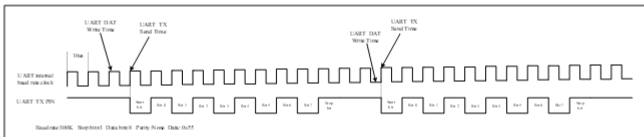
图 18-5 发送时差
