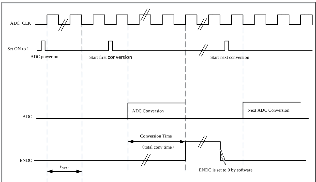
图 15-3 时序图
