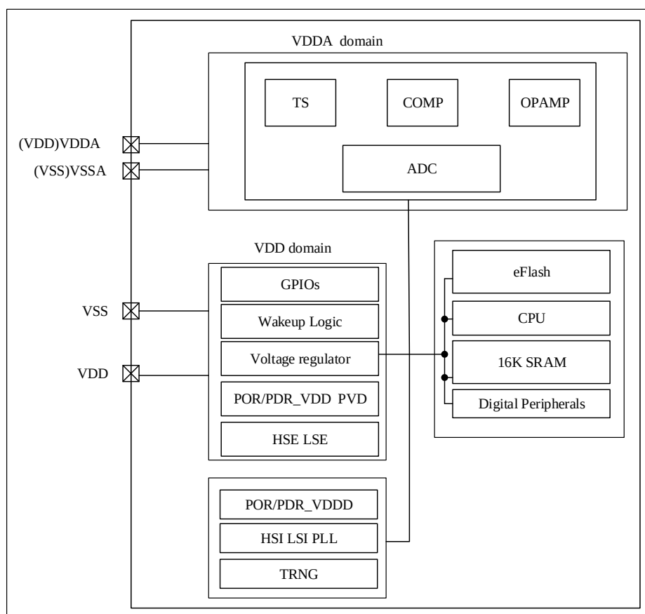
图 3-1 电源框图
