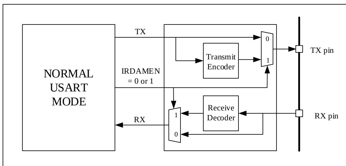
图 18-20 IrDA 数据调制(3/16)-正常模式
