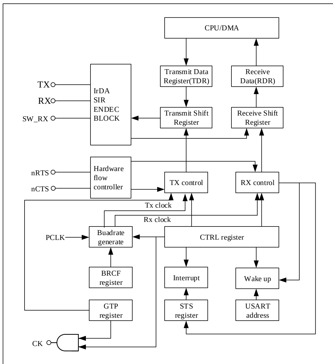
图 18-1 USART 框图
