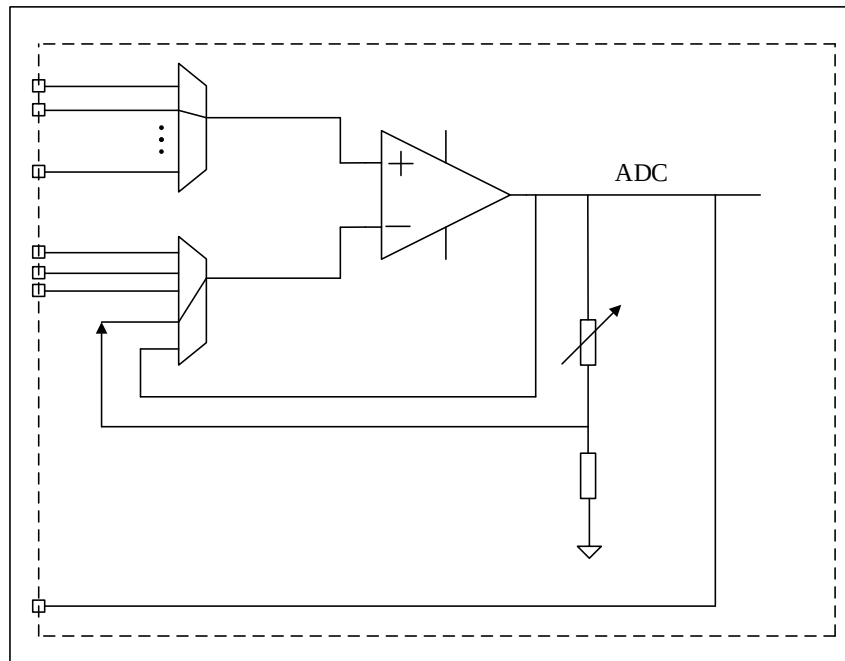
图 22-4 内部增益模式
