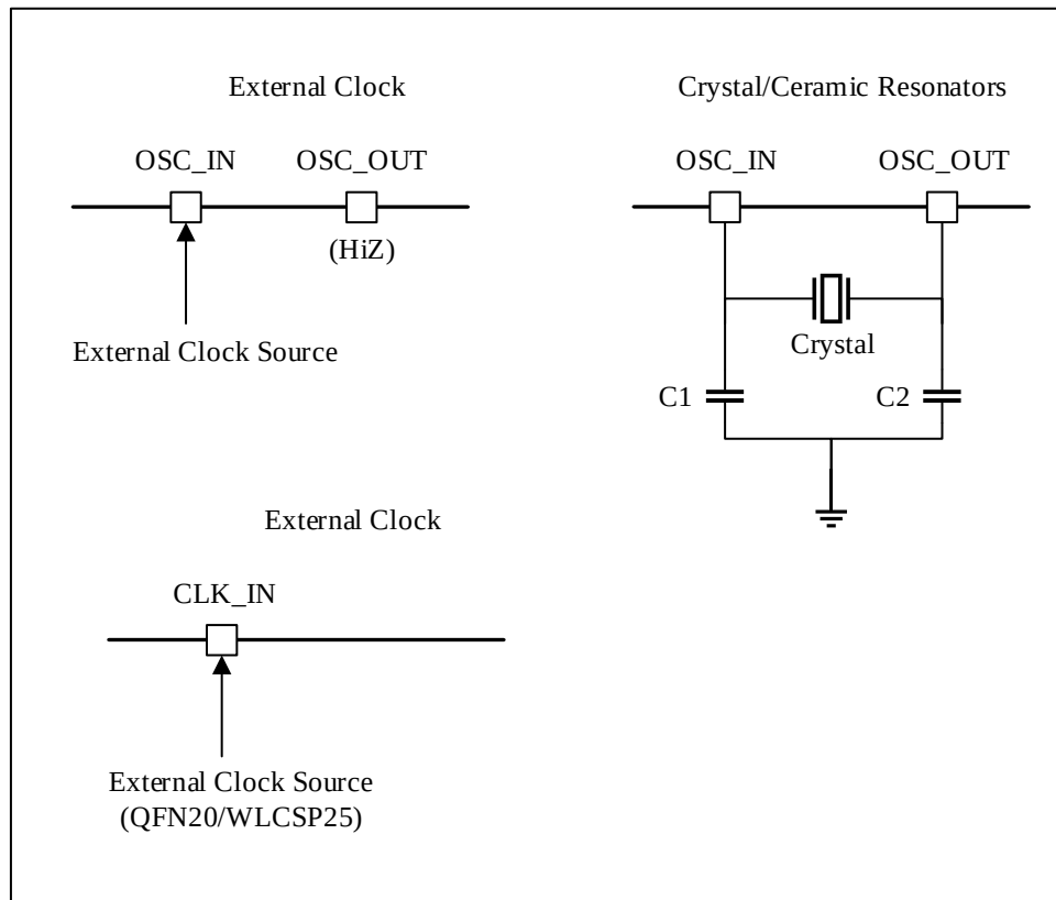
图 4-3 HSE 时钟源
