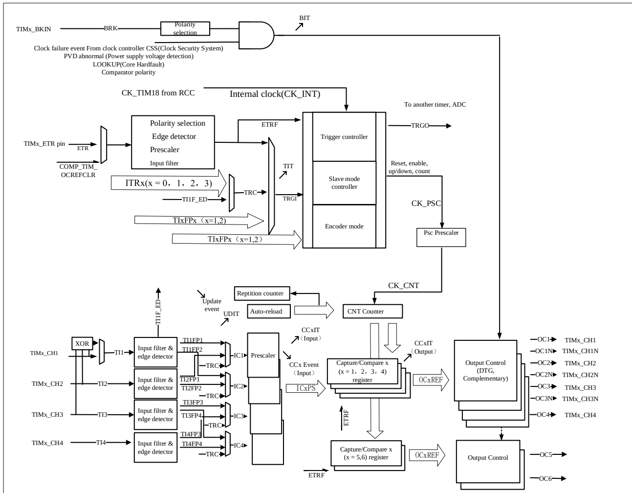
图 9-1 TIMx(x=1/8)框图
