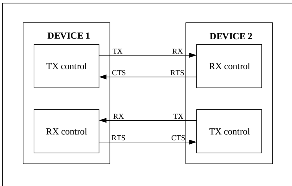
图 18-10 两个 USART 间的硬件流控制
