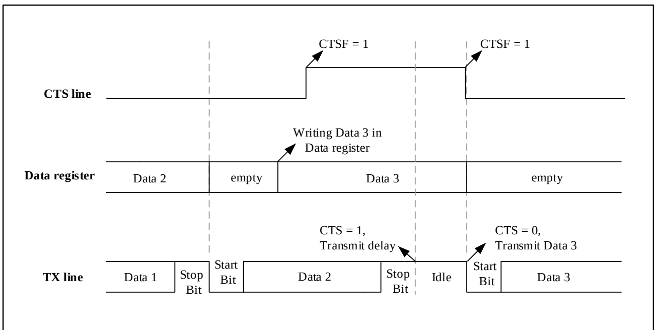
图 18-12 CTS 流控制
