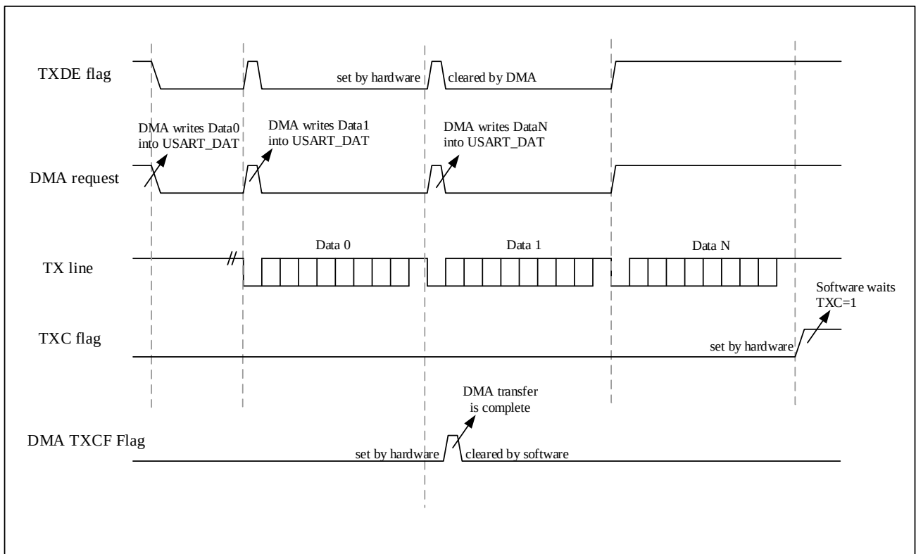
图 18-8 DMA 发送
