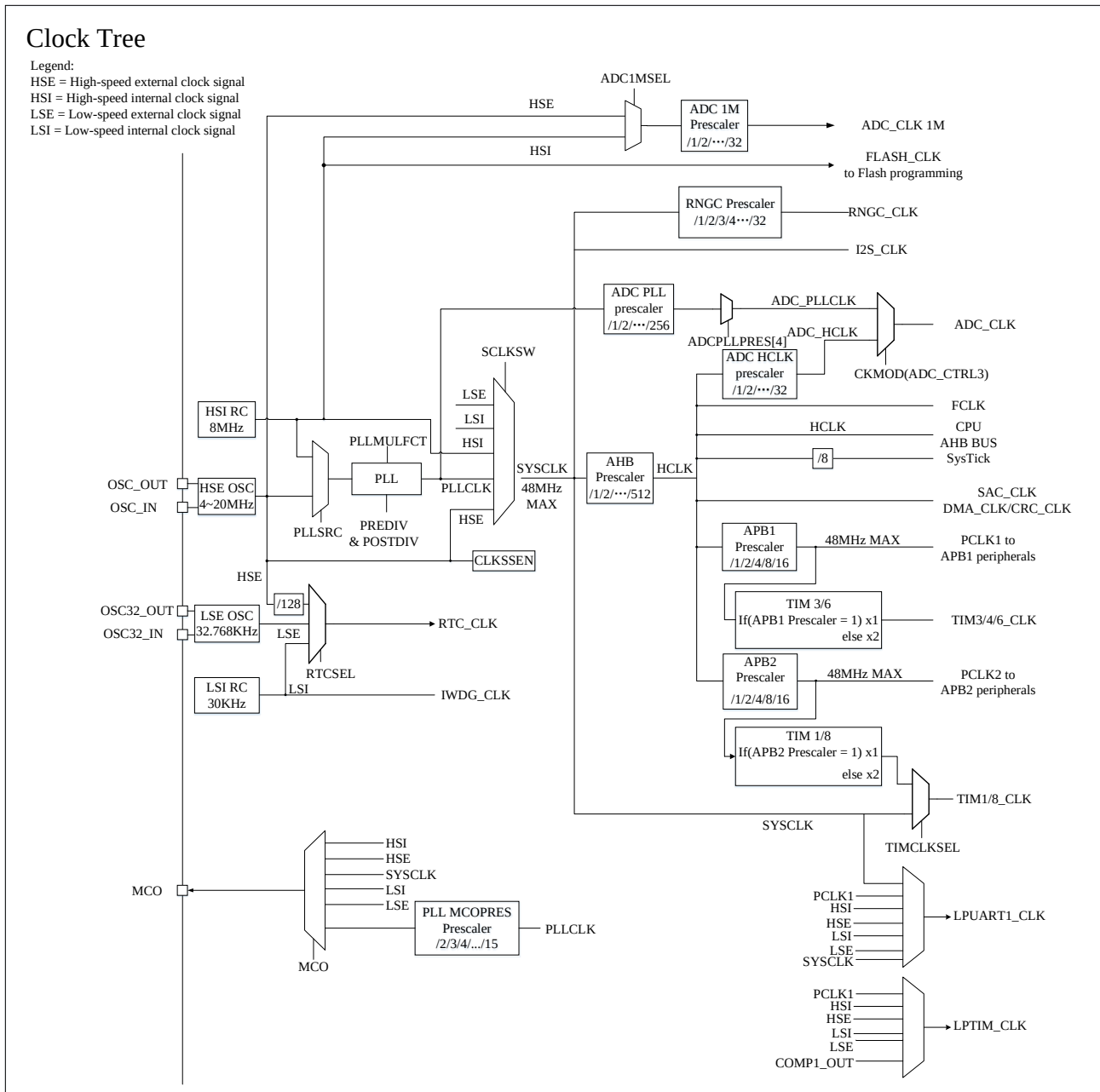
图 4-2 时钟树
