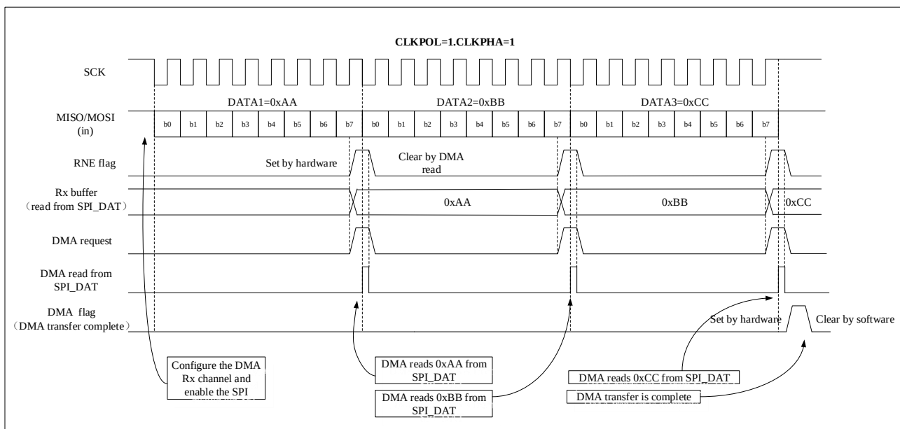
图 20-12 使用 DMA 接收
