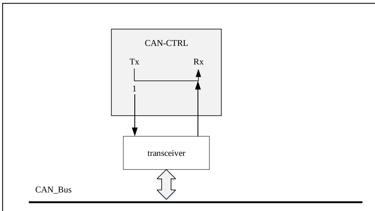
图 25-5 静默模式
