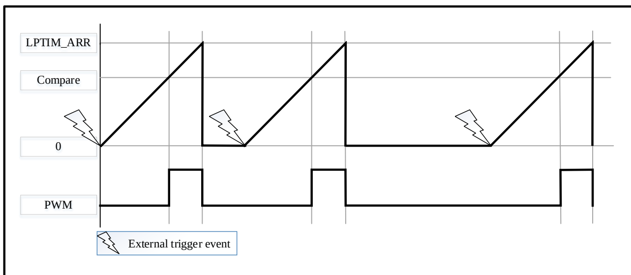
图 12-4 LPTIM 输出波形，单触发计数模式配置
