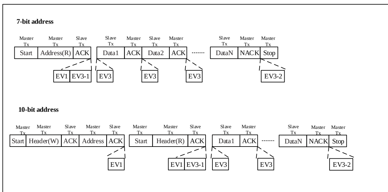
图 17-3 从发送器传送序列
