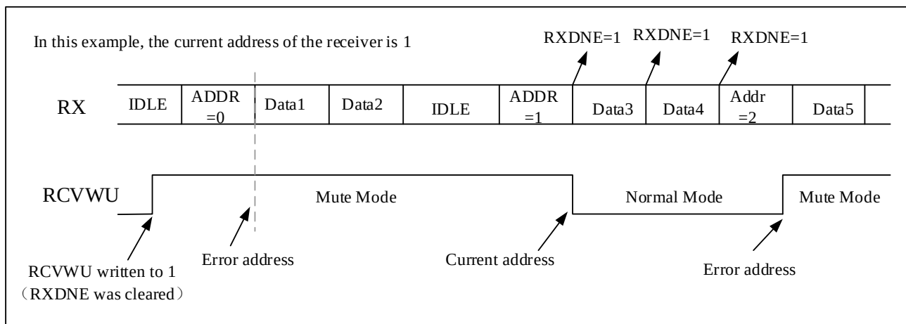
图 18-14 静默模式下的地址标识检测
