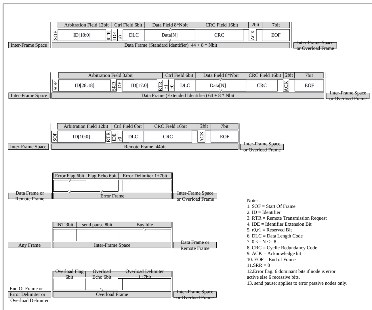
图 25-12 各类帧格式
