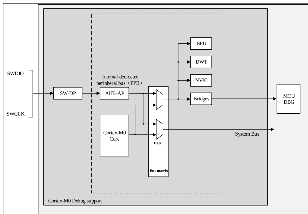
图 27-1 N32G032 级别和 Cortex®-M0 级别的调试框图
