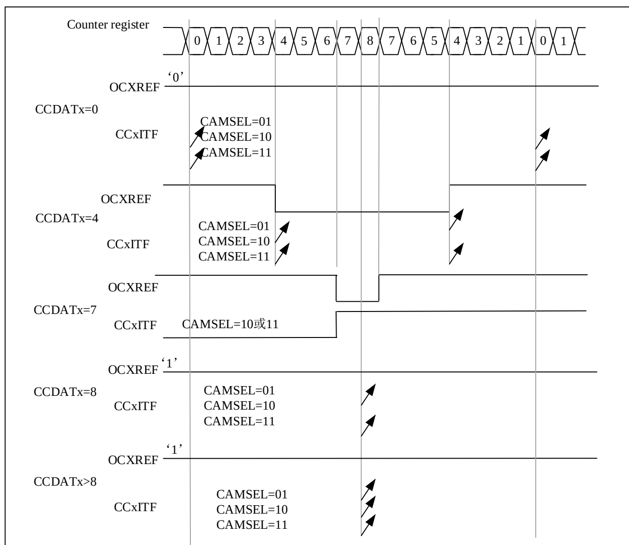
图 9-22 中央对齐的 PWM 波形 (AR=8)
