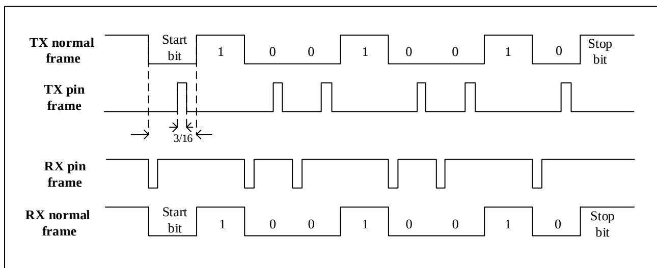
图 18-20 IrDA 数据调制(3/16)-正常模式
