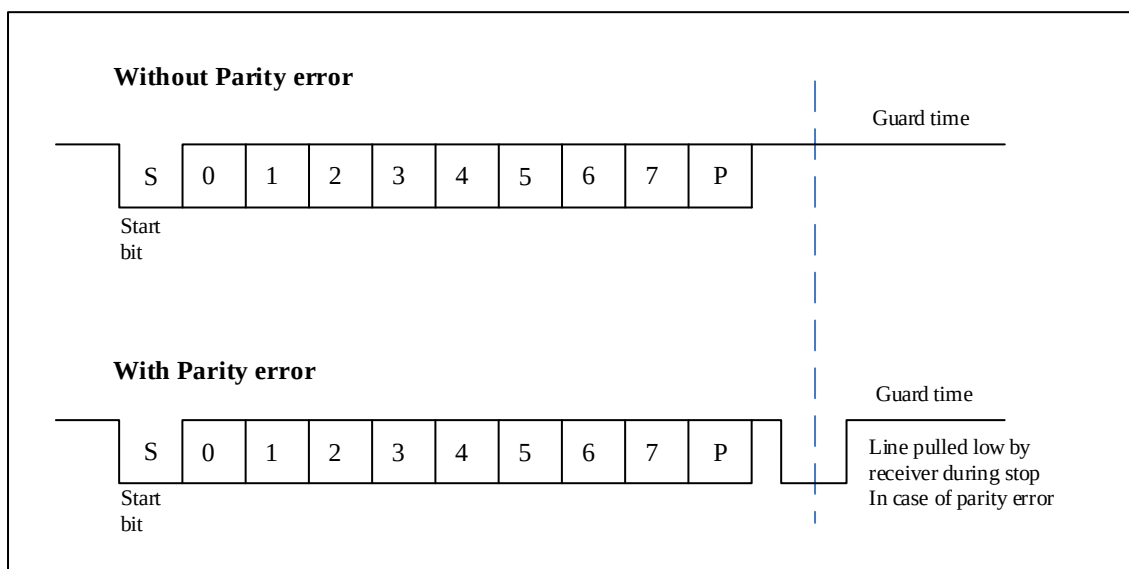
图 18-23 ISO7816-3 异步协议
