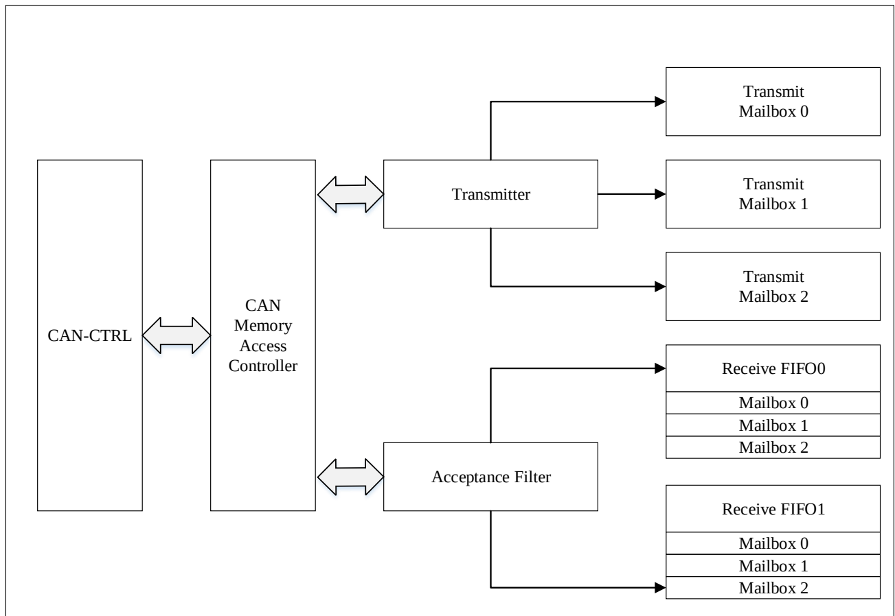
图 25-3 单 CAN 框图
