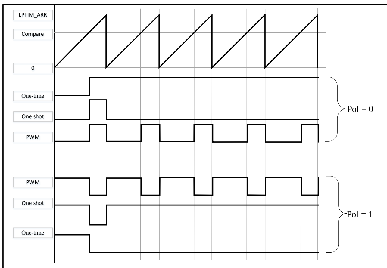
图 12-6 波形发生器
