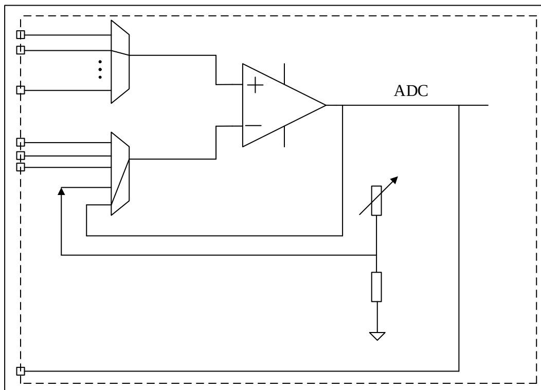
图 22-3 OPAMP 跟随模式
