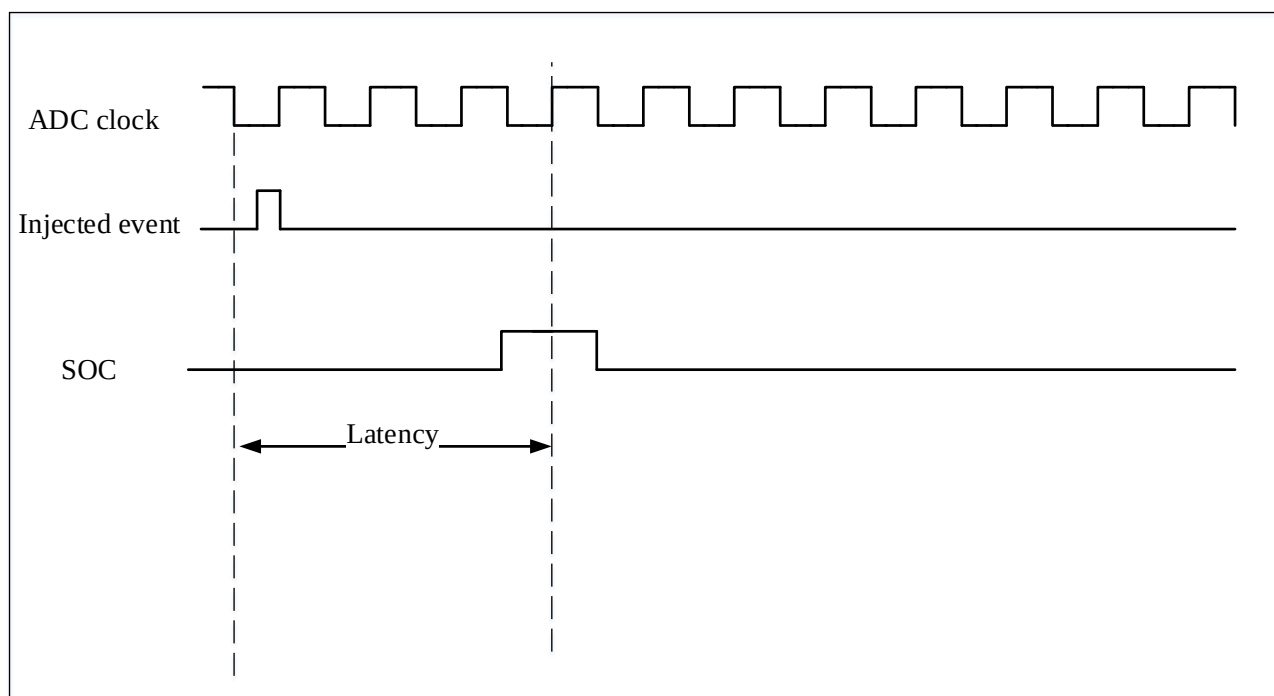
图 15-4 注入转换延时
