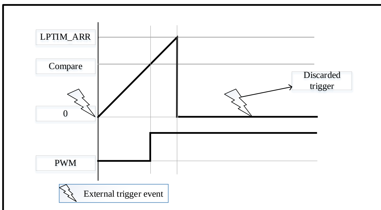
图 12-5 LPTIM 输出波形，一次模式
