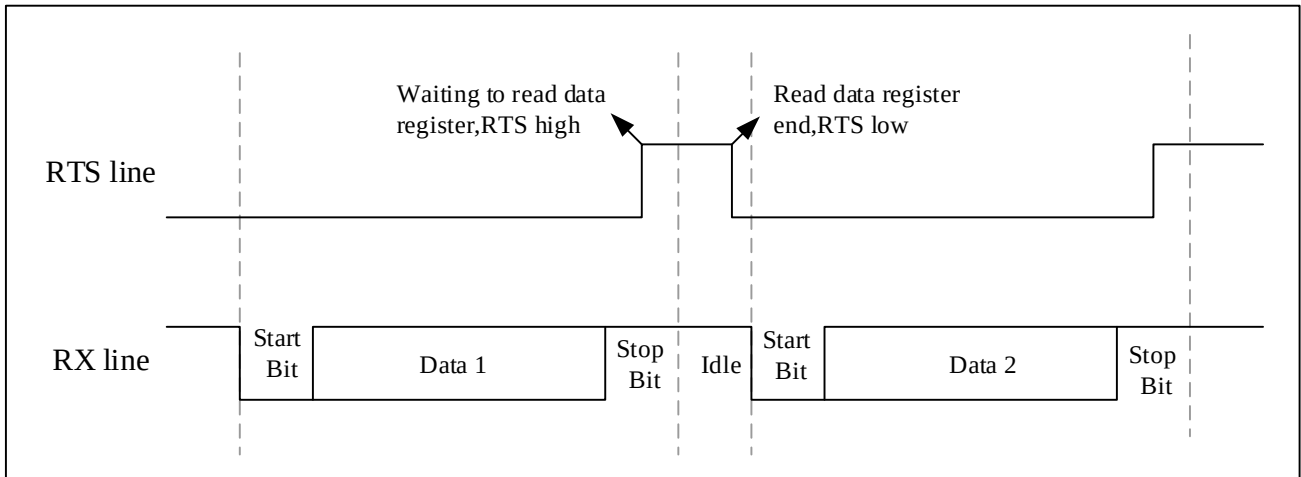
图 18-11 RTS 流控制
