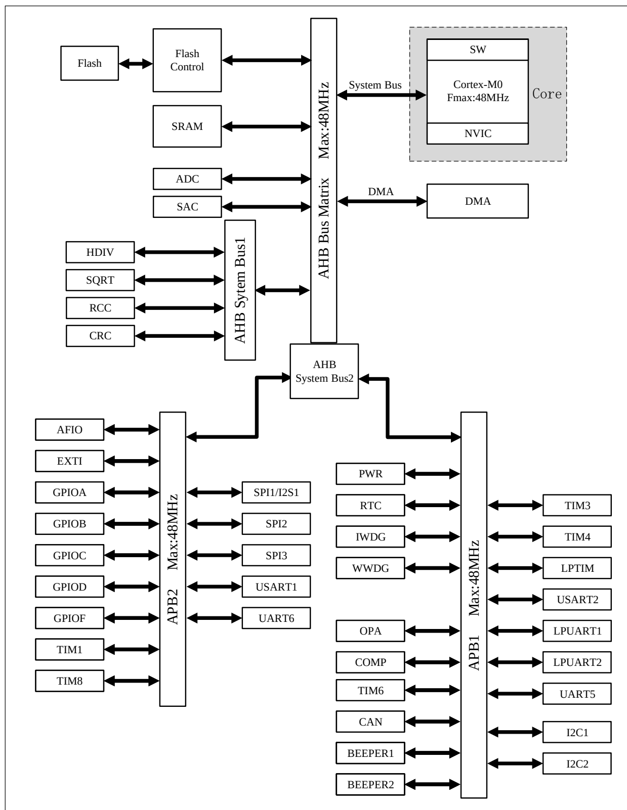
图 2-1 总线架构图
