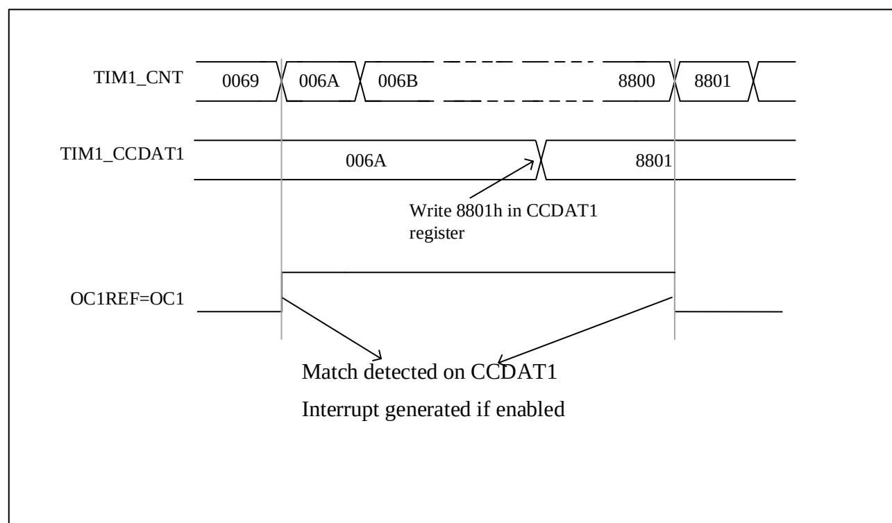
图 9-21 输出比较模式，开启 OC1
