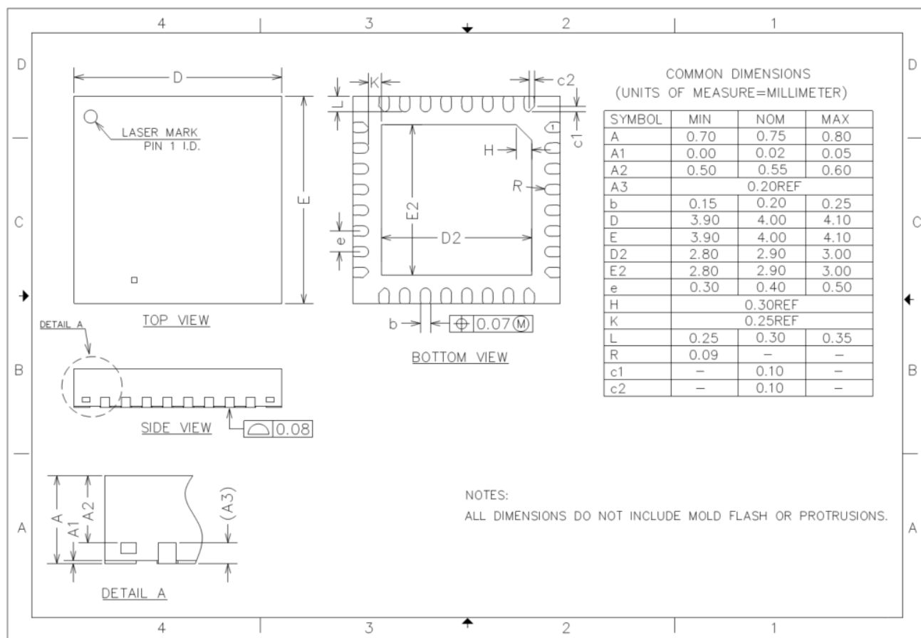
图 5-9 QFN32(4mmx4mm)封装尺寸
