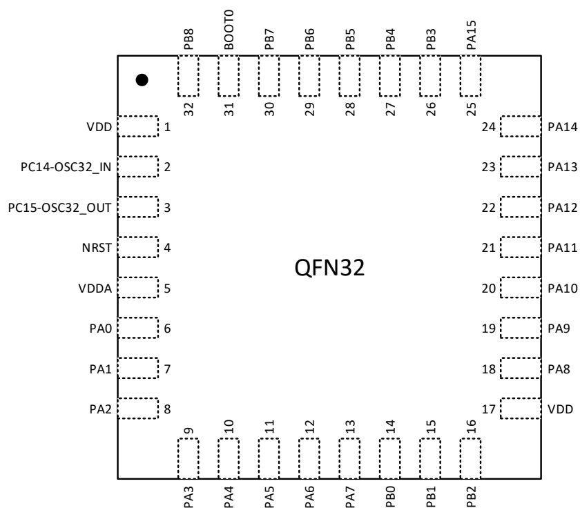
图 3-5 N32G030系列QFN32(4mmx4mm)引脚分布
