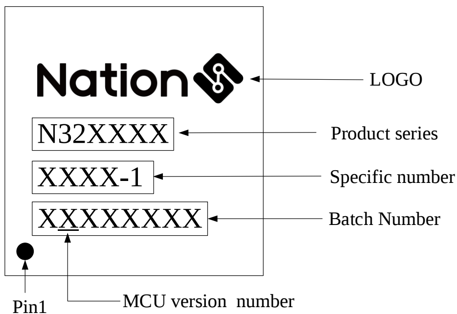
图 5-16 QFN32(4mm x 4mm)丝印说明图
