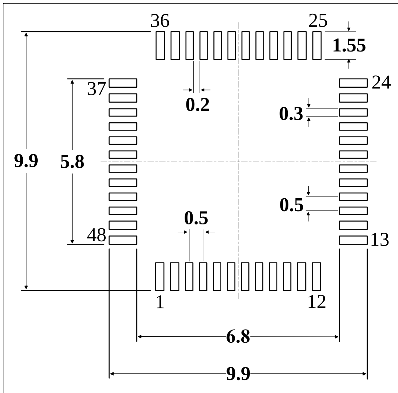
图 5-4 TQFP48封装焊盘建议 (1)
