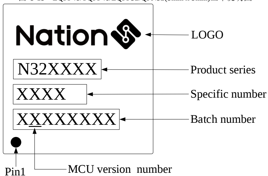
图 5-16 QFN32(4mm x 4mm)丝印说明图
