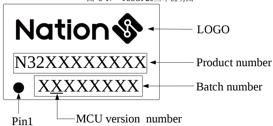
图 5-17 TSSOP20丝印说明图
