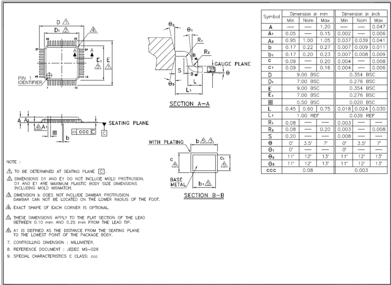
图 5-3 TQFP48封装尺寸
