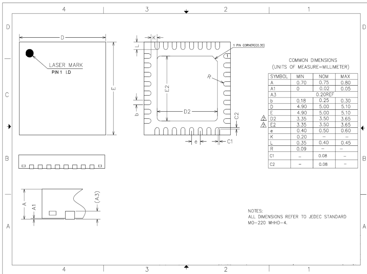
图 5-7 QFN32(5mmx5mm)封装尺寸
