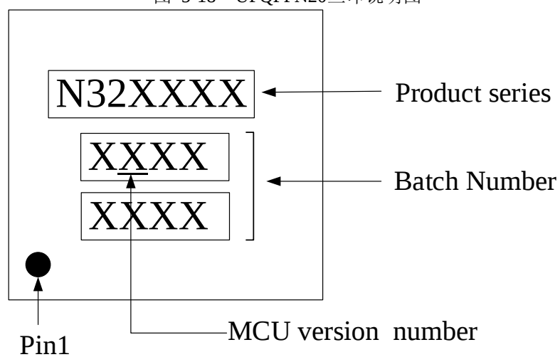
图 5-18 UFQFPN20丝印说明图
