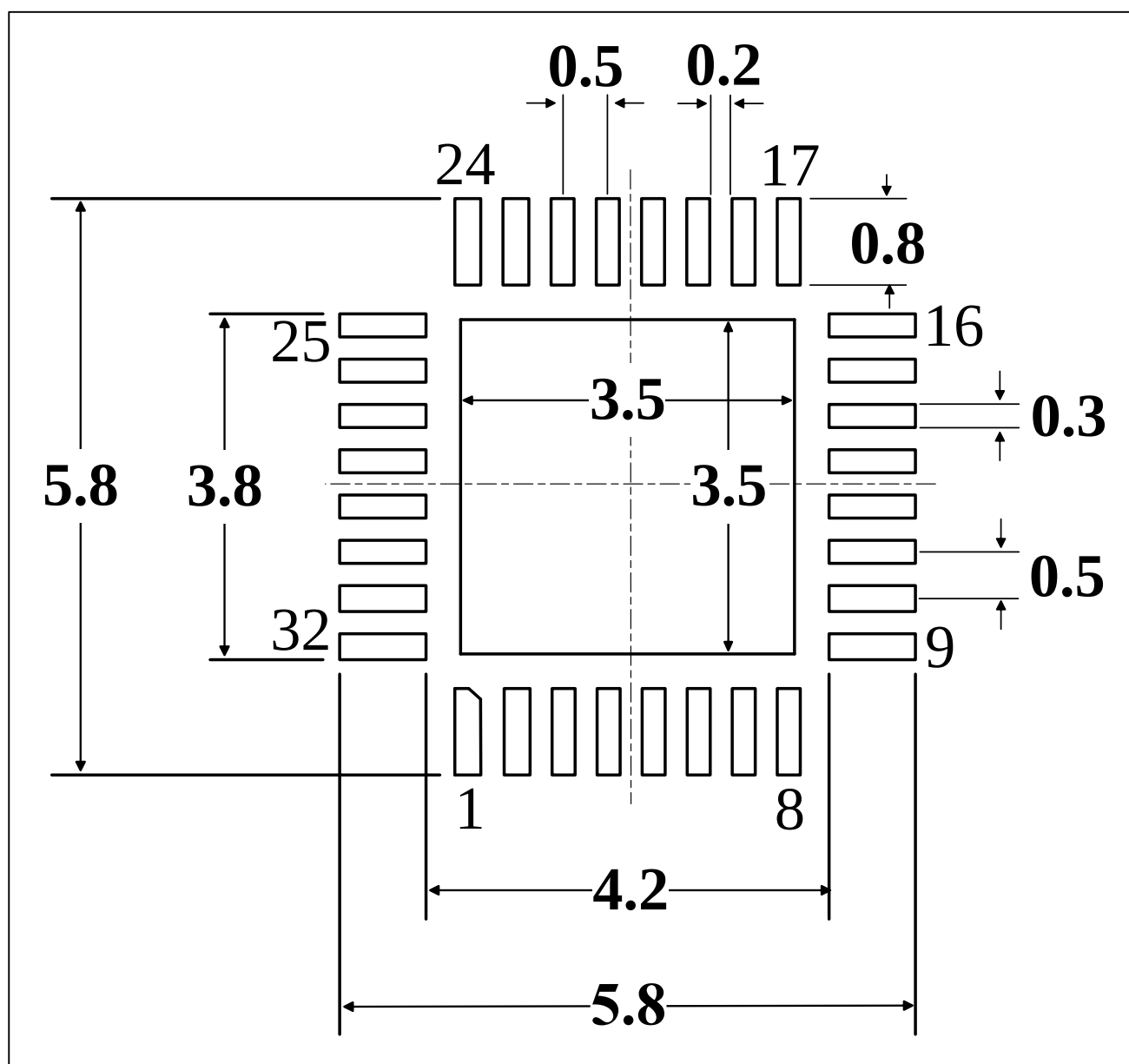
图 5-8 QFP32(5mm x 5mm)封装焊盘建议 (1)
