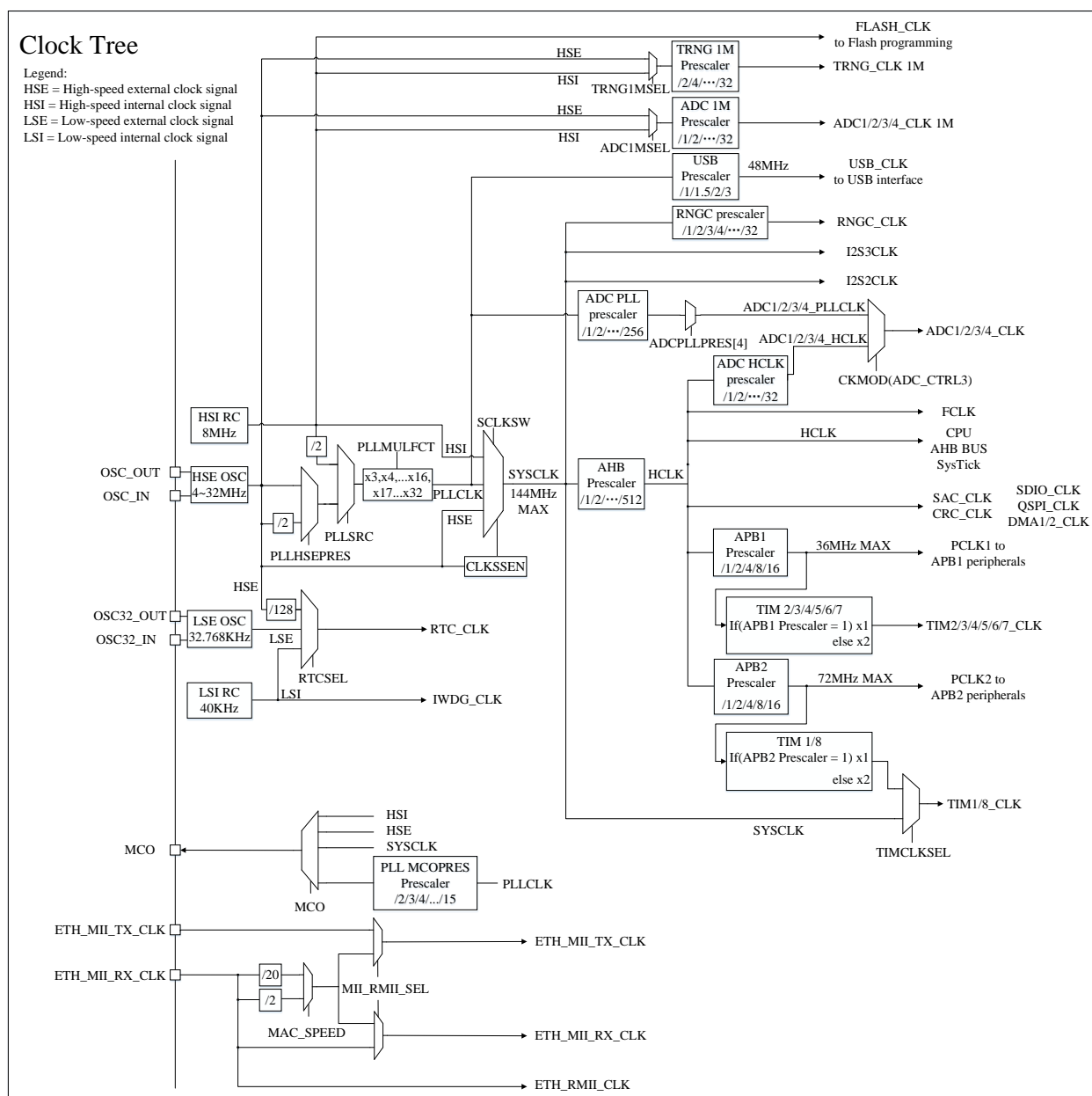
图 6-2 时钟树
