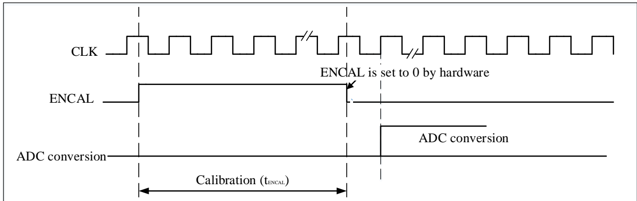
图 9-7 校准时序图
