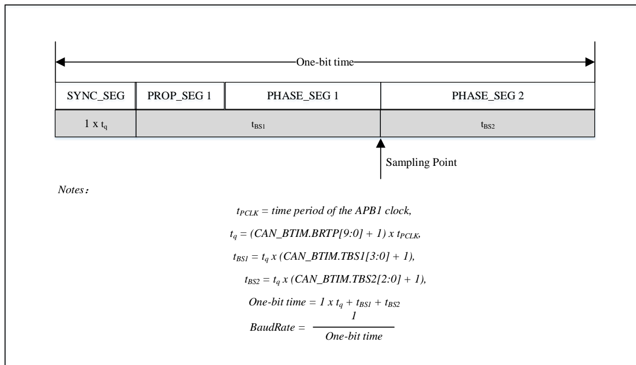
图 20-11 位时序
