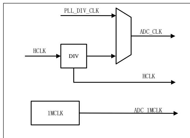
图 9-2 ADC 时钟
