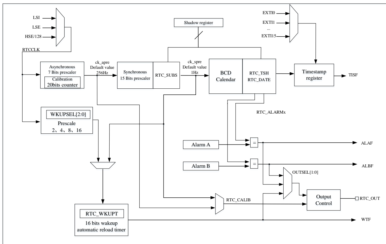
图 14-1 RTC 功能框图
