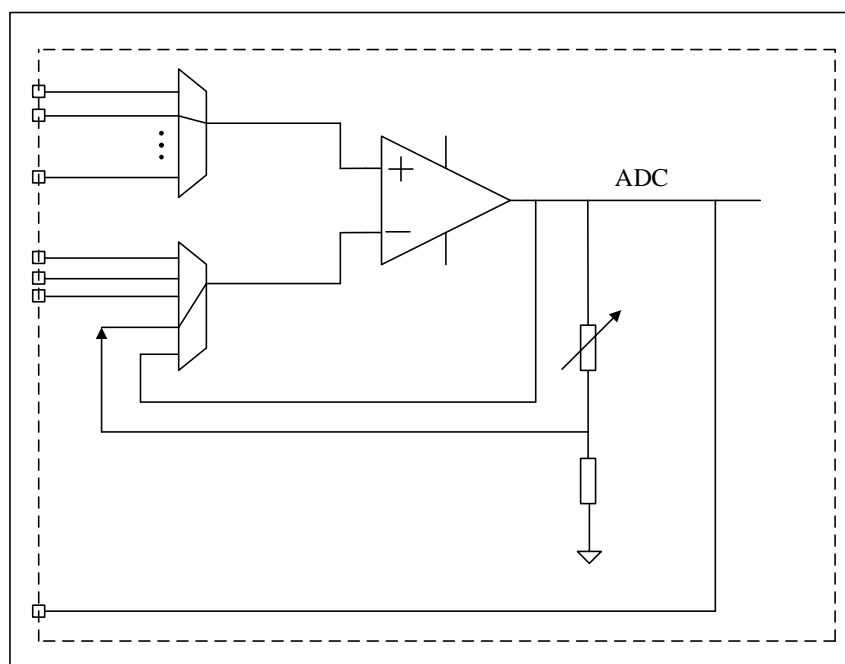
图 27-7 内部可编程增益模式
