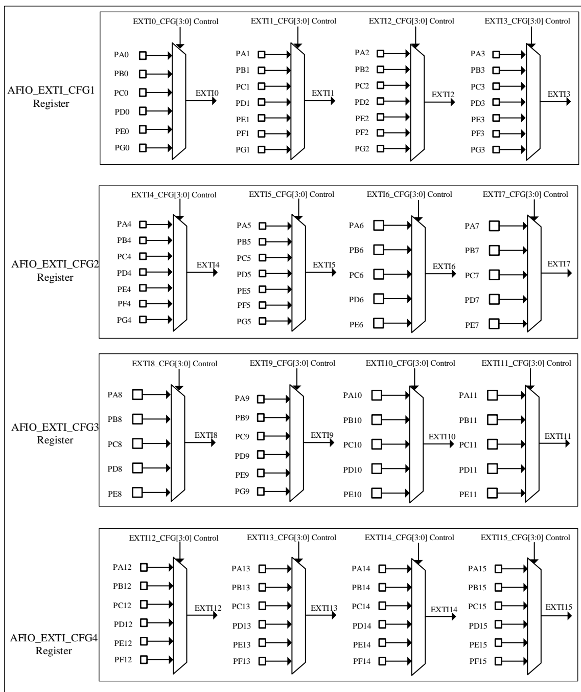
图 2-2 外部中断通用 I/O 映射
