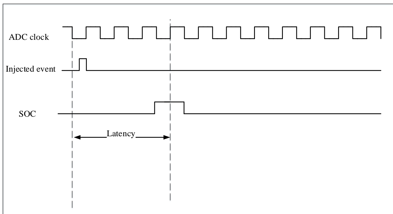
图 9-6 注入转换延时
