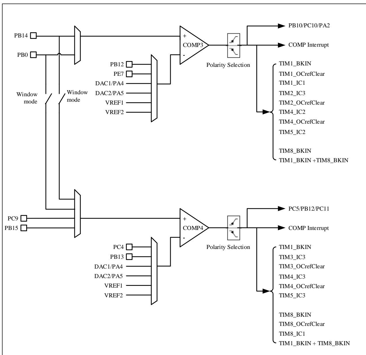
图 26-2 比较器 3 和比较器 4 系统连接图
