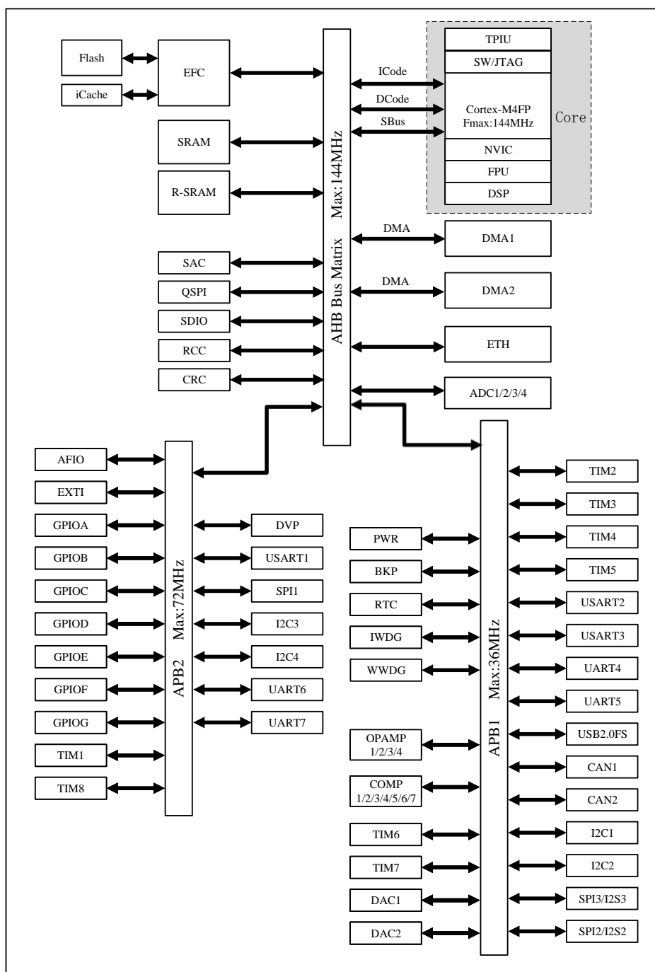
图 3-1 总线架构图
