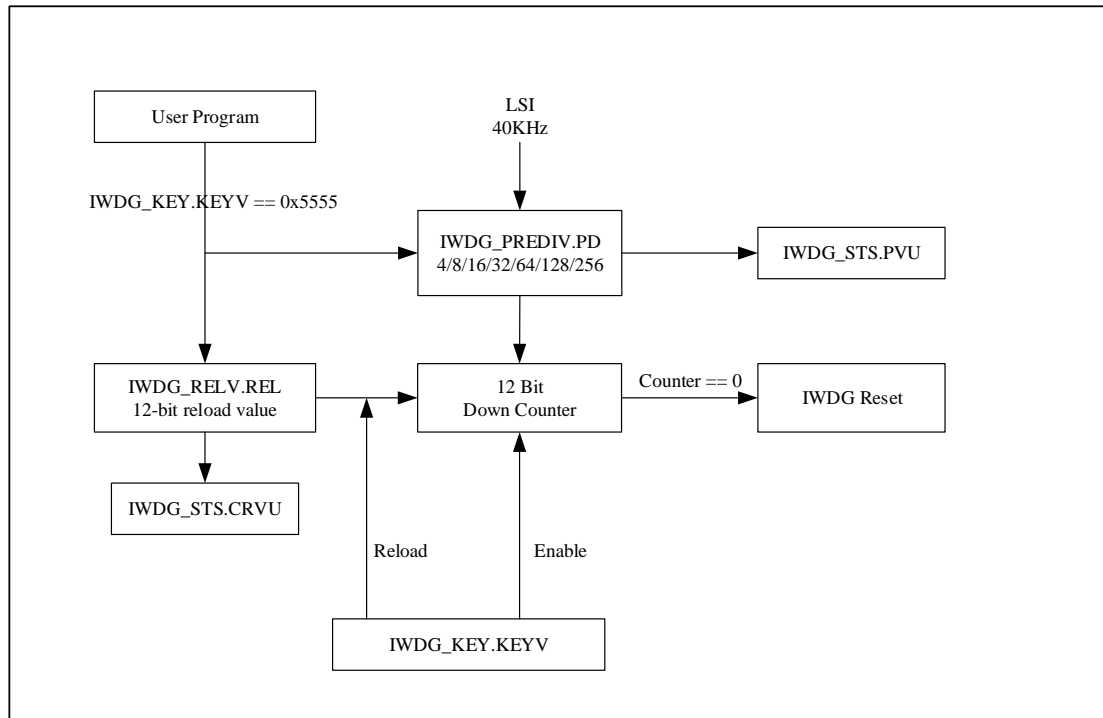
图 16-1 独立看门功能框图
