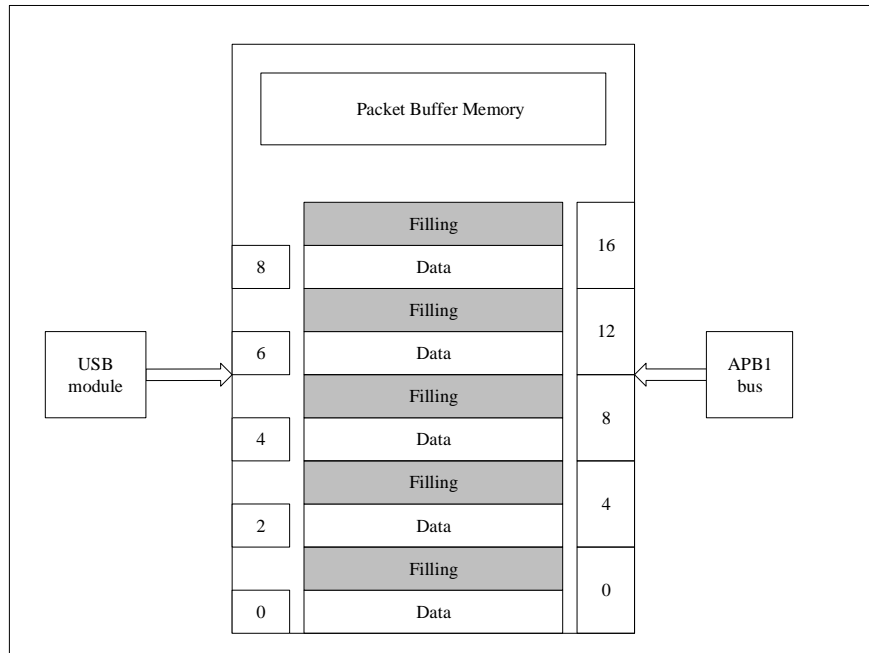
图 19-2 USB 模块和微控制器上的用户应用程序访问 Packet Buffer Memory 方式
