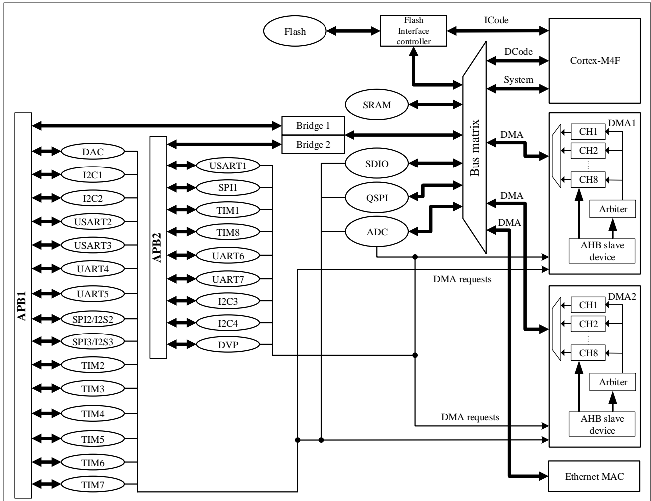
图 8-1 DMA 框图
