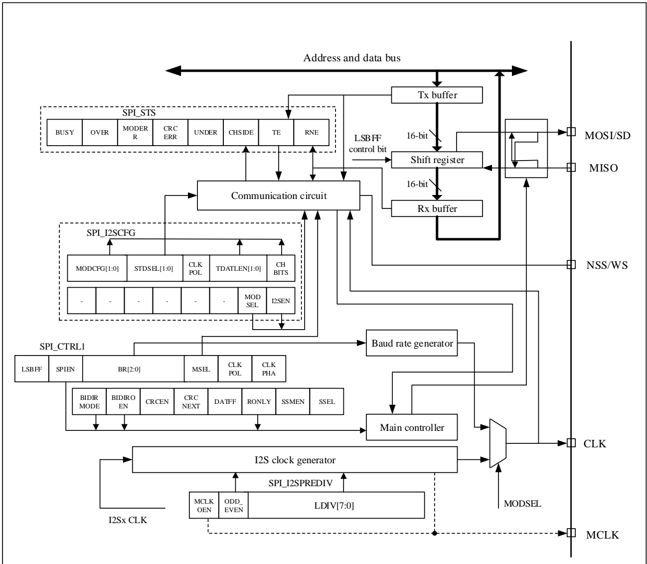
图 21-13 I 2 S 框图
