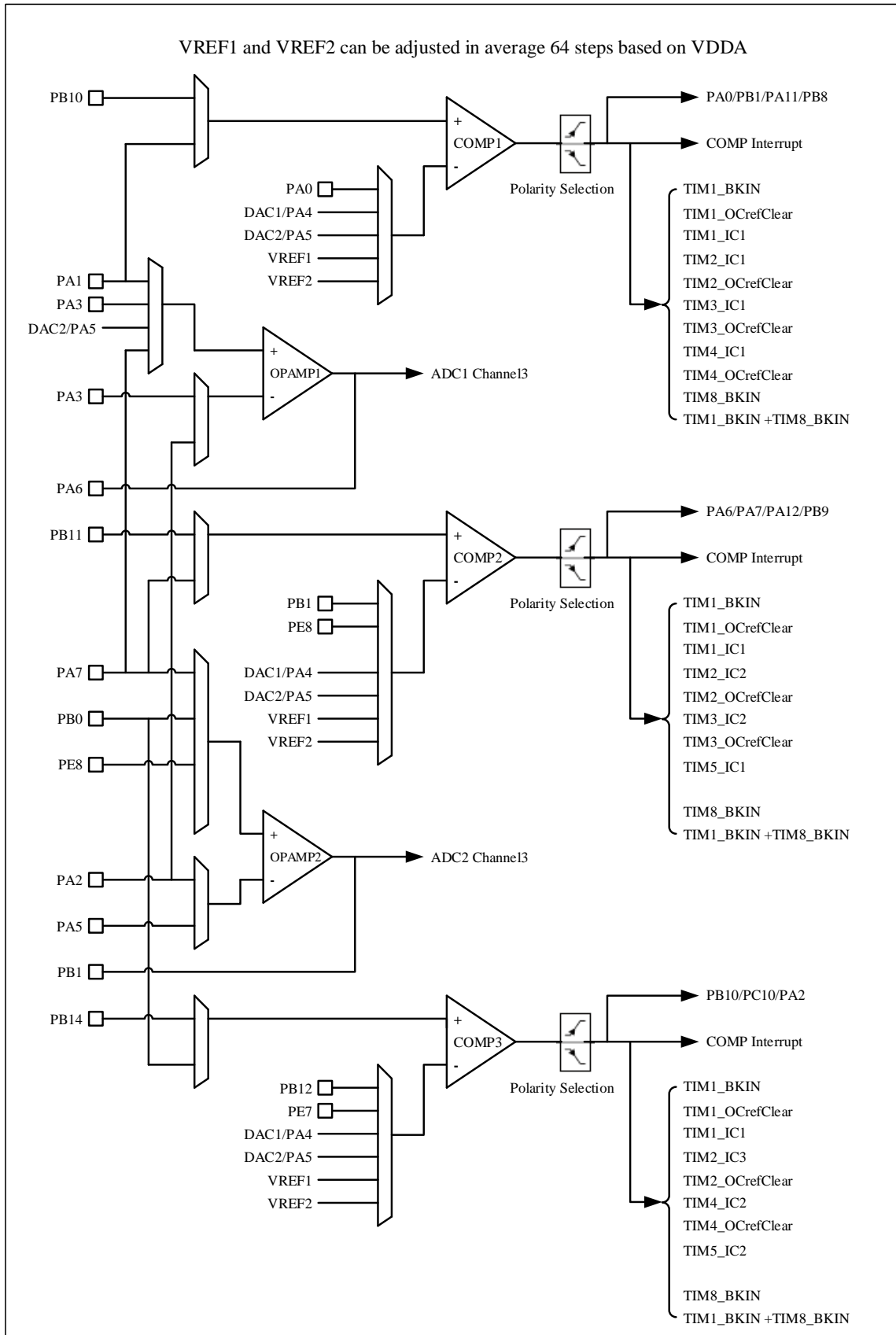
图 27-3 模拟模块联动关系 1
