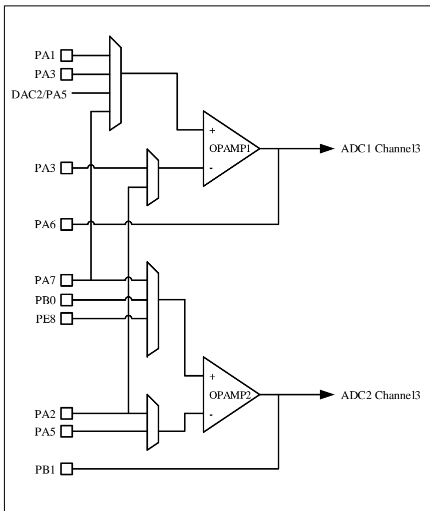
图 27-1 OPAMP1 和 OPAMP2 连接图框图
