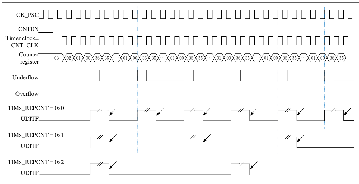
图 11-8 向下计数模式下的重复计数时序图
