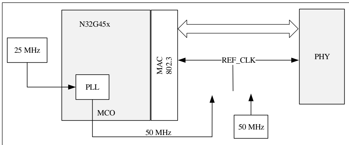
图 25-7 RMII 时钟源
