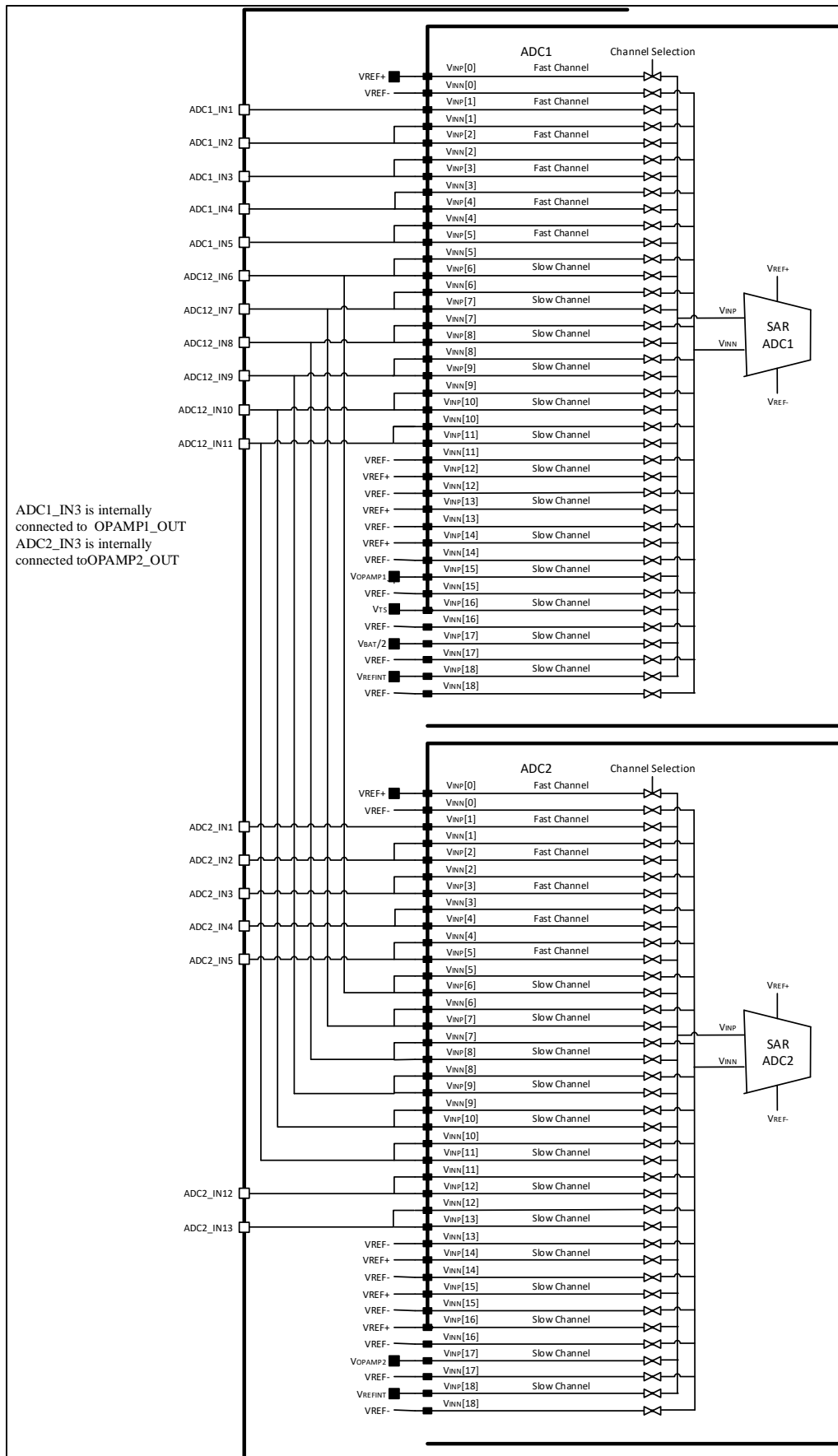
图 9-3 ADC1 和 ADC2 通道引脚连接
