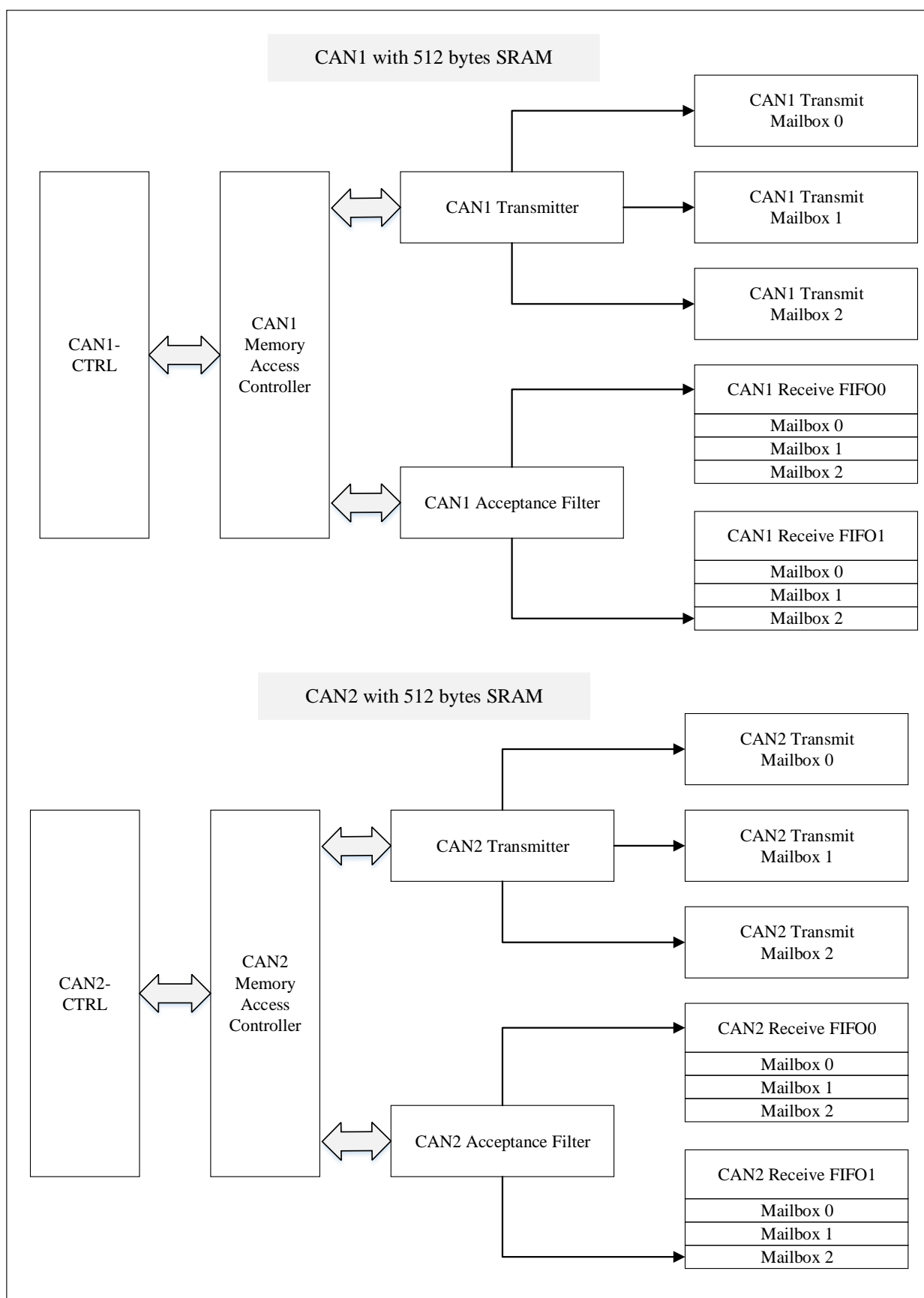
图 20-3 双 CAN 框图
