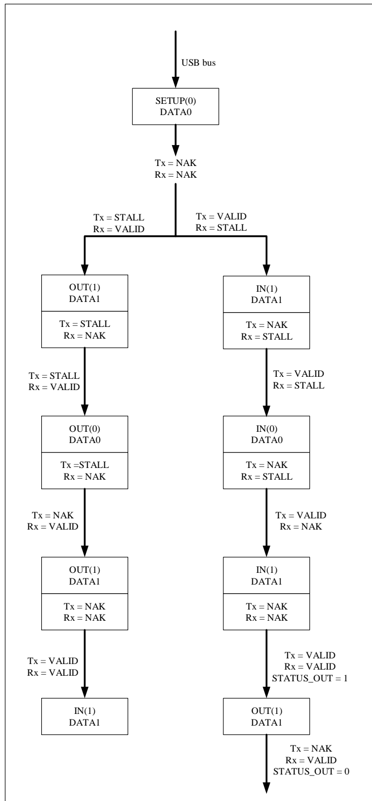
图 19-5 控制传输
