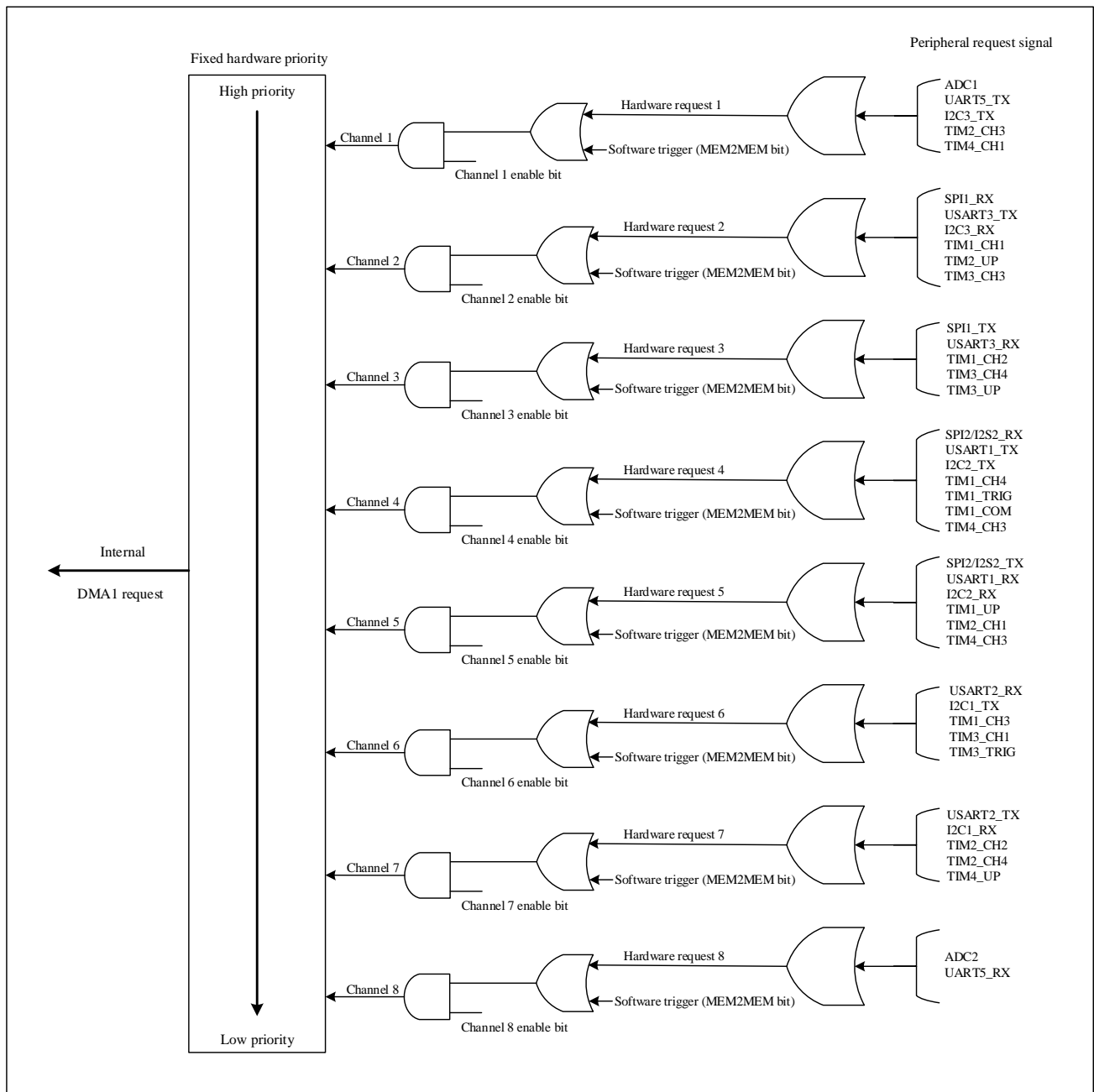
图 8-2 DMA1 请求映像
