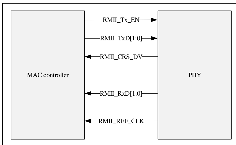
图 25-6 RMII 接口信号线
