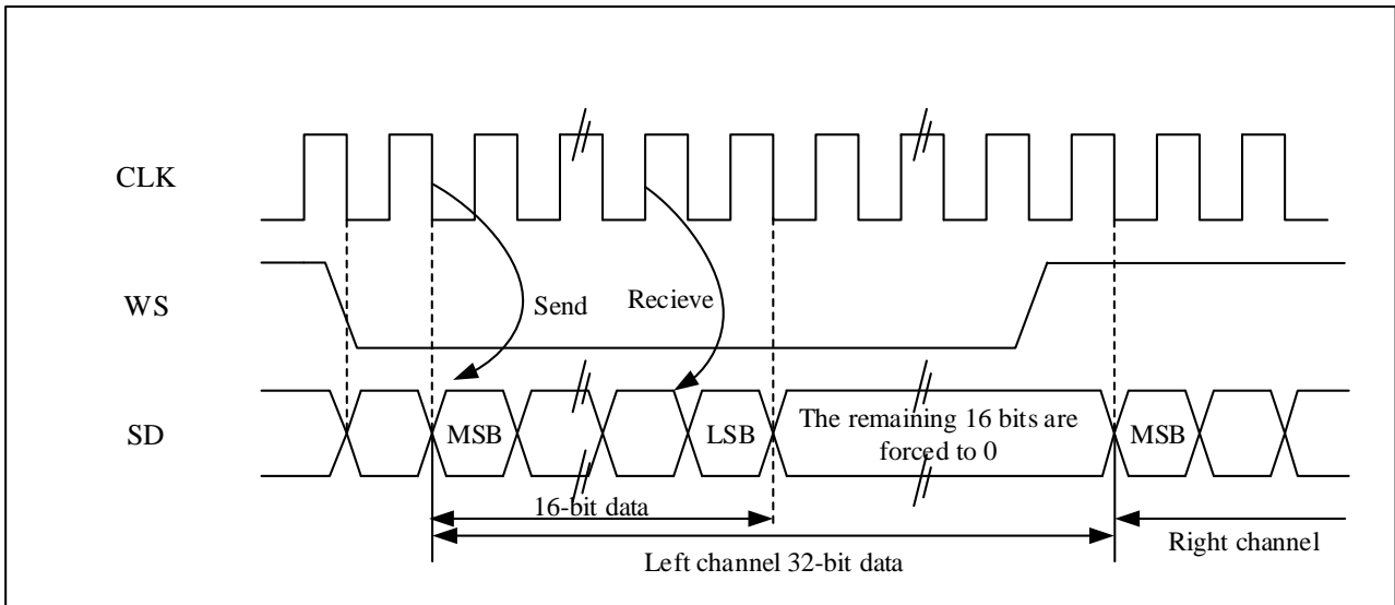
图 21-16 I 2 S 飞利浦协议标准波形（16 位扩展至 32 位包帧，CLKPOL = 0）
