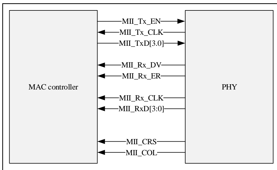
图 25-4 MII 接口信号线
