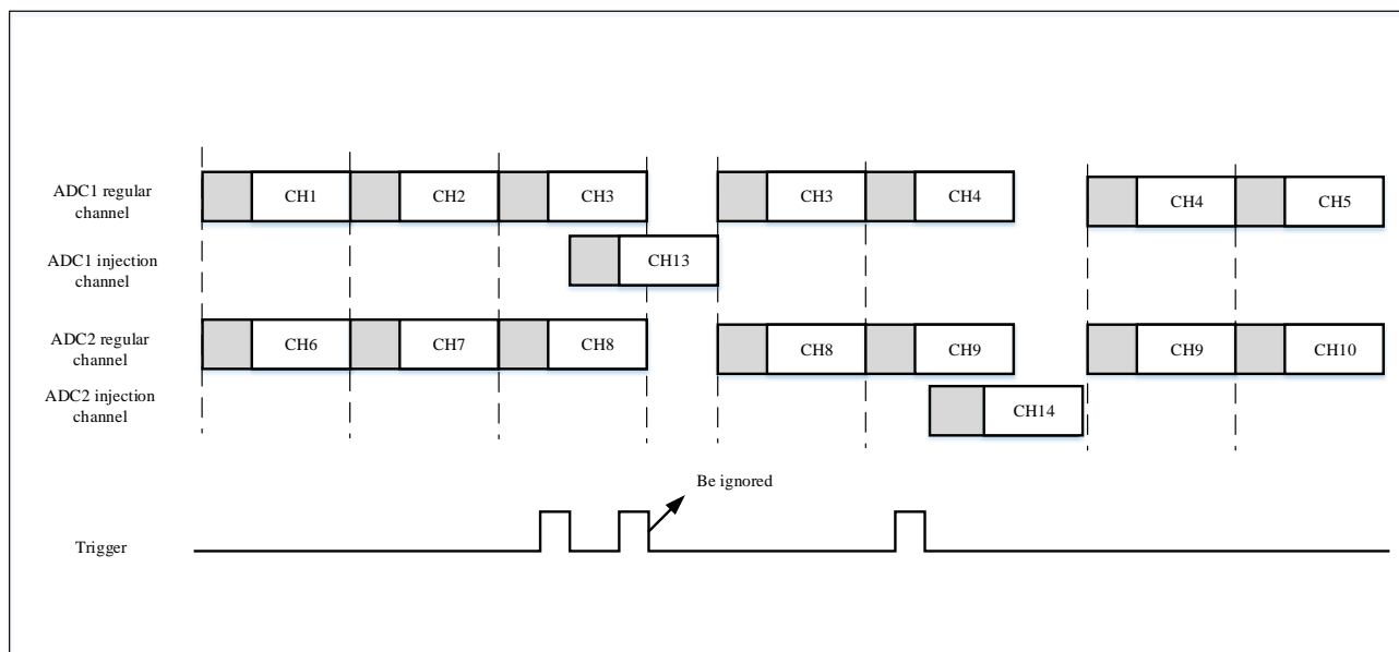
图 9-16 在注入转换期间发生注入触发
