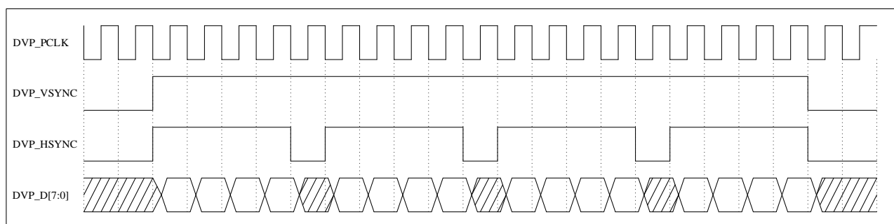
图 28-1 DVP 接口时序示例
