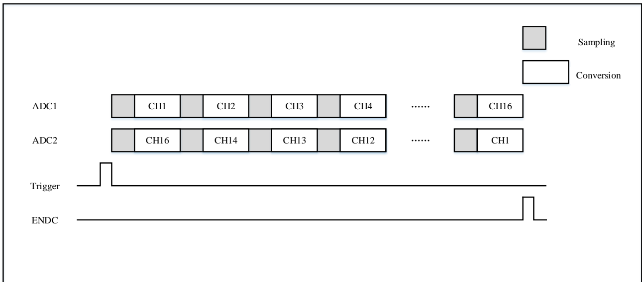
图 9-9 16 个通道的同步规则模式转换示意图
