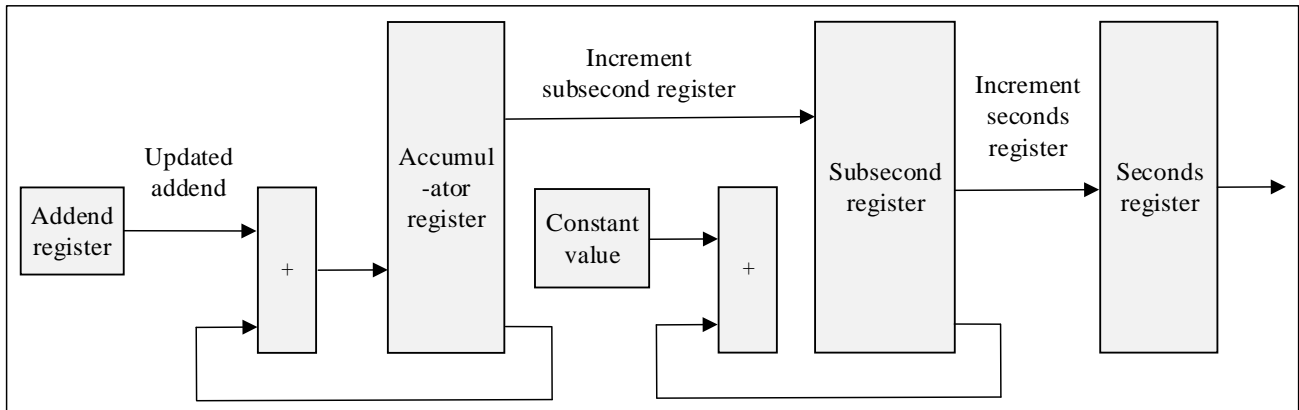
图 25-9 系统时间精密校准
