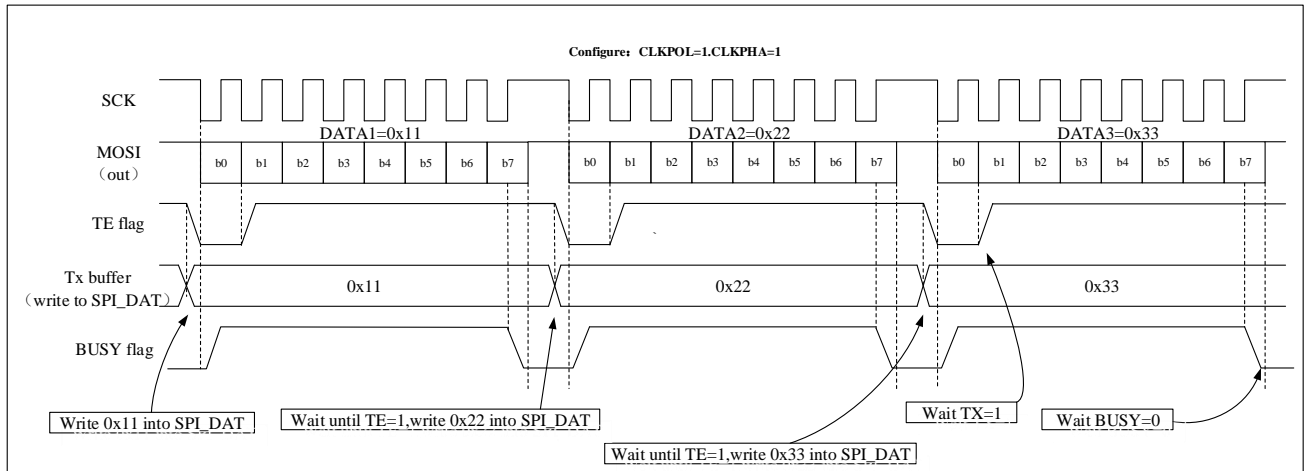
图 21-10 BIDIRMODE = 0, RONLY = 0 非连续传输发送时，SPI_STE.TE/BUSY 变化示意图
