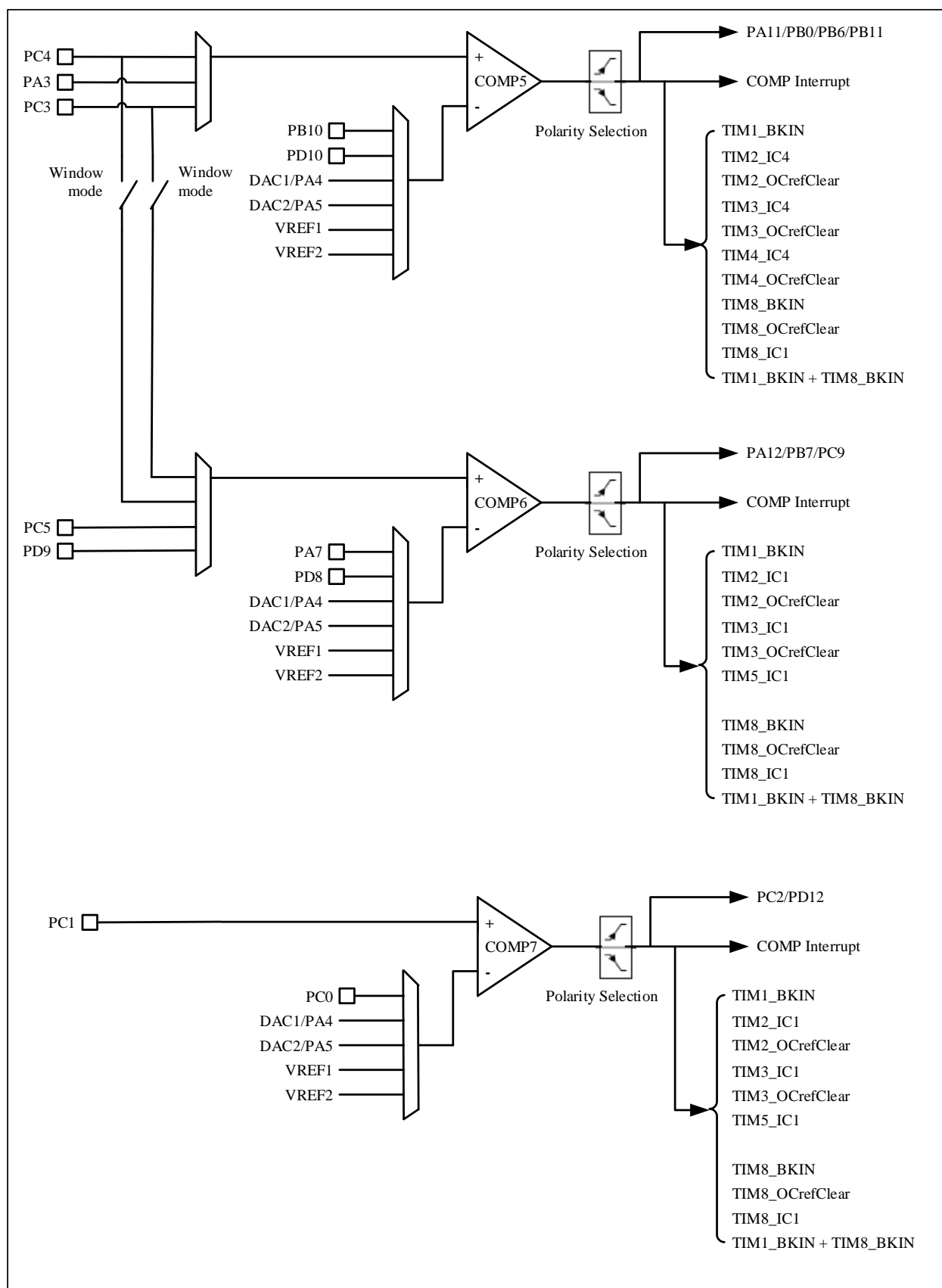
图 26-3 比较器 5，比较器 6，比较器 7 系统连接图
