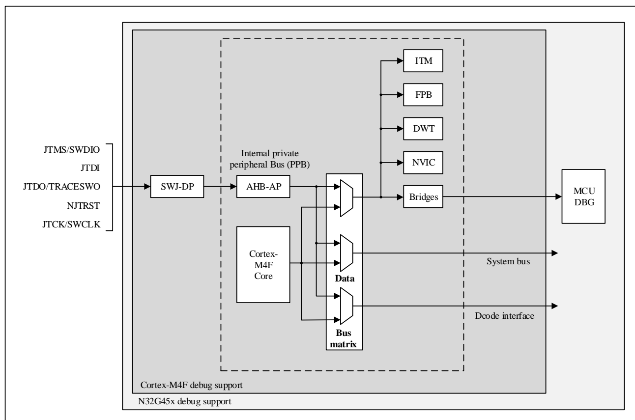
图 29-1 N32G45x 级别和 Cortex™-M4F 级别的调试框图
