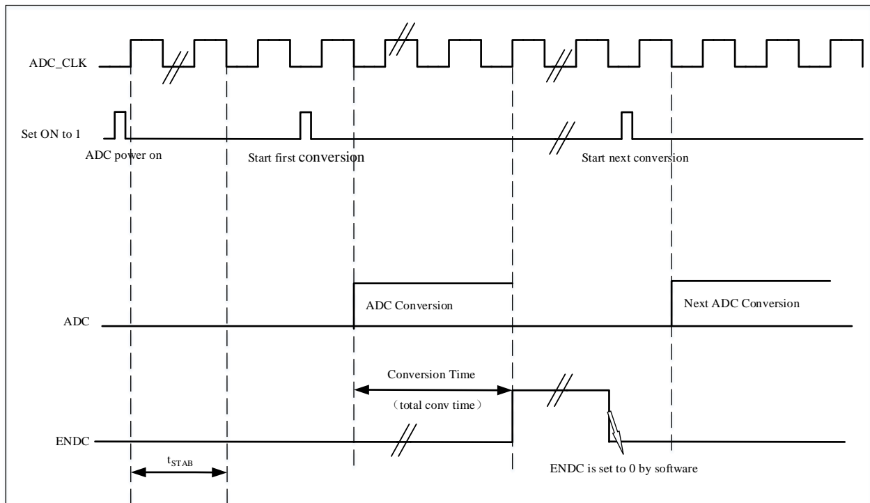
图 9-5 时序图
