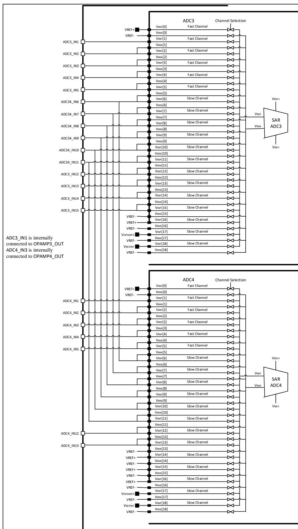
图 9-4 ADC3 和 ADC4 通道引脚连接
