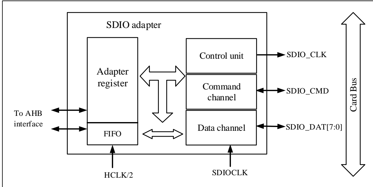
图 18-7 SDIO 适配器
