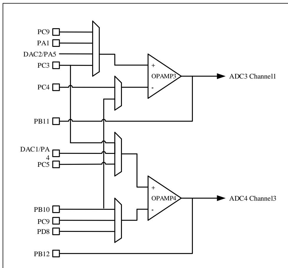
图 27-2 OPAMP3 和 OPAMP4 连接图框图
