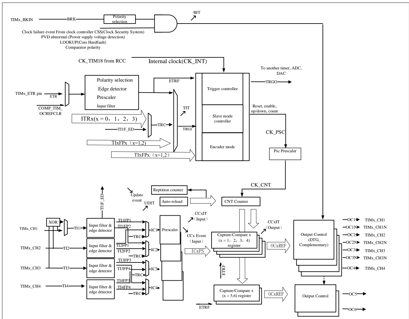
图 11-1 TIMx(x=1/8)框图
