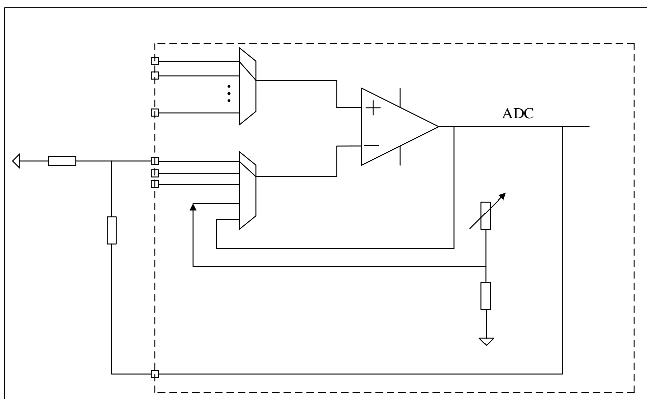
图 27-5 OPAMP 独立运算放大器模式
