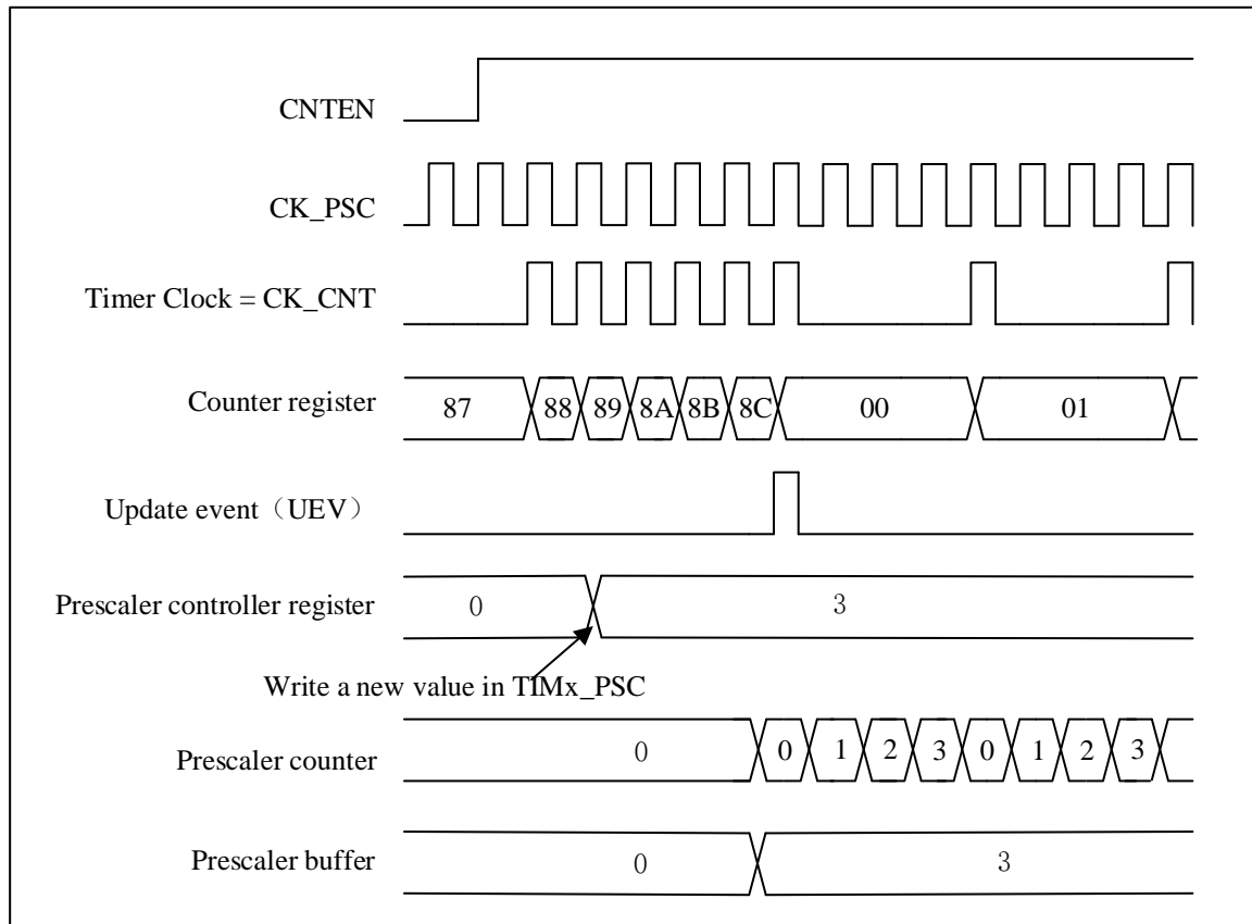
图 13-2 预分频器分频从 1 到 4 的计数器时序图
