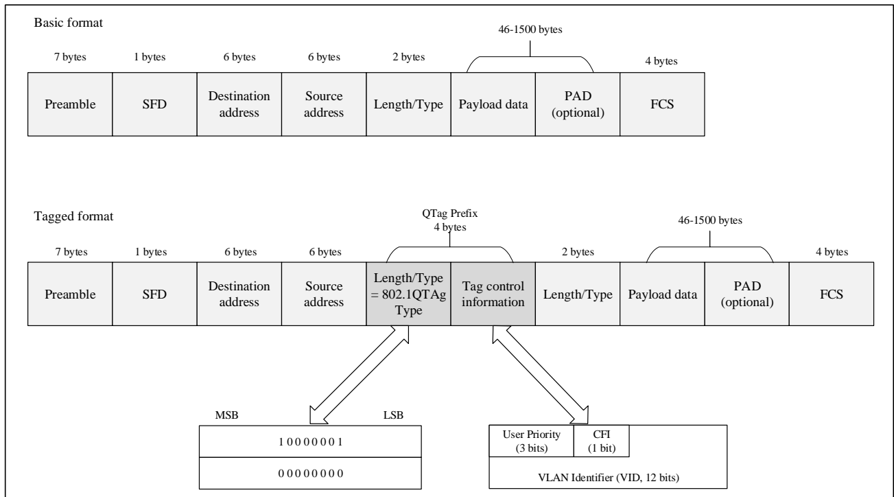
图 25-2 MAC 帧格式与帧结构
