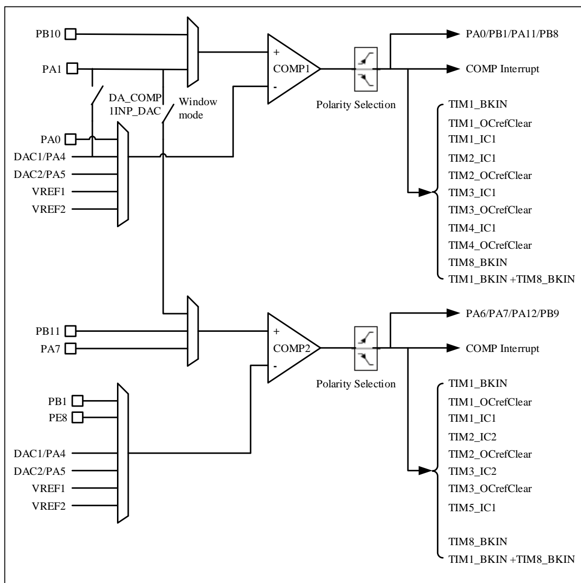
图 26-1 比较器 1 和比较器 2 系统连接图
