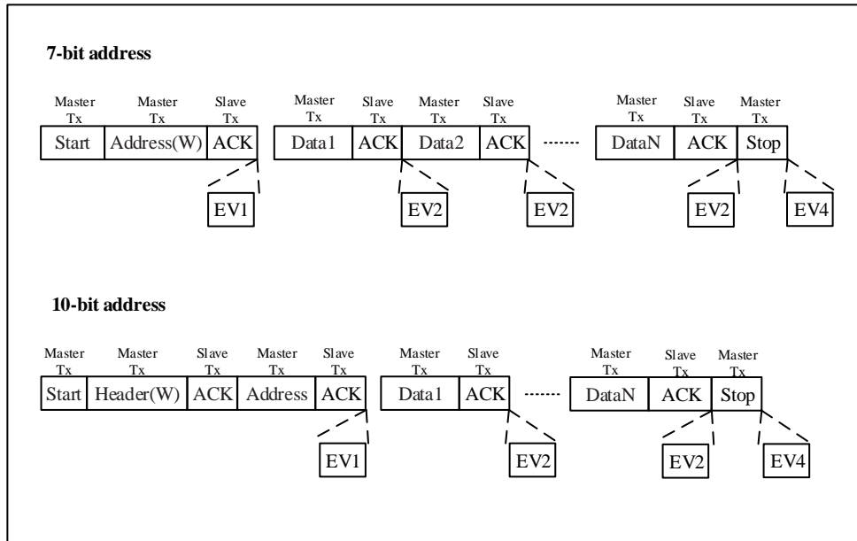
图 22-4 从机接收器传送序列
