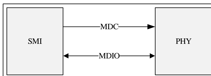
图 25-3 SMI 接口信号线
