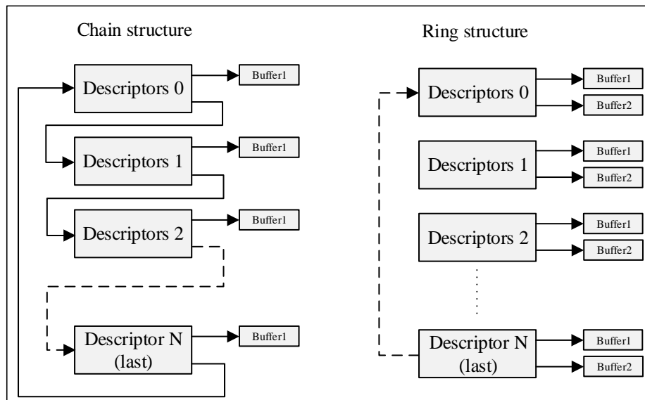
图 25-8 描述符的两种结构
