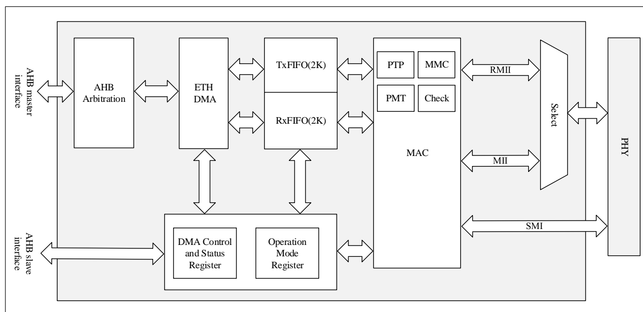
图 25-1 以太网模块框图
