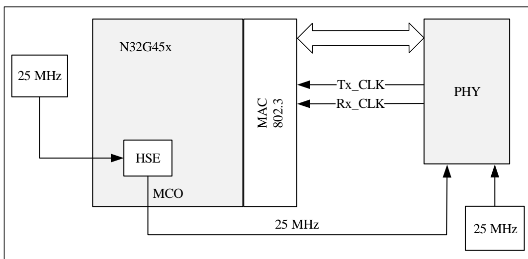
图 25-5 MII 时钟源
