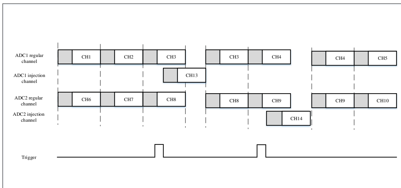
图 9-15 交替模式和规则同步模式组合
