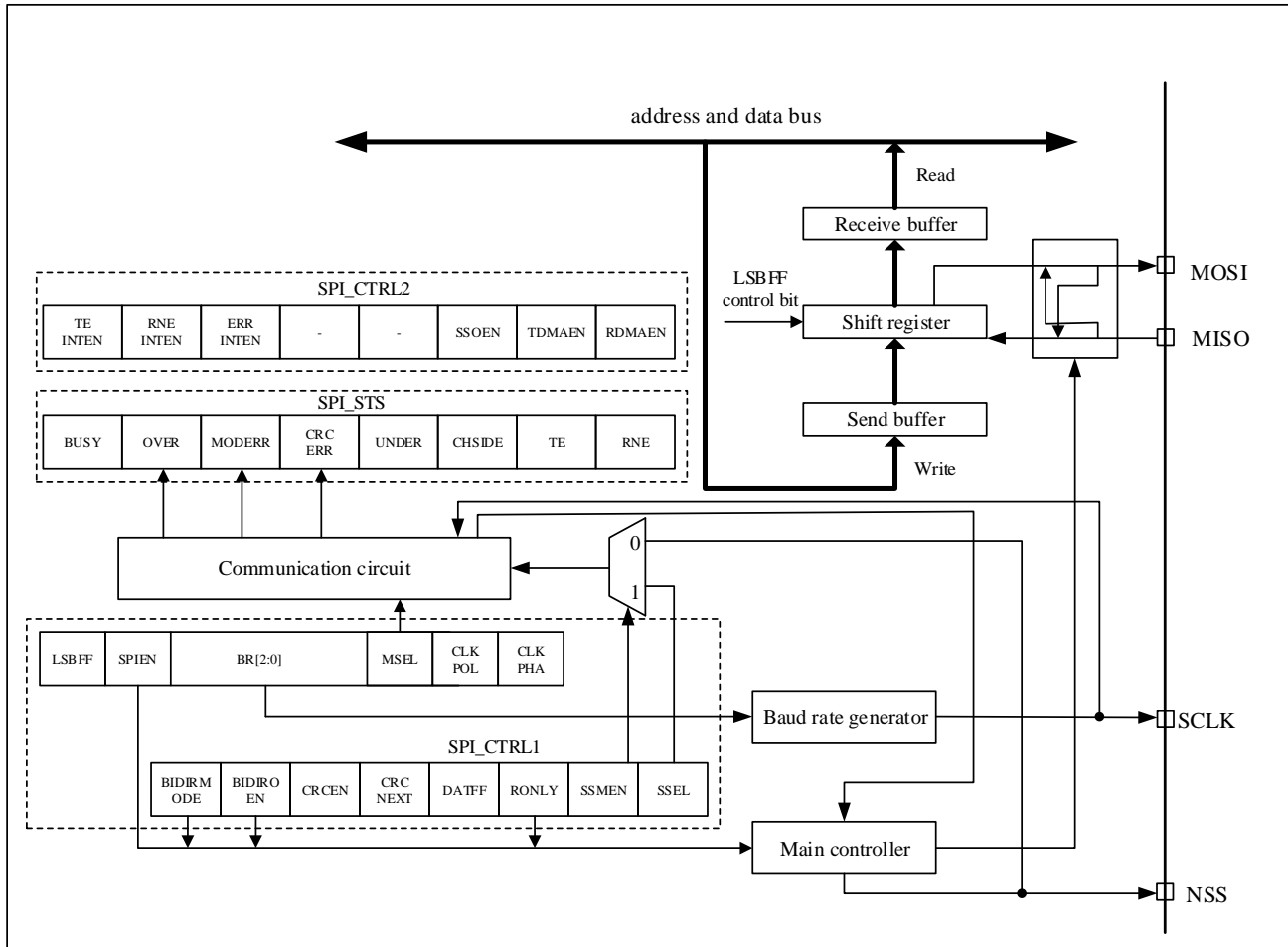
图 21-1 SPI 框图
