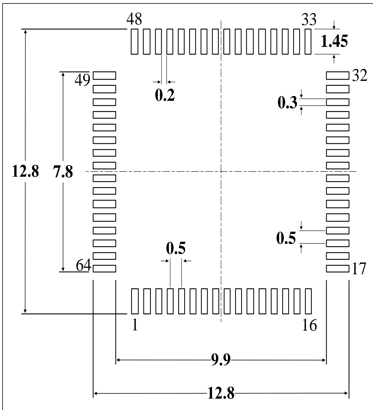
图 5-6 LQFP64 (10mm x 10mm) 封装焊盘建议 (1)
