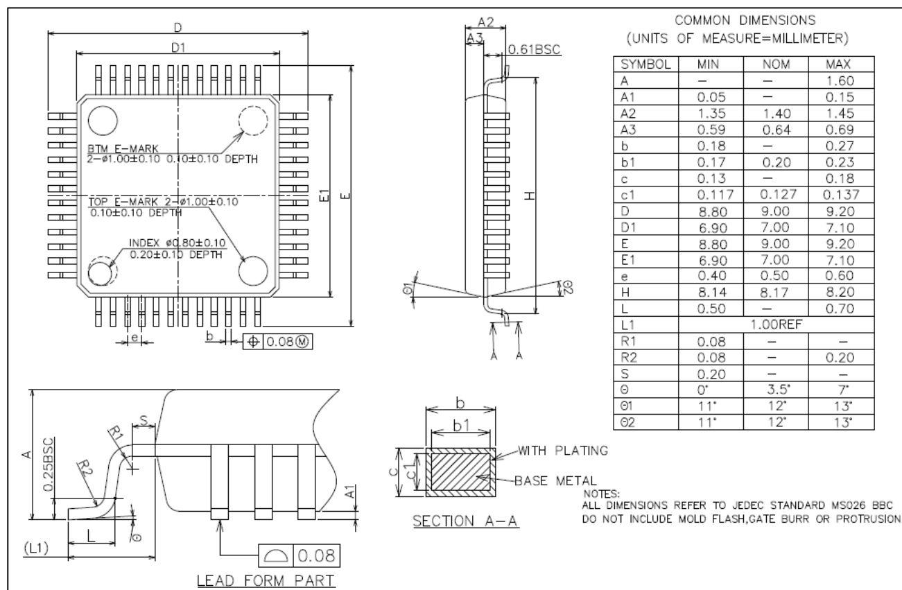
图 5-3 LQFP48(7mm x 7mm)封装尺寸
