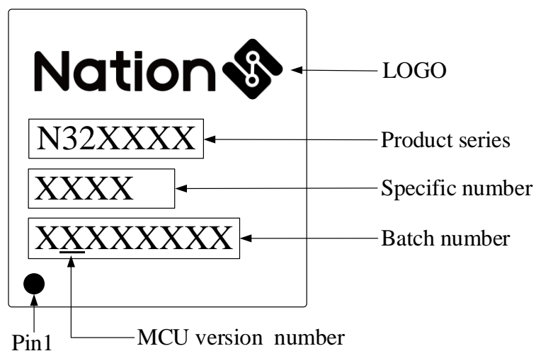
图 5-7 丝印说明
