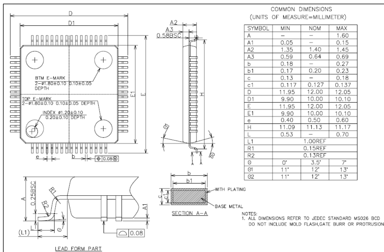
图 5-5 LQFP64(10mmx10mm)封装尺寸
