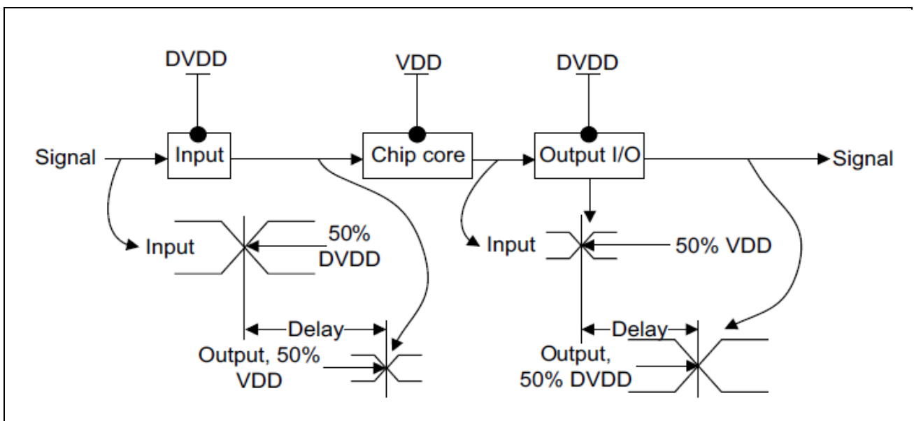
图 4-10 传输延迟
