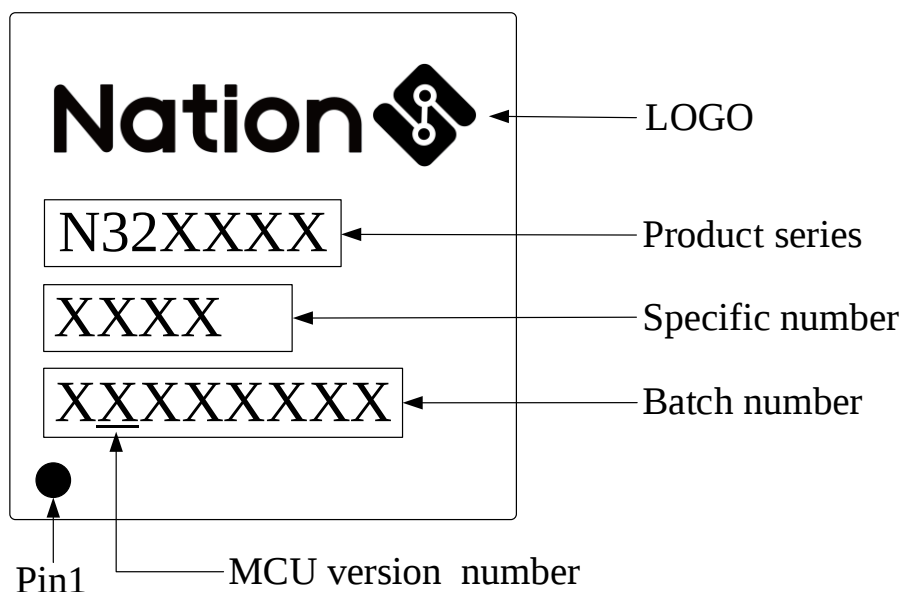
图 5-15 LQFP48/LQFP32/QFN48/QFN32/QFN28丝印说明
