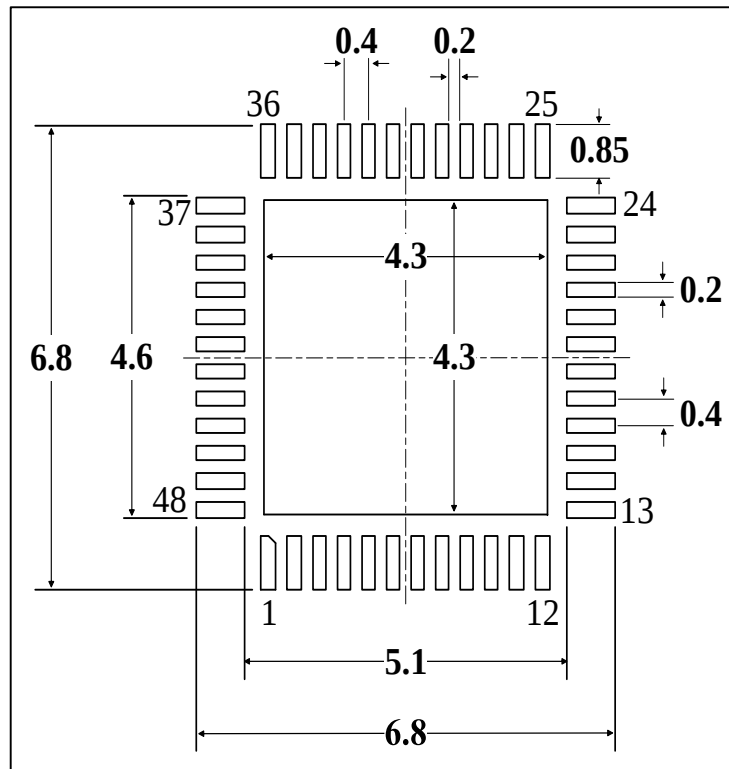
图 5-12 QFN48封装焊盘建议 (1)
