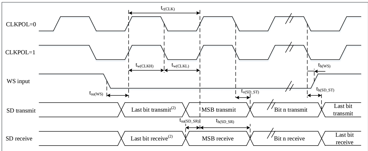
图 4-16 I²S从模式时序图(飞利浦协议) (1)
