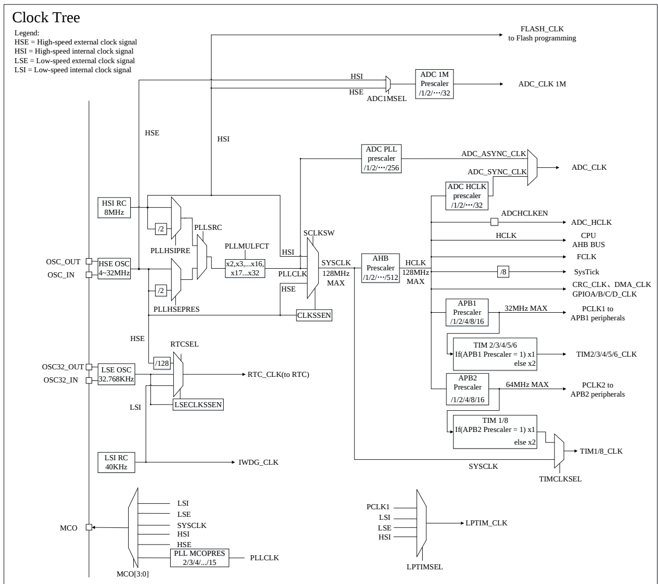
图 2-2 时钟树
