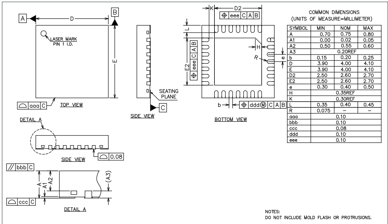
图 5-7 QFN28封装尺寸
