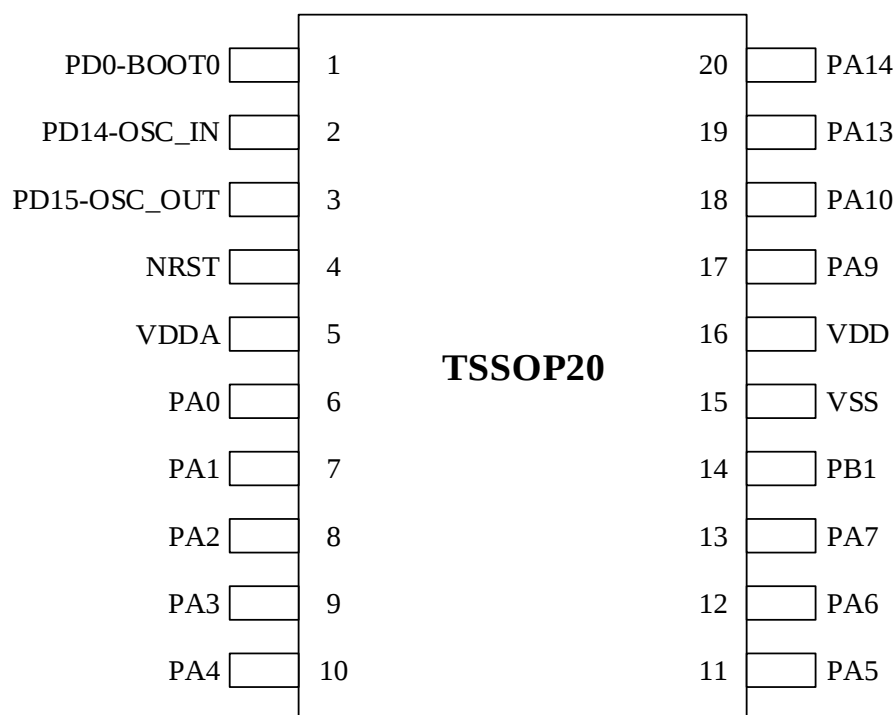
图 3-9 N32G401 系列 TSSOP20 引脚分布
