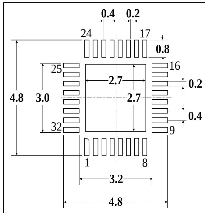
图 5-14 QFN32-2封装焊盘建议 (1)
