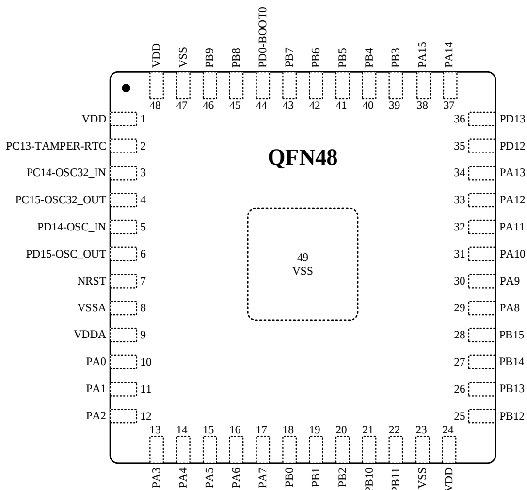
图 3-8 N32G401 系列 QFN48 引脚分布
