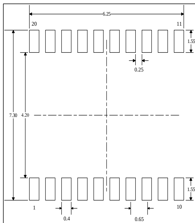
图 5-18 TSSOP20封装焊盘建议 (1)
