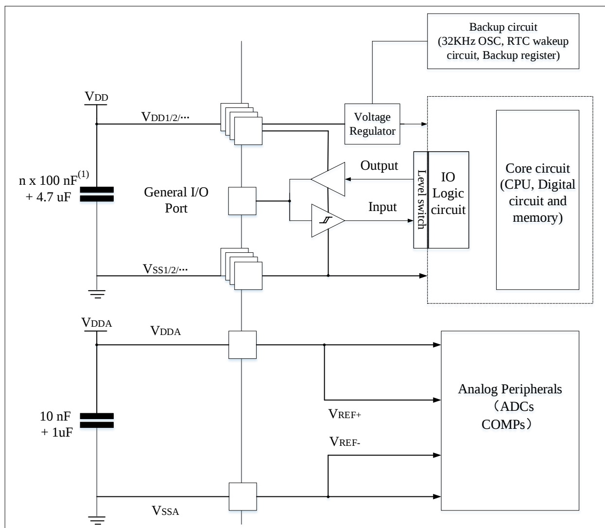
图 4-3 供电方案
