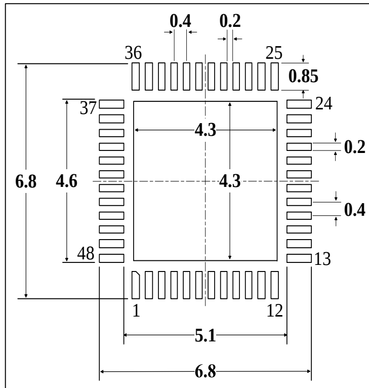
图 5-16 QFN48封装焊盘建议 (1)
