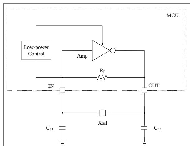
图 4-8 使用 32.768KHz 晶体的典型应用
