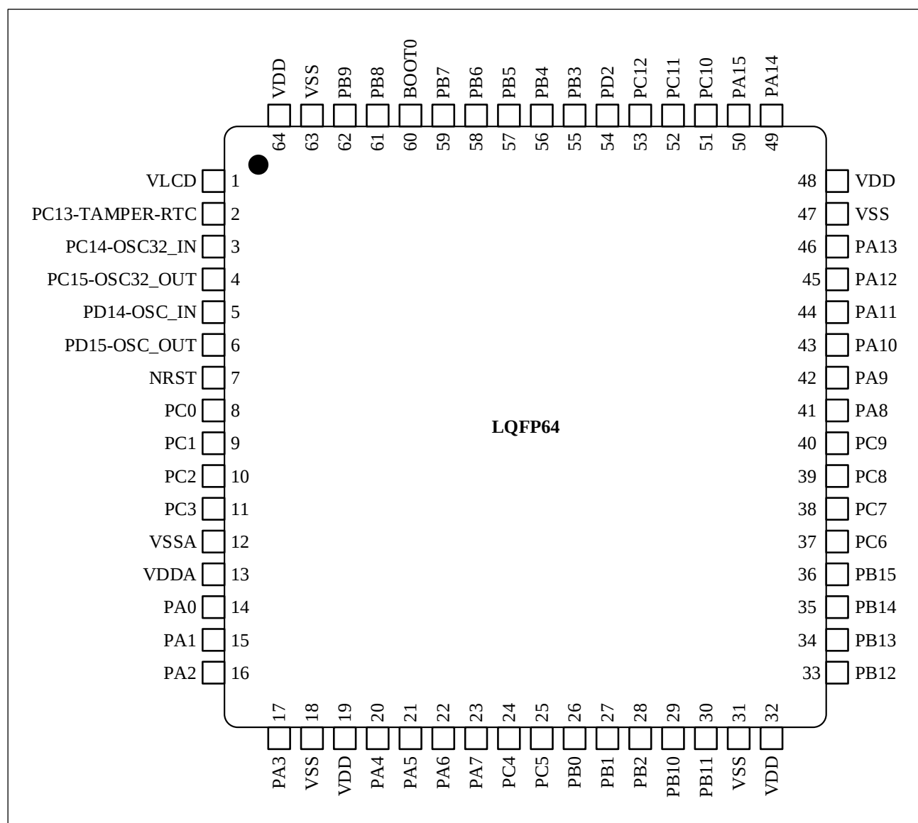
图 3-3 N32L436 系列 LQFP64 引脚分布
