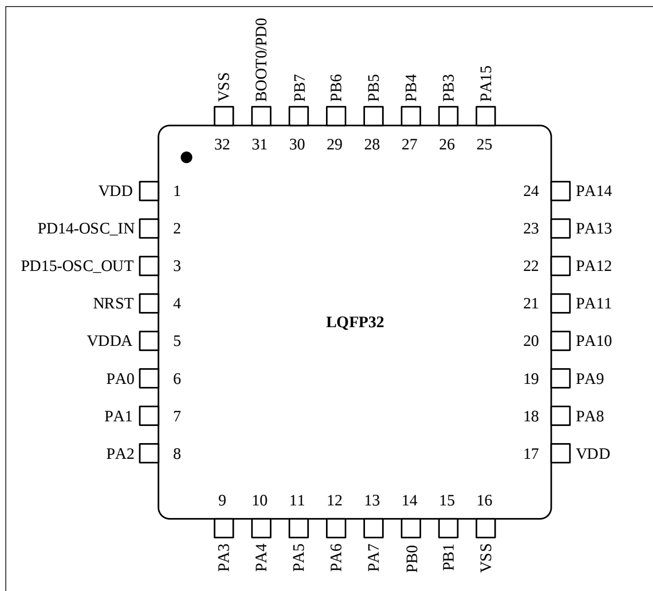
图 3-1 N32L433 系列 LQFP32 引脚分布
