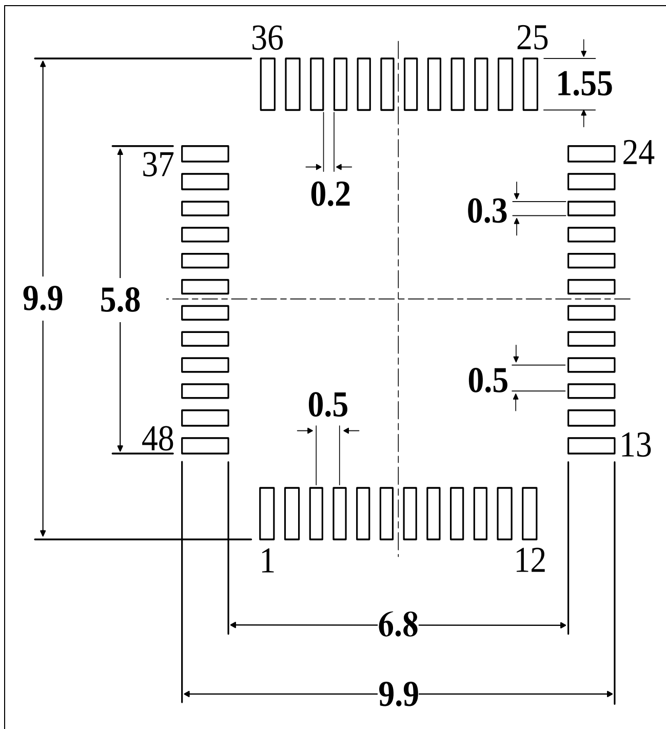
图 5-4 LQFP48 封装焊盘建议 (1)
