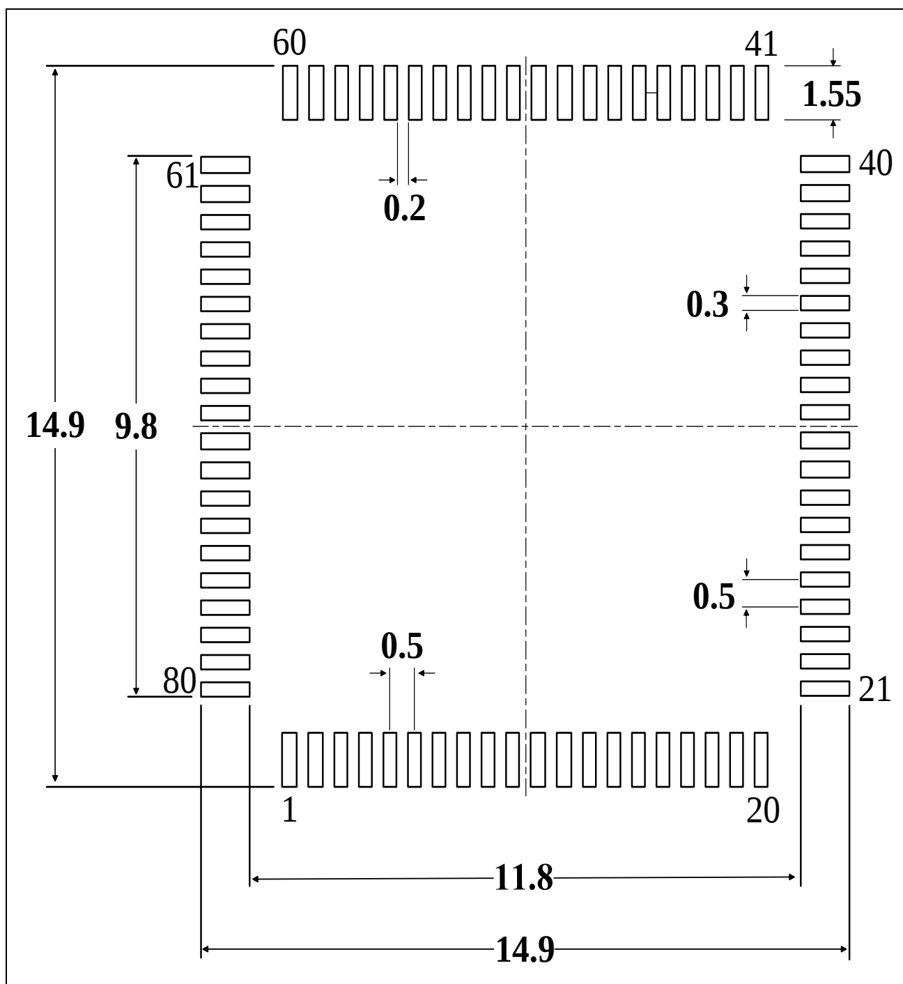
图 5-8 LQFP80封装焊盘建议 (1)
