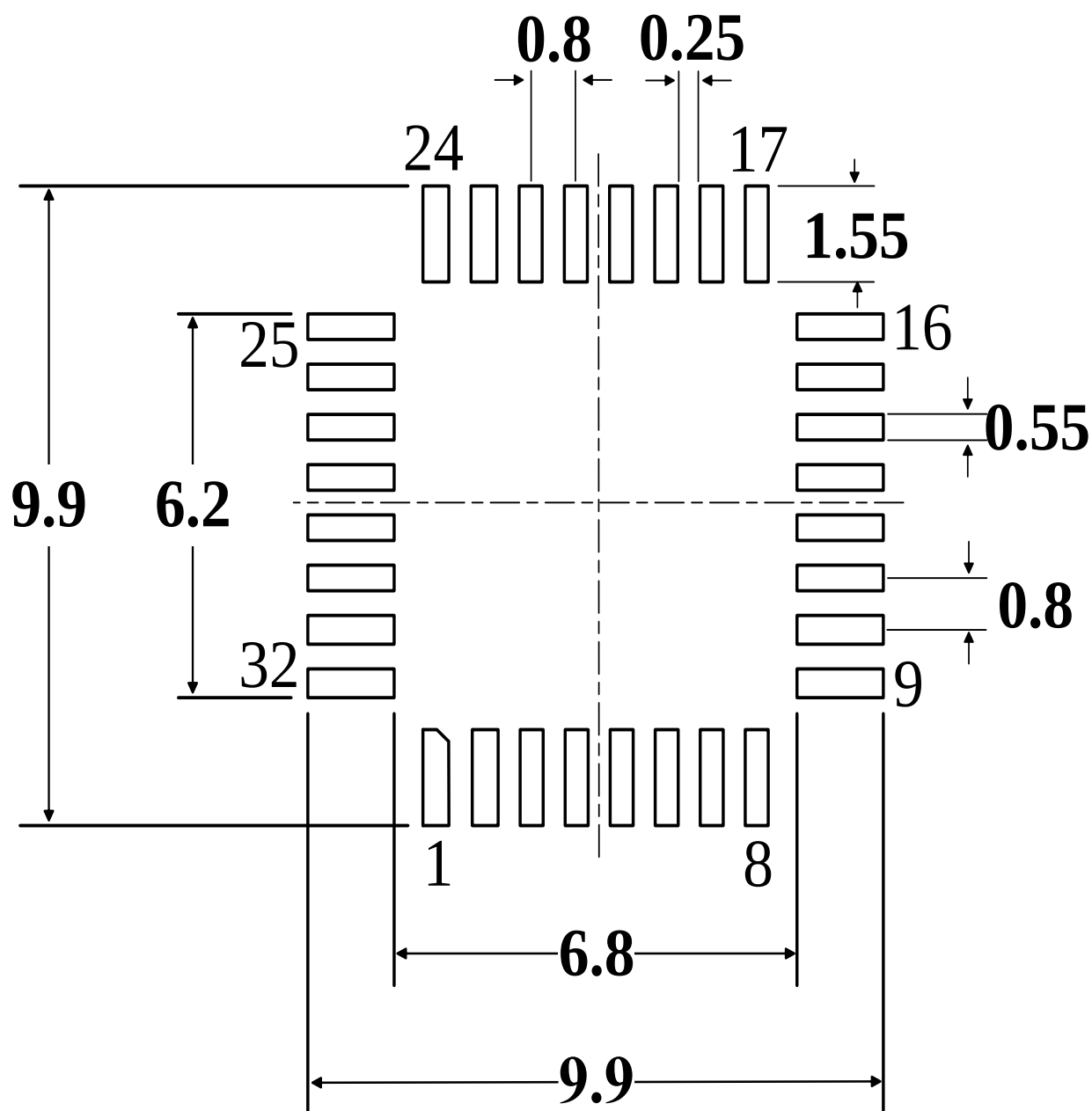
图 5-2 LQFP32 封装焊盘建议 (1)
