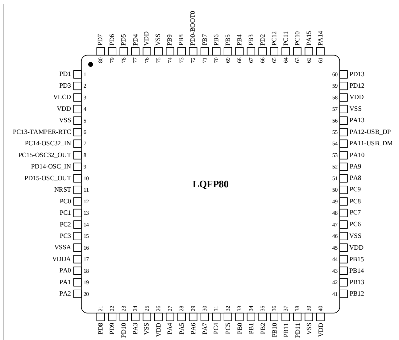
图 3-4 N32L436 系列 LQFP80 引脚分布
