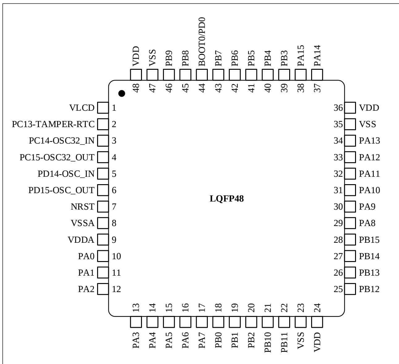
图 3-2 N32L436 系列 LQFP48 引脚分布
