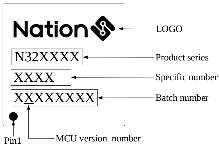
图 5-9 丝印说明
