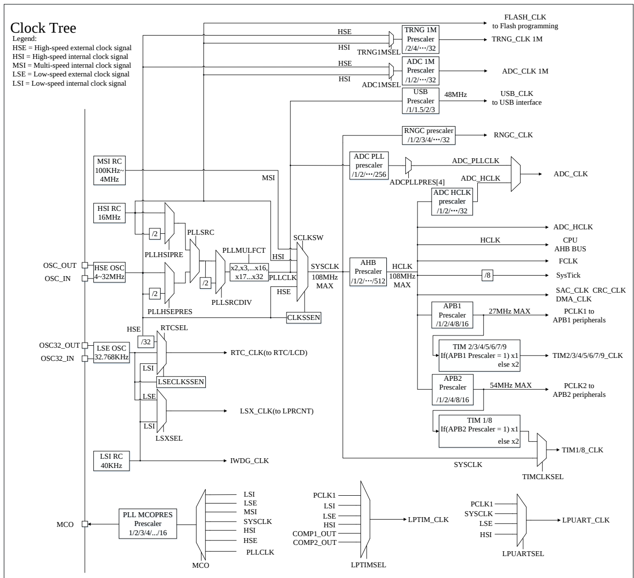
图 2-2 时钟树
