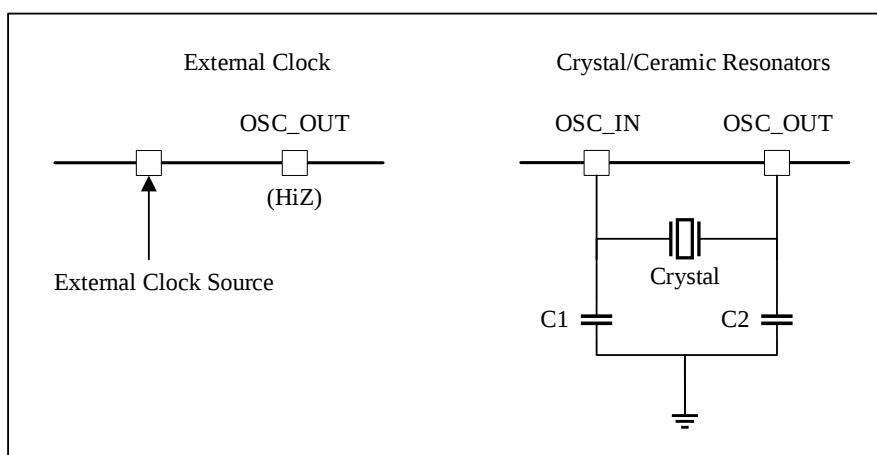
图 4-3 HSE/LSE 时钟源
