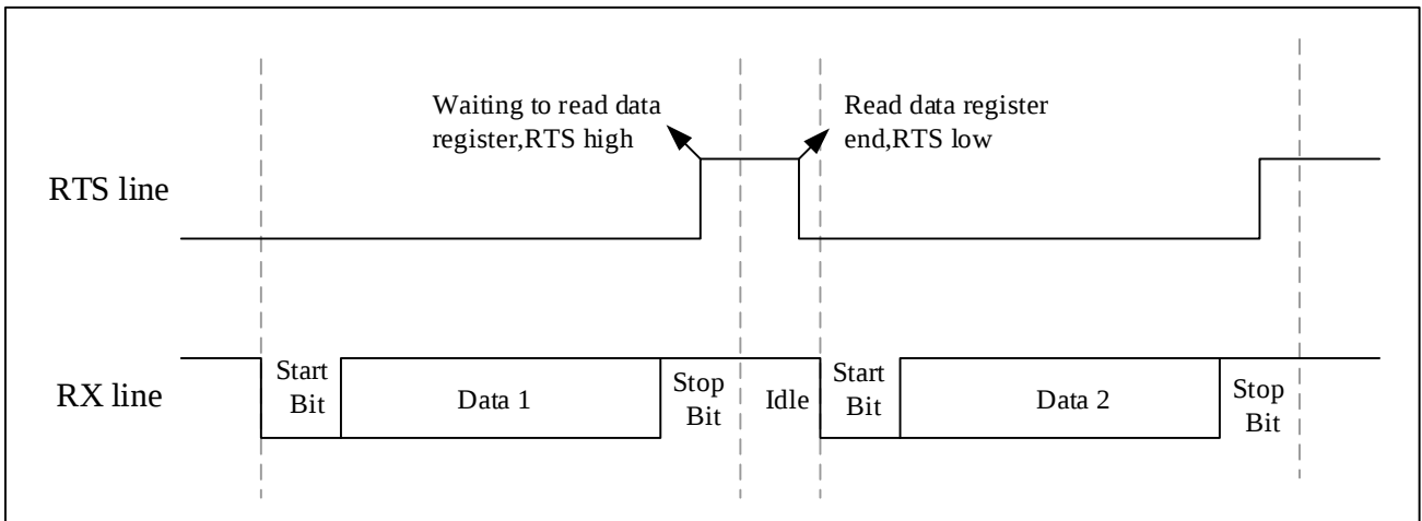
图 24-11 RTS 流控制
