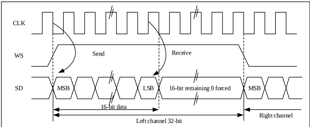
图 26-19 MSB 对齐 16 位数据扩展到 32 位包帧，CLKPOL = 0
