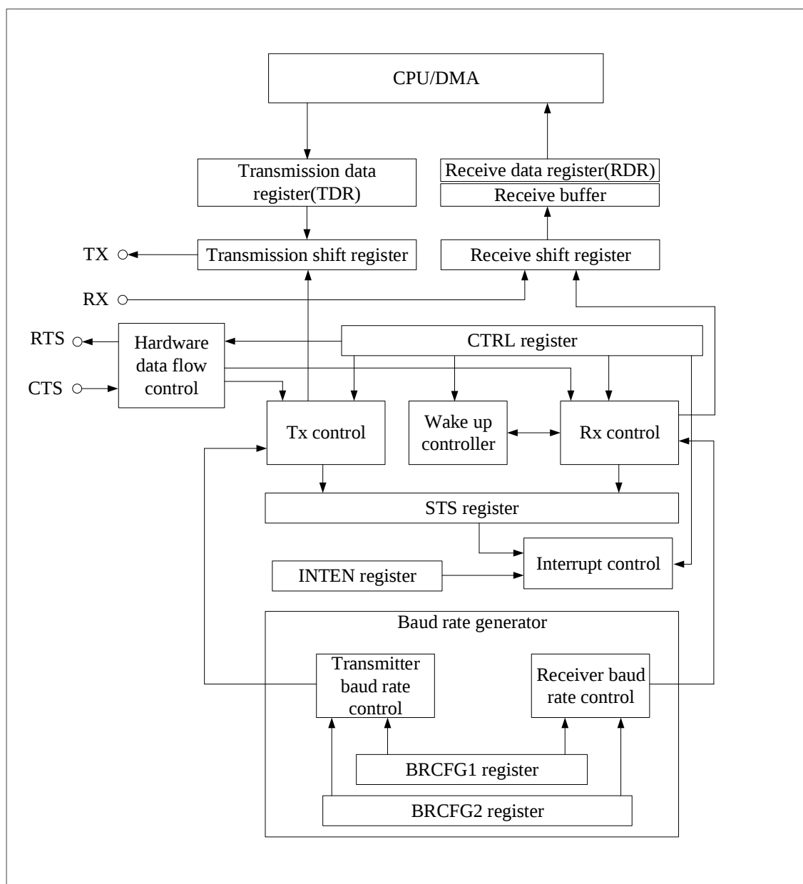
图 25-1 LPUART 框图
