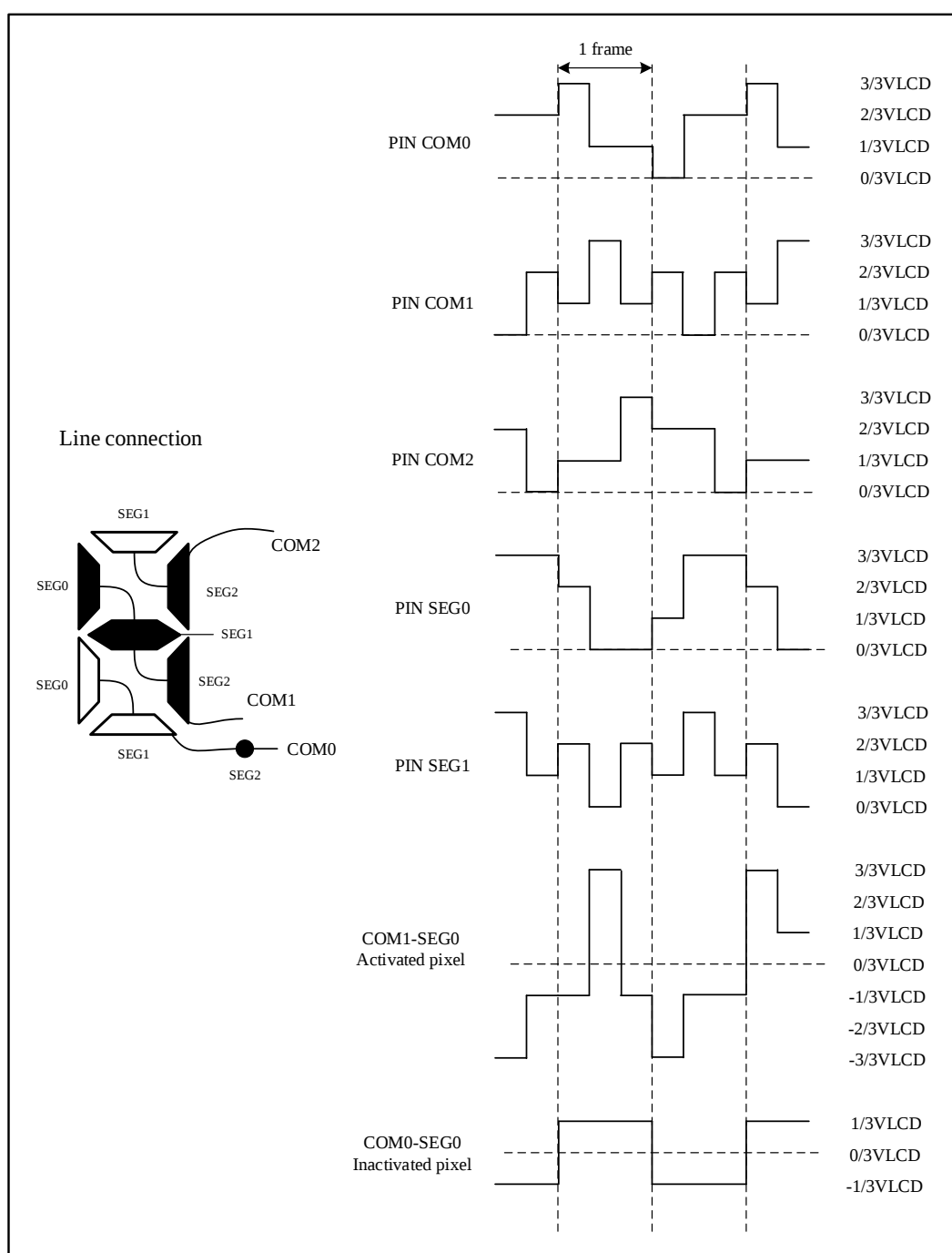
图 22-5 1/3 占空比, 1/3 偏置
