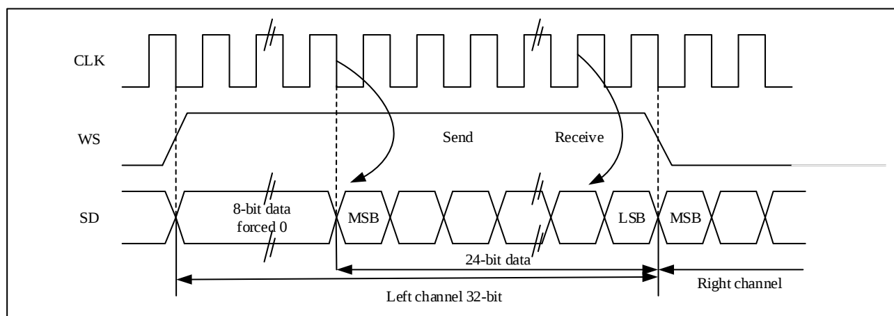
图 26-21 LSB 对齐 24 位数据，CLKPOL = 0
