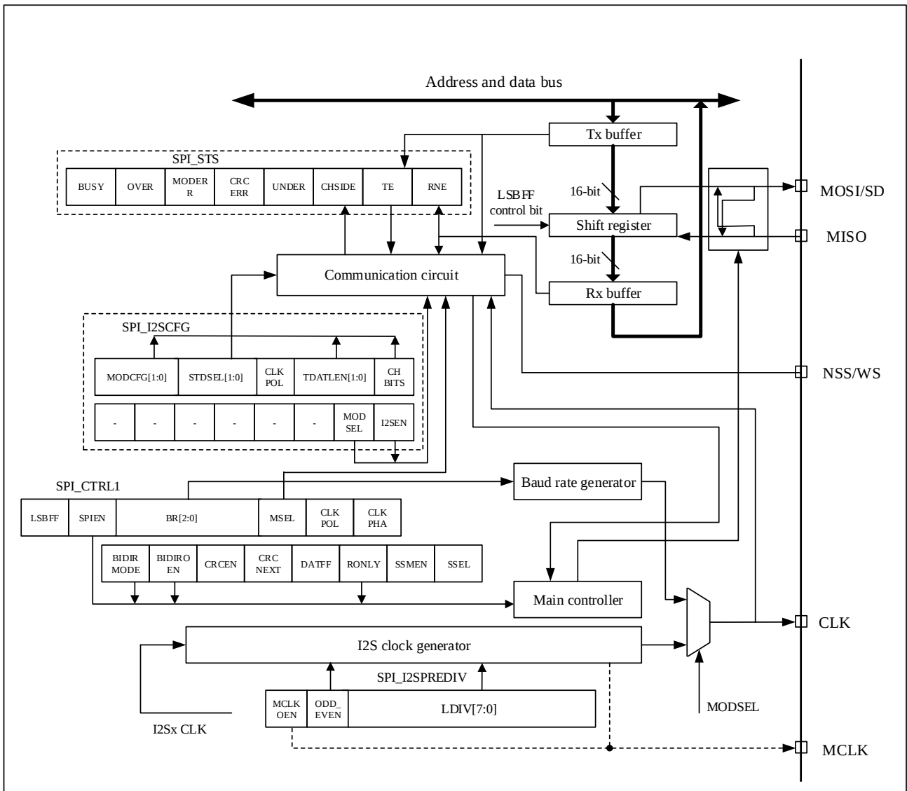
图 26-13 I 2 S 框图
