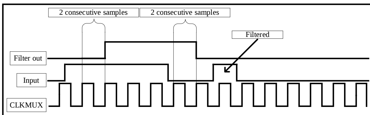
图 13-2 毛刺滤波器时序图
