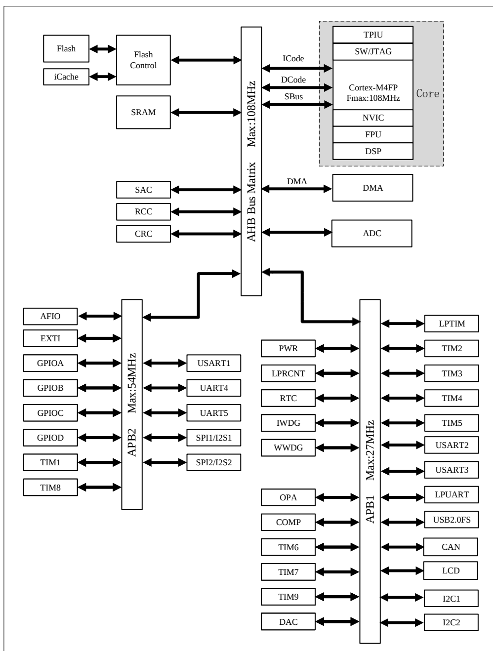
图 2-1 总线架构图
