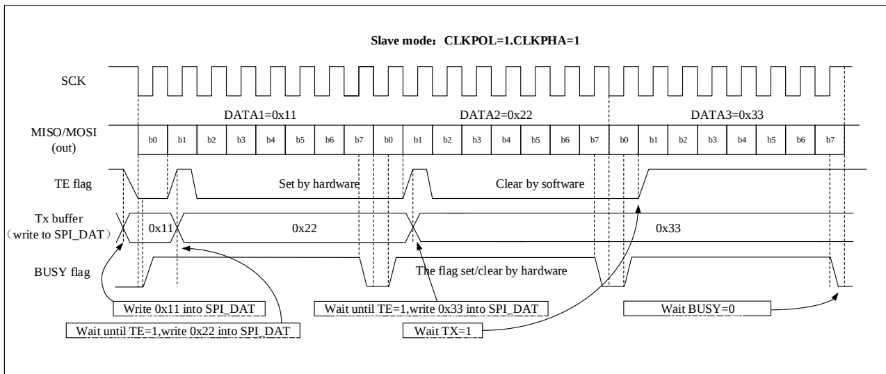
图 26-9 从机单向只发送模式下连续传输时，SPI_STS.TE/BUSY 变化示意图
