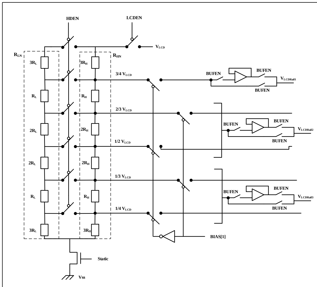
图 22-8 LCD 驱动电压控制
