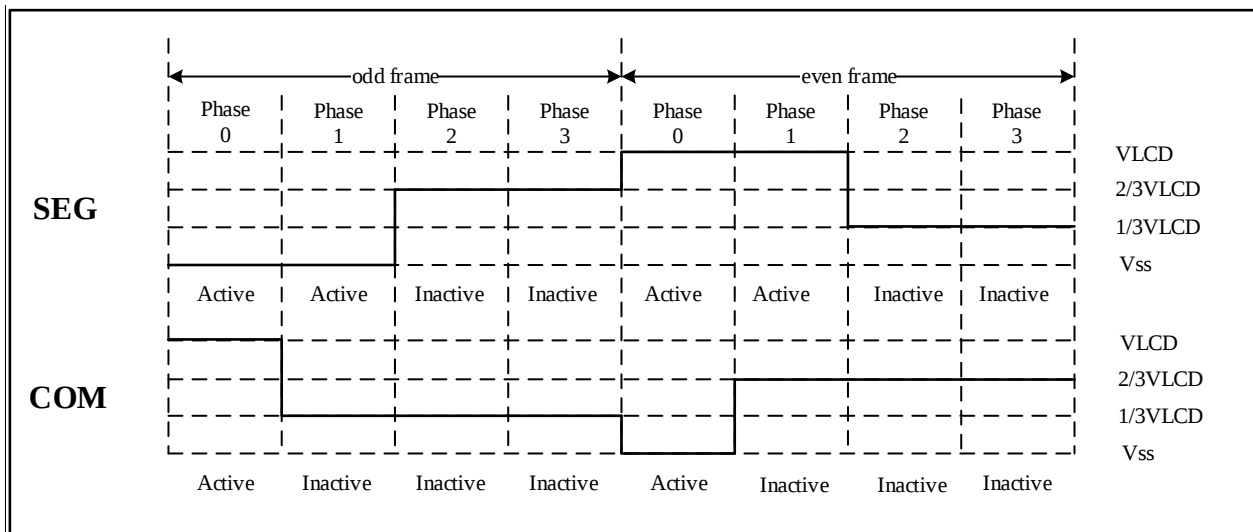
图 22-2 奇偶帧示例图（1/4 占空比，1/3 偏置）
