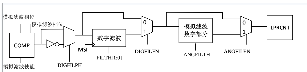
图 21-3 LPRCNT 模块比较器滤波框图
