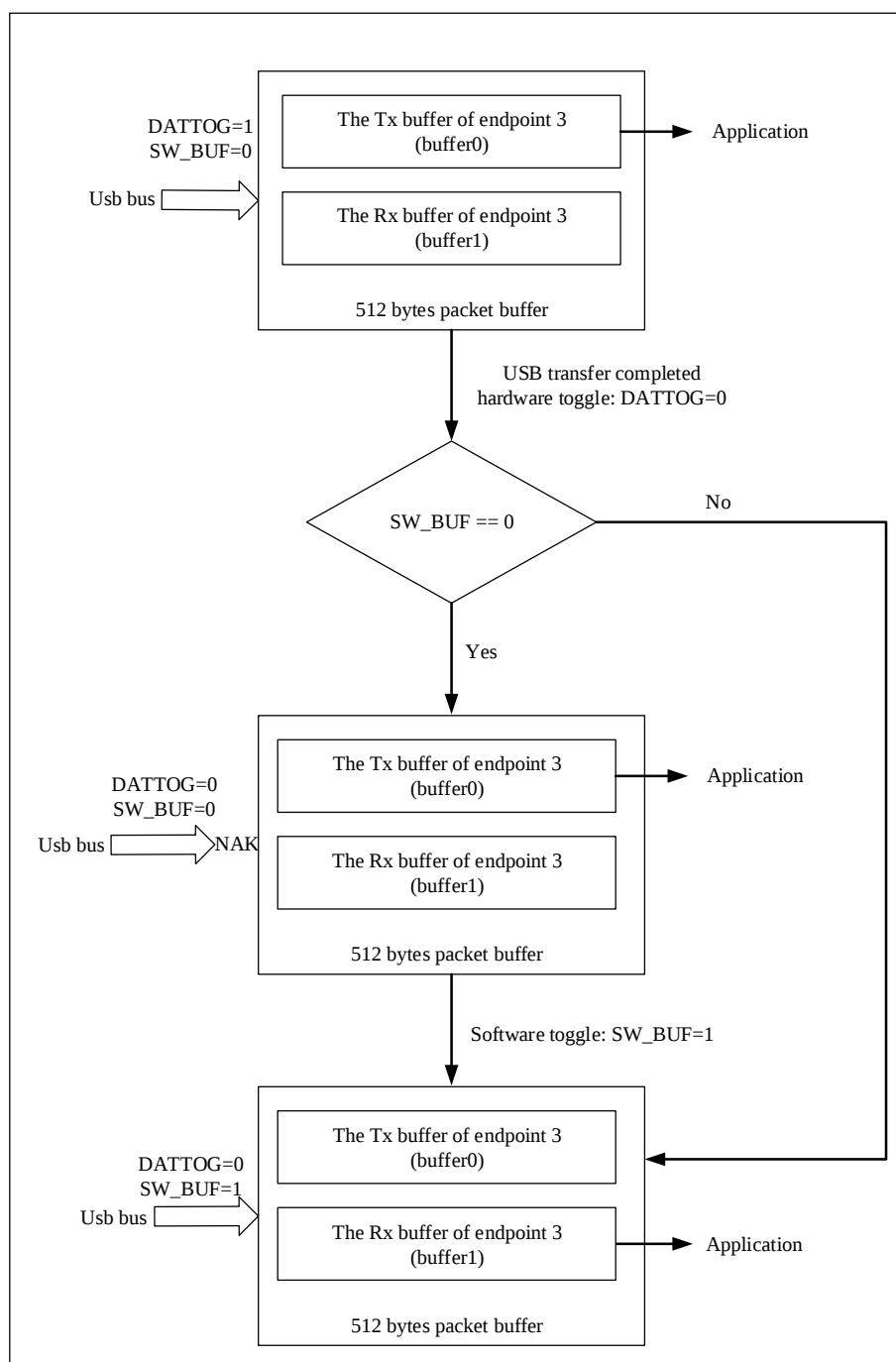
图 28-4 双缓冲批量端点示例
