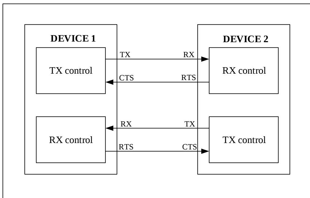
图 25-7 两个 LPUART 间的硬件流控制
