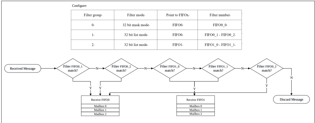
图 27-10 过滤机制示例
