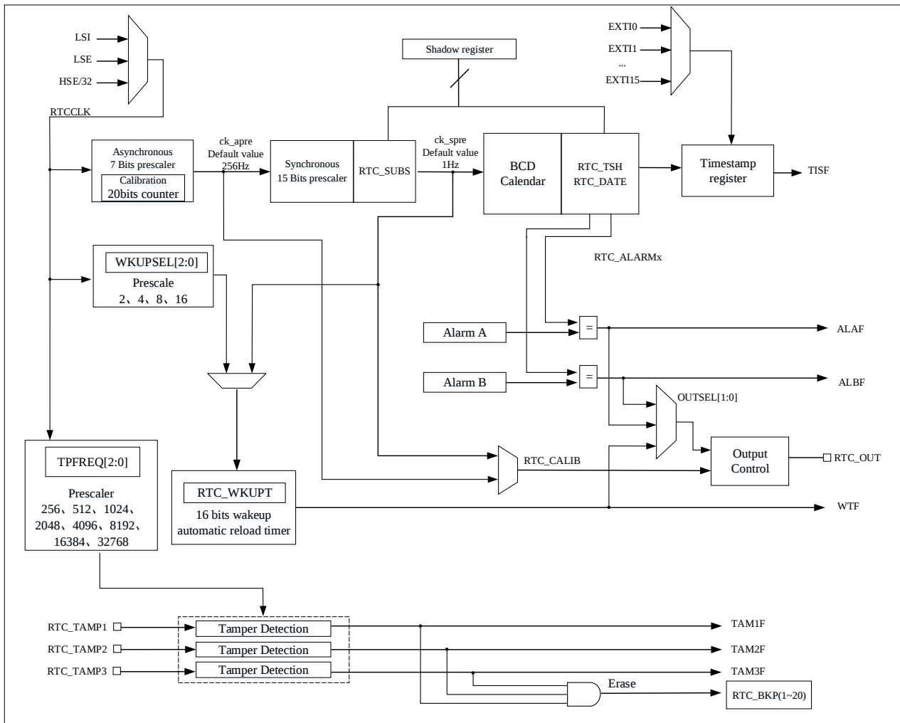
图 14-1 RTC 框图
