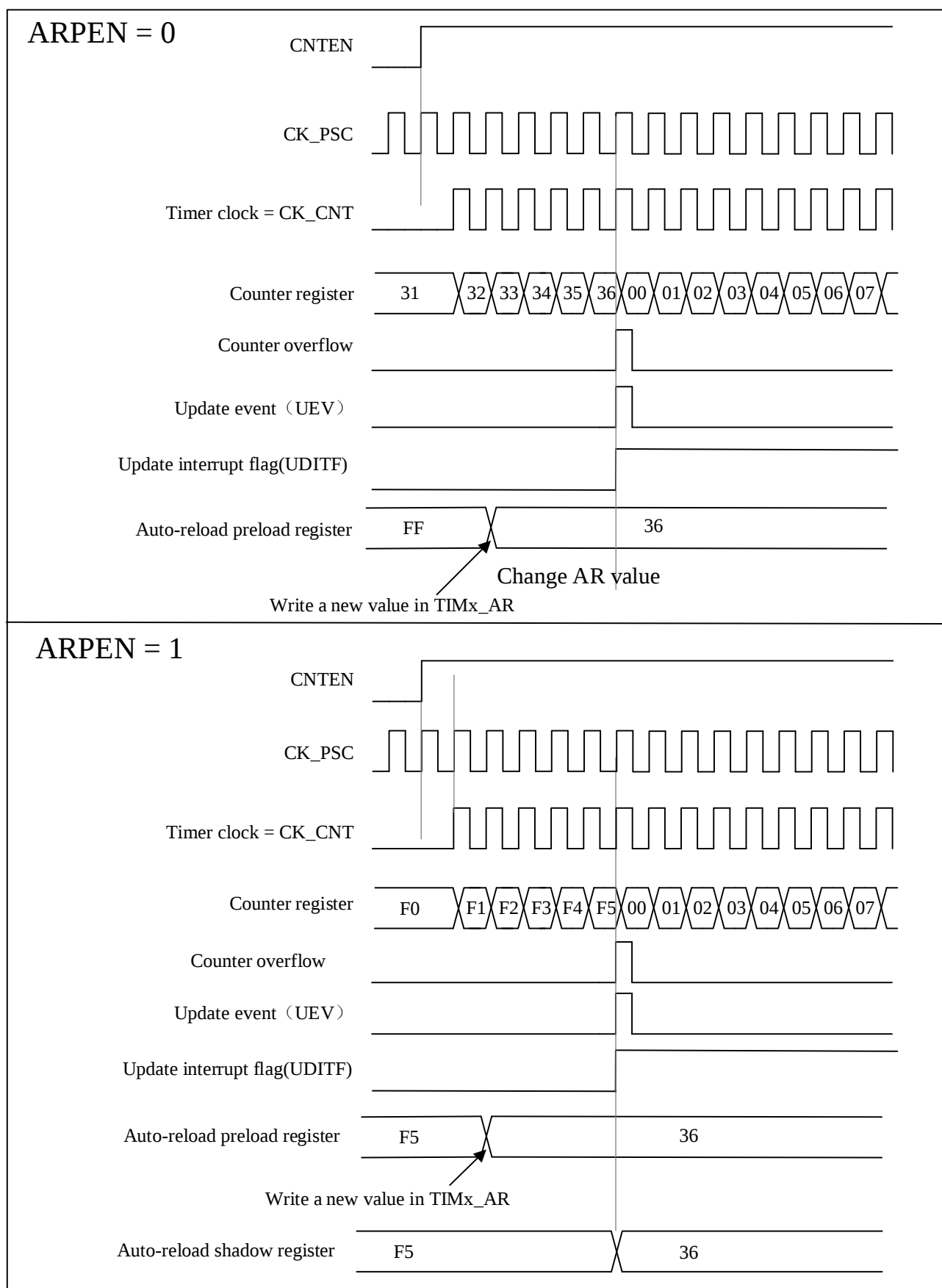
图 12-4 ARPEN=0/1 时向上计数、更新事件的时序图
