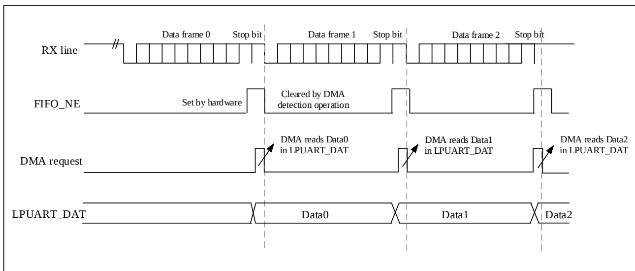
图 25-6 利用 DMA 接收
