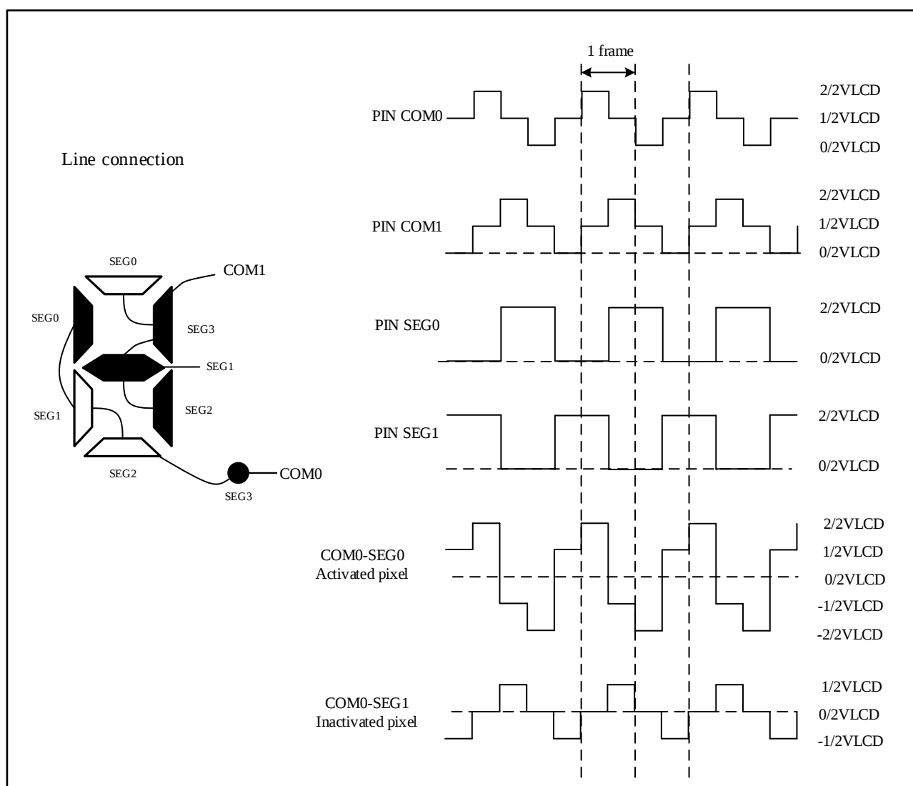
图 22-4 1/2 占空比, 1/2 偏置
