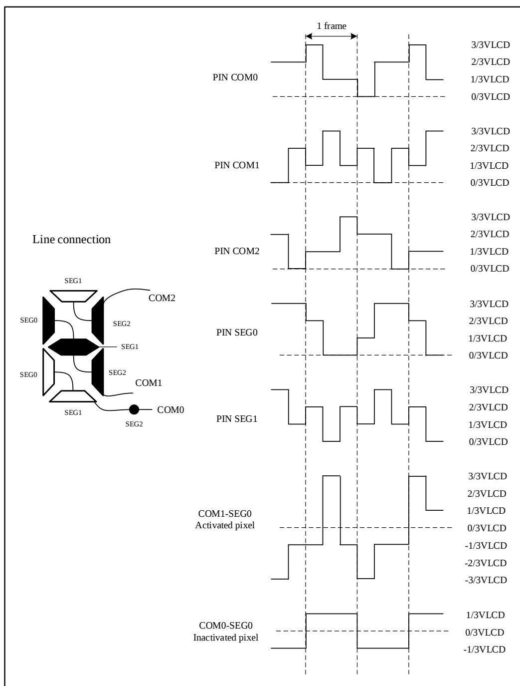
图 22-6 1/4 占空比, 1/3 偏置
