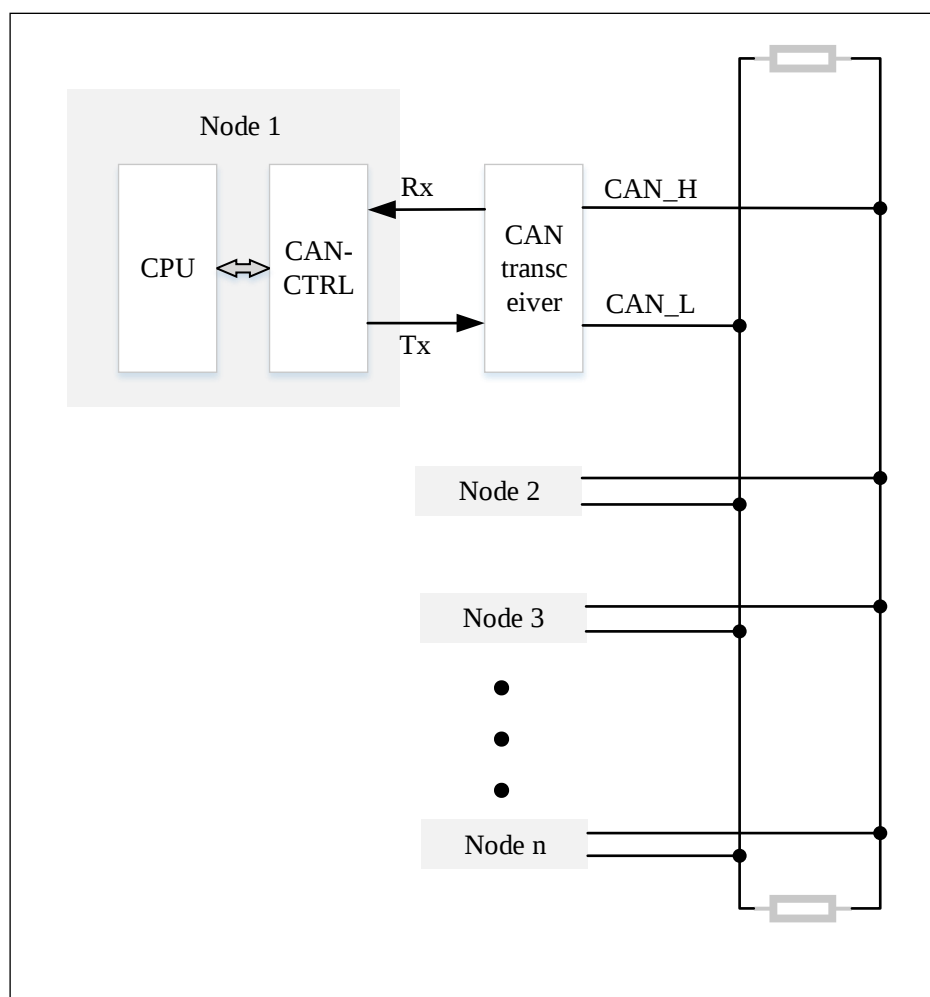
图 27-1 CAN 网络拓扑
