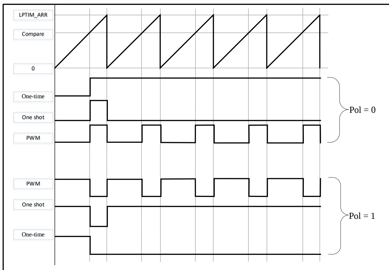
图 13-6 波形发生器
