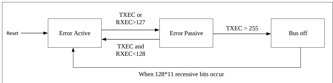
图 27-14 CAN 错误状态框图
