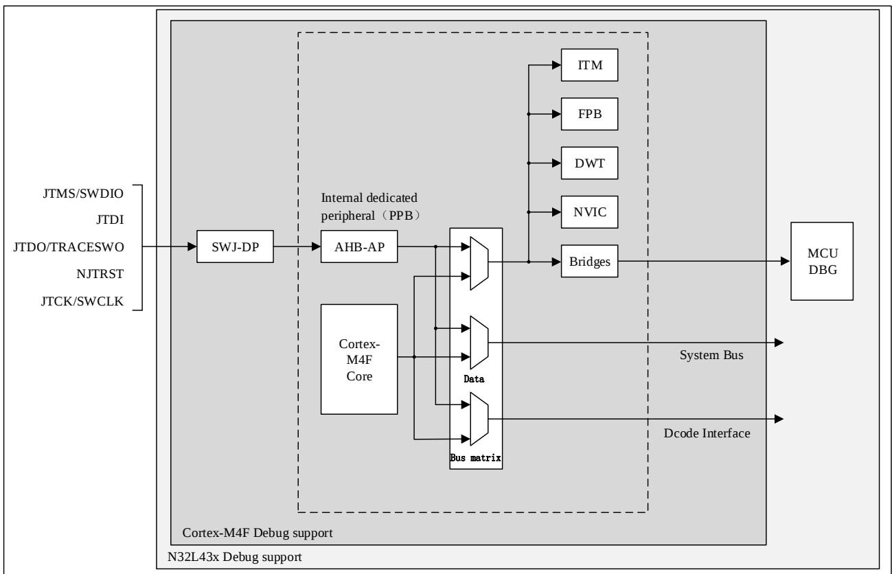
图 29-1 N32L43x 级和 Cortex™-M4F 级调试框图
