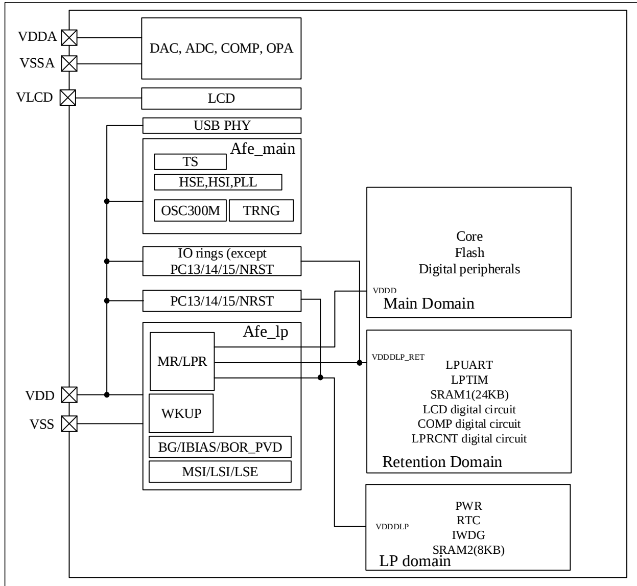
图 3-1 电源框图
