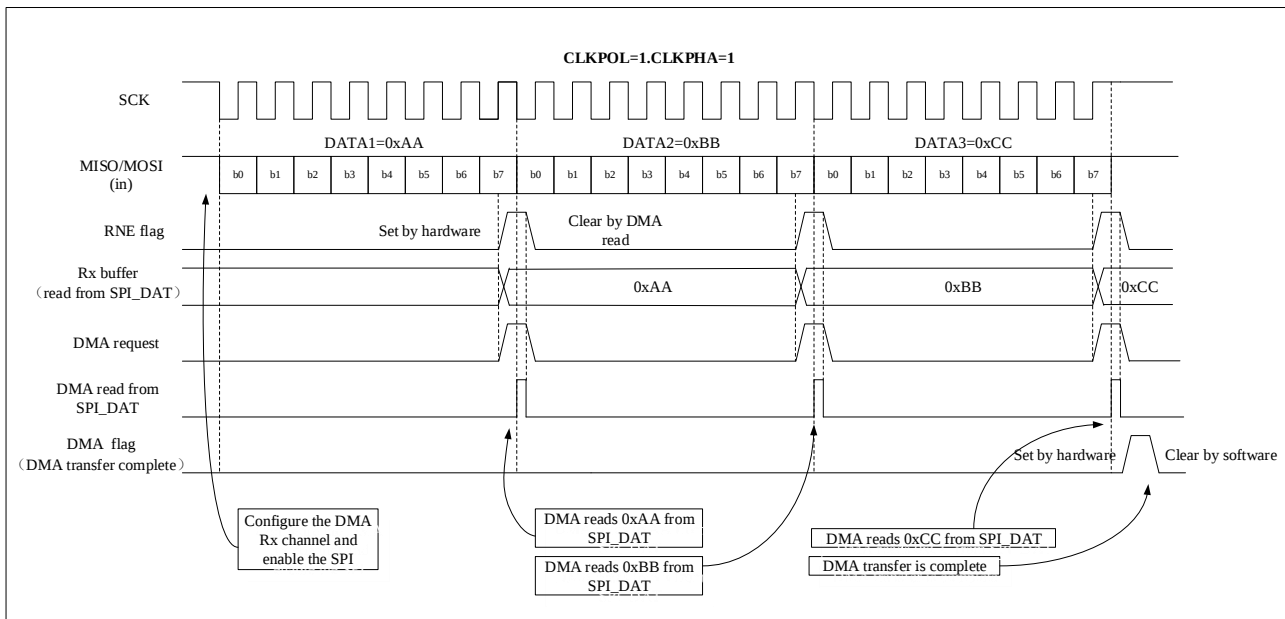
图 26-12 使用 DMA 接收
