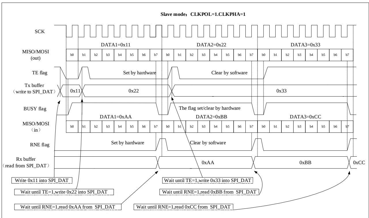
图 26-8 从机全双工模式下连续传输时，SPI_STS.TE/RNE/BUSY 的变化示意图
