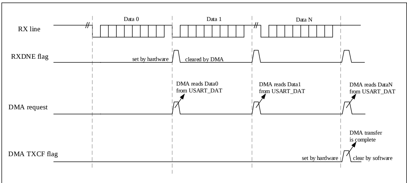
图 24-9 DMA 接收
