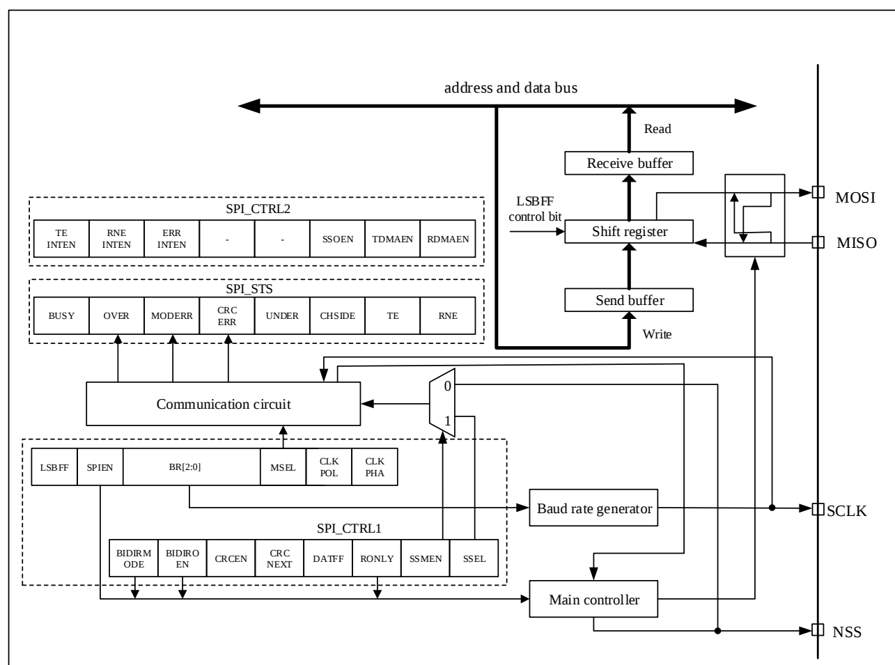
图 26-1 SPI 框图
