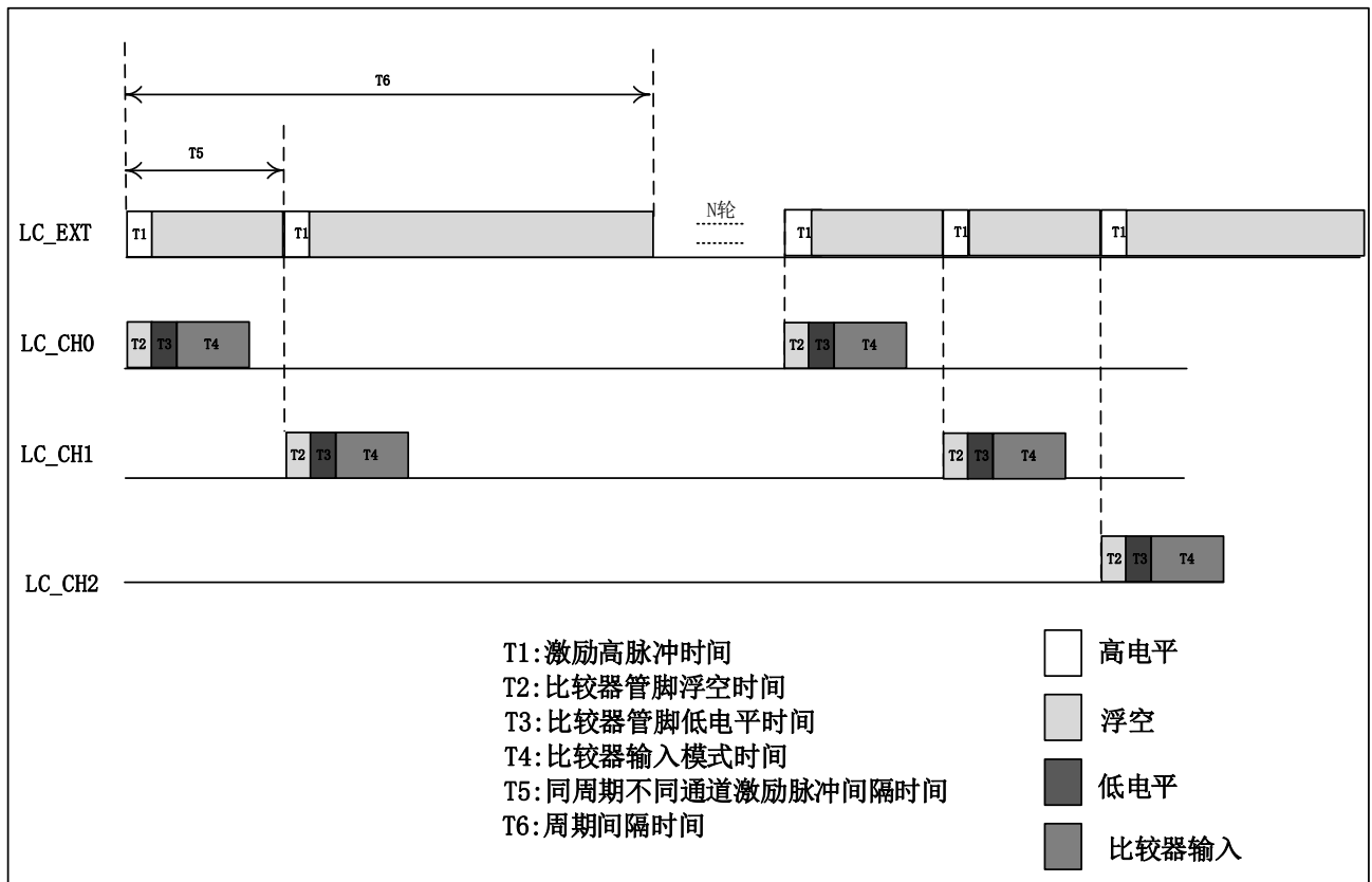
图 21-5 三路 LC 工作时序图
