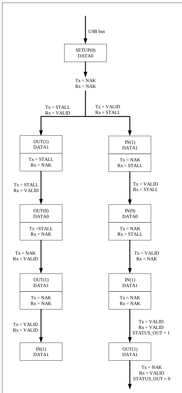
图 28-5 控制传输
