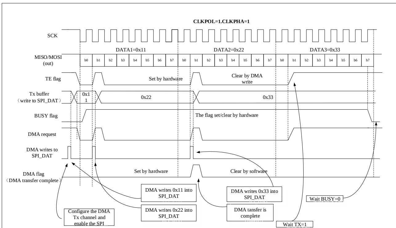
图 26-11 使用 DMA 发送
