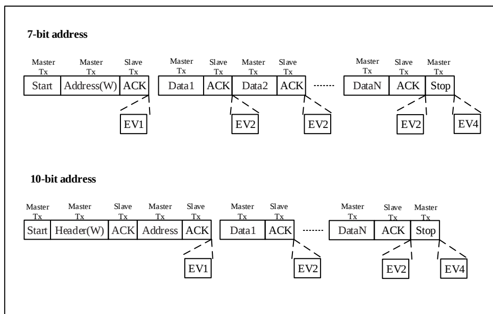
图 23-4 从机接收器传送序列
