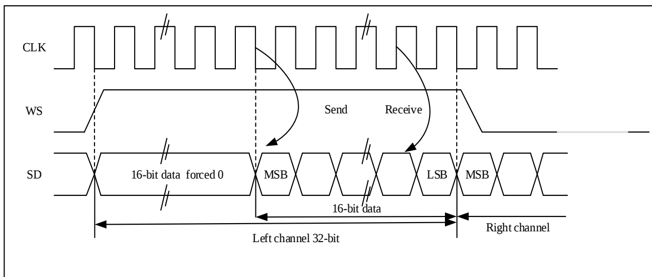
图 26-22 LSB 对齐 16 位数据扩展到 32 位包帧，CLKPOL = 0
