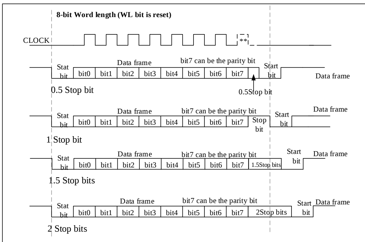
图 24-4 停止位配置
