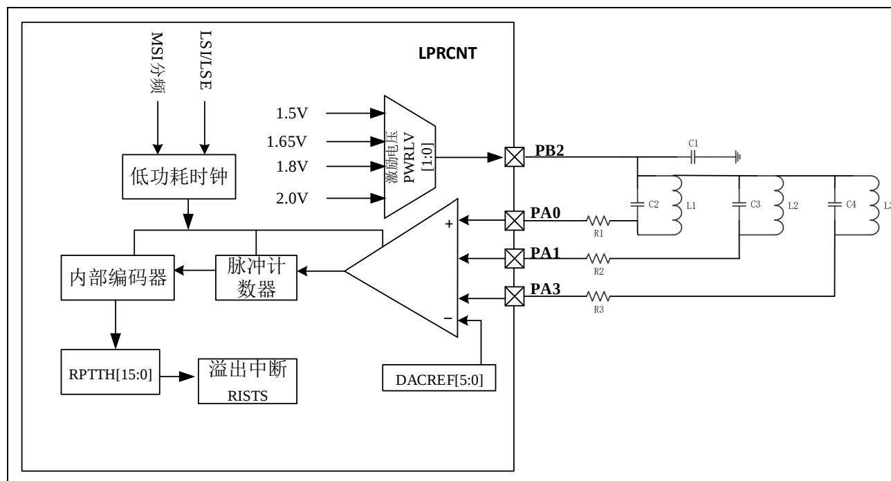
图 21-1 LPRCNT 框图
