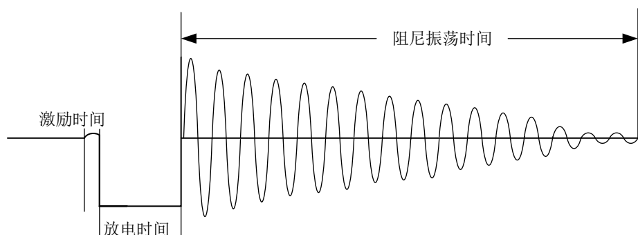
图 21-4 LC 阻尼振荡过程
