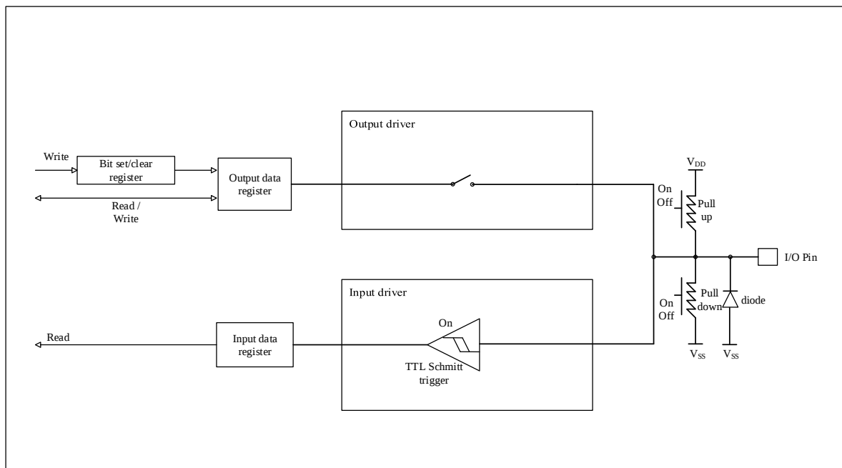
图 5-2 输入浮空/上拉/下拉配置
