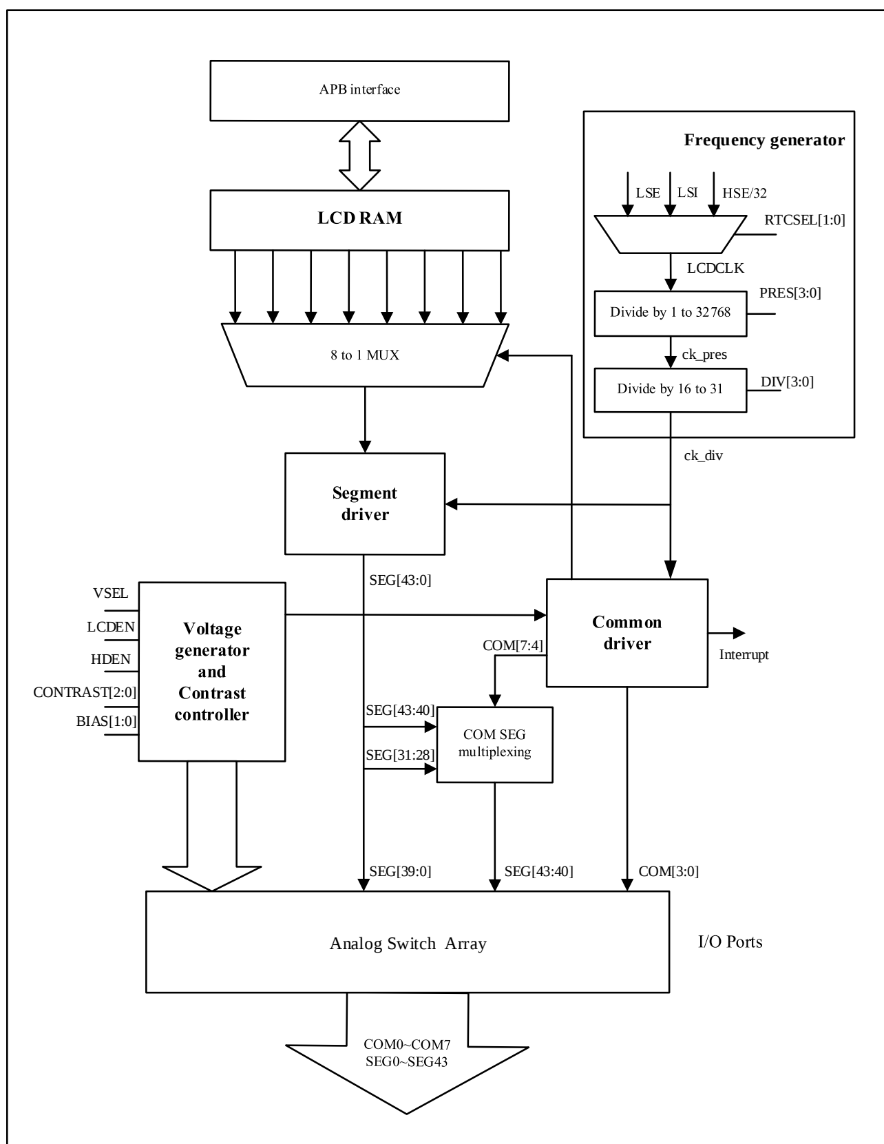
图 22-1 LCD 控制器框图
