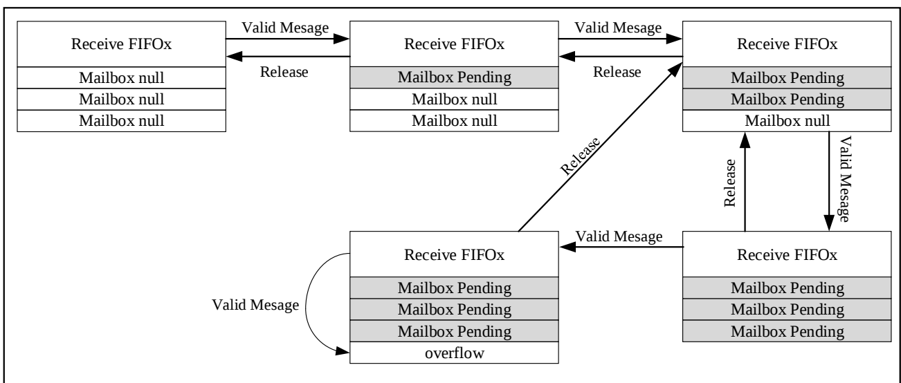
图 27-8 接收邮箱状态
