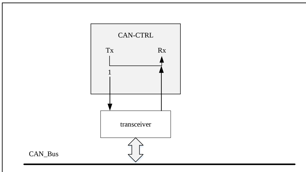
图 27-5 静默模式
