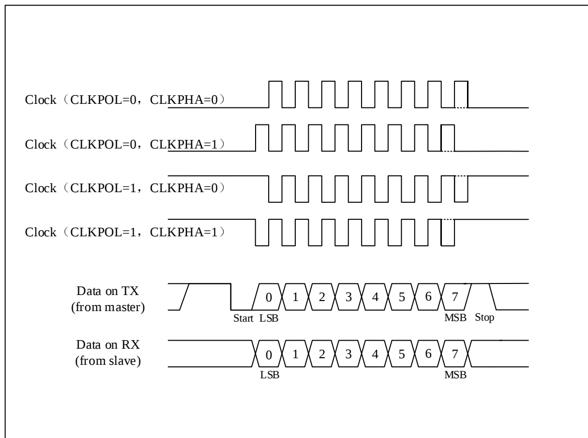
图 24-16 USART 数据时钟时序示例 (WL=0)
