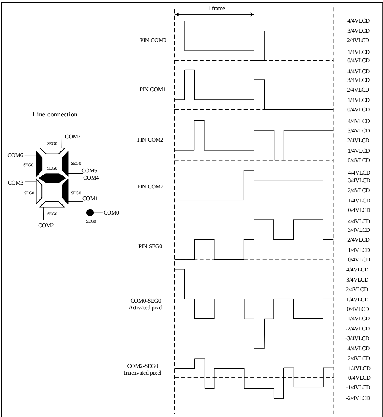
图 22-7 1/8 占空比, 1/4 偏置
