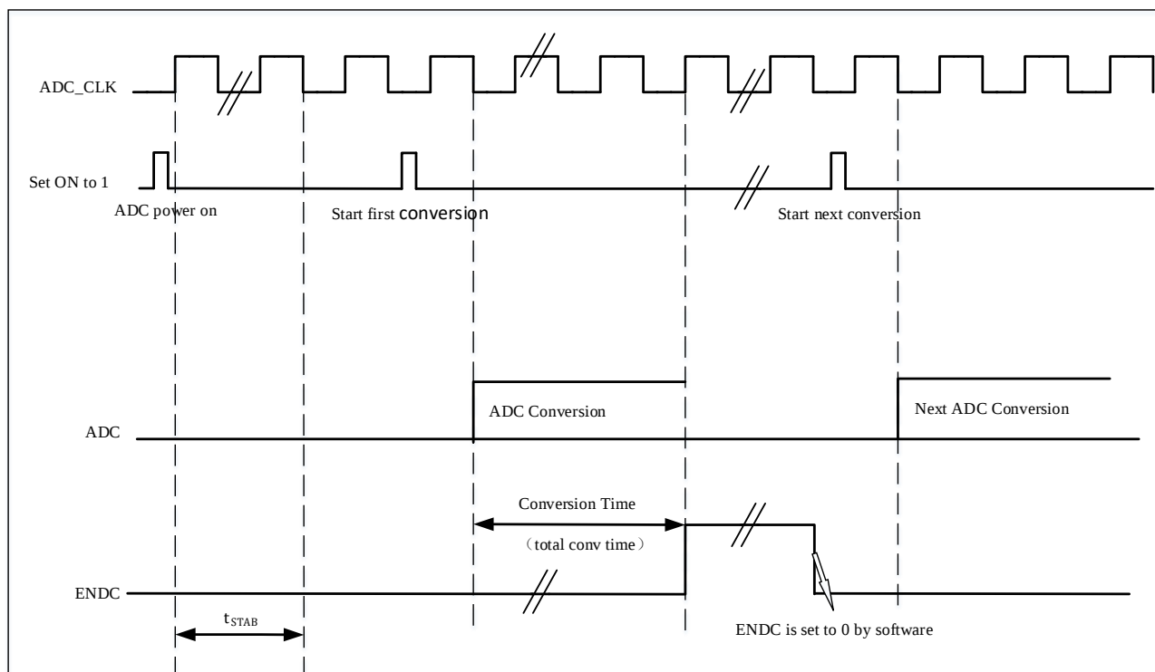
图 17-4 时序图
