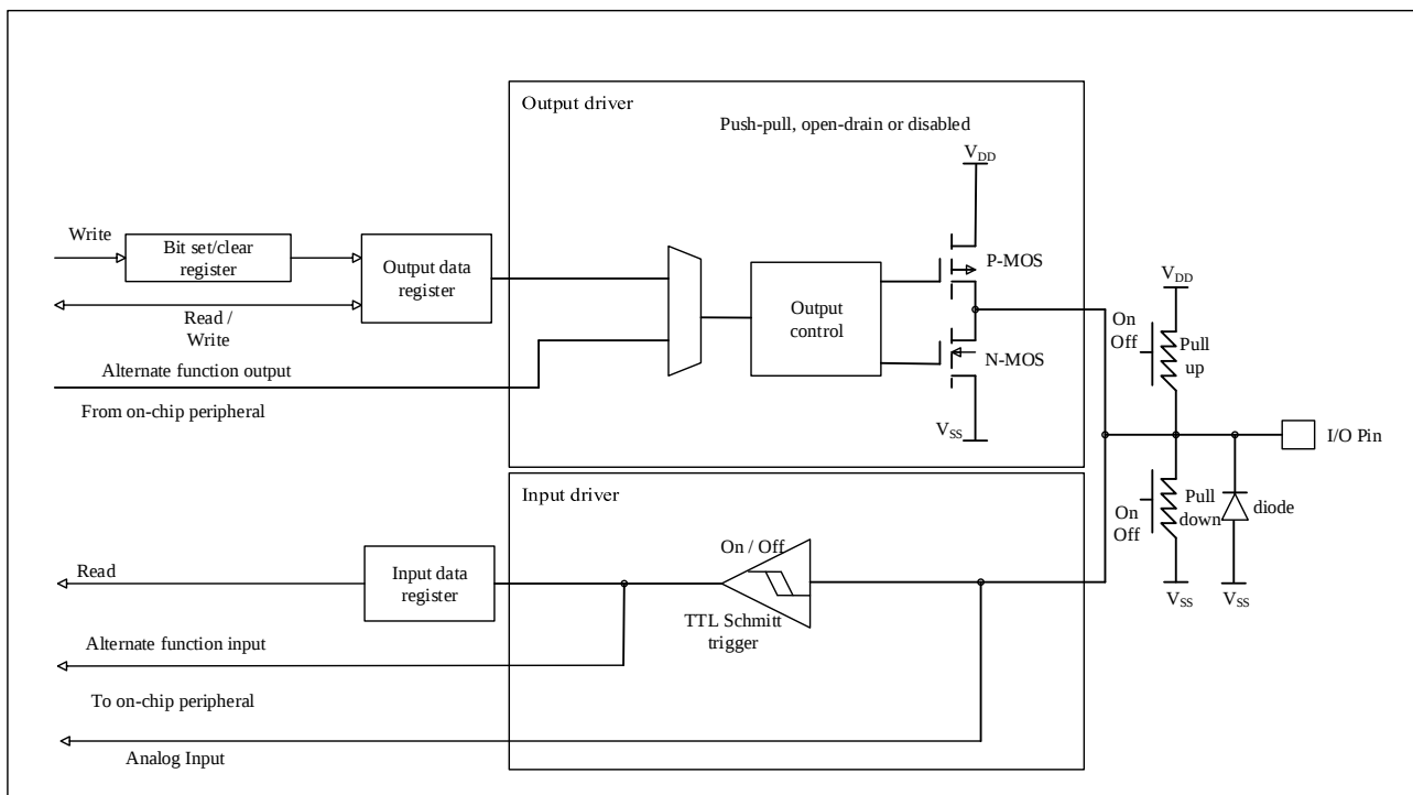
图 5-1 I/O 端口的基本结构
