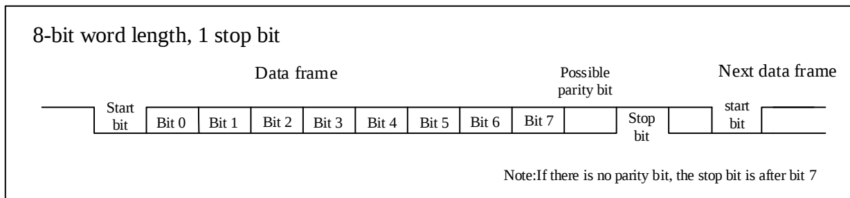
图 25-2 帧格式
