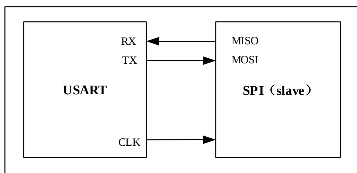
图 24-15 USART 同步传输示例
