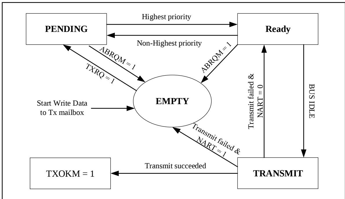
图 27-7 发送邮箱状态
