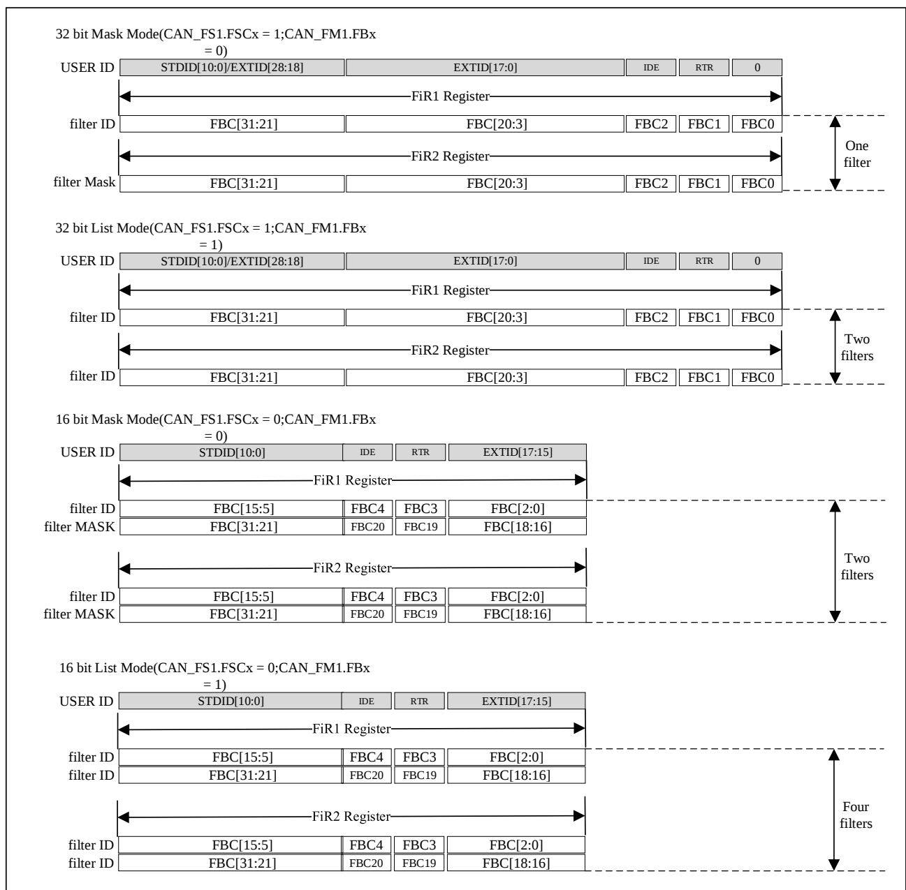
图 27-9 过滤器位宽设置-寄存器组织
