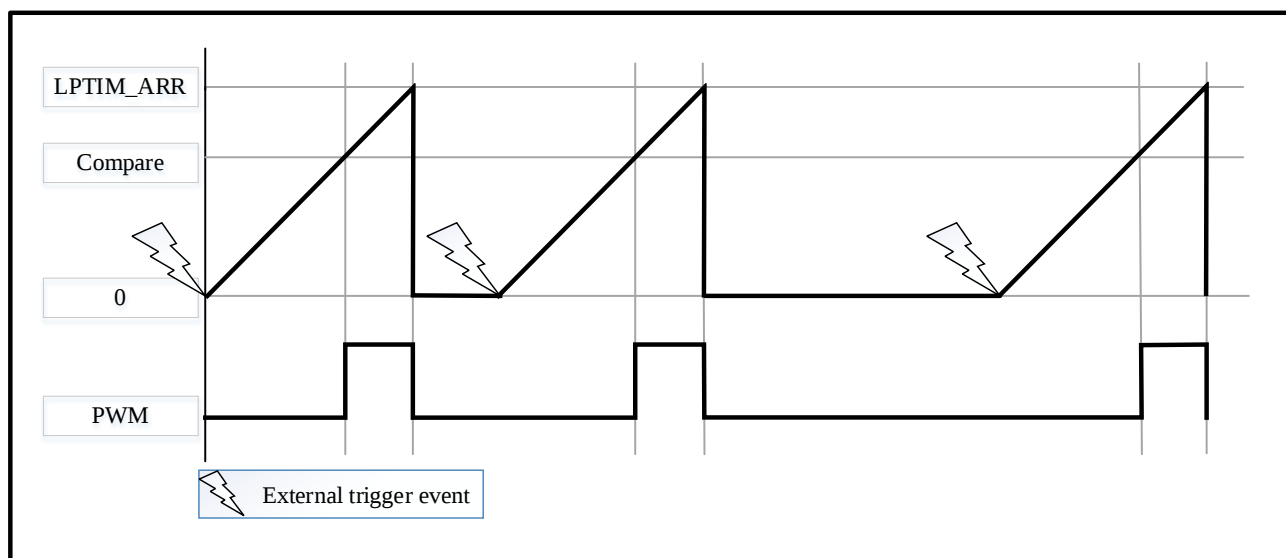
图 13-13-4 LPTIM 输出波形，单触发计数模式配置
