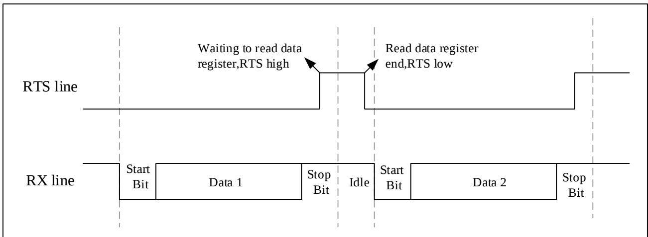
图 25-8 RTS 流控制
