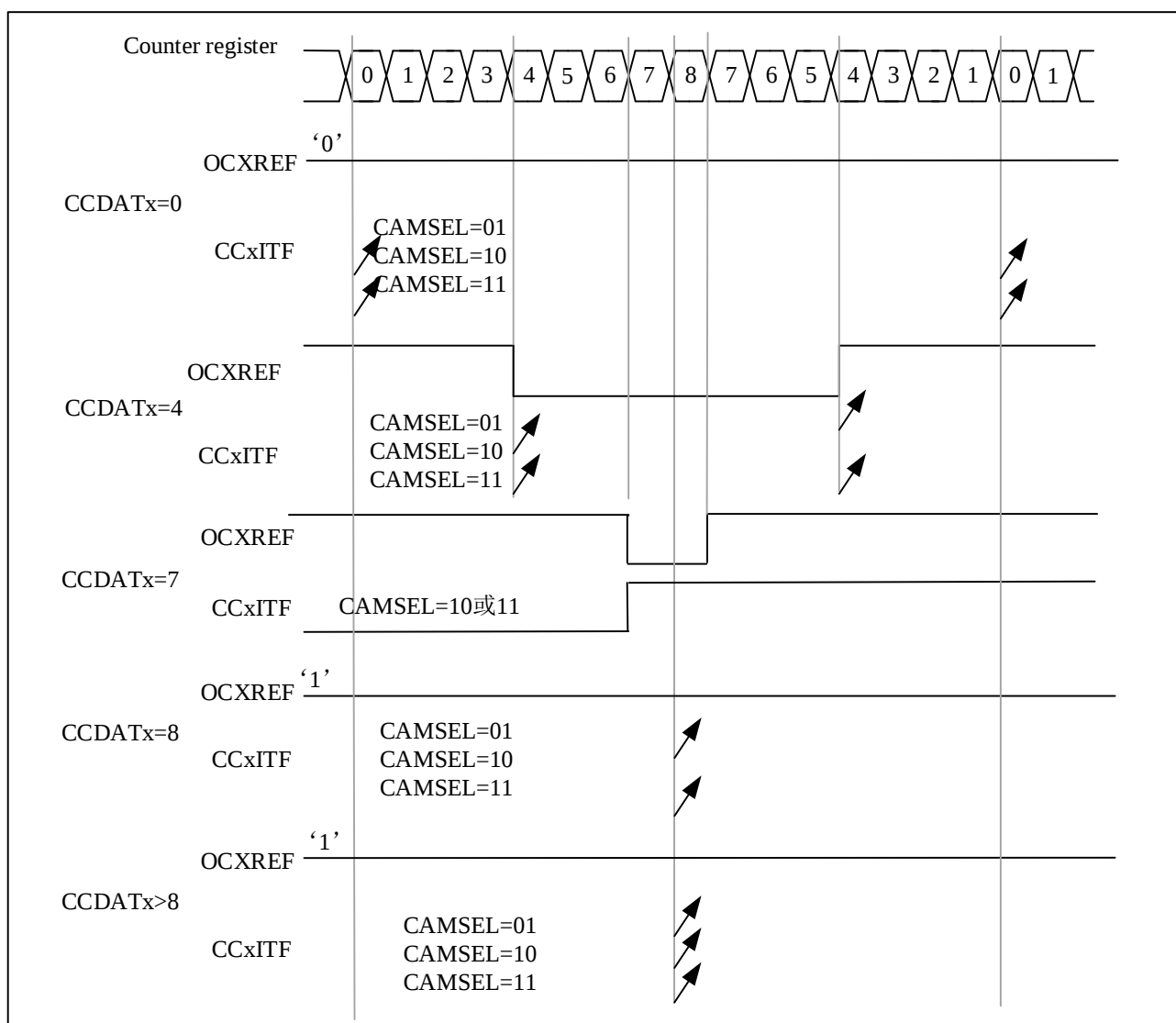
图 10-22 中央对齐的 PWM 波形(AR=8)
