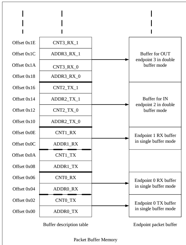
图 28-3 缓冲区描述表和端点数据包缓冲区的关系
