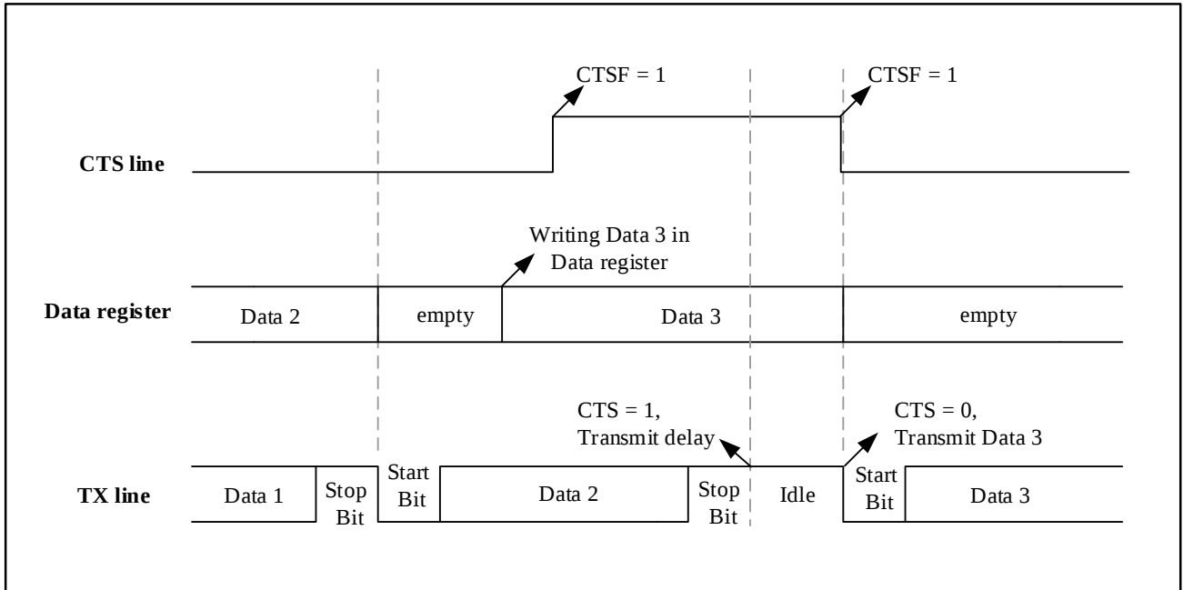
图 25-9 CTS 流控制
