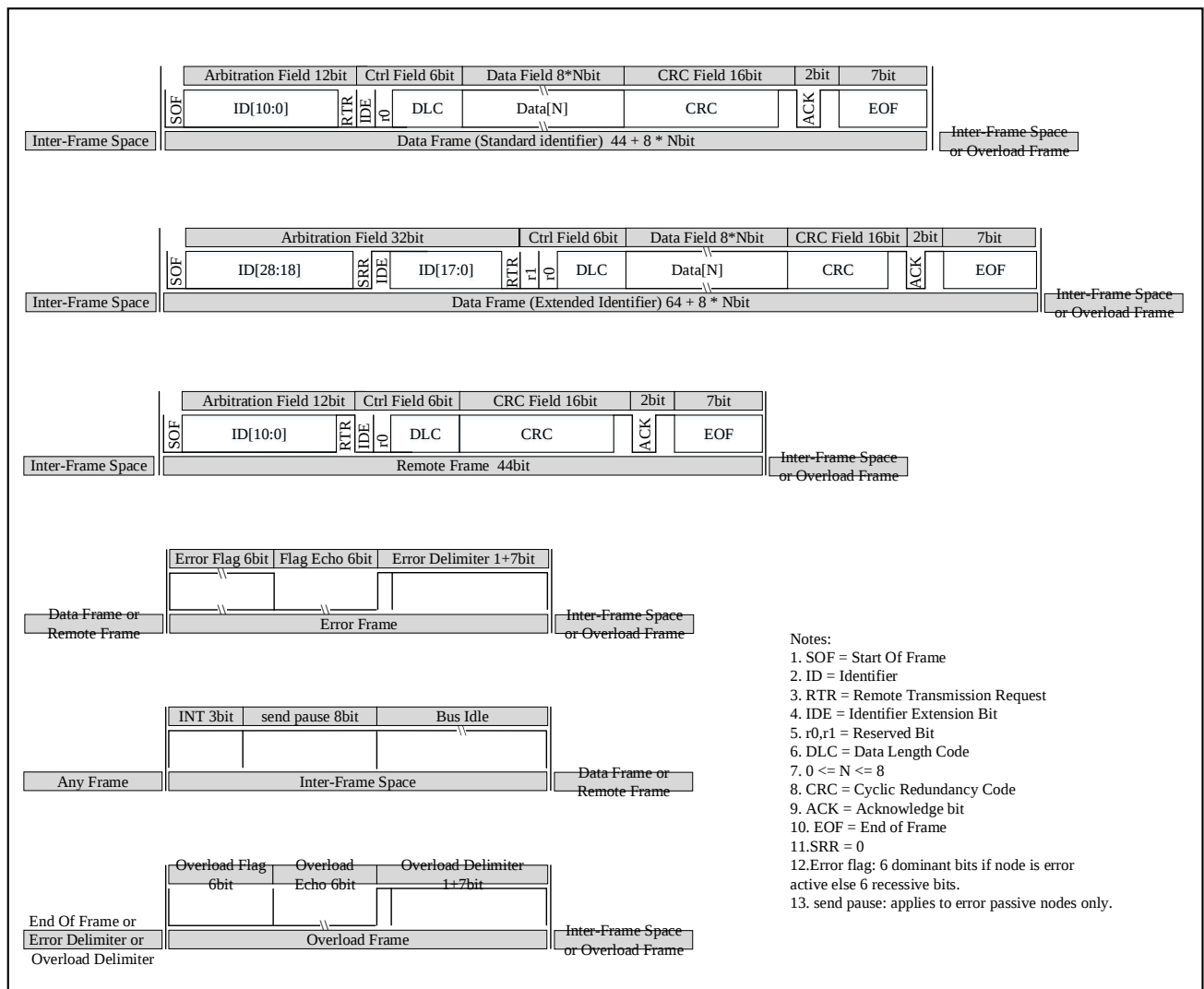
图 27-12 各类帧格式
