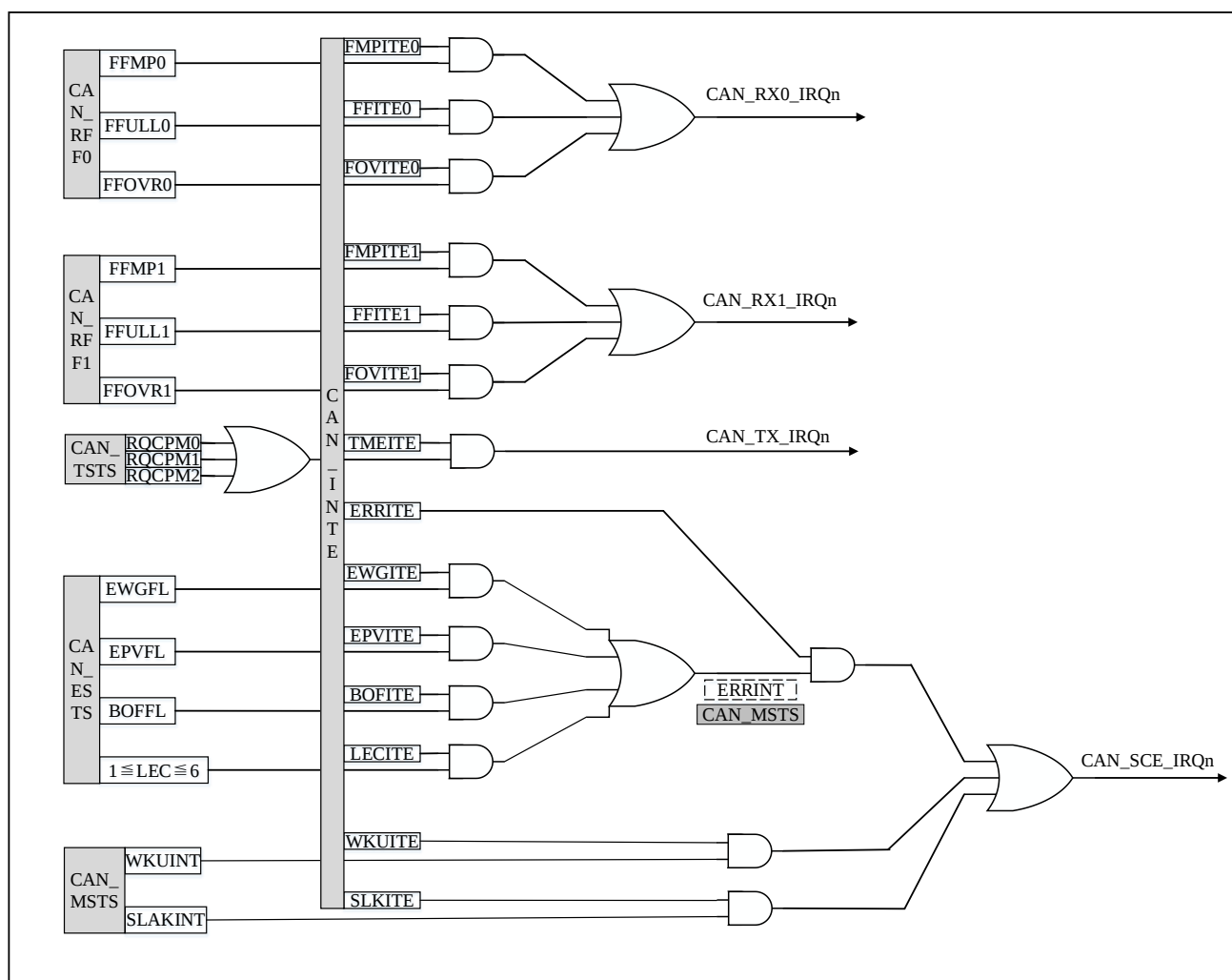
图 27-13 事件标志和中断产生
