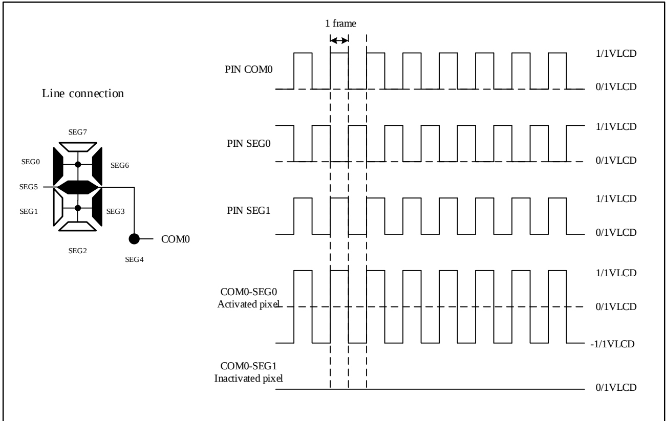
图 22-3 静态占空比示例
