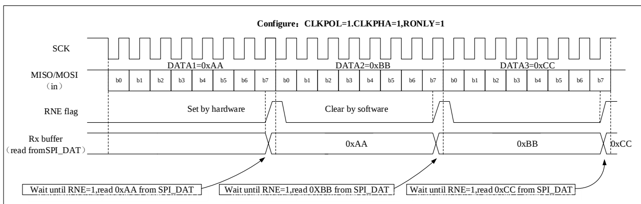
图 26-7 只接收模式（BIDIRMODE = 0 并且 ONLY = 1）下连续传输时，RNE 变化示意图
