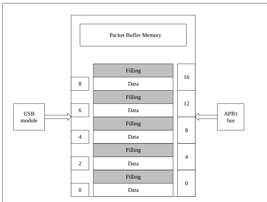
图 28-2 USB 模块和微控制器上的用户应用程序访问 Packet Buffer Memory 方式
