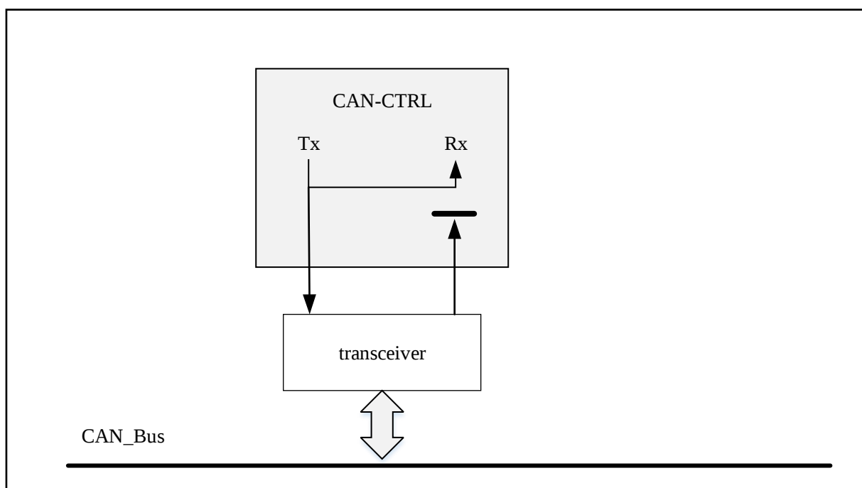
图 27-4 回环模式
