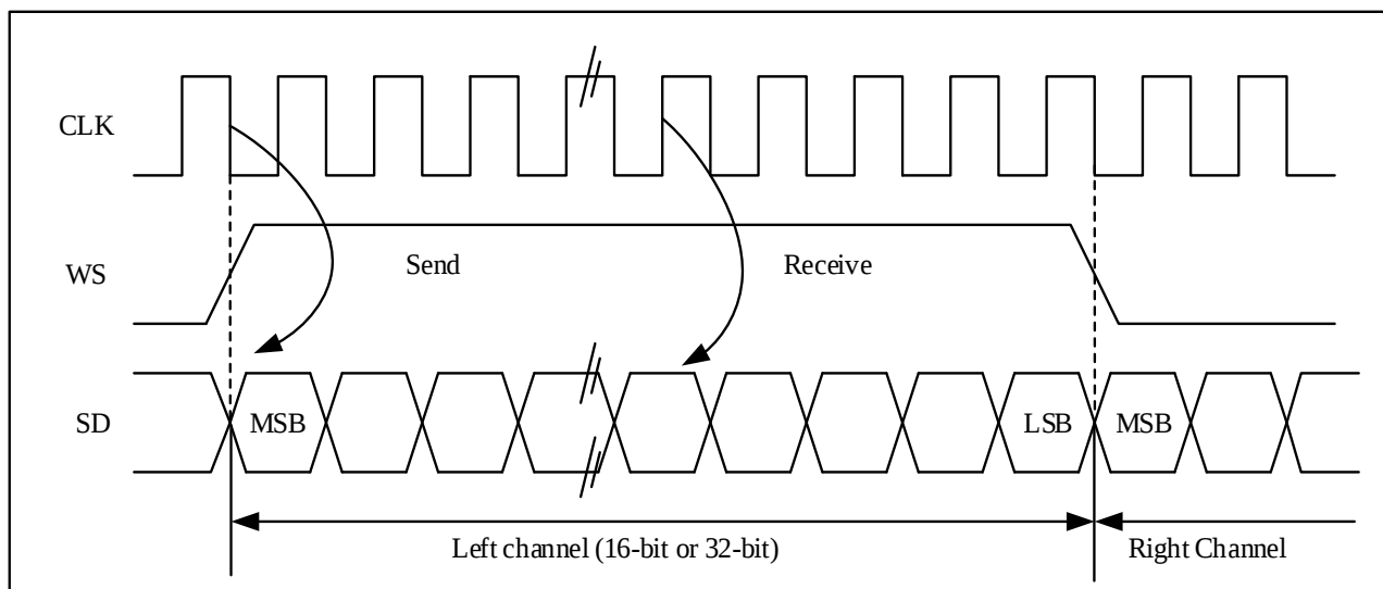
图 26-17 MSB 对齐 16 位或 32 位全精度，CLKPOL = 0
