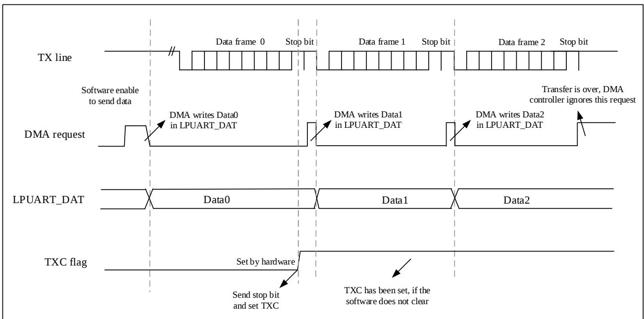
图 25-5 利用 DMA 发送
