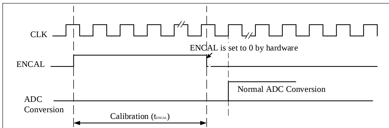
图 17-6 校准时序图
