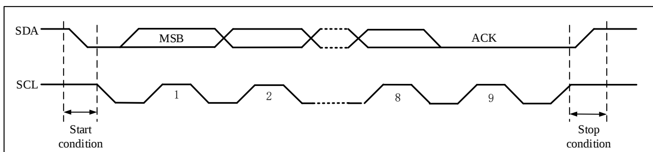
图 23-2 I 2 C 总线协议
