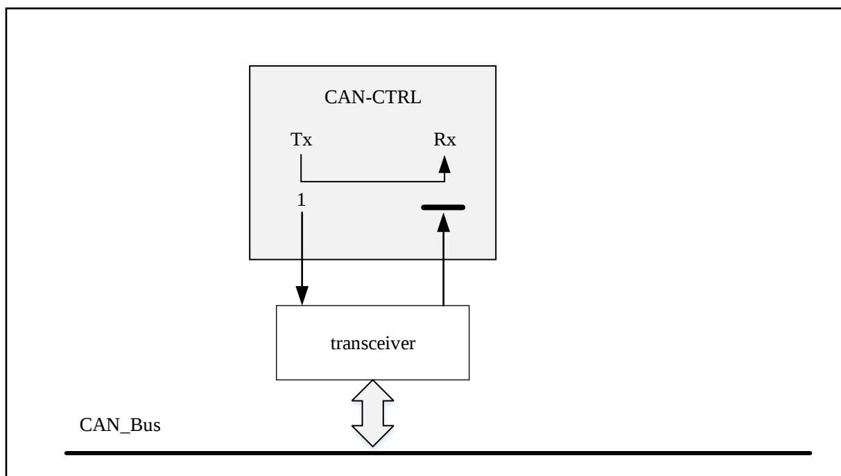
图 27-6 回环静默模式
