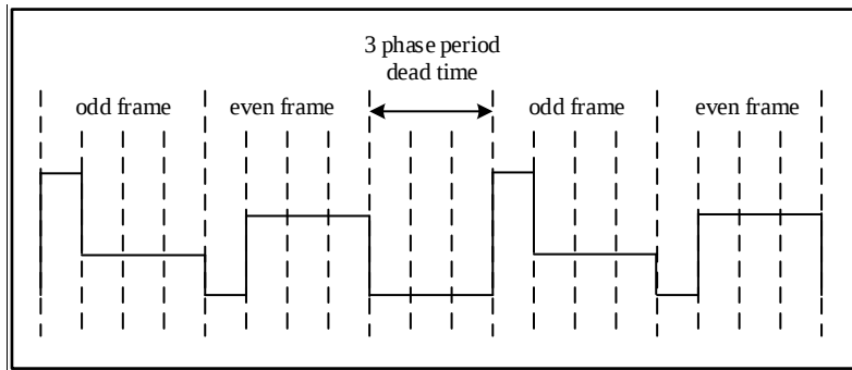
图 22-9 死区时间
