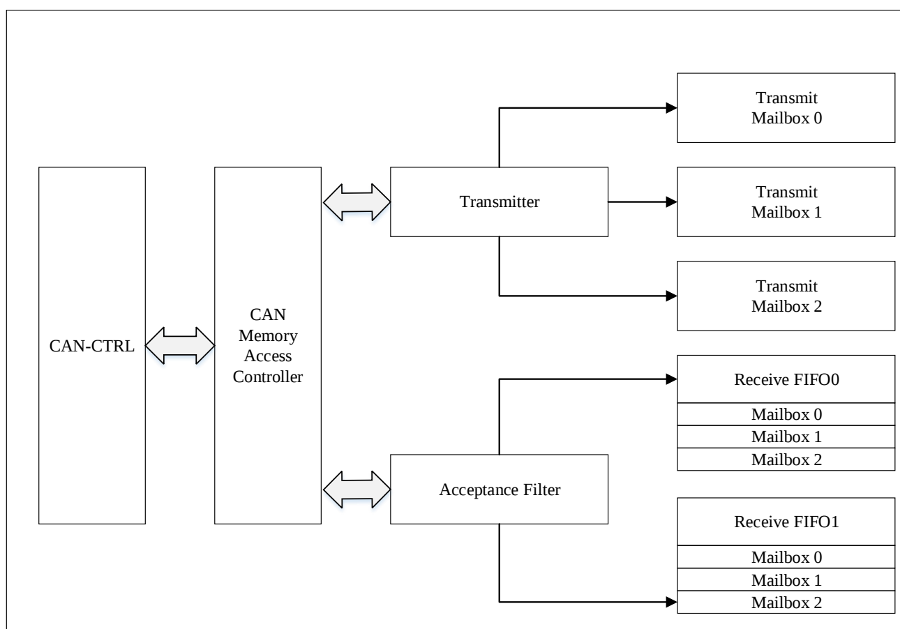
图 27-3 单 CAN 框图
