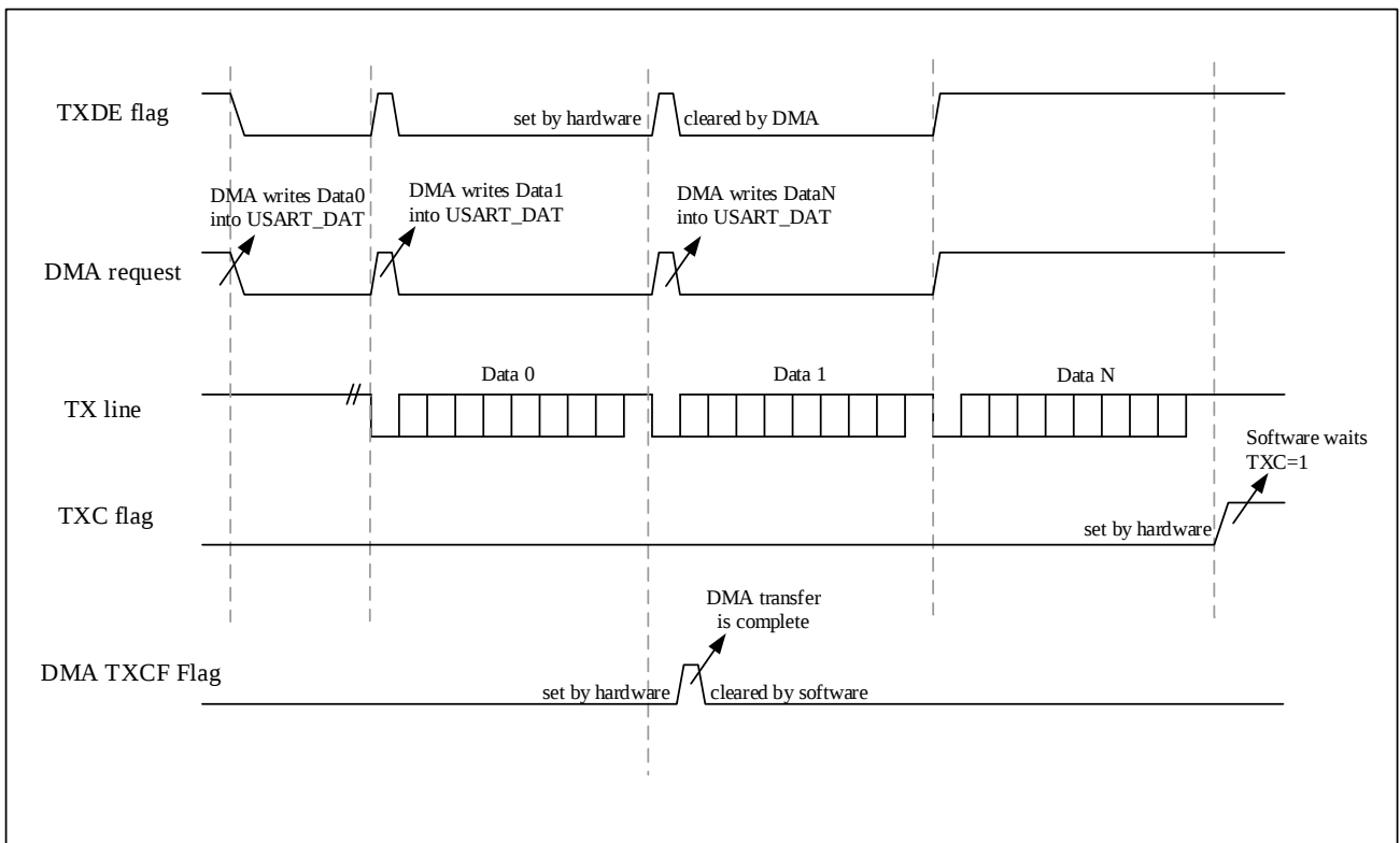
图 24-8 DMA 发送
