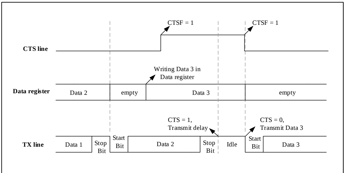
图 24-12 CTS 流控制
