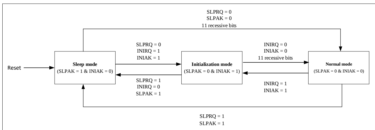
图 27-2 CAN 工作模式
