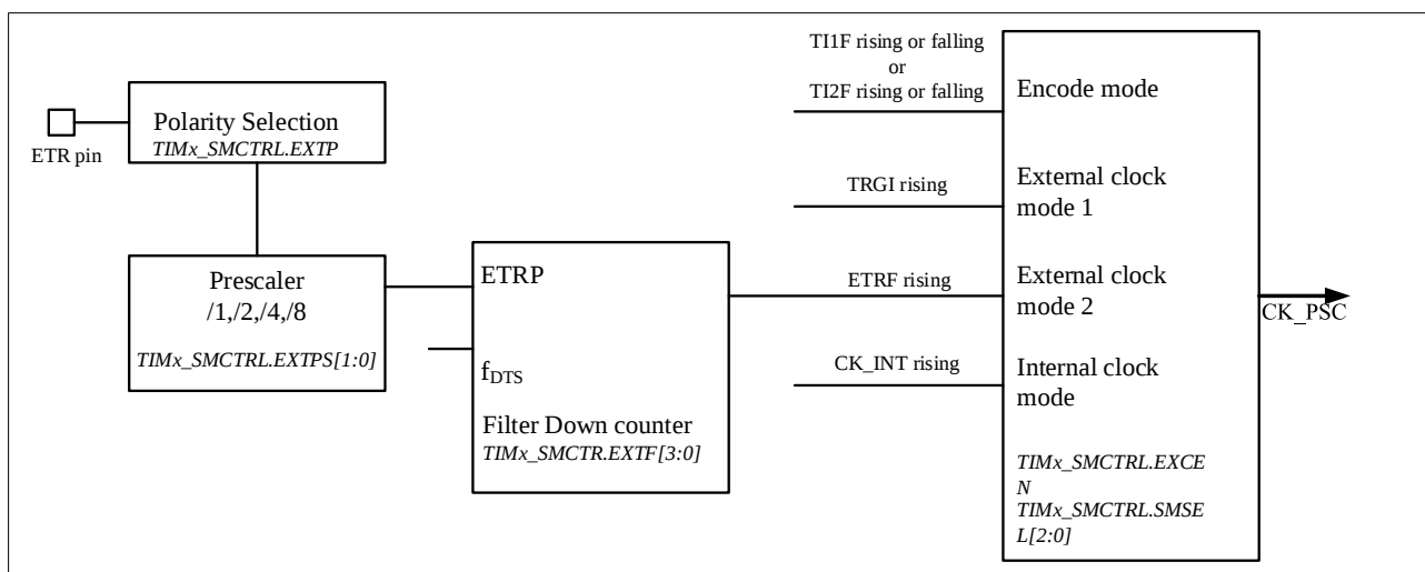
图 11-11 外部触发输入框图
