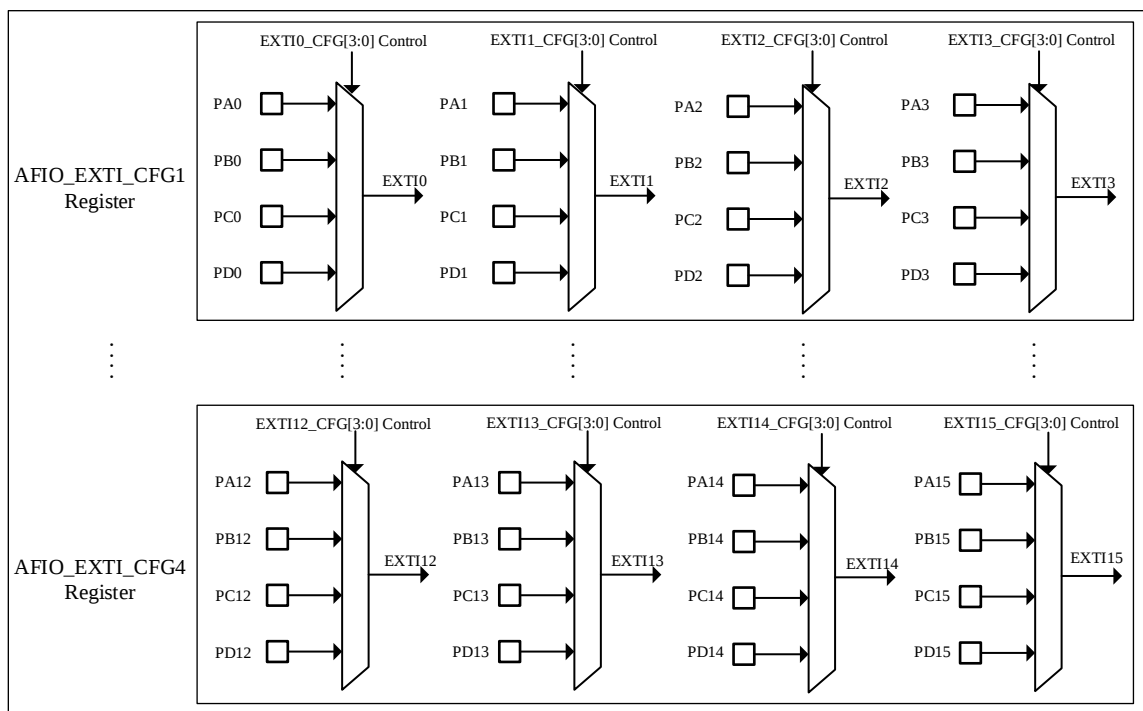
图 6-2 外部中断通用 I/O 映射
