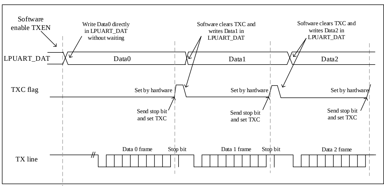
图 25-3 发送时 TXC 的变化情况
