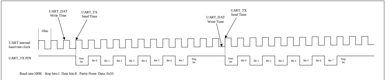
图 24-5 发送时差
