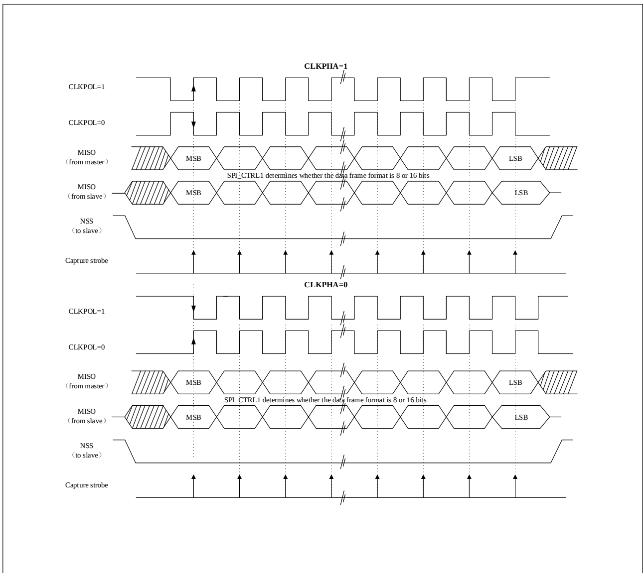
图 26-4 数据时钟时序图
