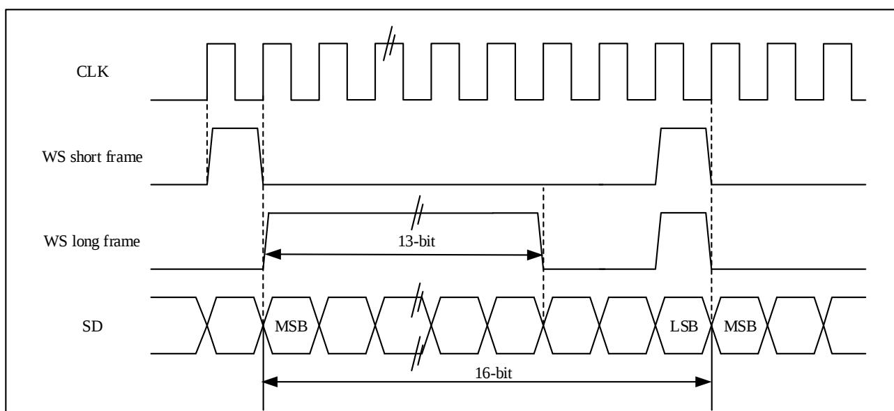
图 26-23 PCM 标准波形（16 位）
