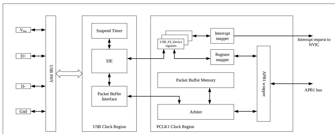
图 28-1 USB 设备框图
