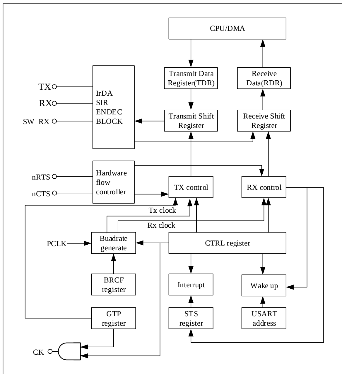
图 24-1 USART 框图
