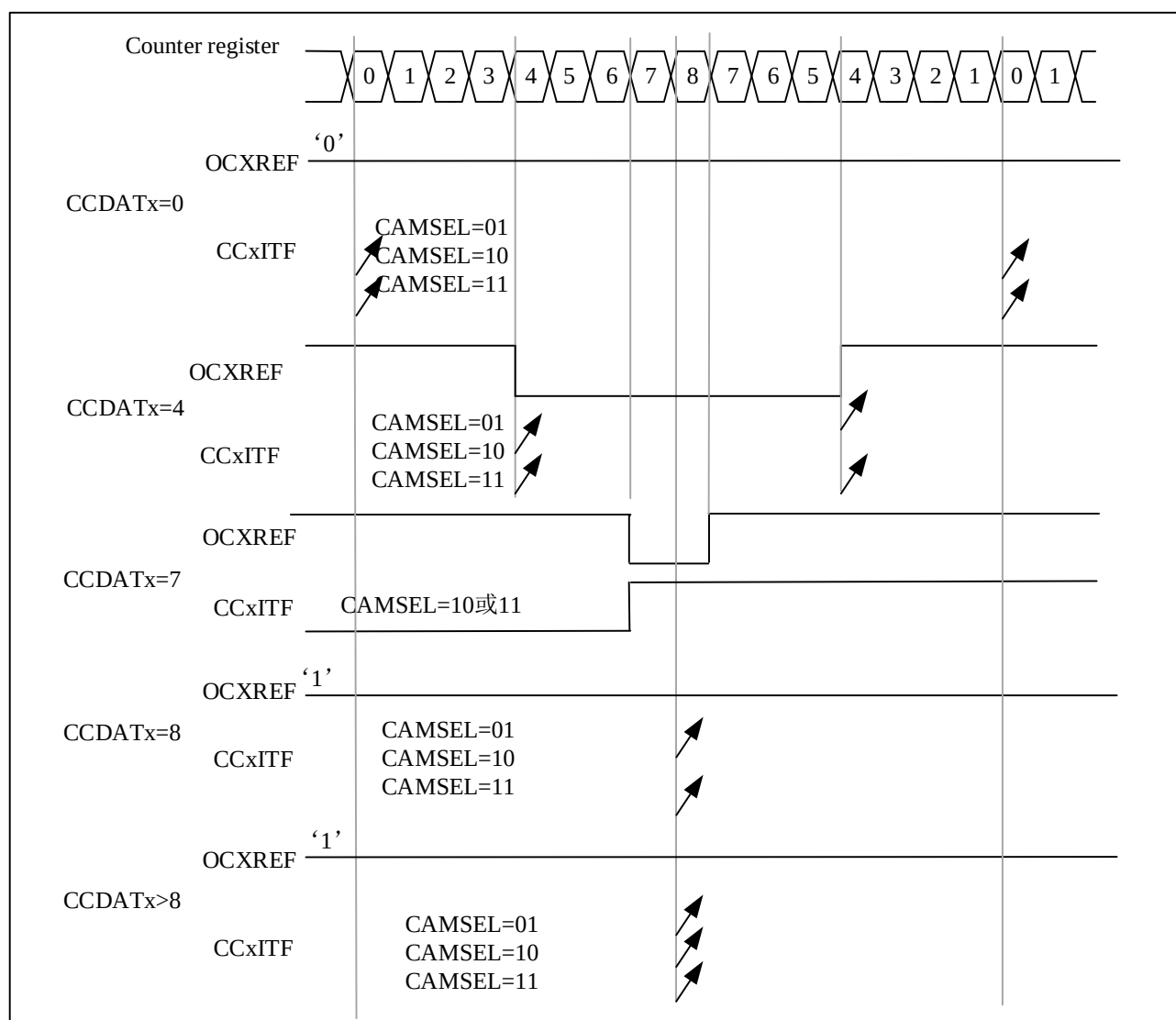
图 11-18 中央对齐的 PWM 波形(AR=8)
