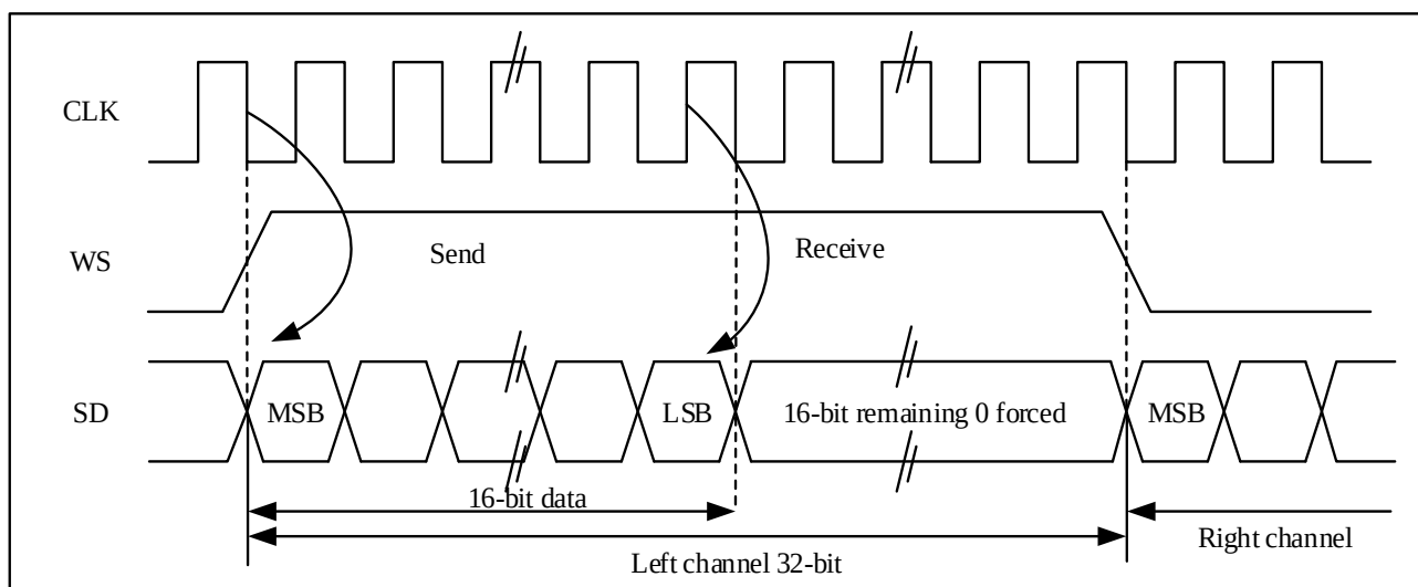
图 25-19 MSB 对齐 16 位数据扩展到 32 位包帧，CLKPOL = 0
