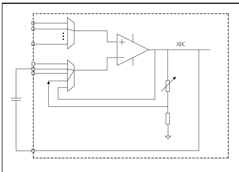
图 20-5 带滤波内部增益模式
