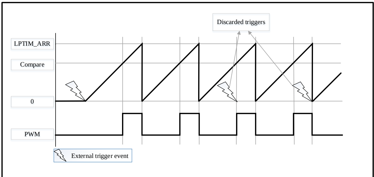
图 13-3 LPTIM 输出波形，连续计数模式配置
