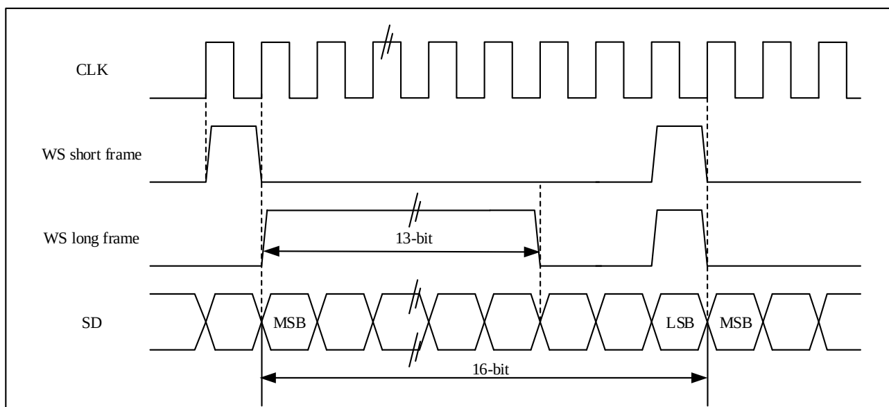
图 25-23 PCM 标准波形（16 位）
