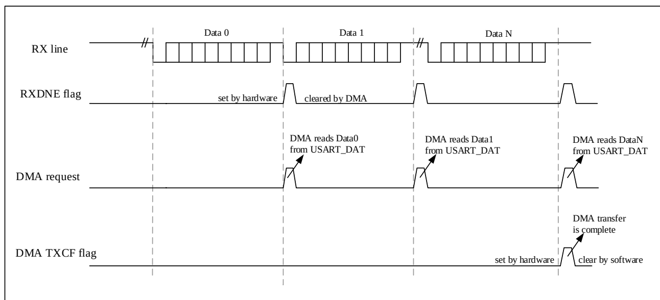
图 23-9 DMA 接收
