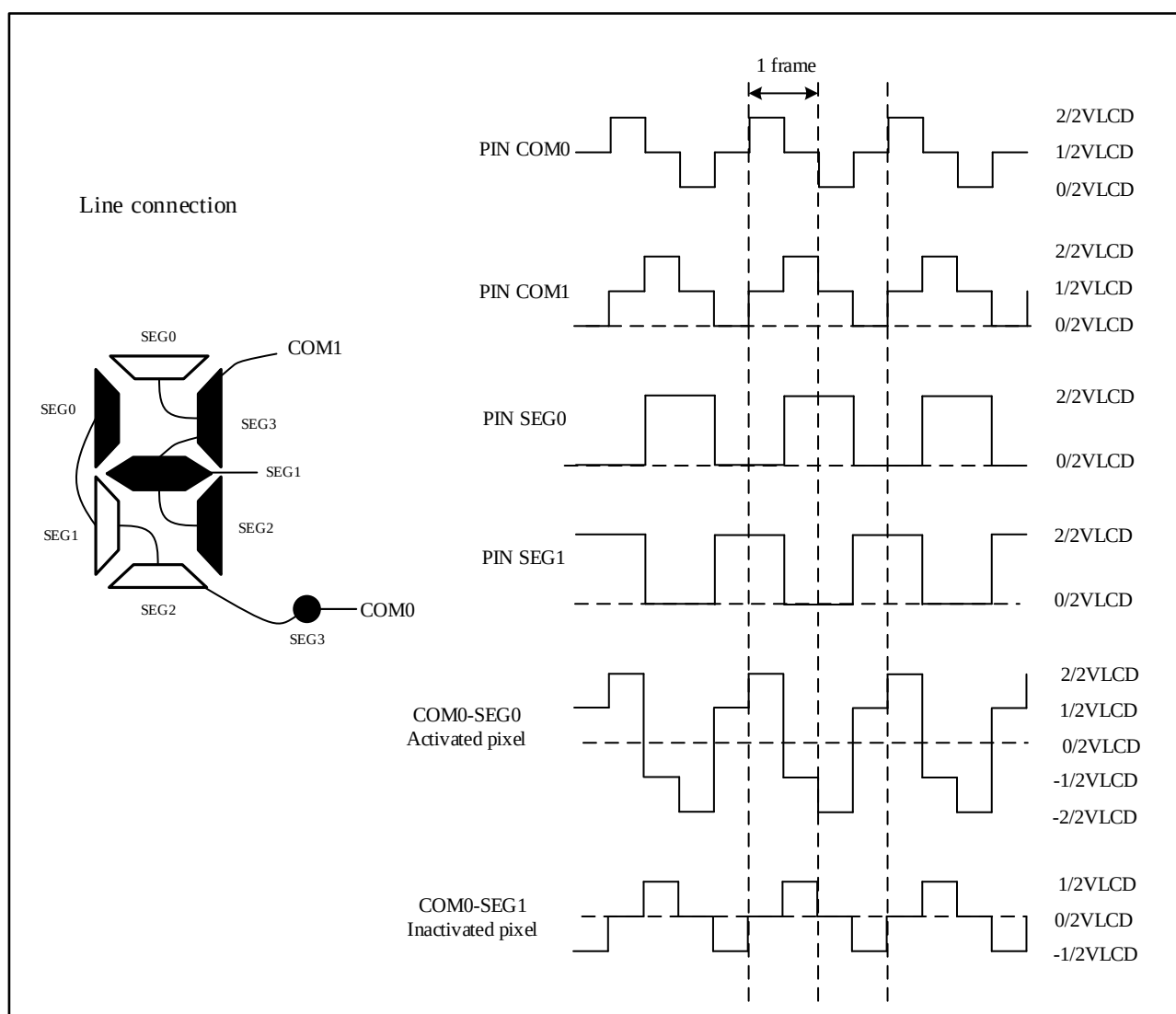
图 21-4 1/2 占空比, 1/2 偏置
