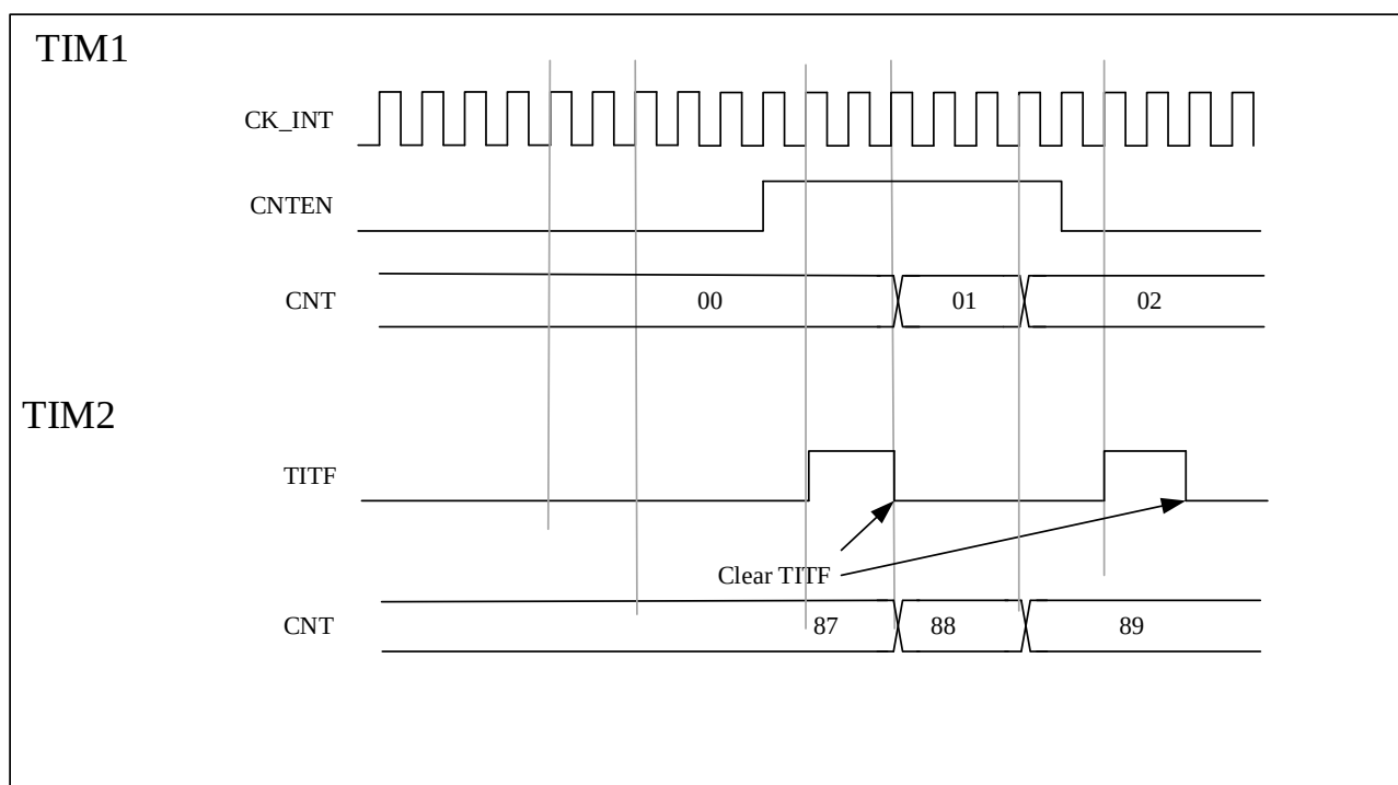
图 11-24 定时器 2 由定时器 1 的使能门控
