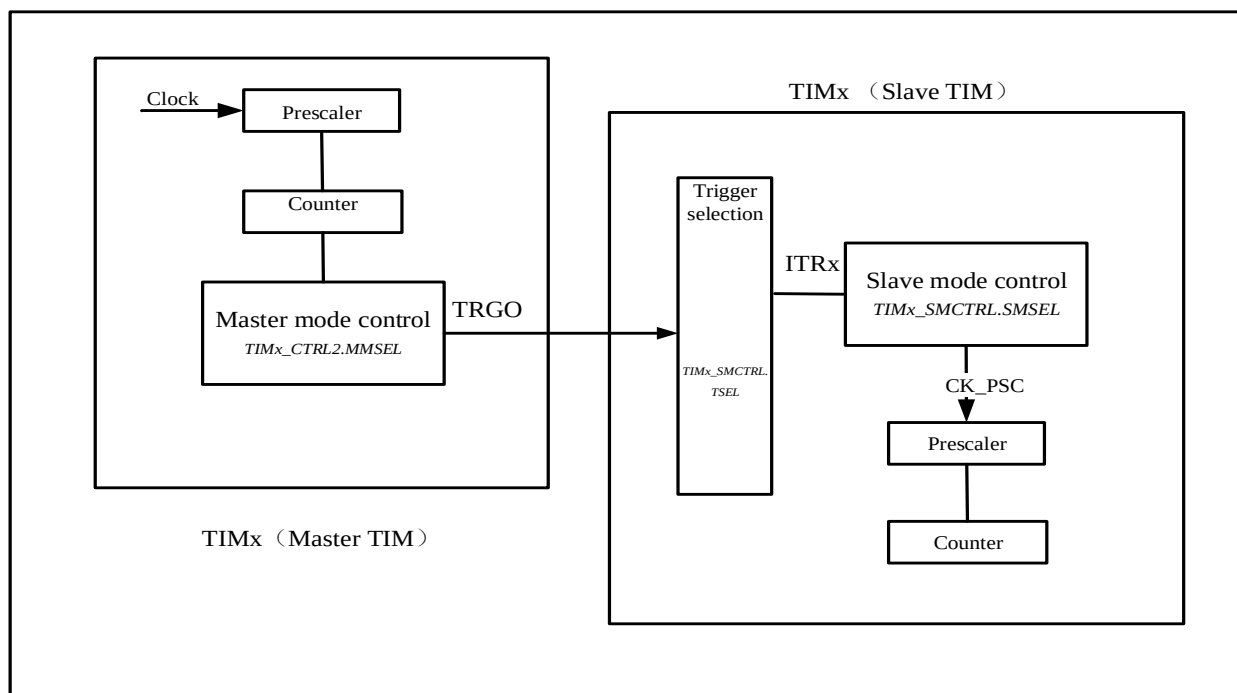
图 11-22 主/从定时器的例子
