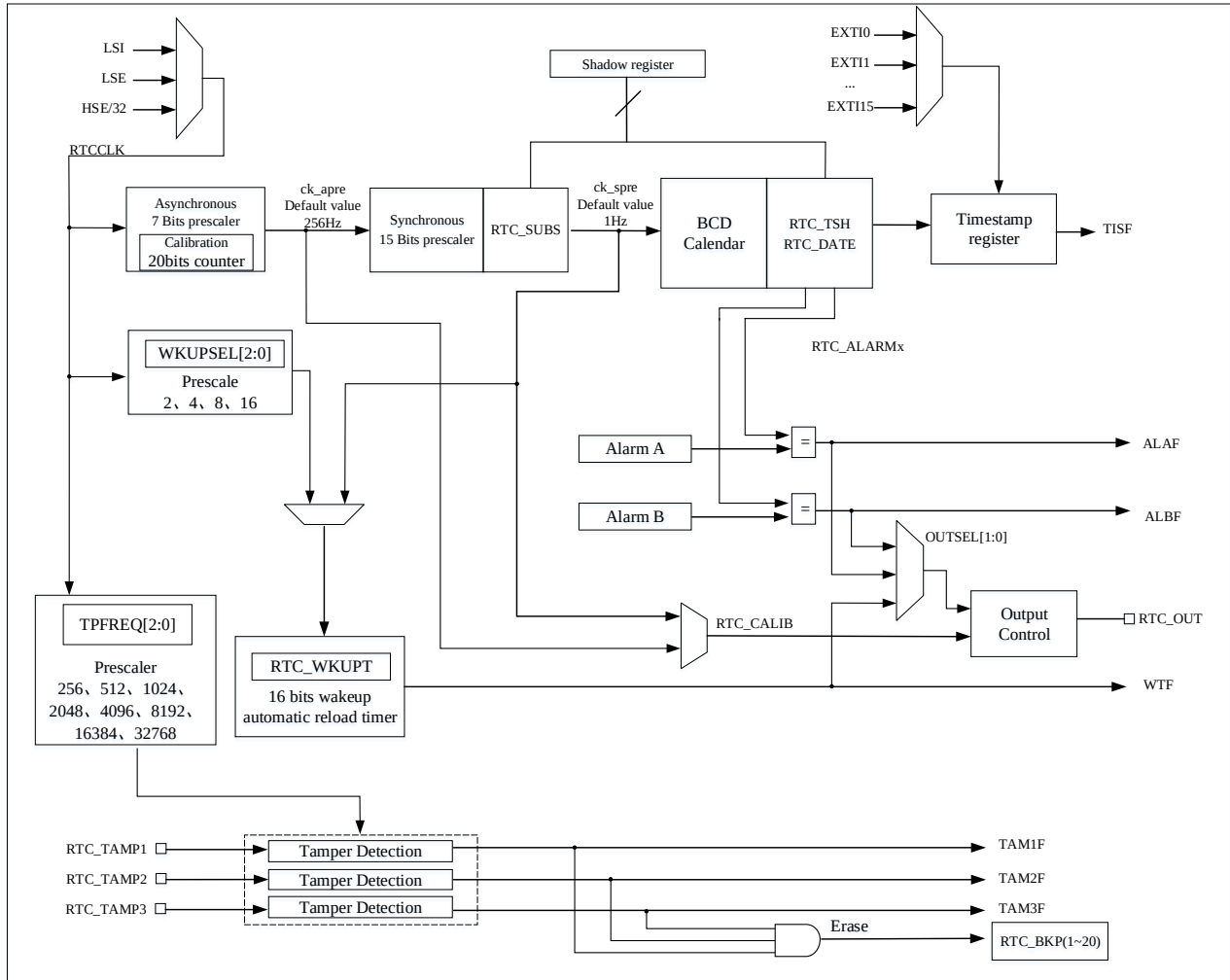
图 14-1 RTC 框图
