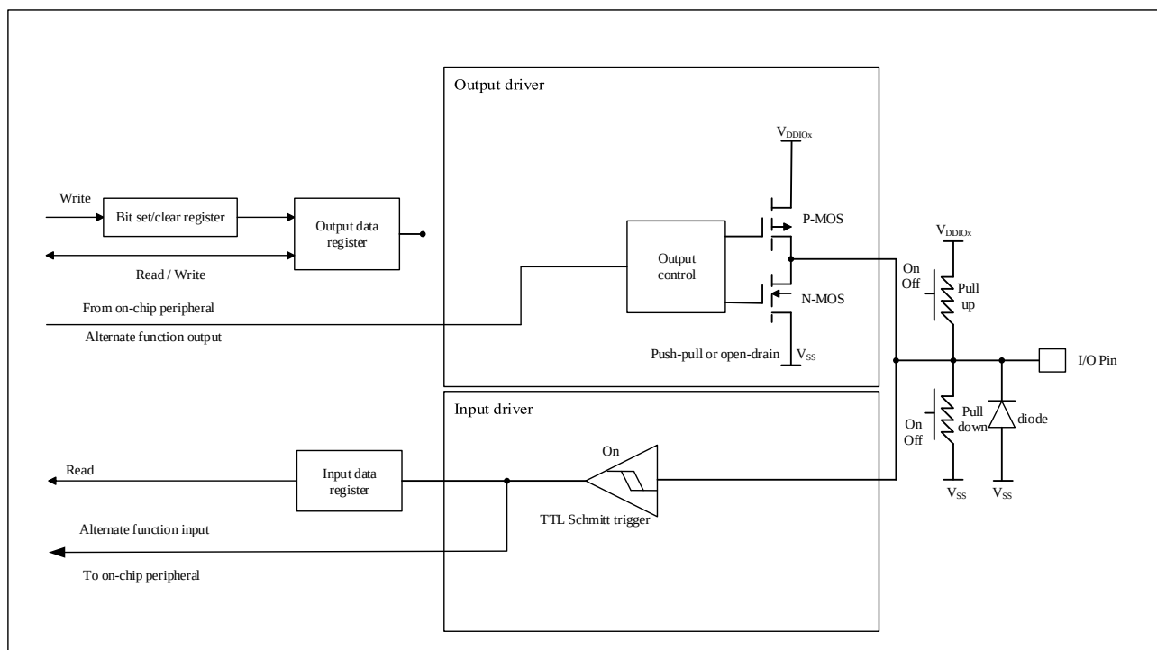
图 5-4 复用功能配置
