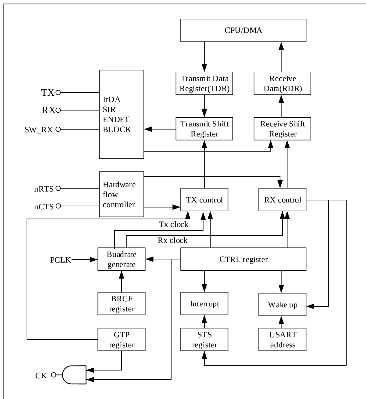
图 23-1 USART 框图
