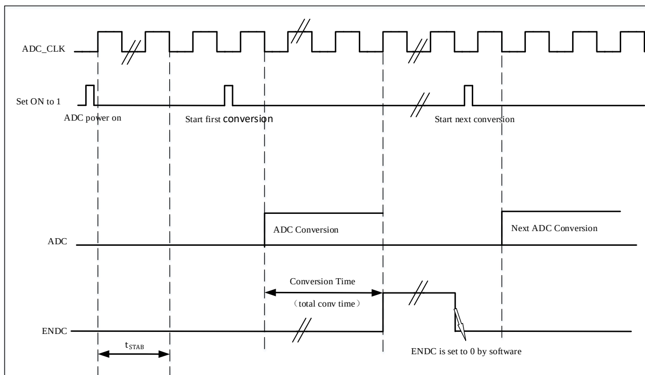
图 17-4 时序图
