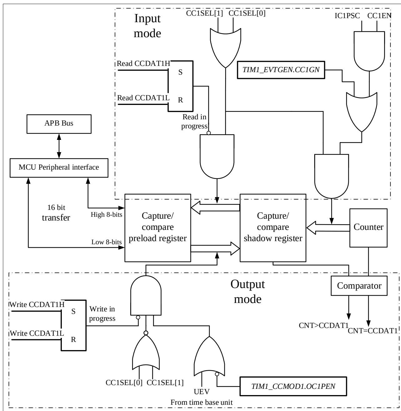
图 11-14 捕获/比较通道 1 主电路
