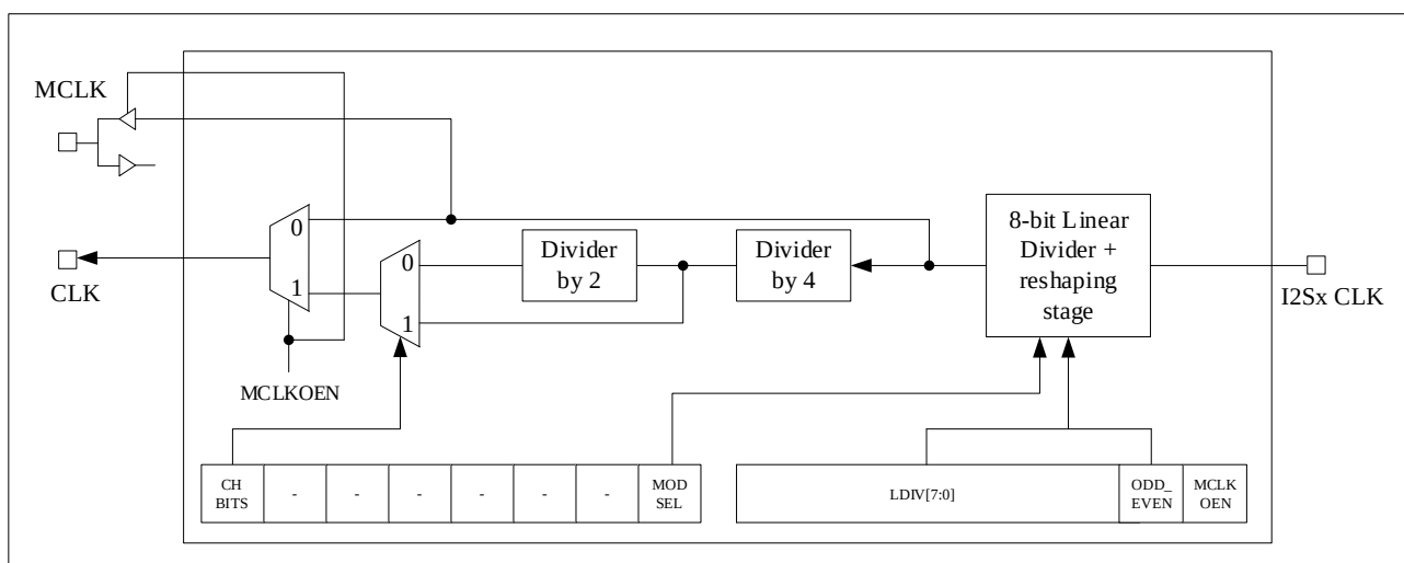
图 25-25 I²S 时钟发生器结构
