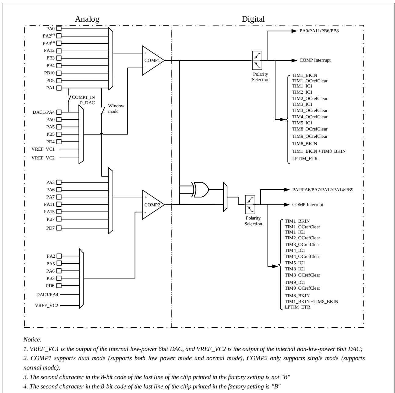
图 19-1 比较器 1 和比较器 2 系统连接图
