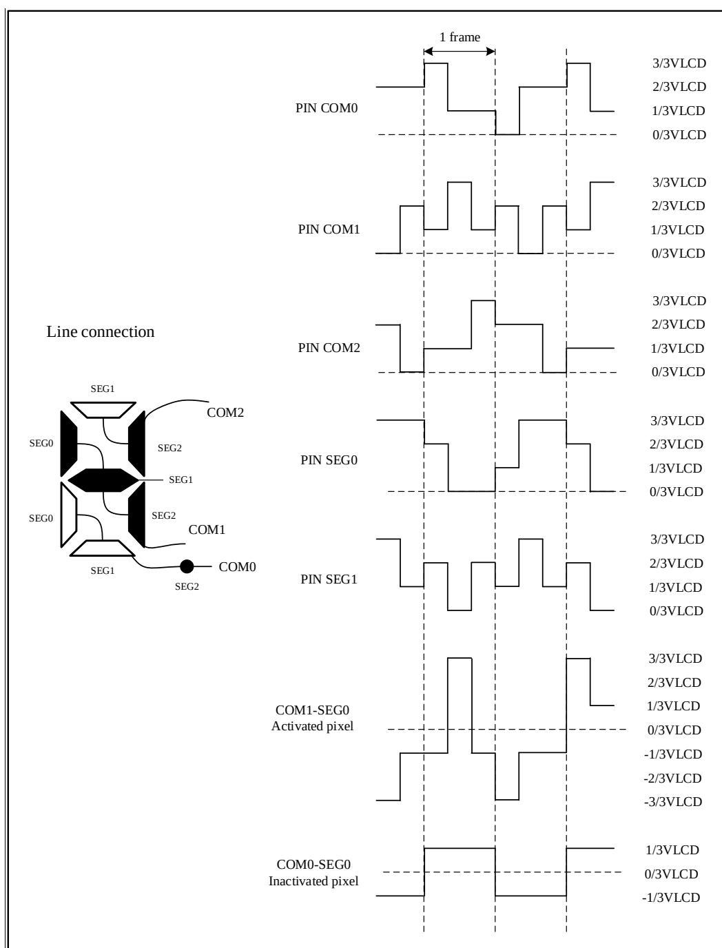
图 21-5 1/3 占空比, 1/3 偏置
