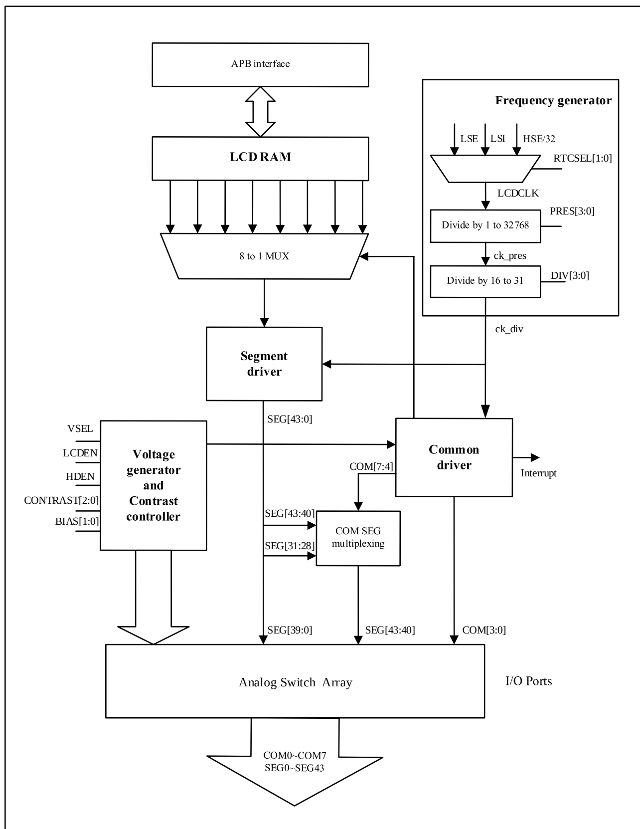
图 21-1 LCD 控制器框图
