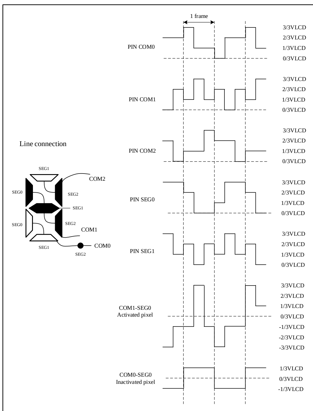
图 21-6 1/4 占空比, 1/3 偏置
