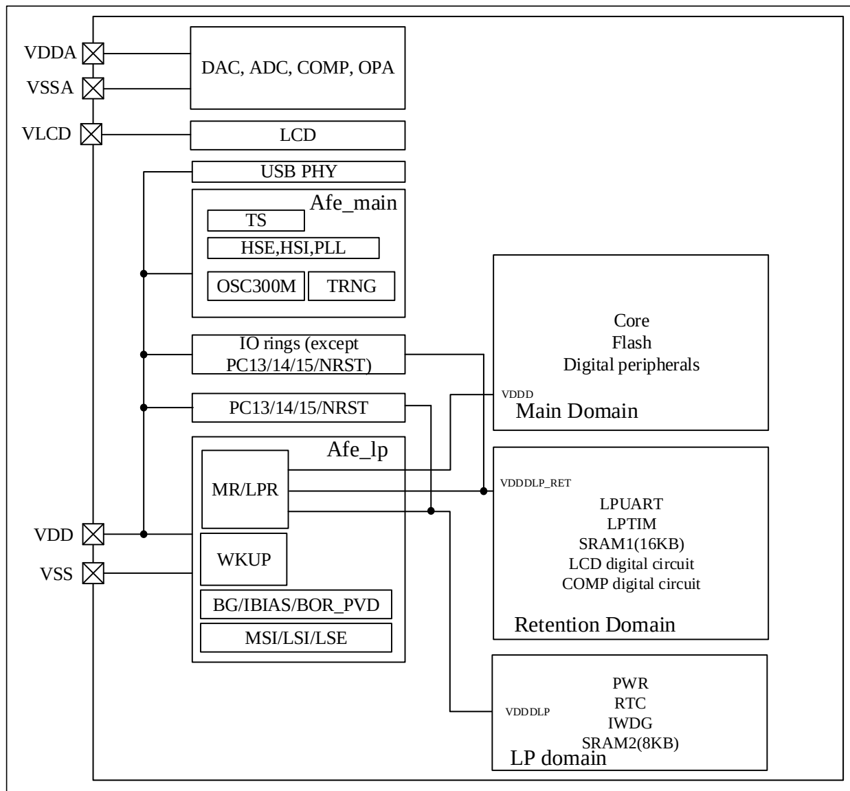
图 3-1 电源框图
