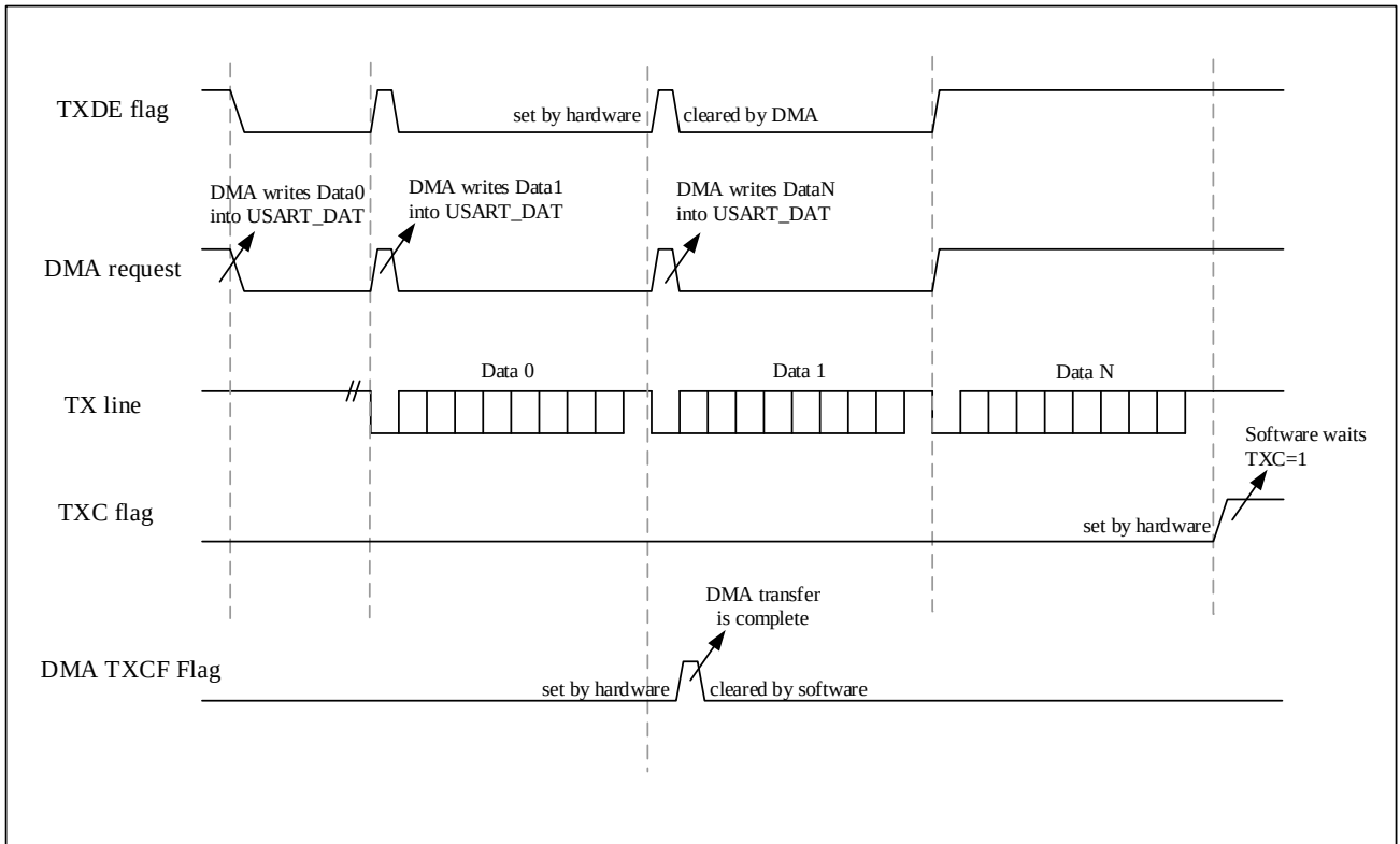
图 23-8 DMA 发送
