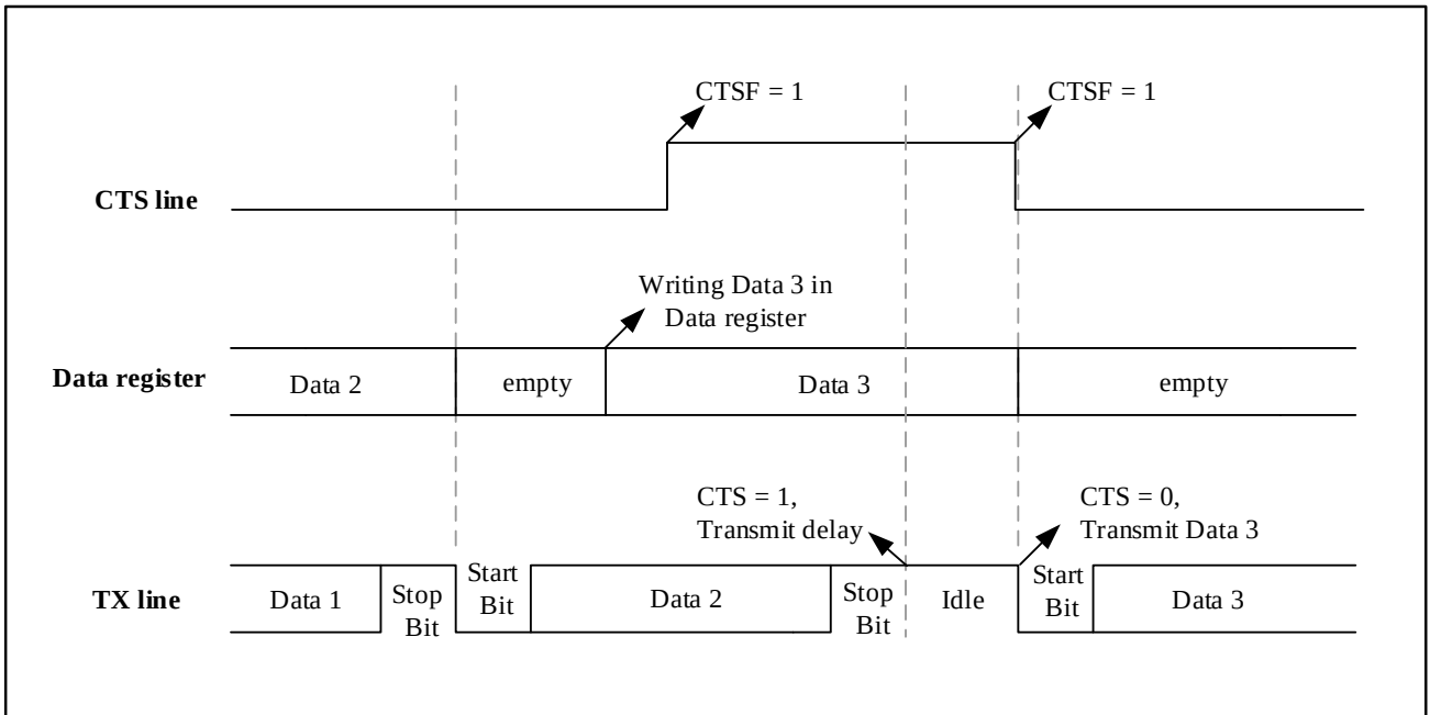
图 23-12 CTS 流控制
