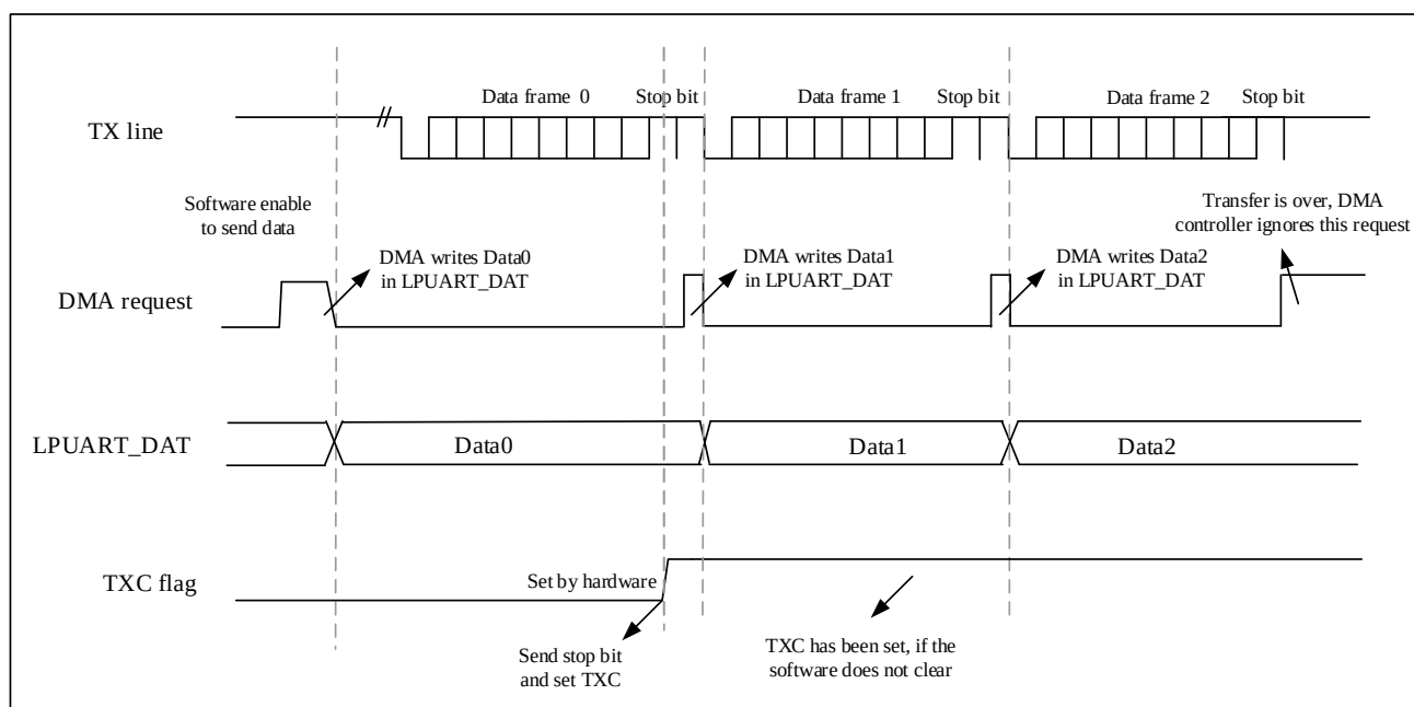
图 24-5 利用 DMA 发送
