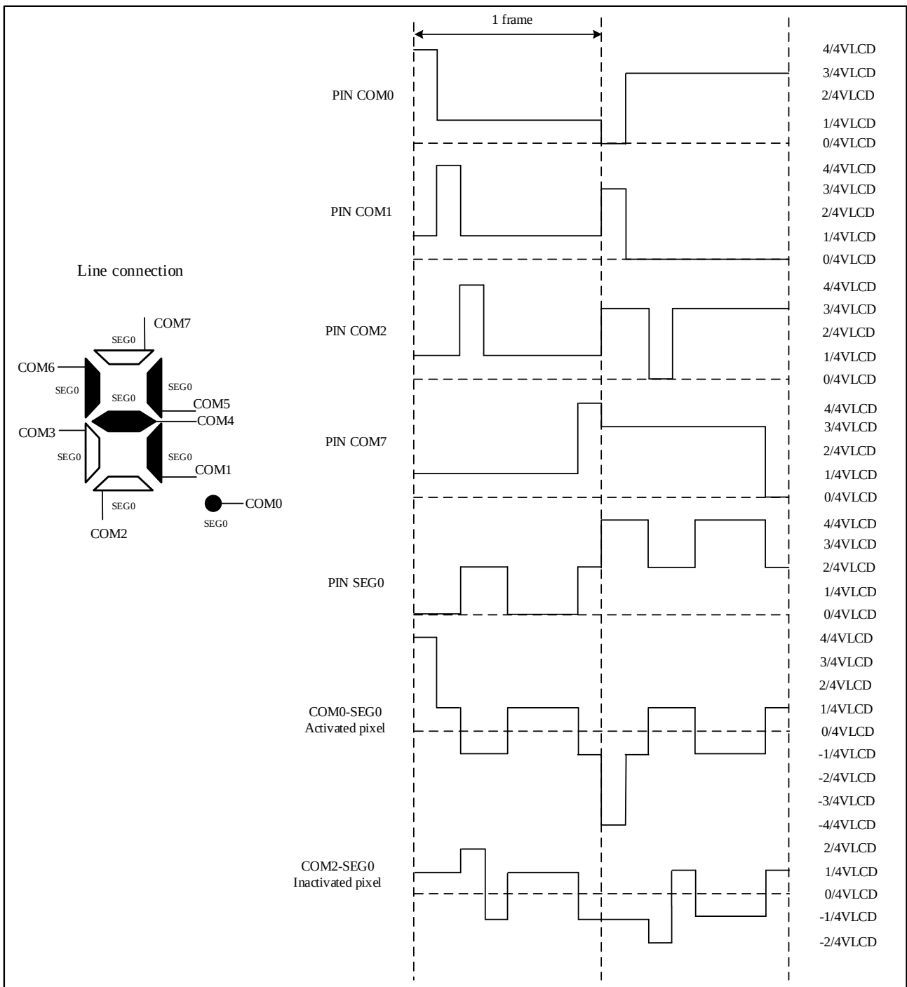
图 21-7 1/8 占空比, 1/4 偏置
