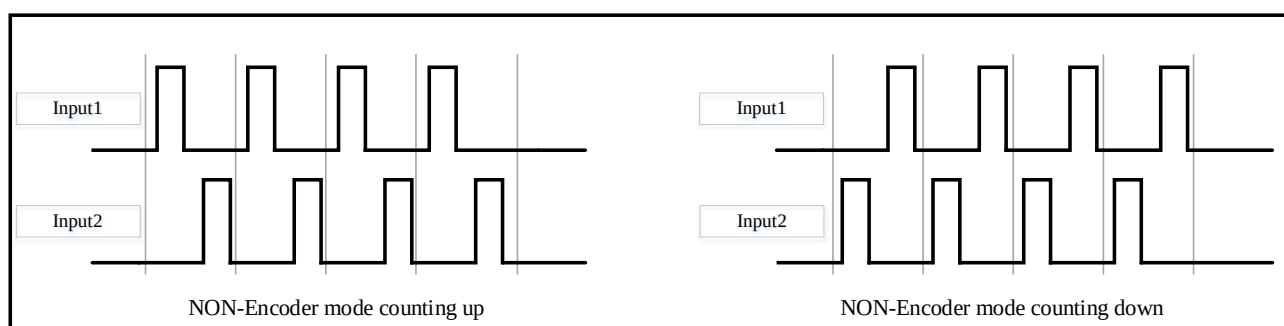
图 13-8 非正交编码器正常工作 Input1、Input2 波形
