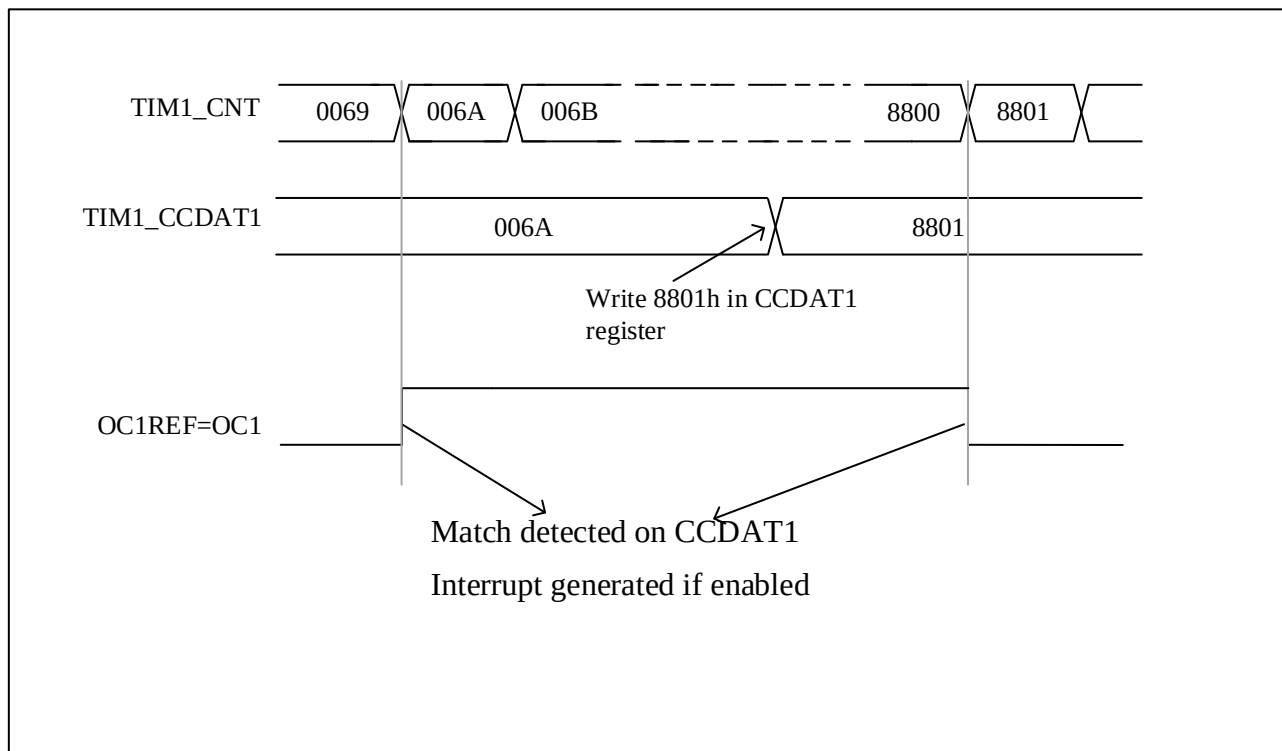
图 11-17 输出比较模式，开启 OC1
