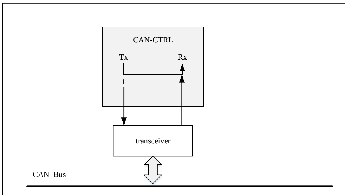
图 26-5 静默模式
