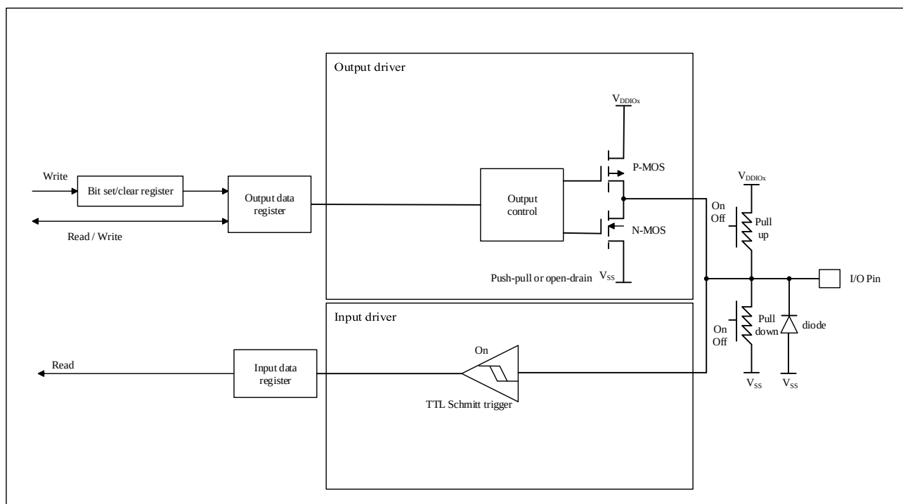
图 5-3 输出模式配置
