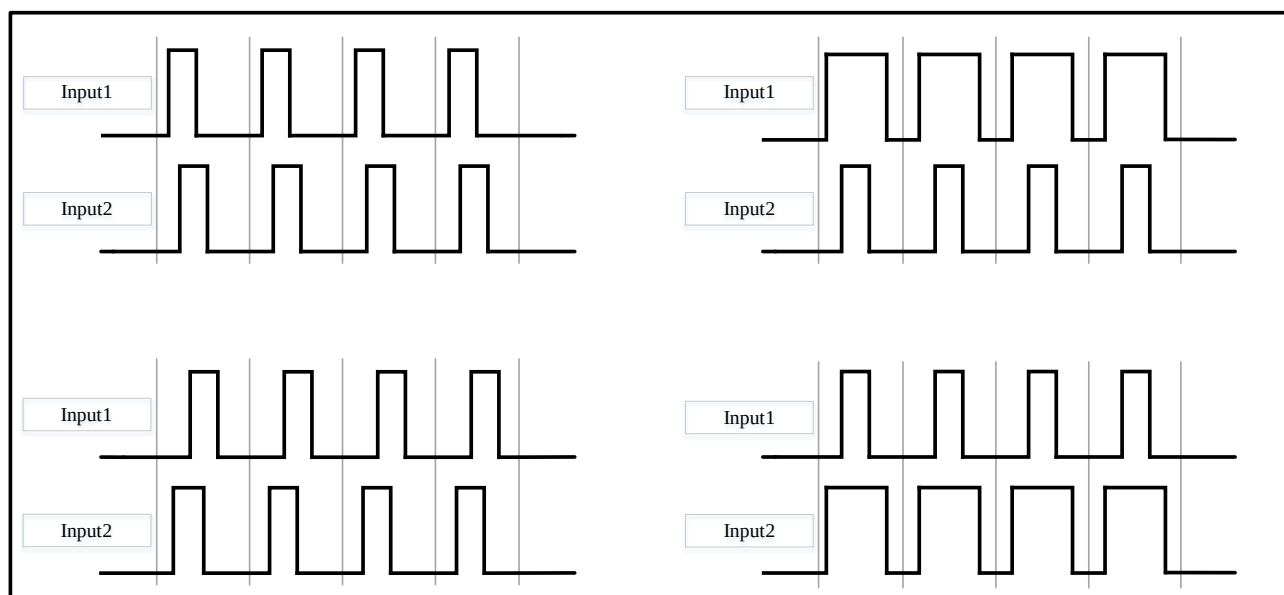
图 13-9 非正交编码器非正常工作 Input1、Input2 波形
