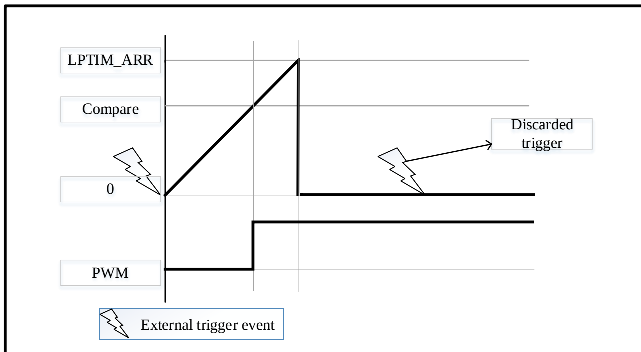
图 13-5 LPTIM 输出波形，一次模式
