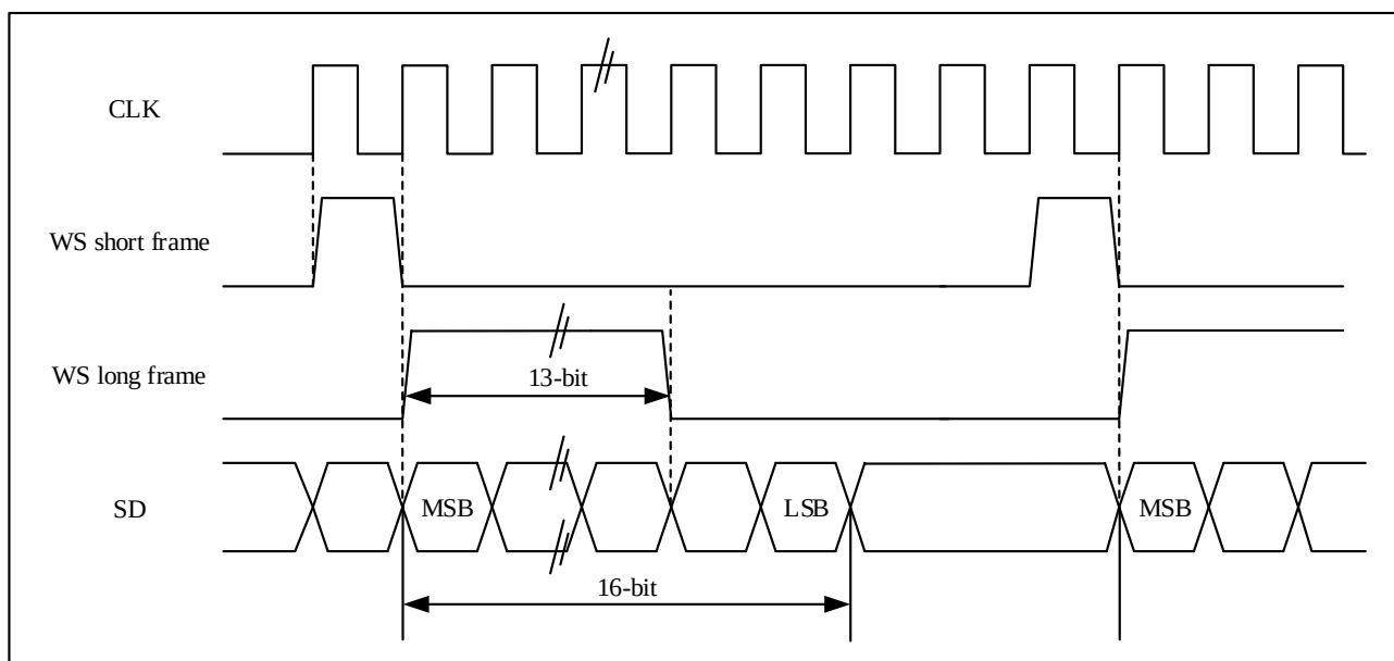
图 25-24 PCM 标准波形（16 位扩展到 32 位包帧）
