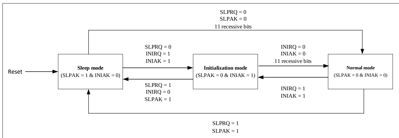
图 26-2 CAN 工作模式
