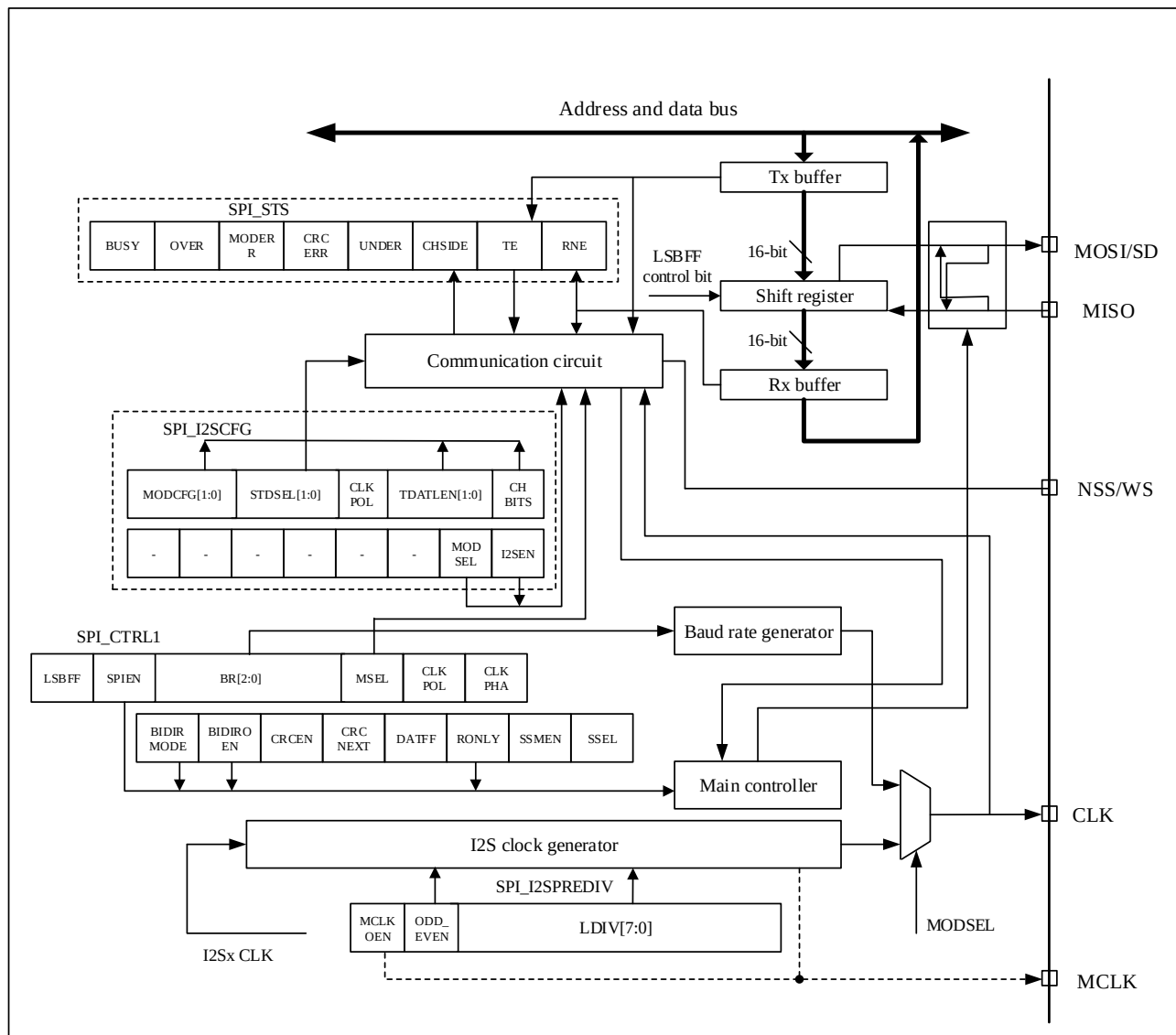
图 25-13 I 2 S 框图
