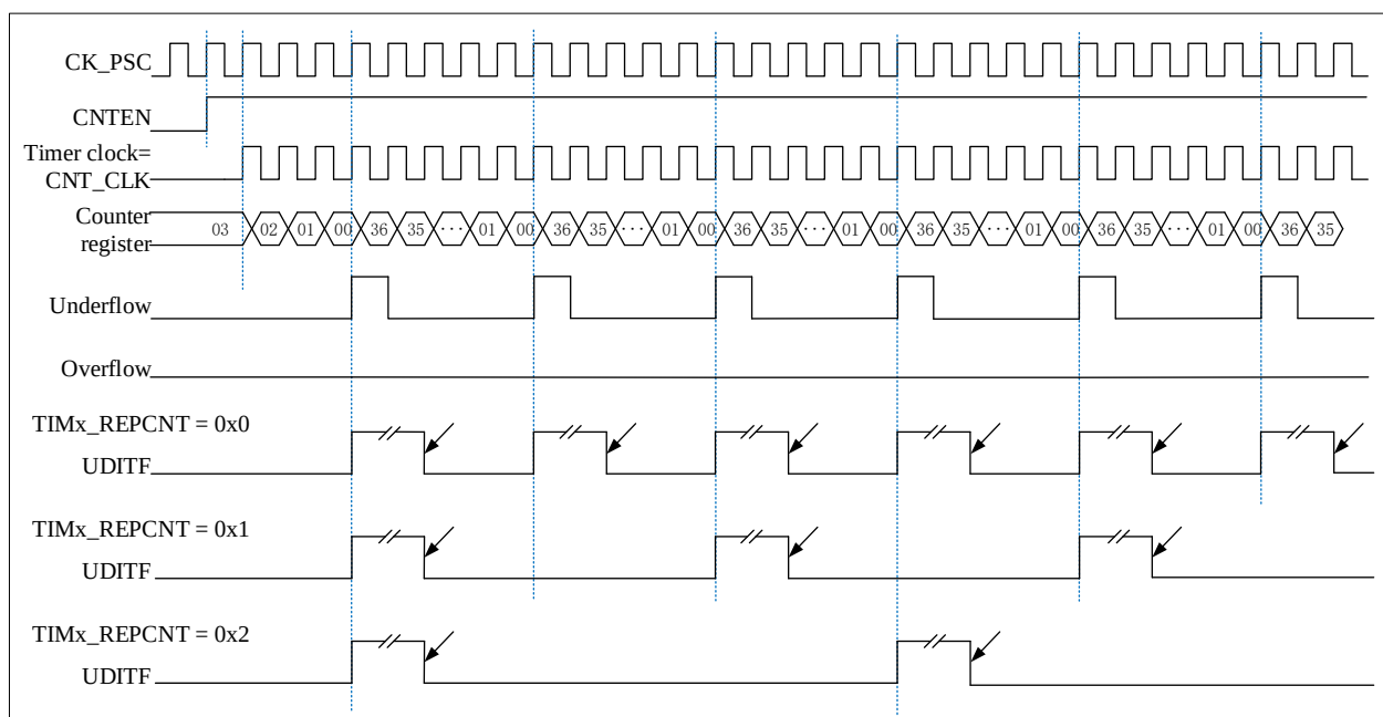
图 10-8 向下计数模式下的重复计数时序图
