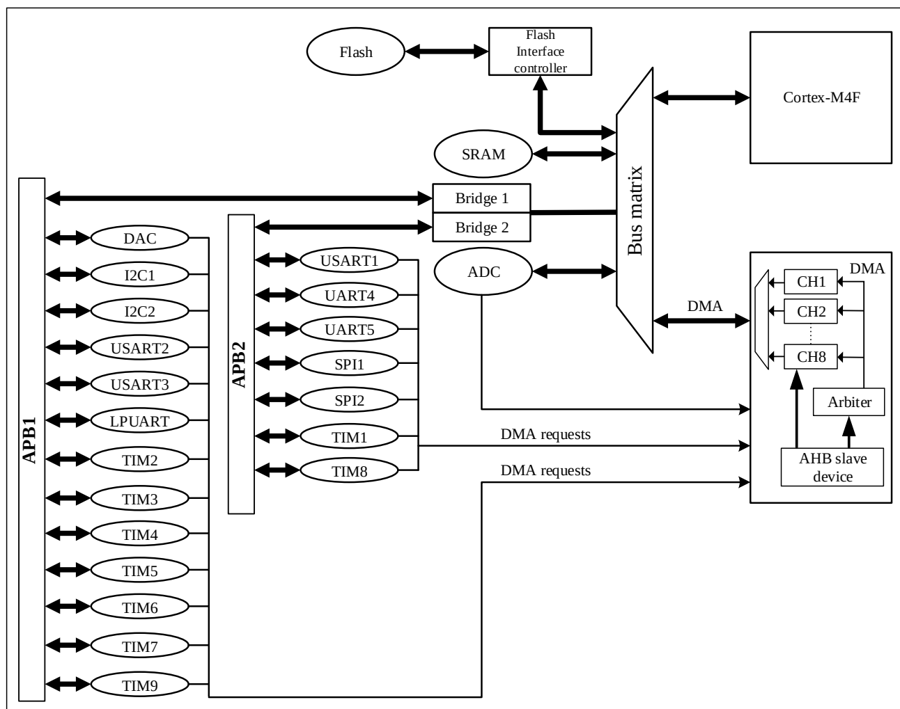
图 7-1 DMA 框图
