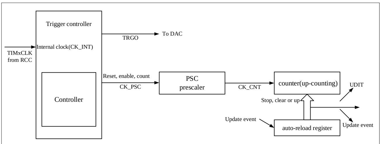
图 12-1 TIMx 的框图 (x = 6/7)
