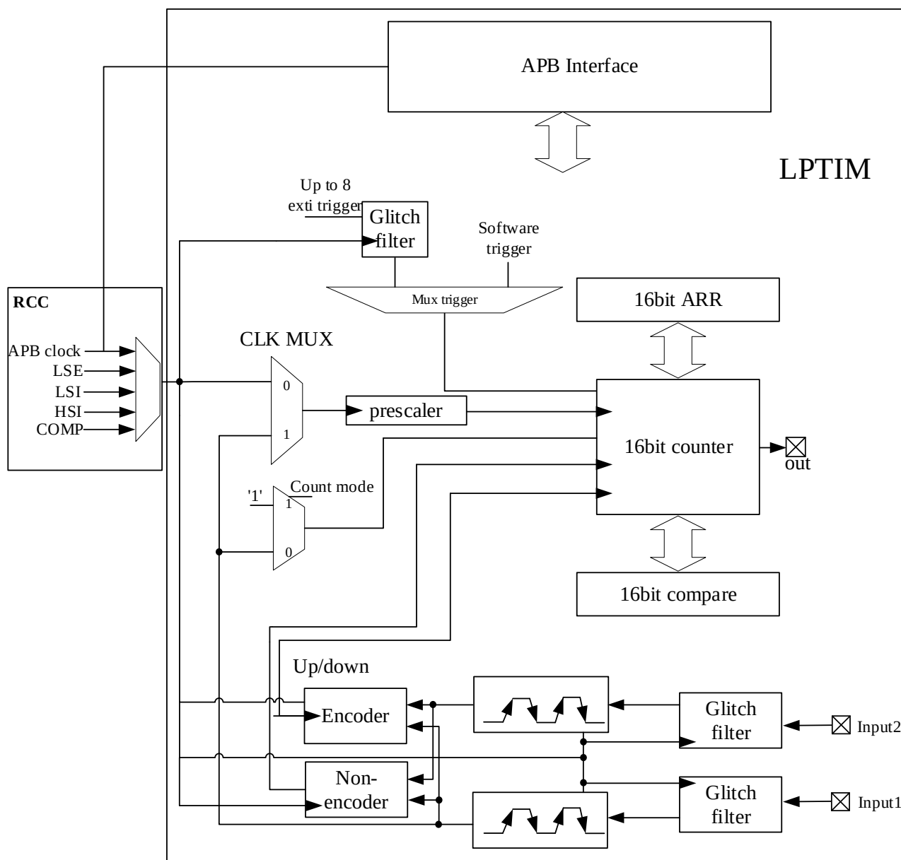
图 13-1 LPTIM 主框图
