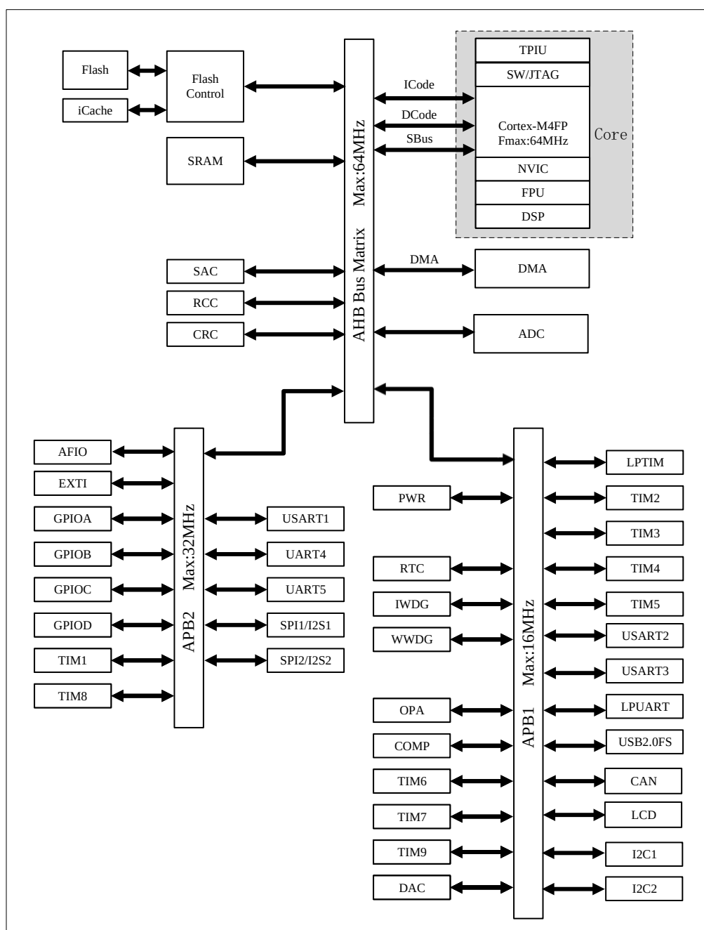
图 2-1 总线架构图
