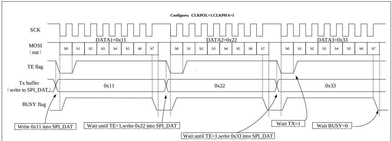
图 25-10 BIDIRMODE = 0，ONLY = 0 非连续传输发送时，SPI_STS.TE/BUSY 变化示意图
