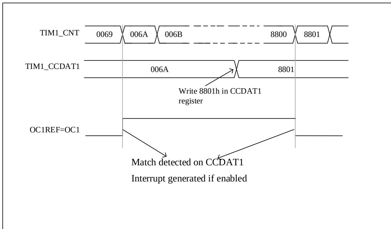
图 10-21 输出比较模式，开启 OC1
