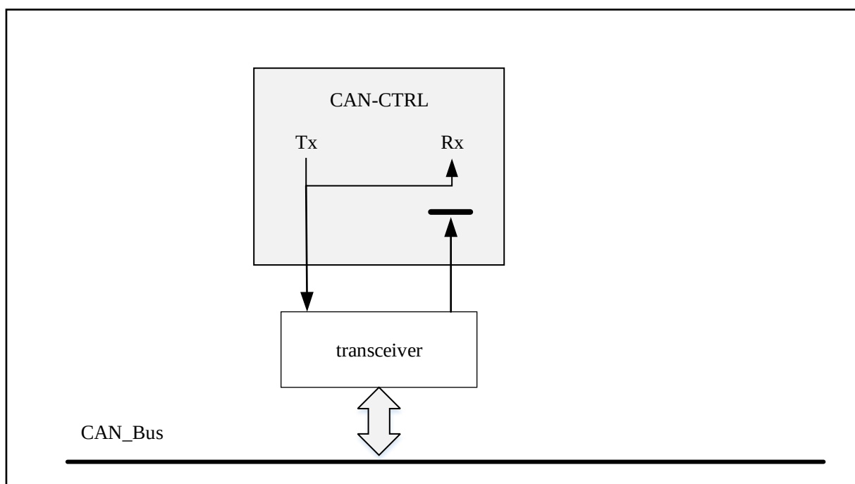
图 26-4 回环模式
