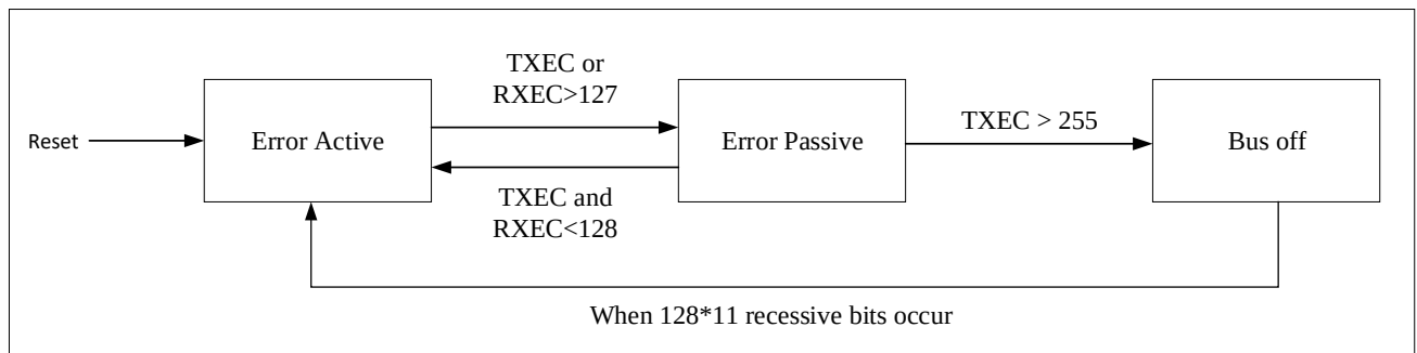
图 26-14 CAN 错误状态框图
