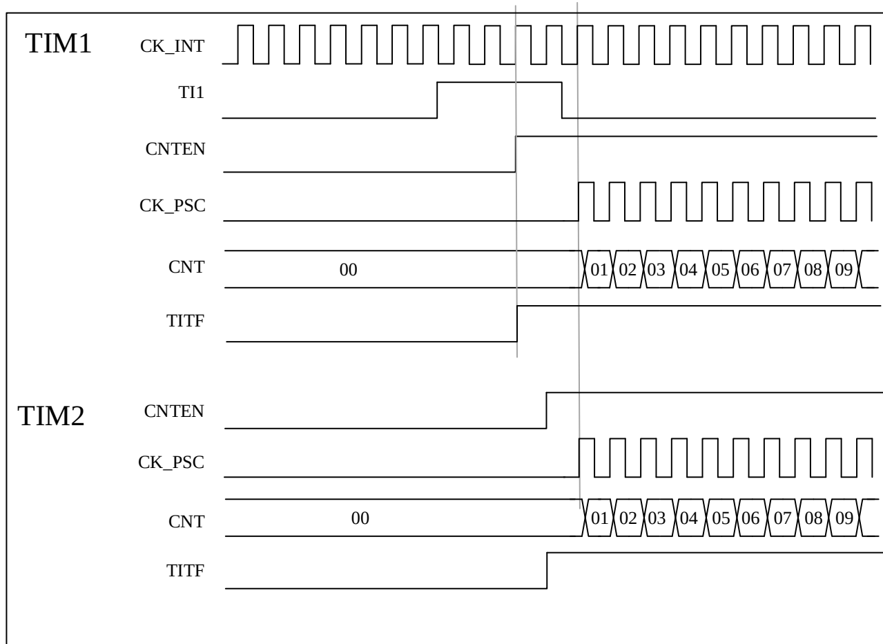
图 11-26 使用定时器 1 的 TI1 输入触发定时器 1 和定时器 2
