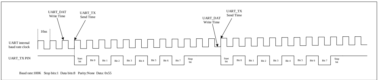
图 23-5 发送时差
