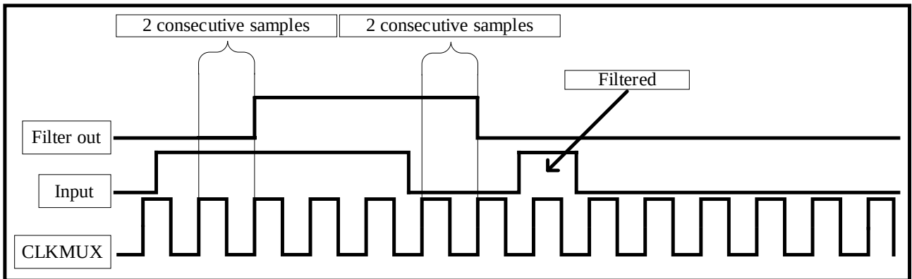
图 13-2 毛刺滤波器时序图
