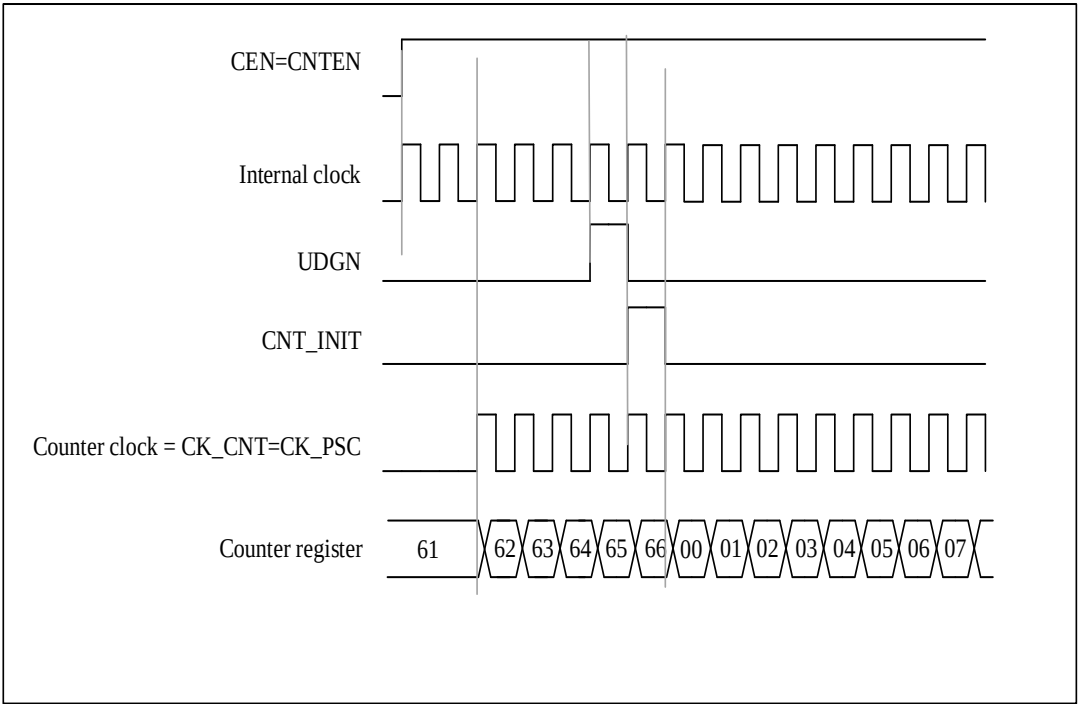
图 12-5 正常模式下的控制电路，内部时钟分频系数为 1
