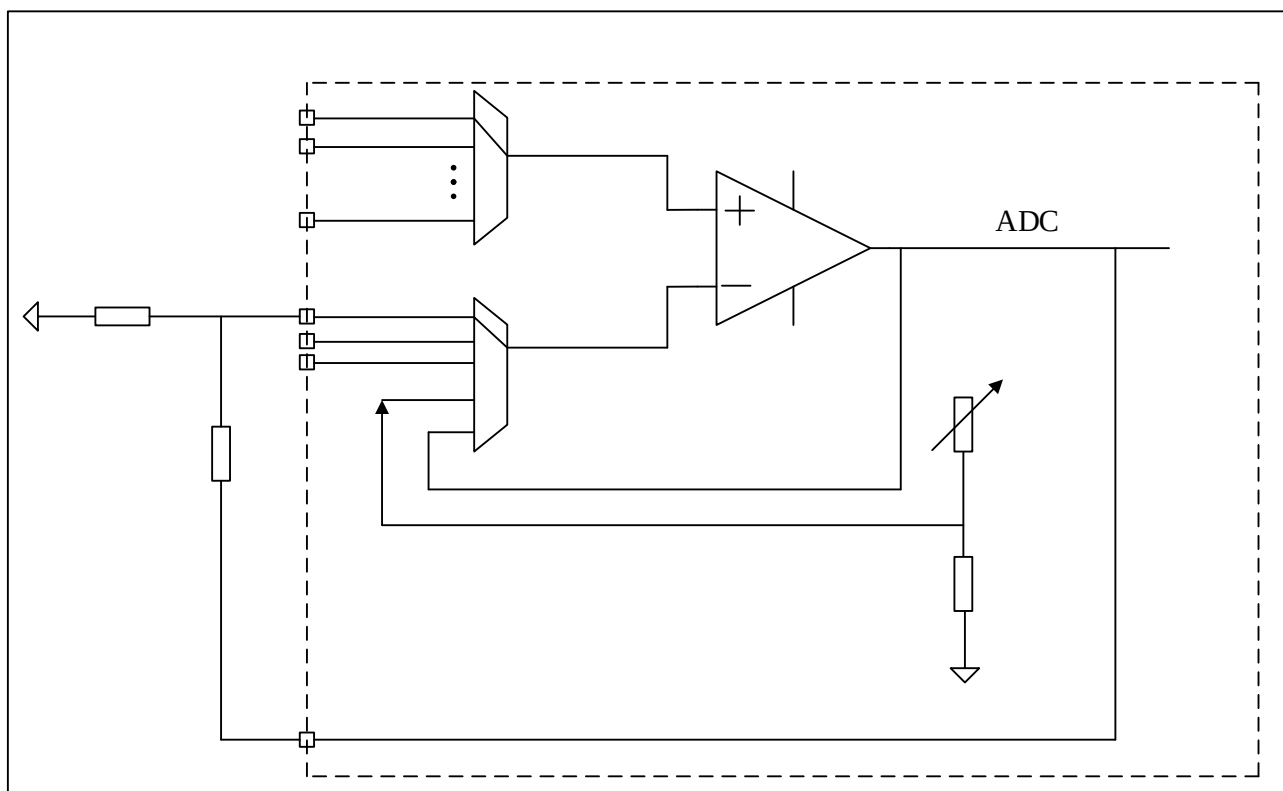
图 20-2 OPAMP 外部放大模式
