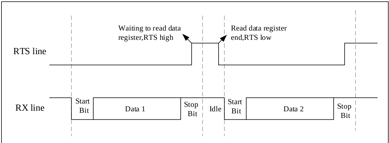
图 23-11 RTS 流控制
