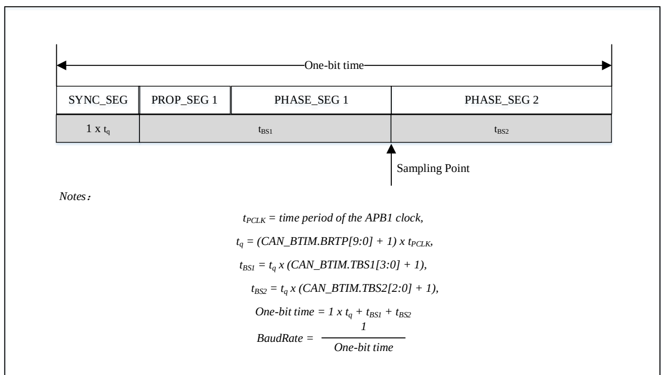
图 26-11 位时序
