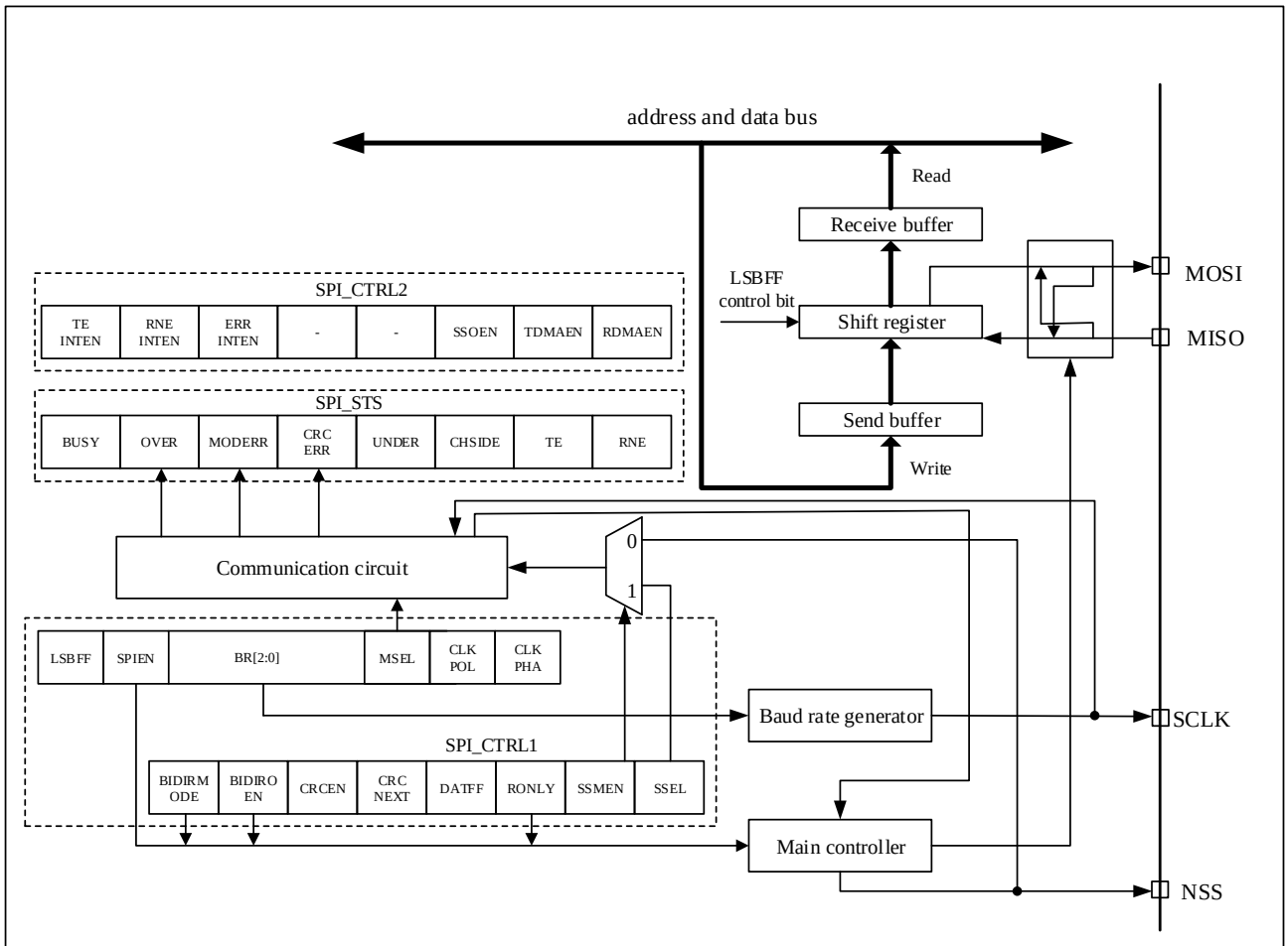
图 25-1 SPI 框图
