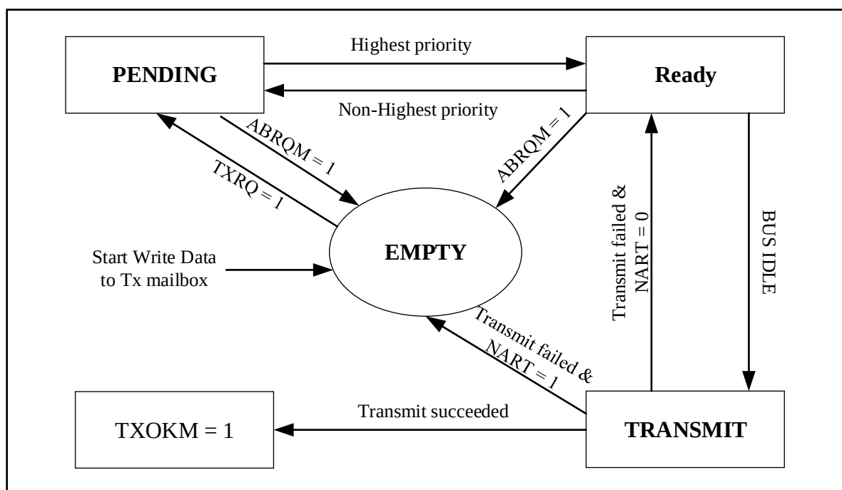
图 26-7 发送邮箱状态
