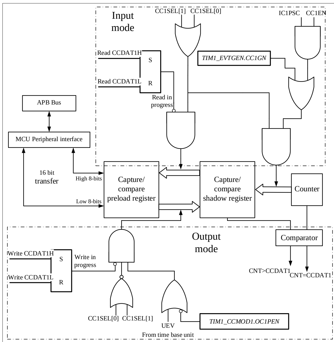
图 10-17 捕获/比较通道 1 主电路
