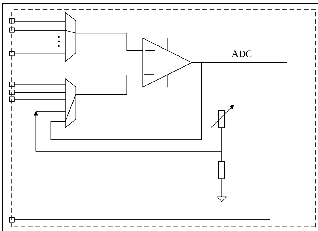
图 20-3 跟随模式
