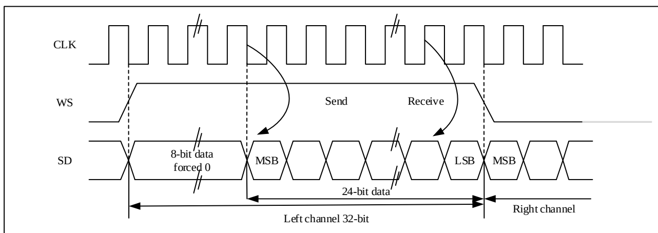
图 25-21 LSB 对齐 24 位数据，CLKPOL = 0
