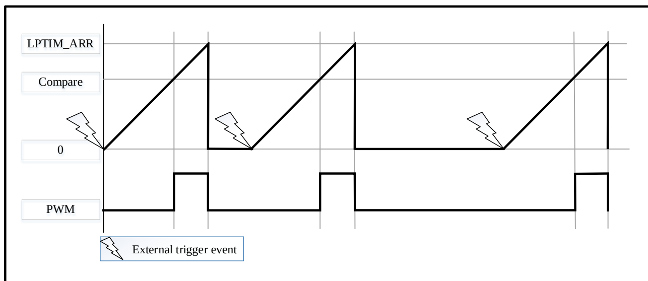
图 13-4 LPTIM 输出波形，单触发计数模式配置
