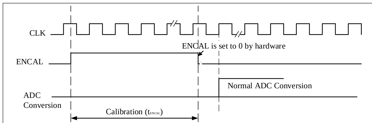
图 17-6 校准时序图
