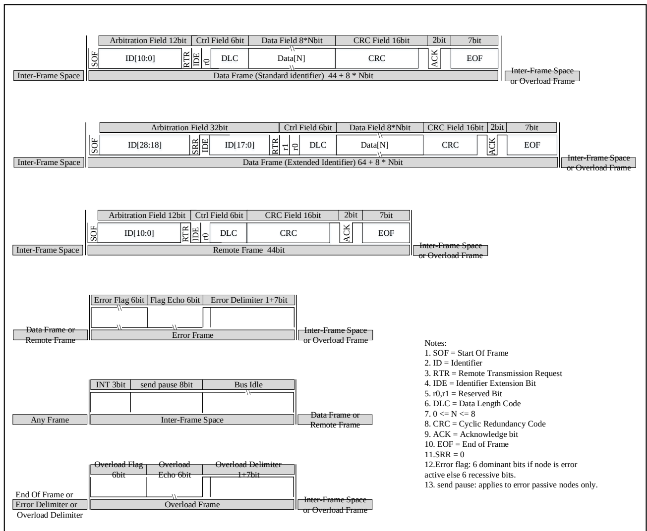
图 26-12 各类帧格式
