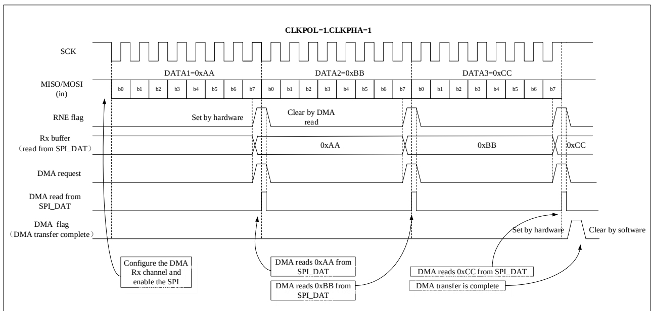
图 25-12 使用 DMA 接收
