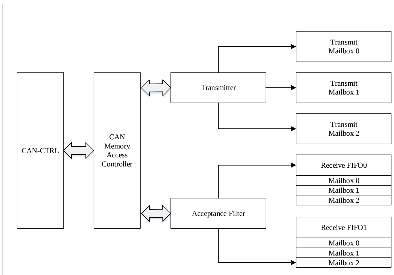
图 26-3 单 CAN 框图
