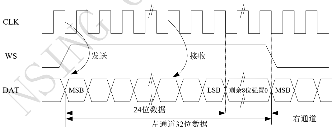
图 19-18 MSB 对齐 24 位数据，CLKPOL = 0
