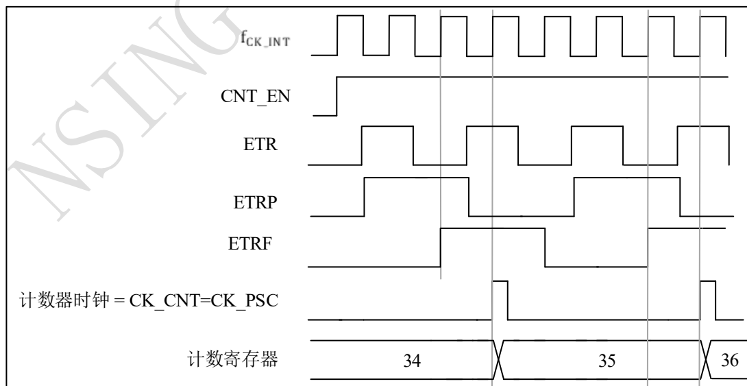
图 9-26 外部时钟模式 2 下的控制电路
