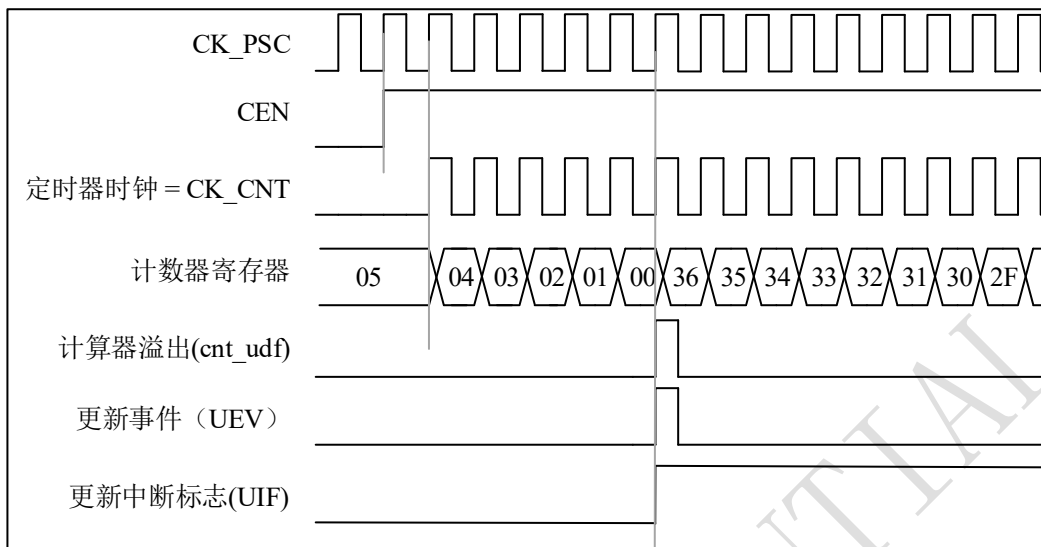
图 10-11 计数器时序图，内部时钟分频因子为 2
