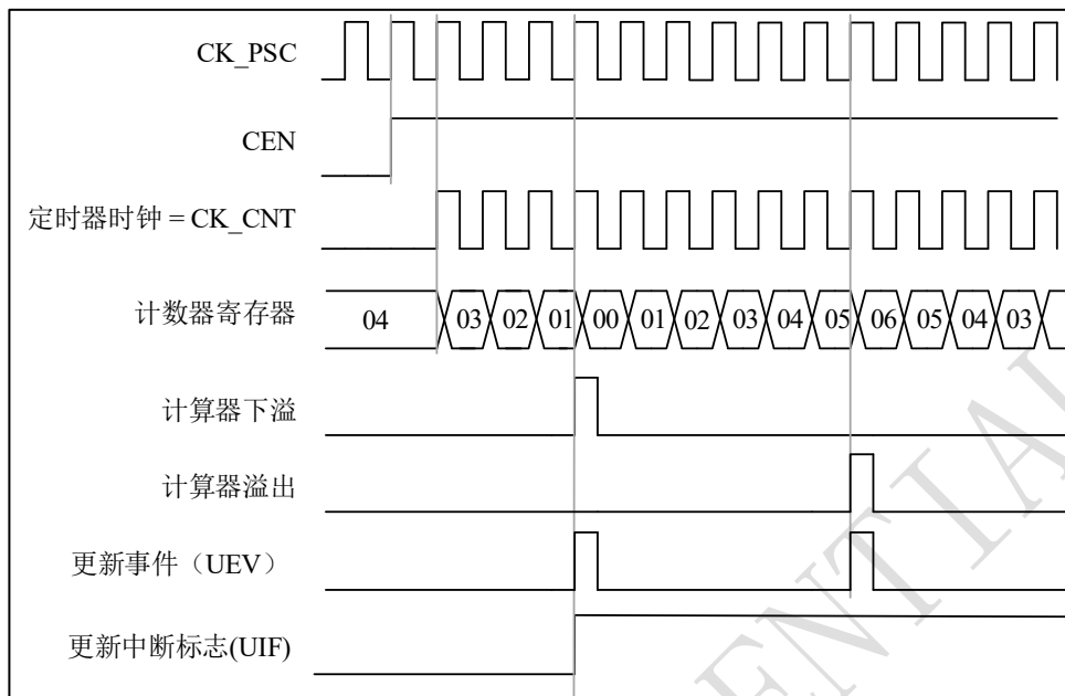
图 10-15 计数器时序图，内部时钟分频因子为 1，TIMx_AR=0x6
