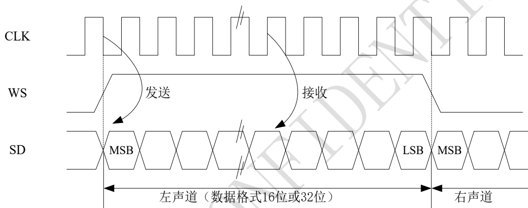
图 19-17 MSB 对齐 16 位或 32 位全精度，CLKPOL = 0
