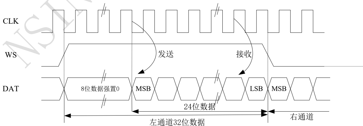
图 19-21 LSB 对齐 24 位数据，CLKPOL = 0
