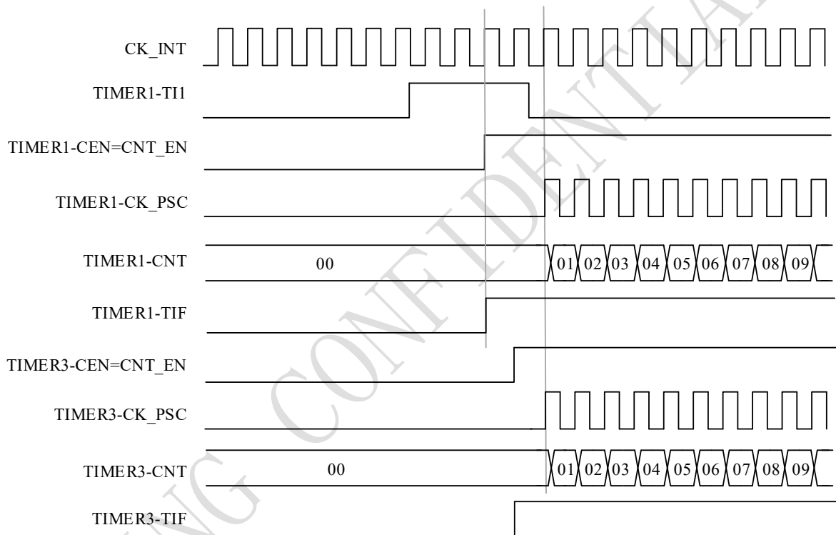
图 10-42 使用定时器 1 的 TI1 输入触发定时器 1 和定时器 3
