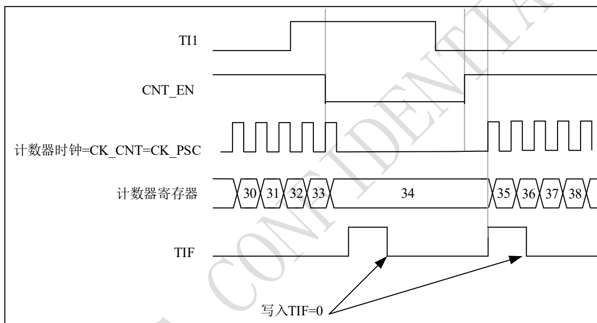
图 9-46 门控模式下的控制电路
