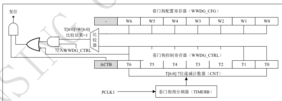
图 14-1 看门狗框图
