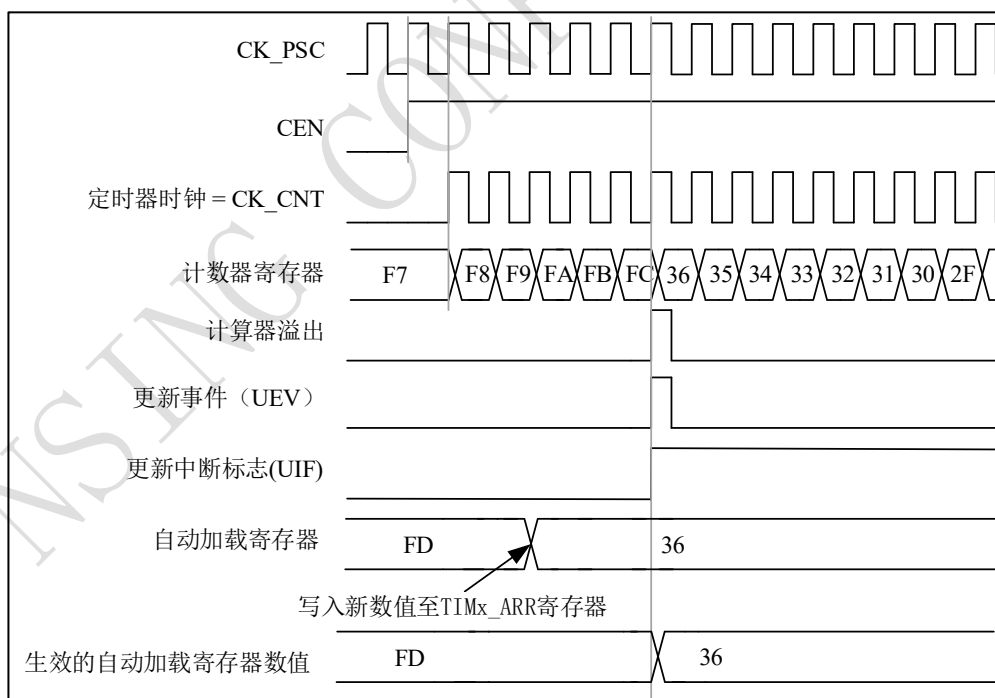
图 9-20 计数器时序图，ARPE=1 时的更新事件（计数器溢出）
