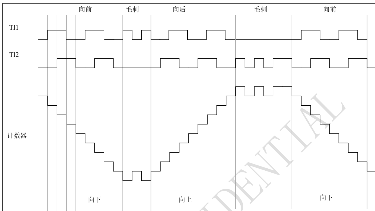
图 9-43 IC1FP1 反相的编码器接口模式实例
