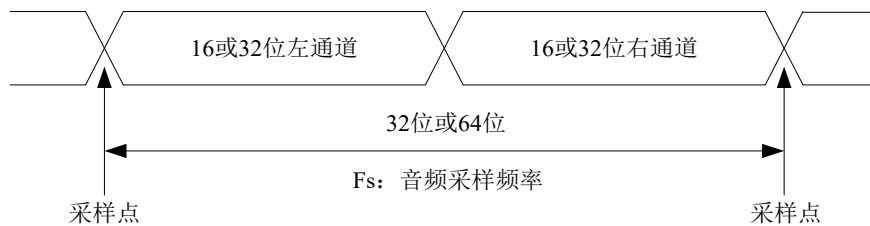
图 19-26 音频采样频率定义
