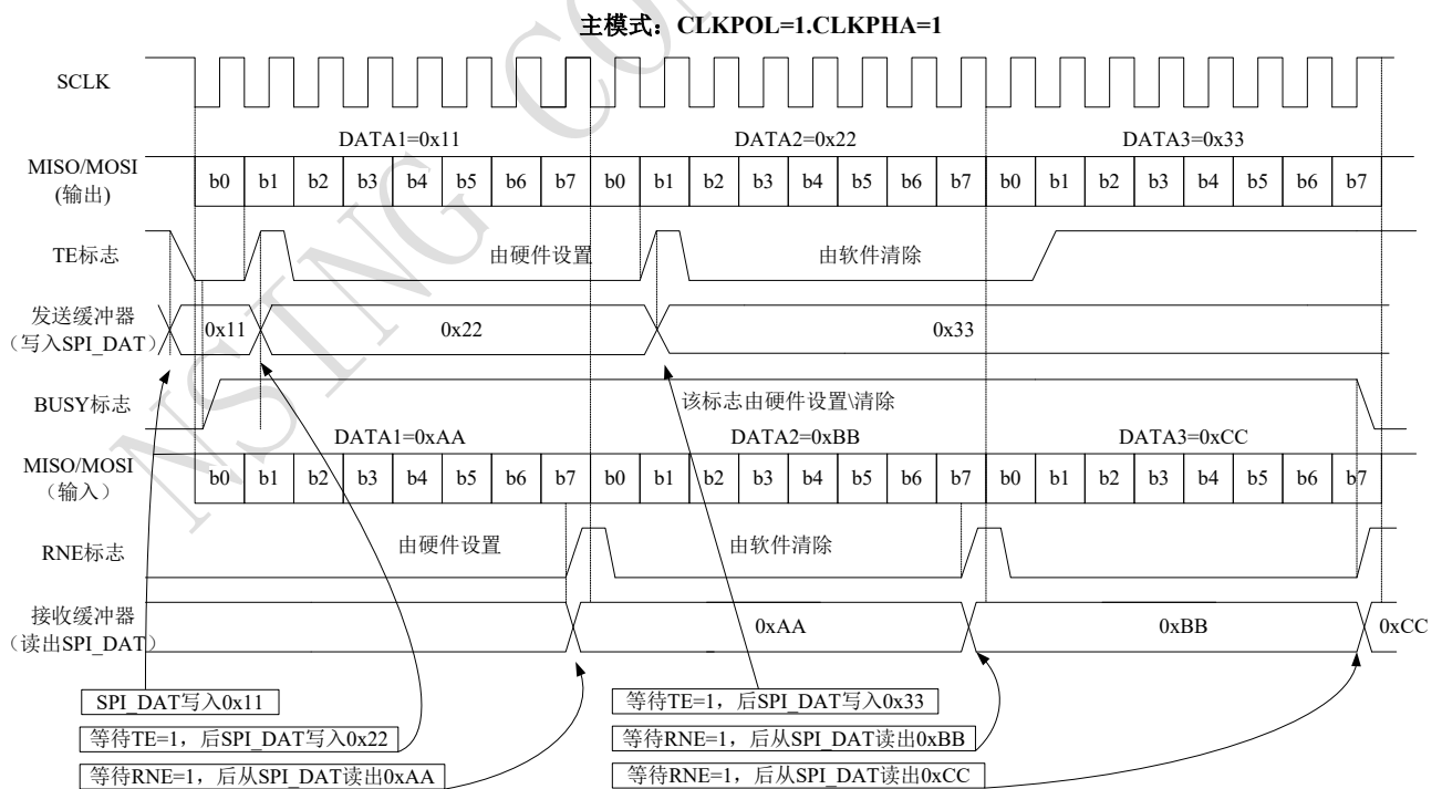
图 19-5 主机全双工模式下连续传输时, TE/RNE/BUSY 的变化示意图
