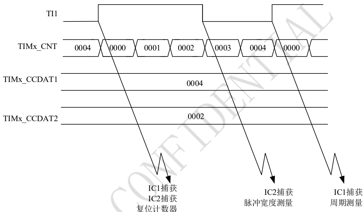
图 10-27 PWM 输入模式时序
