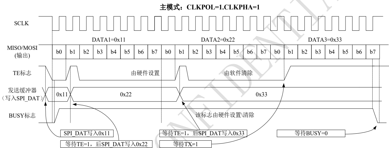
图 19-6 主机单向只发送模式下连续传输时，TE/BUSY 变化示意图
