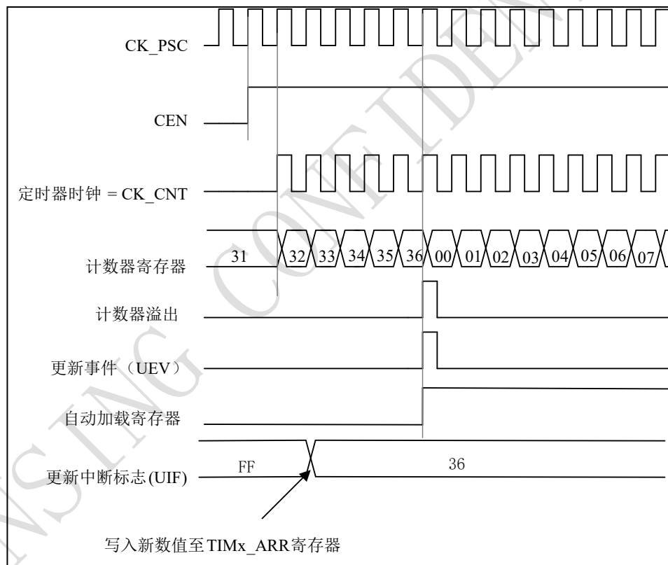
图 9-8 计数器时序图，当 ARPEN=0 时的更新事件 (TIMx_ARR 没有预装入)
