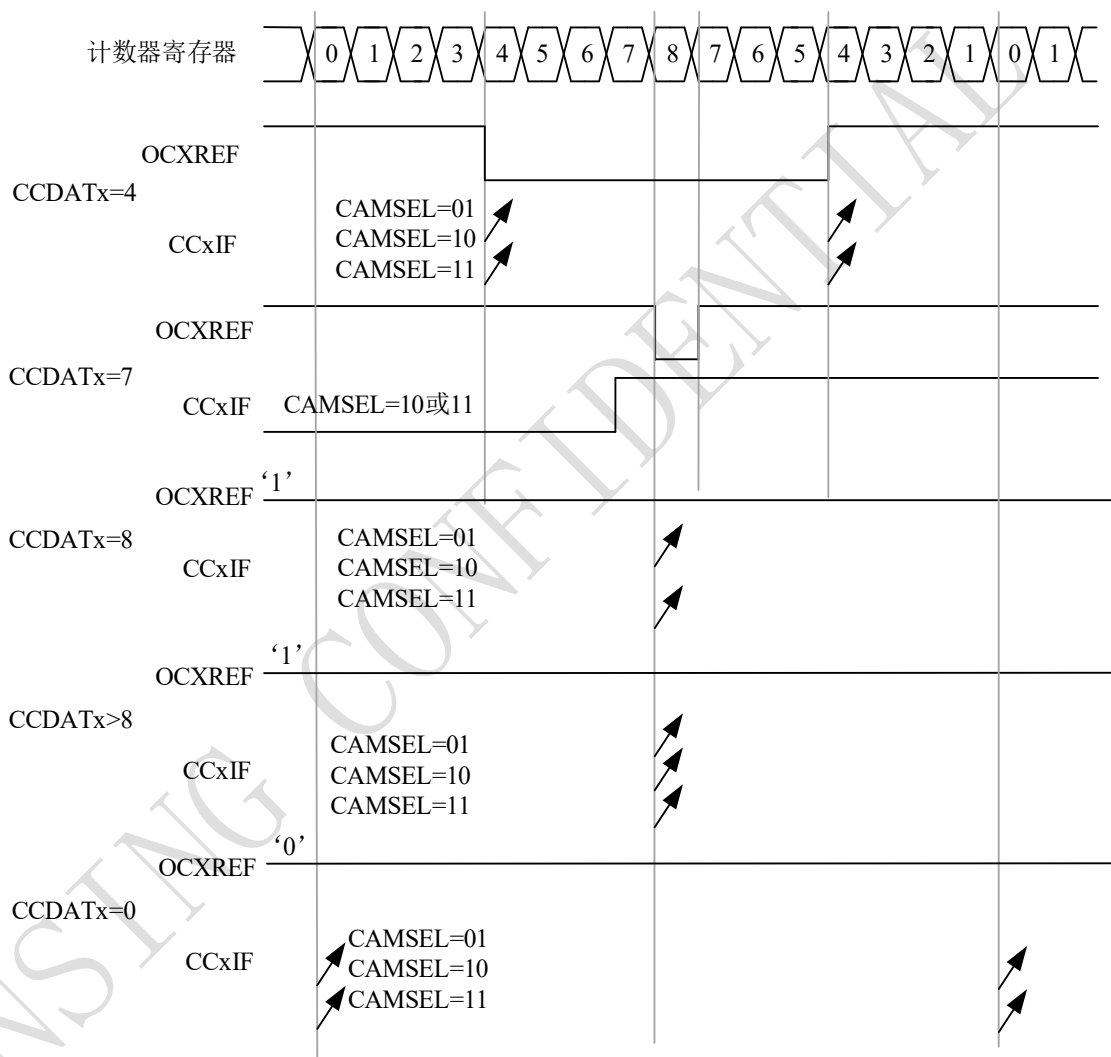
图 10-30 中央对齐的 PWM 波形（APR=8）
