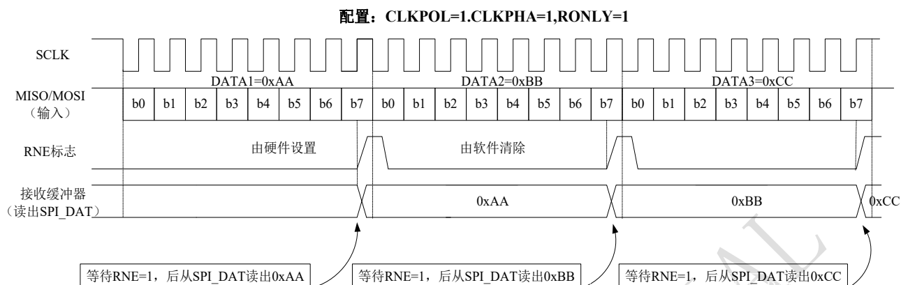
图 19-7 只接收模式（BIDIRMODE=0 并且 RONLY=1）下连续传输时，RNE 变化示意图
