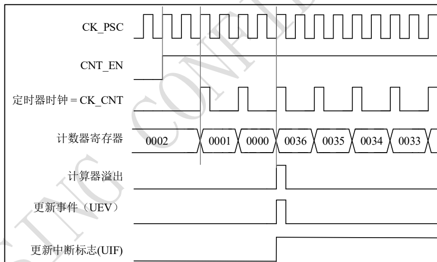
图 9-11 计数器时序图，内部时钟分频因子为 2
