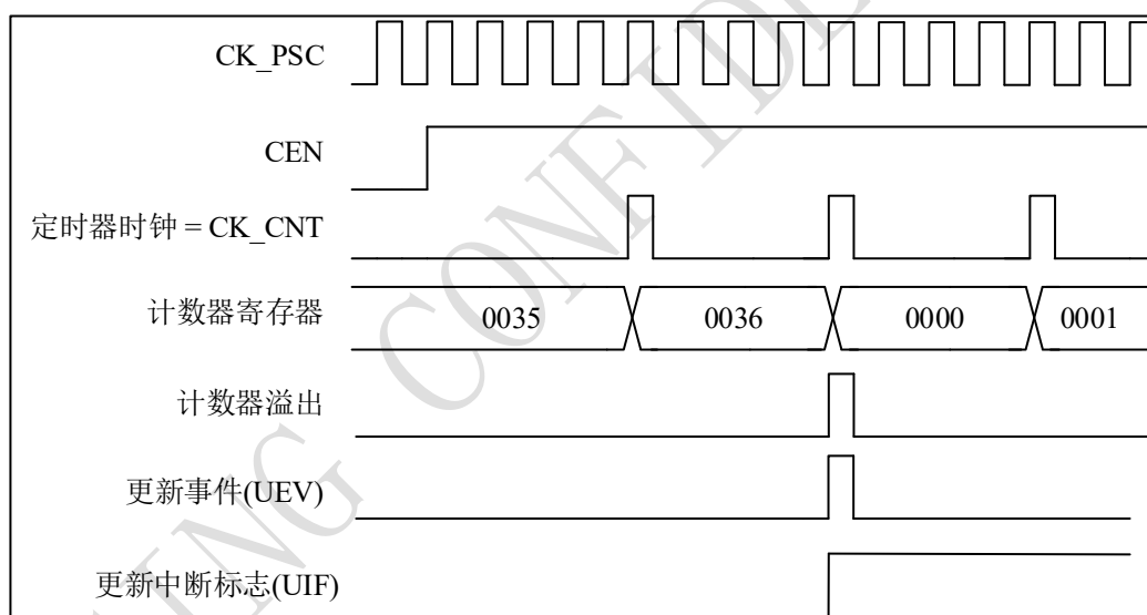
图 11-7 计数器时序图，内部时钟分频系数为 N
