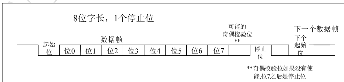
图 18-2 帧格式
