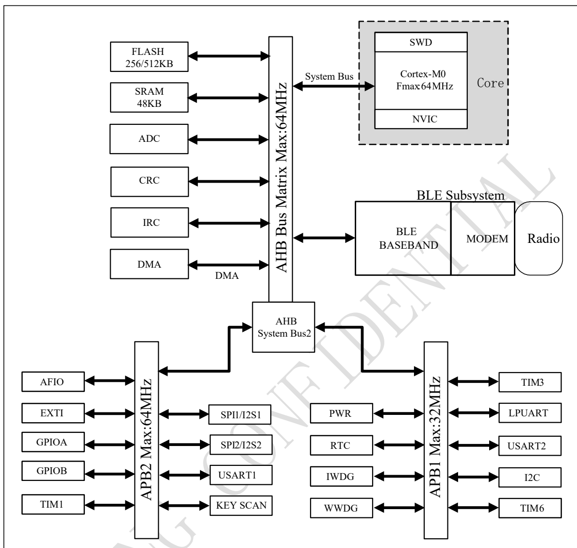
图 2-1 总线架构图
