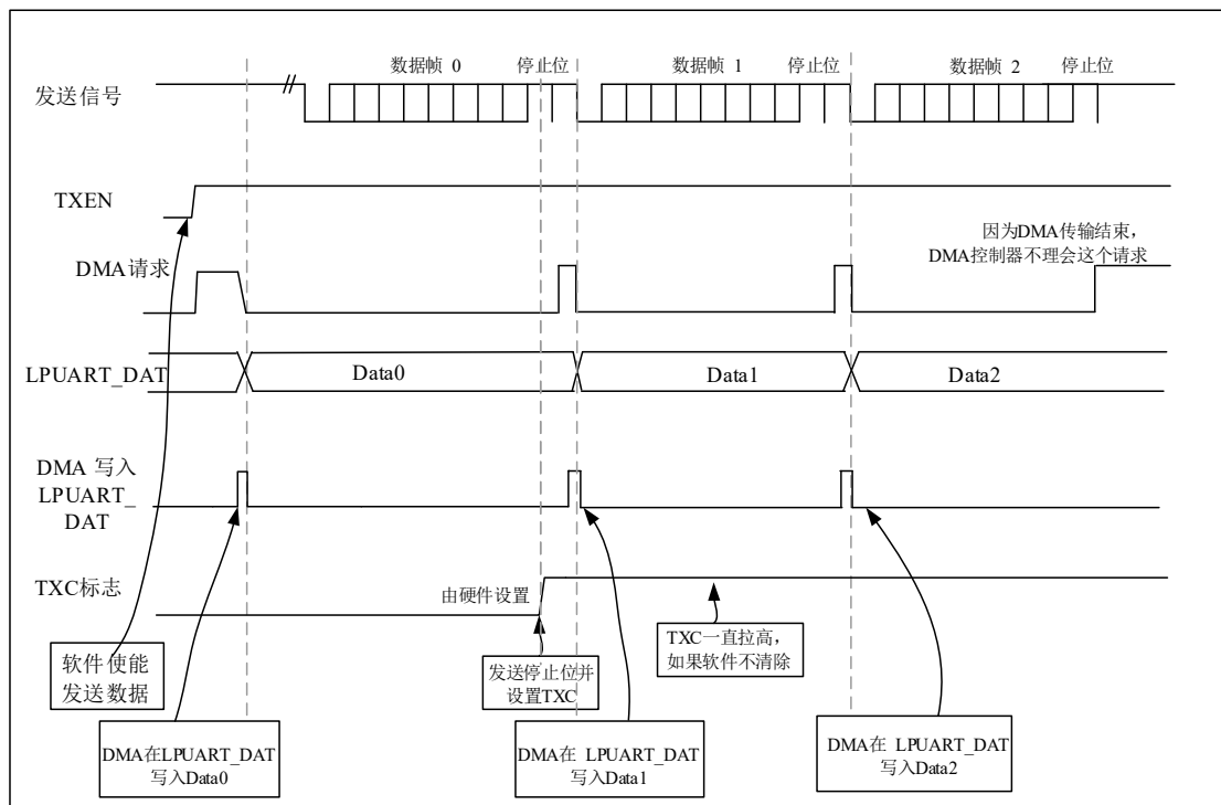
图 18-5 利用 DMA 发送
