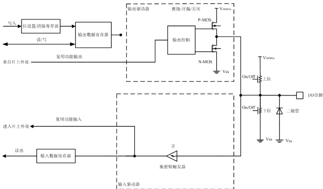
图 5-4 复用功能配置
