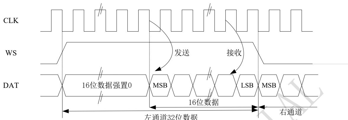
图 19-22 LSB 对齐 16 位数据扩展到 32 位包帧，CLKPOL = 0
