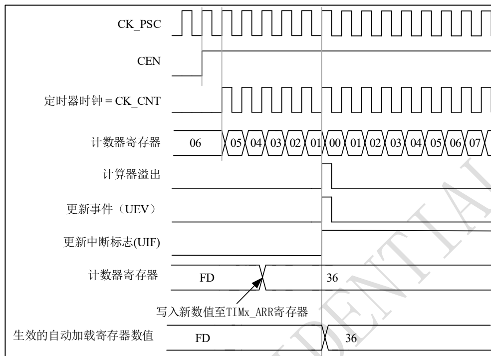
图 9-20 计数器时序图，ARPE=1 时的更新事件（计数器溢出）
