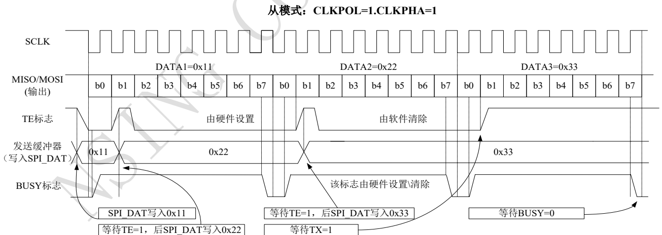
图 19-9 从机单向只发送模式下连续传输时，TE/BUSY 变化示意图
