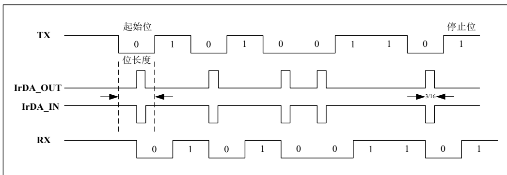
图 17-18 IrDA 数据调制 (3/16) - 普通模式
