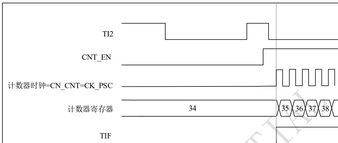
图 10-36 触发器模式下的控制电路
