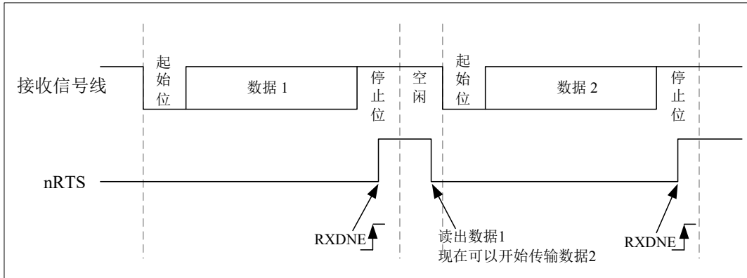
图 17-22 RTS 流控制
