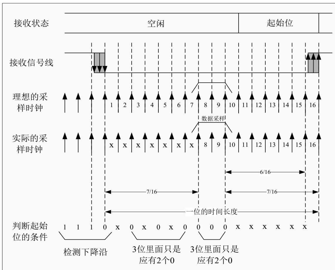
图 17-5 起始位检测
