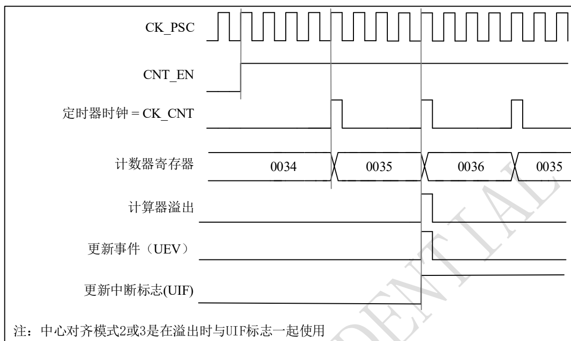
图 9-18 计数器时序图，内部时钟分频因子为 N
