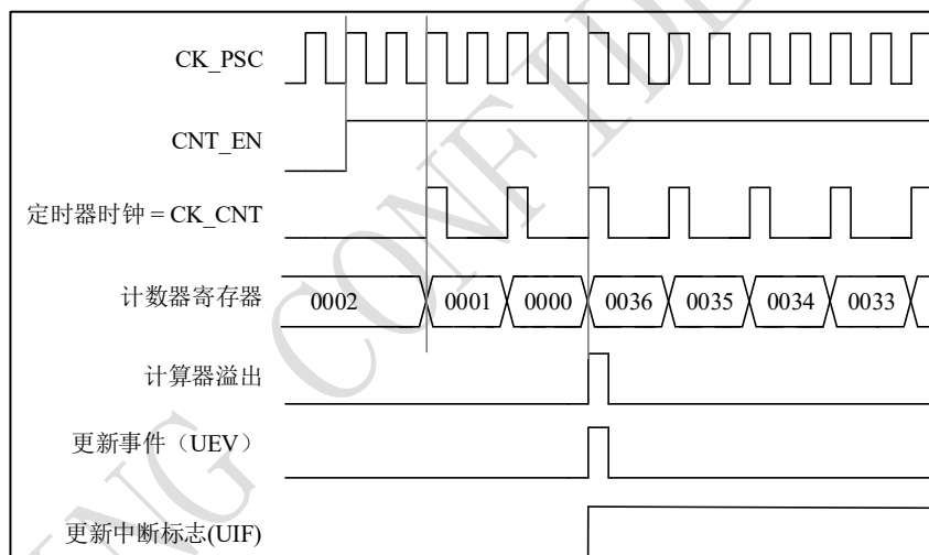
图 10-11 计数器时序图，内部时钟分频因子为 2
