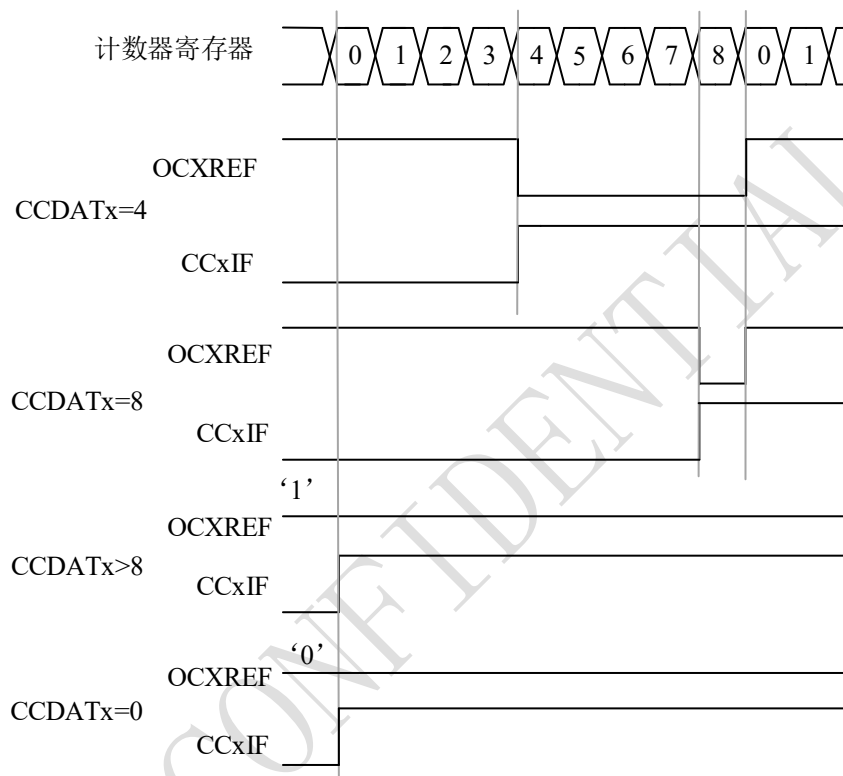
图 9-33 边沿对齐的 PWM 波形 (AR=8)
