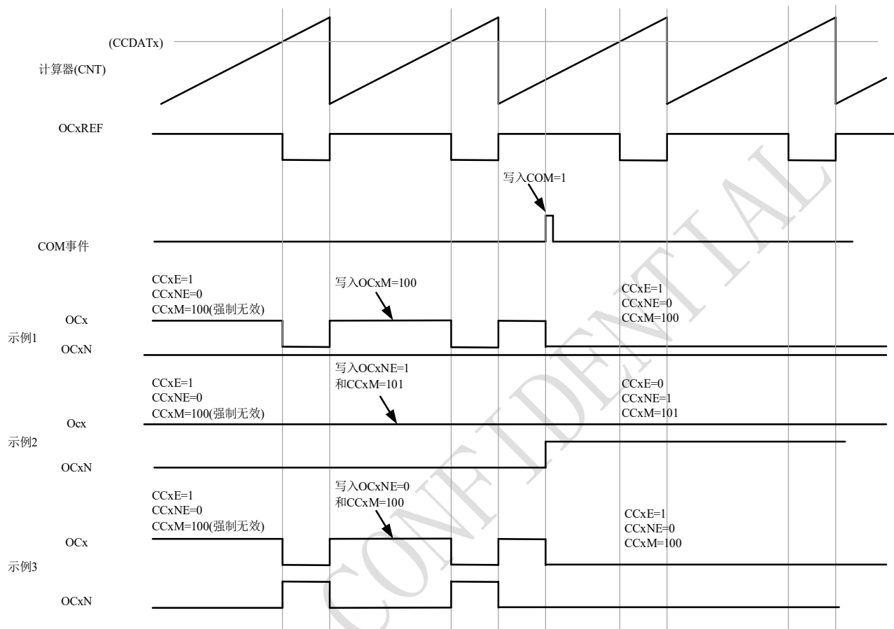
图 9-40 产生六步 PWM，使用 COM 的例子 (OSSR=1)
