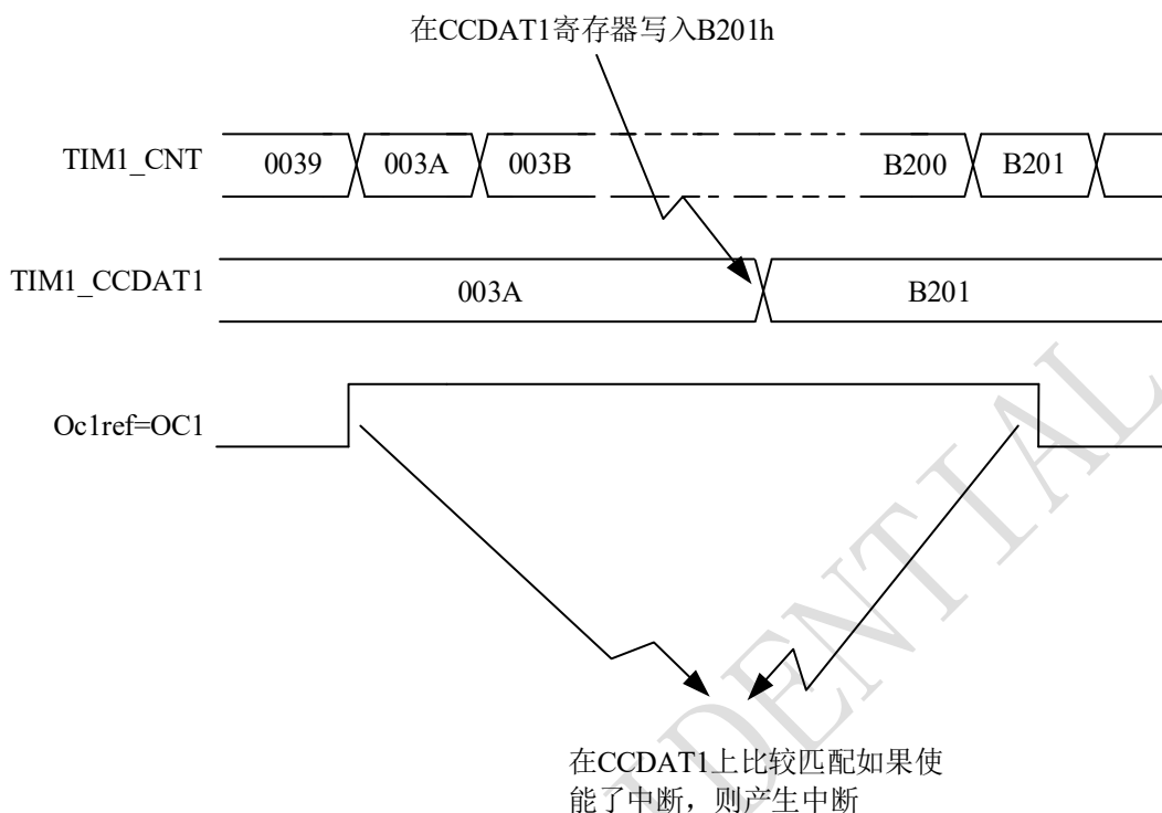
图 9-32 输出比较模式，翻转 OC1
