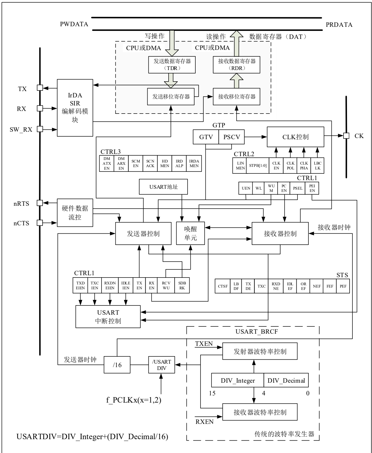
图 17-1 USART 框图
