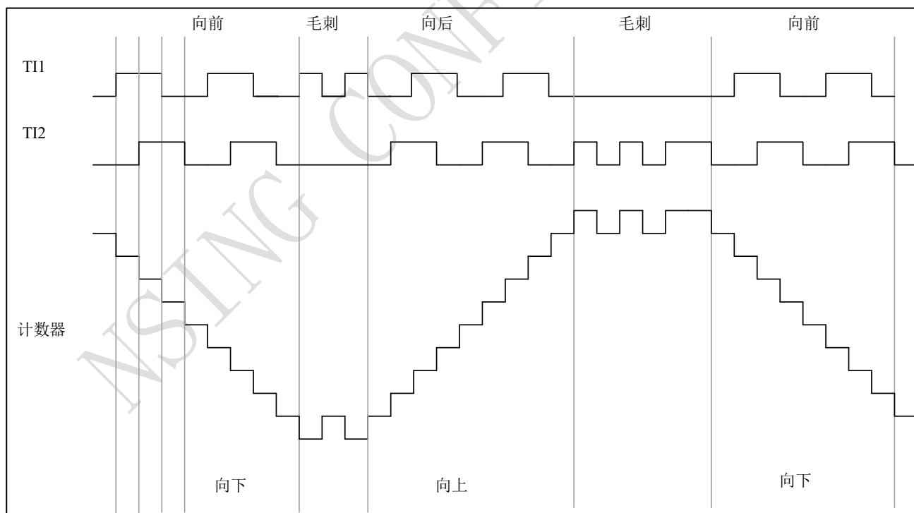
图 10-33 IC1FP1 反相的编码器接口模式实例
