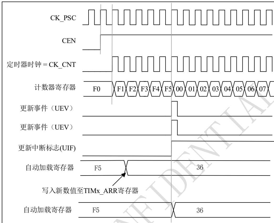
图 11-9 计数器时序图，当 ARPEN=1 时的更新事件（预装载 TIMx_AR）
