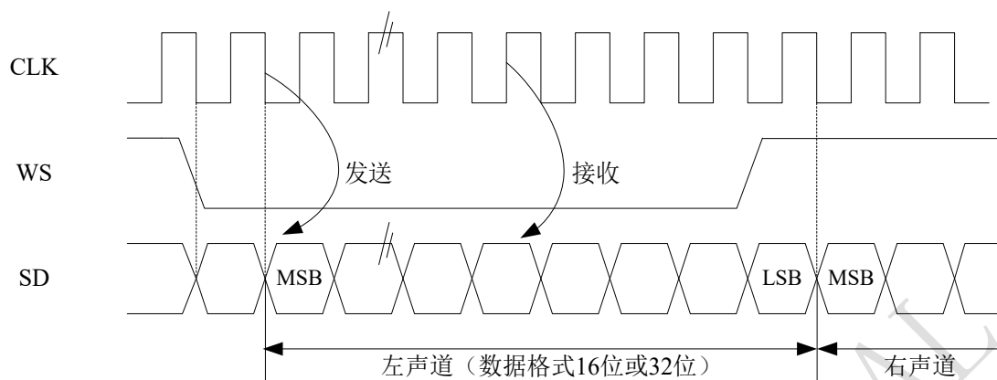
图 19-14 I 2 S 飞利浦协议波形（16/32 位全精度，CLKPOL = 0）
