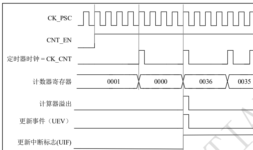
图 9-13 计数器时序图，内部时钟分频因子为 N
