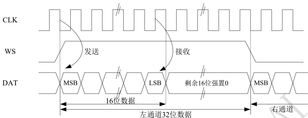
图 19-19 MSB 对齐 16 位数据扩展到 32 位包帧，CLKPOL = 0
