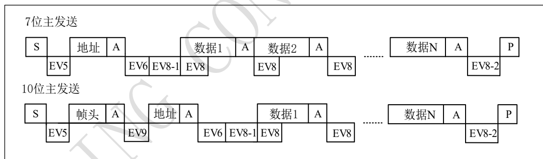
图 16-5 主发送器传送序列图
