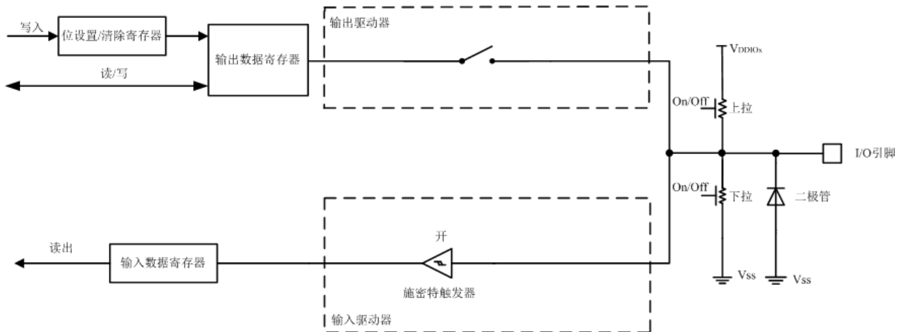
图 5-2 输入浮空/上拉/下拉配置
