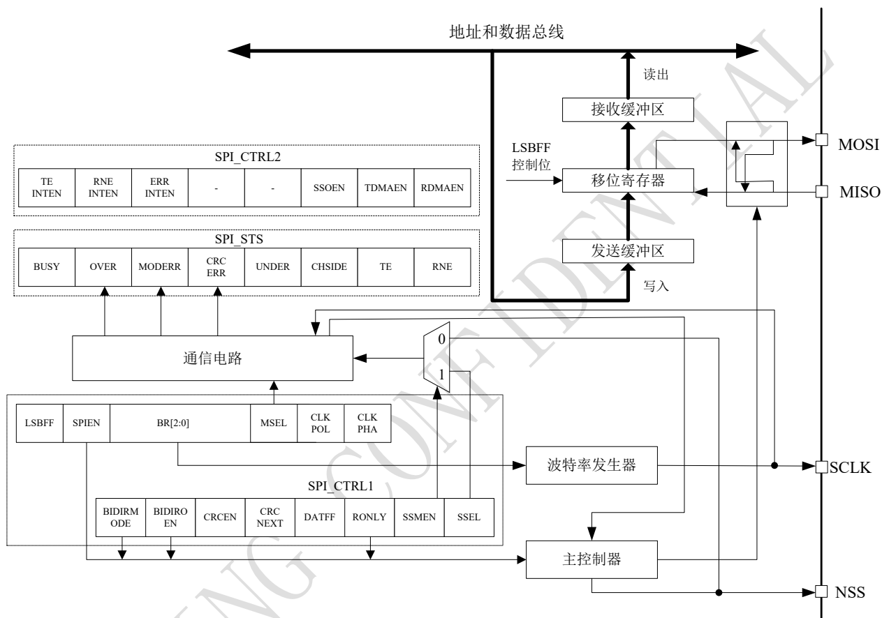
图 19-1 SPI 框图
