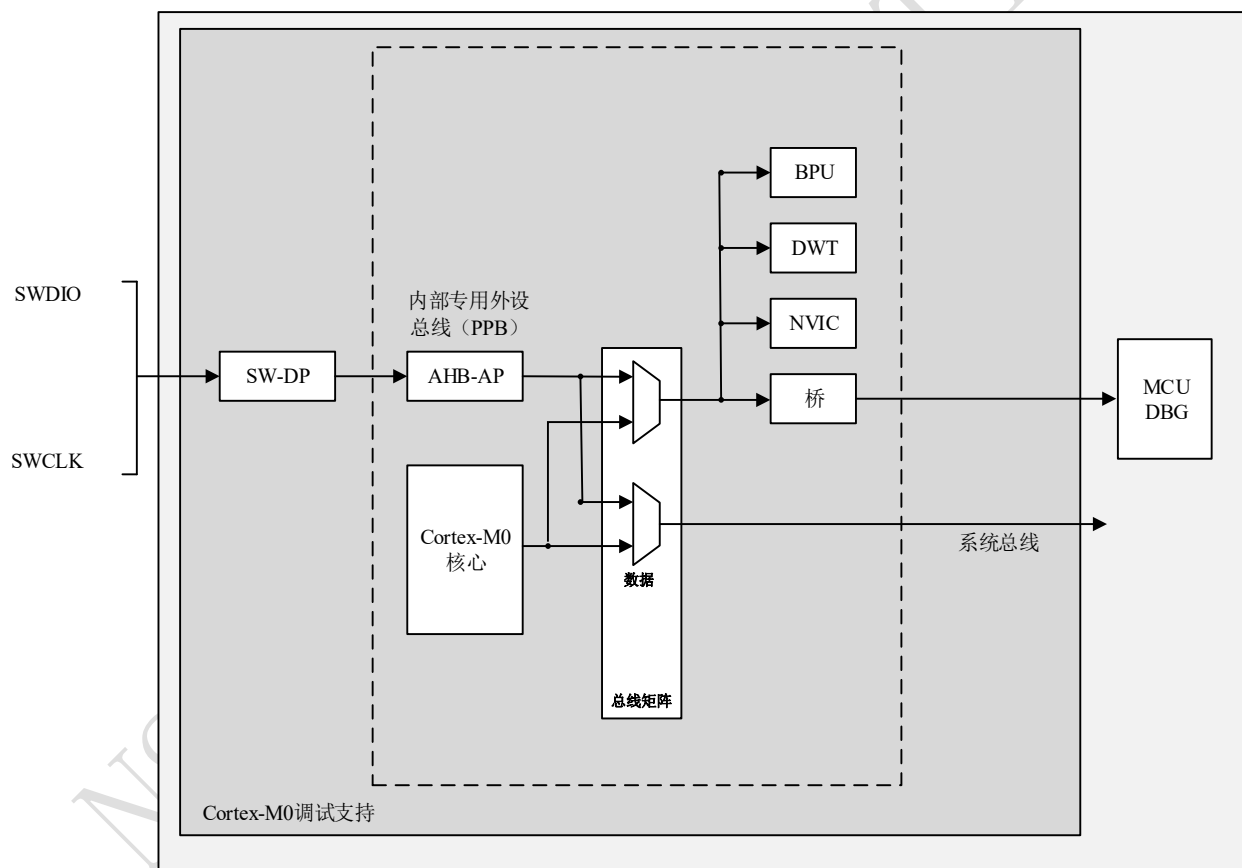
图 23-1 N32WB03x 级别和 Cortex®-M0 级别的调试框图
