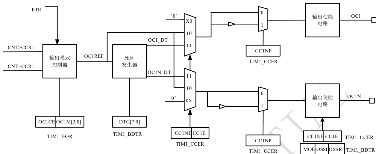
图 9-30 捕获/比较通道的输出部分（通道 4）
