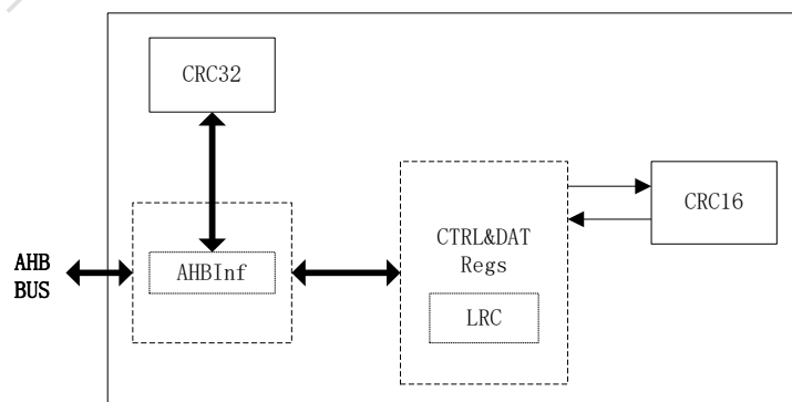
图 8-1 CRC 计算单元框图
