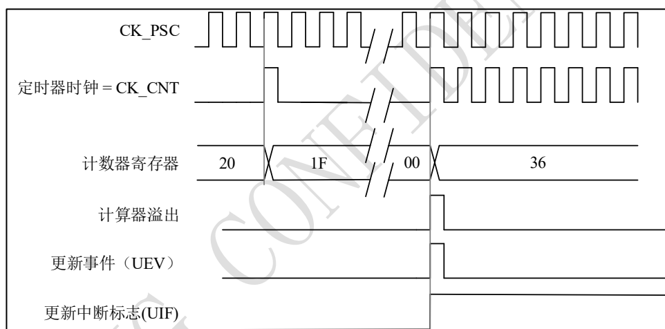
图 9-13 计数器时序图，内部时钟分频因子为 N
