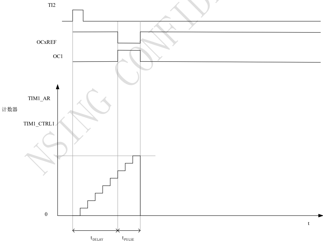
图 10-31 单脉冲模式的例子
