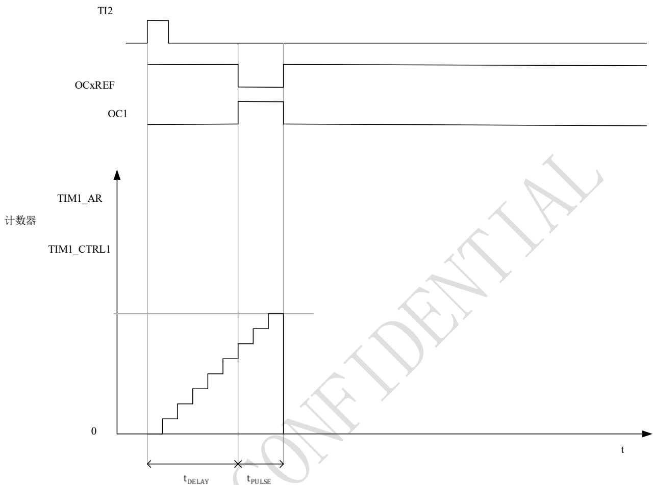
图 9-41 单脉冲模式的例子
