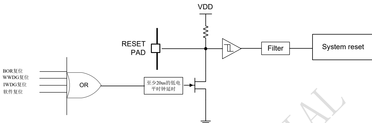
图 4-1 复位电路
