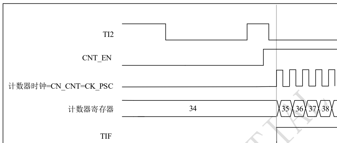
图 9-47 触发器模式下的控制电路
