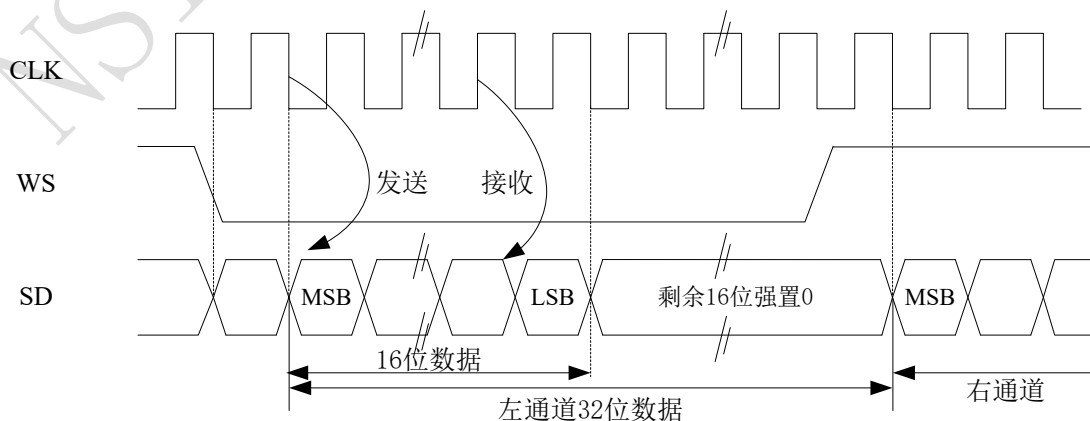
图 19-16 I 2 S 飞利浦协议标准波形（16 位扩展至 32 位包帧，CLKPOL = 0）
