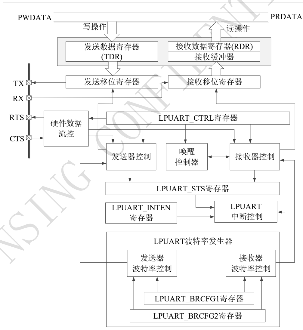
图 18-1 LPUART 框图
