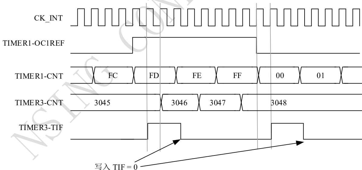
图 10-38 定时器 1 的 OC1REF 控制定时器 3
