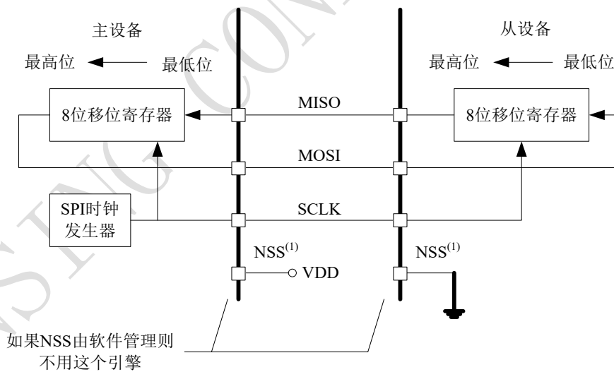
图 19-3 单主和单从应用
