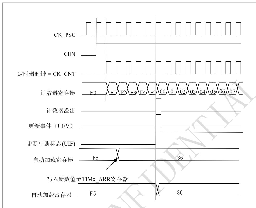
图 9-9 计数器时序图，当 ARPEN=1 时的更新事件（预装入了 TIMx_AR）
