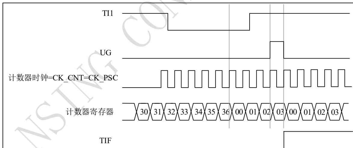
图 9-45 复位模式下的控制电路
