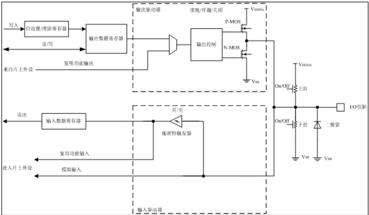
图 5-1 I/O 端口的基本结构
