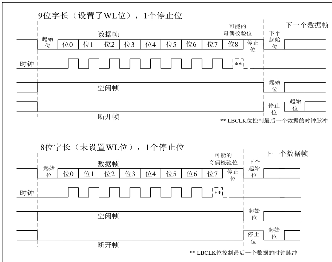
图 17-2 字长设置
