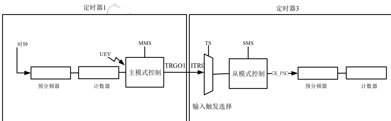
图 10-37 主/从定时器的例子
