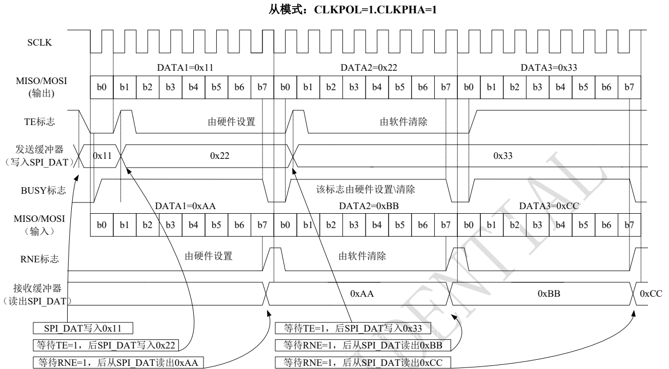
图 19-8 从机全双工模式下连续传输时，TE/RNE/BUSY 的变化示意图
