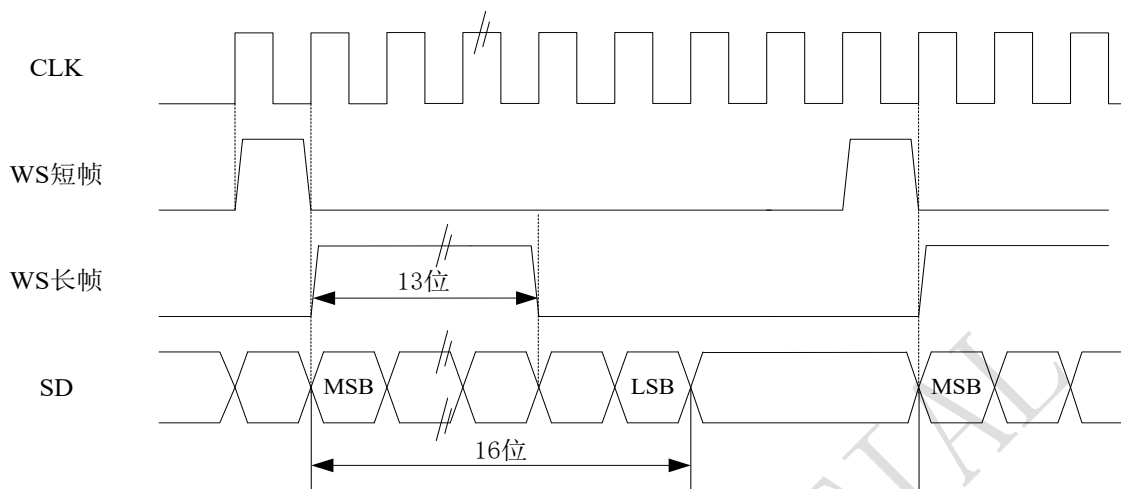
图 19-24 PCM 标准波形（16 位扩展到 32 位包帧）
