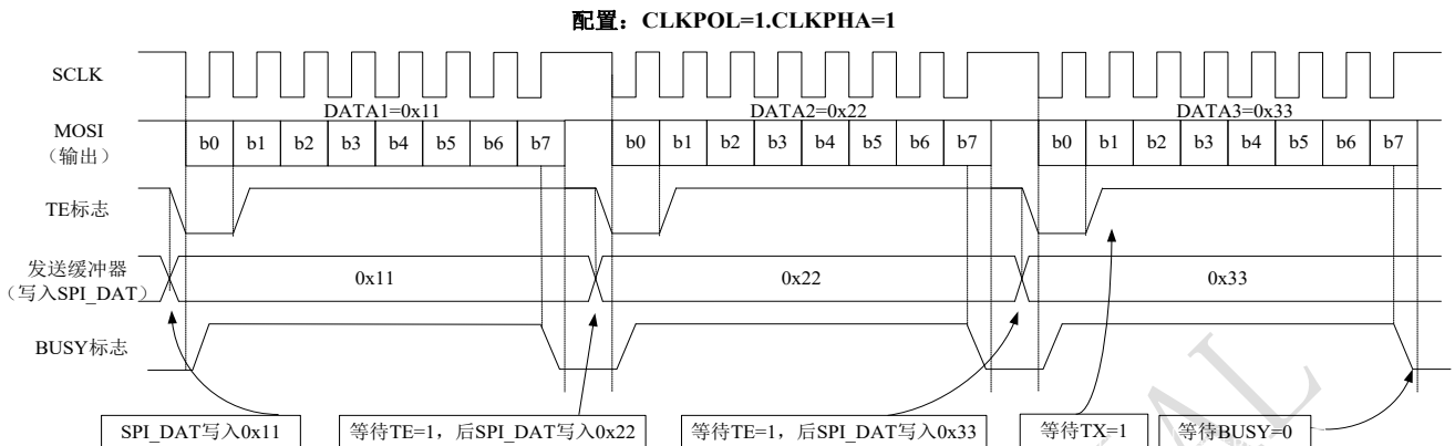
图 19-10 BIDIRMODE=0, RONLY=0 非连续传输发送时, TE/BUSY 变化示意图
