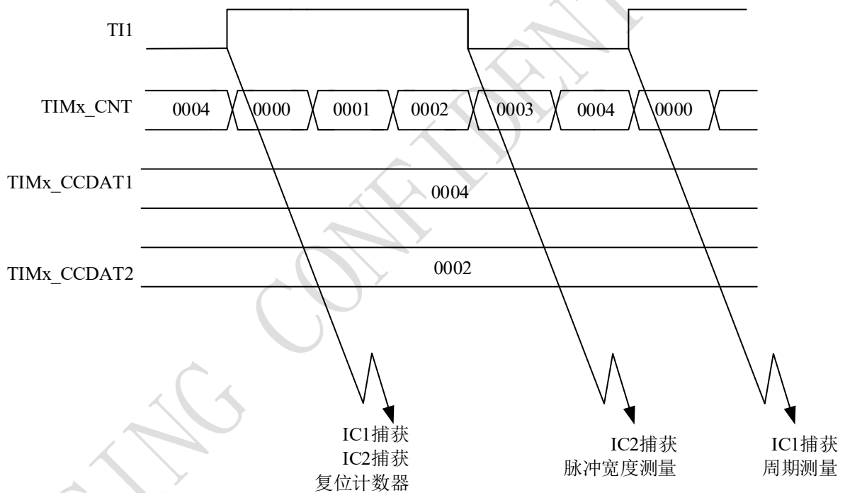
图 9-31 PWM 输入模式时序
