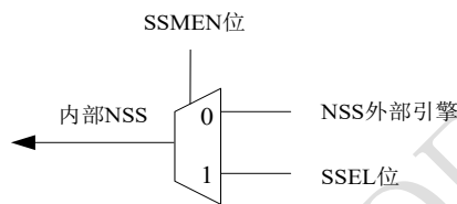
图 19-2 硬件/软件的从选择管理
