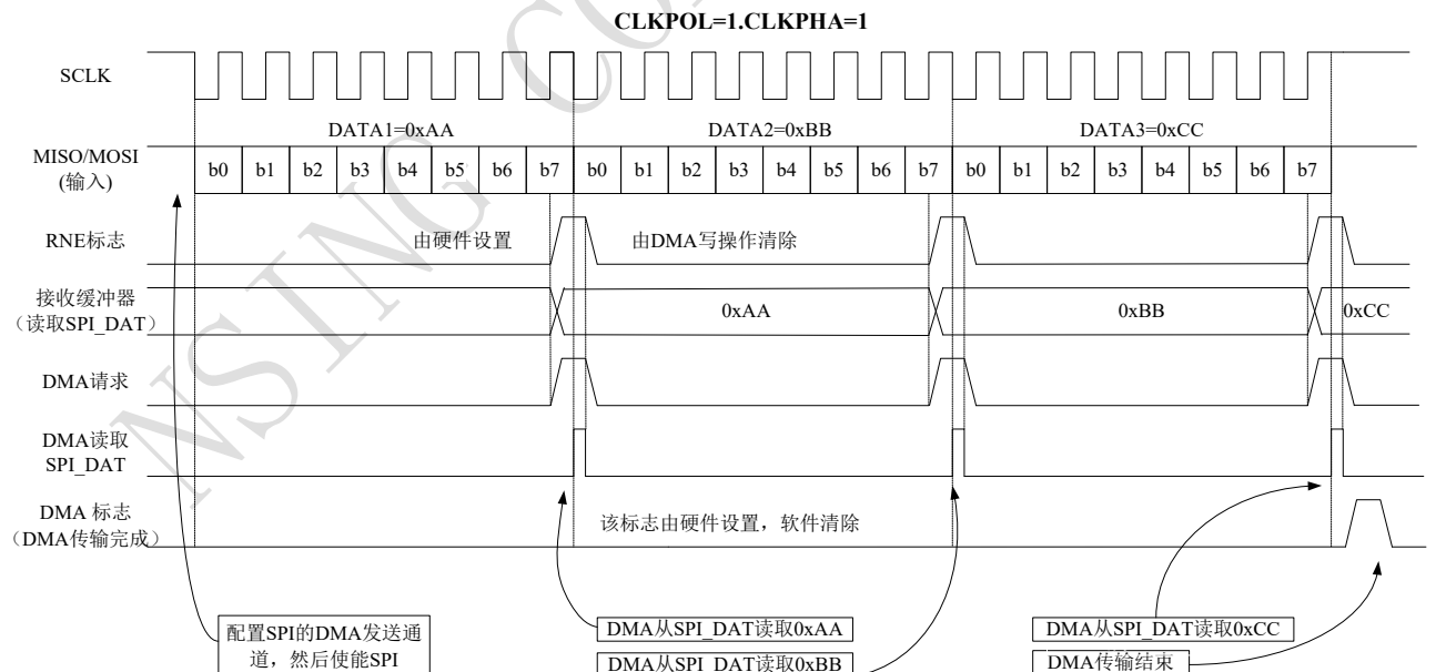
图 19-12 使用 DMA 接收
