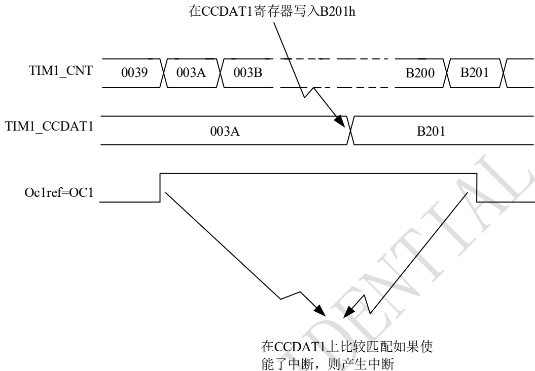
图 10-28 输出比较模式，翻转 OC1
