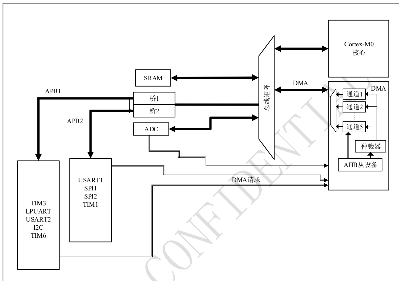
图 7-1 DMA 框图
