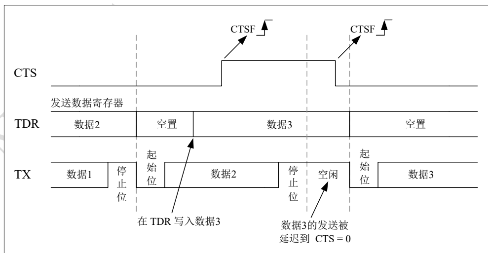
图 17-23 CTS 流控制
