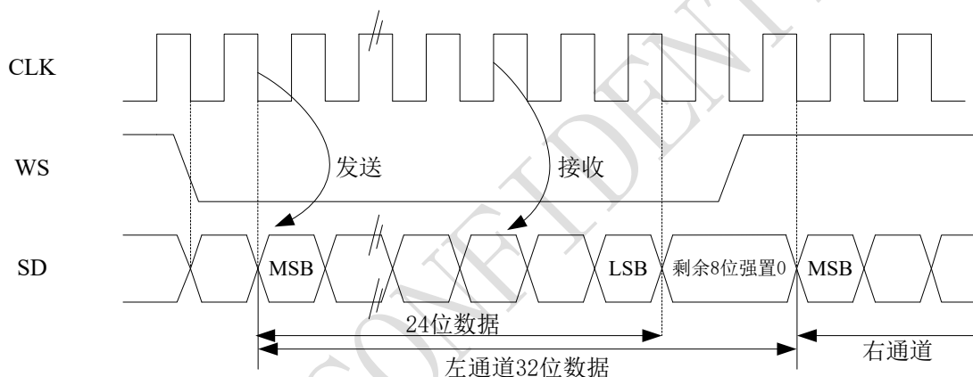
图 19-15 I 2 S 飞利浦协议标准波形（24 位帧，CLKPOL = 0）
