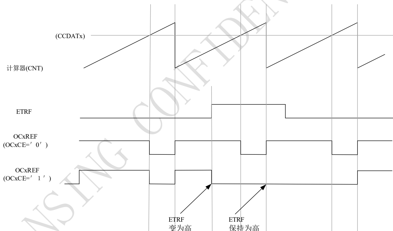
图 9-39 清除 TIMx 的 OCxREF
