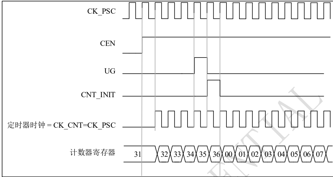
图 11-10 普通模式时序图，内部时钟分频系数为 1
