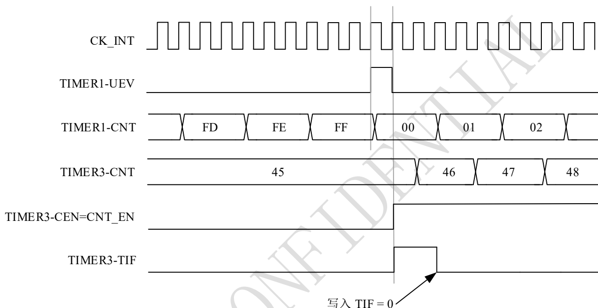
图 10-40 使用定时器 1 的更新触发定时器 3
