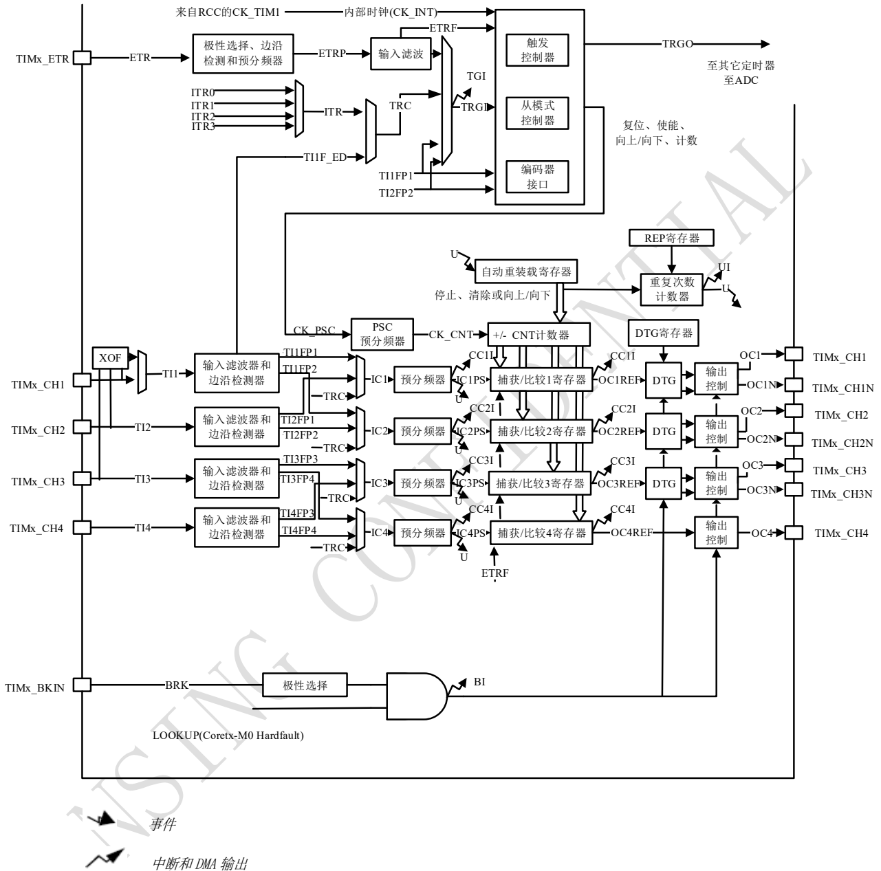
图 9-1 高级控制定时器框图
