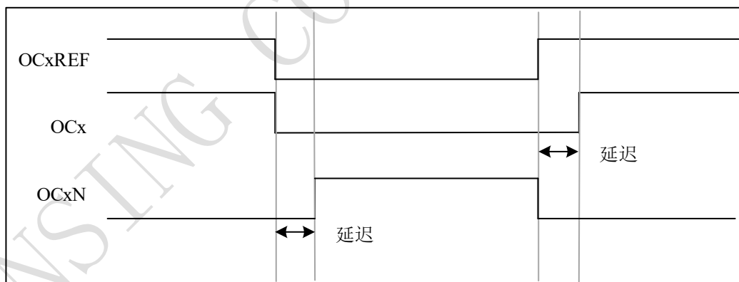
图 9-35 带死区插入的互补输出
