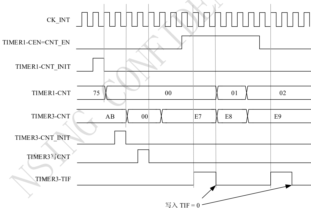
图 10-39 通过使能定时器 1 可以控制定时器 3
