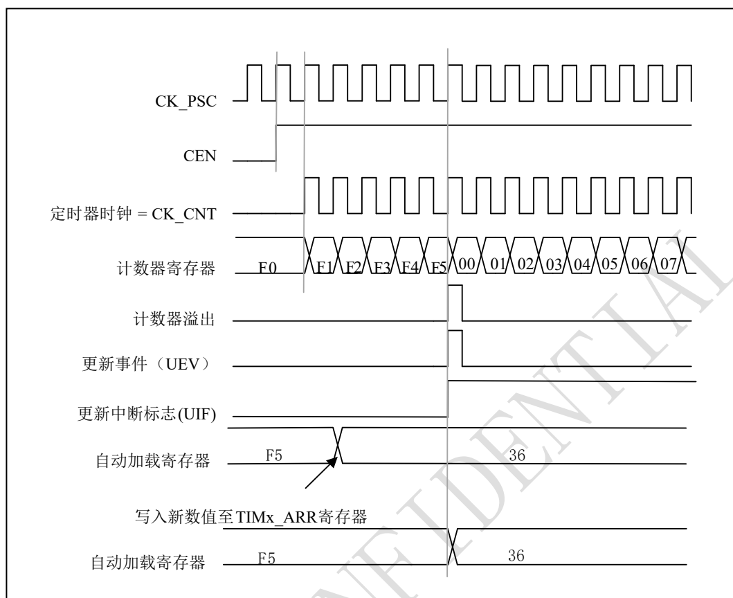
图 10-9 计数器时序图，当 ARPEN=1 时的更新事件（预装入了 TIMx_AR）
