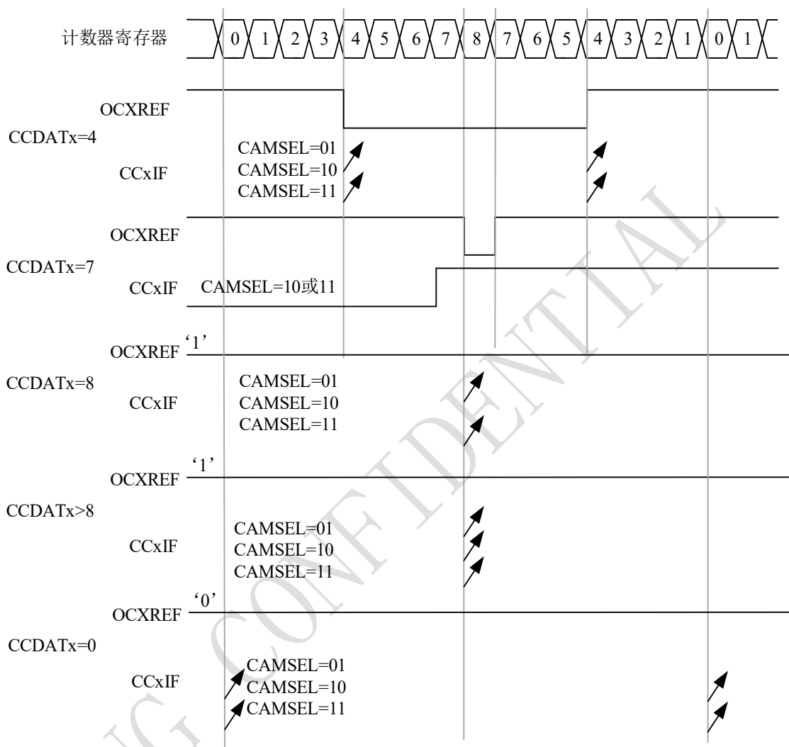
图 9-34 中央对齐的 PWM 波形 (APR=8)
