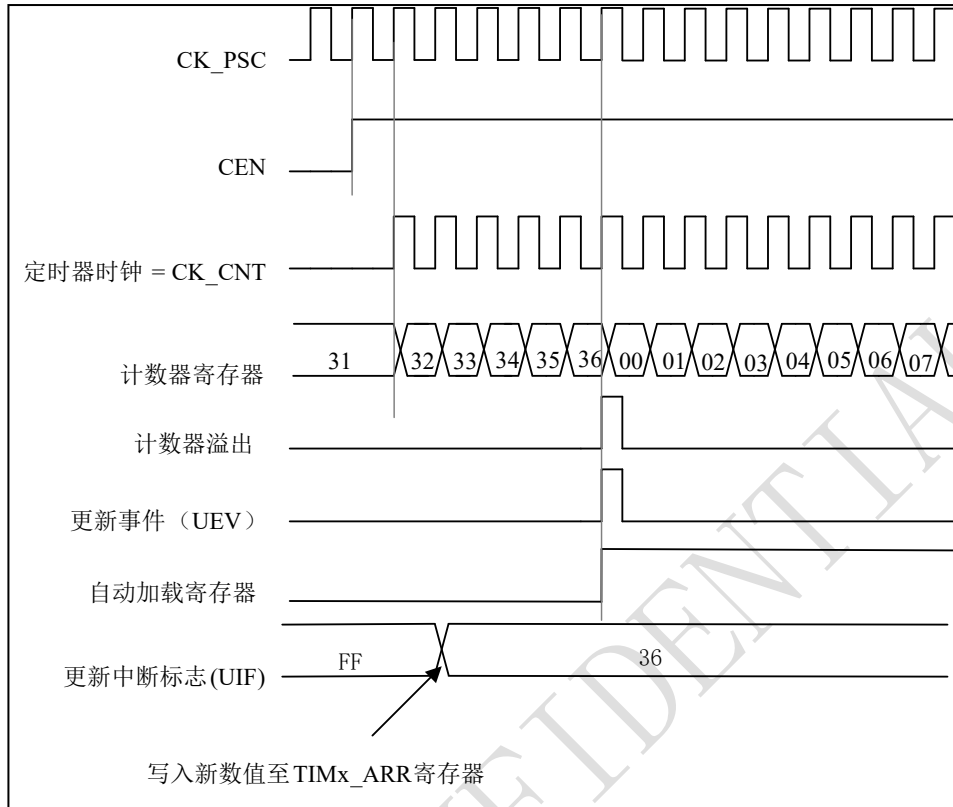
图 10-8 计数器时序图，当 ARPEN=0 时的更新事件（TIMx_AR 没有预装入）
