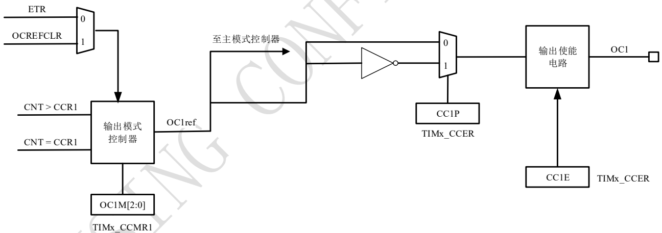
图 10-26 捕获/比较通道的输出部分（通道 1）
