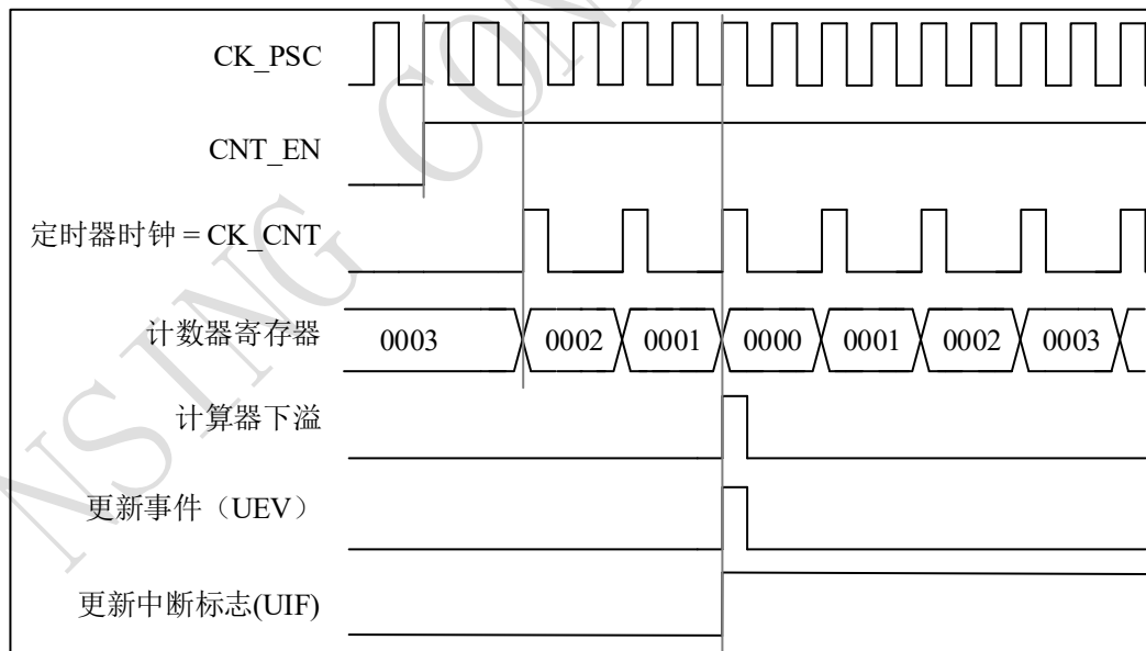
图 9-16 计数器时序图，内部时钟分频因子为 2
