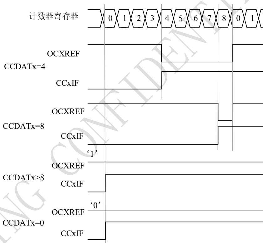
图 10-29 边沿对齐的 PWM 波形 (AR=8)
