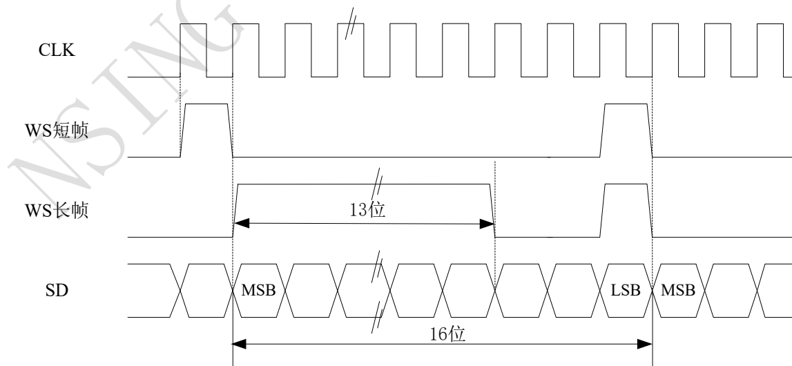
图 19-23 PCM 标准波形（16 位）
