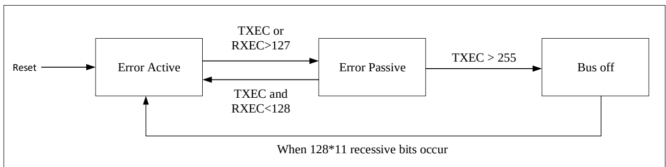
图 21-14 CAN 错误状态框图
