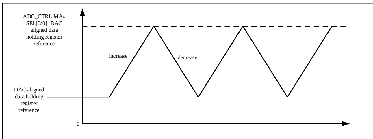
图 11-8 带三角生成的 DAC 转换（使能软件触发）
