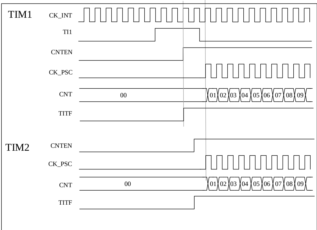
图 13-26 使用定时器 1 的 TI1 输入触发定时器 1 和定时器 2
