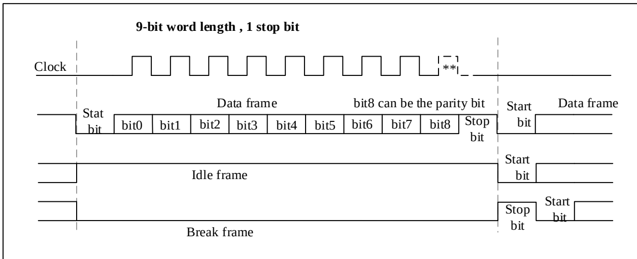
图 24-3 字长=9 设置
