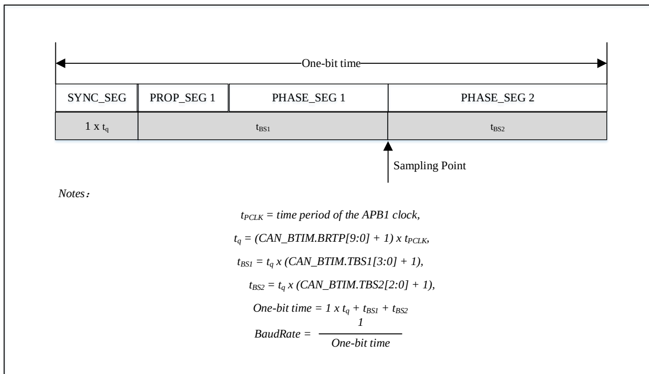
图 21-11 位时序
