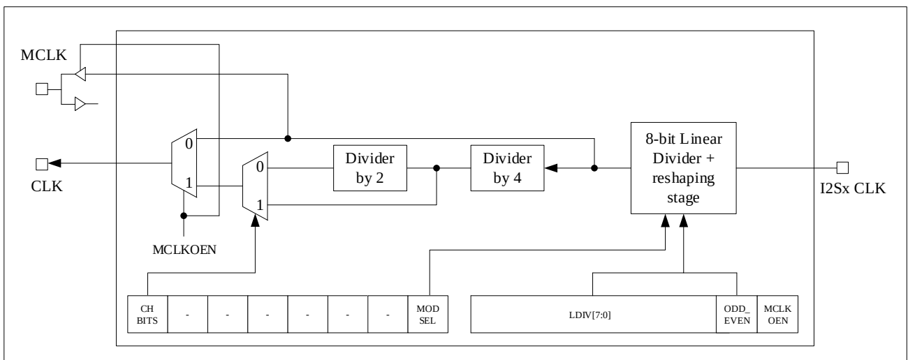
图 22-25 I 2 S 时钟发生器结构
