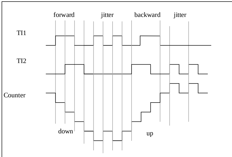
图 13-28 IC1FP1 反相的编码器接口模式实例
