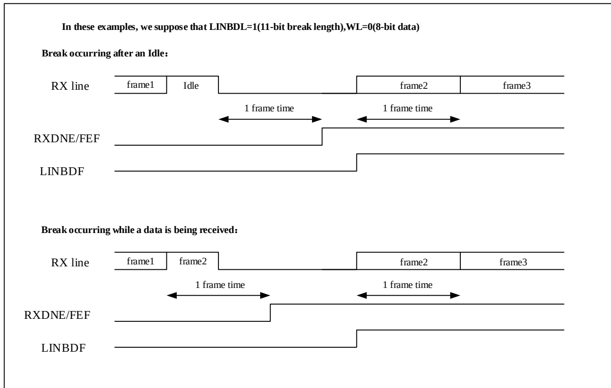
图 24-22 LIN 模式下的断开检测与帧错误的检测
