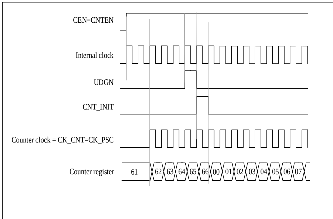
图 14-5 正常模式下的控制电路，内部时钟分频系数为 1
