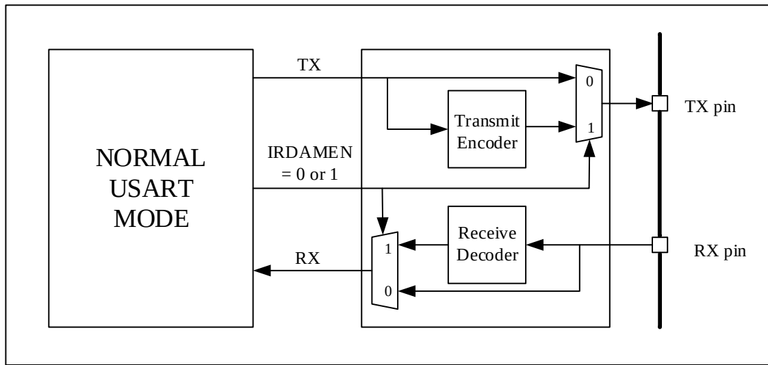
图 24-20 IrDA 数据调制 (3/16)-正常模式
