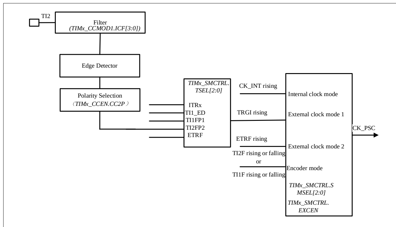
图 12-12 TI2 外部时钟连接示例
