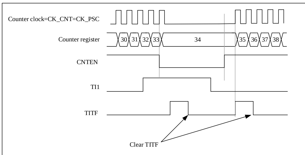
图 12-30 门控模式下的控制电路
