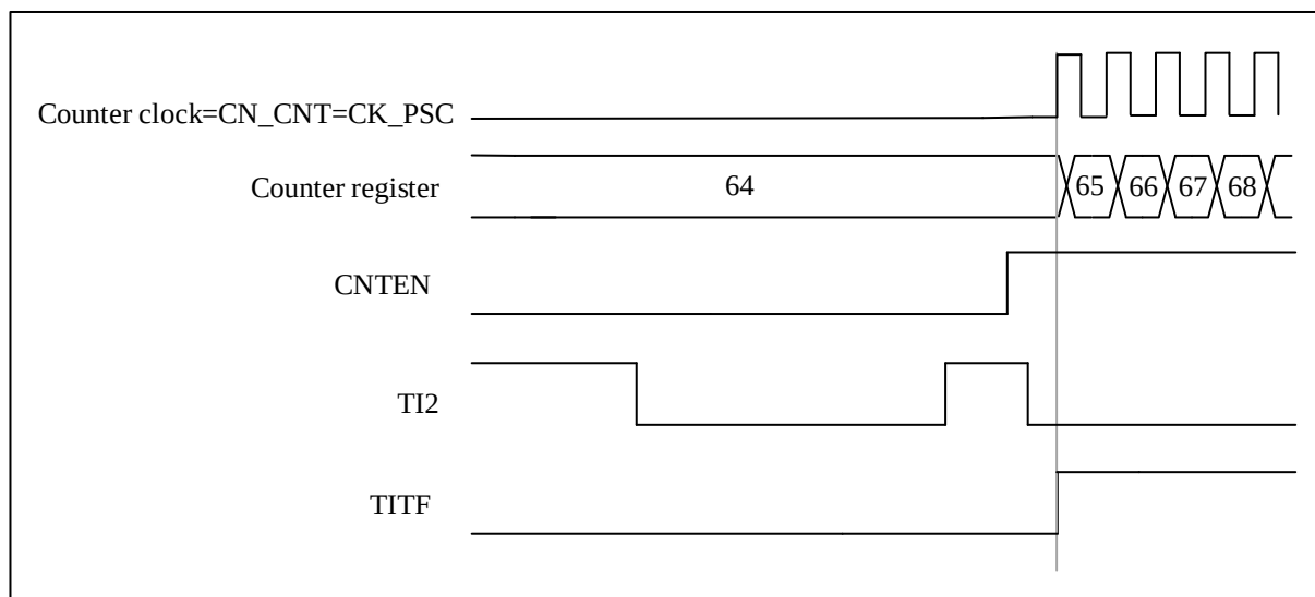
图 12-29 触发器模式下的控制电路
