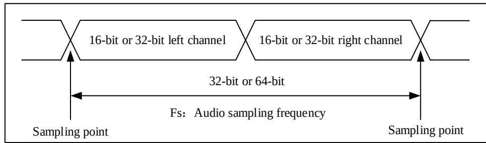
图 22-26 音频采样频率定义
