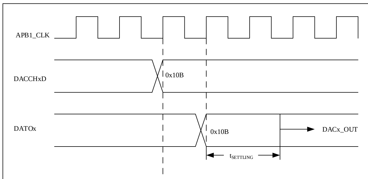
图 11-4 触发禁用时转换的时间框图
