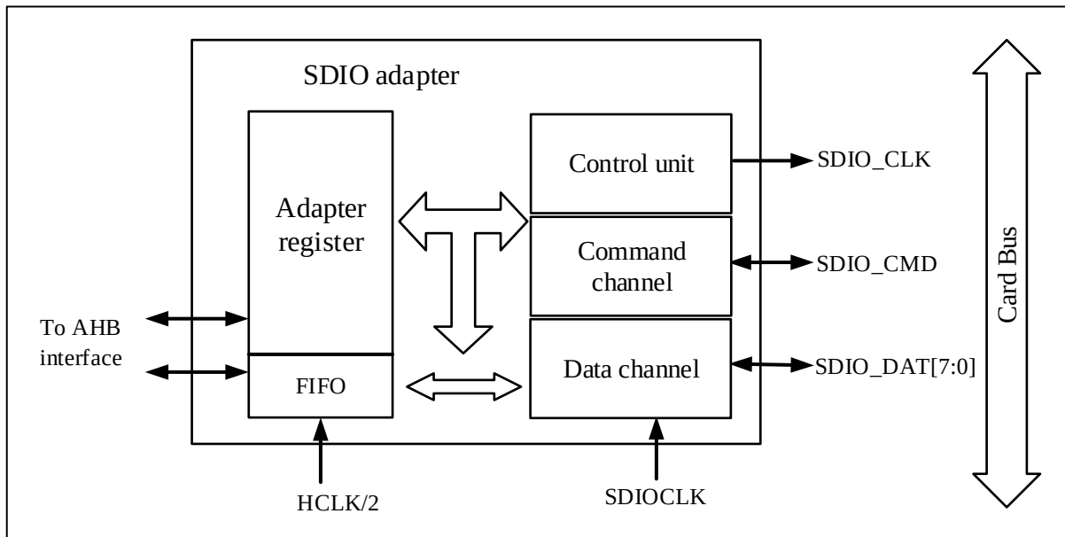
图 19-7 SDIO 适配器
