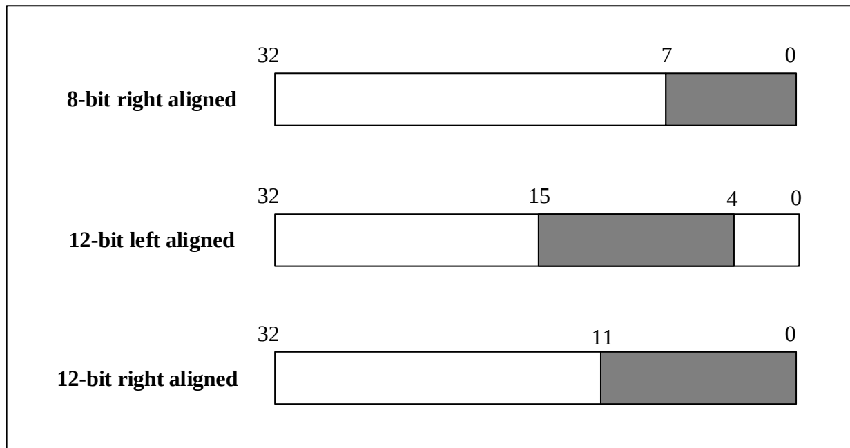
图 11-2 DAC 独立输出时的数据格式
