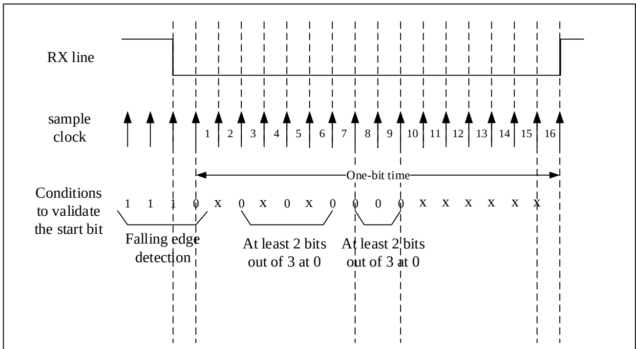
图 24-7 起始位检测
