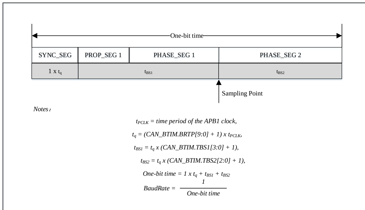
图 21-11 位时序
