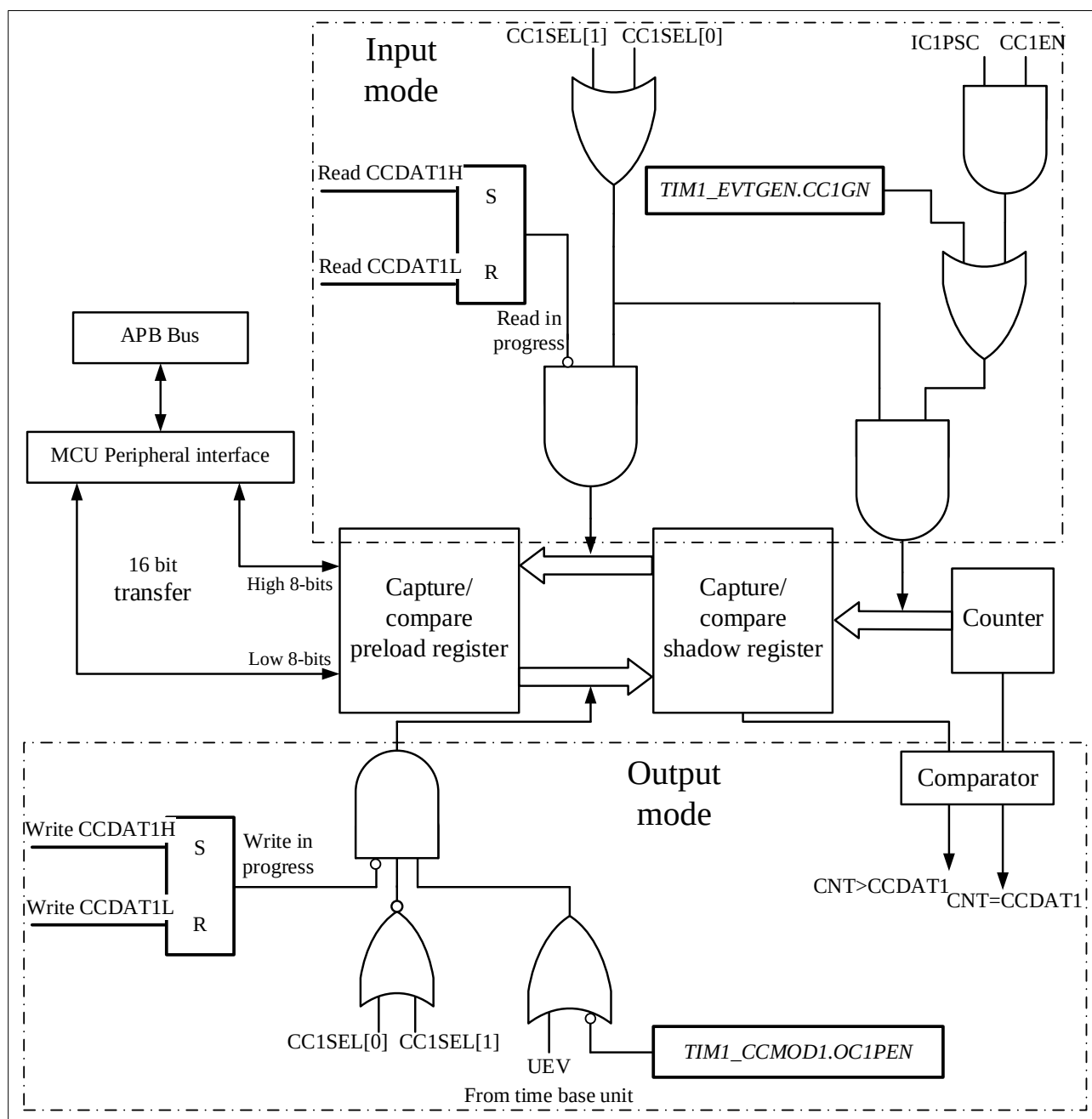
图 12-17 捕获/比较通道 1 主电路
