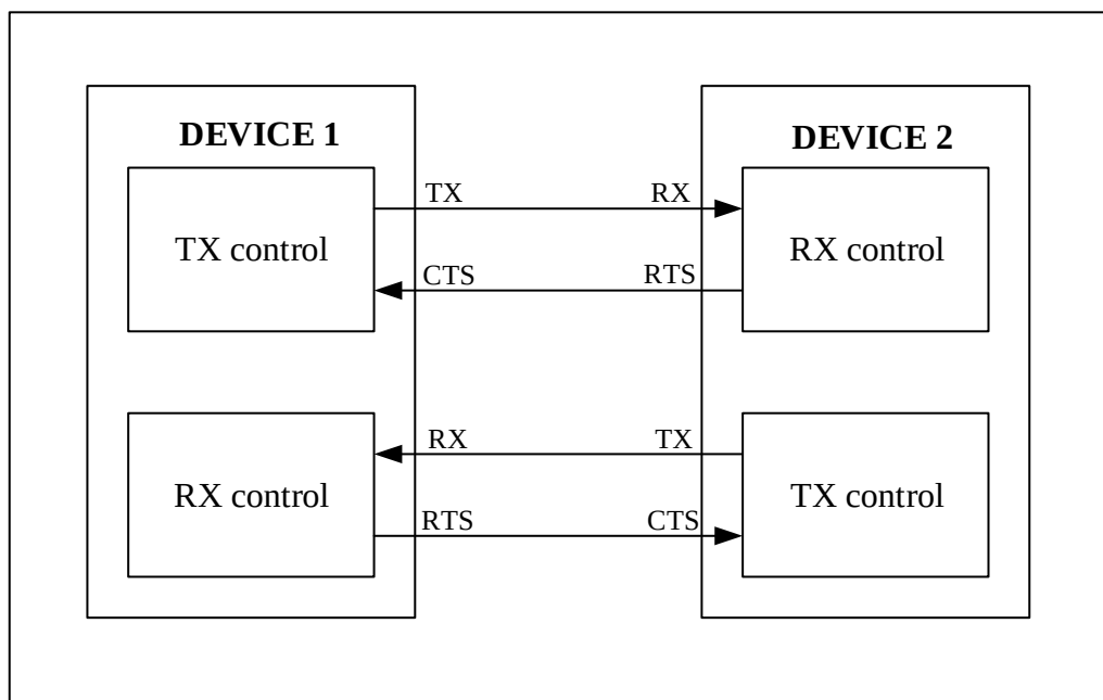
图 24-10 两个 USART 间的硬件流控制
