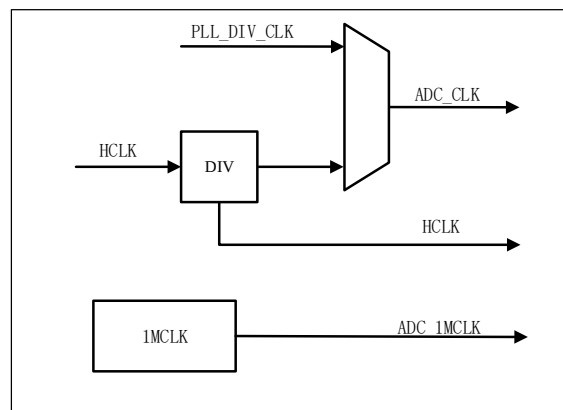
图 10-2 ADC 时钟
