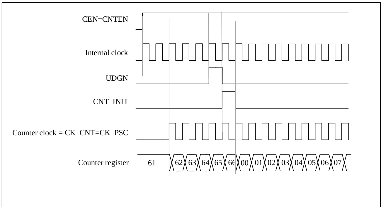
图 12-11 正常模式下的控制电路，内部时钟除以 1
