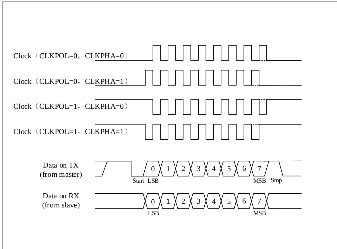
图 24-16 USART 数据时钟时序示例 (WL=0)
