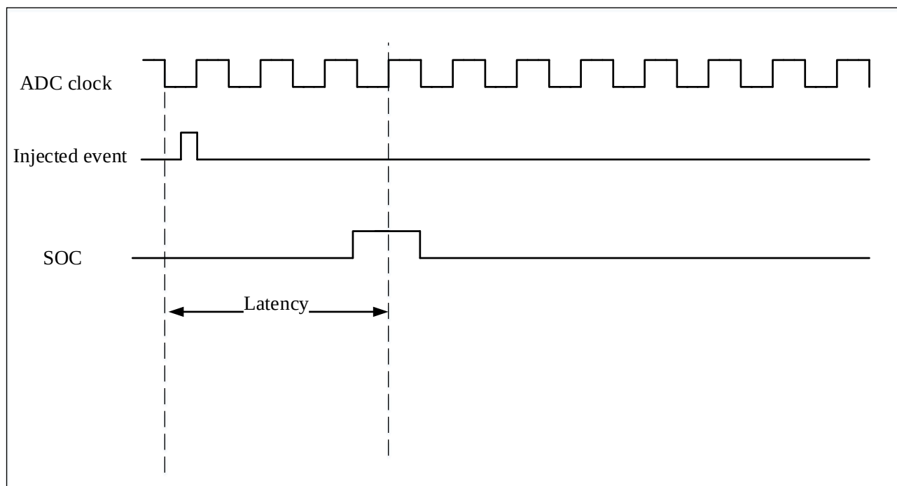
图 10-5 注入转换延时
