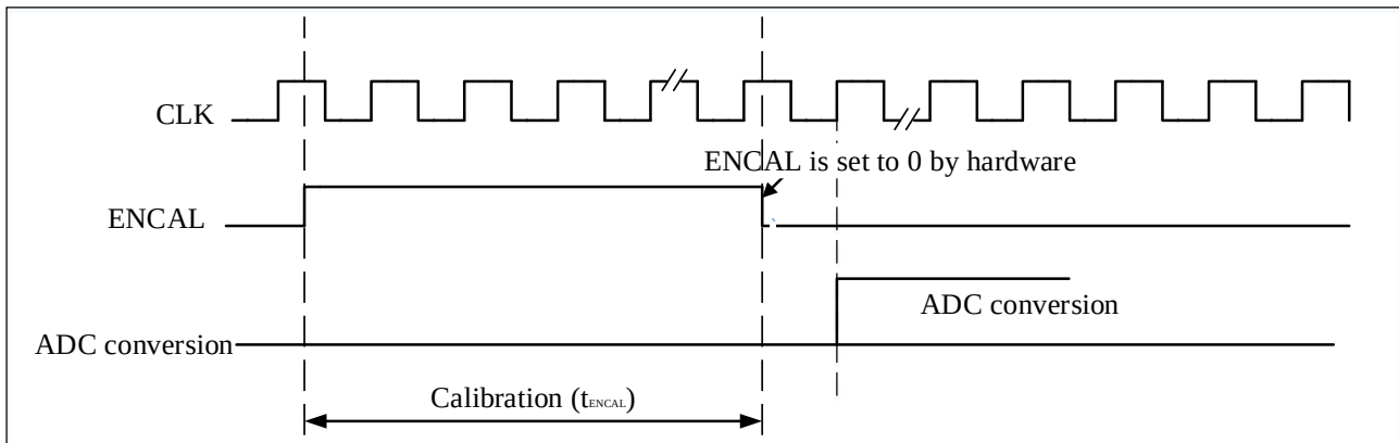
图 10-6 校准时序图
