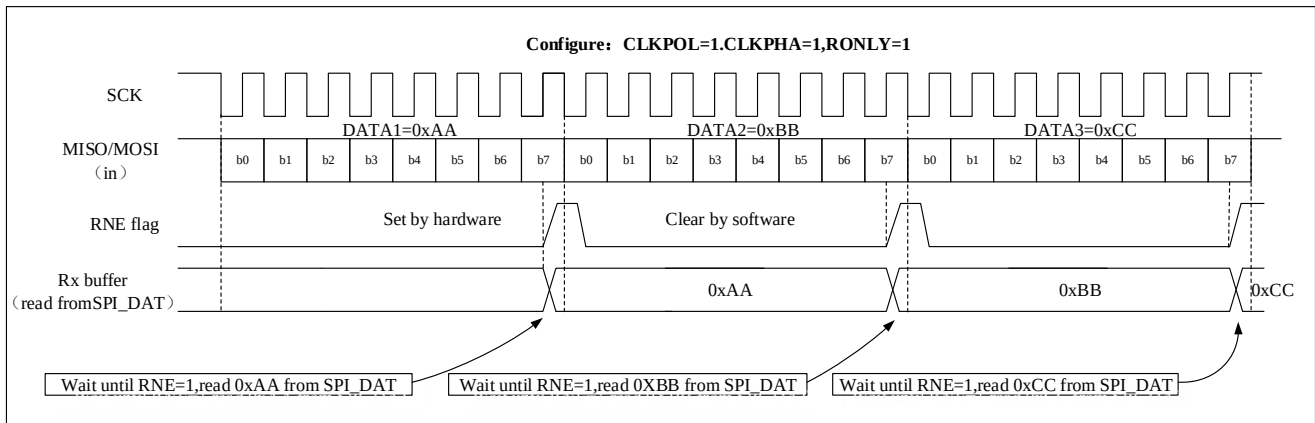
图 22-7 只接收模式（BIDIRMODE = 0 且 RONLY = 1）下连续传输时，RNE 变化示意图
