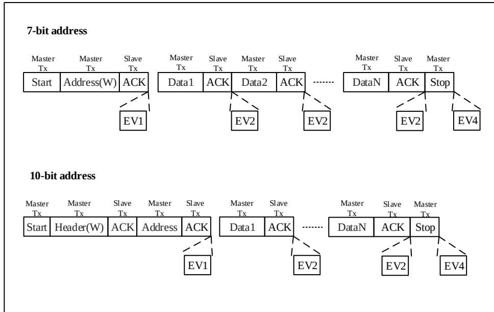
图 23-4 从机接收器传送序列
