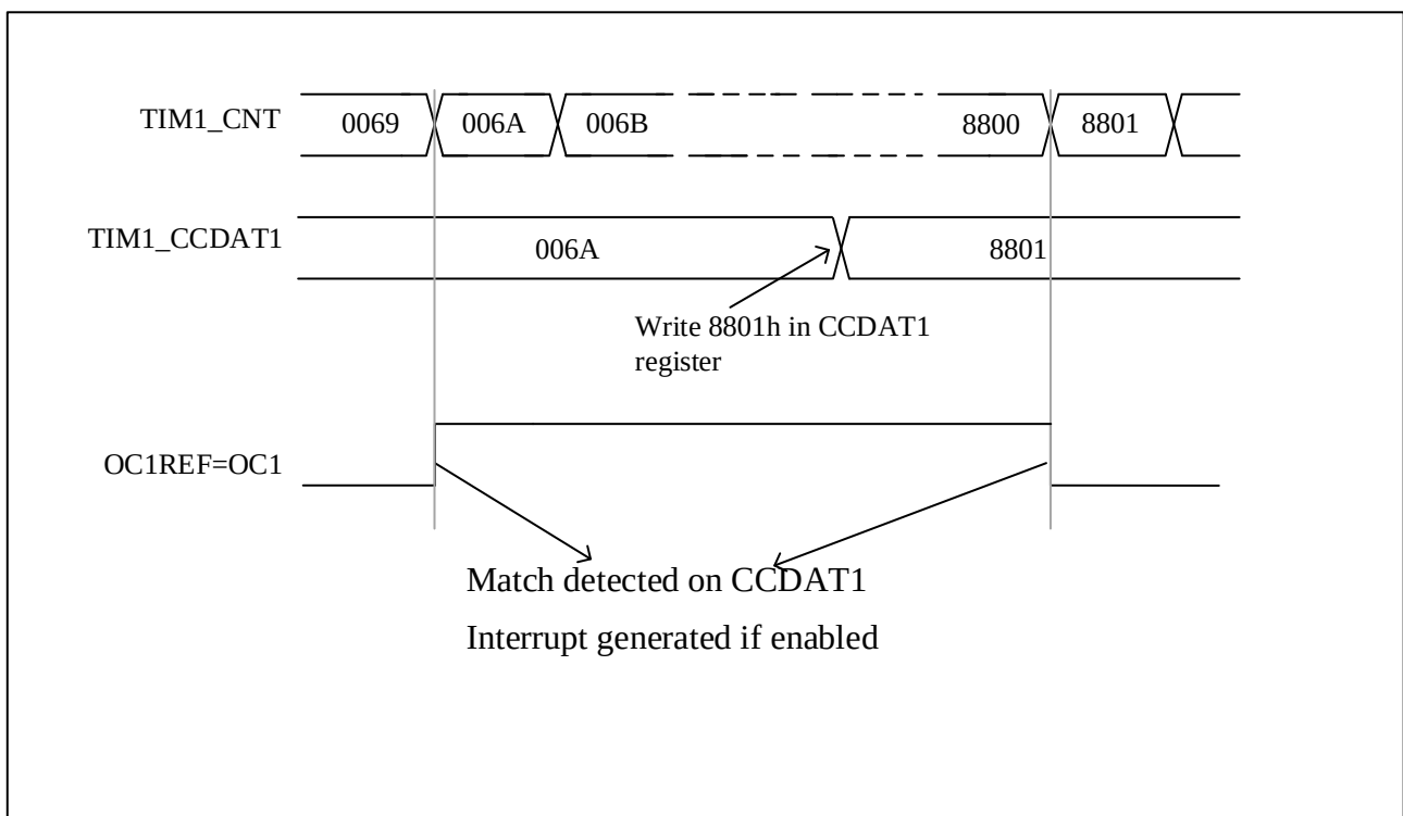
图 12-21 输出比较模式，开启 OC1
