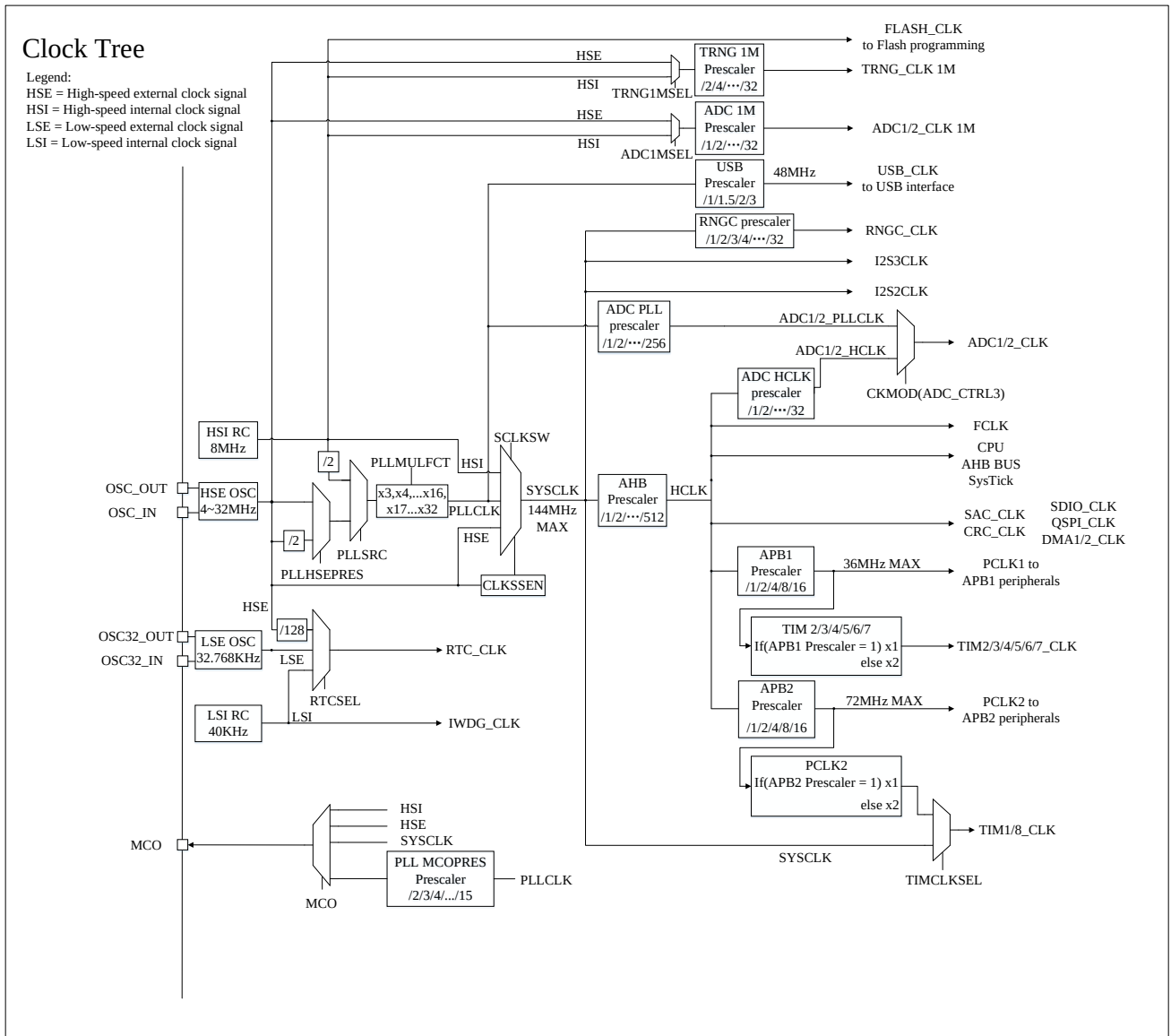
图 5-2 时钟树
