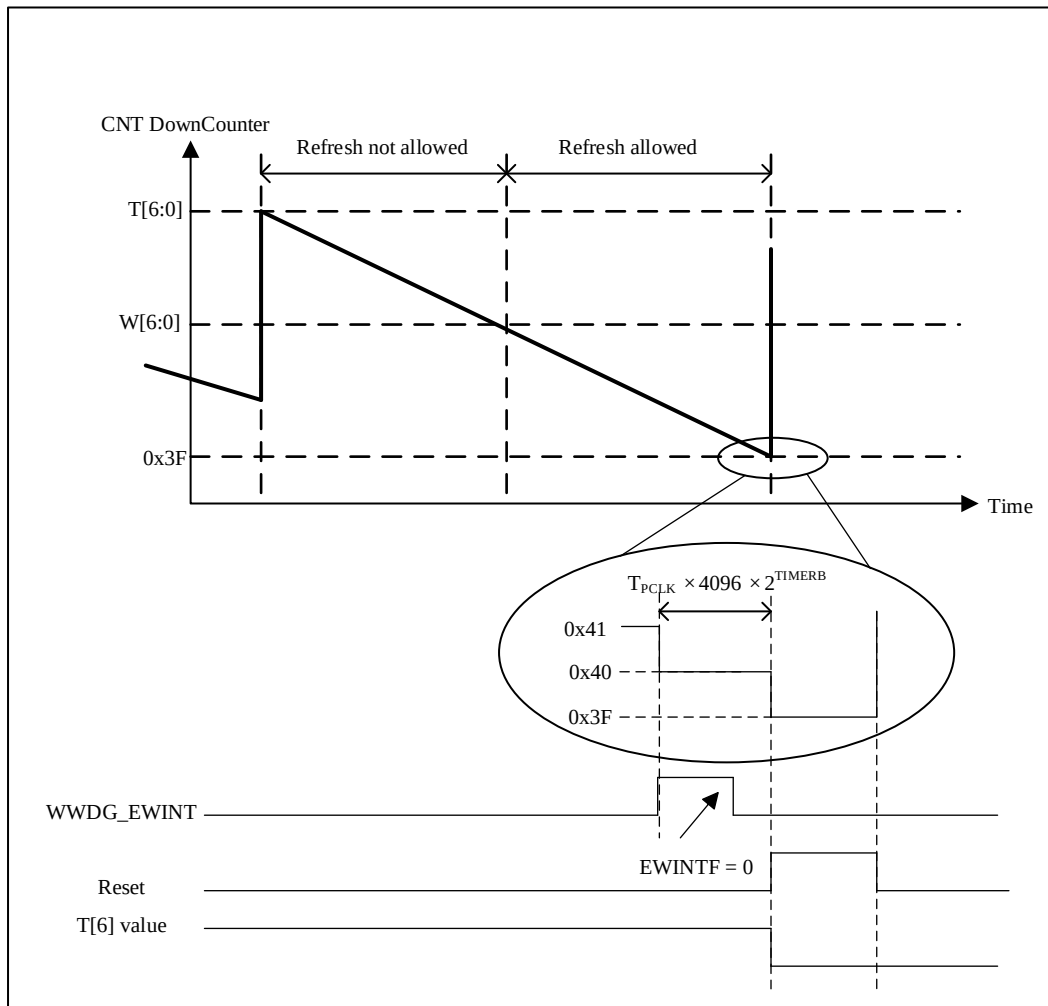
图 18-2 WWDG 的刷新窗口和中断时序
