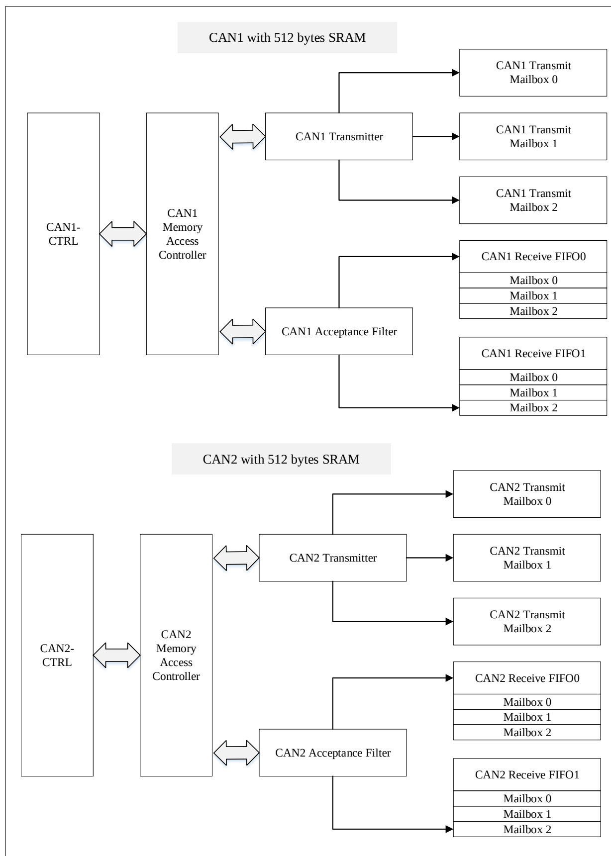
图 21-3 双 CAN 框图
