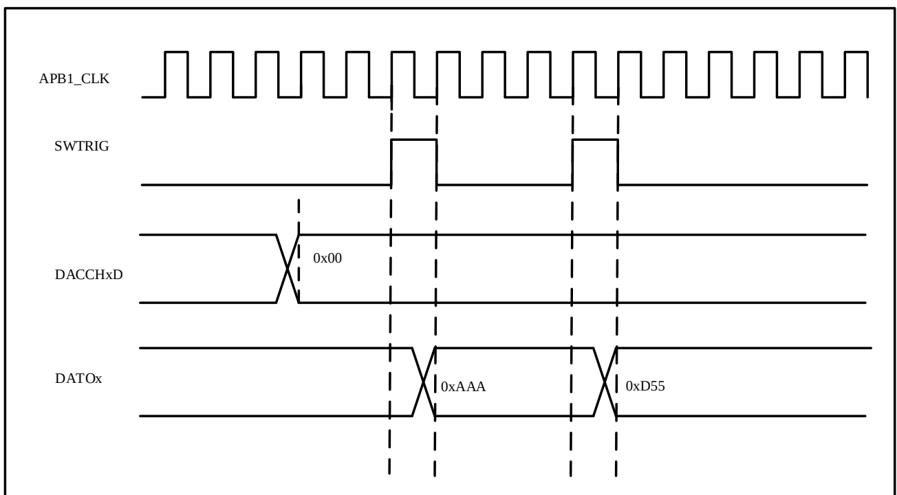
图 11-6 带 LFSR 波形生成的 DAC 转换（使能软件触发）
