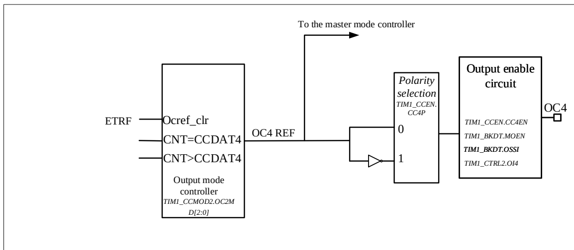
图 12-19 通道 x 的输出部分 (x=4)
