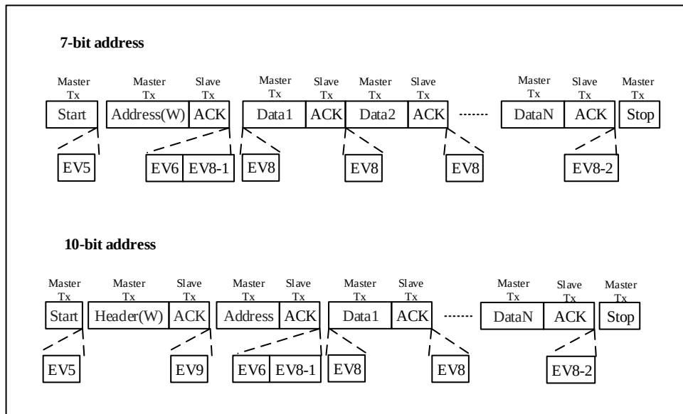
图 23-5 主发送器传送序列
