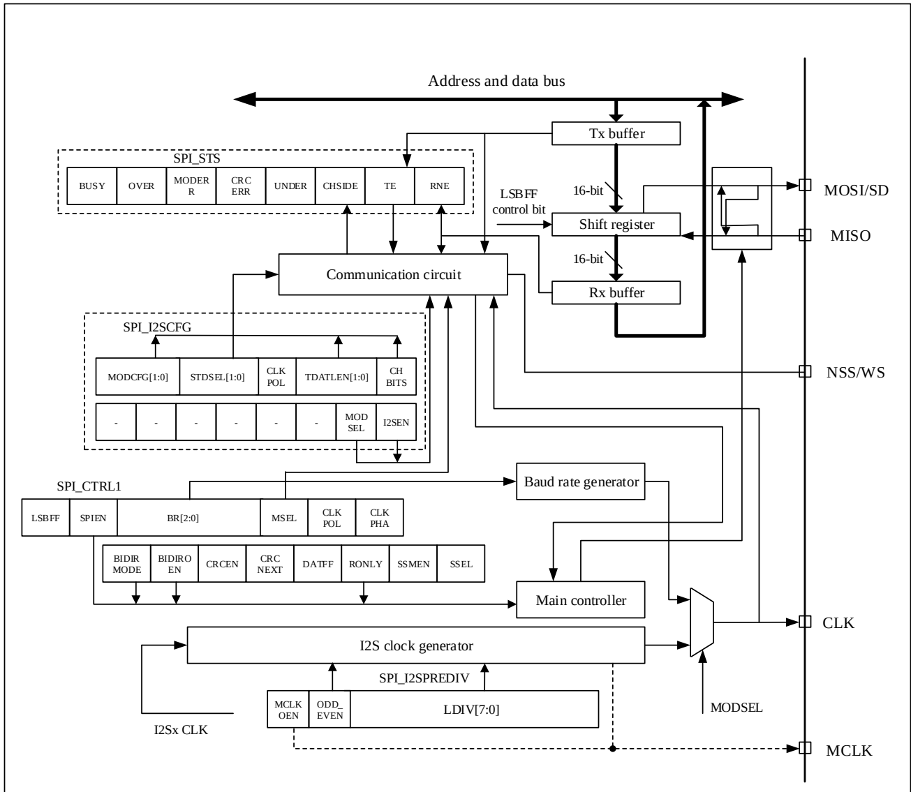
图 22-13 I 2 S 框图
