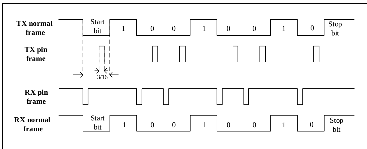
图 24-20 IrDA 数据调制 (3/16)-正常模式
