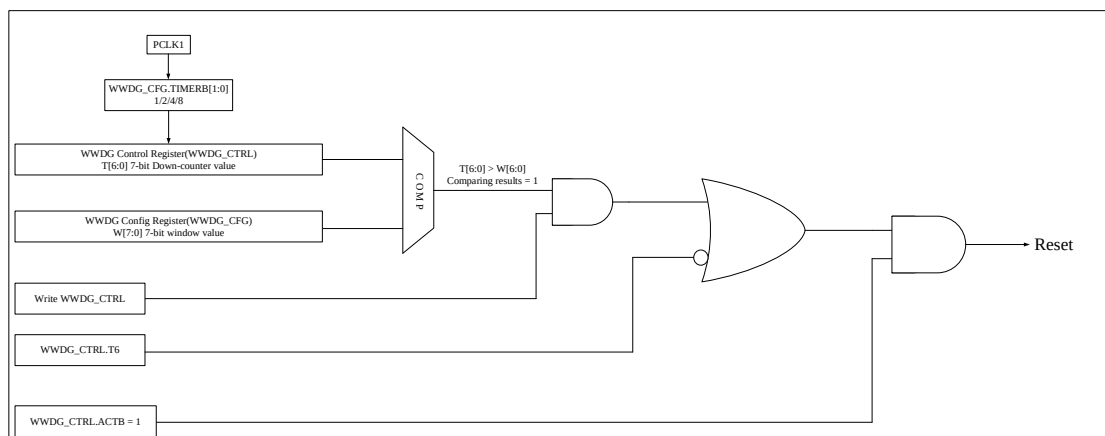
图 18-1 窗口看门狗功能框图
