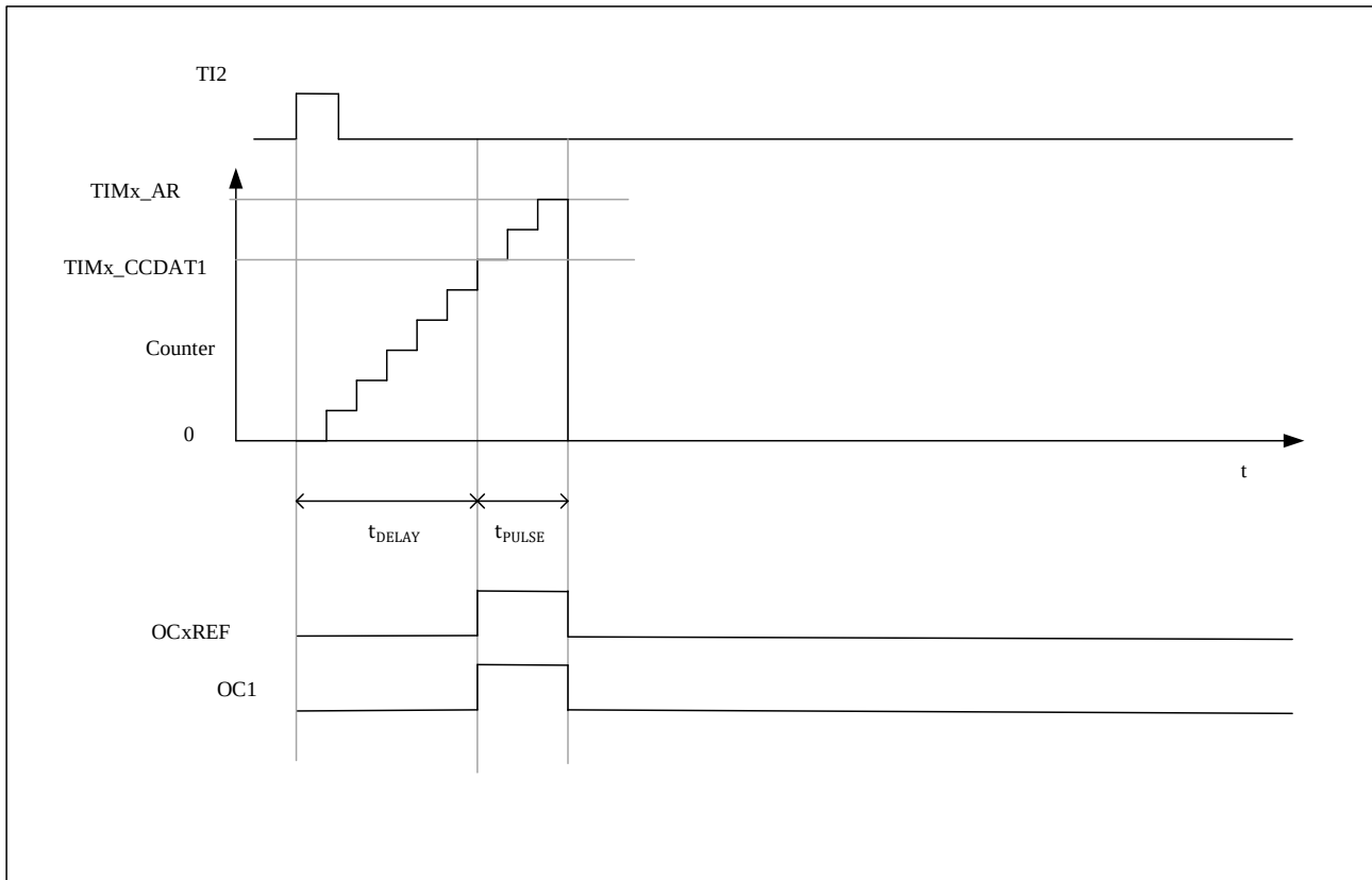
图 13-20 单脉冲模式示例
