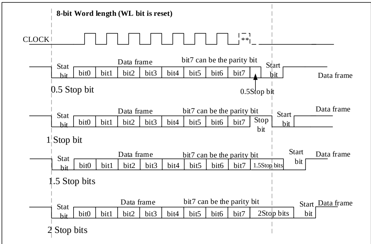
图 24-4 停止位配置
