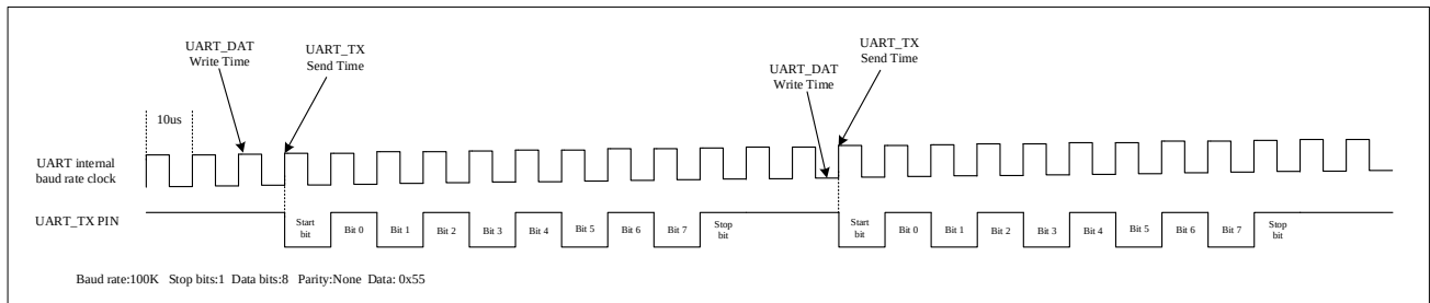
图 24-5 发送时序
