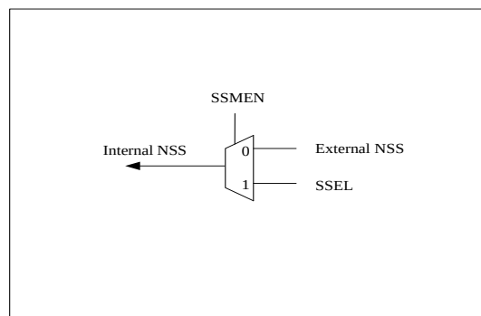
图 22-2 硬件/软件的从选择管理
