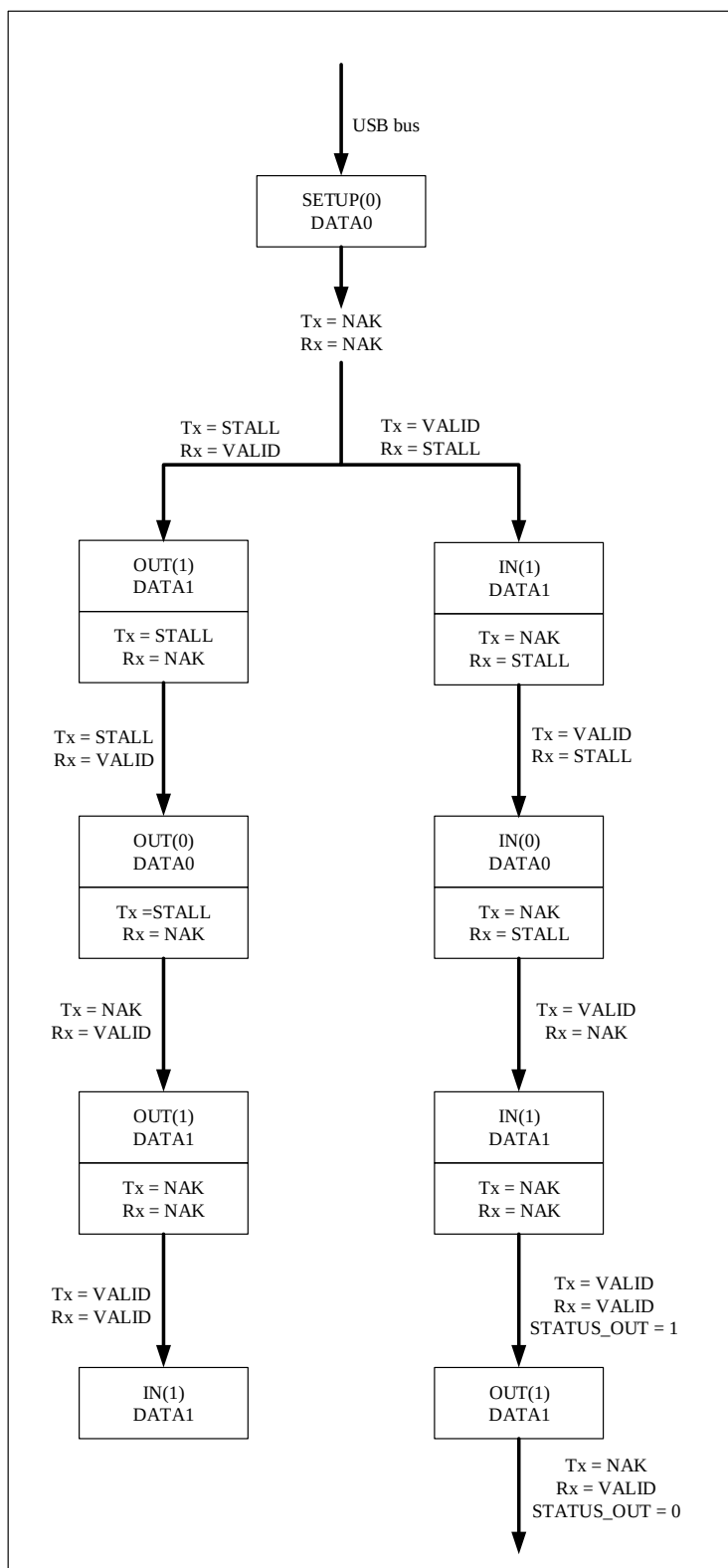
图 20-5 控制传输
