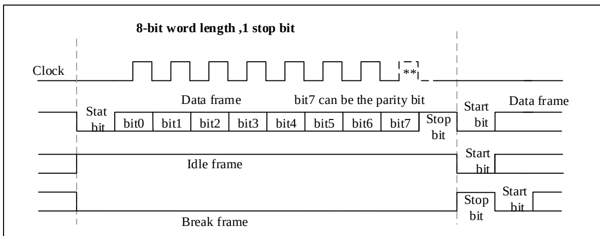
图 24-2 字长=8 设置
