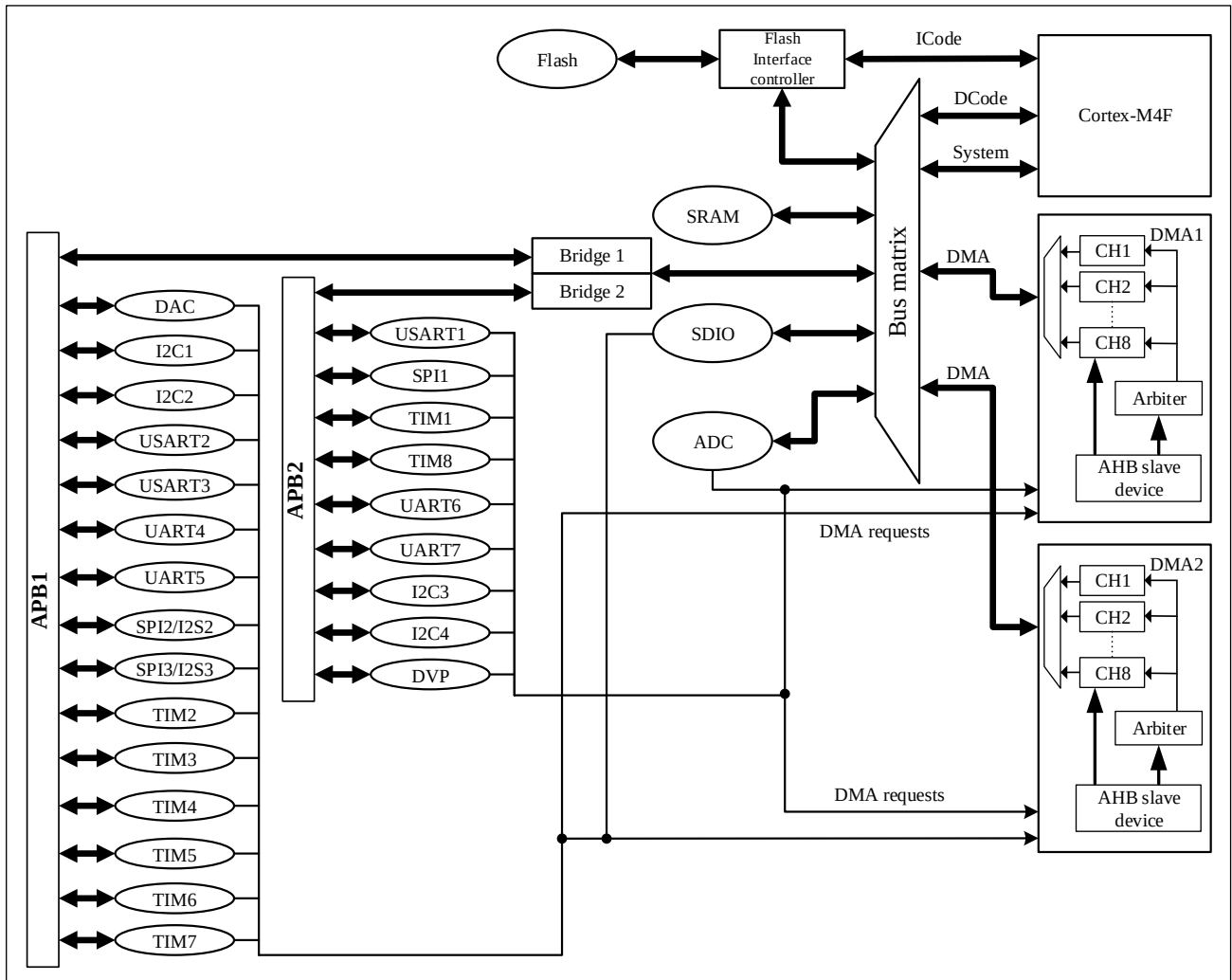
图 9-1 DMA 框图
