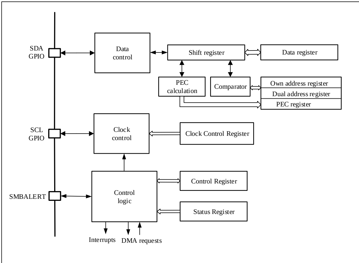
图 23-1 I 2 C 功能框图
