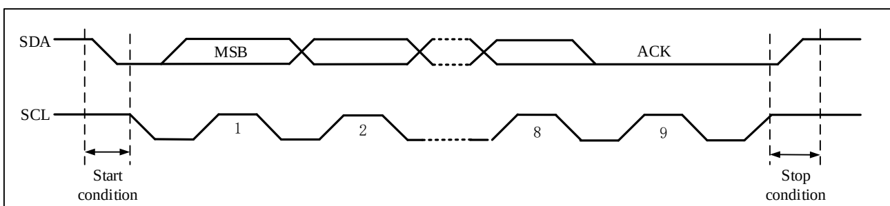
图 23-2 I 2 C 总线协议
