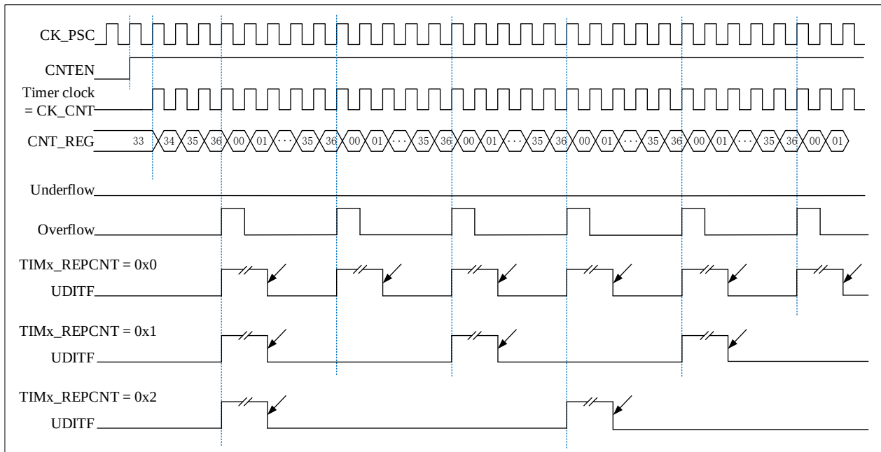
图 12-9 向上计数模式下的重复计数时序图
