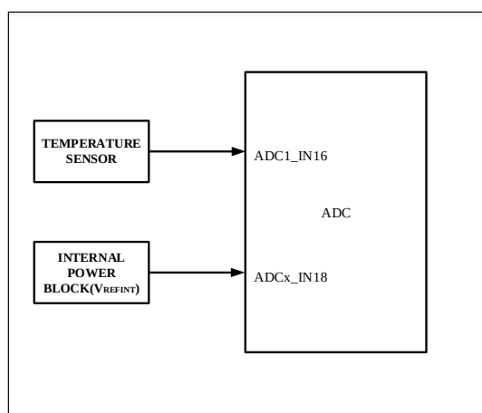
图 10-17 温度传感器和 V_{REFINT} 通道框图
