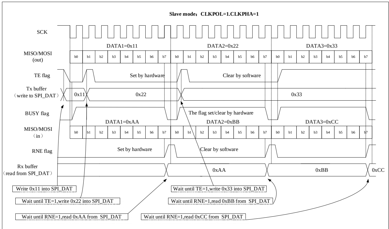
图 22-8 从机全双工模式下连续传输时，SPI_STS.TE/RNE/BUSY 的变化示意图
