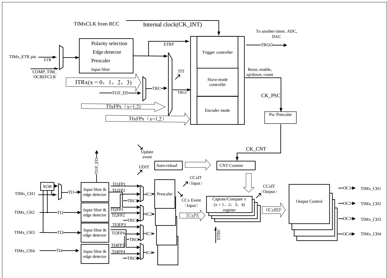
图 13-1 TIMx (x=2,3,4 and 5) 框图
