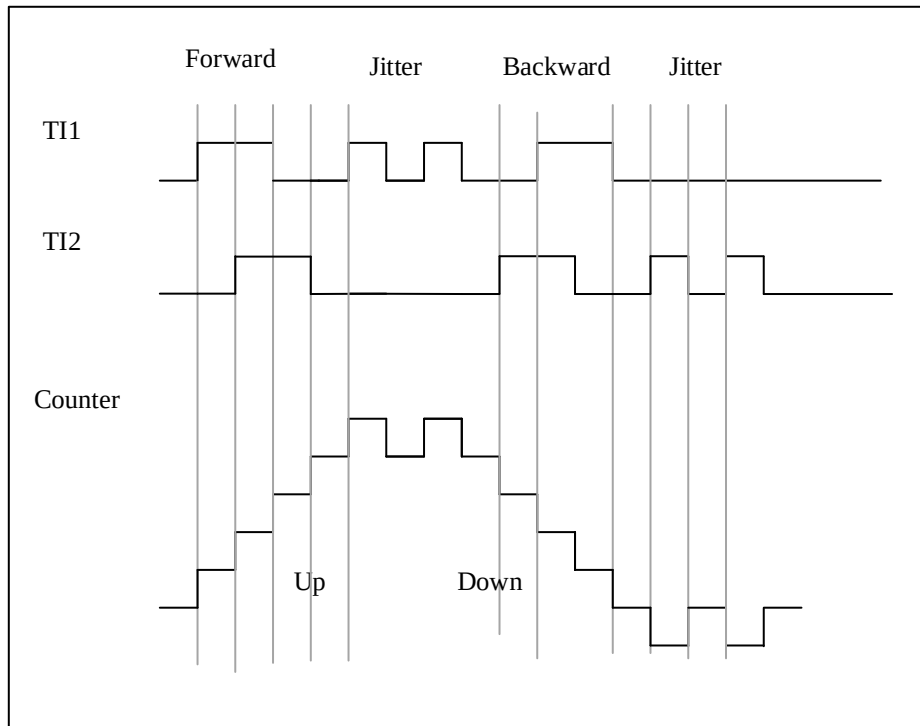
图 13-27 编码器模式下的计数器操作实例
