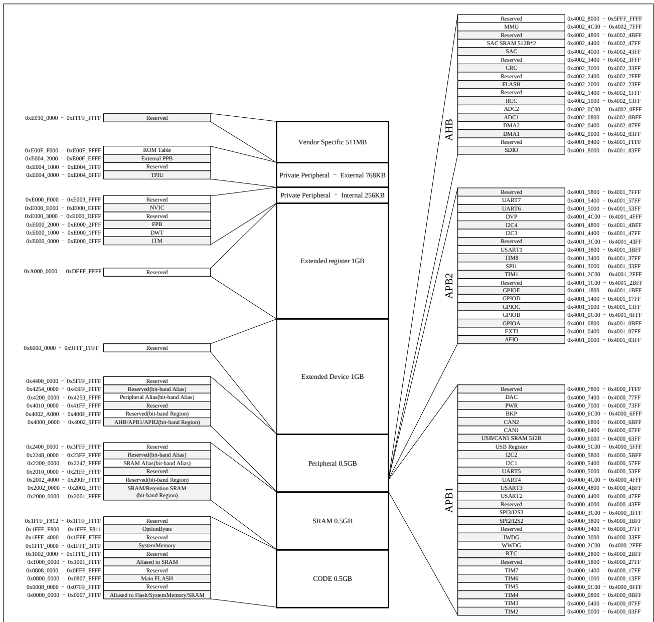
图 2-3 总线地址映射图
