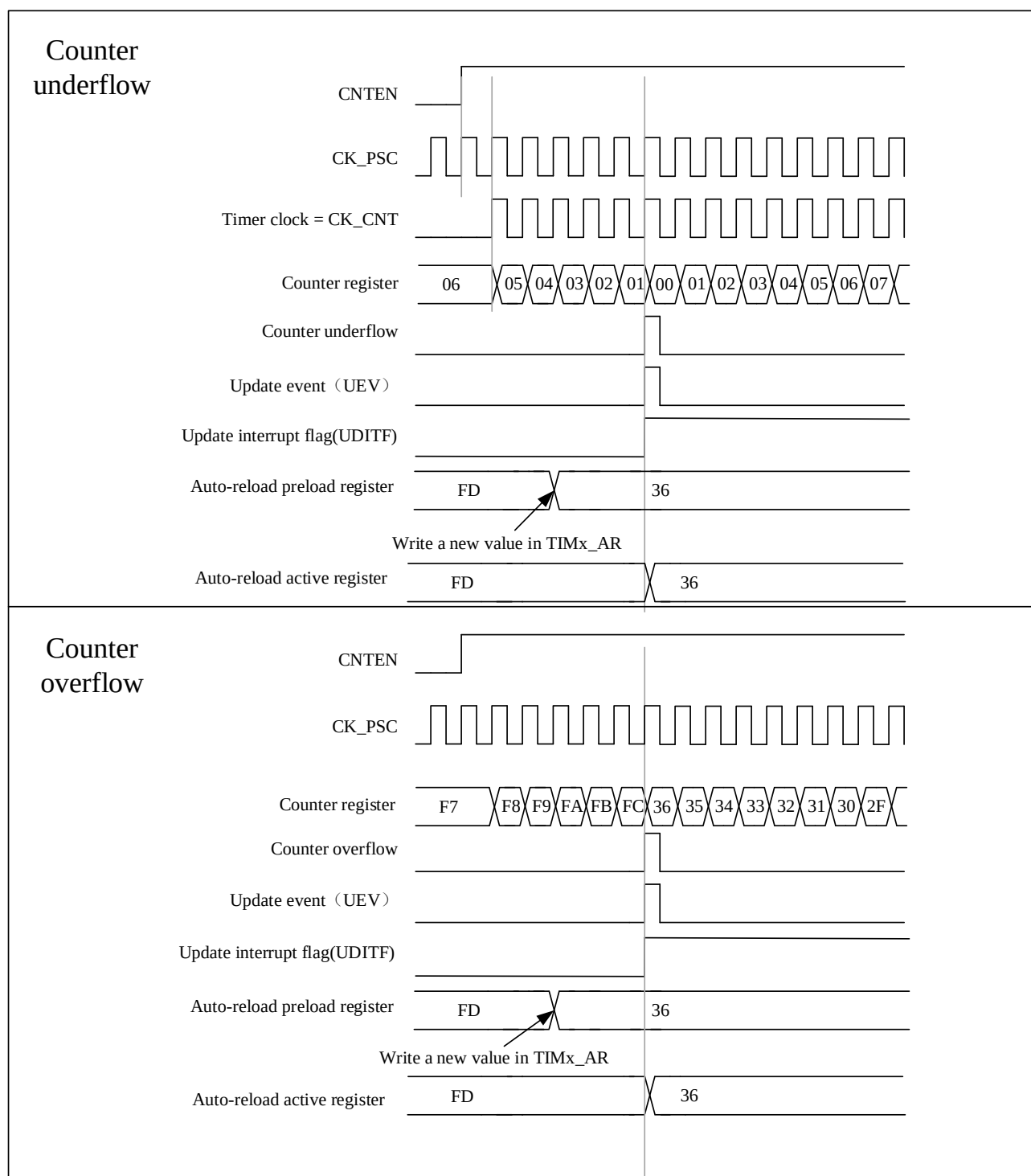
图 13-7 包含计数器上溢和下溢的中央对齐时序图(ARPEN=1)
