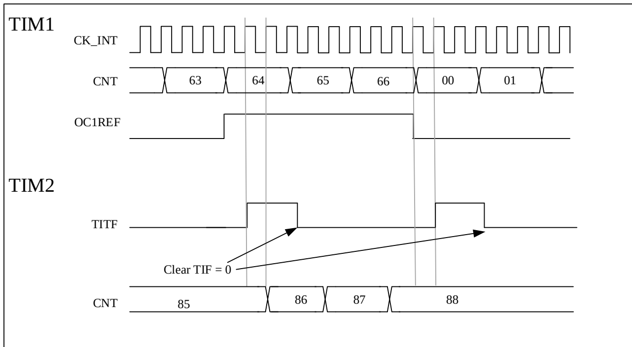
图 13-23 定时器 2 由定时器 1 的 OC1REF 门控
