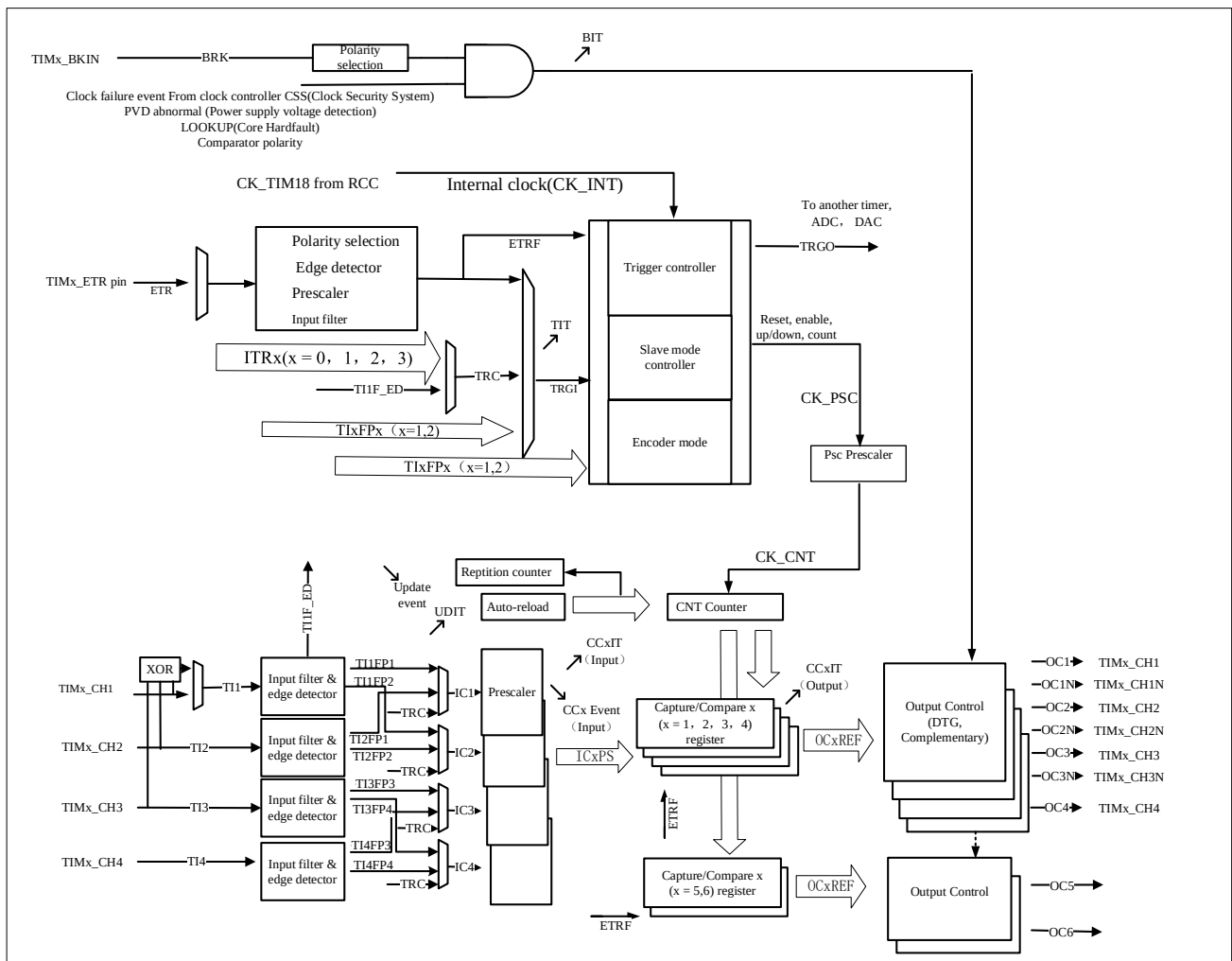
图 12-1 TIMx(x=1/8)框图
