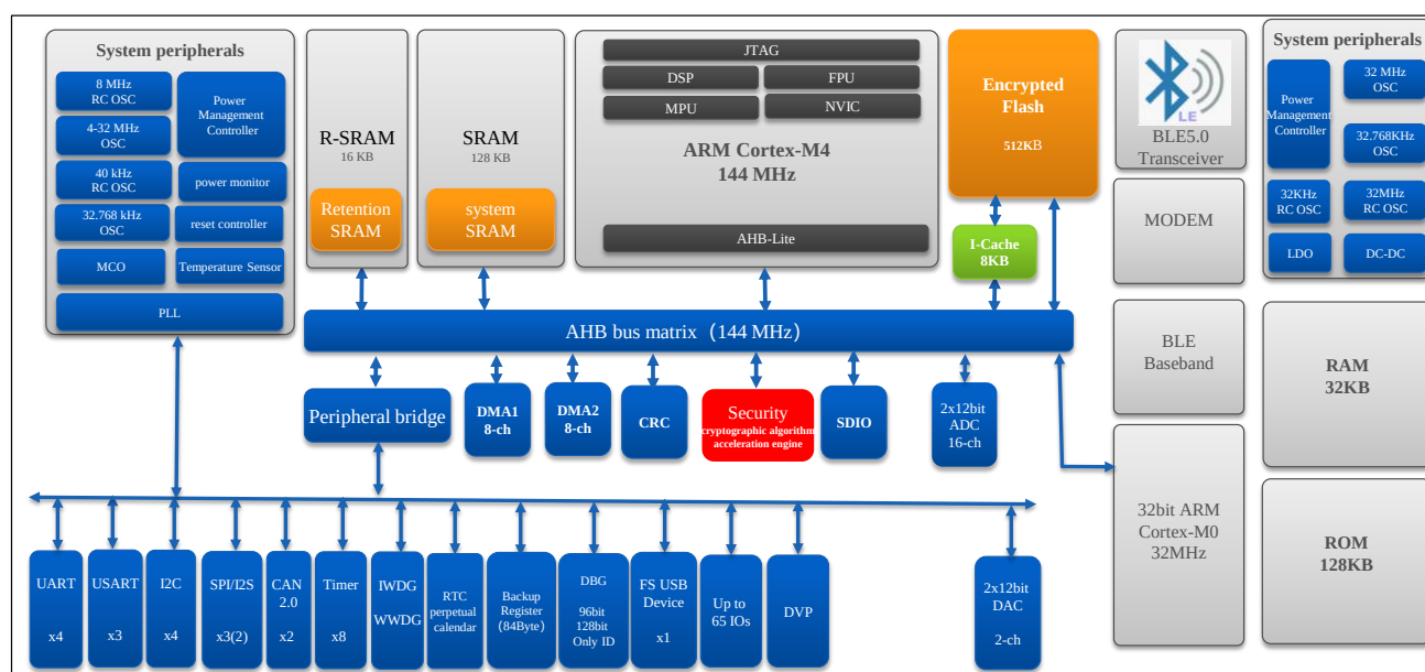
图 2-1 N32WB452 系统原理框图
