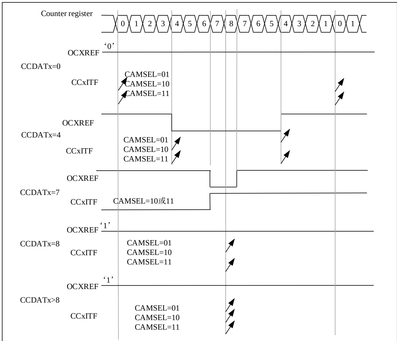
图 13-18 中央对齐的 PWM 波形 (AR=8)
