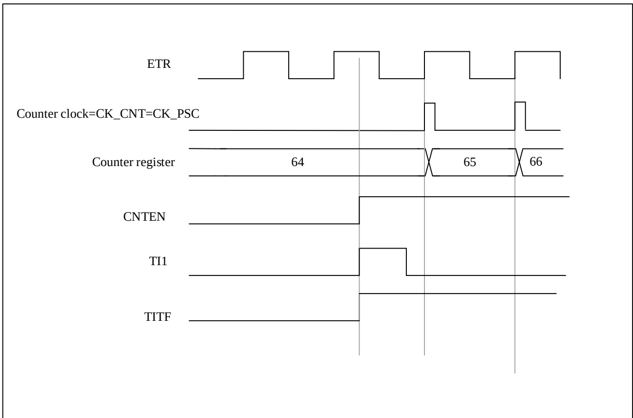
图 12-31 外部时钟模式 2+触发模式下的控制电路
