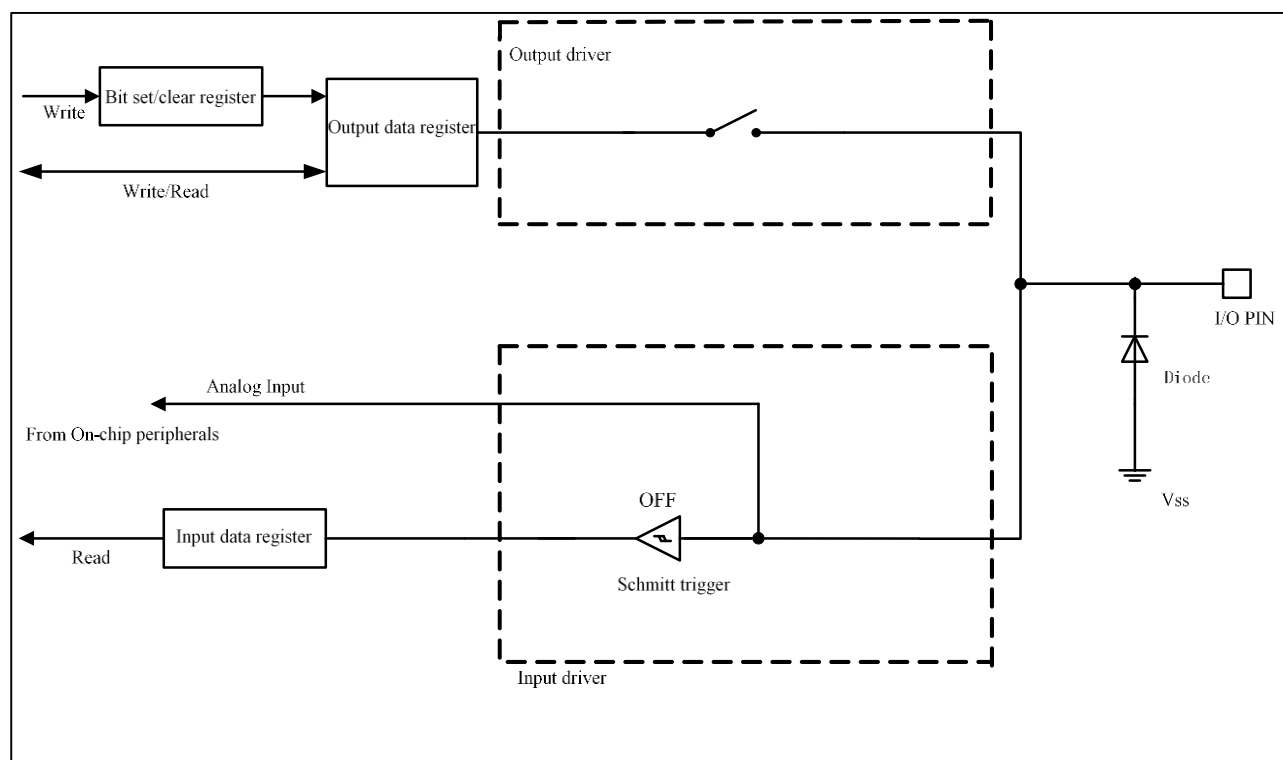
图 7-5 高阻抗的模拟模式配置
