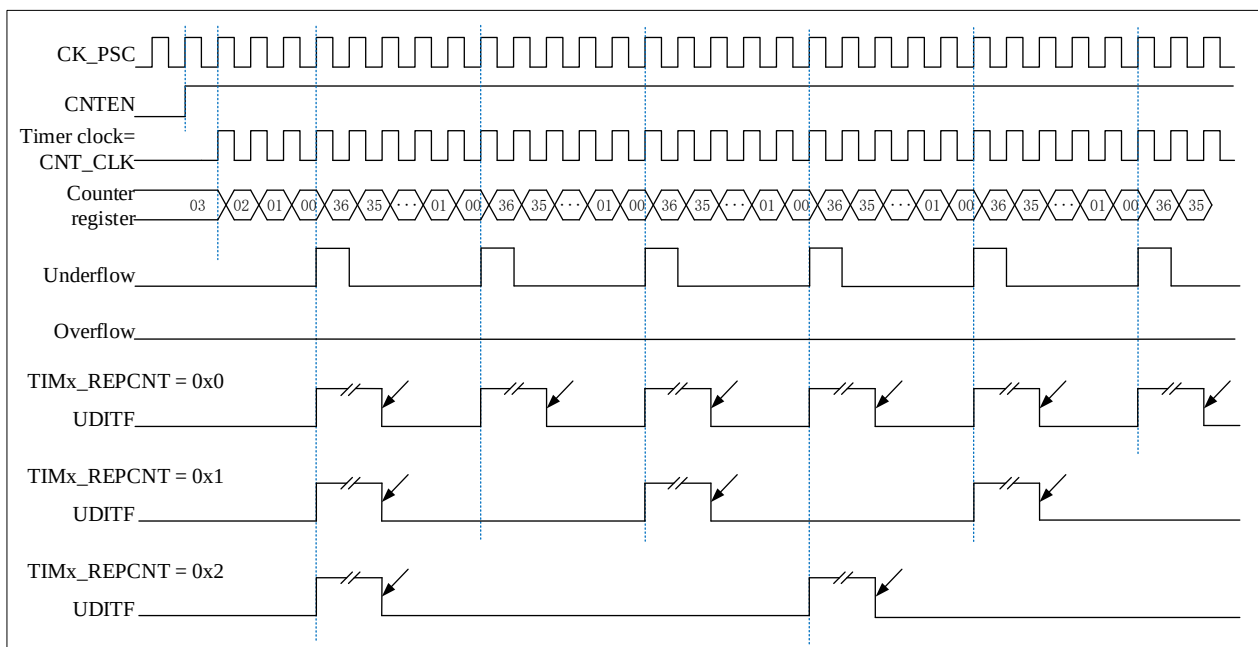
图 12-8 向下计数模式下的重复计数时序图
