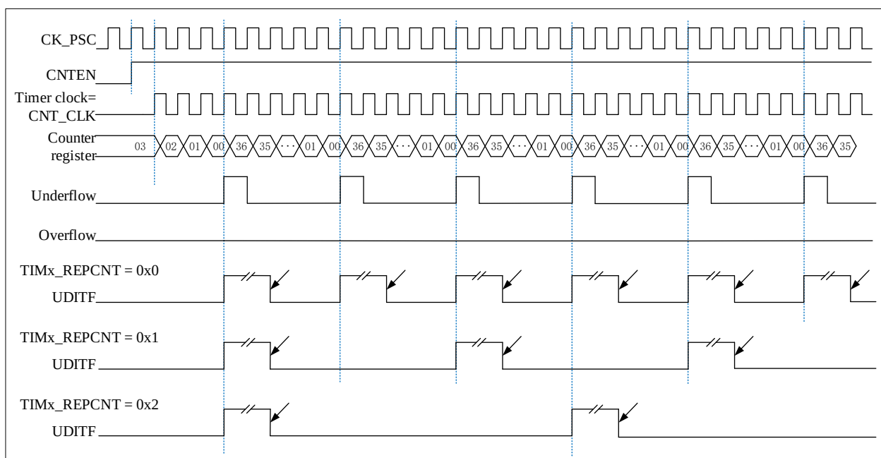
图 12-8 向下计数模式下的重复计数时序图
