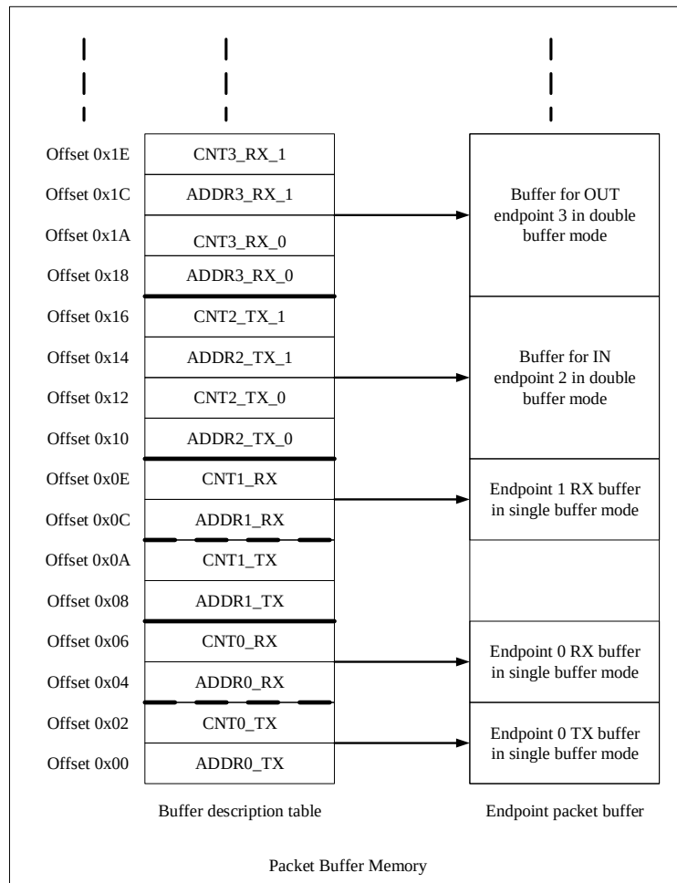
图 20-3 缓冲区描述表和端点数据包缓冲区的关系
