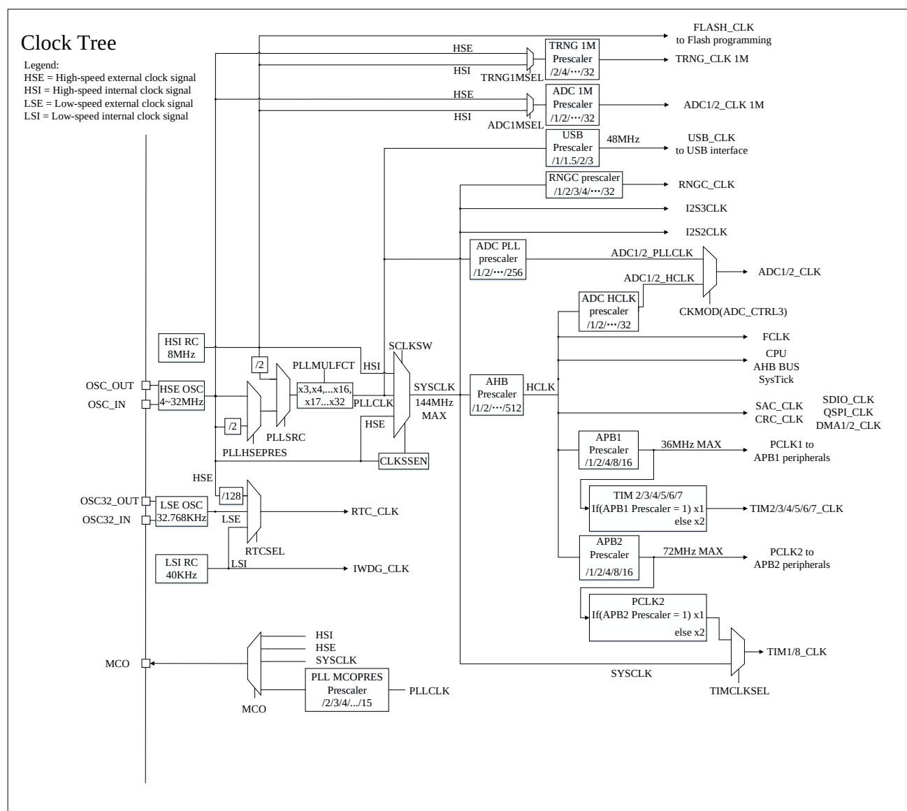
图 5-2 时钟树
