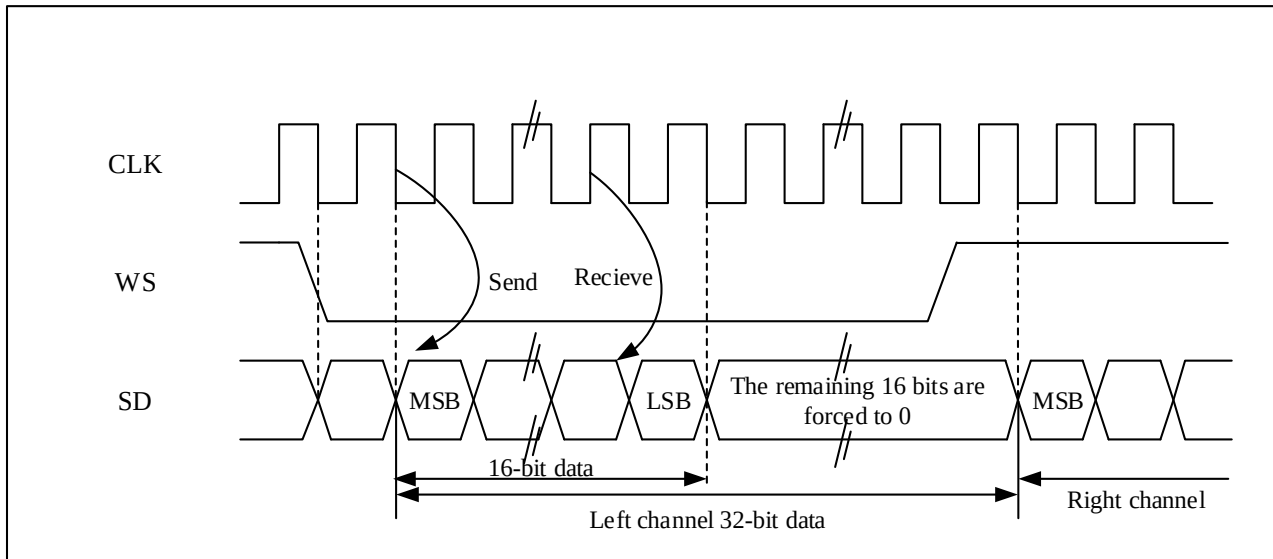
图 22-16 PS 飞利浦协议标准波形（16 位扩展至 32 位包帧，CLKPOL = 0）
