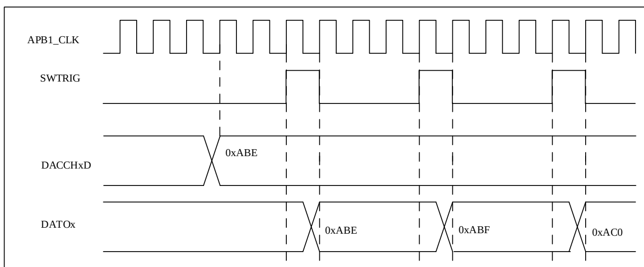
图 11-8 带三角生成的 DAC 转换（使能软件触发）
