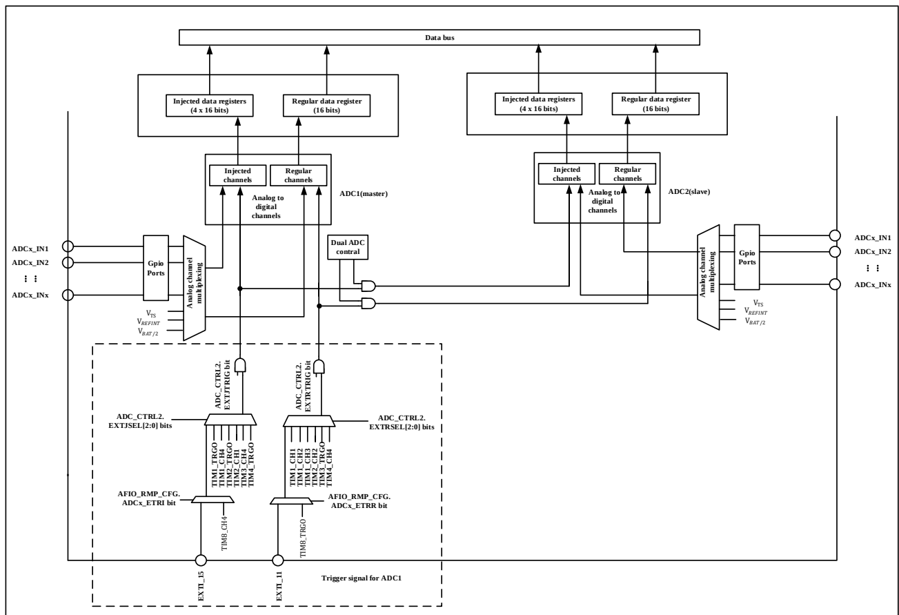
图 10-7 双 ADC 框图
