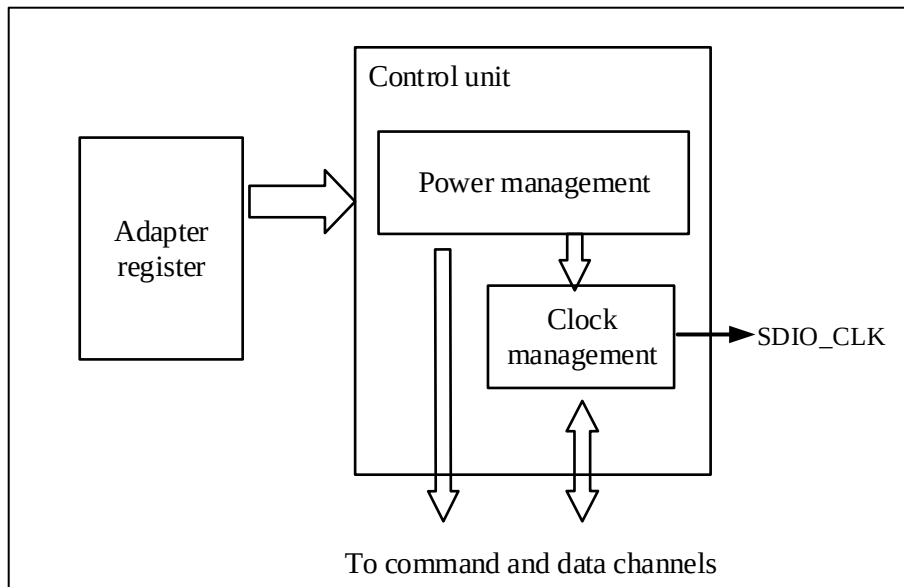
图 19-8 控制单元
