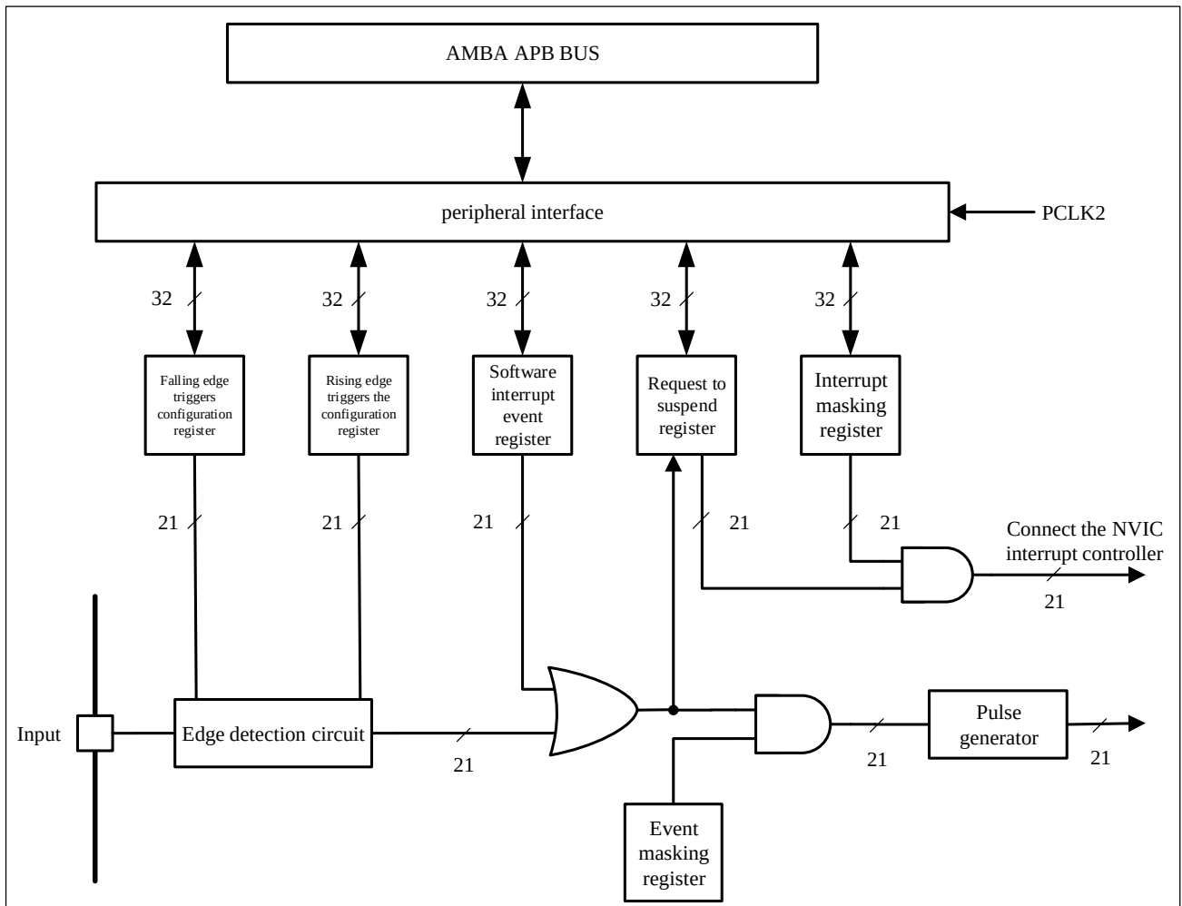
图 8-1 外部中断/事件控制器框图
