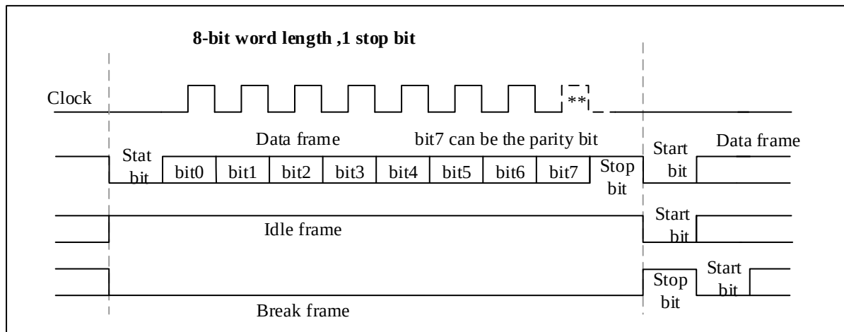
图 24-2 字长=8 设置
