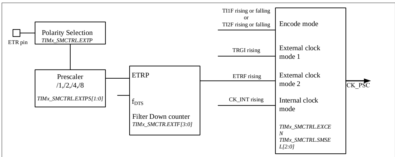
图 13-11 外部触发输入框图
