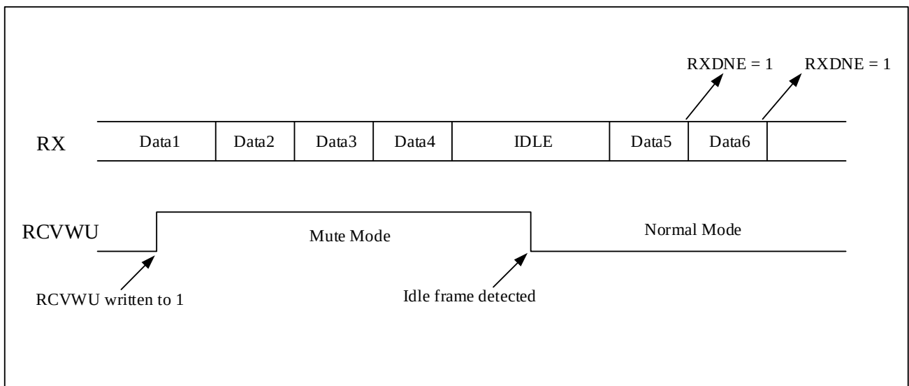
图 24-13 静默模式下的空闲总线检测
