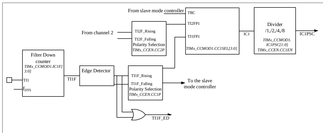
图 13-13 捕获/比较通道（例如：通道 1 输入级）
