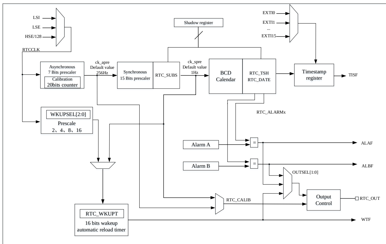
图 15-1 RTC 功能框图
