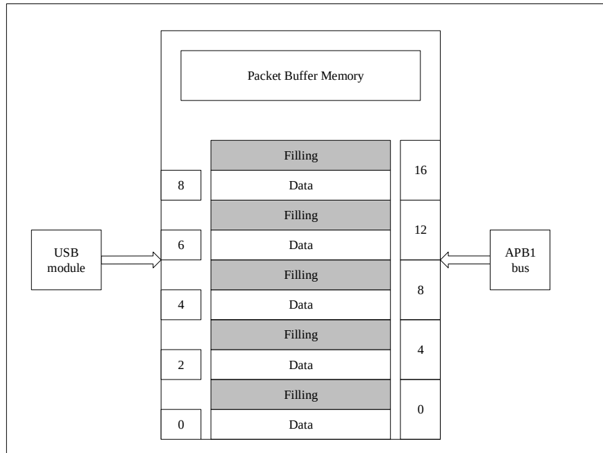
图 20-2 USB 模块和微控制器上的用户应用程序访问 Packet Buffer Memory 方式
