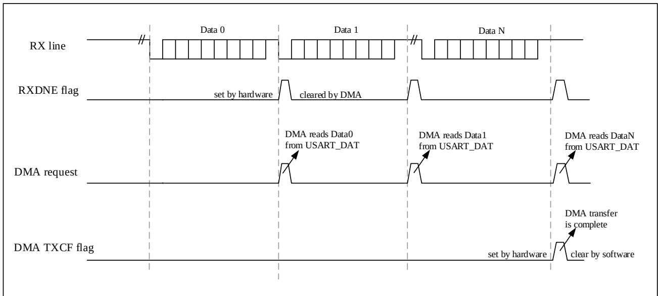
图 24-9 DMA 接收
