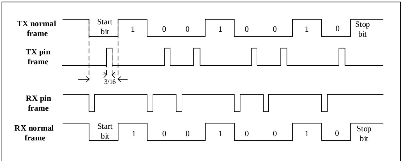
图 24-20 IrDA 数据调制 (3/16)-正常模式
