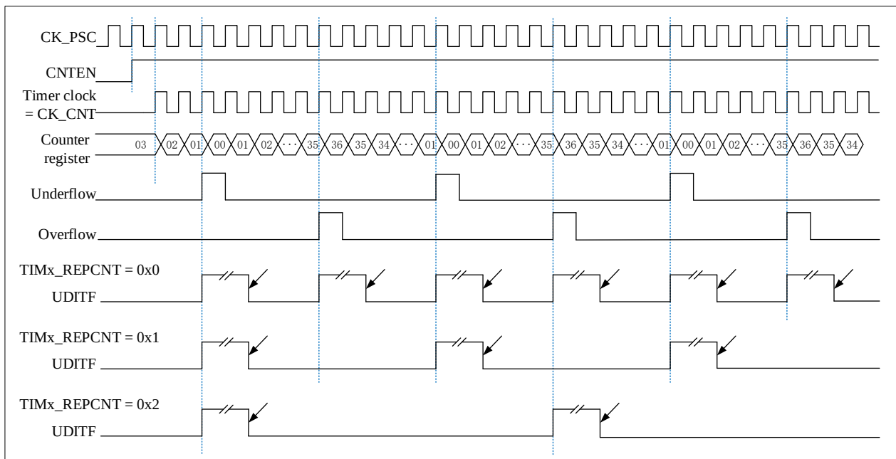
图 12-10 中央对齐模式下的重复计数时序图
