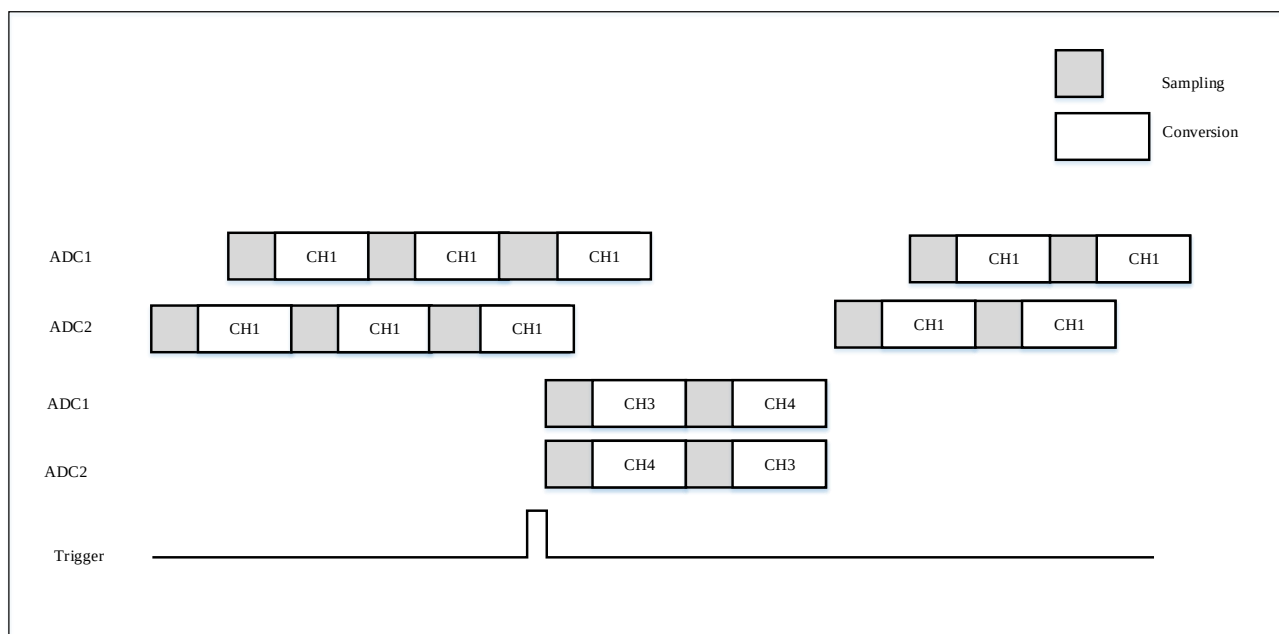
图 10-16 交叉的单通道转换被注入序列 CH3 和 CH4 中断
