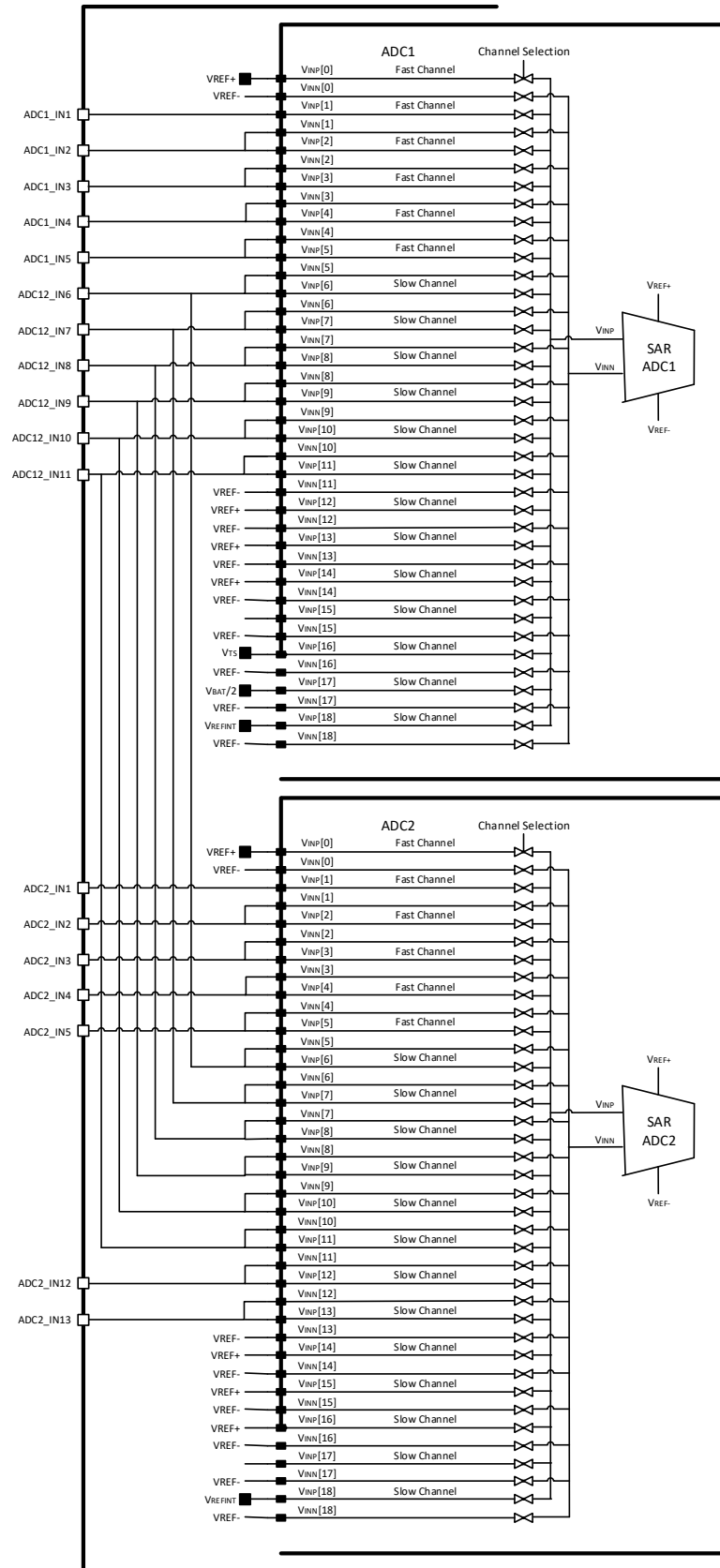
图 10-3 ADC1 和 ADC2 通道引脚连接
