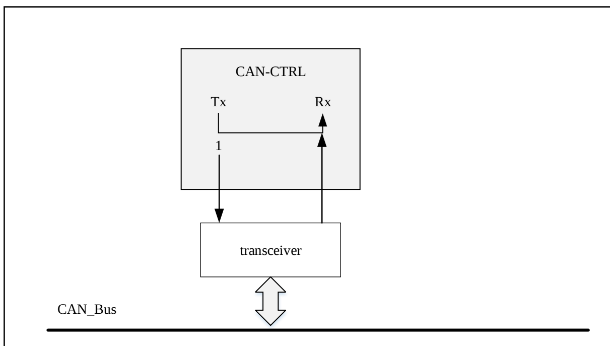
图 21-5 静默模式
