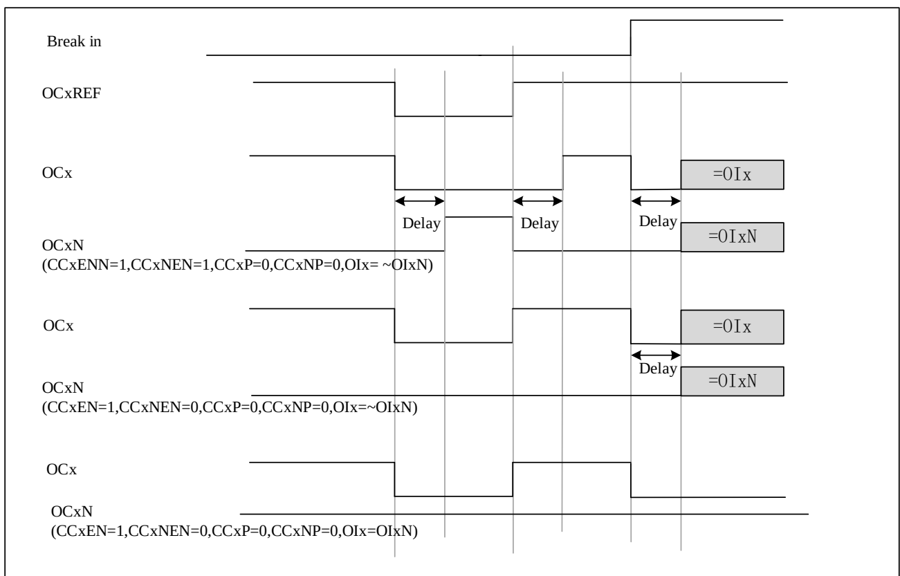
图 12-27 响应刹车的输出行为
