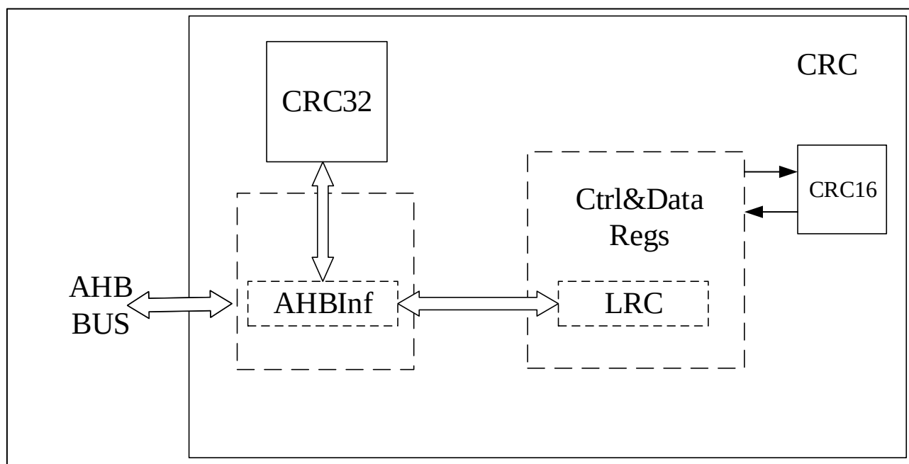
图 16-1 CRC 计算单元框图
