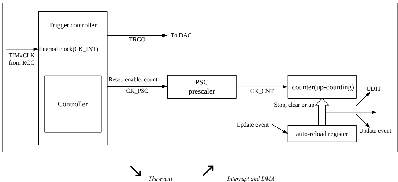
图 14-1 TIMx 的框图 (x = 6/7)
