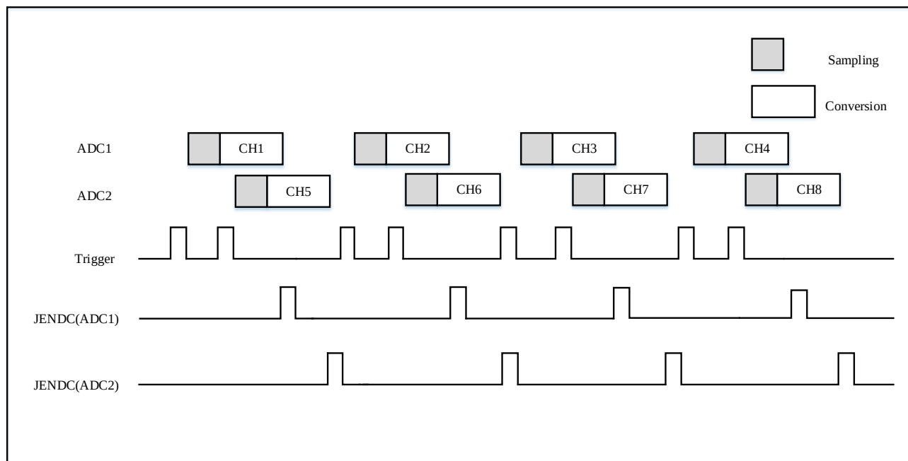
图 10-13 交替触发：在间断模式下注入通道组
