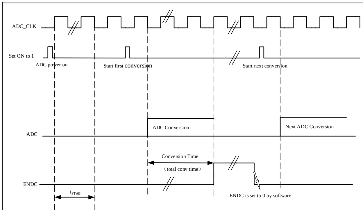
图 10-4 时序图
