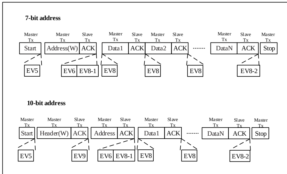
图 23-5 主发送器传送序列
