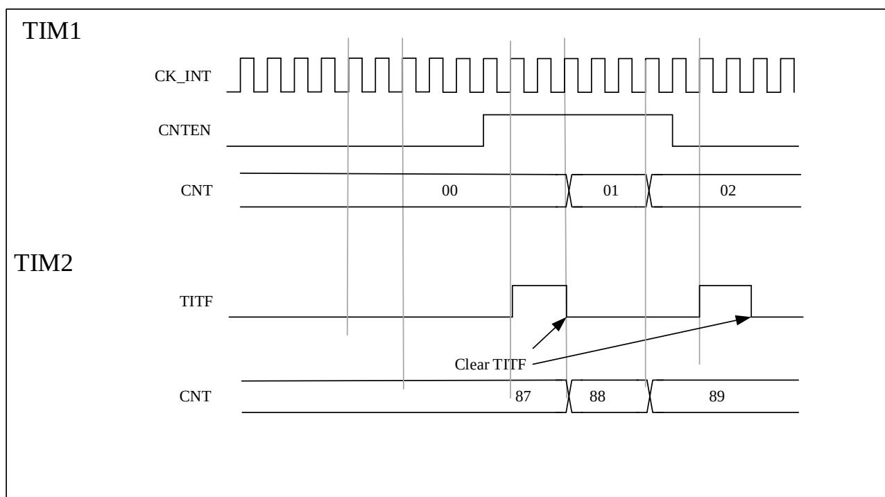
图 13-24 定时器 2 由定时器 1 的使能门控
