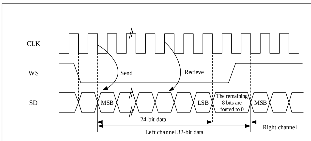
图 22-15 I 2 S 飞利浦协议标准波形（24 位帧，CLKPOL = 0）
