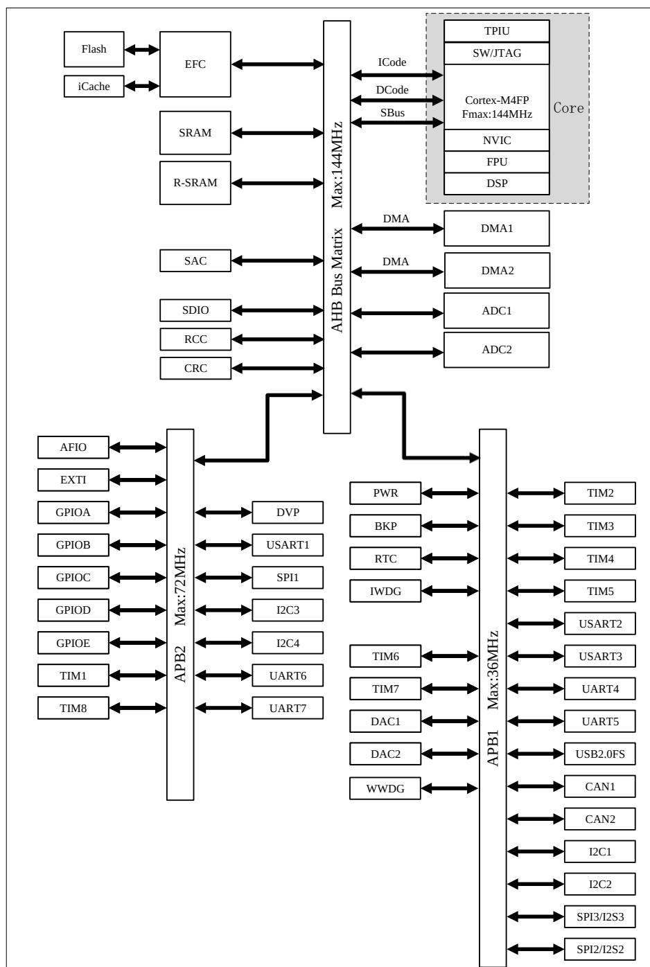
图 2-2 总线架构图
