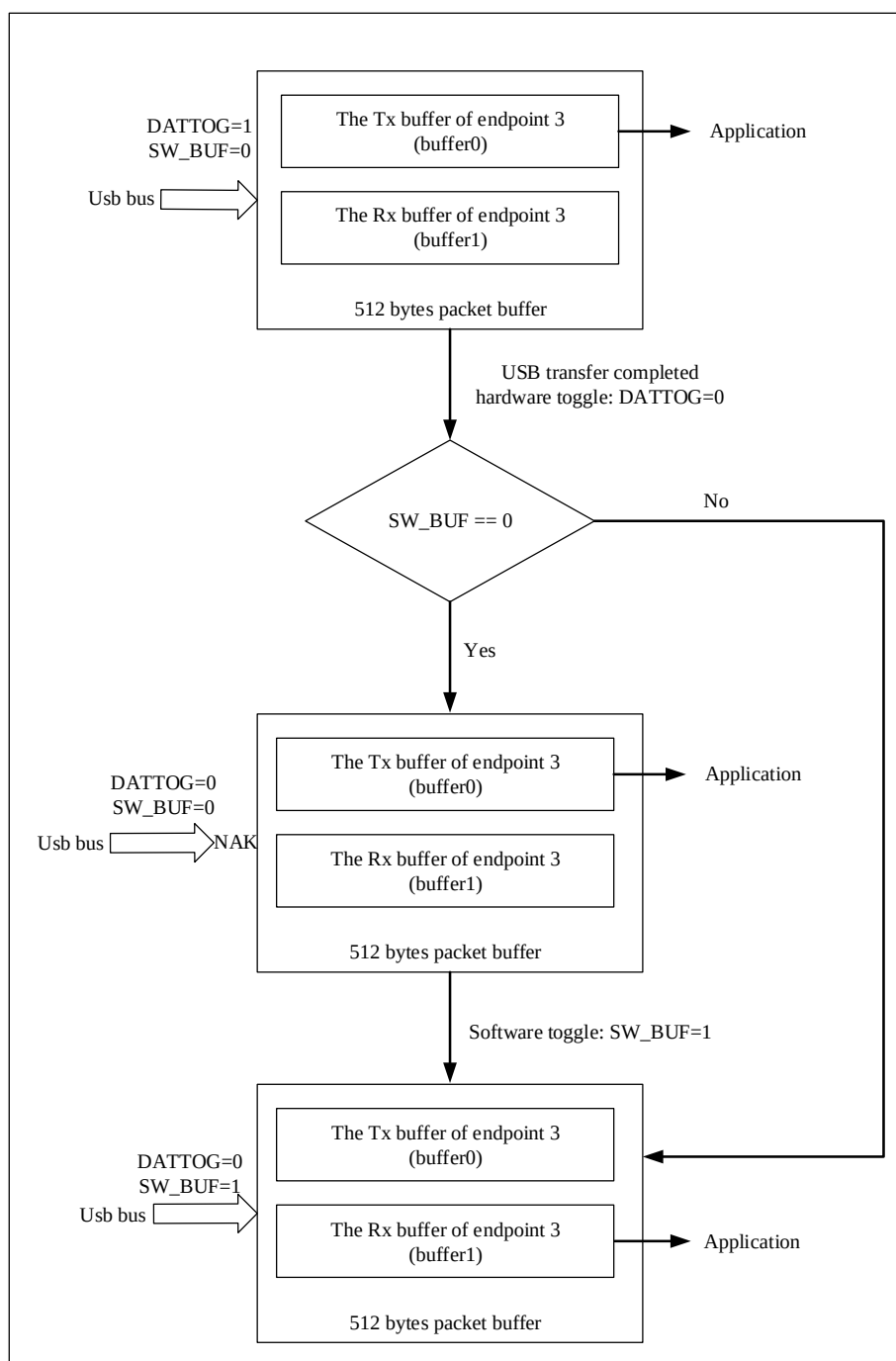
图 20-4 双缓冲批量端点示例
