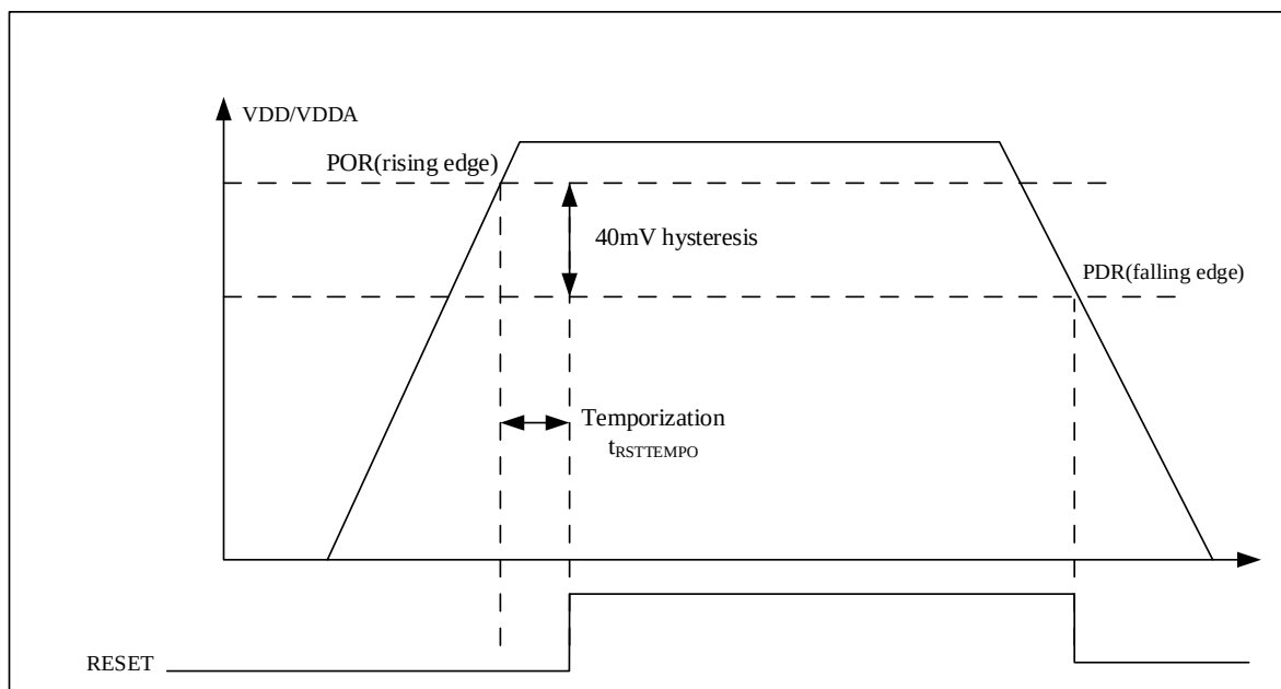
图 3-2 上电复位和掉电复位的波形图
