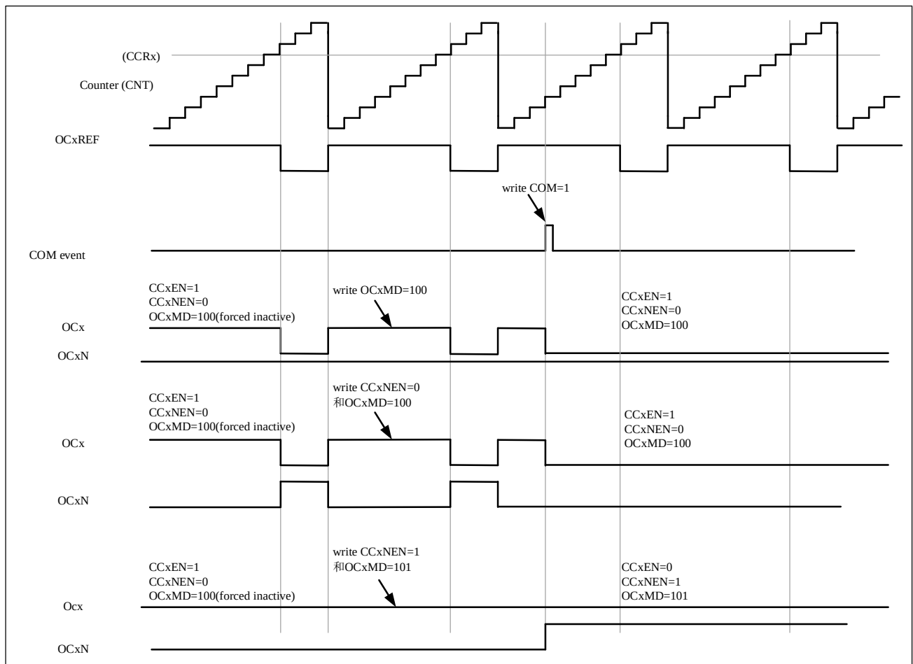
图 12-32 产生六步 PWM，使用 COM 的例子（OSSR=1）
