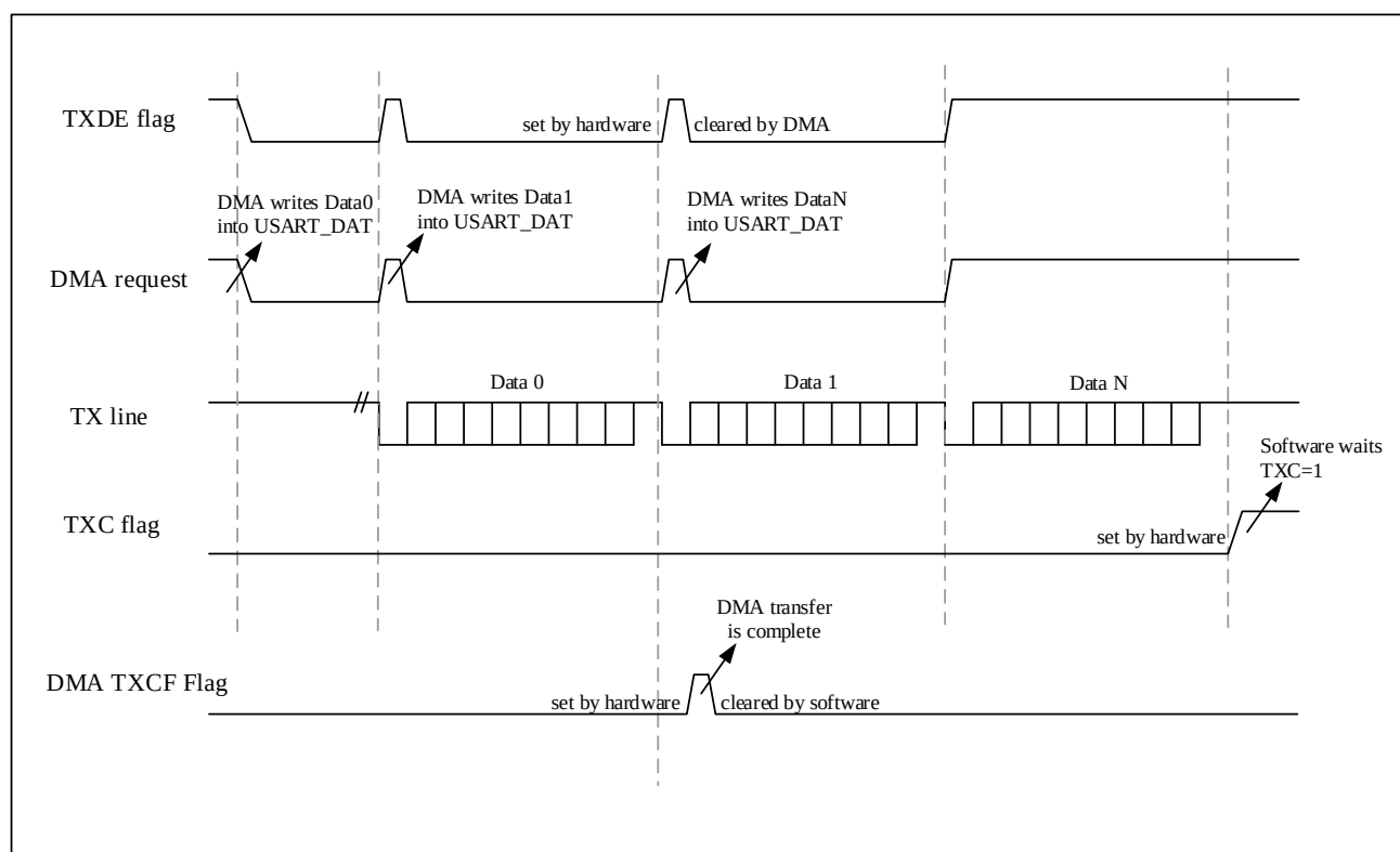
图 24-8 DMA 发送
