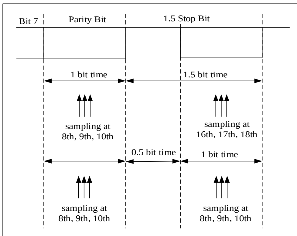
图 24-24 使用 1.5 停止位检测奇偶检验错误
