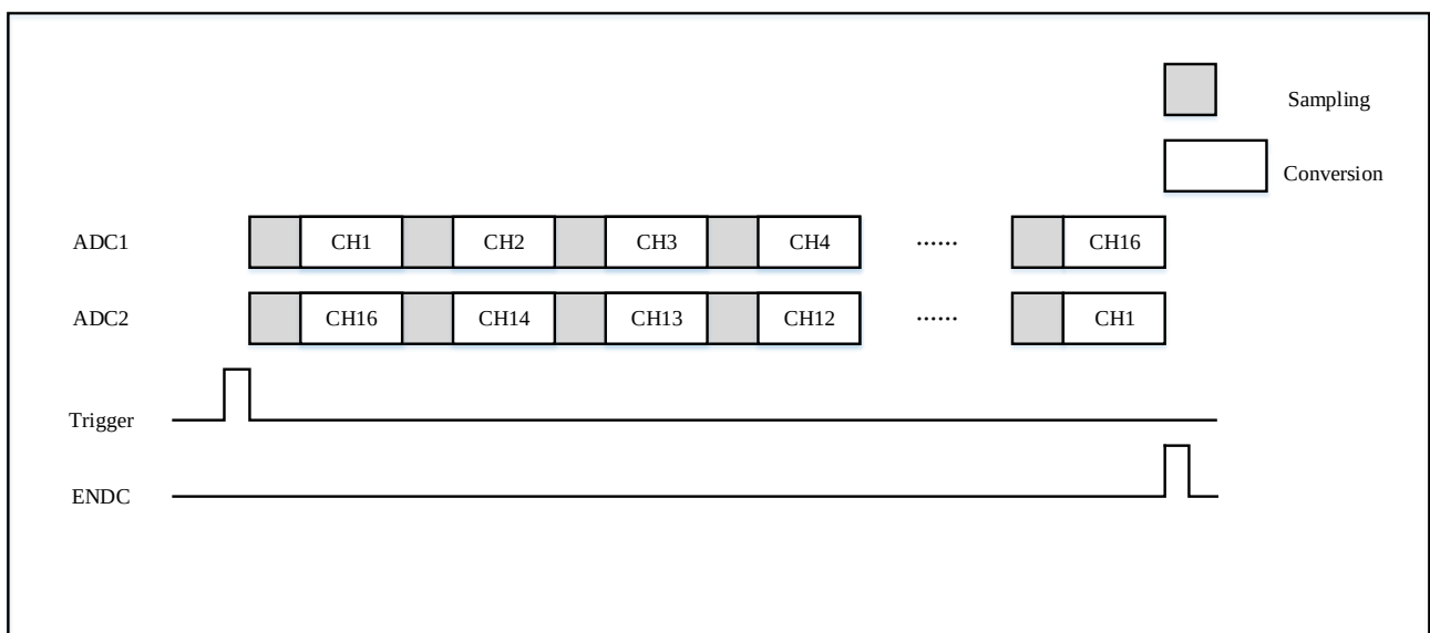
图 10-8 16 个通道的同步规则模式转换示意图
