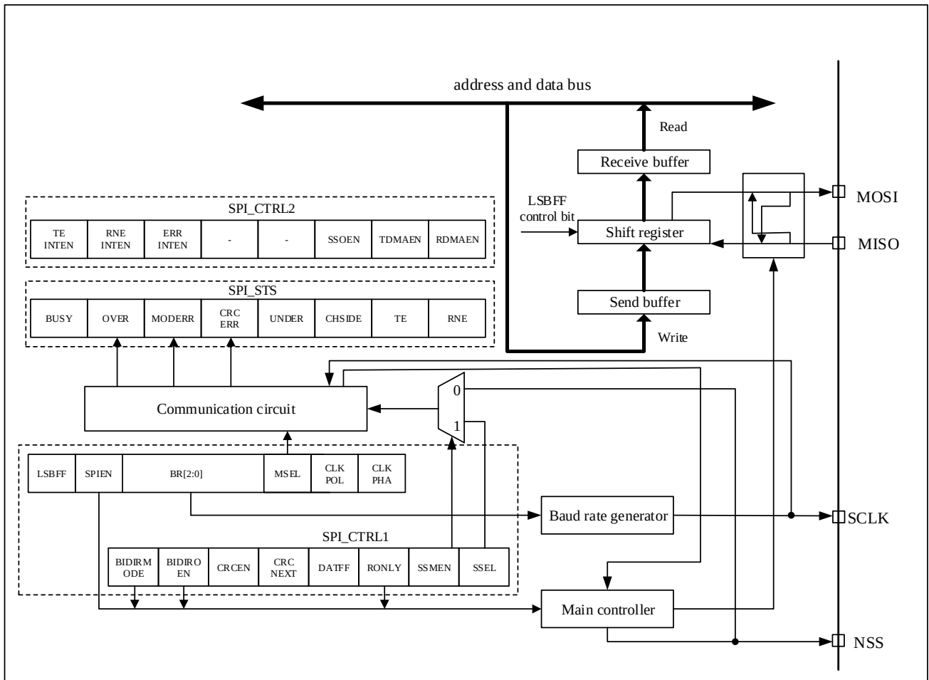
图 22-1 SPI 框图
