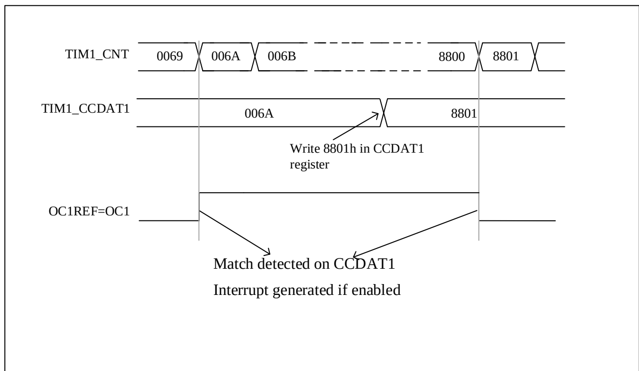
图 13-17 输出比较模式，开启 OC1
