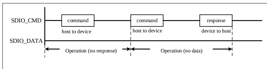
图 19-2 SDIO（多）数据块读操作
