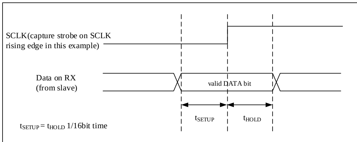
图 24-18 RX 数据采样/保持时间
