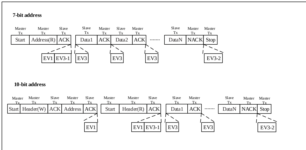
图 23-3 从发送器传送序列
