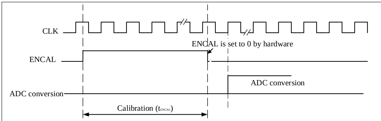
图 10-6 校准时序图
