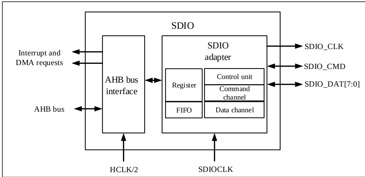
图 19-6 SDIO 框图
