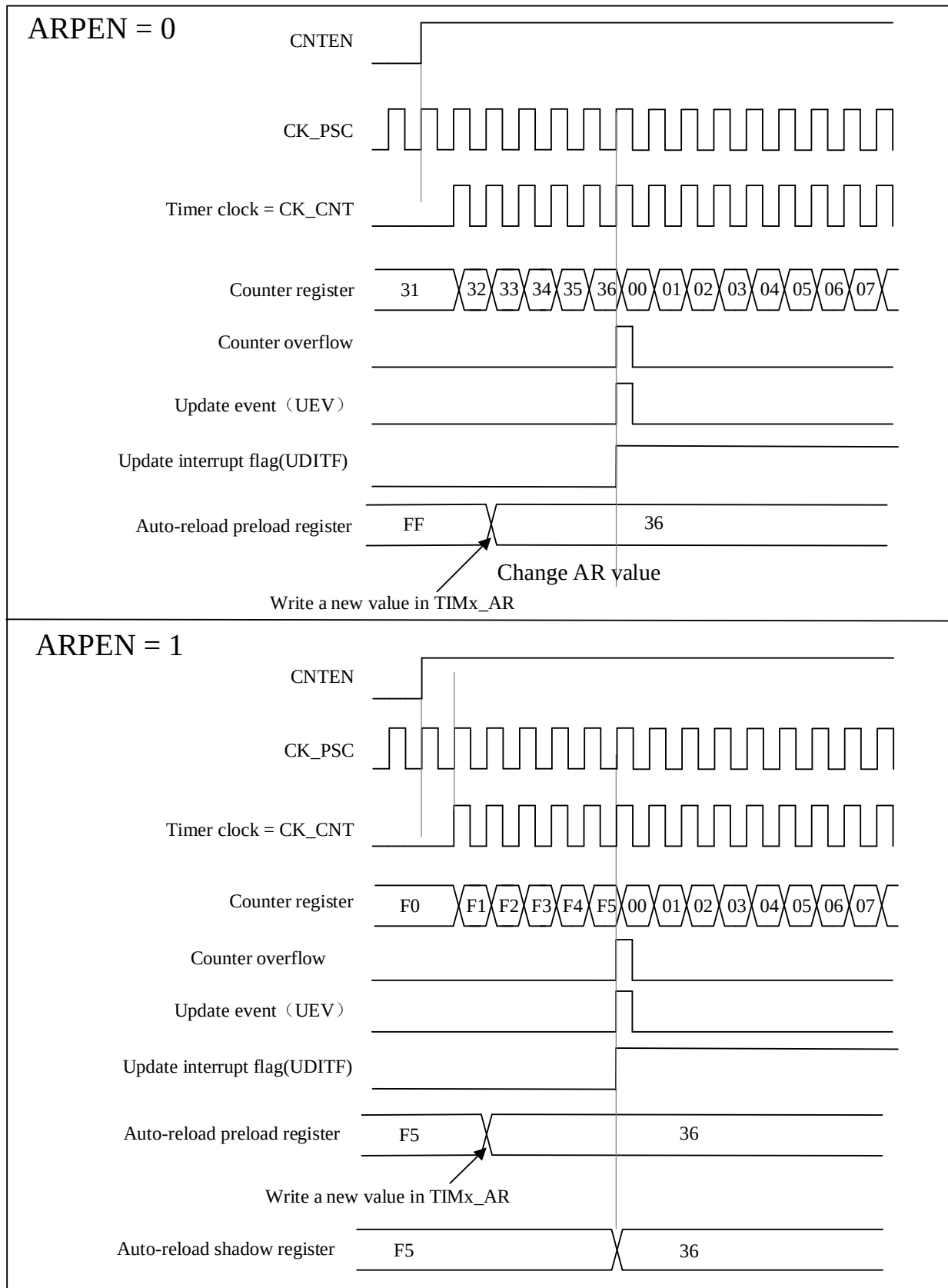
图 14-4 ARPEN=0/1 时向上计数、更新事件的时序图
