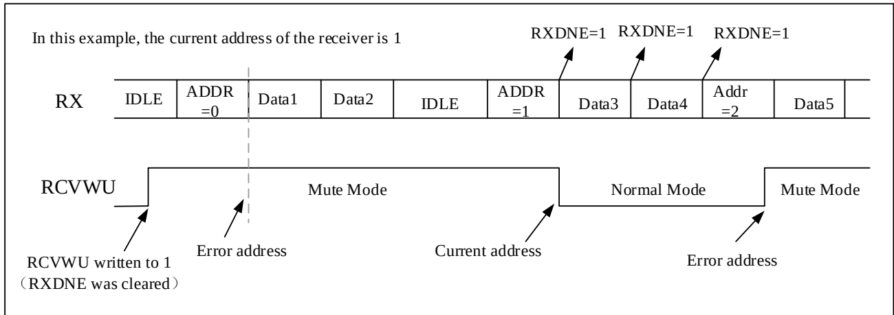
图 24-14 静默模式下的地址标识检测
