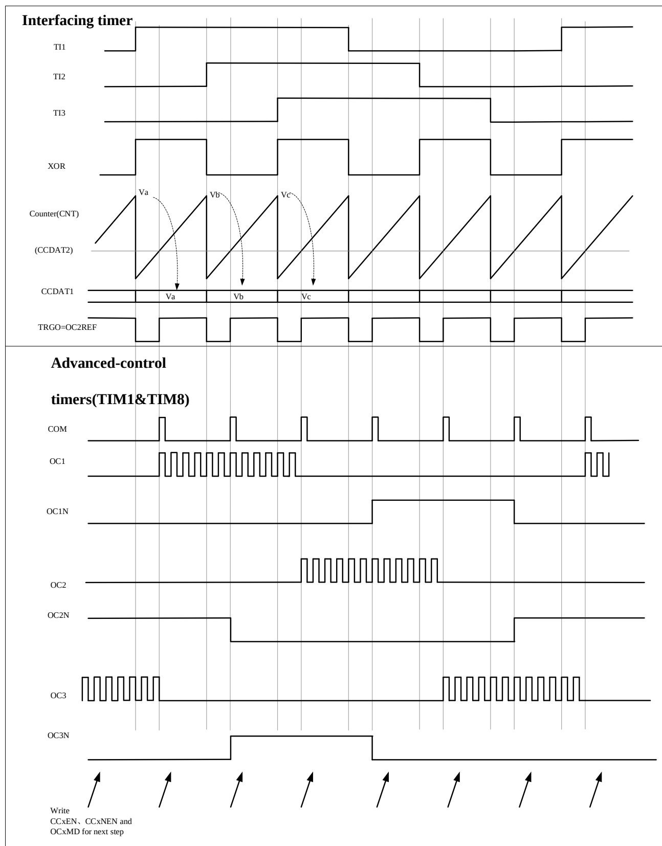
图 12-35 霍尔传感器接口的实例
