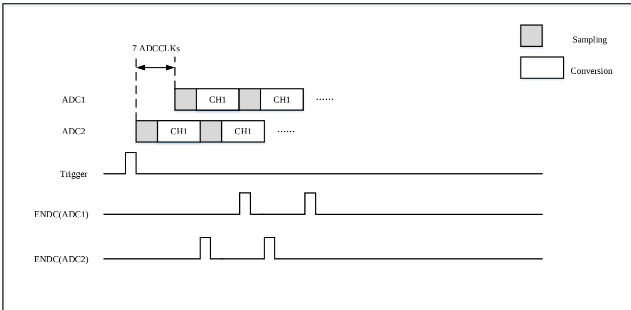
图 10-10 1 个通道的连续转换的快速交叉模式转换示意图
