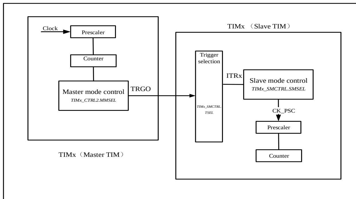
图 13-22 主/从定时器的例子
