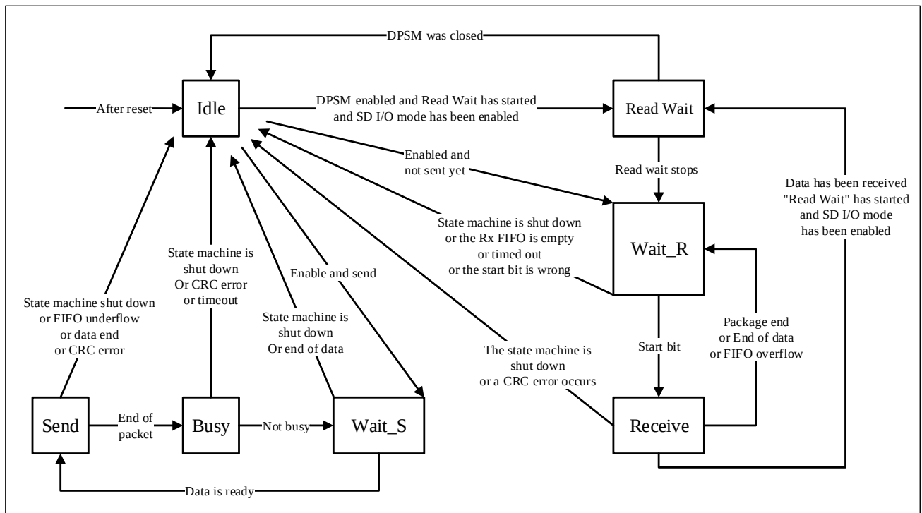
图 19-13 数据通道状态机（DPSM）
