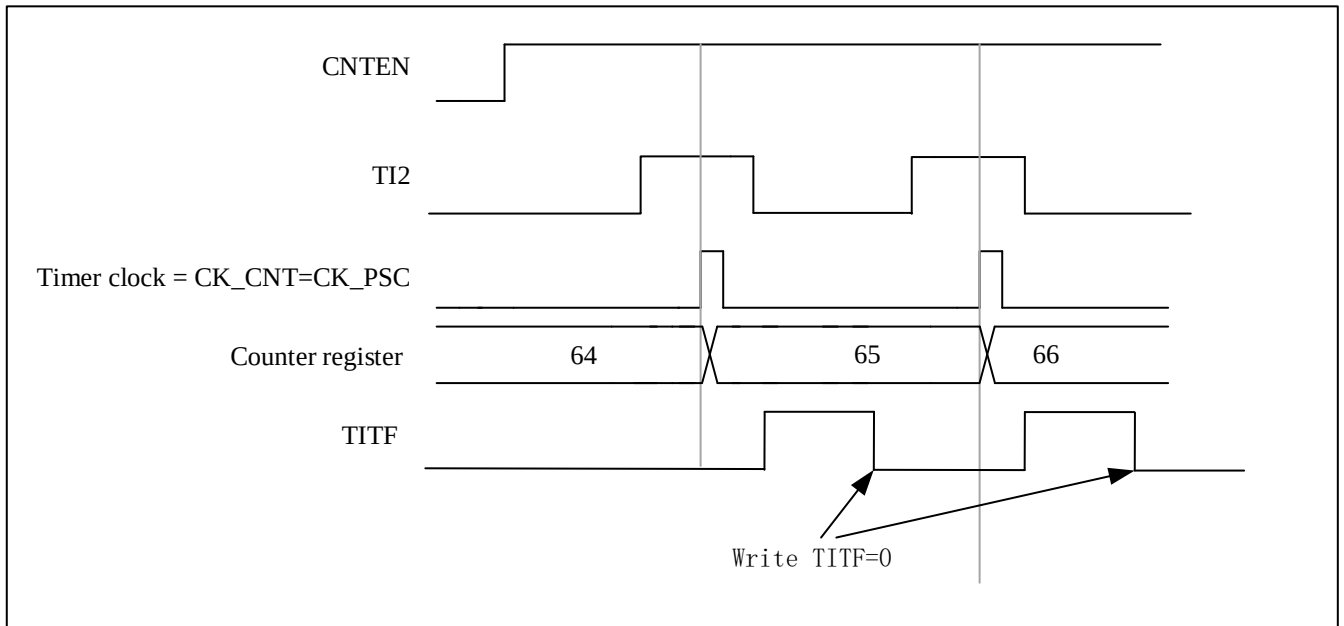
图 12-13 外部时钟模式 1 的控制电路
