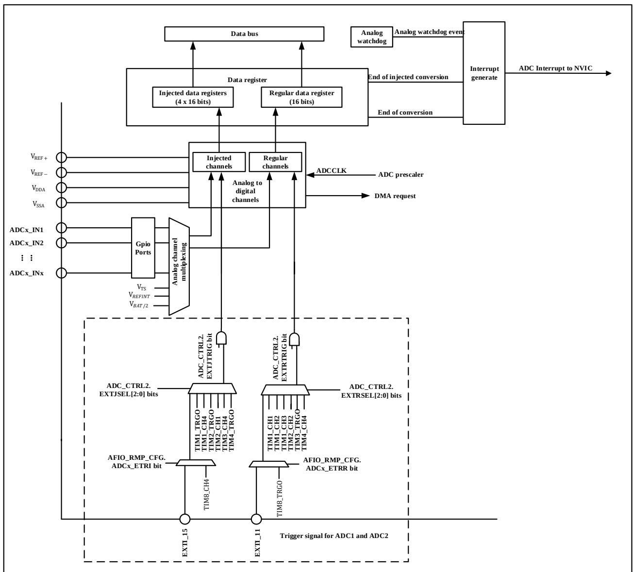
图 10-1 ADC 框图
