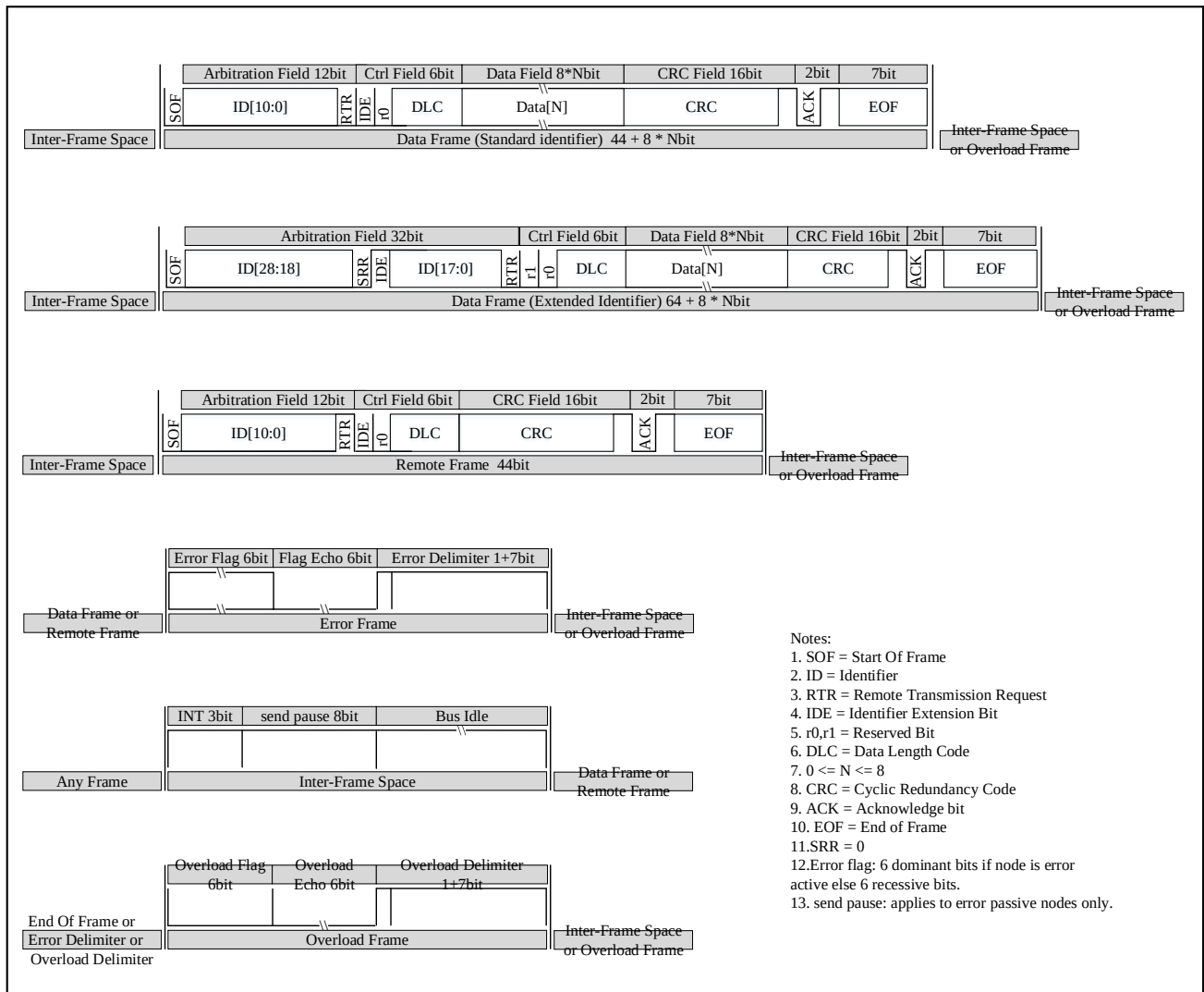
图 21-12 各类帧格式
