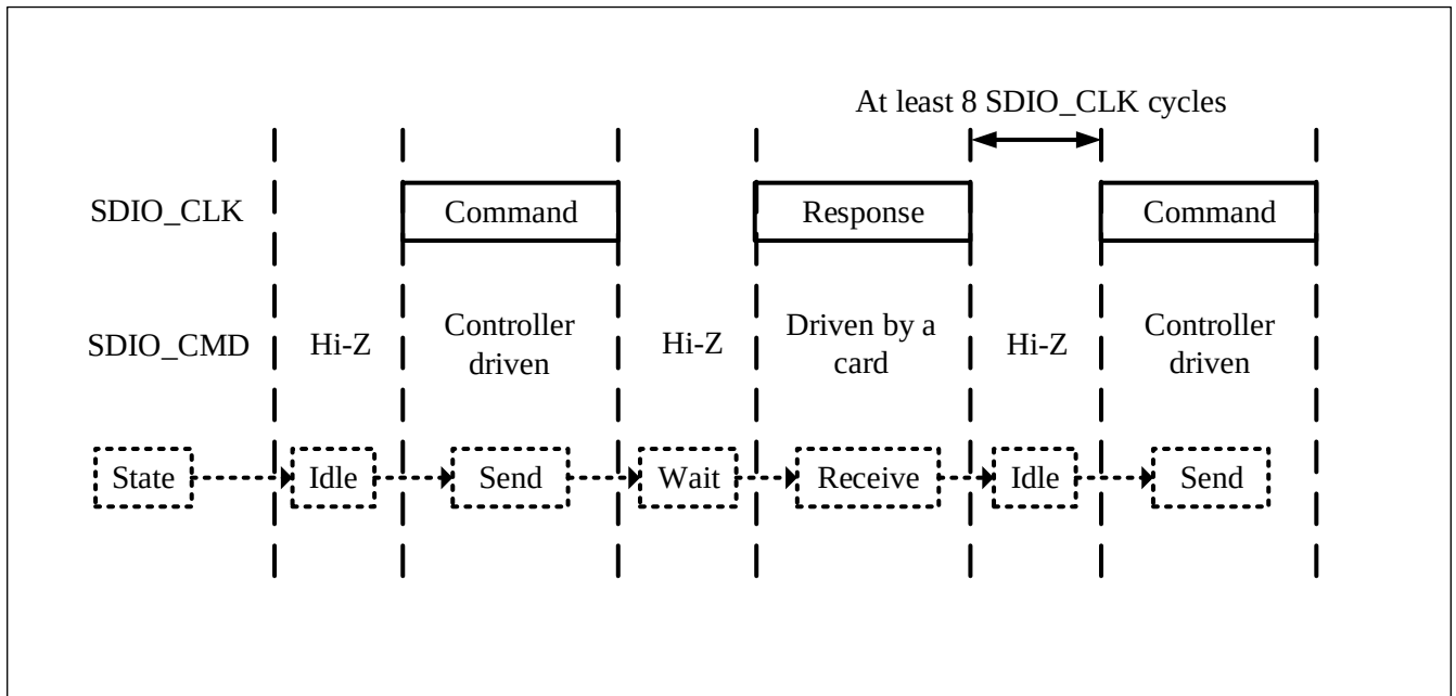
图 19-11 SDIO 命令传输
