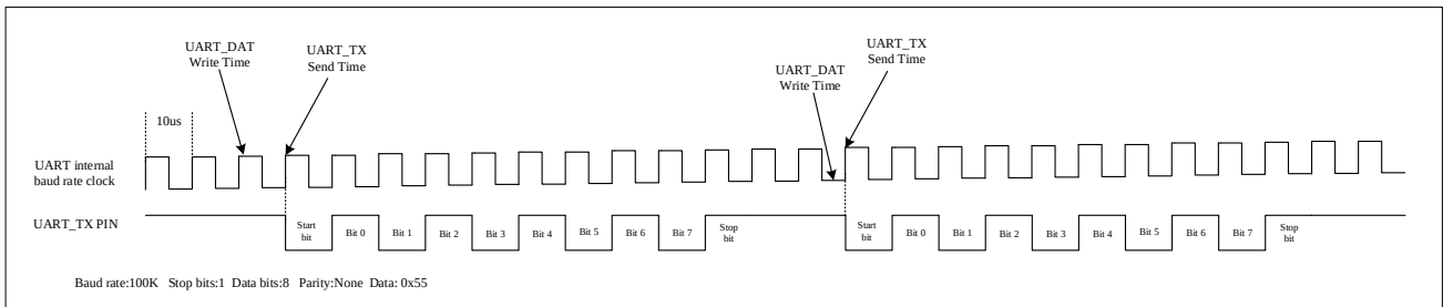
图 24-5 发送时差
