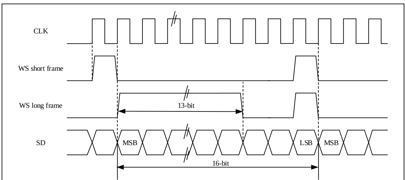
图 22-23 PCM 标准波形（16 位）
