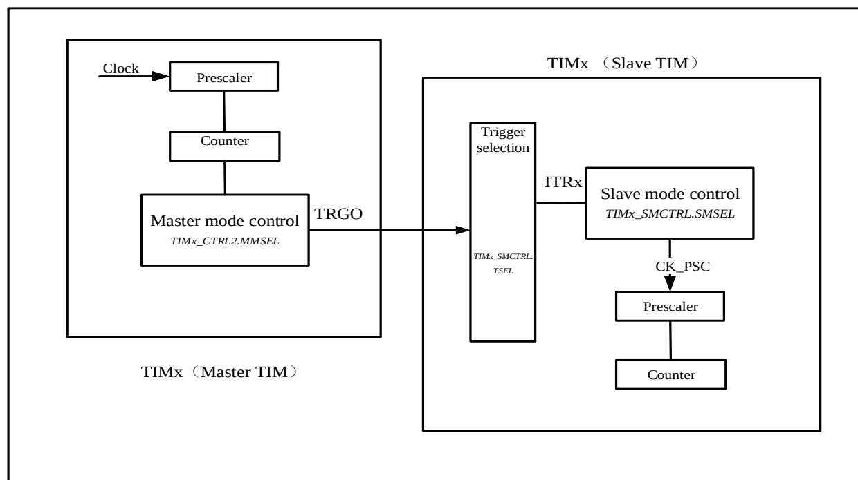
图 13-22 主/从定时器的例子
