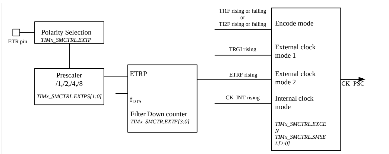
图 12-14 外部触发输入框图
