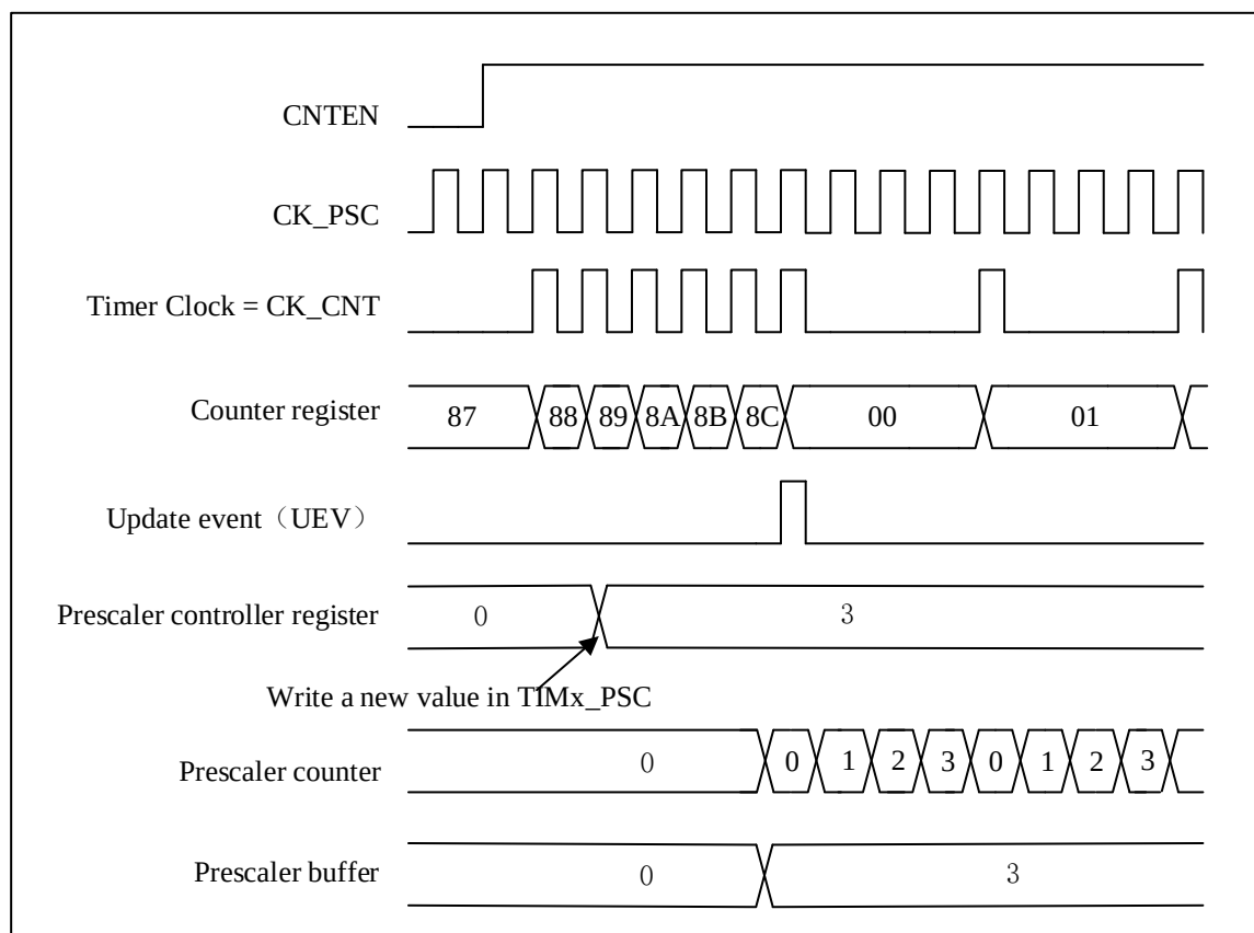
图 14-2 预分频器分频从 1 到 4 的计数器时序图
