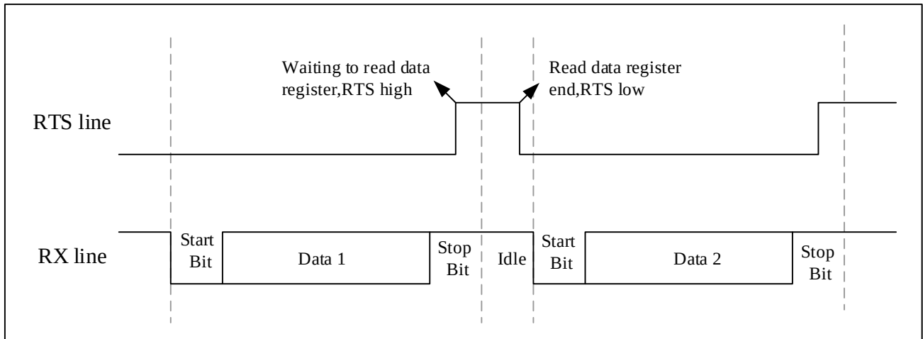
图 24-11 RTS 流控制
