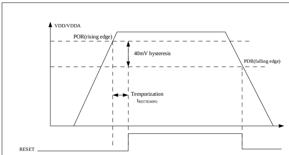
图 3-2 上电复位和掉电复位的波形图
