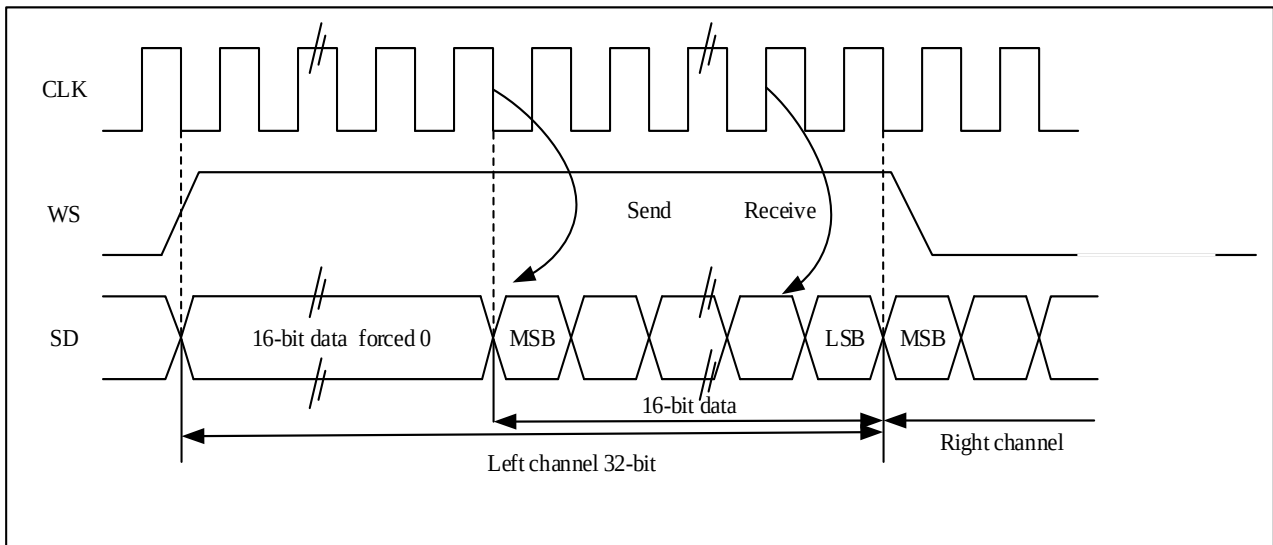
图 22-22 LSB 对齐 16 位数据扩展到 32 位包帧，CLKPOL = 0
