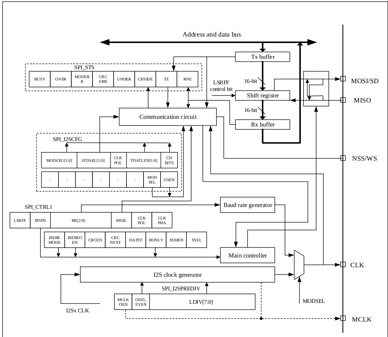
图 22-13 I 2 S 框图
