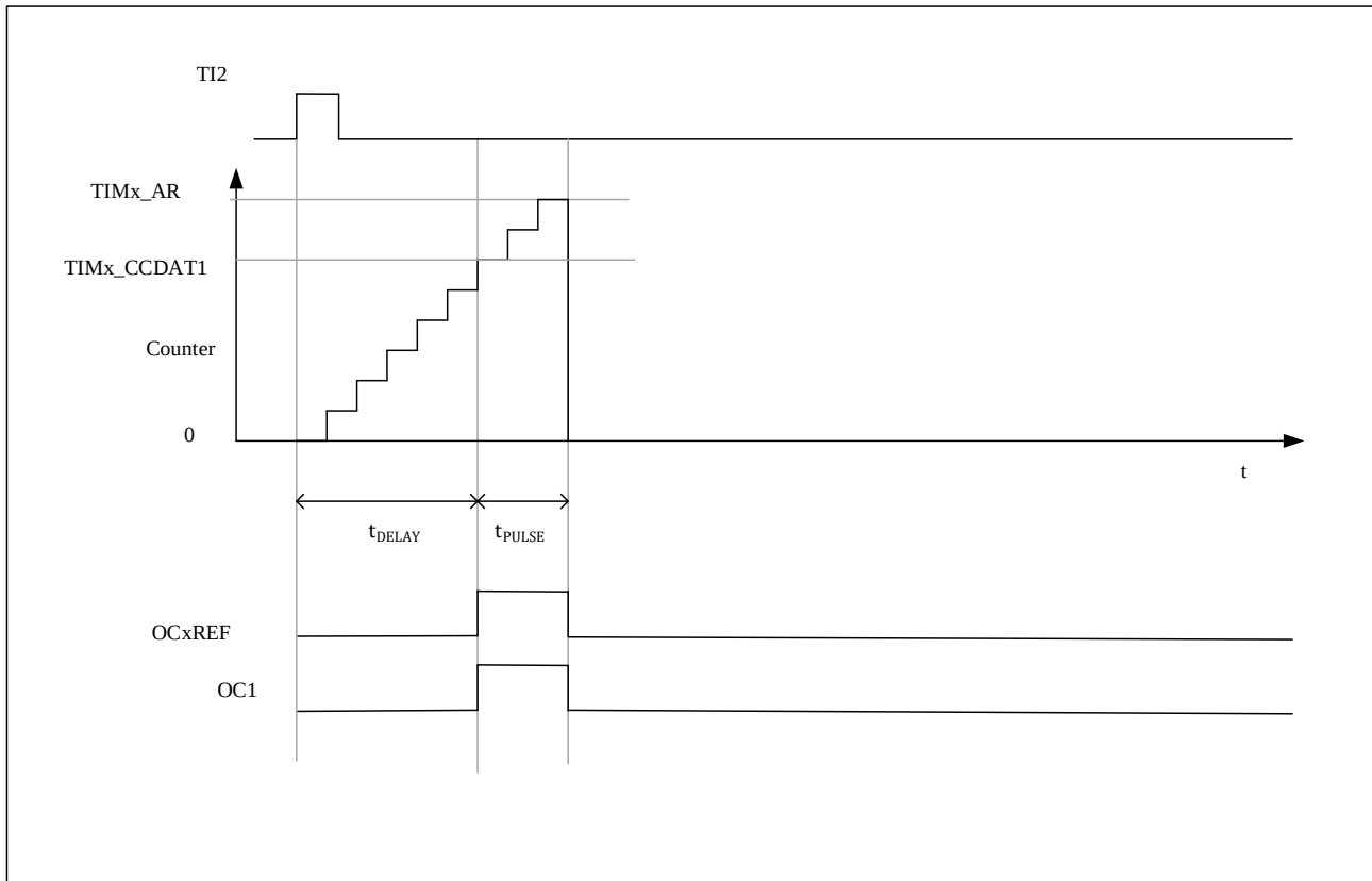
图 12-24 单脉冲模式示例
