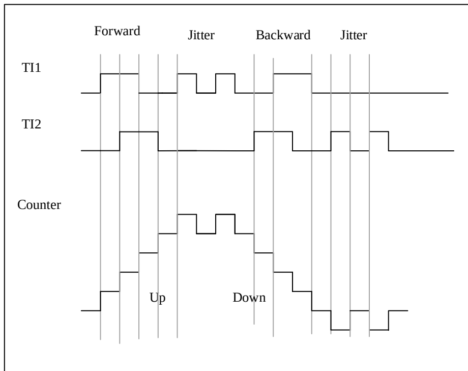
图 12-33 编码器模式下的计数器操作实例
