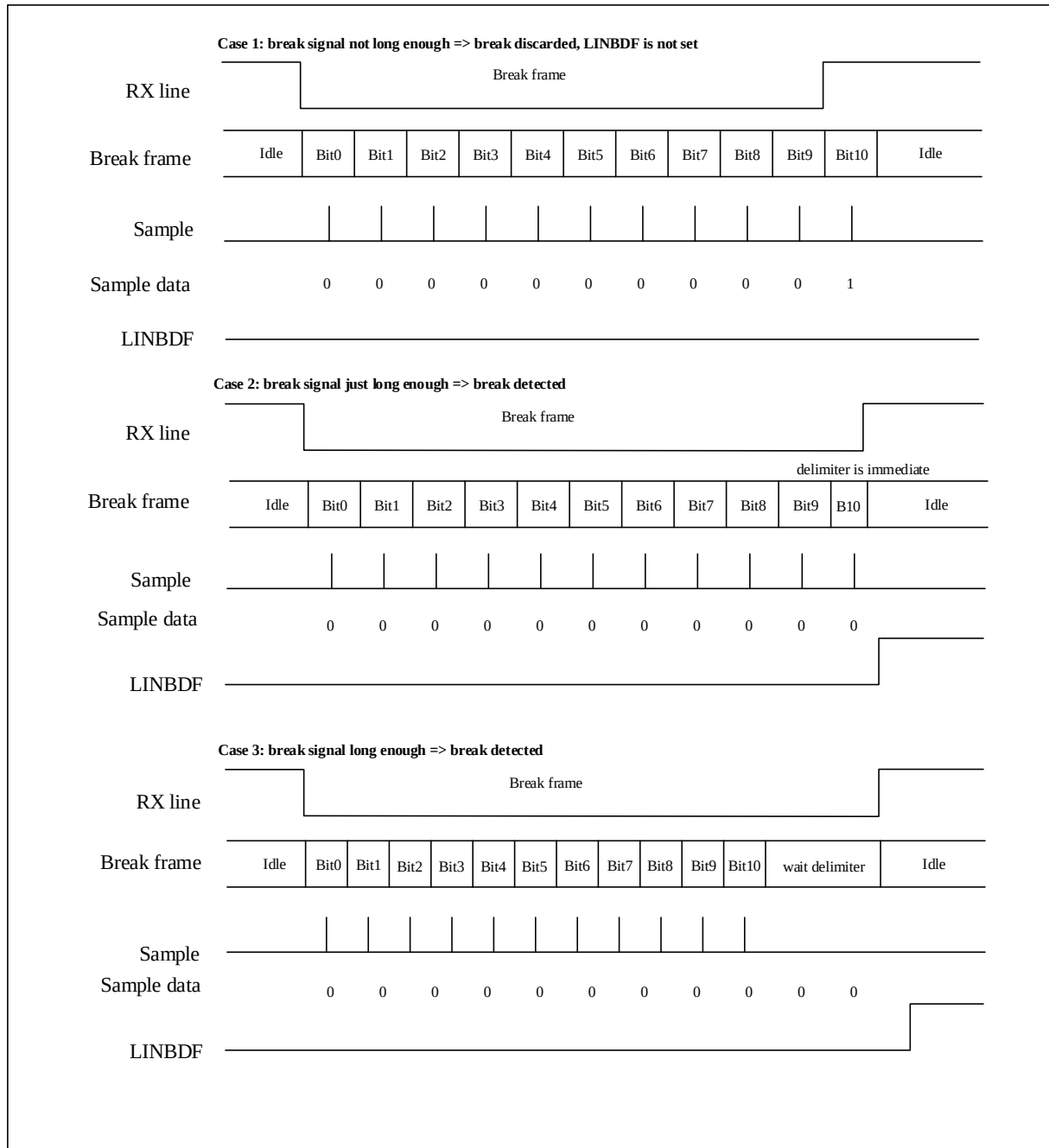
图 24-21 LIN 模式下的断开检测（11 位断开帧长度-设置了 LINBDL 位）
