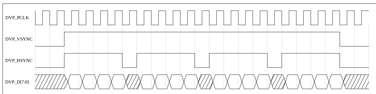
图 25-1 DVP 接口时序示例
