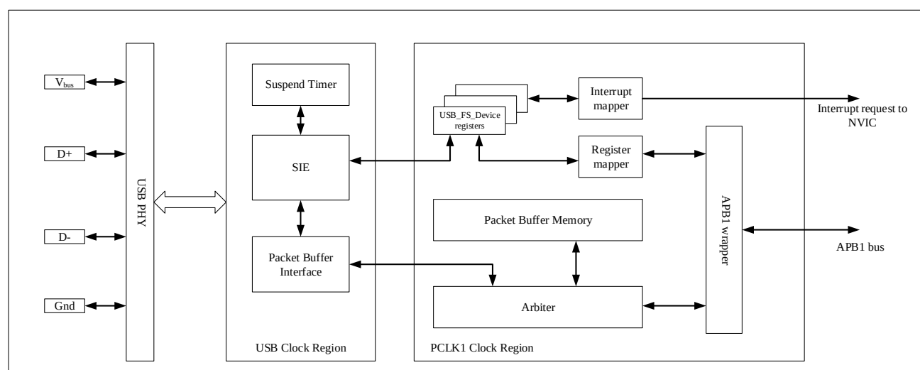
图 20-1 USB 设备框图
