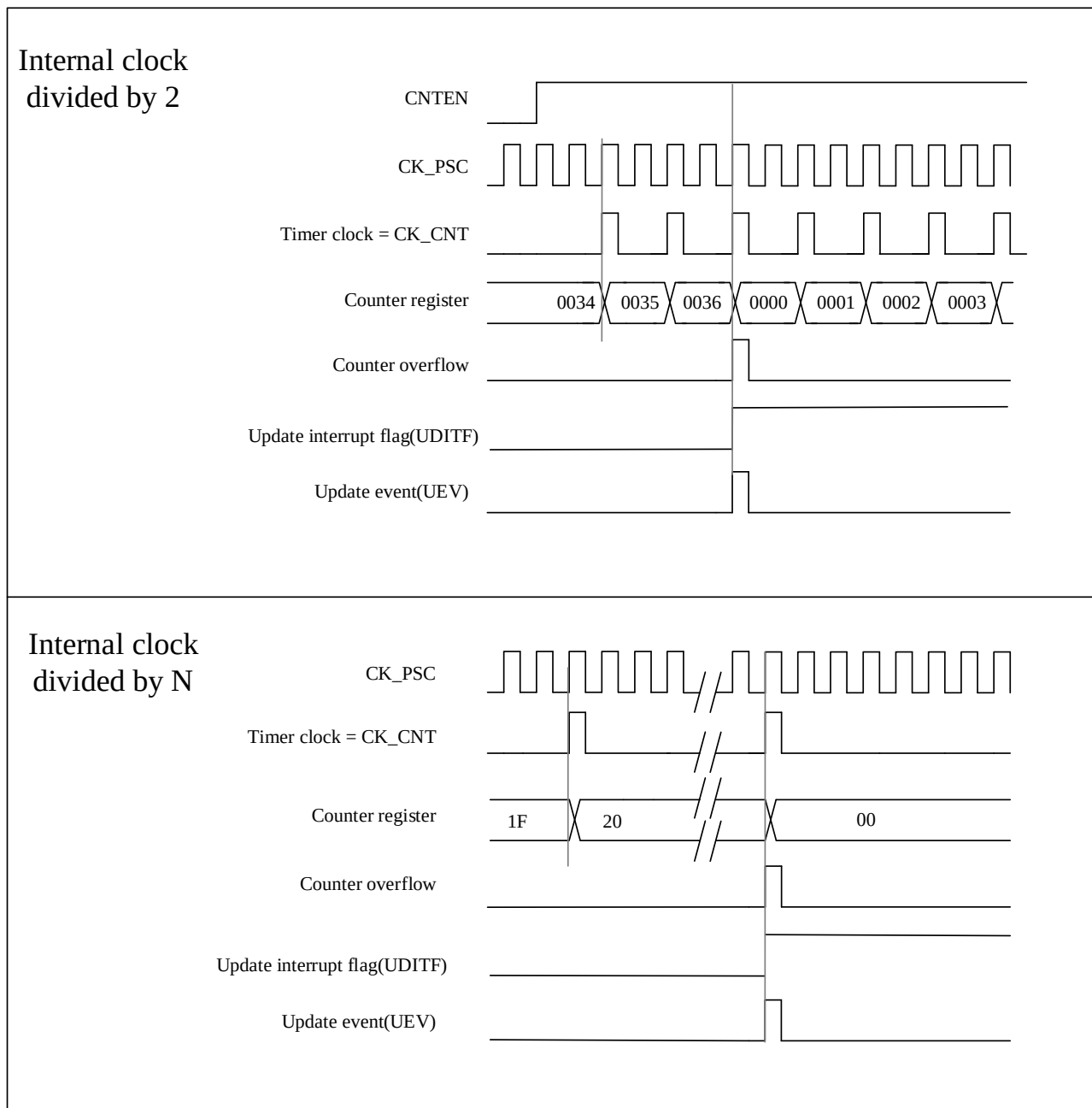
图 14-3 向上计数时序图，内部时钟分频因子 = 2/N
