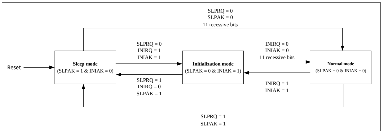
图 21-2 CAN 工作模式
