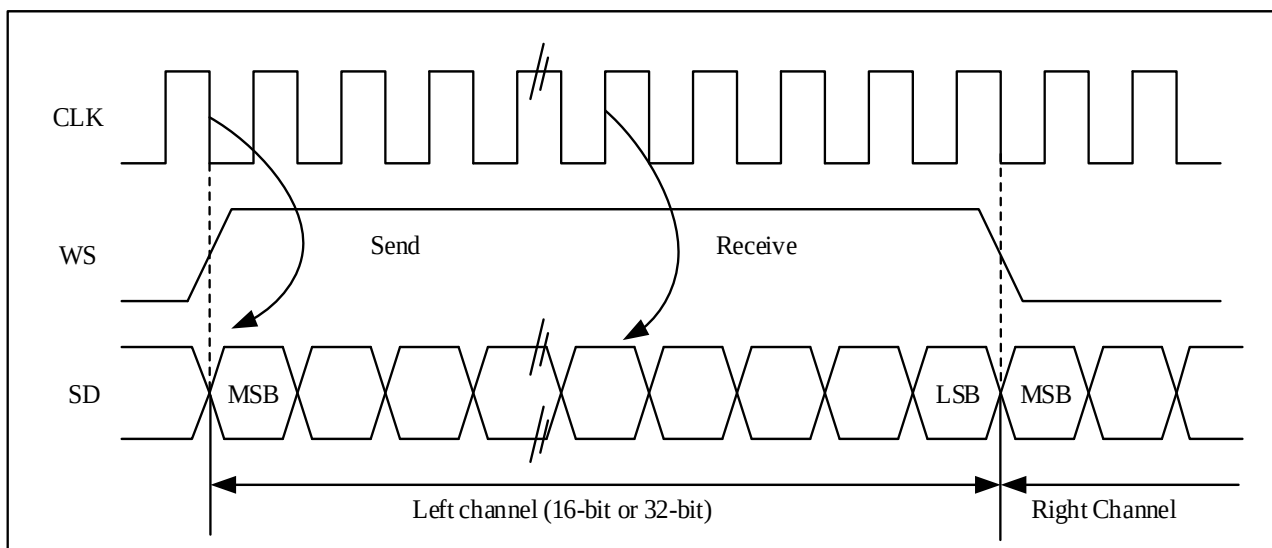
图 22-17 MSB 对齐 16 位或 32 位全精度，CLKPOL = 0
