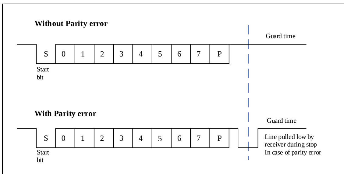
图 24-23 ISO7816-3 异步协议
