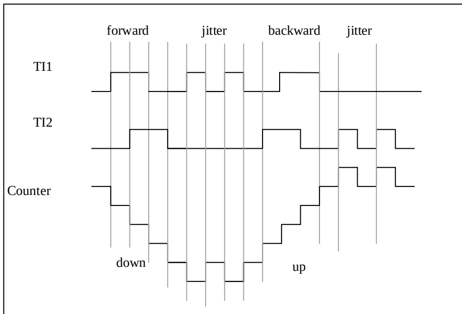
图 12-34 IC1FP1 反相的编码器接口模式实例
