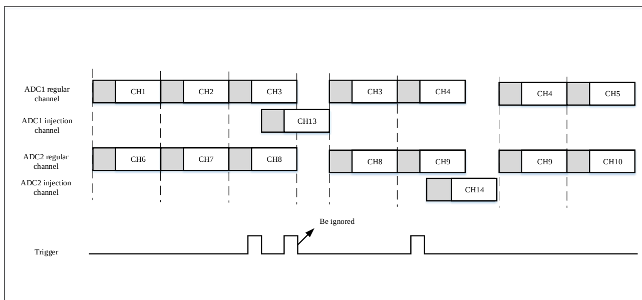
图 10-15 在注入转换期间发生注入触发
