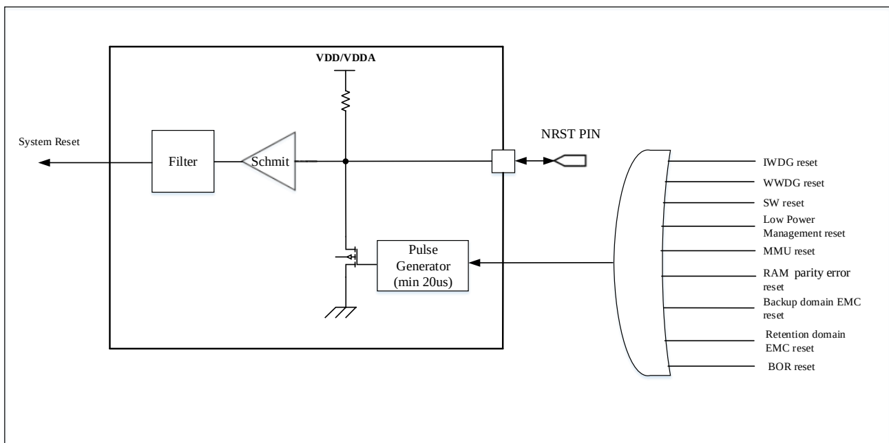
图 5-1 复位电路
