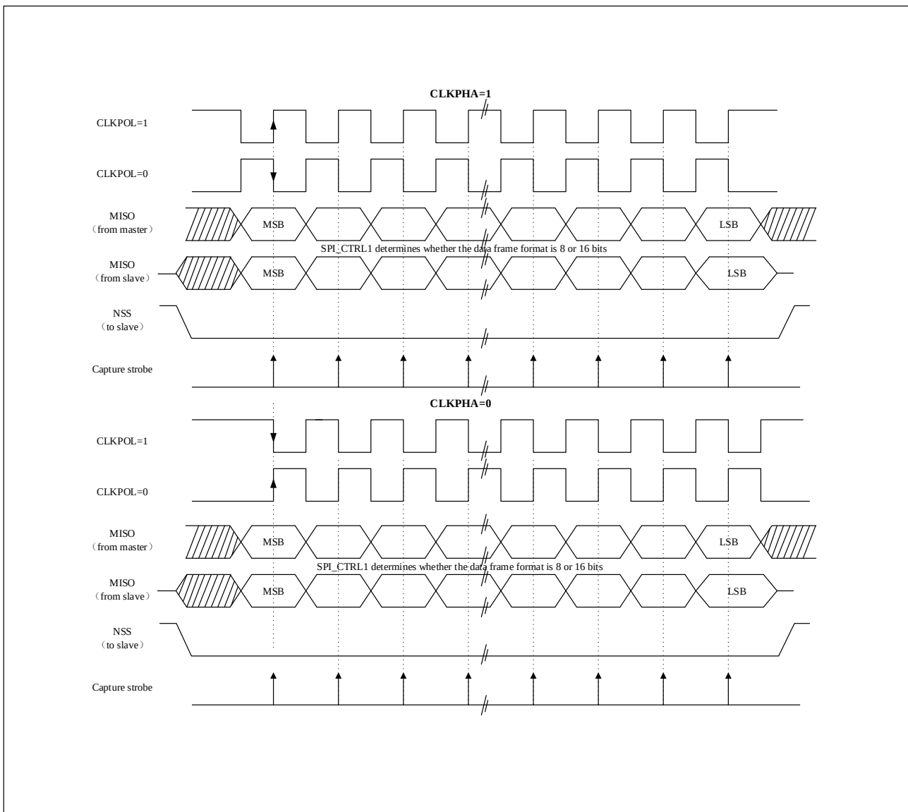
图 22-4 数据时钟时序图
