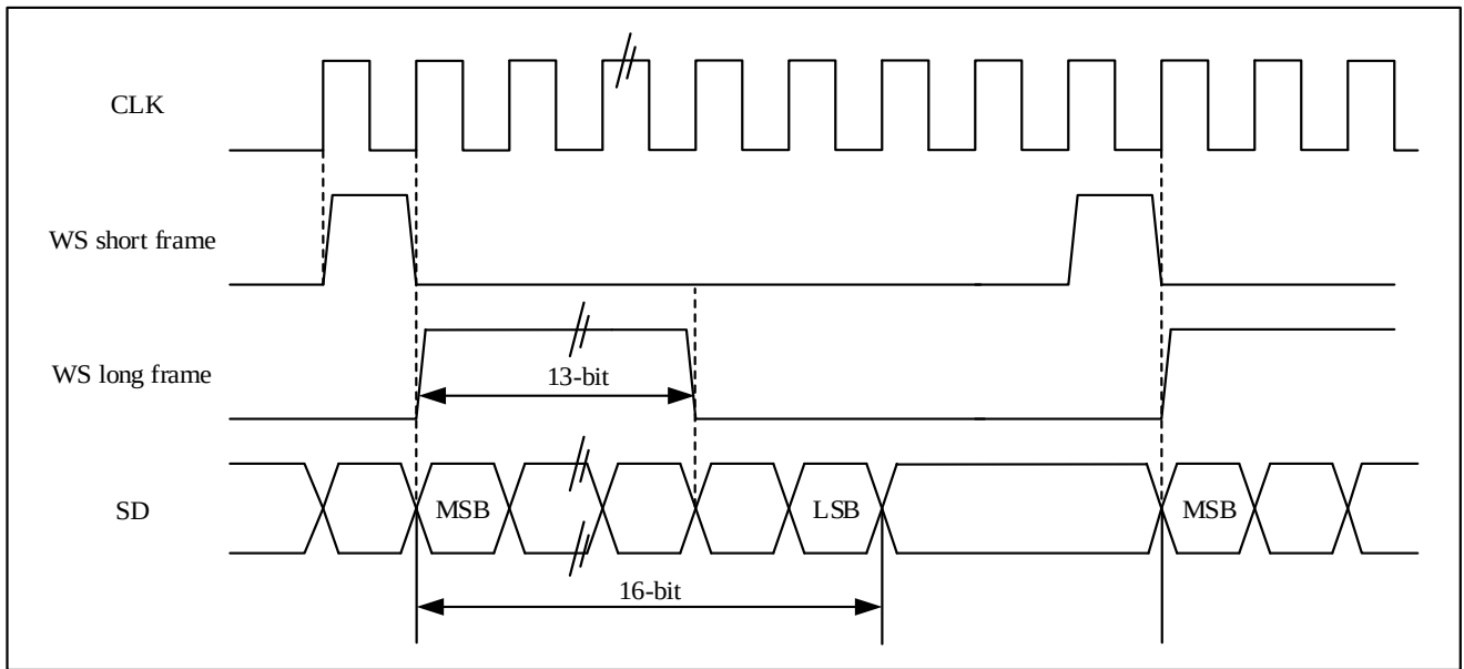
图 22-24 PCM 标准波形（16 位扩展到 32 位包帧）
