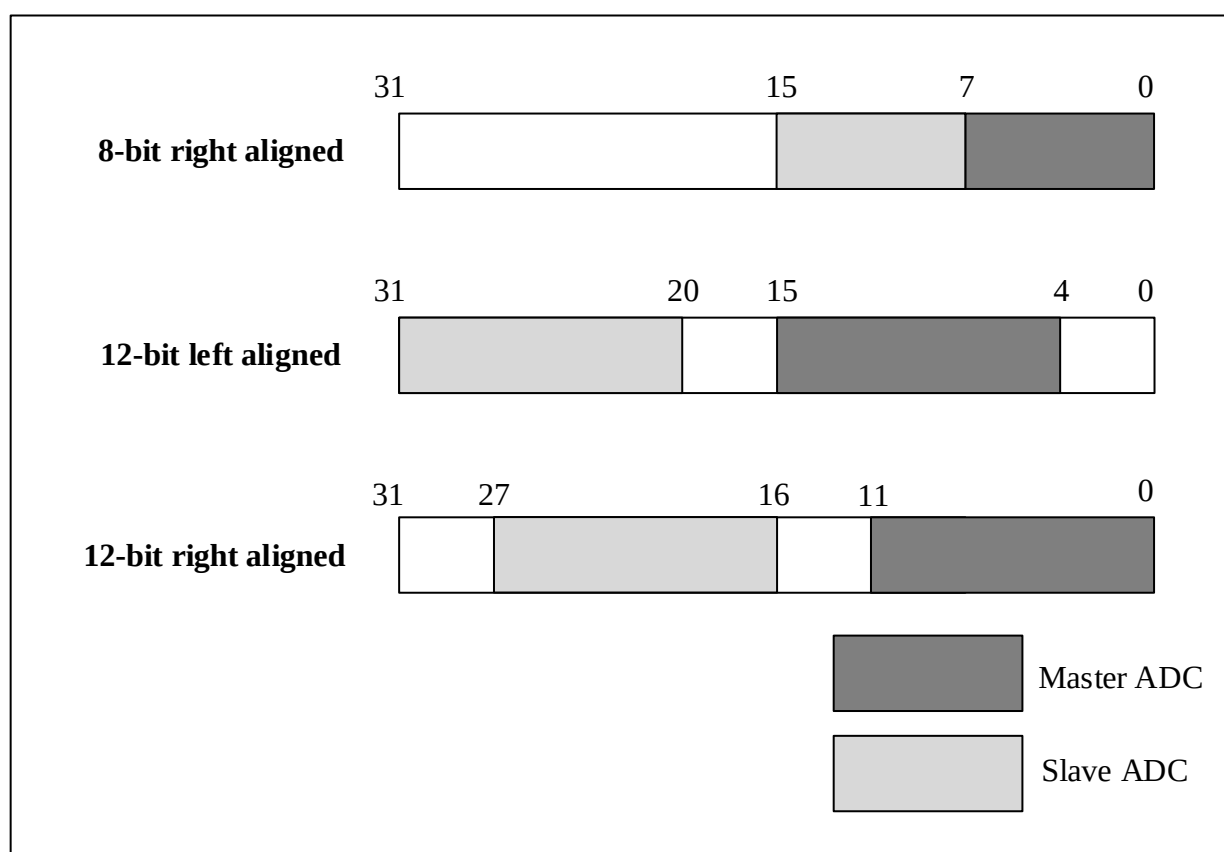
图 11-3 DAC 同步输出时的数据格式
