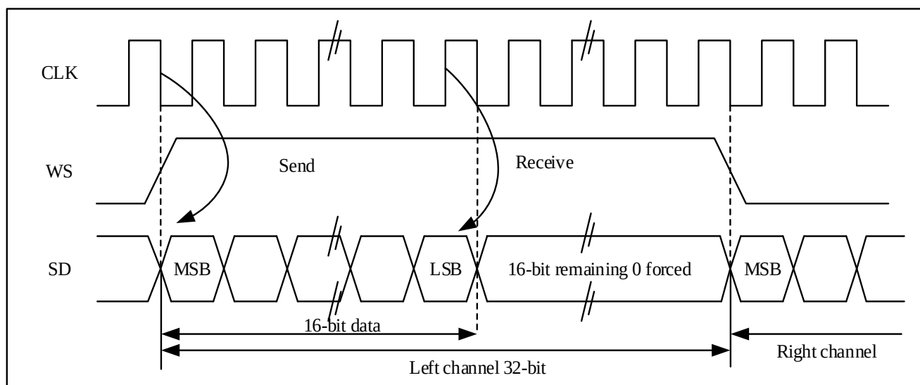
图 22-19 MSB 对齐 16 位数据扩展到 32 位包帧，CLKPOL = 0
