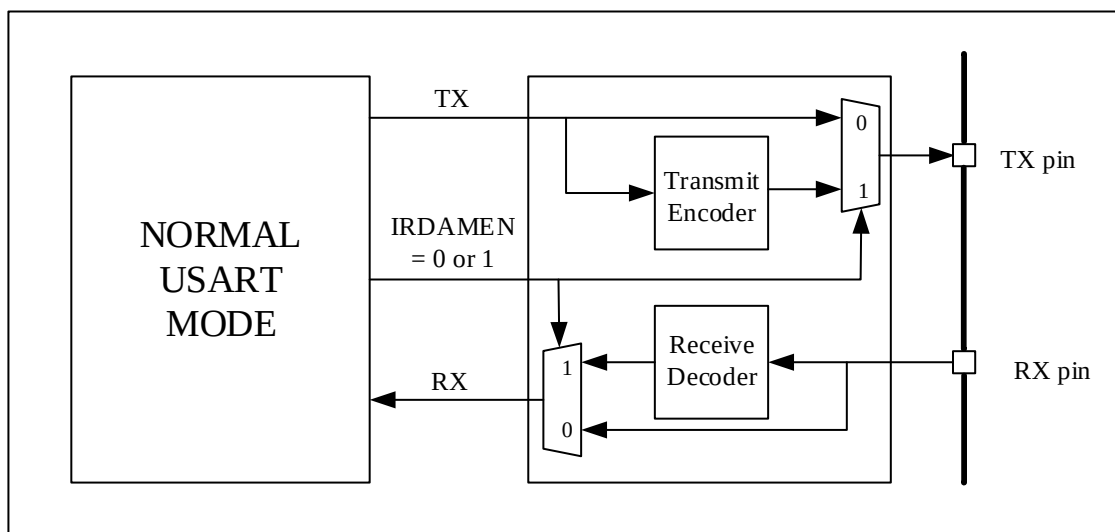
图 24-20 IrDA 数据调制 (3/16)-正常模式
