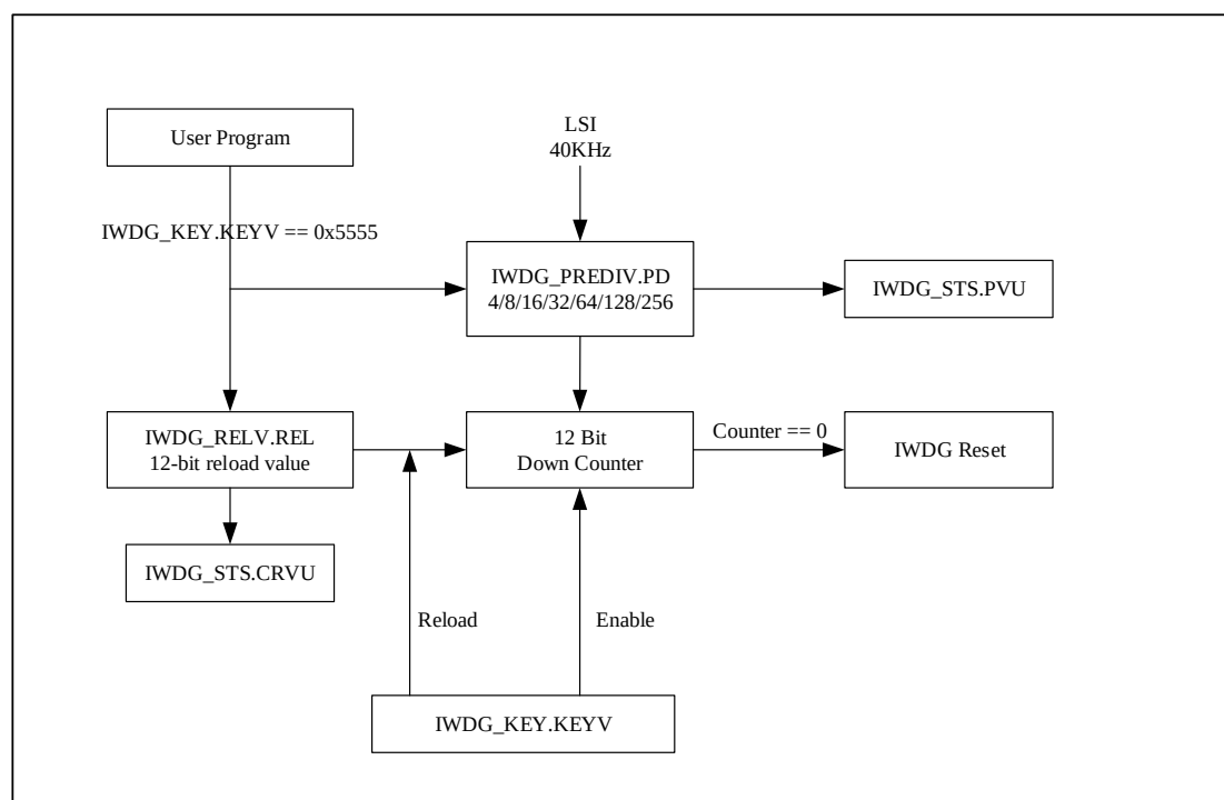
图 17-1 独立看门功能框图
