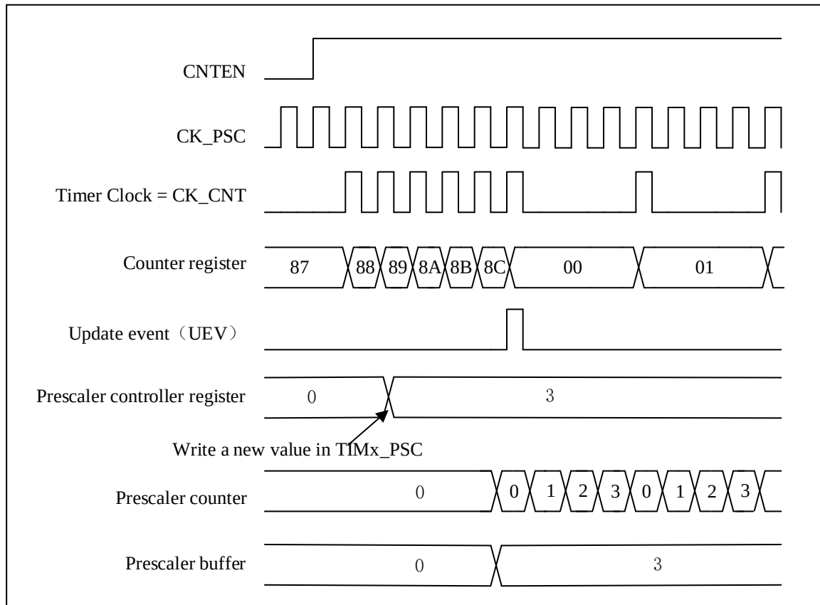
图 14-2 预分频器分频从 1 到 4 的计数器时序图
