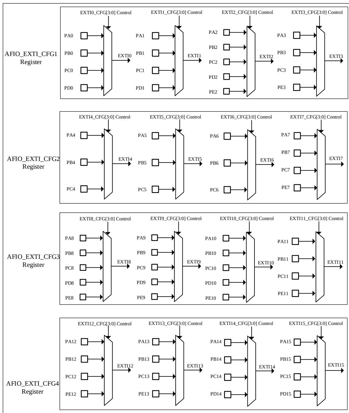
图 8-2 外部中断通用 I/O 映射
