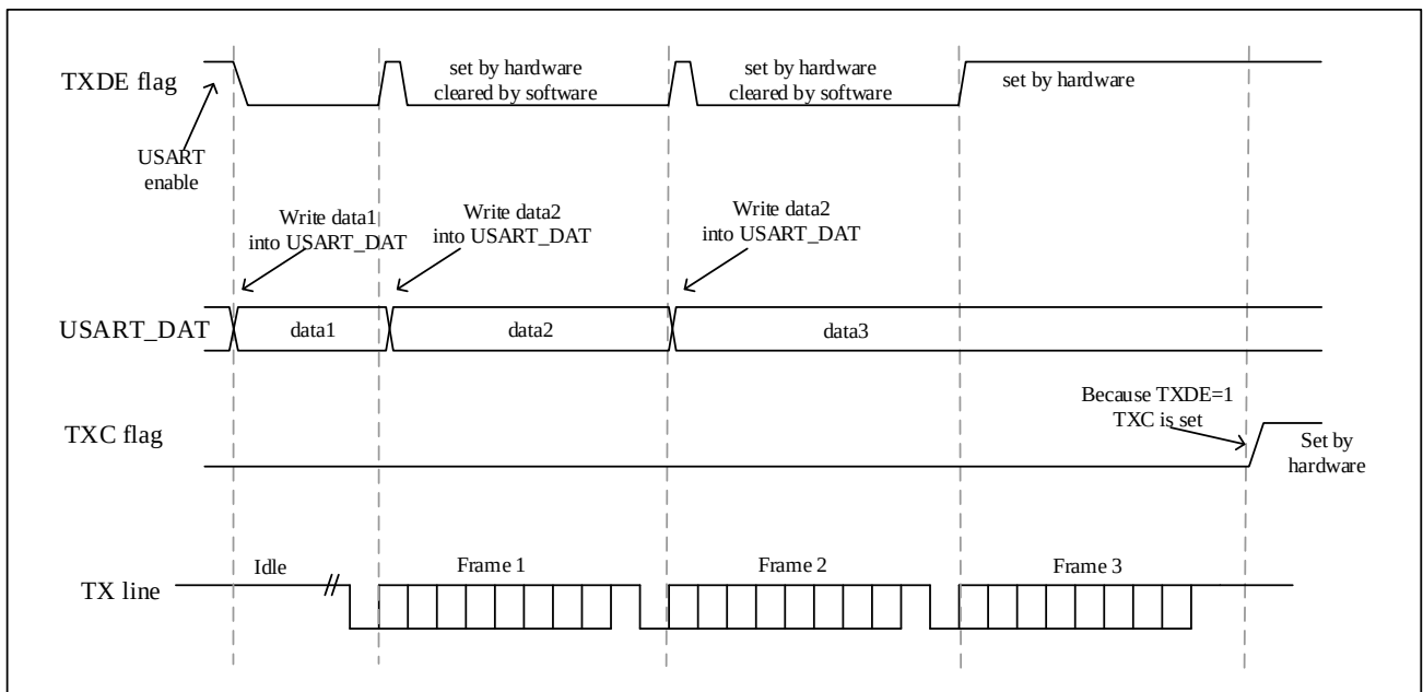
图 24-6 发送时 TXC/TXDE 的变化情况
