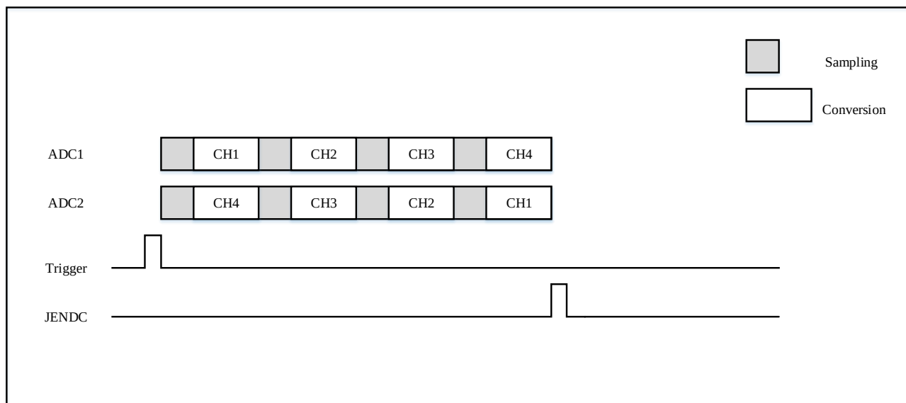
图 10-9 4 个通道的同步注入模式转换示意图
