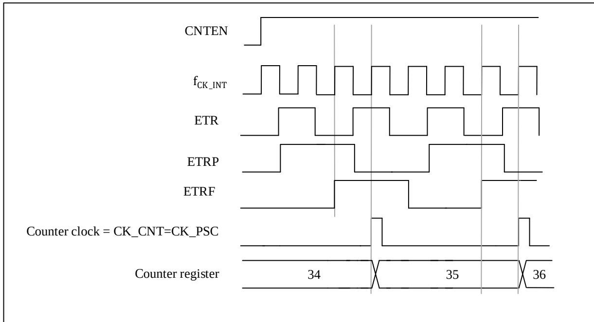
图 12-15 外部时钟模式 2 的控制电路
