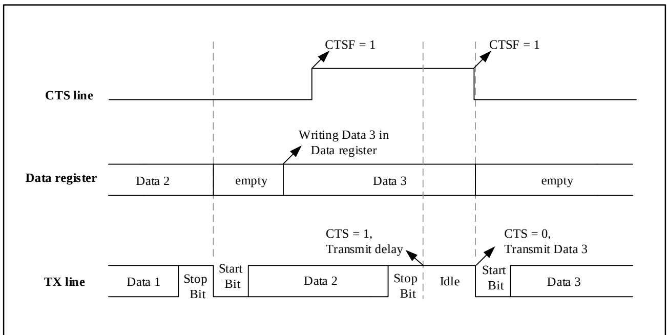
图 24-12 CTS 流控制
