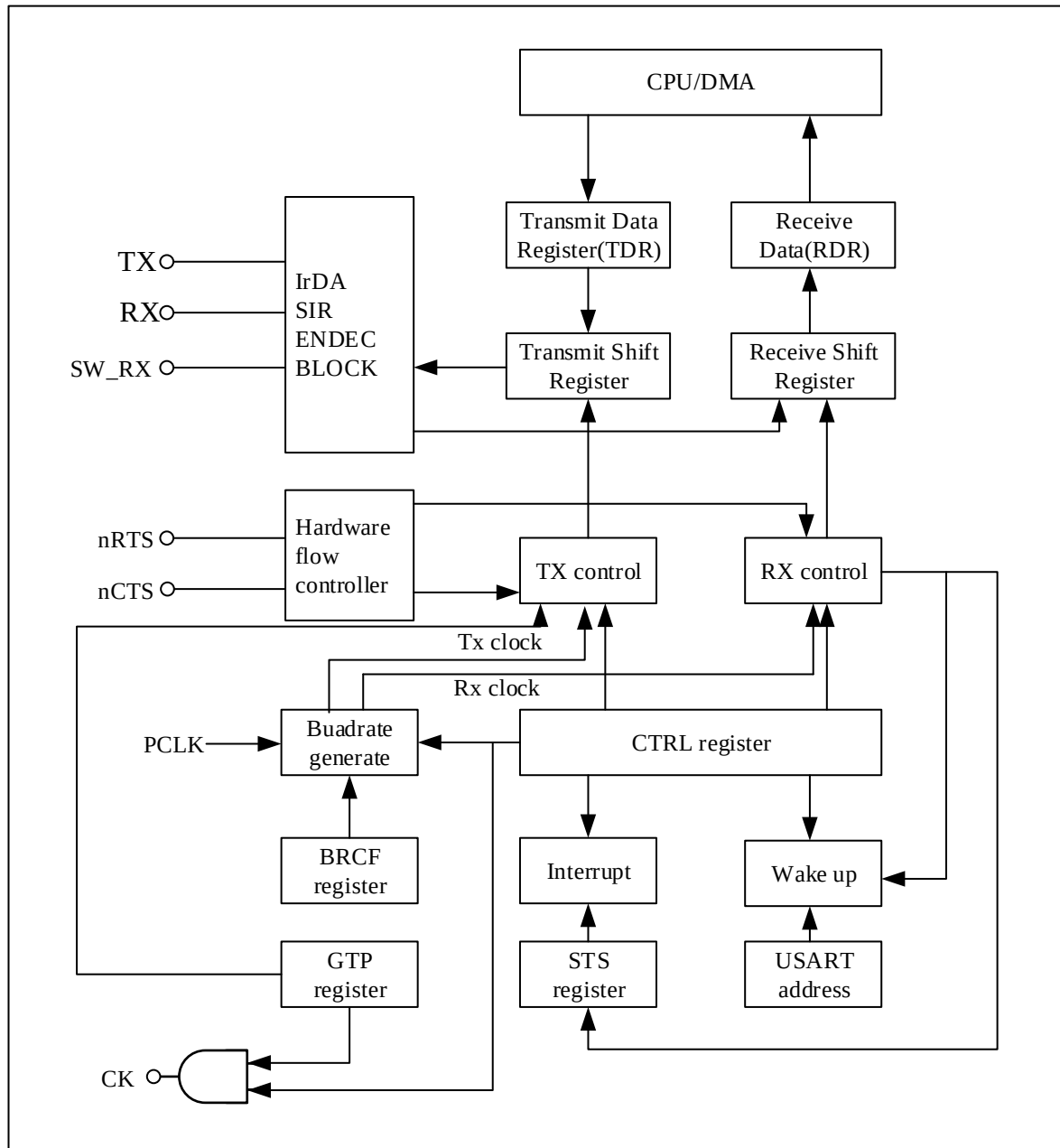
图 24-1 USART 框图
