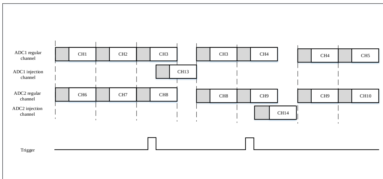
图 10-14 交替模式和规则同步模式组合
