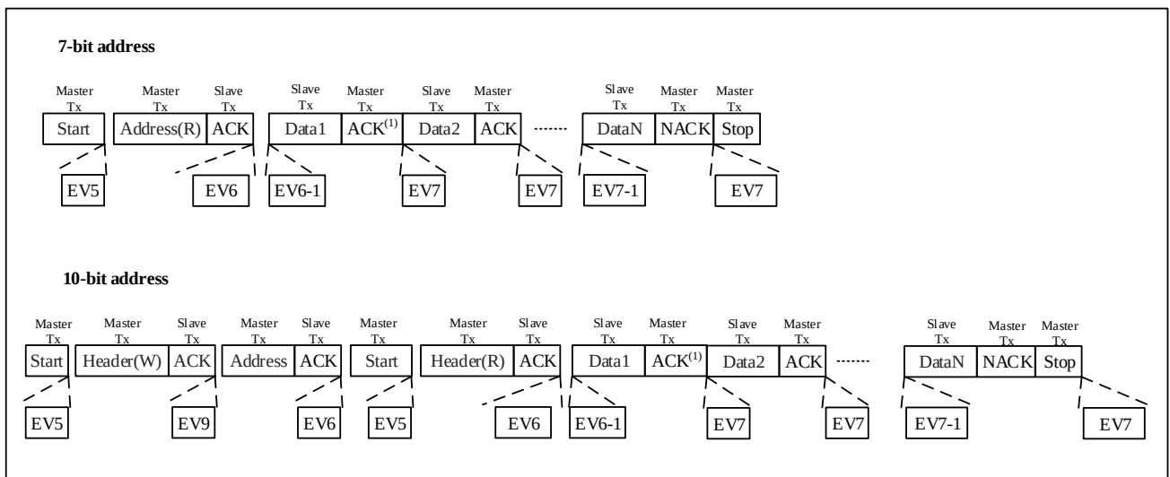
图 23-6 主接收器传送序列图
