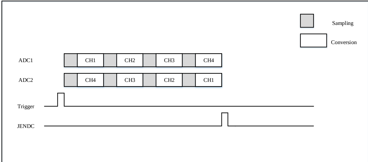
图 10-9 4 个通道的同步注入模式转换示意图
