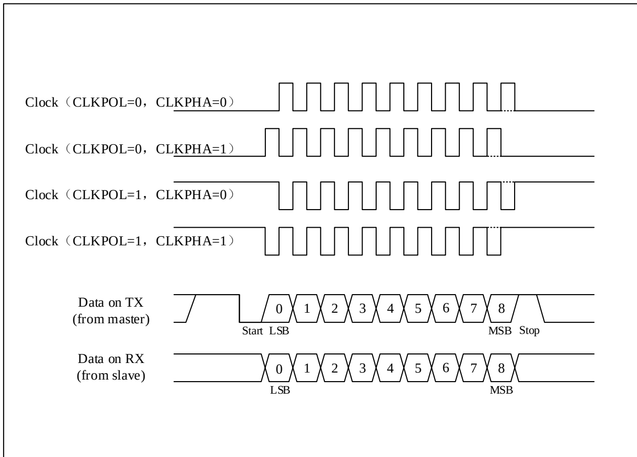
图 24-18 RX 数据采样/保持时间
