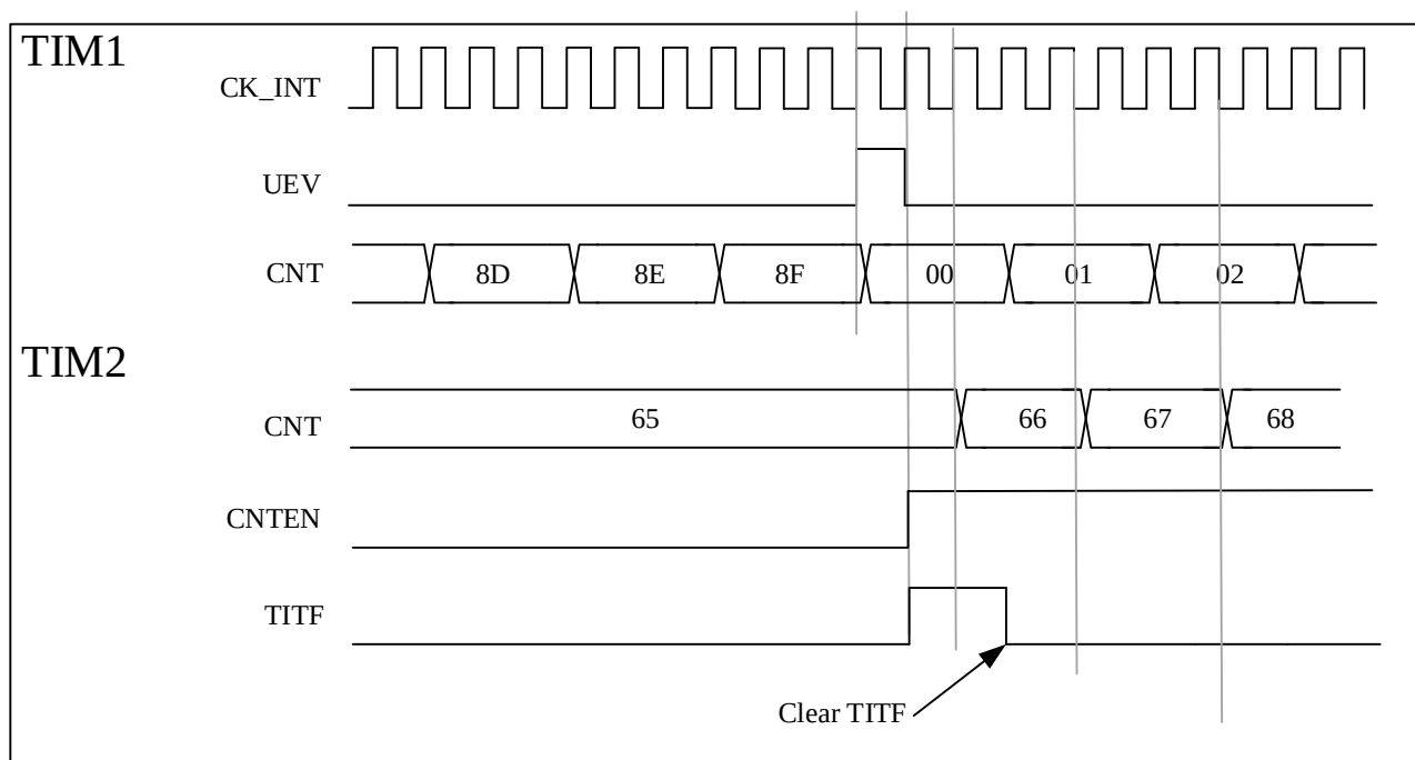
图 13-25 使用定时器 1 的更新触发定时器 2
