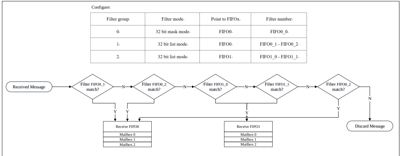
图 21-10 过滤机制示例
