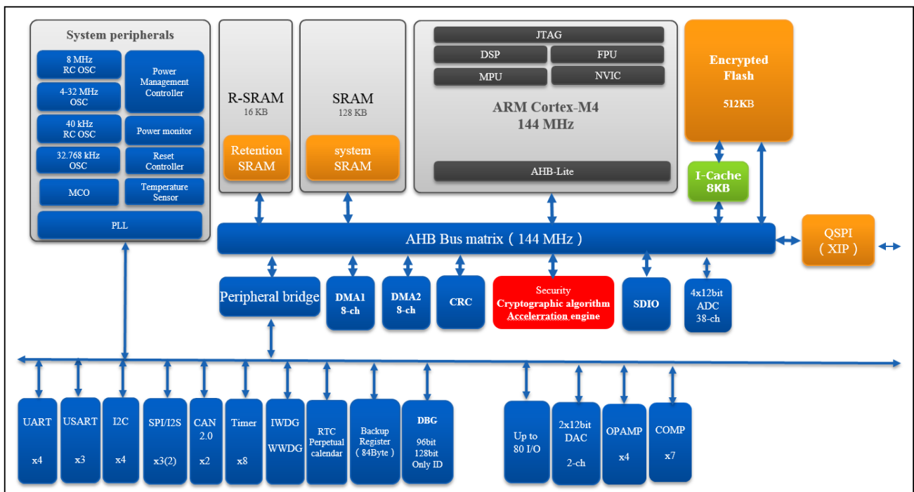
图 1-1 N32A455xxL7系列框图
