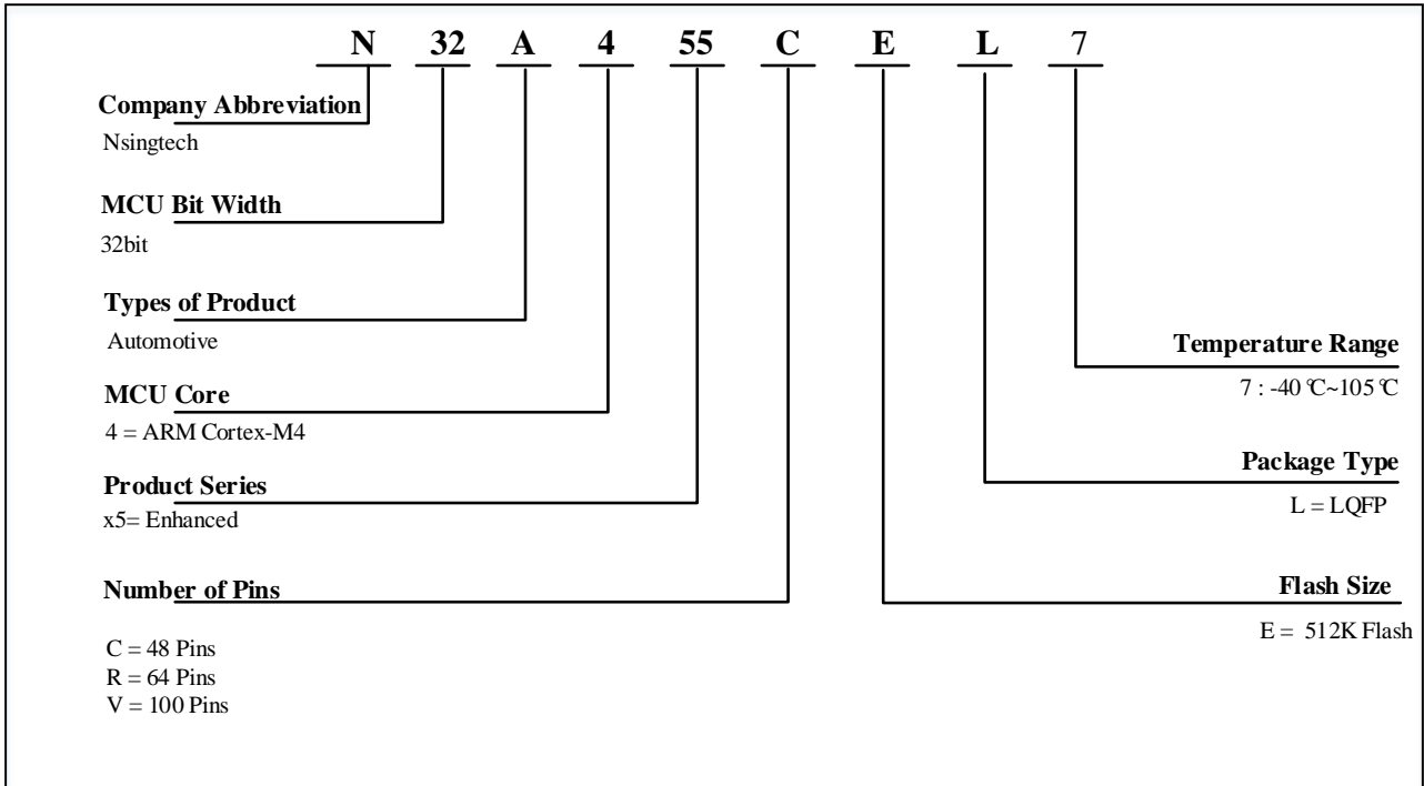
图 6-1 N32A455系列订货代码信息图示
