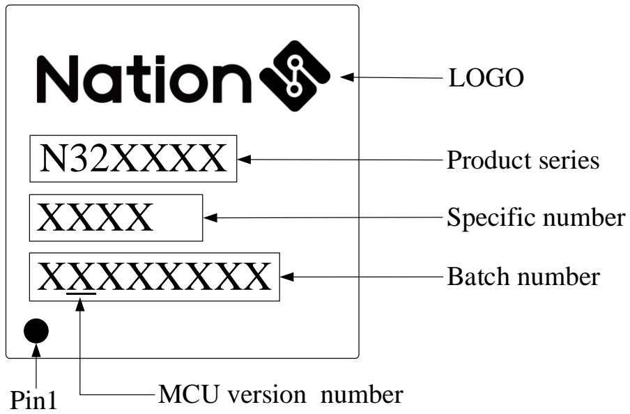
图 5-7 LQFP48/LQFP64/LQFP100 丝印说明
