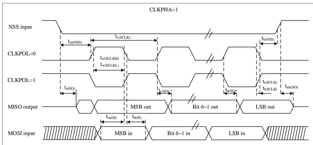
图 4-14 SPI时序图 – 从模式和CPHA=1 (1)
