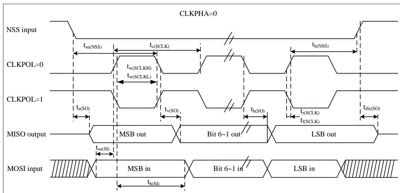
图 4-13 SPI时序图 – 从模式和CPHA=0
