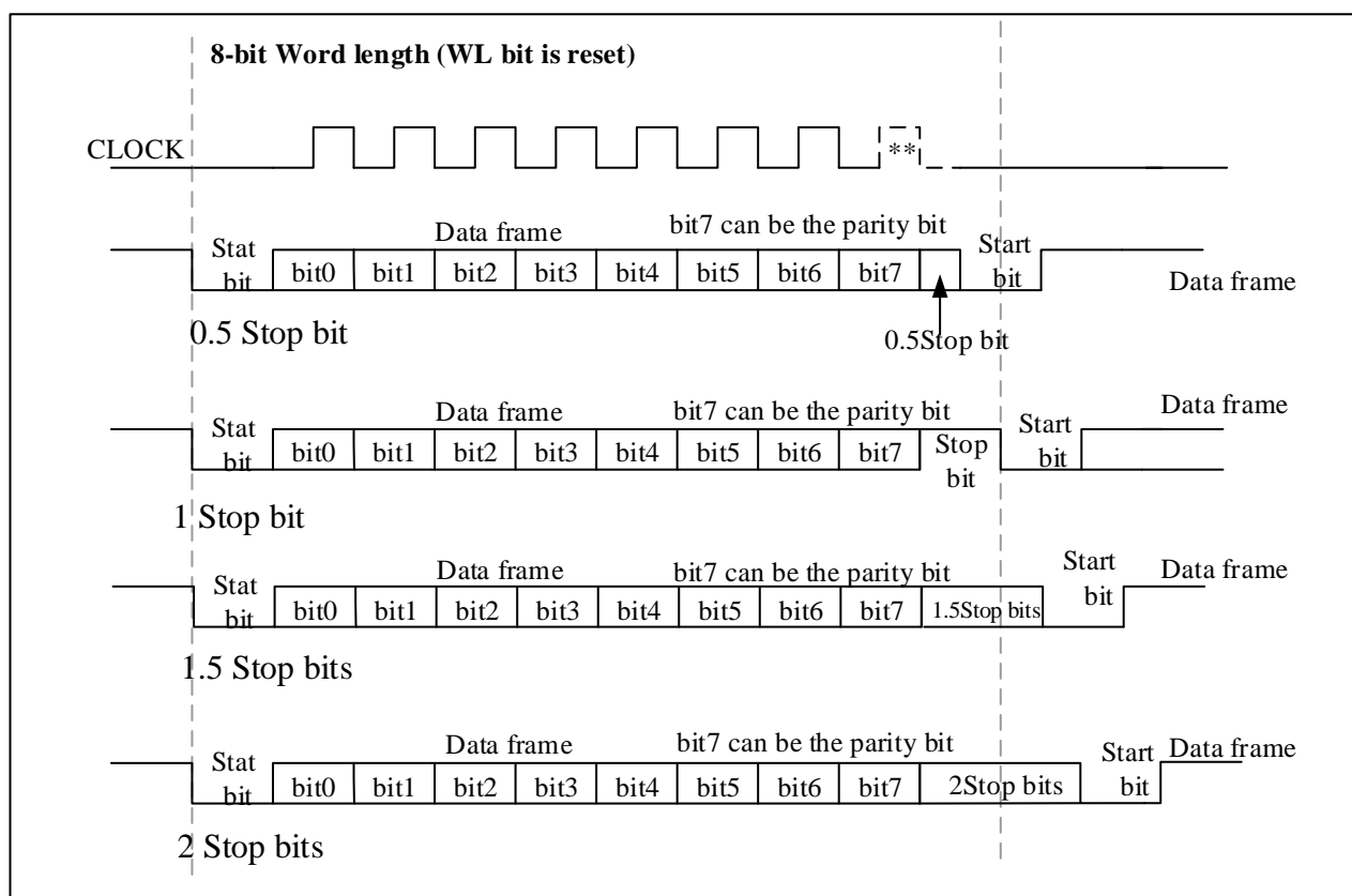
图 22-4 停止位配置
