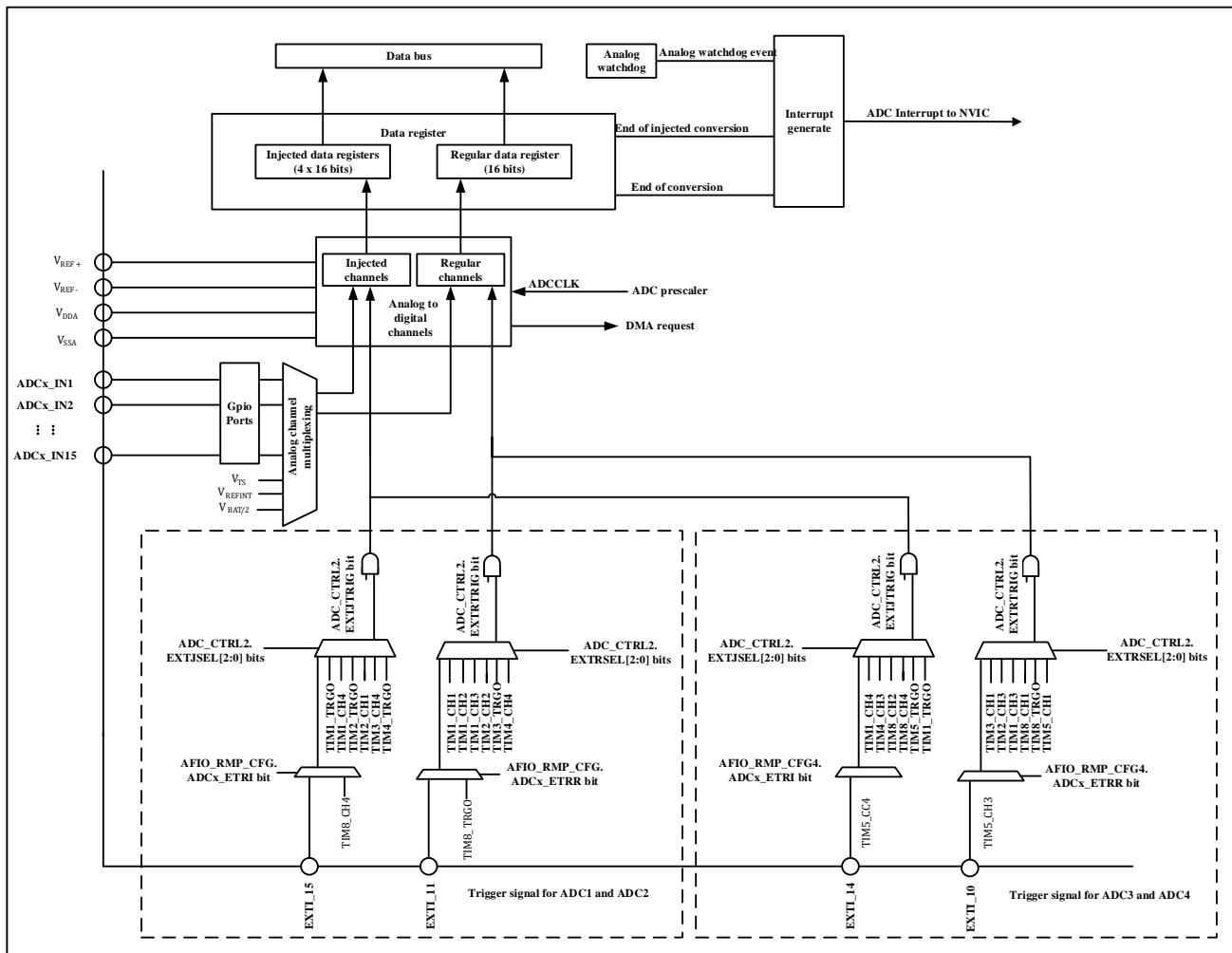
图 9-1 ADC 框图
