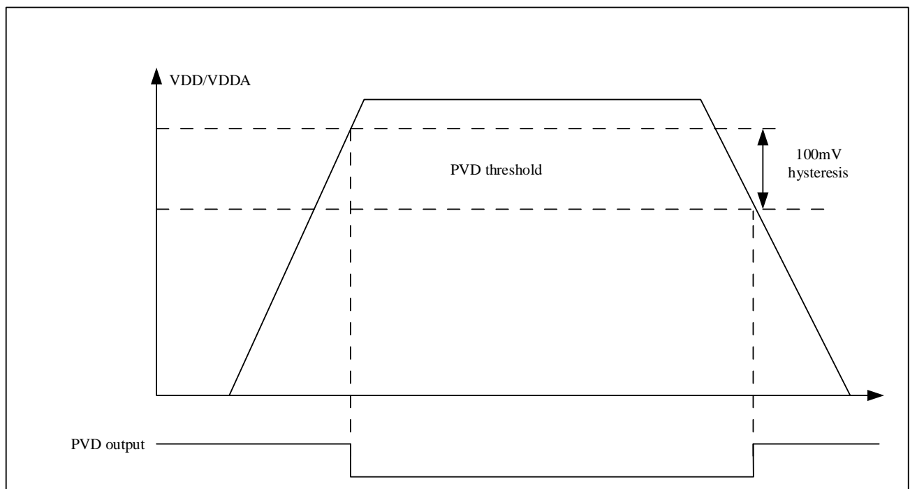
图 4-3 PVD 阈值波形图
