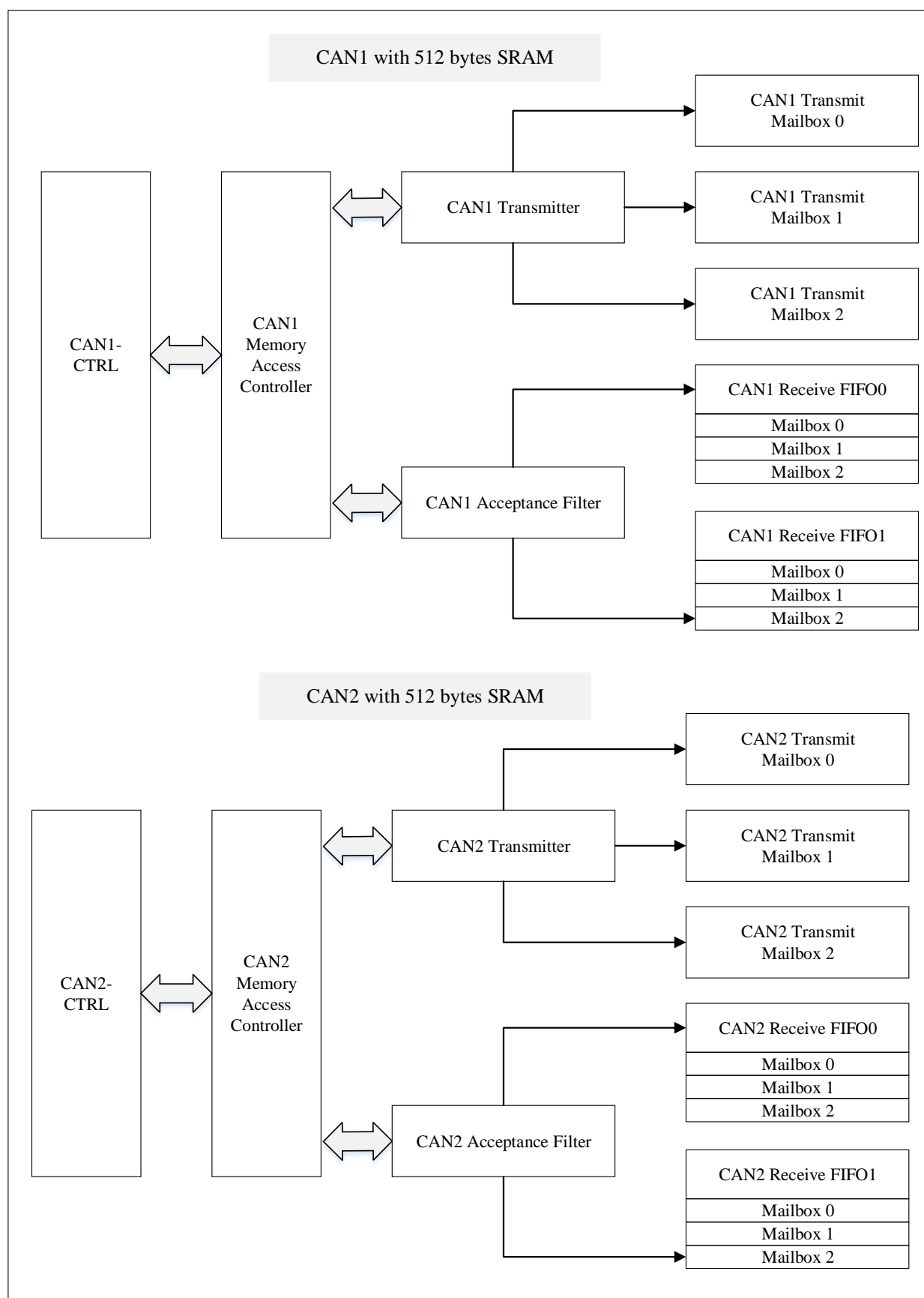
图 19-3 双 CAN 框图
