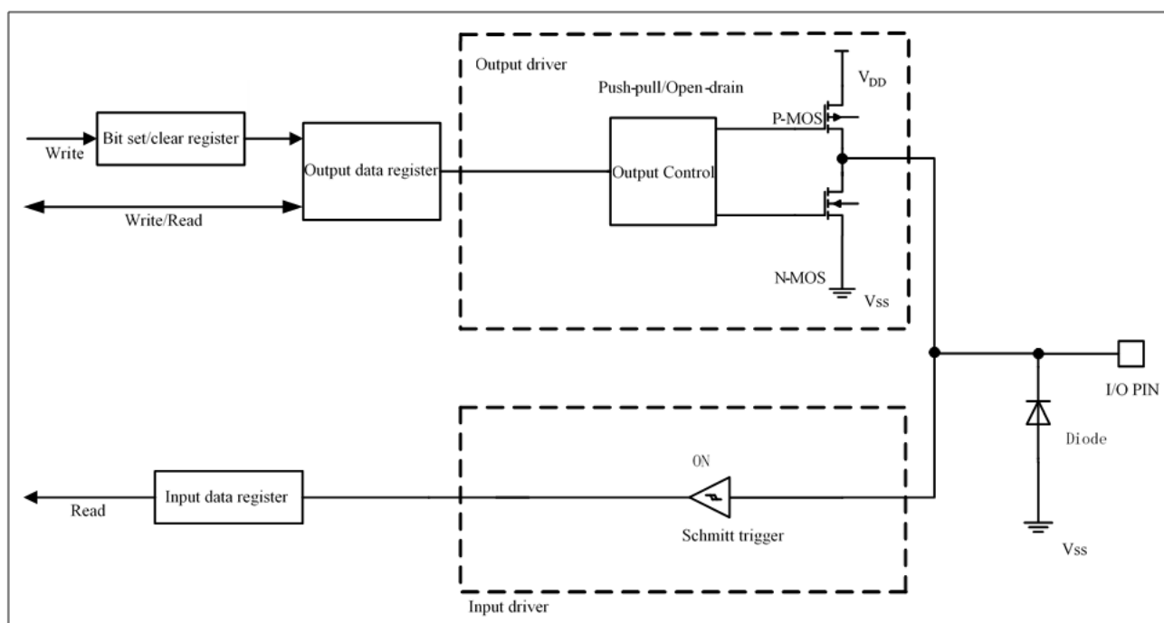
图 7-3 输出模式配置
