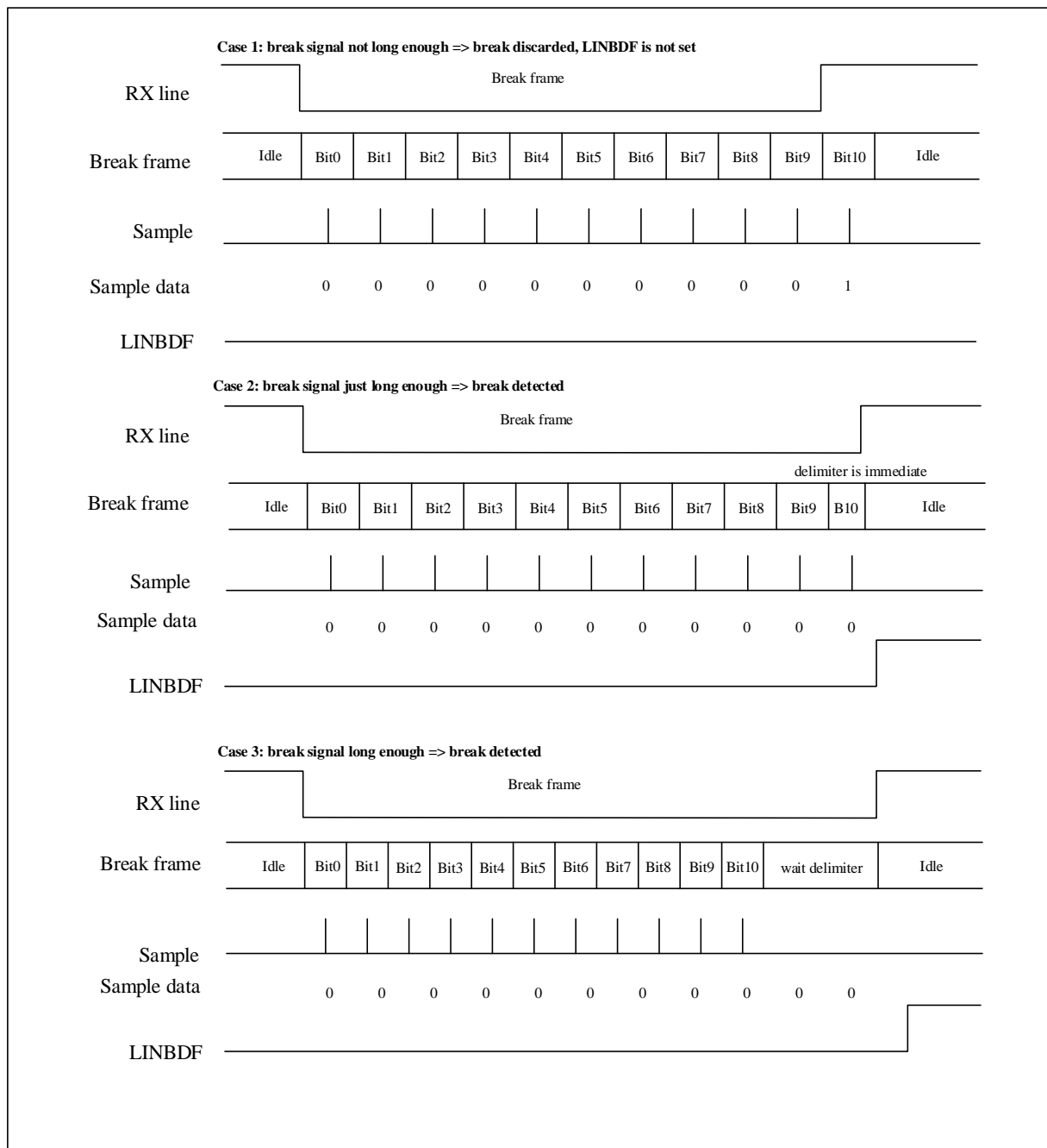
图 22-21 LIN 模式下的断开检测（11 位断开帧长度-设置了 LINBDL 位）
