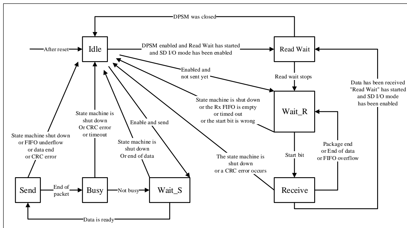
图 18-13 数据通道状态机（DPSM）
