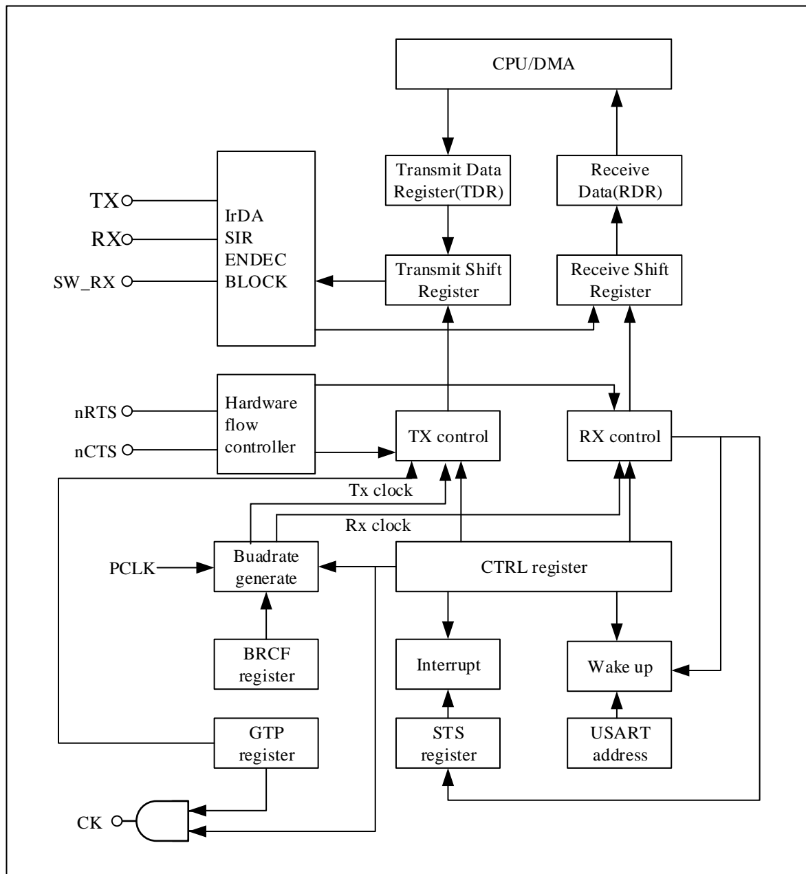
图 22-1 USART 框图
