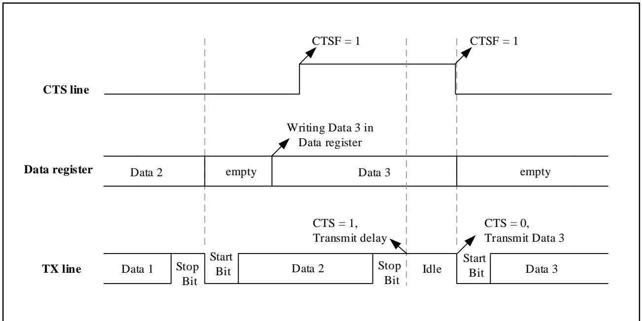
图 22-12 CTS 流控制
