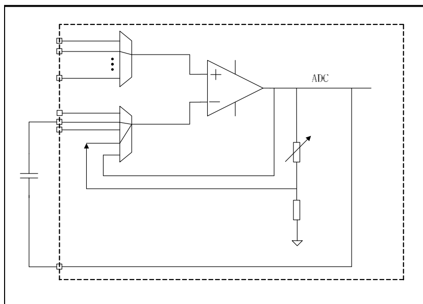
图 25-8 带滤波内部增益模式
