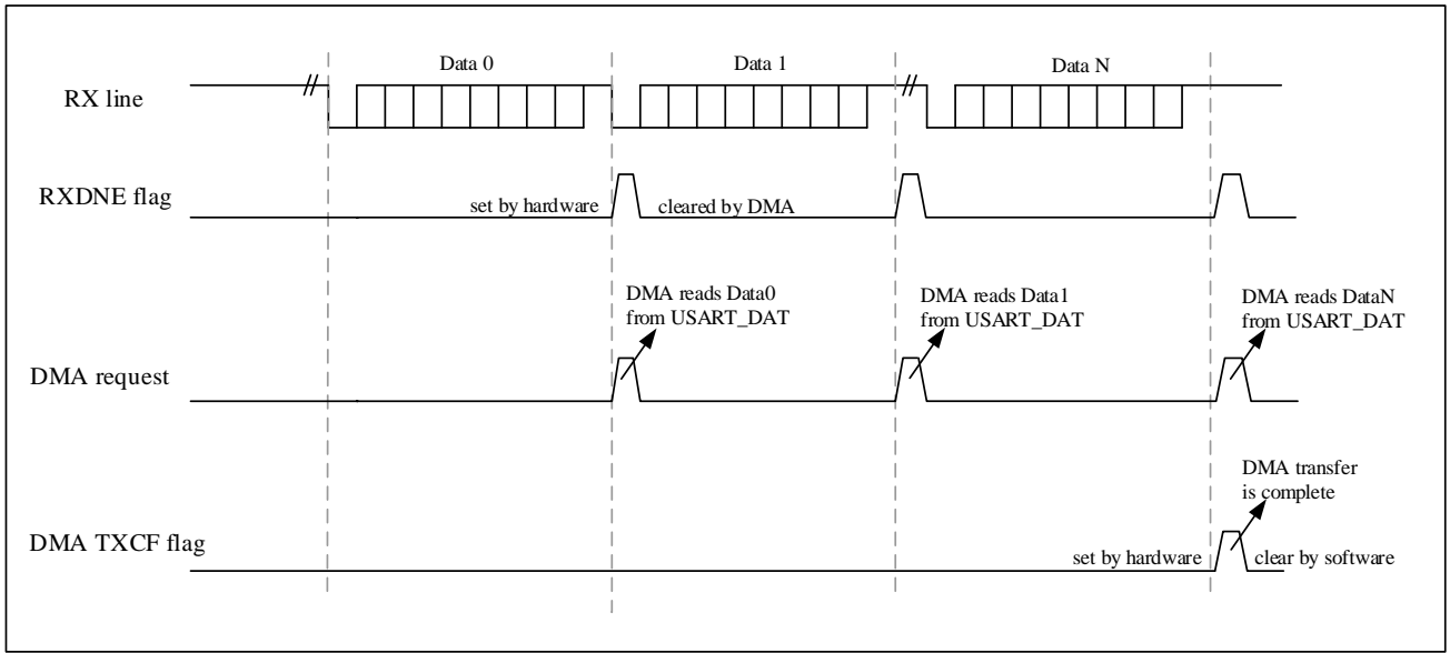
图 22-9 DMA 接收
