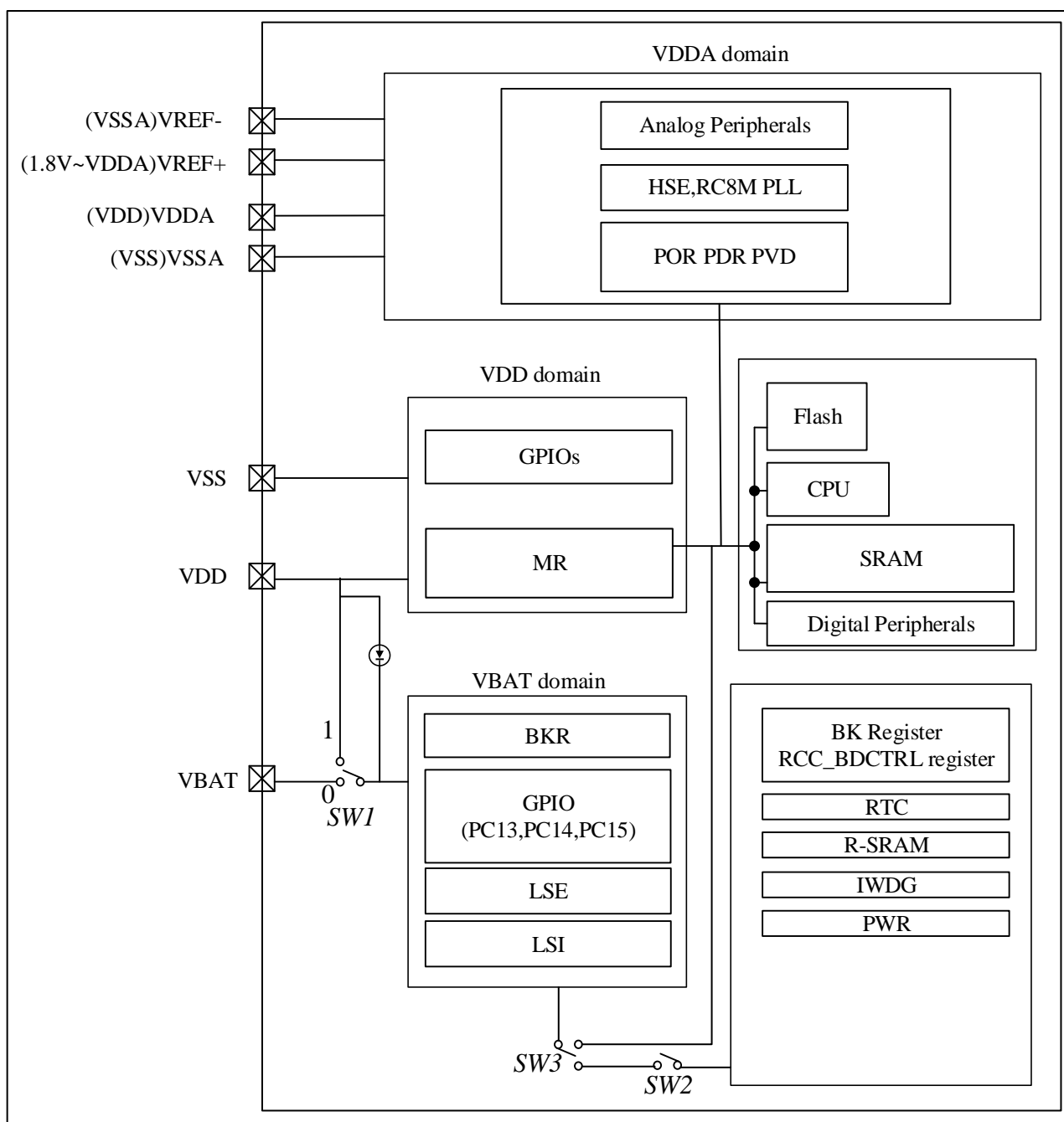
图 4-1 电源框图
