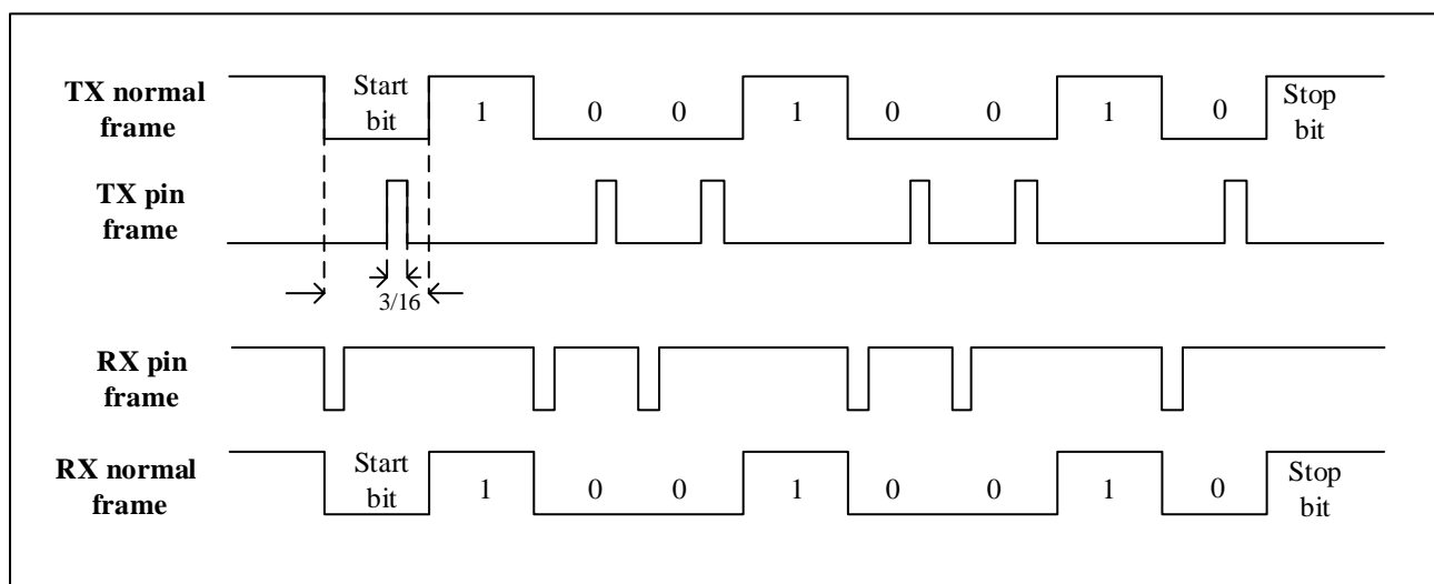
图 22-20 IrDA 数据调制 (3/16)-正常模式
