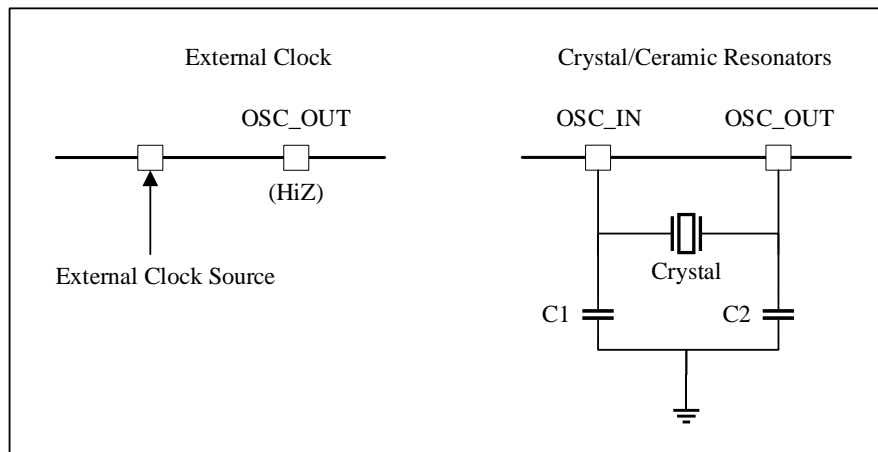
图 6-3 HSE/LSE 时钟源
