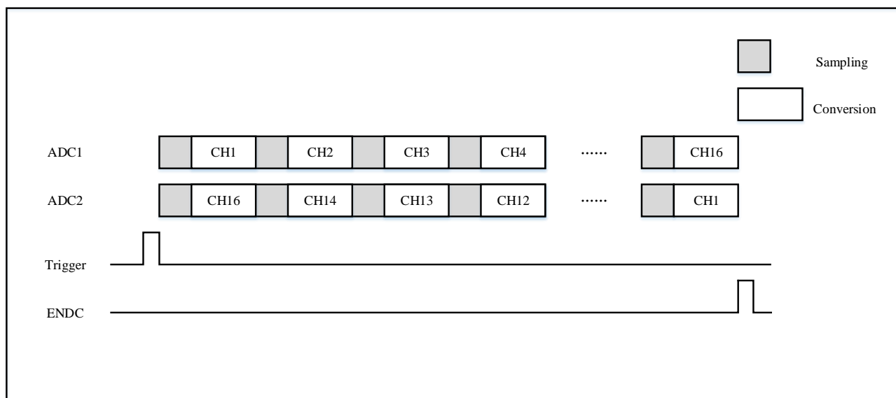
图 9-9 16 个通道的同步规则模式转换示意图
