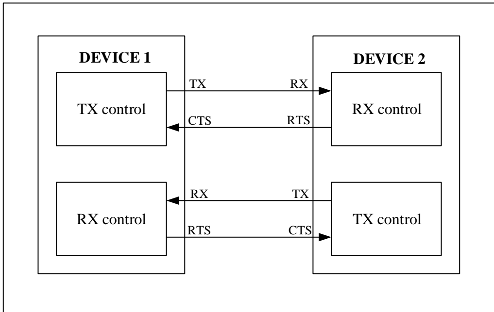
图 22-10 两个 USART 间的硬件流控制
