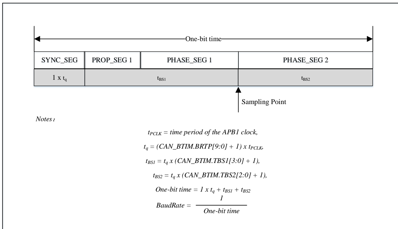
图 19-11 位时序
