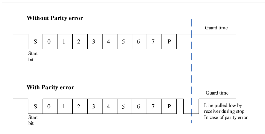
图 22-23 ISO7816-3 异步协议
