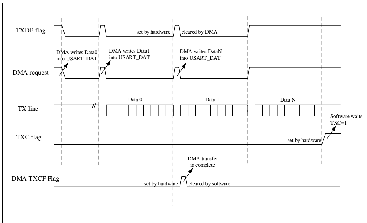
图 22-8 DMA 发送
