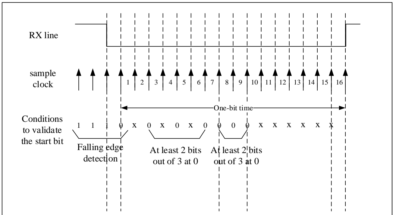
图 22-7 起始位检测
