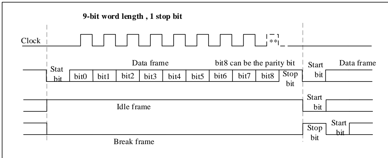
图 22-3 字长=9 设置
