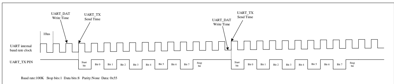
图 22-5 发送时差
