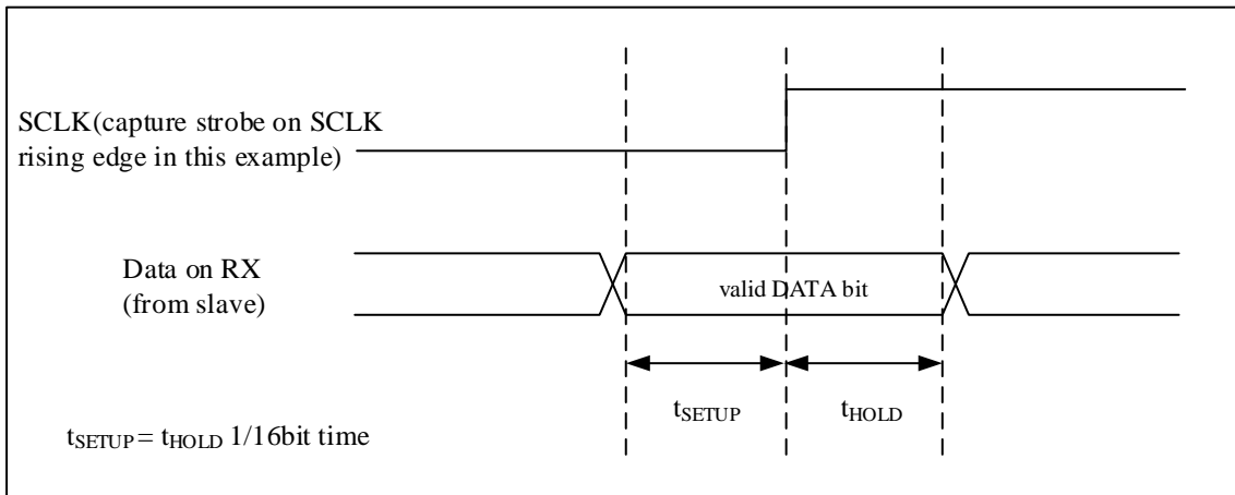
图 22-18 RX 数据采样/保持时间
