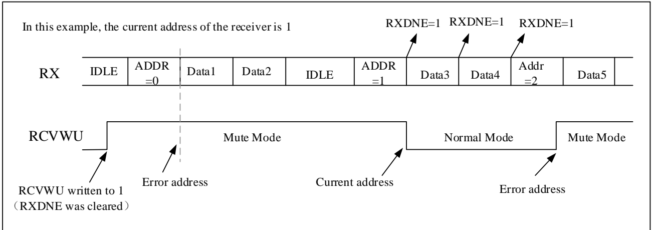
图 22-14 静默模式下的地址标识检测
