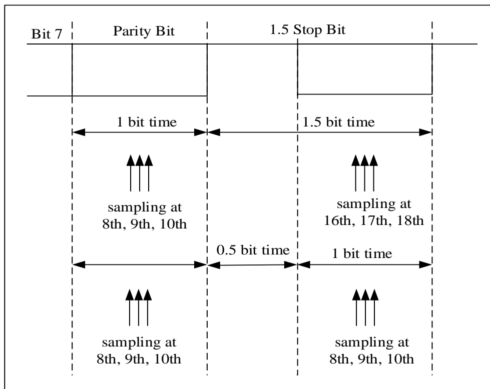
图 22-24 使用 1.5 停止位检测奇偶检验错误
