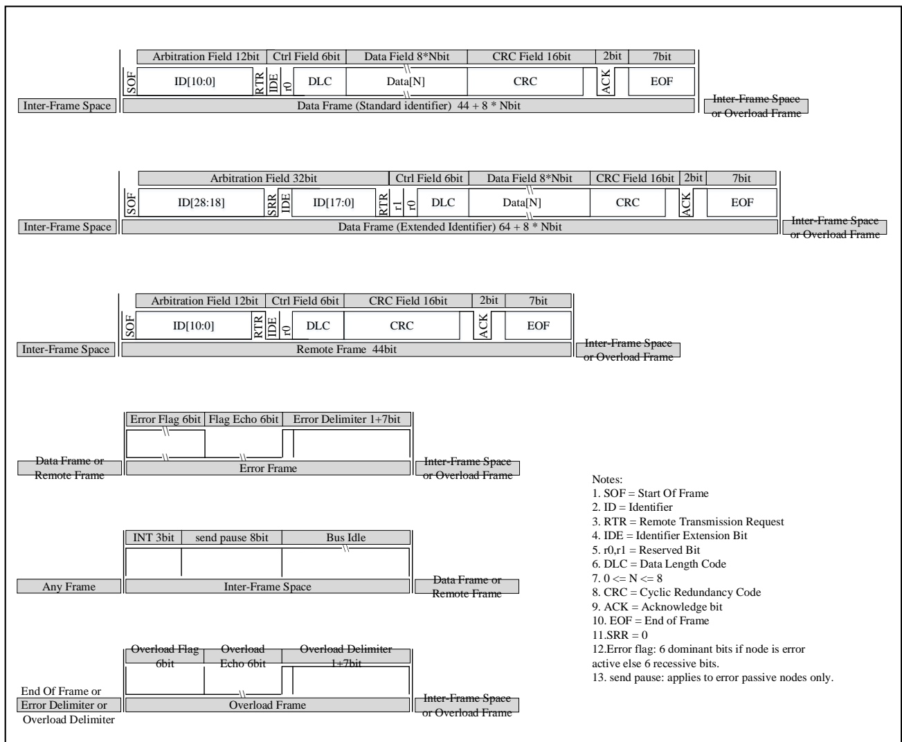
图 19-12 各类帧格式
