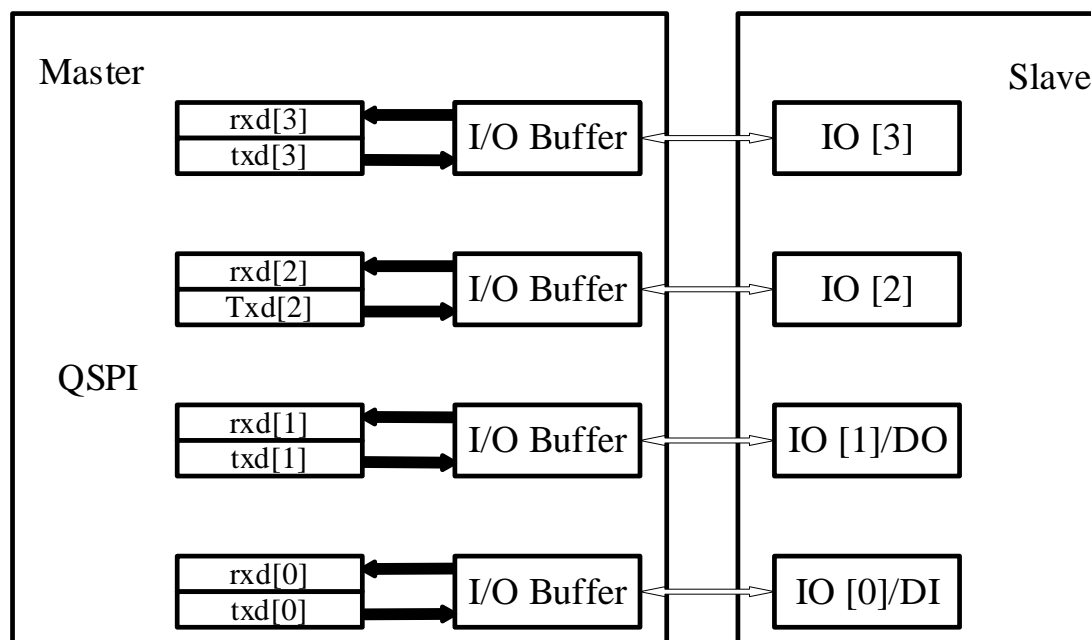
图 23-1 QSPI 功能框图
