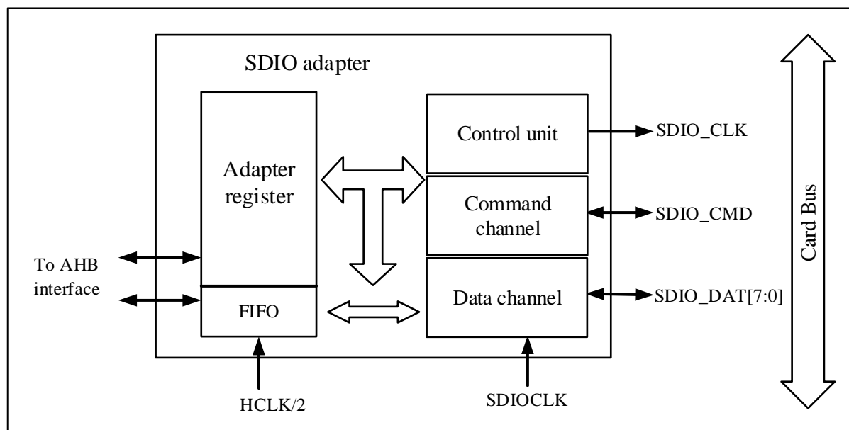
图 18-7 SDIO 适配器
