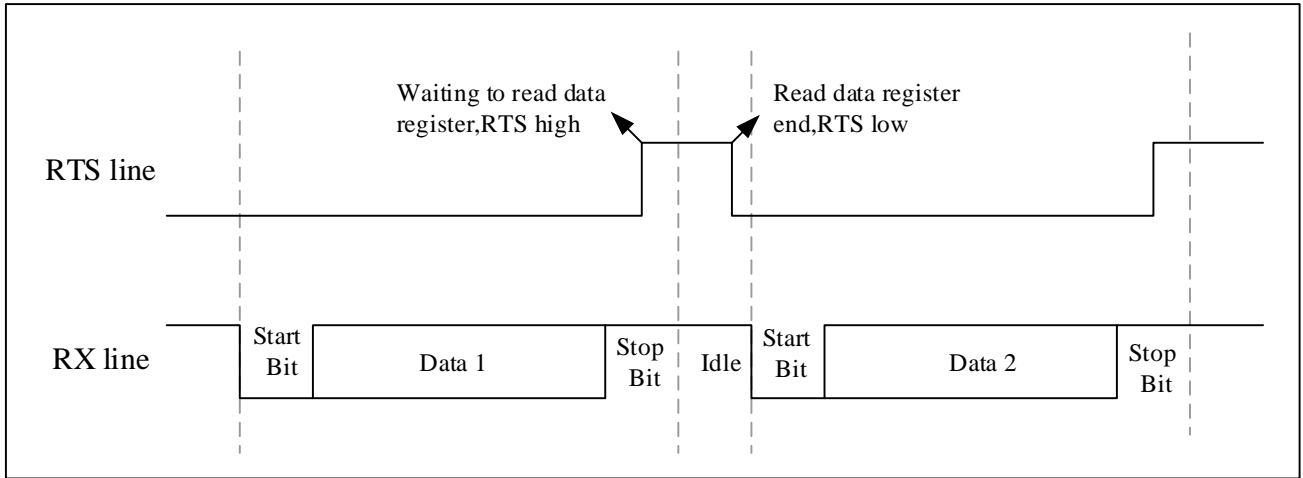
图 22-11 RTS 流控制
