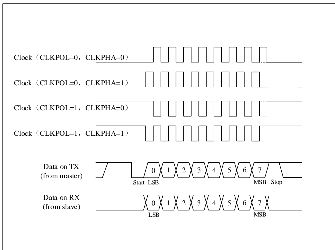
图 22-16 USART 数据时钟时序示例 (WL=0)
