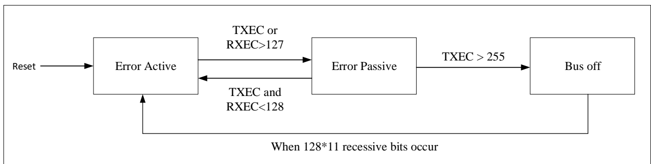
图 19-14 CAN 错误状态框图
