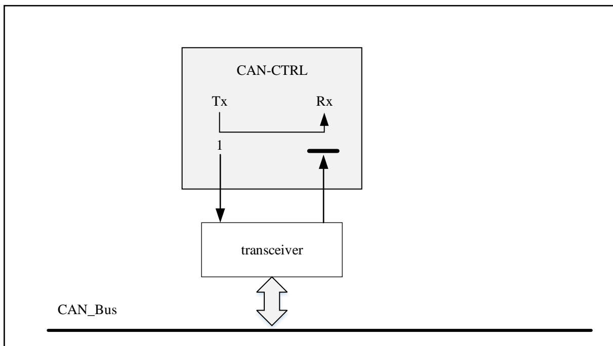
图 19-6 回环静默模式
