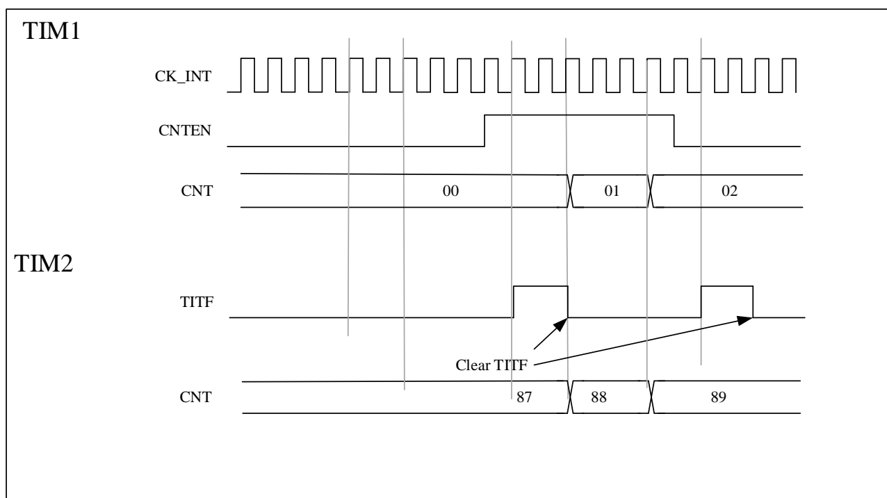
图 12-24 定时器 2 由定时器 1 的使能门控
