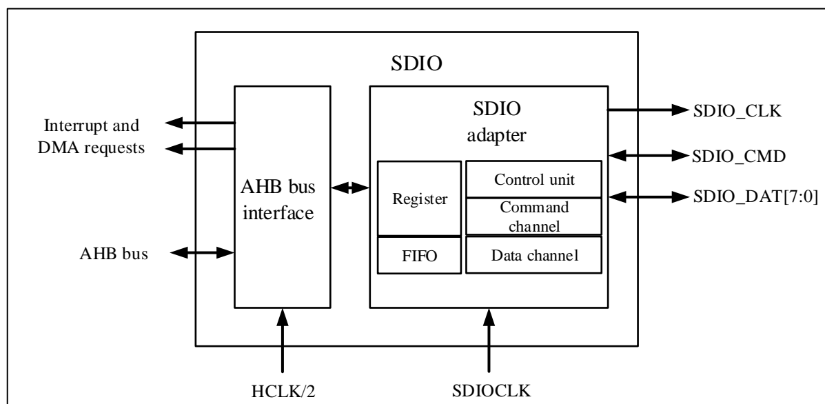
图 18-6 SDIO 框图
