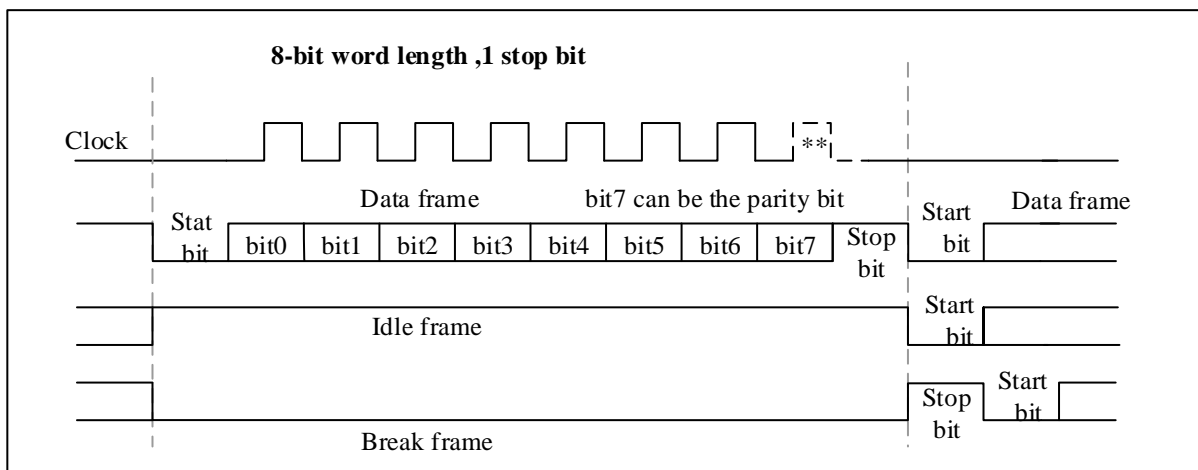
图 22-2 字长=8 设置
