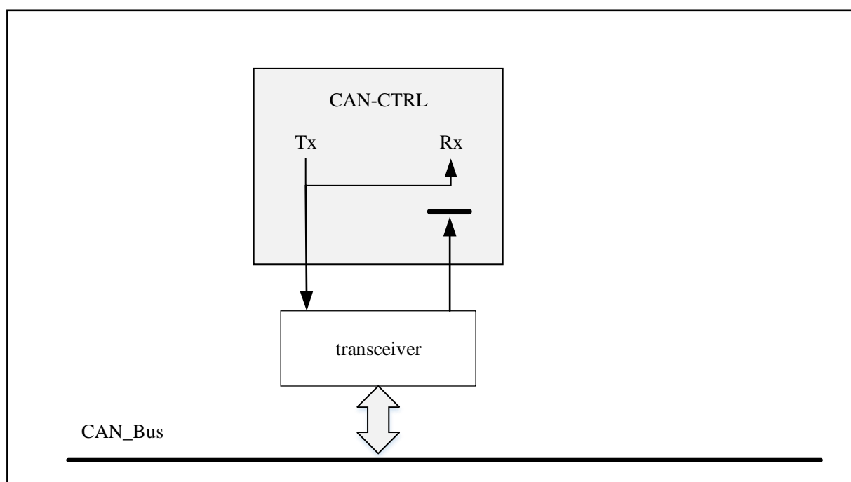
图 19-4 回环模式
