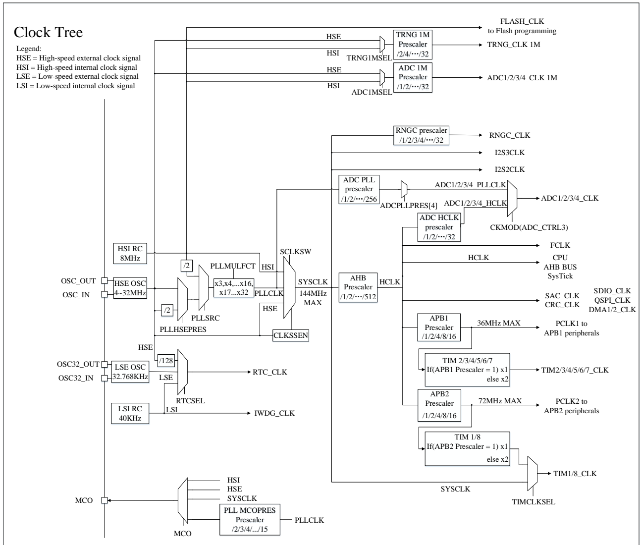
图 6-2 时钟树
