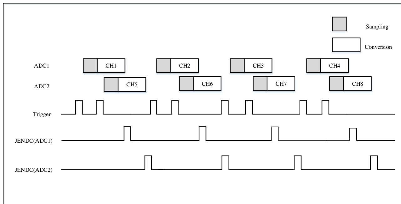
图 9-14 交替触发：在间断模式下注入通道组
