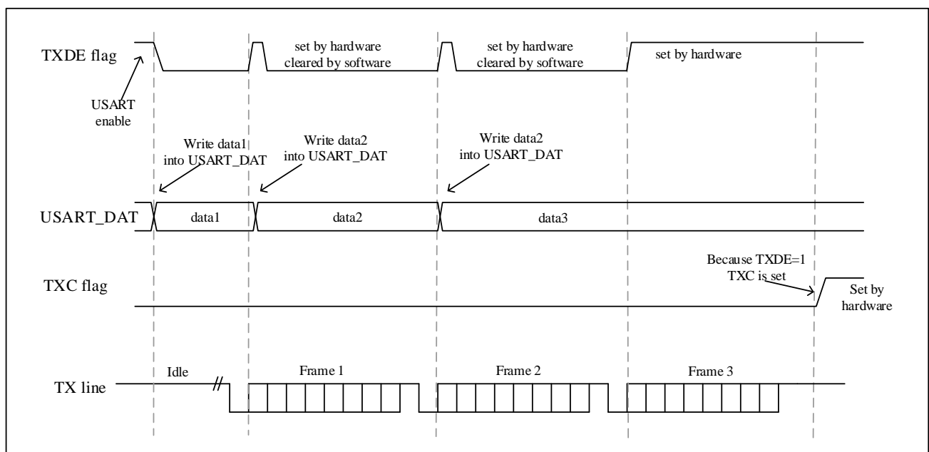
图 22-6 发送时 TXC/TXDE 的变化情况
