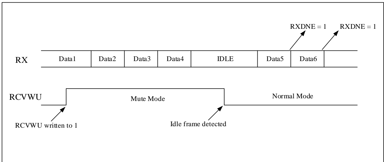
图 22-13 静默模式下的空闲总线检测
