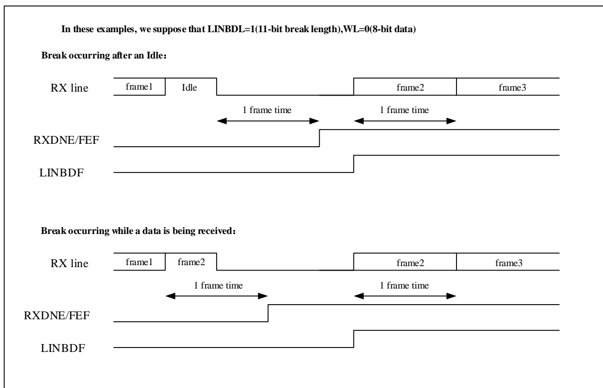
图 22-22 LIN 模式下的断开检测与帧错误的检测
