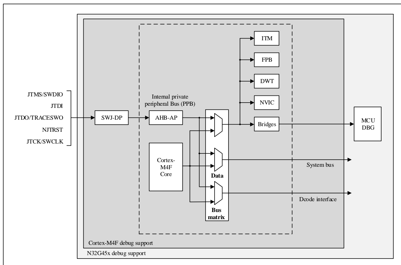
图 26-1 N32A455 级别和 Cortex™-M4F 级别的调试框图
