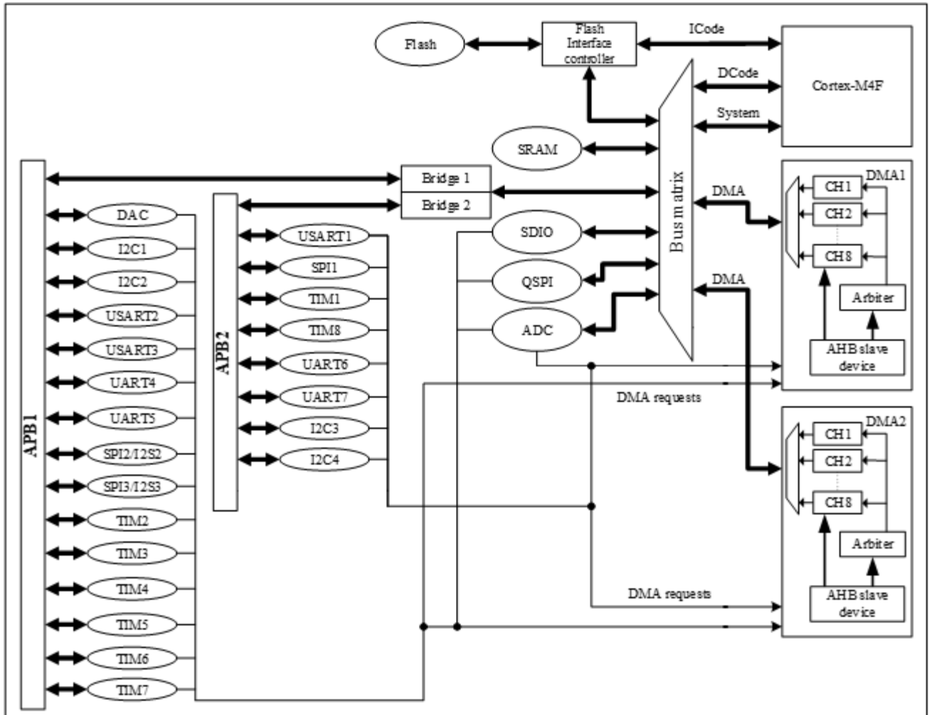
图 8-1 DMA 框图
