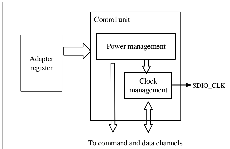
图 18-8 控制单元
