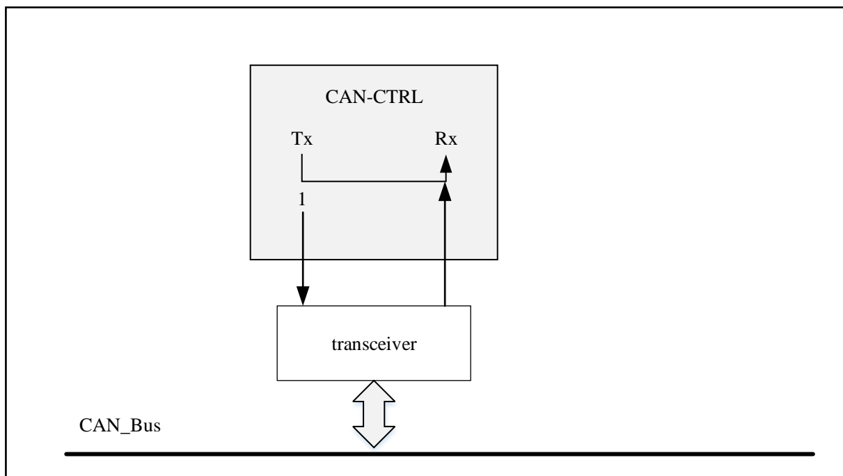
图 19-5 静默模式
