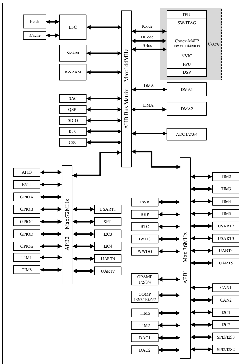
图 3-1 总线架构图
