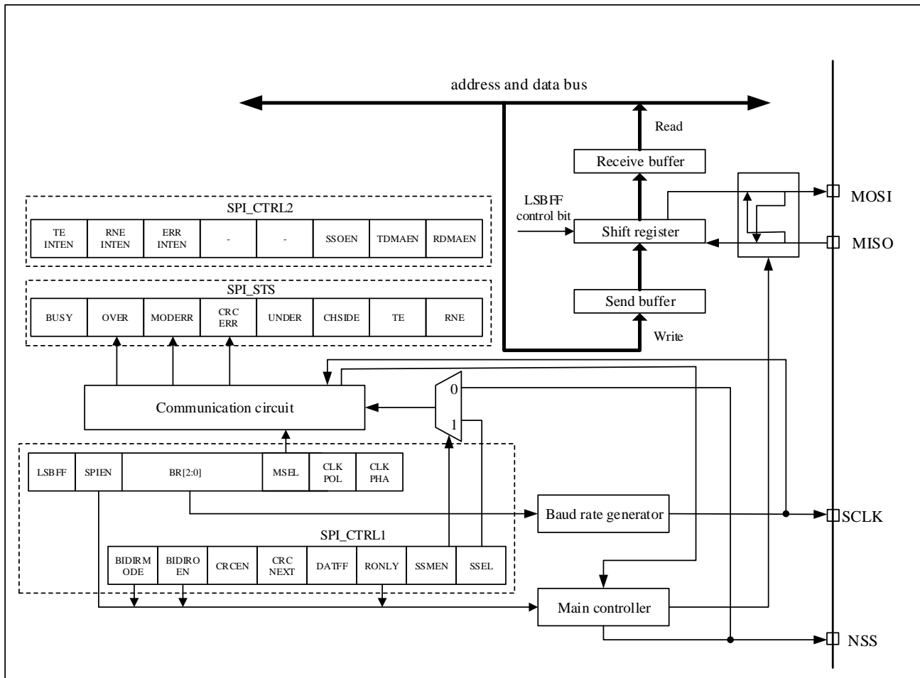
图 20-1 SPI 框图
