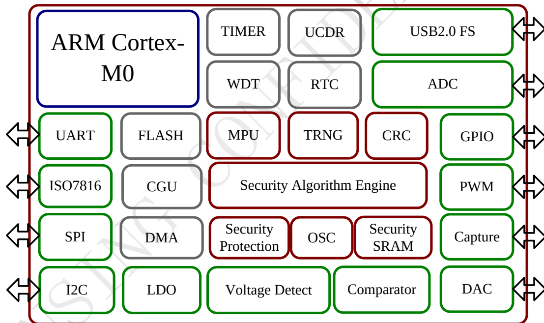
图 1-1 N32S032结构图
