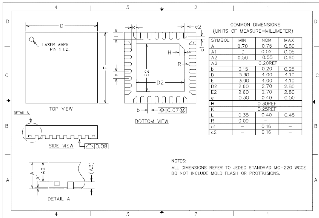
图 3-4 QFN32封装尺寸
