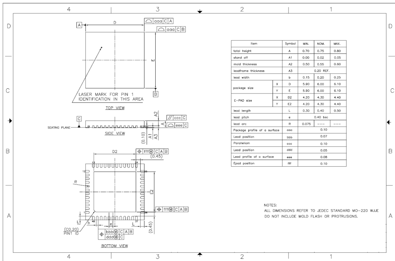
图 3-2 QFN48 封装尺寸
