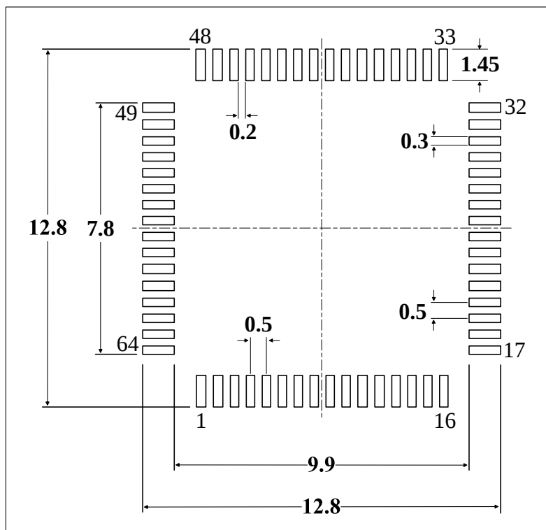
图 5-8 LQFP64 封装焊盘建议 (1)
