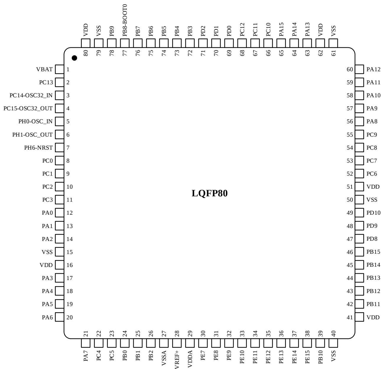
图 3-5 LQFP80 引脚分布
