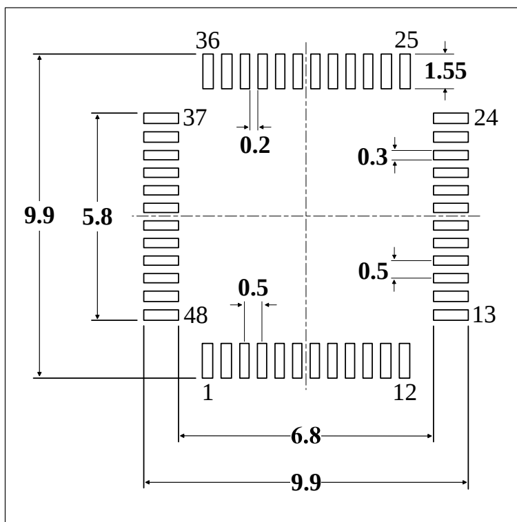
图 5-6 LQFP48 封装焊盘建议 (1)
