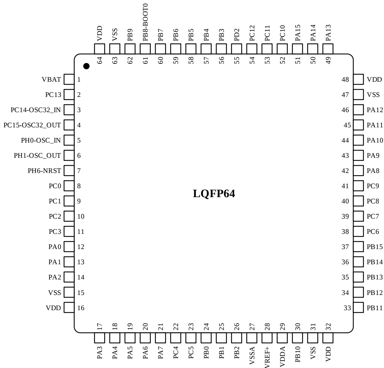
图 3-4 LQFP64 引脚分布
