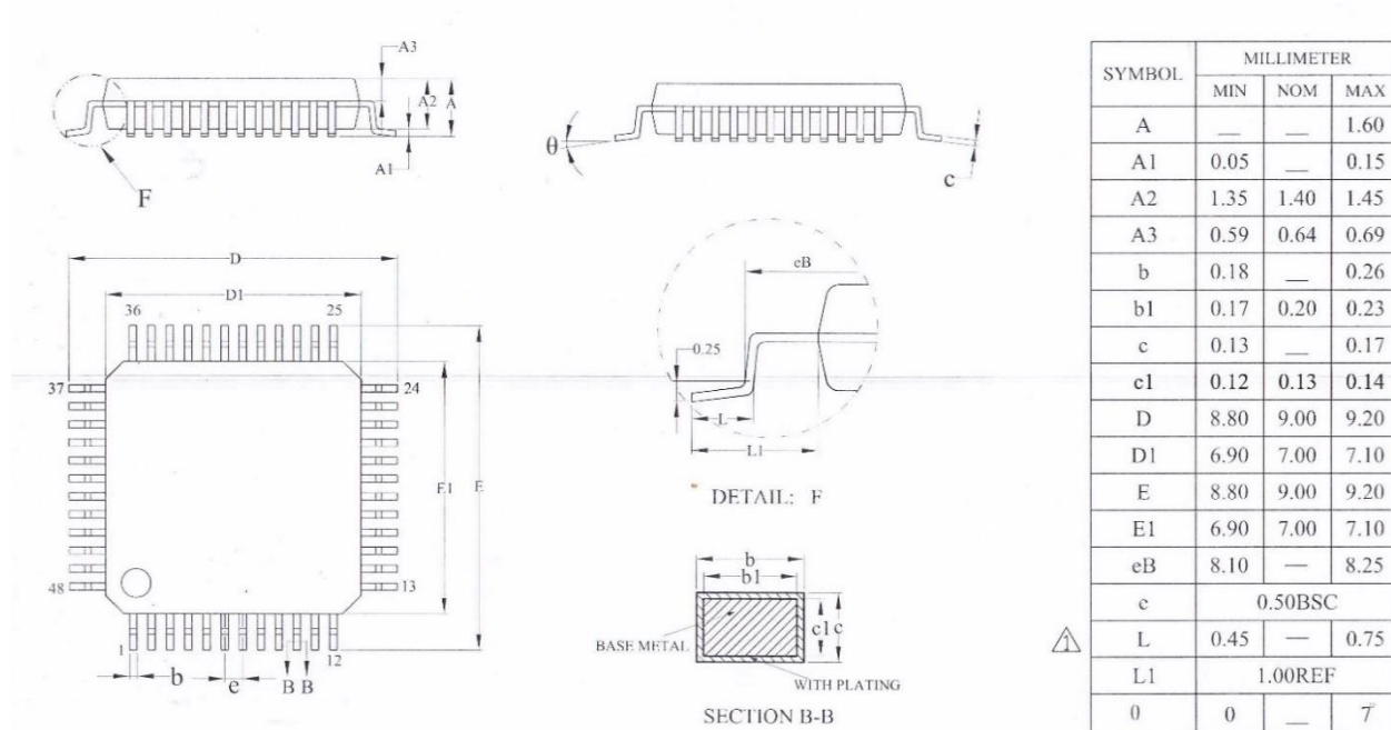
图 5-5 LQFP48 封装尺寸
