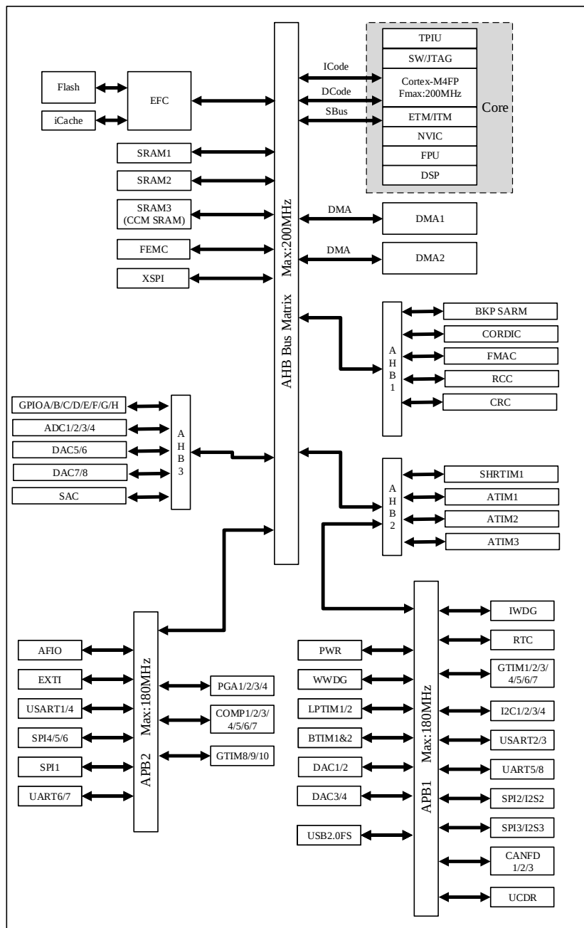
图 1-1 N32H474 系列框图
