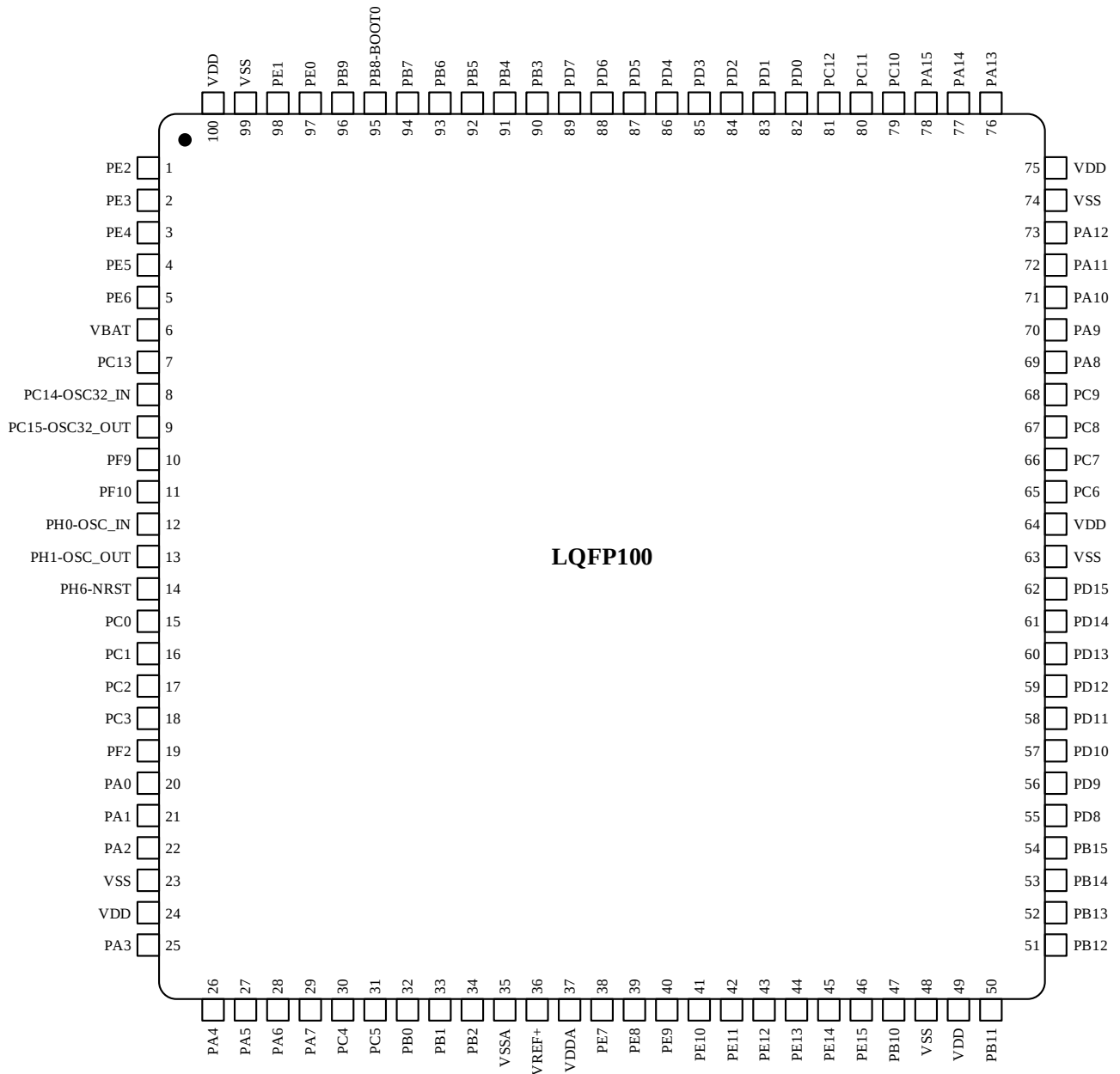
图 3-6 LQFP100 引脚分布
