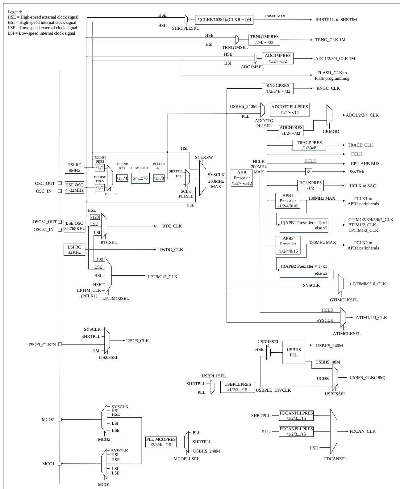
图 2-2 时钟树
