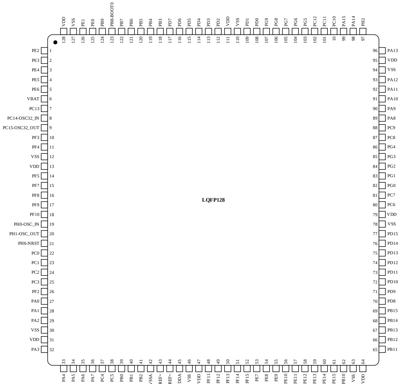
图 3-7 LQFP128 引脚分布
