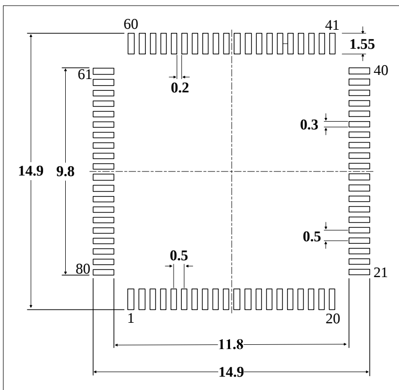
图 5-10 LQFP80 封装焊盘建议 (1)
