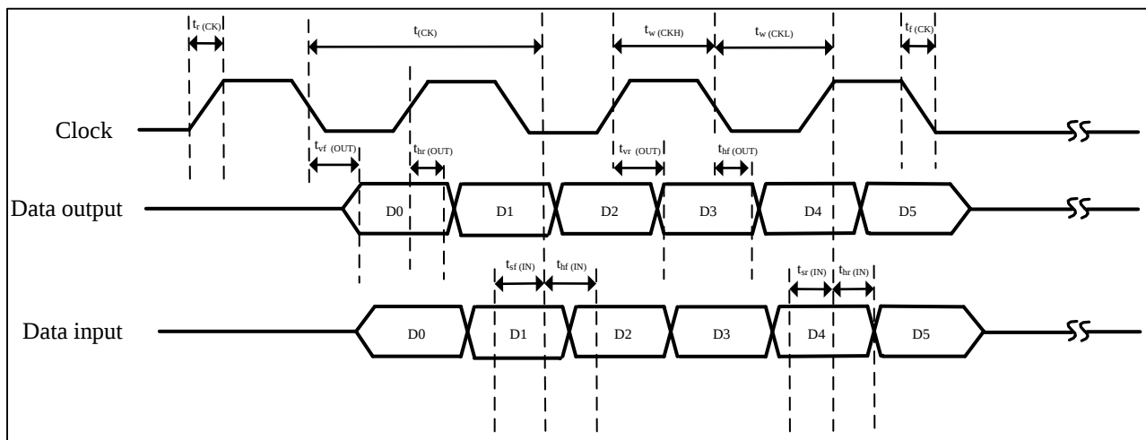
图 4-19 xSPI在DDR模式下的时序
