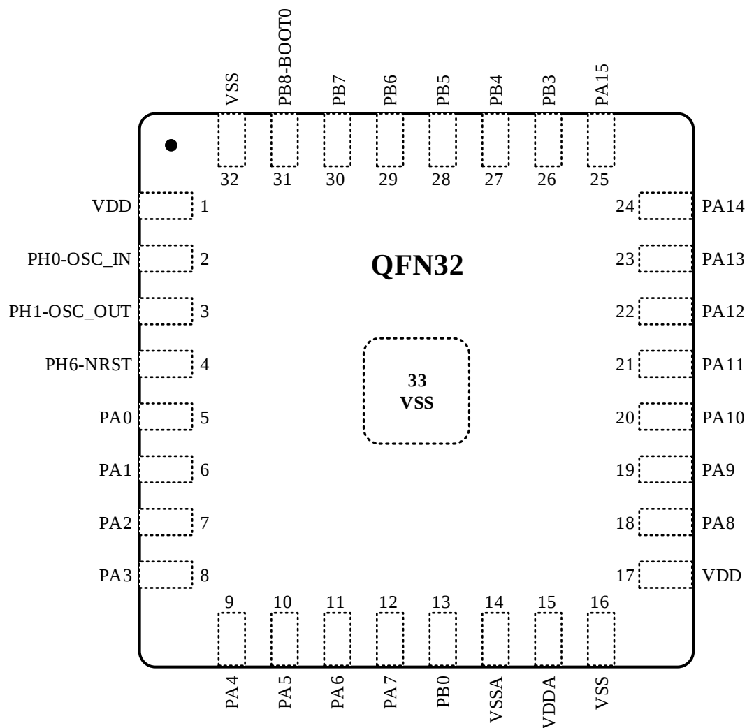
图 3-1 QFN32 引脚分布
