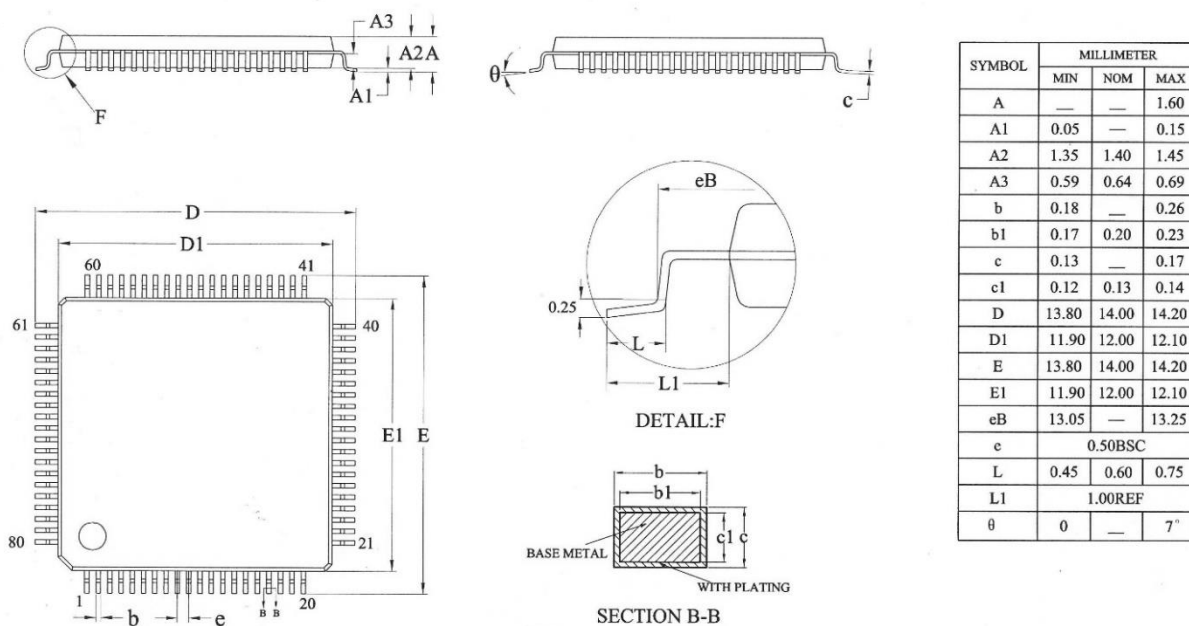
图 5-9 LQFP80 封装尺寸
