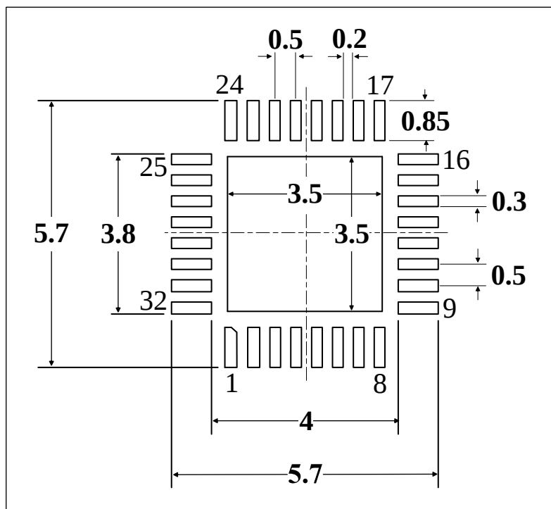
图 5-2 QFN32 封装焊盘建议 (1)
