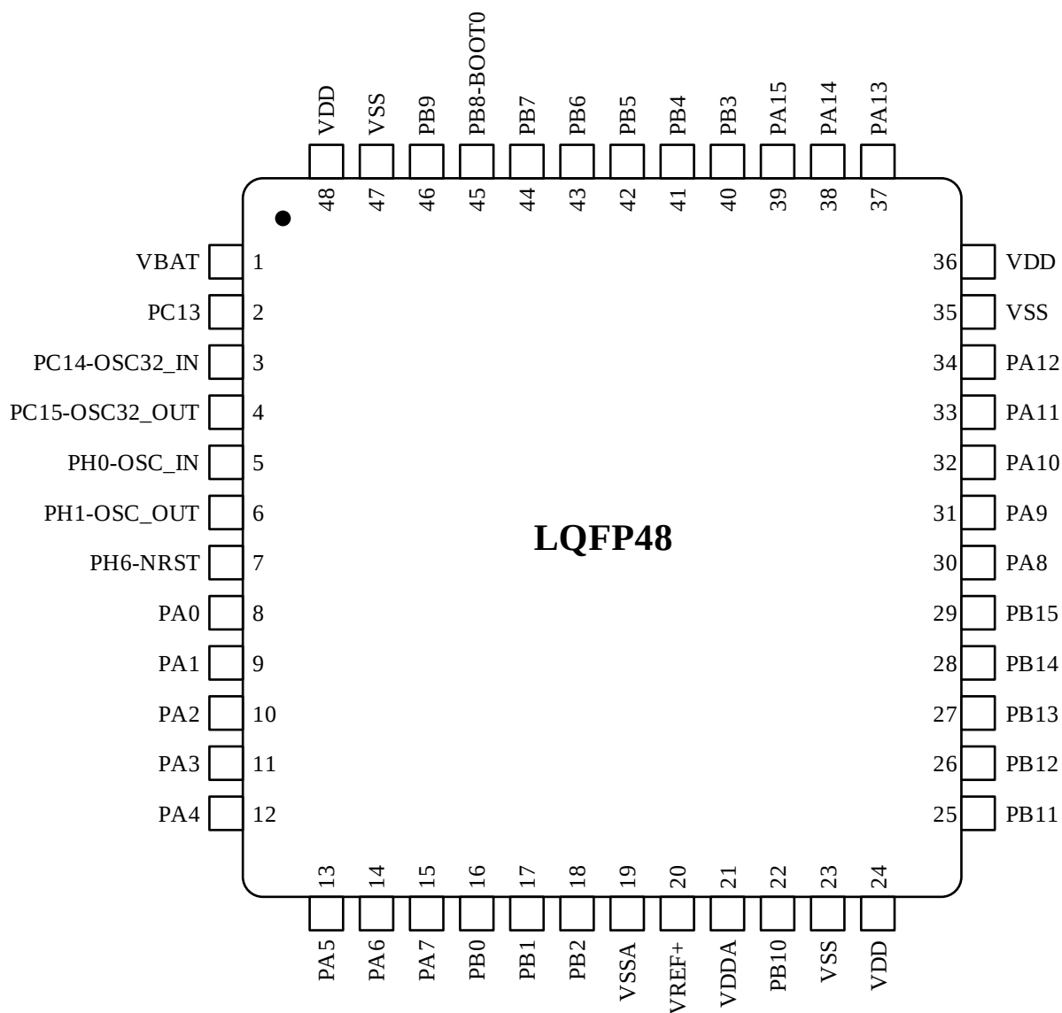
图 3-3 LQFP48 引脚分布
