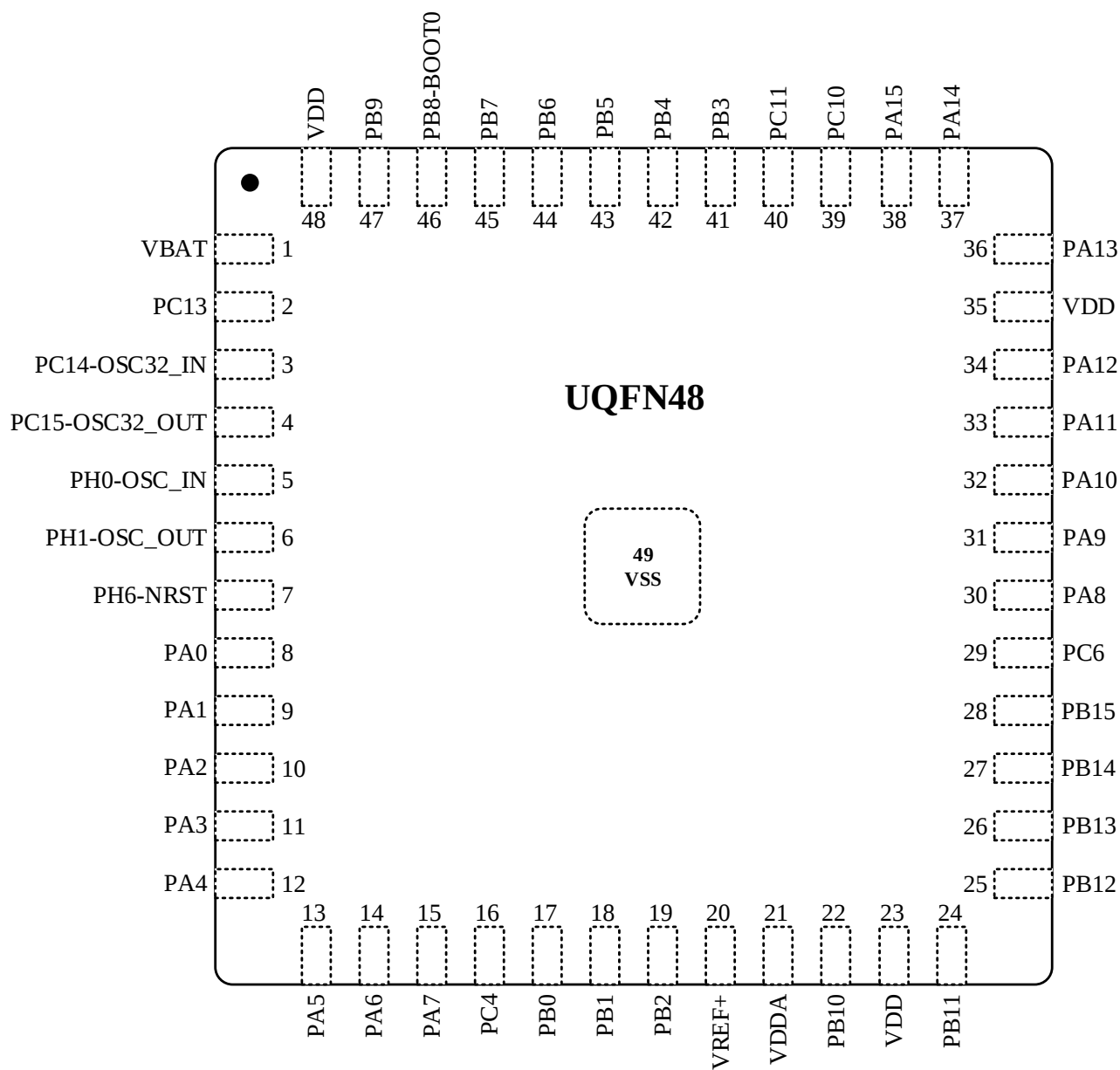
图 3-2 UQFN48 引脚分布
