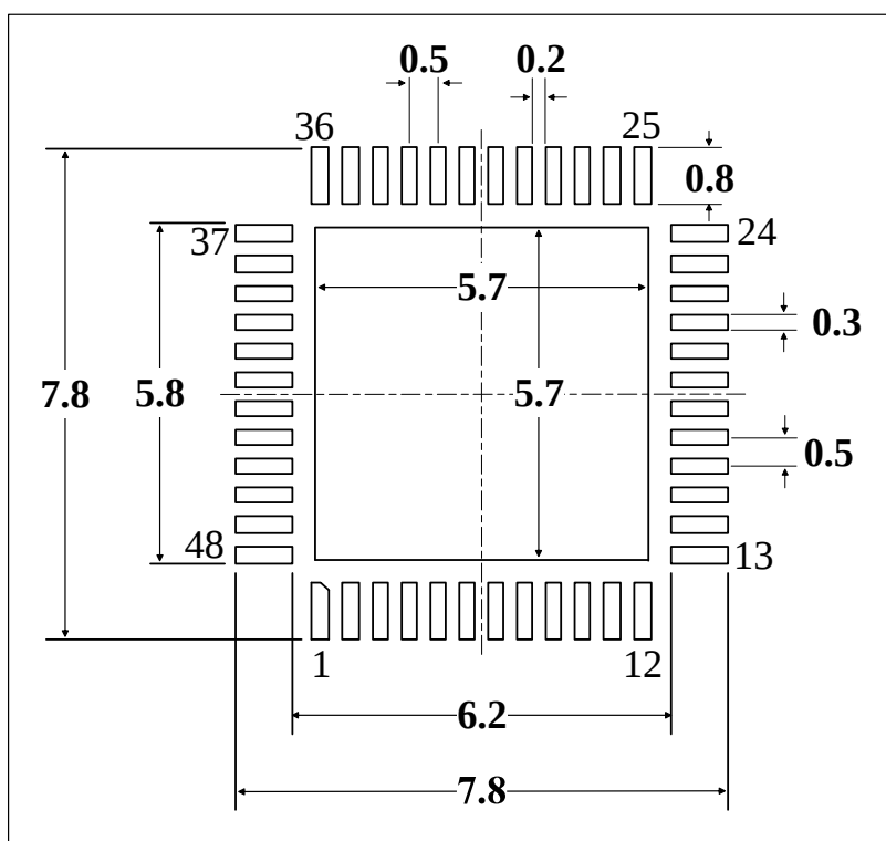
图 5-4 UQFN48 封装焊盘建议 (1)
