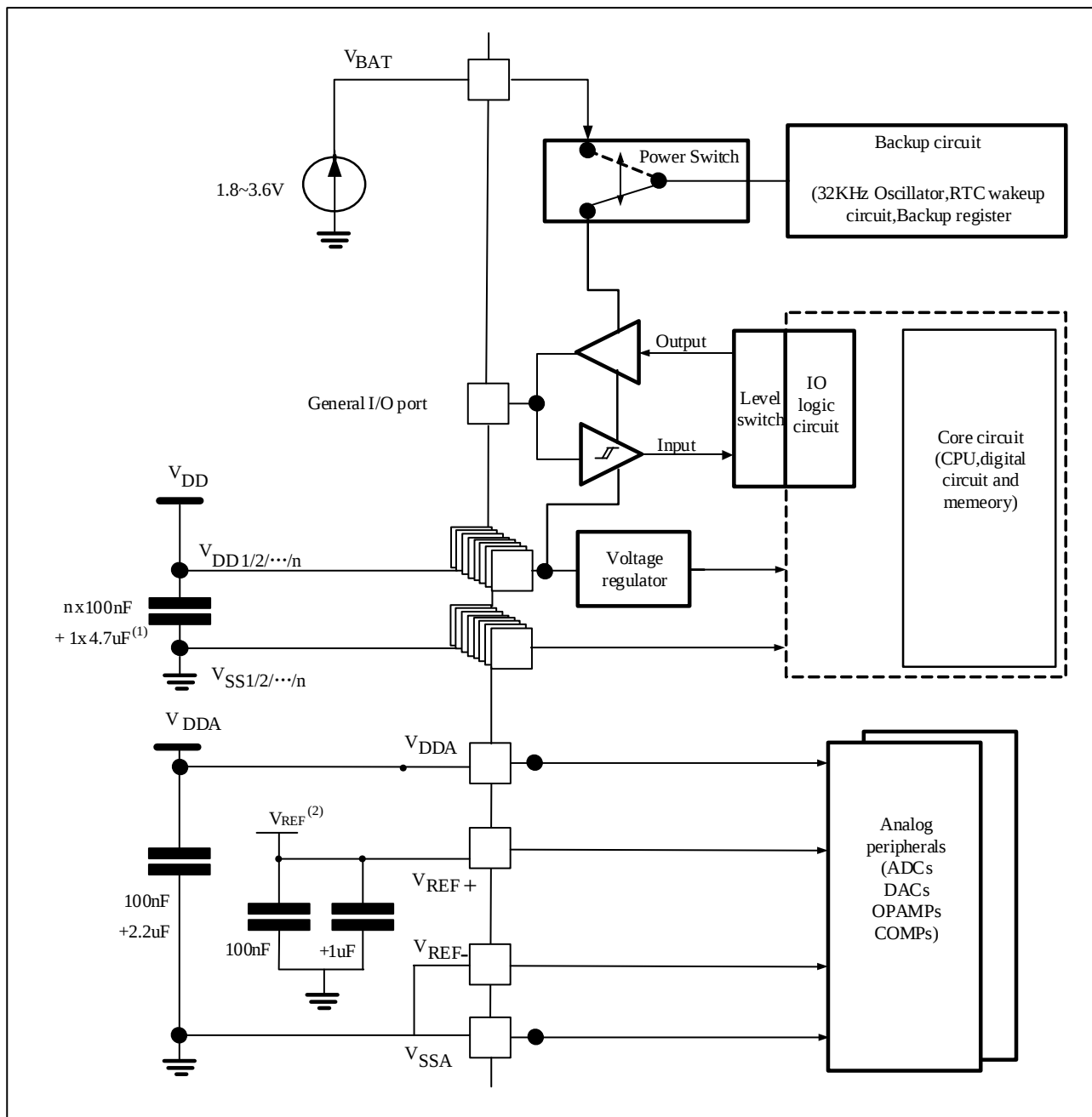
图 4-3 供电方案
