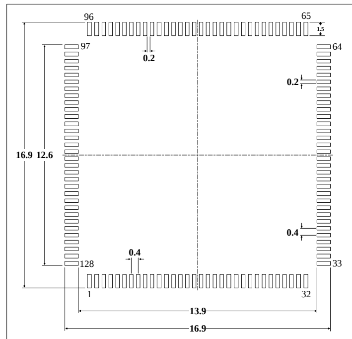
图 5-14 LQFP128 封装焊盘建议 (1)
