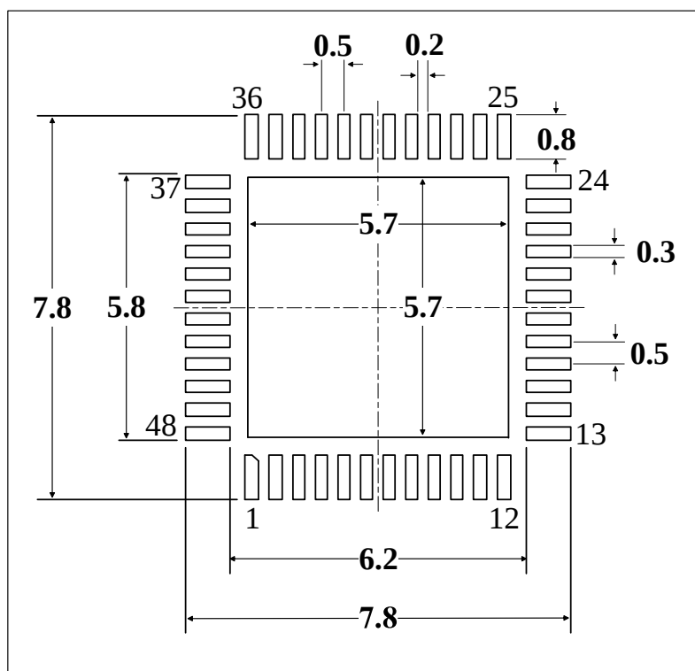
图 5-4 QFN48 封装焊盘建议 (1)
