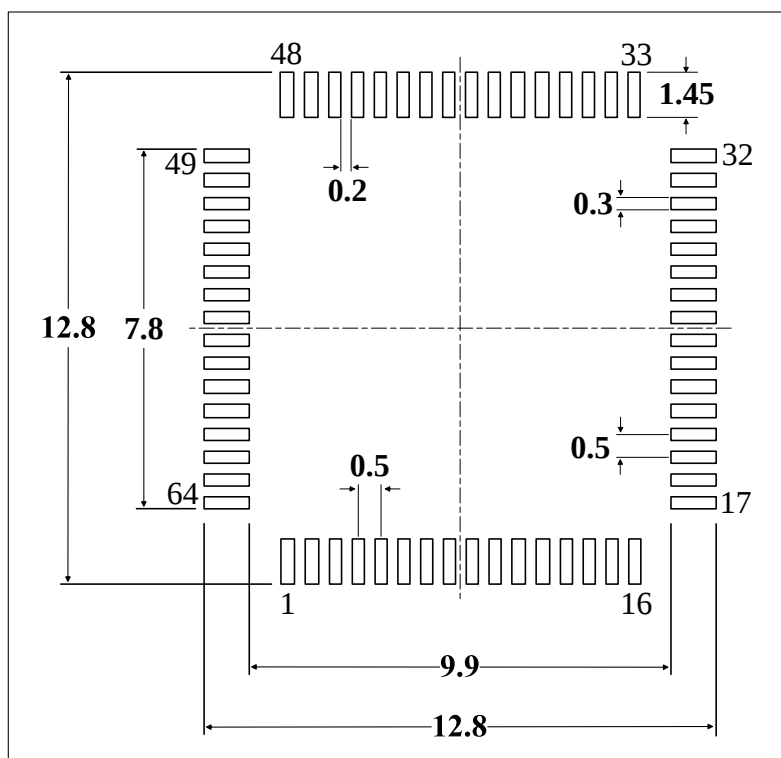
图 5-12 LQFP64 封装焊盘建议 (1)
