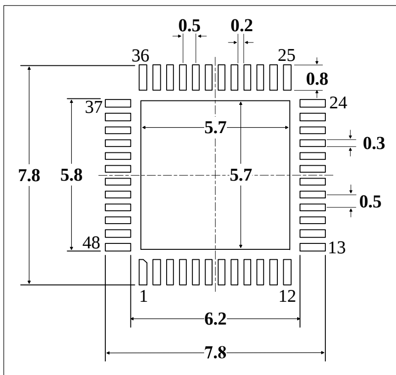
图 5-6 UQFN48/UQFN48-1 封装焊盘建议 (1)
