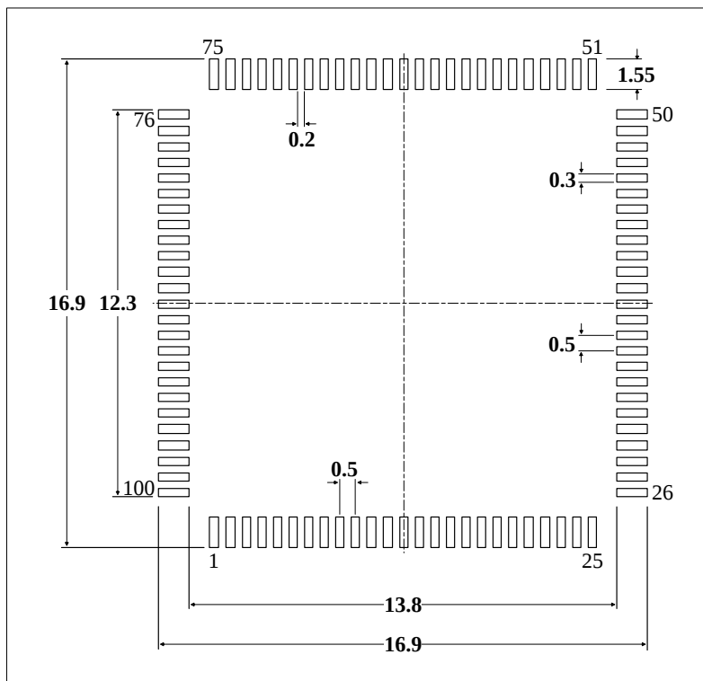
图 5-16 LQFP100 封装焊盘建议 (1)
