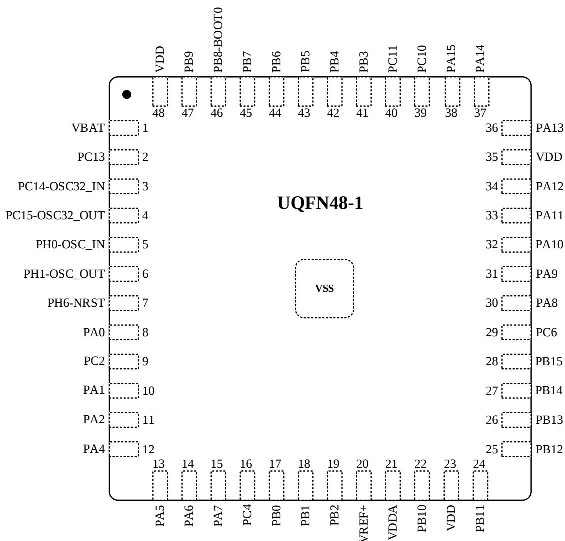
图 3-4 UQFN48-1 引脚分布
