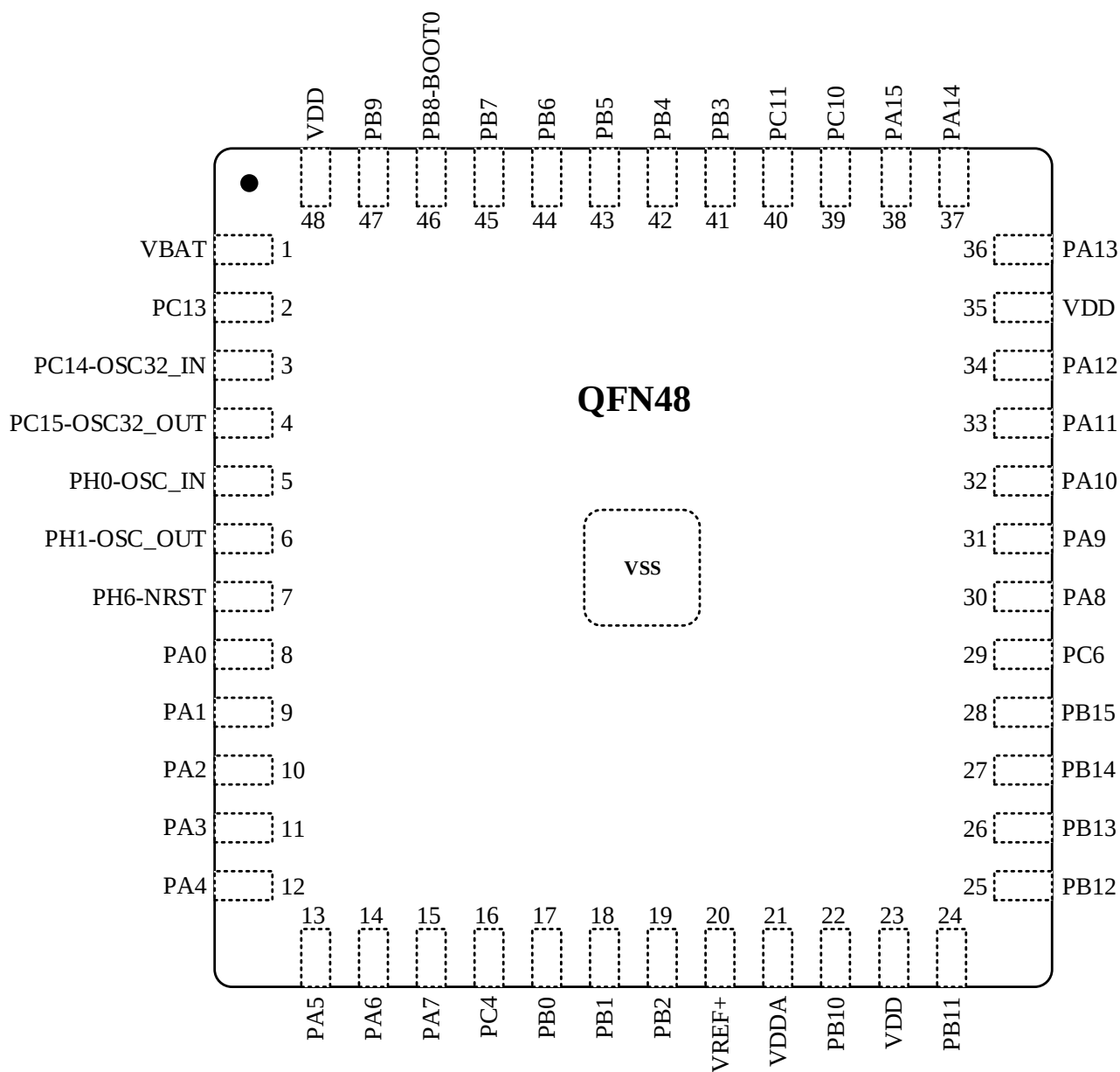
图 3-2 QFN48 引脚分布
