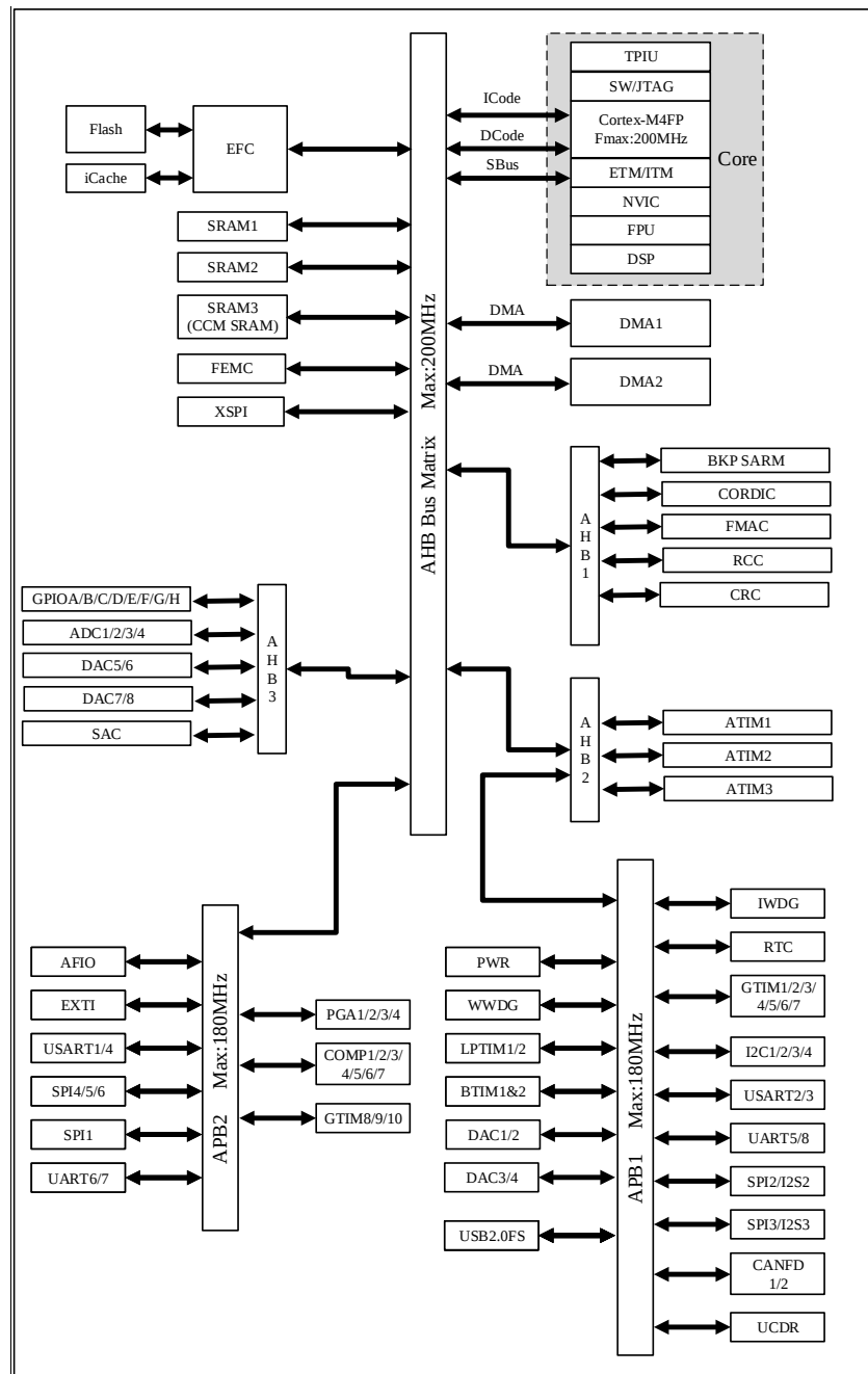
图 1-1 N32H473 系列框图
