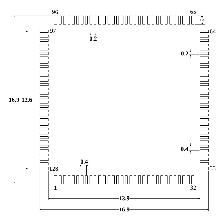
图 5-18 LQFP128 封装焊盘建议 (1)
