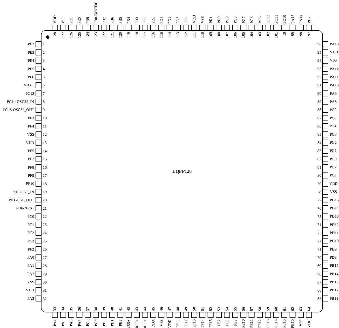
图 3-10 LQFP128 引脚分布
