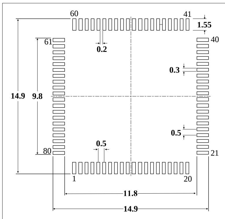
图 5-14 LQFP80 封装焊盘建议 (1)
