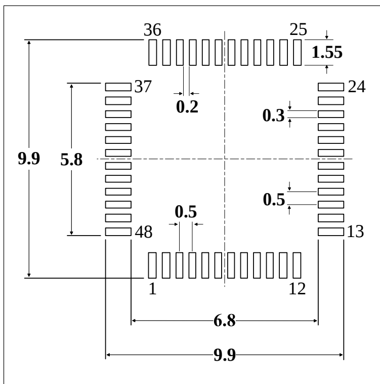
图 5-8 LQFP48 封装焊盘建议 (1)
