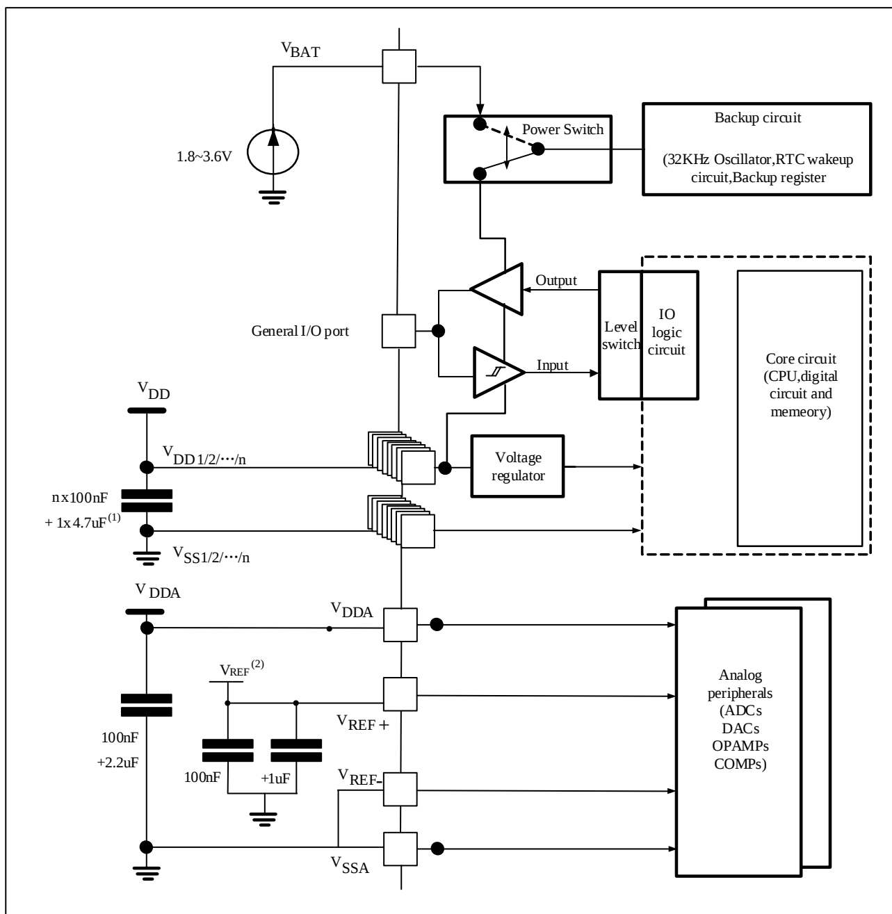
图 4-3 供电方案
