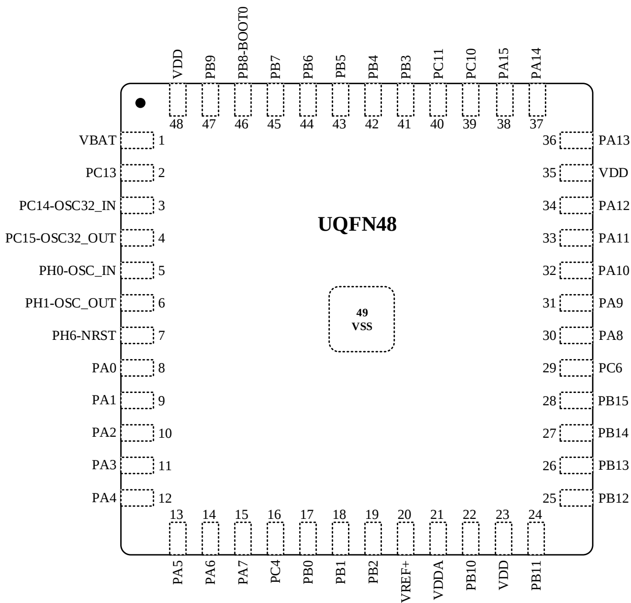
图 3-3 UQFN48 引脚分布
