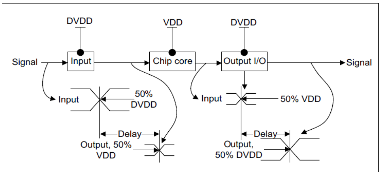
图 4-10 传输延迟
