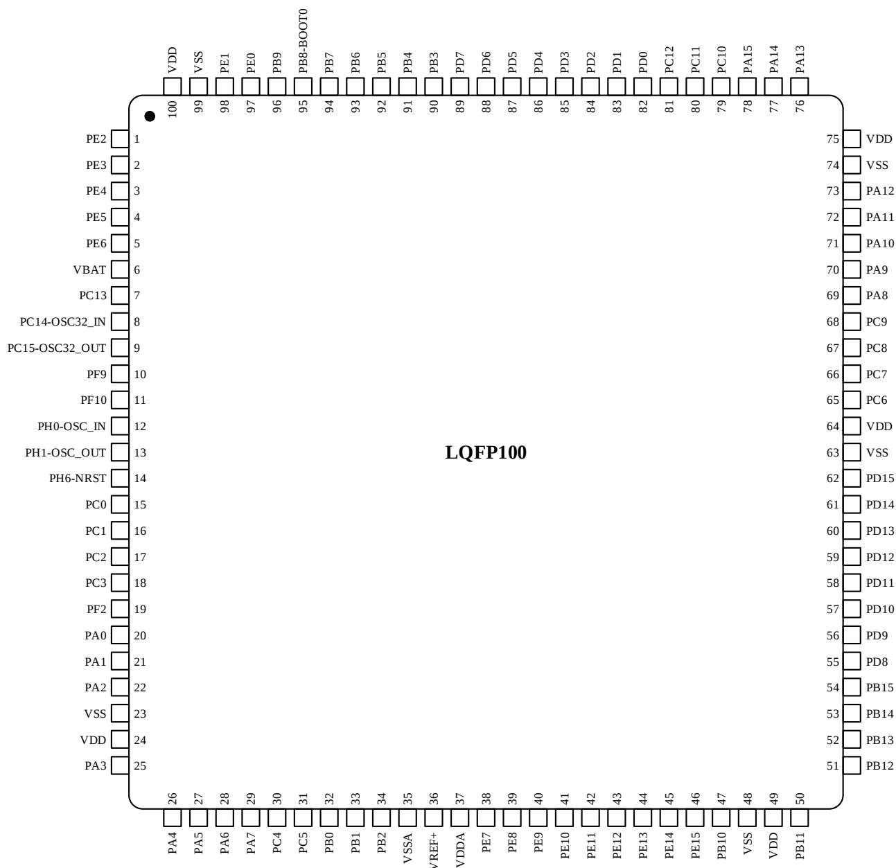
图 3-9 LQFP100 引脚分布
