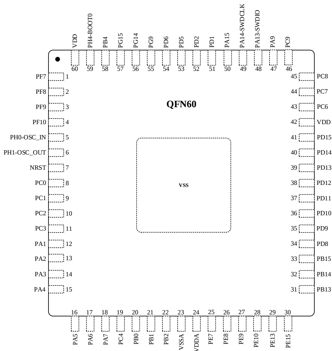
图 3-6 QFN60 引脚分布
