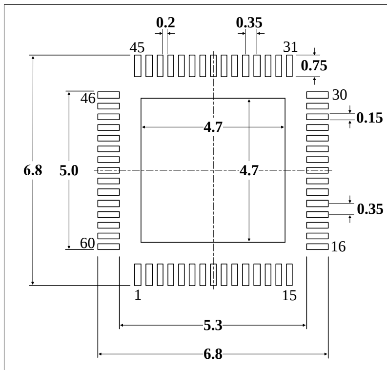
图 5-10 QFN60 封装焊盘建议 (1)
