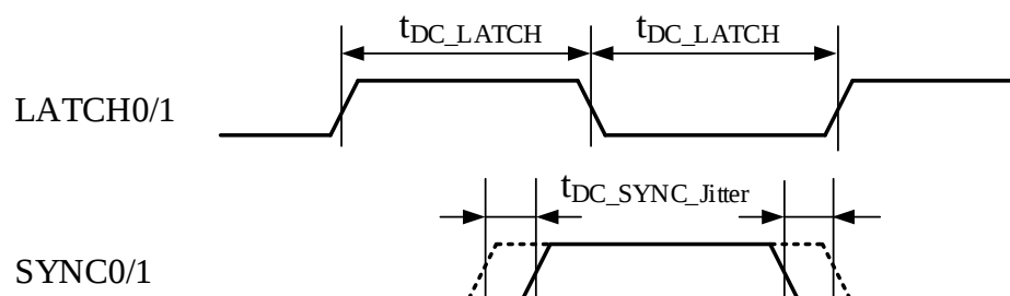
图 4-47 ESC Sync/Latch 信号时序图
