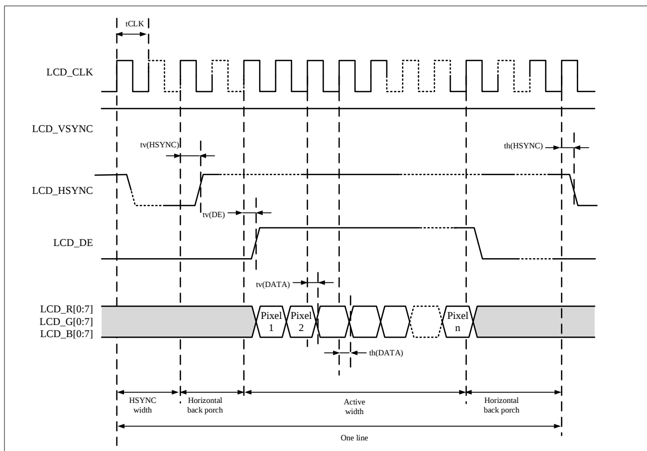
图 4-53 LCDC 水平时序框图
