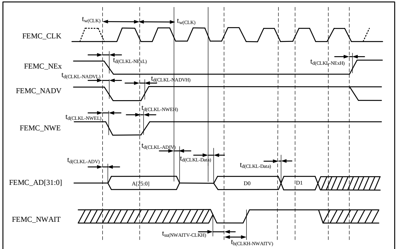
图 4-34 同步复用 PSRAM 写时序
