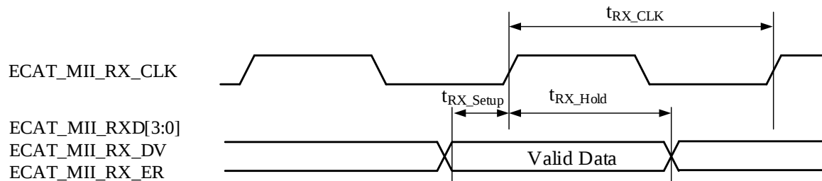
图 4-46 ESC MII RX 信号时序图
