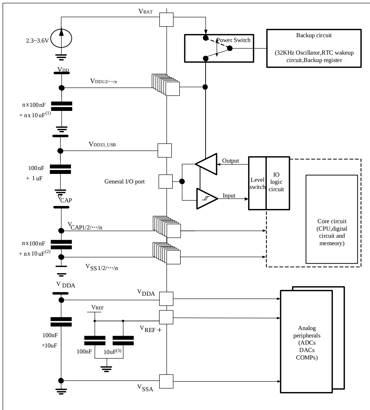
图 4-3 供电方案
