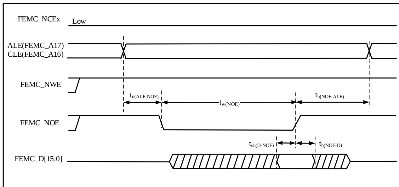
图 4-40 NAND 控制器写操作波形
