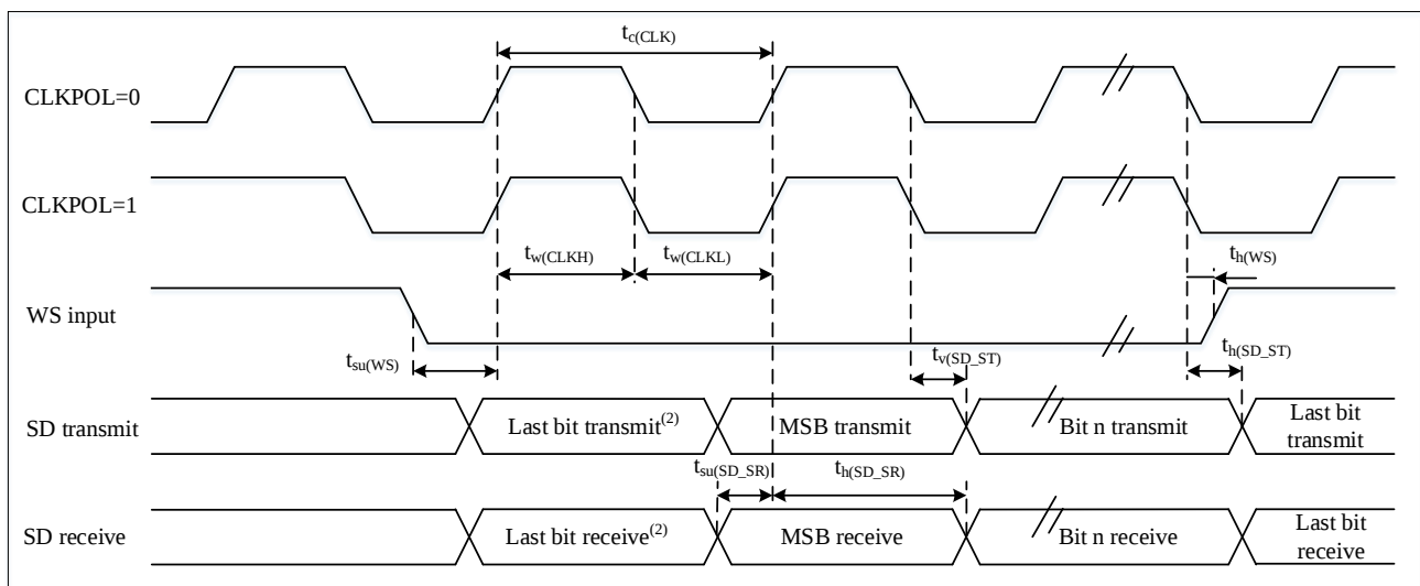
图 4-20 I 2 S 从模式时序图（飞利浦协议） (1)
