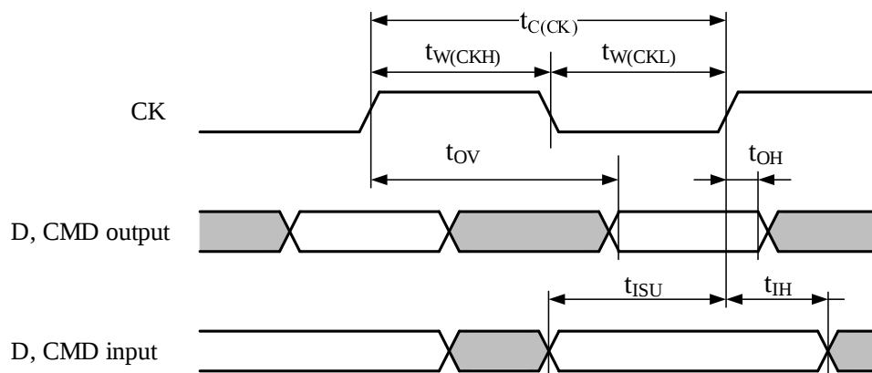
图 4-42 SD 默认模式
