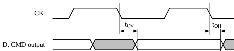
图 4-43 SDMMC DDR 模式
