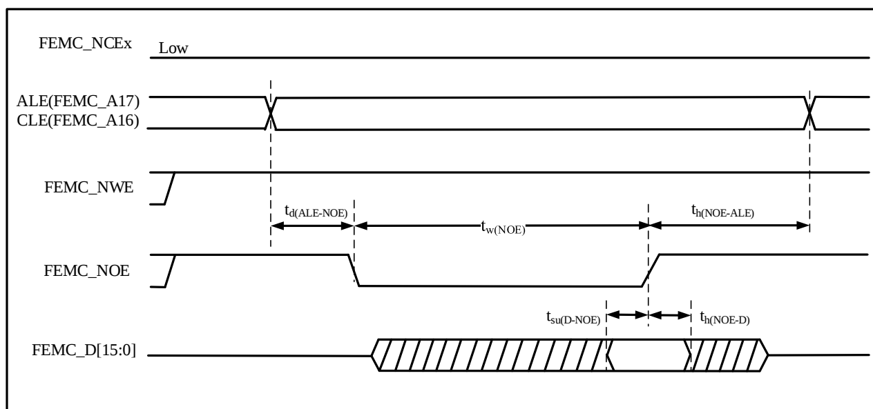
图 4-37 NAND 控制器读操作波形
