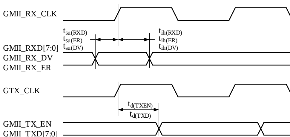
图 4-50 MII 时序图
