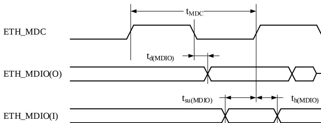
图 4-48 MDIO/SMA 时序图
