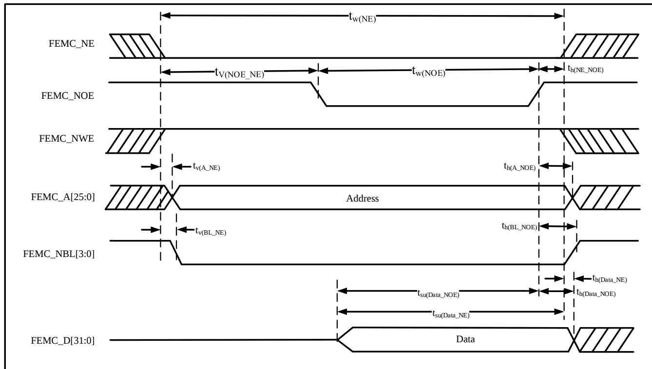
图 4-27 异步非总线复用的 SRAM/PSRAM/NOR 读操作波形
