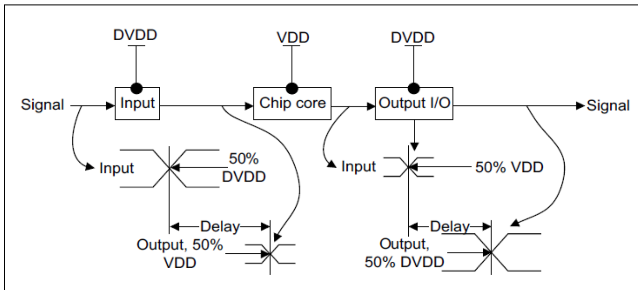
图 4-12 传输延迟
