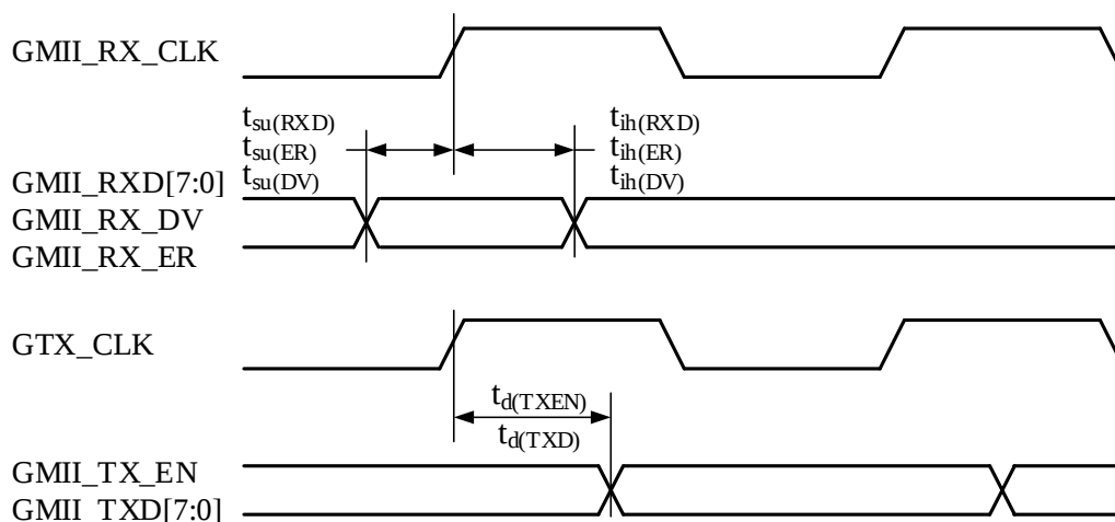
图 4-51 GMII 时序图
