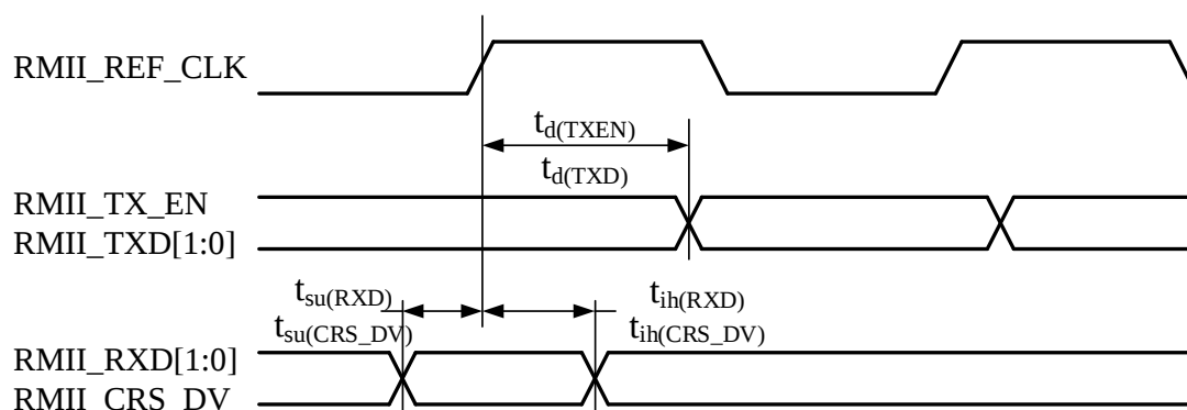
图 4-49 RMII 时序图
