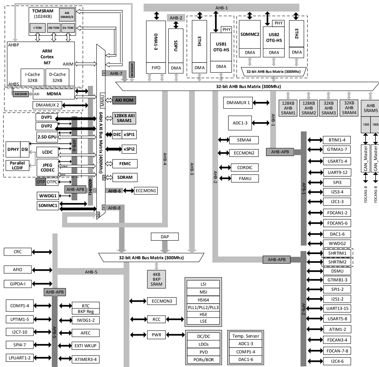
图 1-1 N32H765Ix7EC 系列框图
