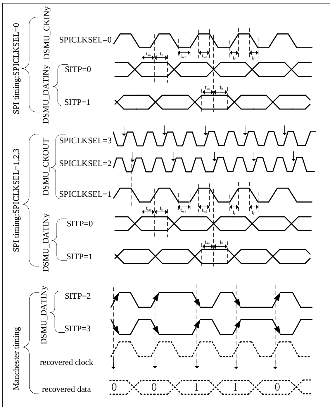
图 4-55 DSMU 通道收发器时序图
