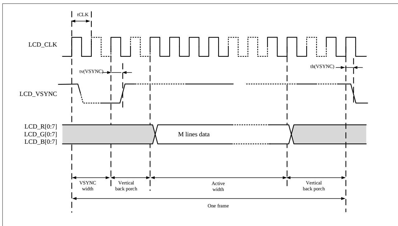
图 4-54 LCDC 垂直时序框图
