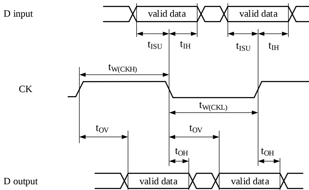
图 4-43 SDMMC DDR 模式
