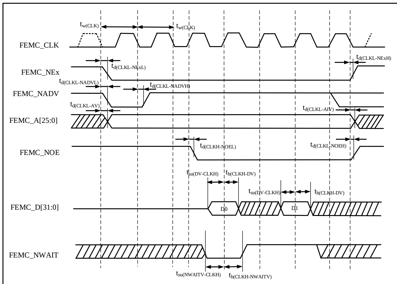
图 4-31 同步非总线复用 NOR/PSRAM 读时序
