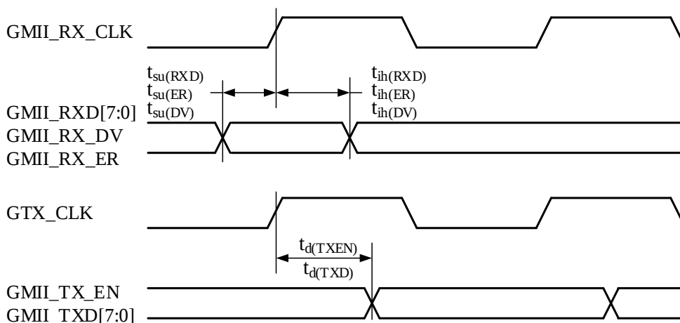
图 4-50 MII 时序图
