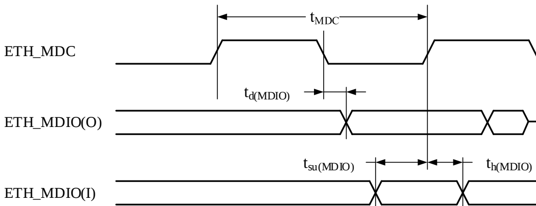
图 4-48 MDIO/SMA 时序图
