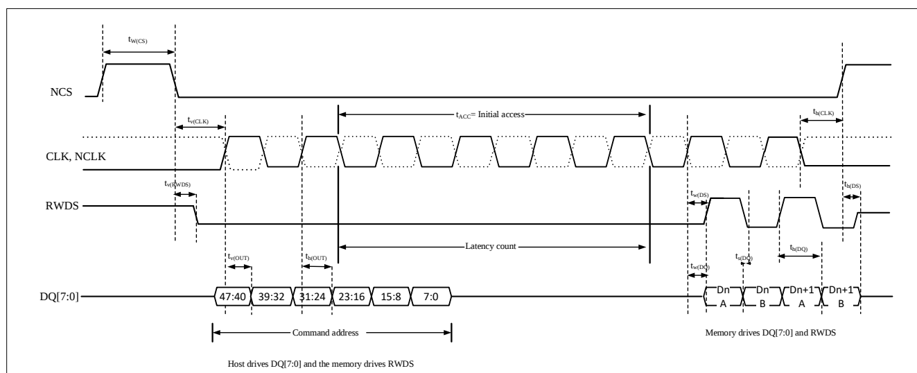
图 4-25 xSPI Hyperbus 时钟读时序图
