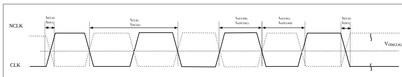
图 4-25 xSPI Hyperbus 时钟读时序图
