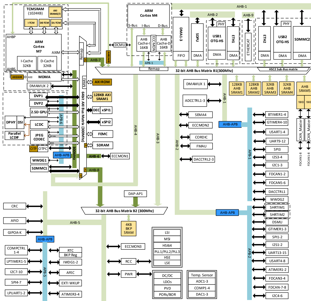
图 1-1 N32H785XxB7EC 系列框图
