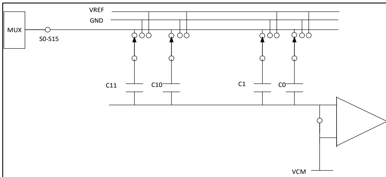
图 1.2-1 ADC 采样阶段等效电路
