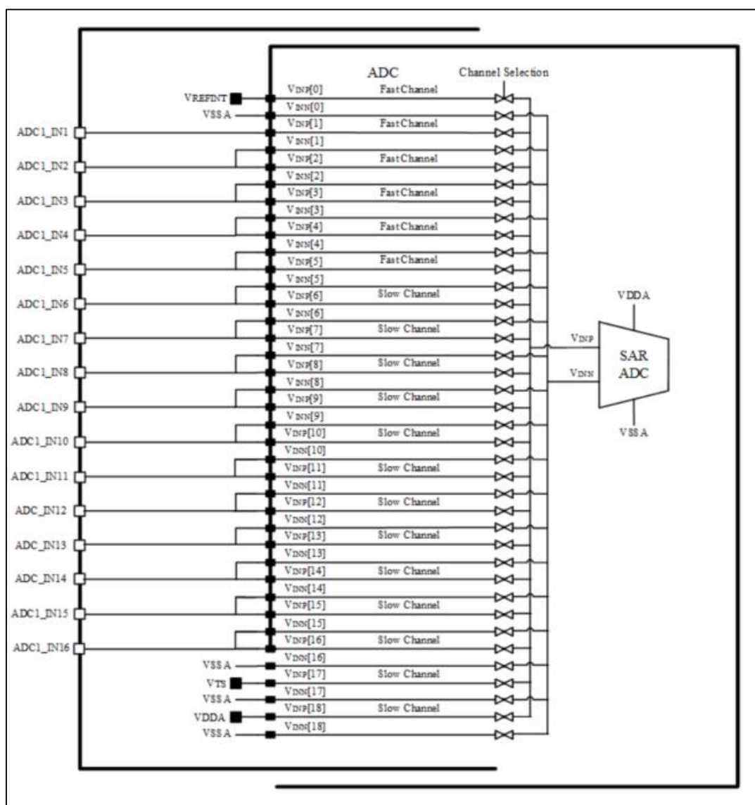
图 2.7-1 ADC 通道和 PIN 脚关系
