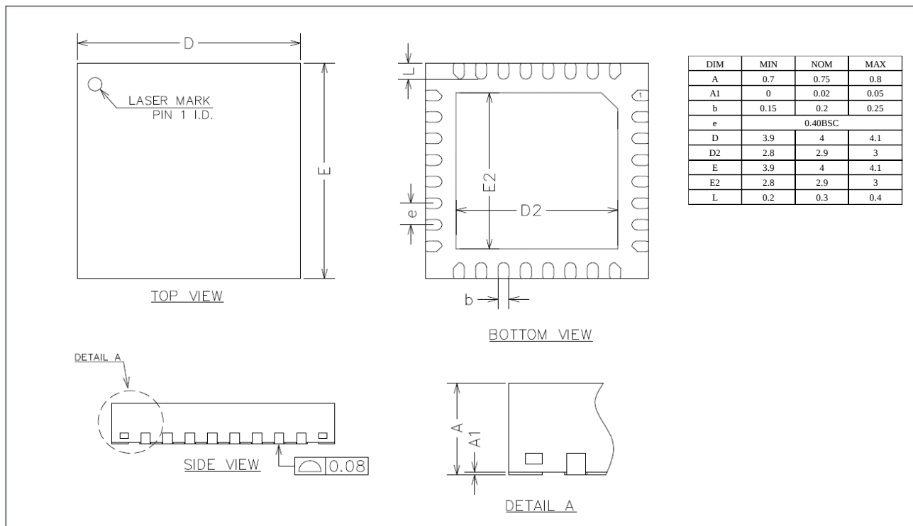
图 5-5 QFN32(4x4mm)封装尺寸
