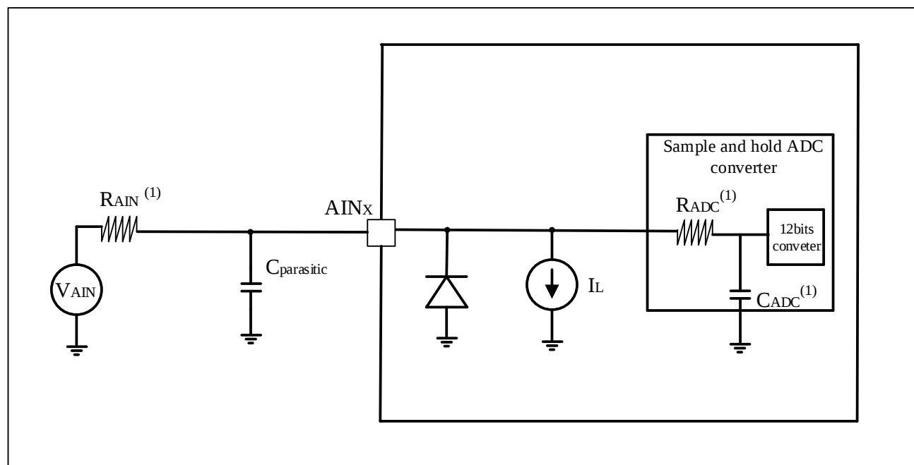
图 4-12 使用 ADC 典型的连接图
