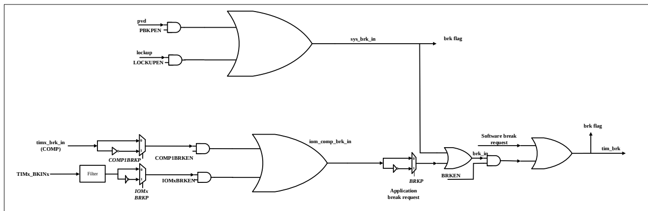
图 13-22 刹车输入
