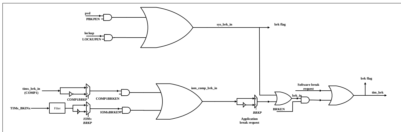
图 12-27 刹车输入
