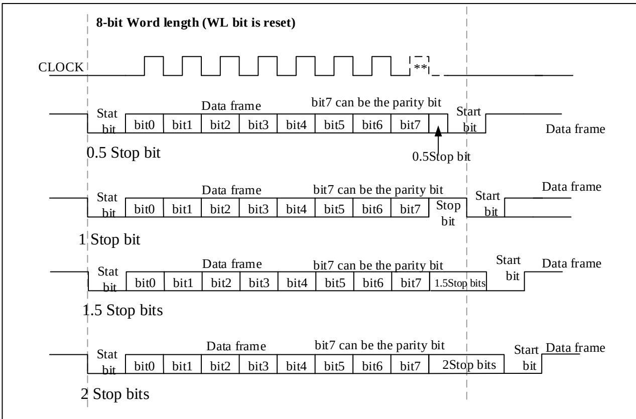
图 9-4 停止位配置
