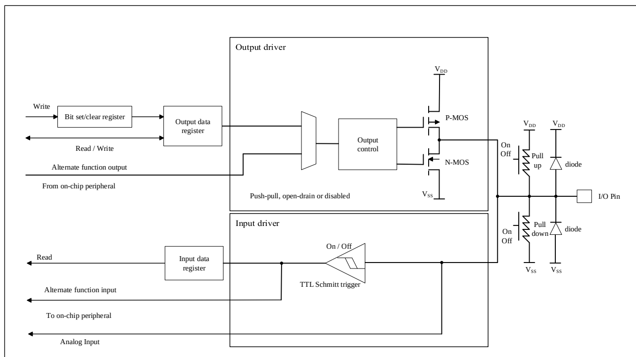
图 6-1 I/O 端口的基本结构（不支持 Fail-safe）
