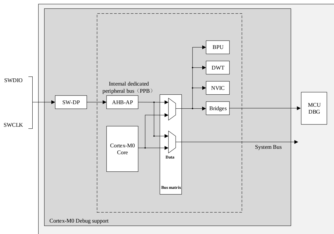
图 21-1 级别和 Cortex®-M0 级别的调试框图
