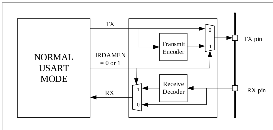
图 9-13 IrDA 数据调制(3/16)-正常模式
