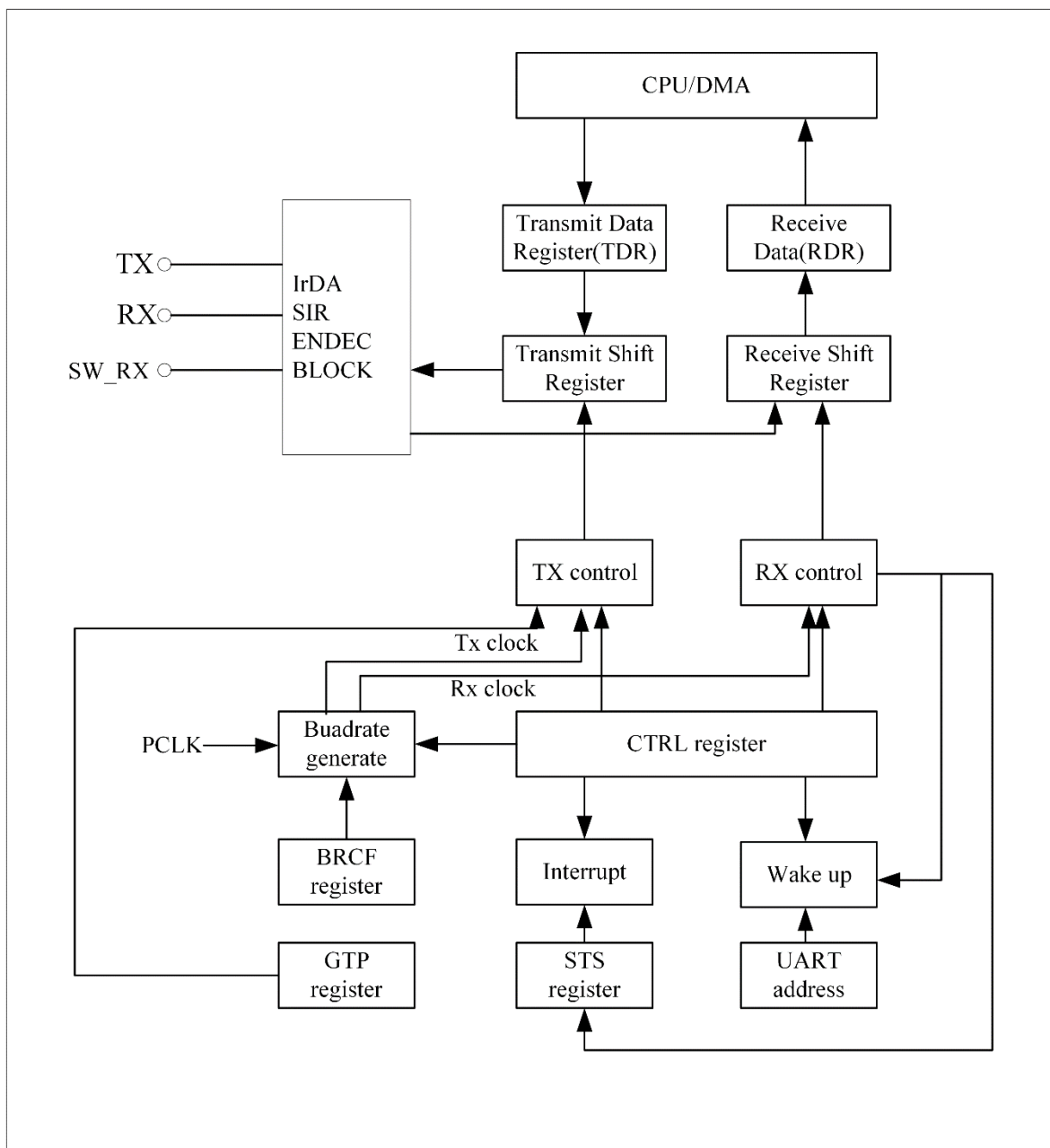
图 9-1 UART 框图
