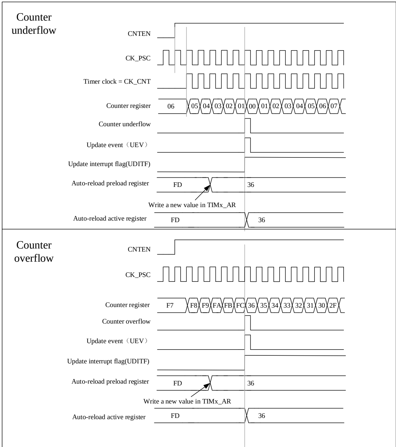
图 14-7 包含计数器上溢和下溢的中央对齐时序图(ARPEN=1)
