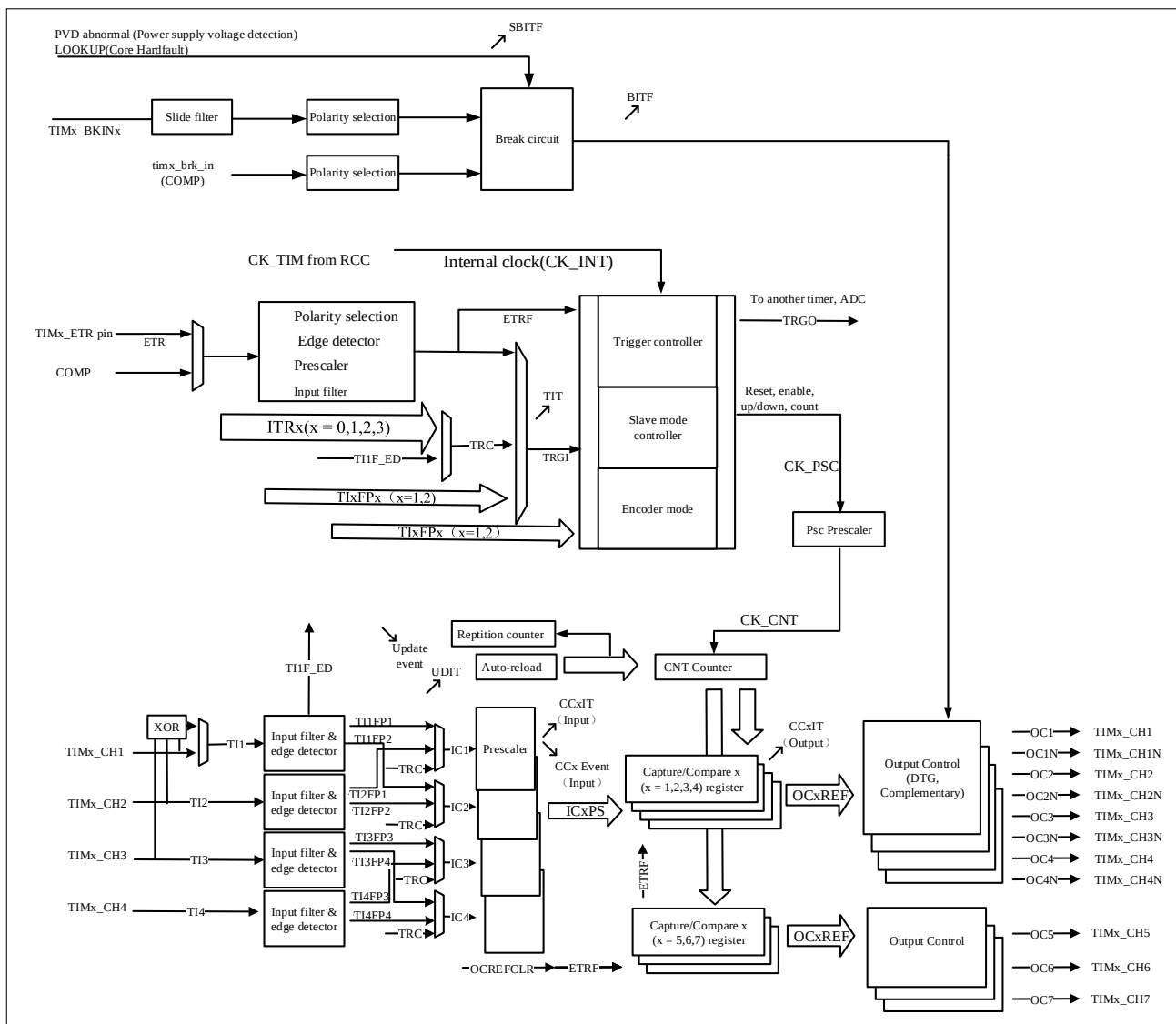
图 12-1 TIM1 框图
