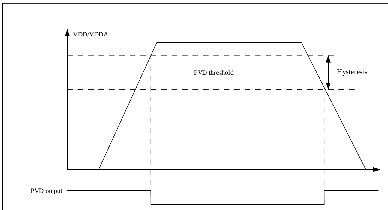
图 3-3 PVD 阈值图
