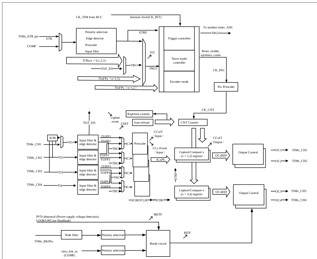
图 13-1 TIM3 框图
