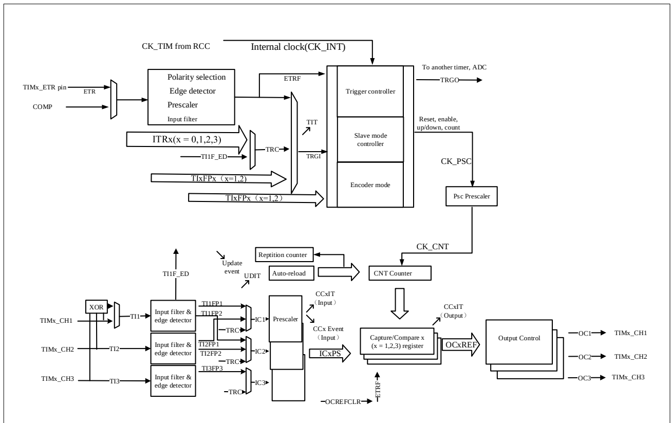
图 14-1 TIM4 框图
