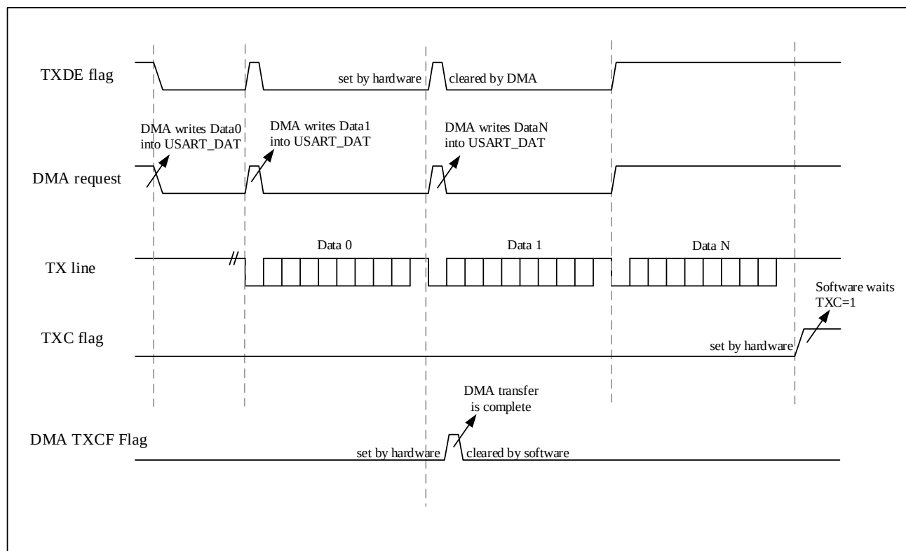
图 9-8 DMA 发送
