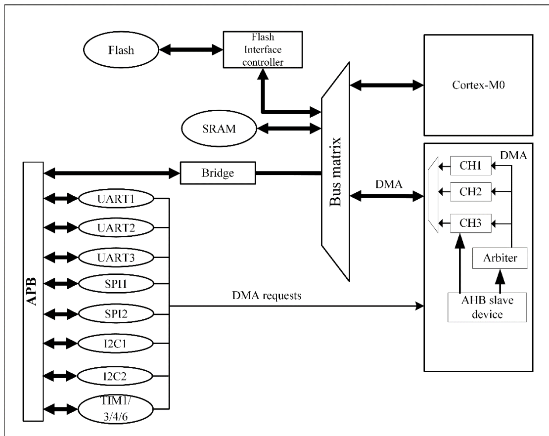
图 7-1 DMA 框图
