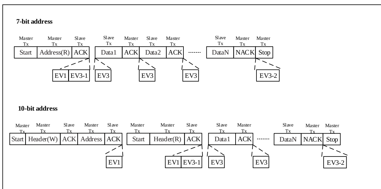
图 8-3 从发送器传送序列
