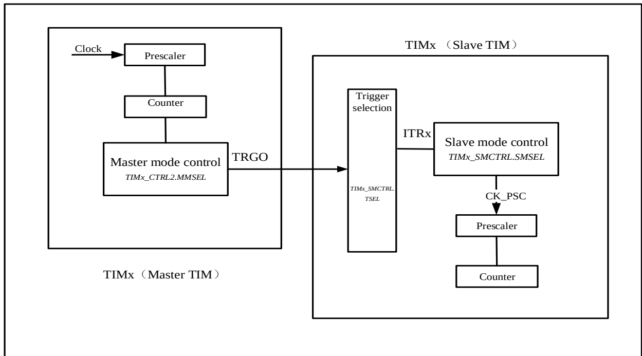
图 13-25 主/从定时器的例子
