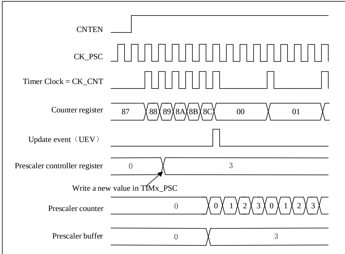
图 15-2 预分频器分频从 1 到 4 的计数器时序图
