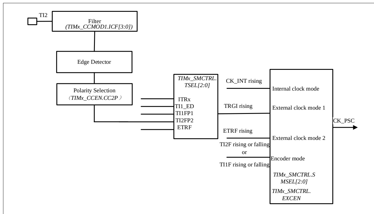
图 12-13 TI2 外部时钟连接示例
