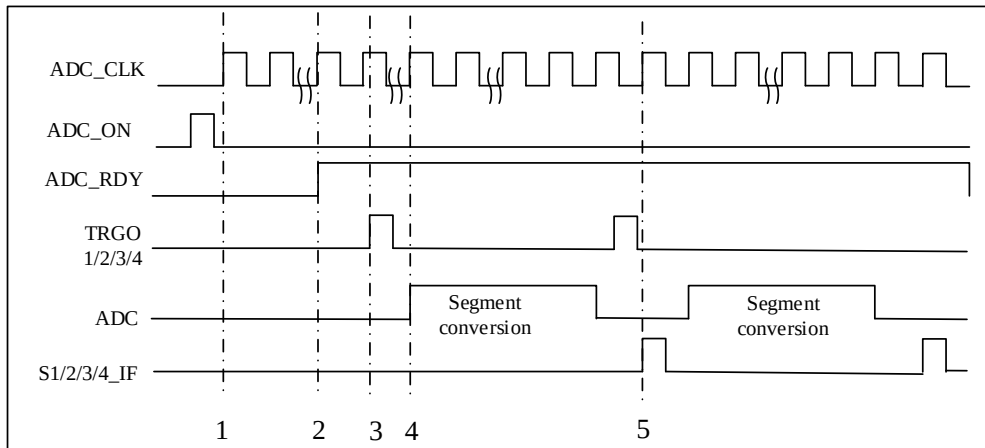
图 16-3 ADC 转换
