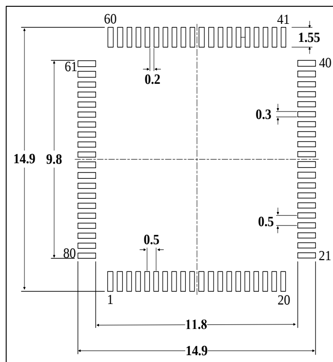
图 5-4 LQFP80封装焊盘建议 (1)
