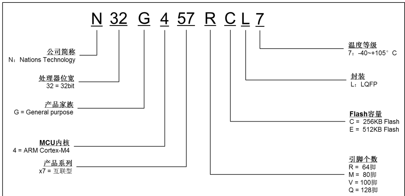
图 6-1 N32G457系列订货代码信息图示
