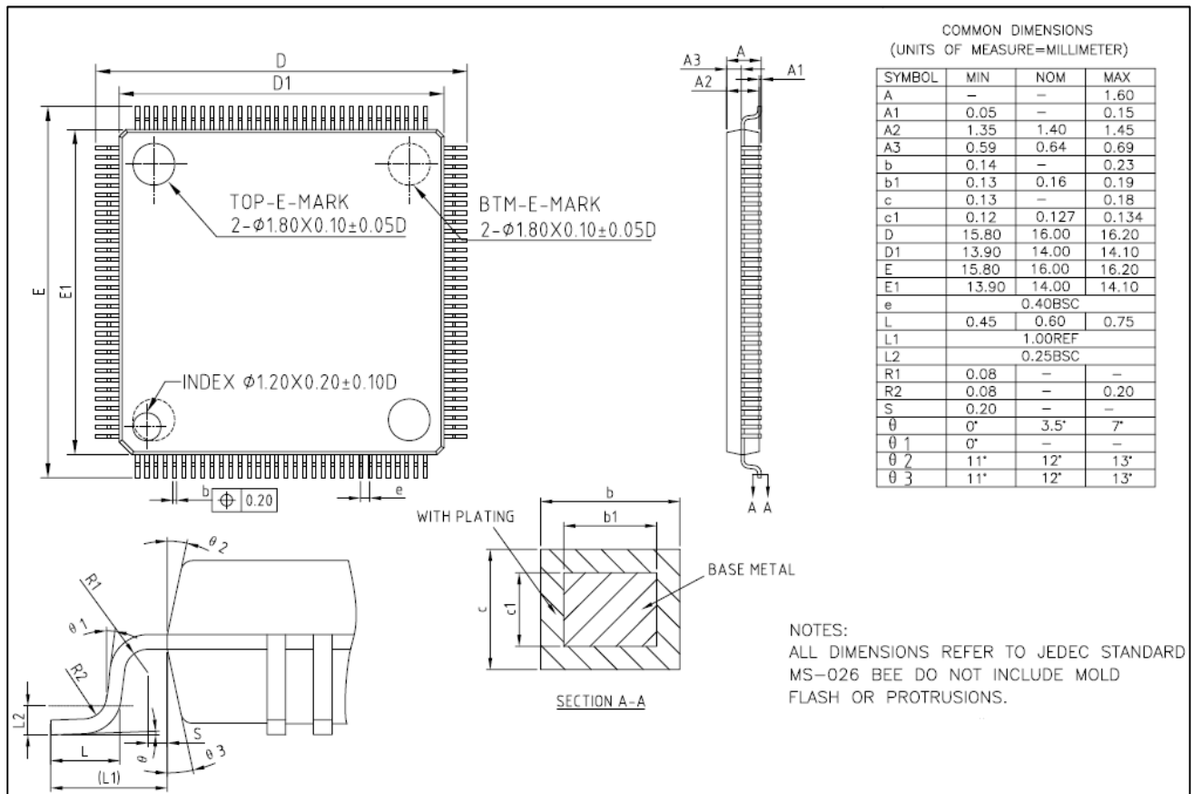
图 5-7 LQFP128封装尺寸
