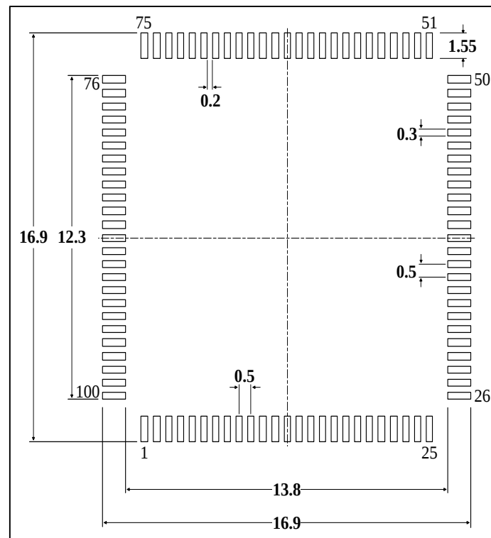
图 5-6 LQFP100封装焊盘建议 (1)
