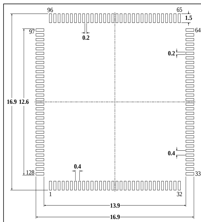
图 5-8 LQFP128封装焊盘建议 (1)
