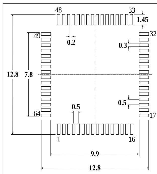
图 5-2 LQFP64封装焊盘建议 (1)
