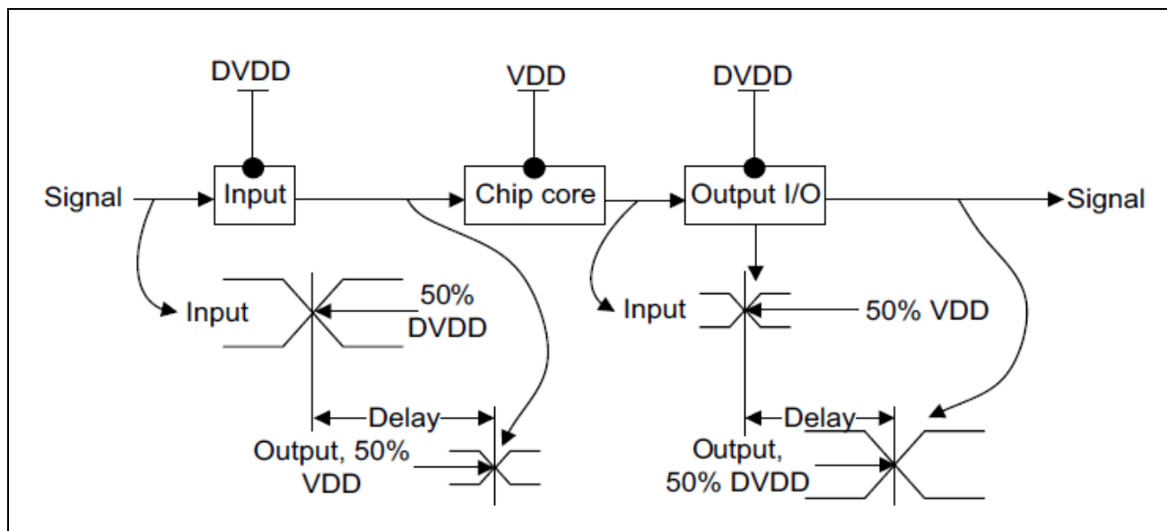
图 4-10 传输延迟
