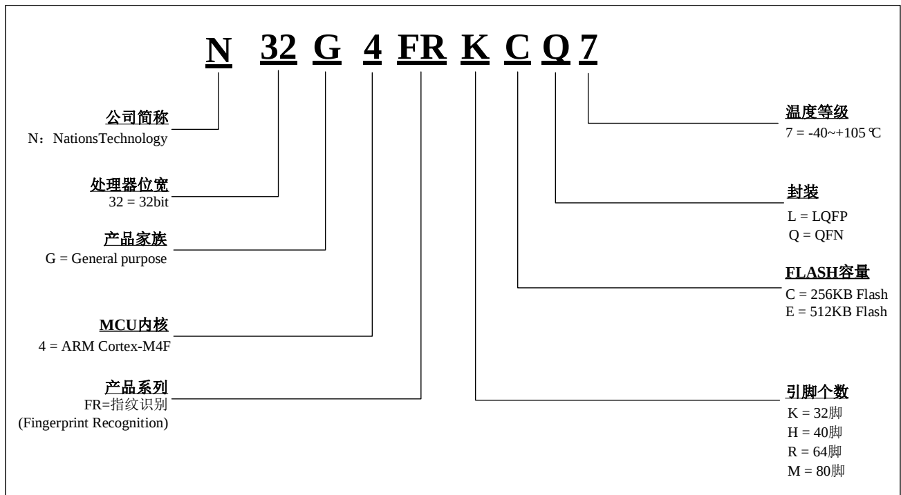
图 6-1 N32G4FR系列订货代码信息图示
