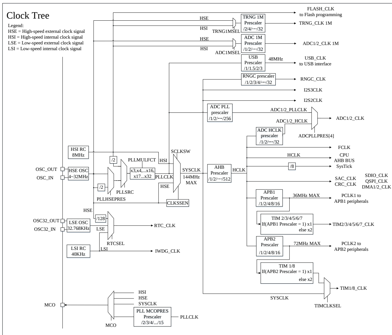
图 2-2 时钟树
