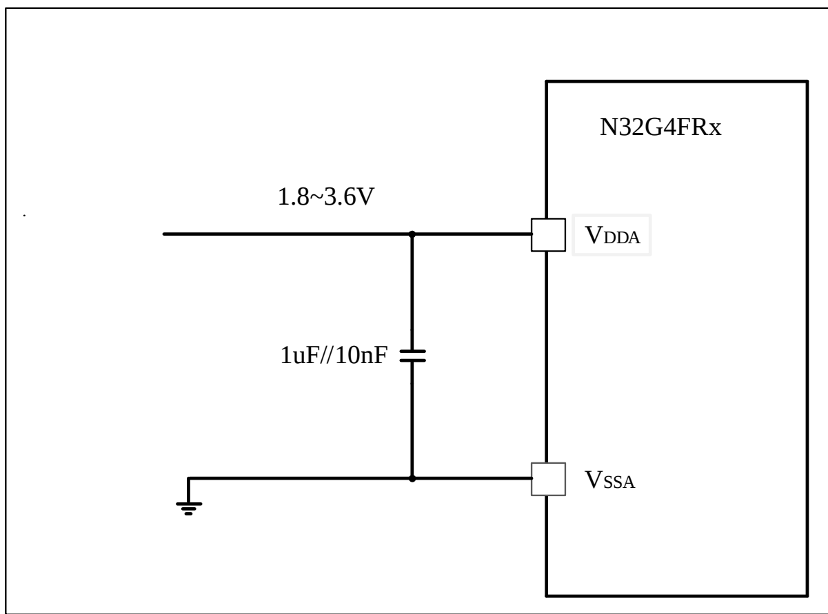
图 4-26 供电电源和参考电源去藕线路
