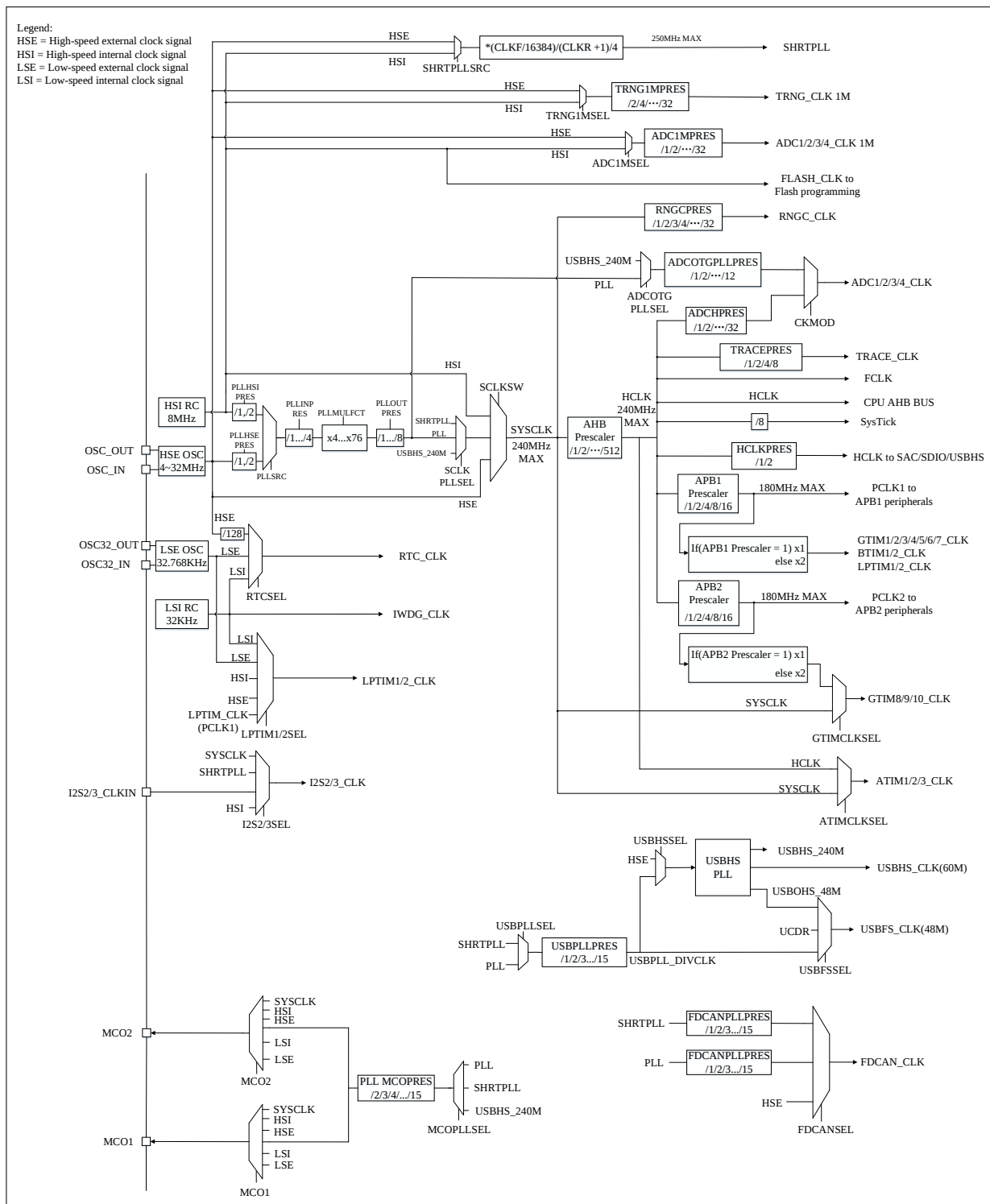
图 2-2 时钟树
