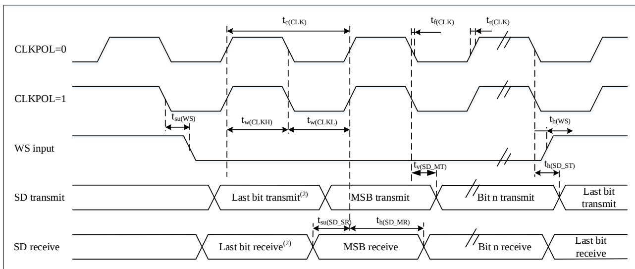
图 4-13 I 2 S主模式时序图(飞利浦协议) (1)
