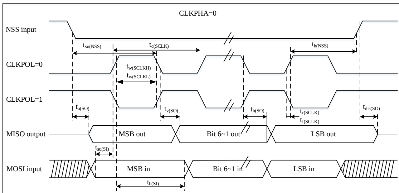
图 4-9 SPI时序图 – 从模式和CLKPHA=0
