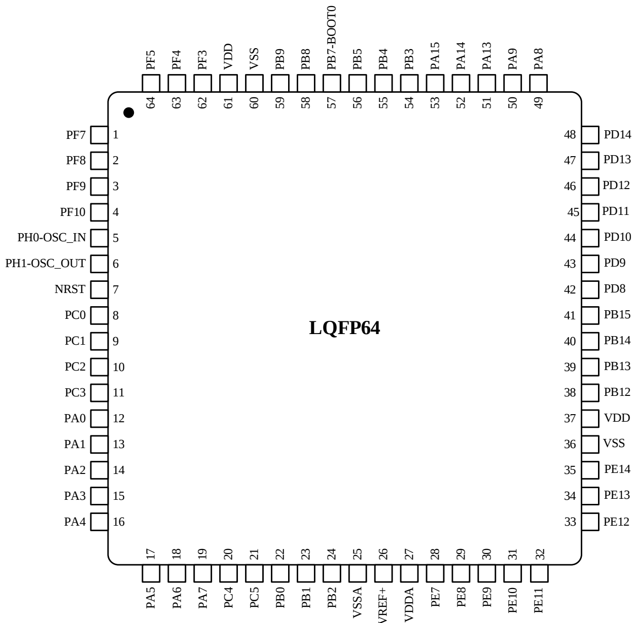
图 3-1 LQFP64 引脚分布
