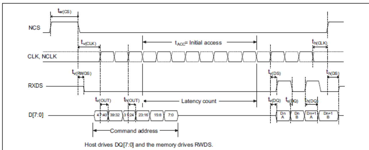
图 4-16 xSPI在RXDS模式下的时序
