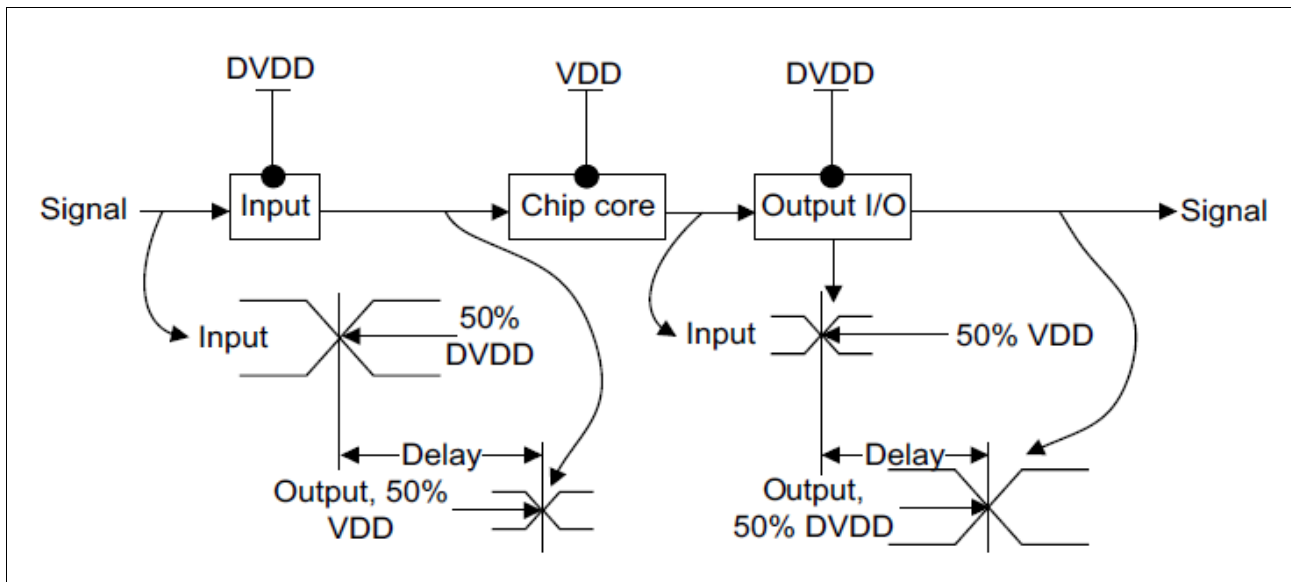
图 4-6 传输延迟
