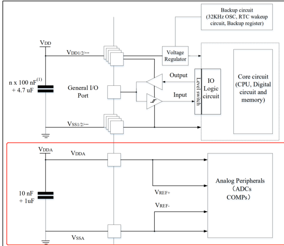
图 2.3-1 芯片供电系统
