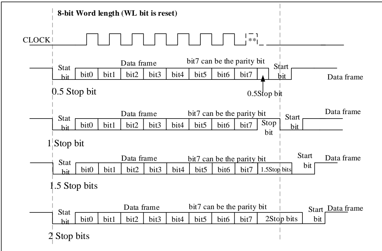
图 24-4 停止位配置
