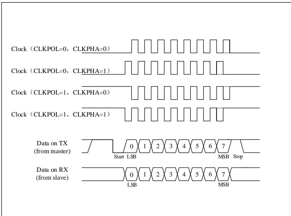
图 24-15 USART 数据时钟时序示例 (WL=0)
