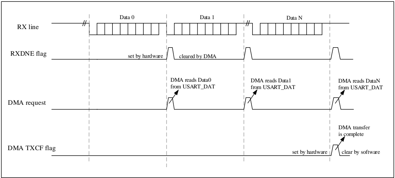
图 24-8 DMA 接收
