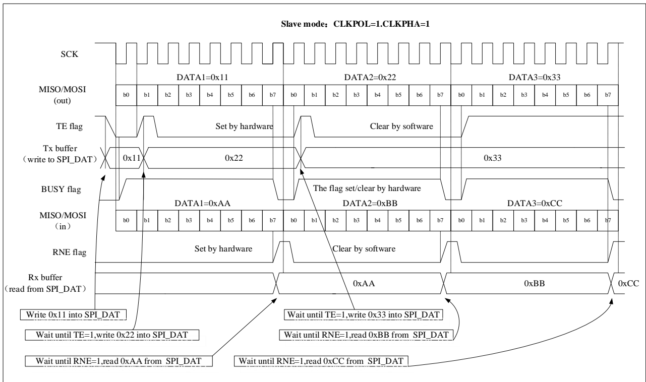
图 26-8 从机全双工模式下连续传输时，SPI_STS.TE/RNE/BUSY 的变化示意图
