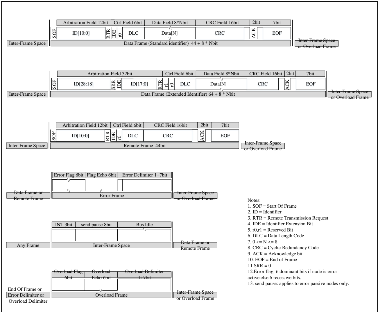
图 27-12 各类帧格式
