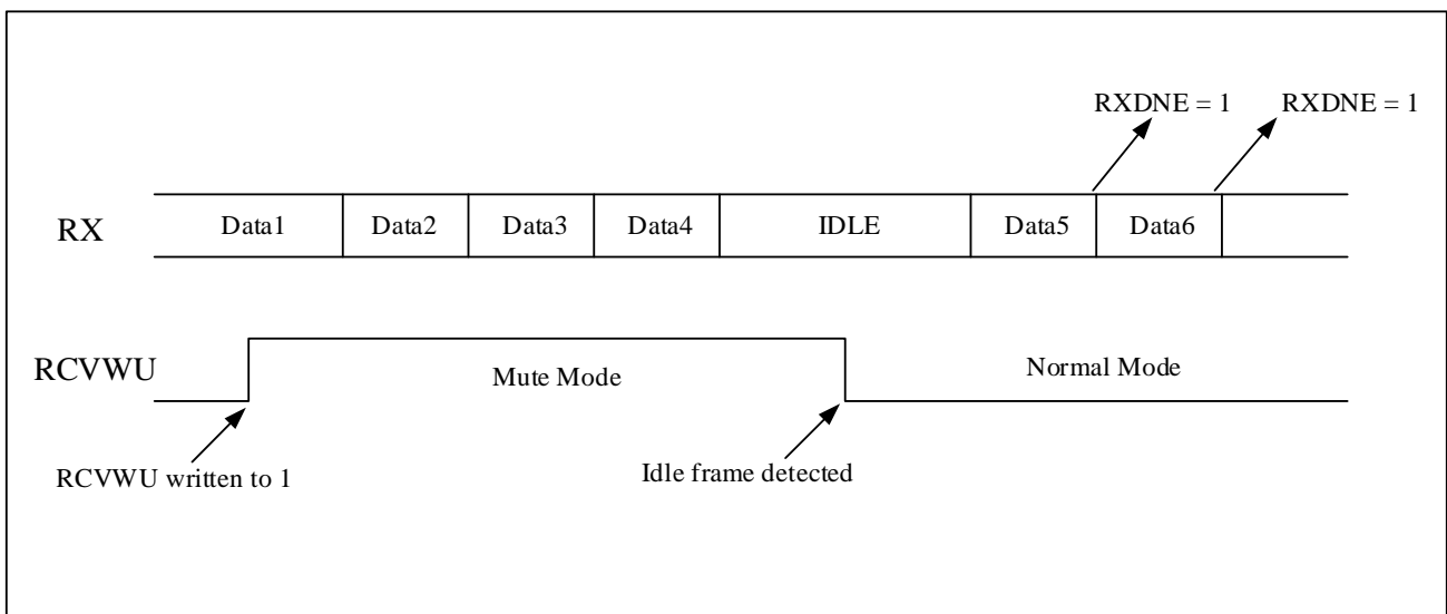
图 24-12 静默模式下的空闲总线检测
