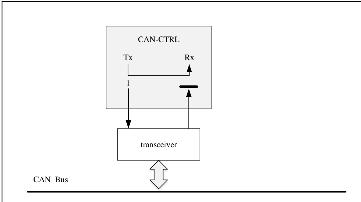
图 27-6 回环静默模式
