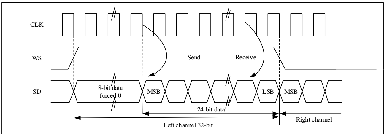
图 26-21 LSB 对齐 24 位数据，CLKPOL = 0
