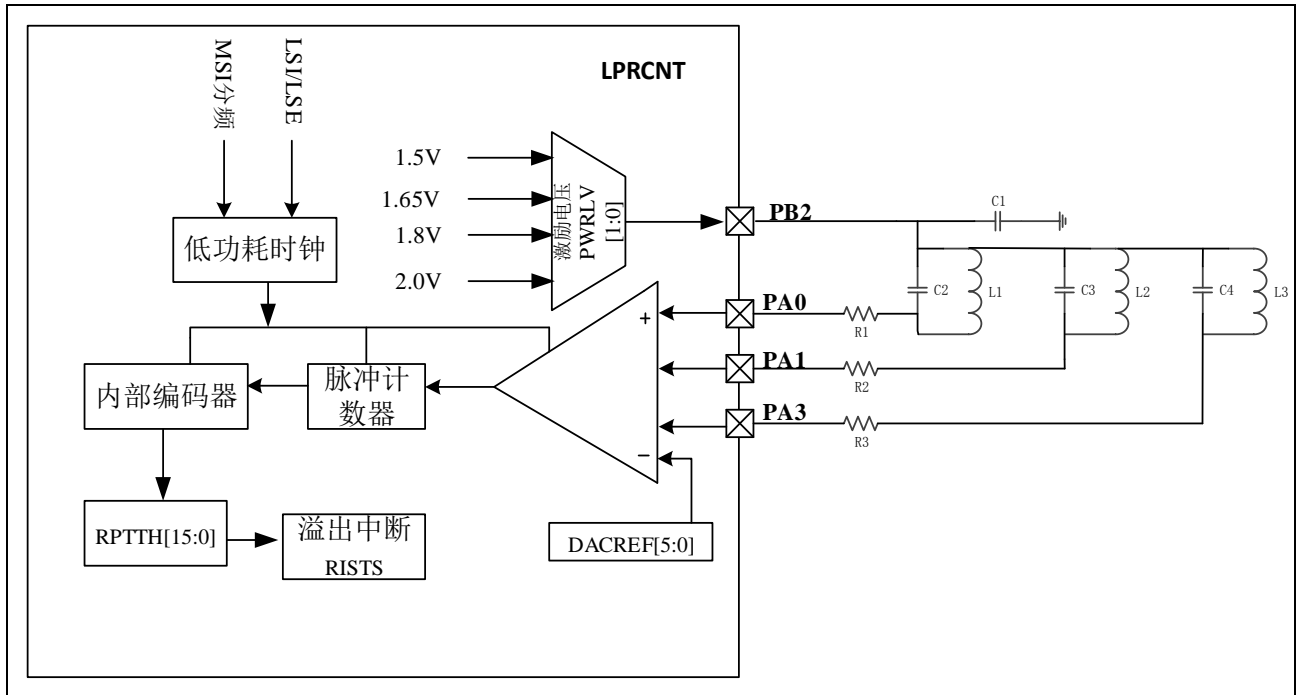
图 21-1 LPRCNT 框图
