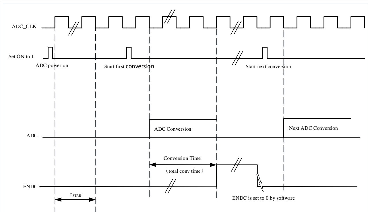
图 17-4 时序图
