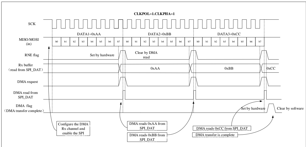
图 26-12 使用 DMA 接收
