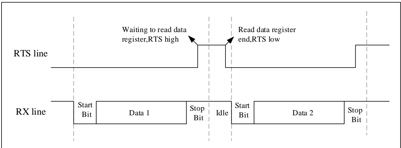
图 24-10 RTS 流控制
