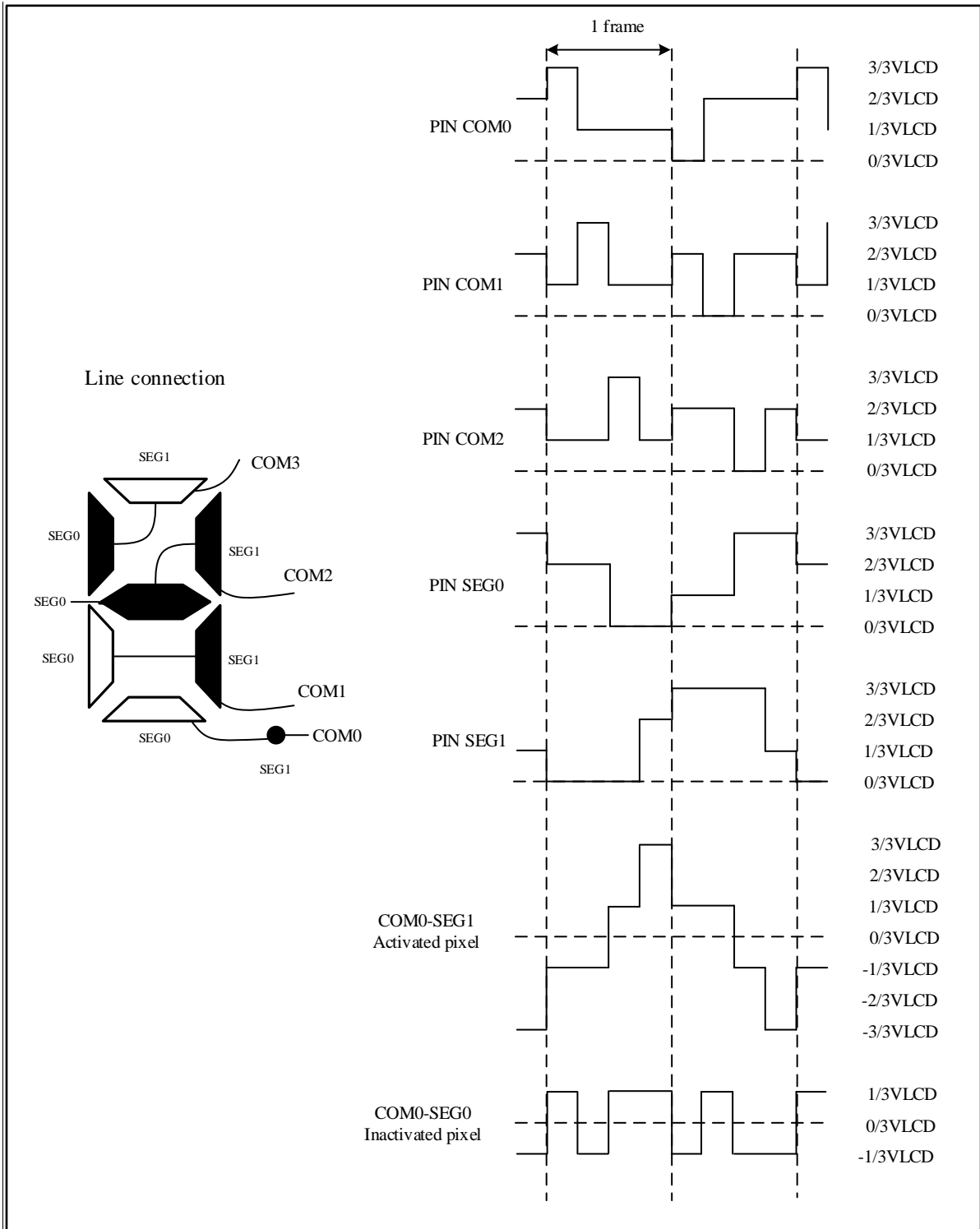
图 22-6 1/4 占空比, 1/3 偏置
