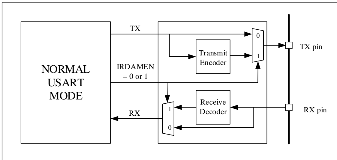
图 24-19 IrDA 数据调制(3/16)-正常模式
