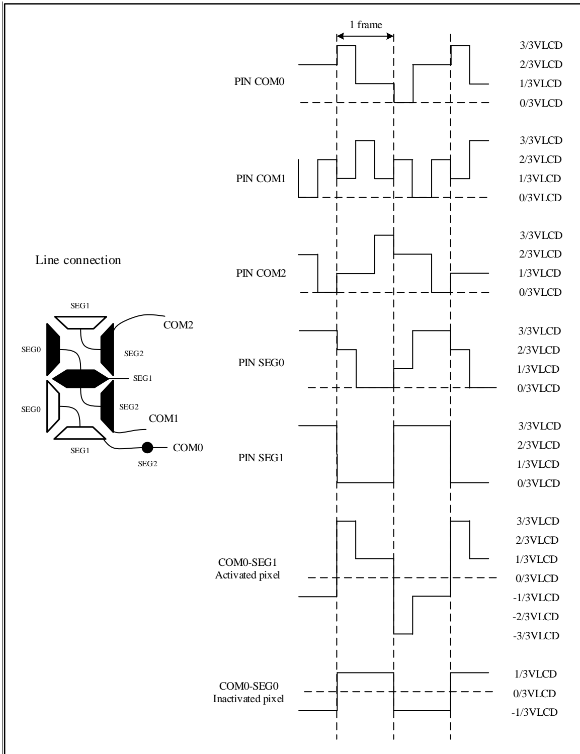
图 22-5 1/3 占空比, 1/3 偏置
