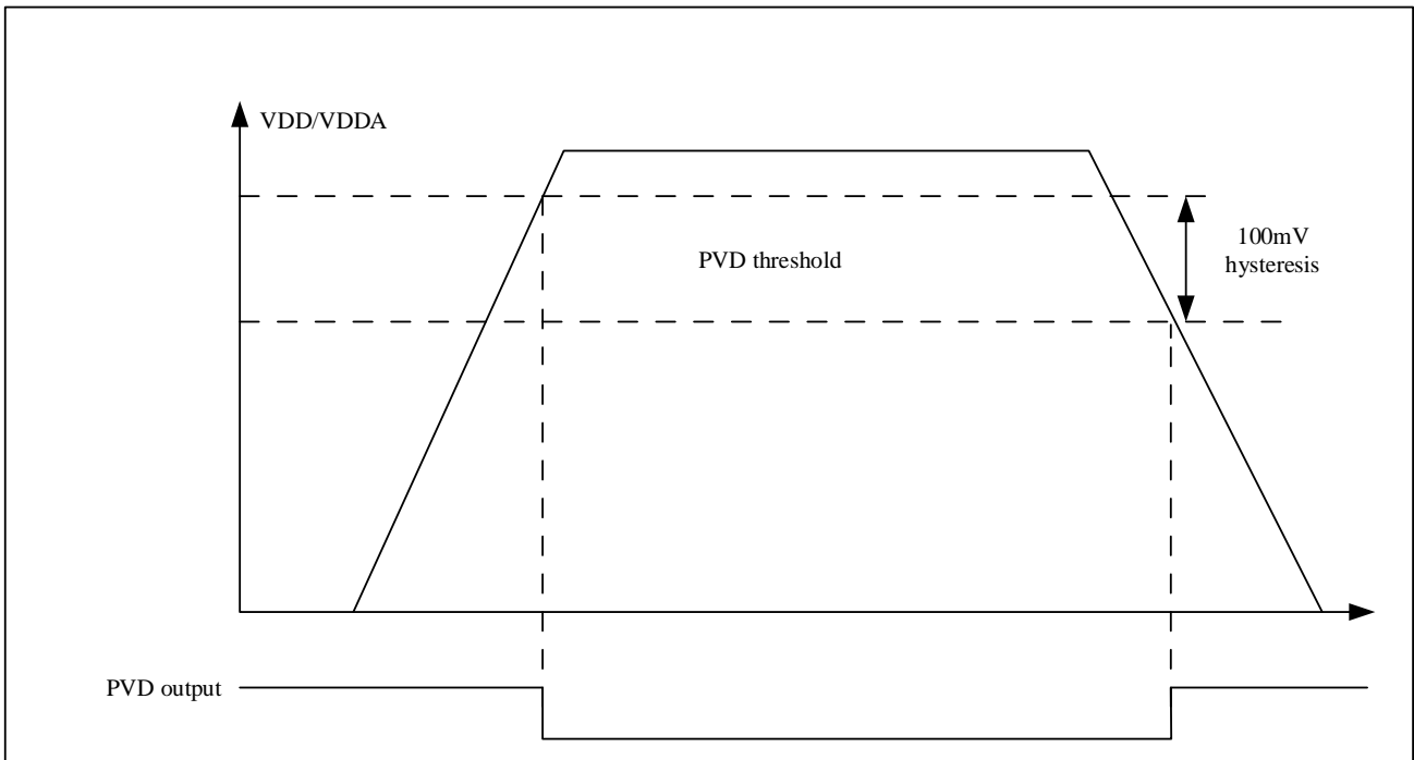
图 3-3 PVD 阈值波形图
