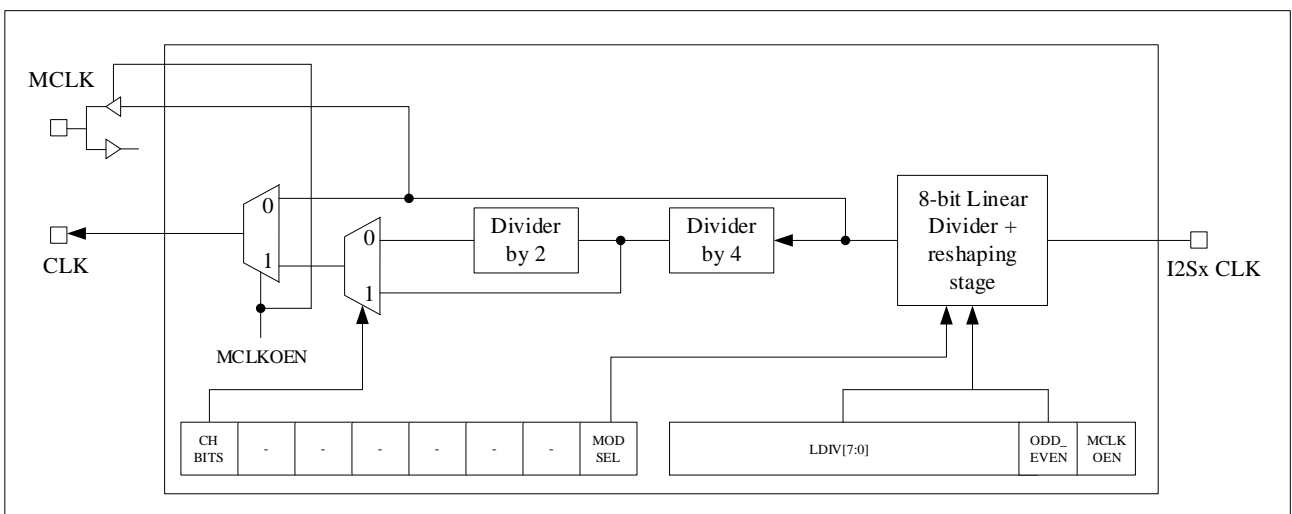
图 26-25 I 2 S 时钟发生器结构
