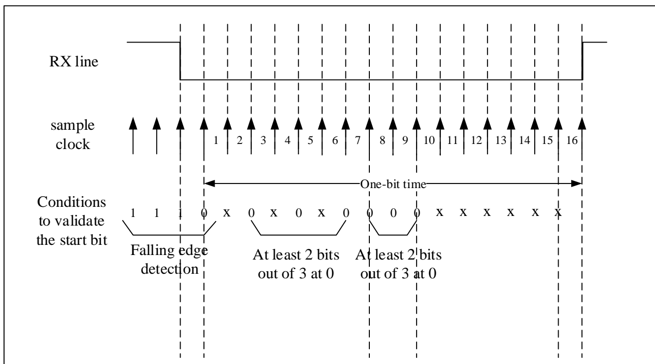
图 24-6 起始位检测
