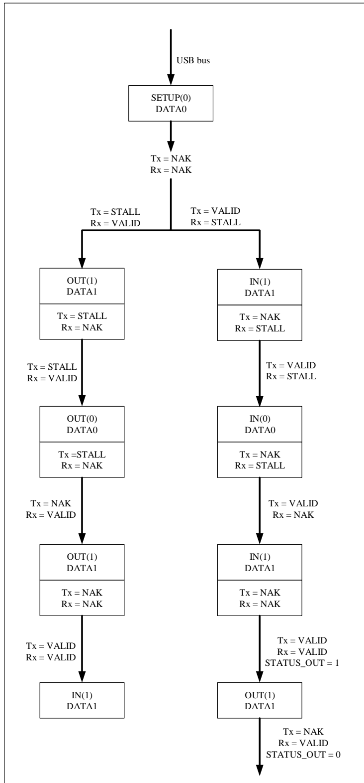
图 28-5 控制传输
