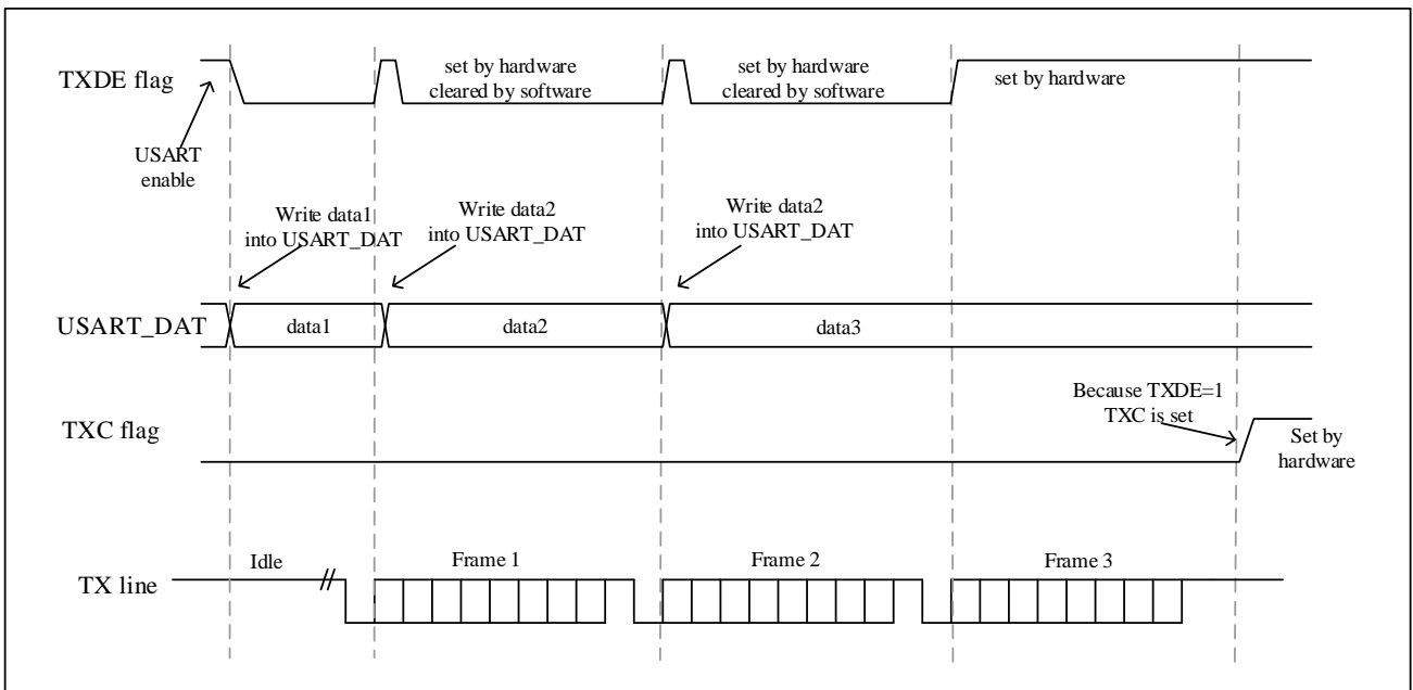
图 24-5 发送时 TXC/TXDE 的变化情况
