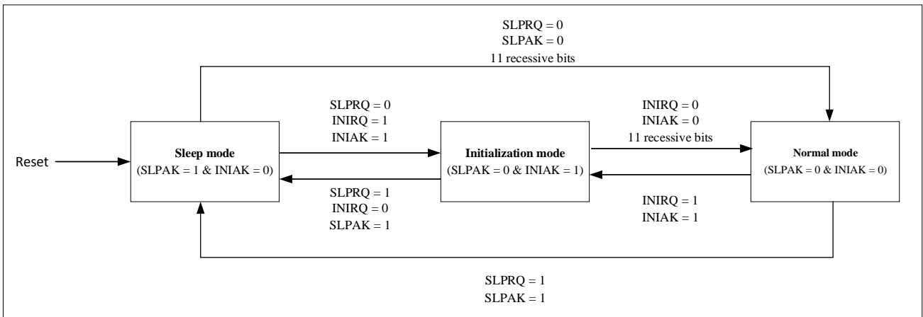
图 27-2 CAN 工作模式
