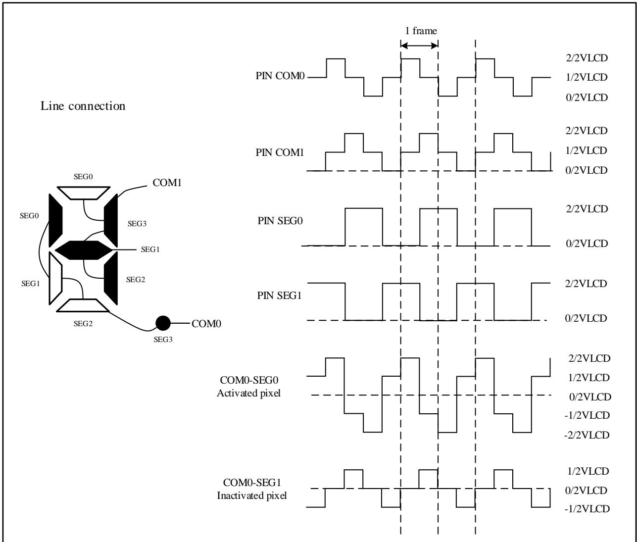
图 22-4 1/2 占空比, 1/2 偏置
