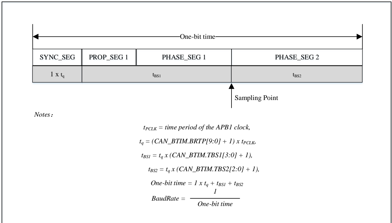
图 27-11 位时序
