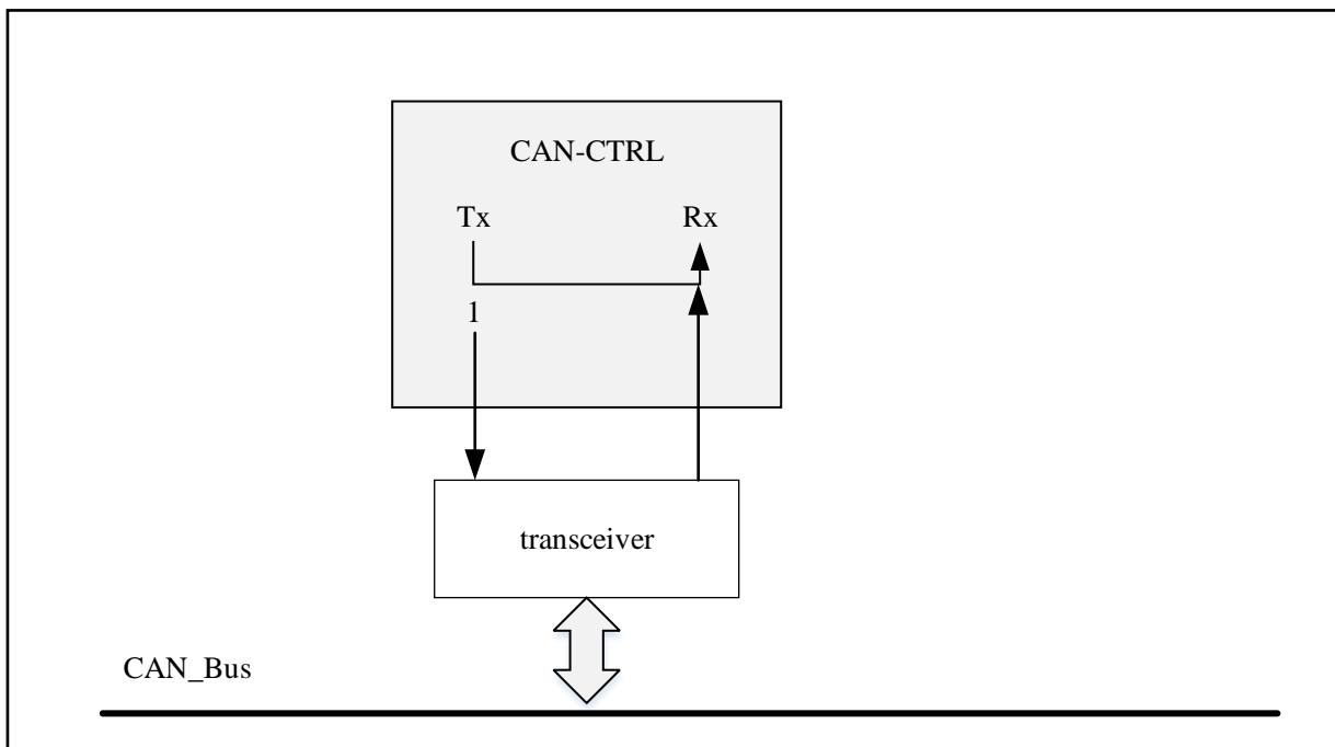
图 27-5 静默模式
