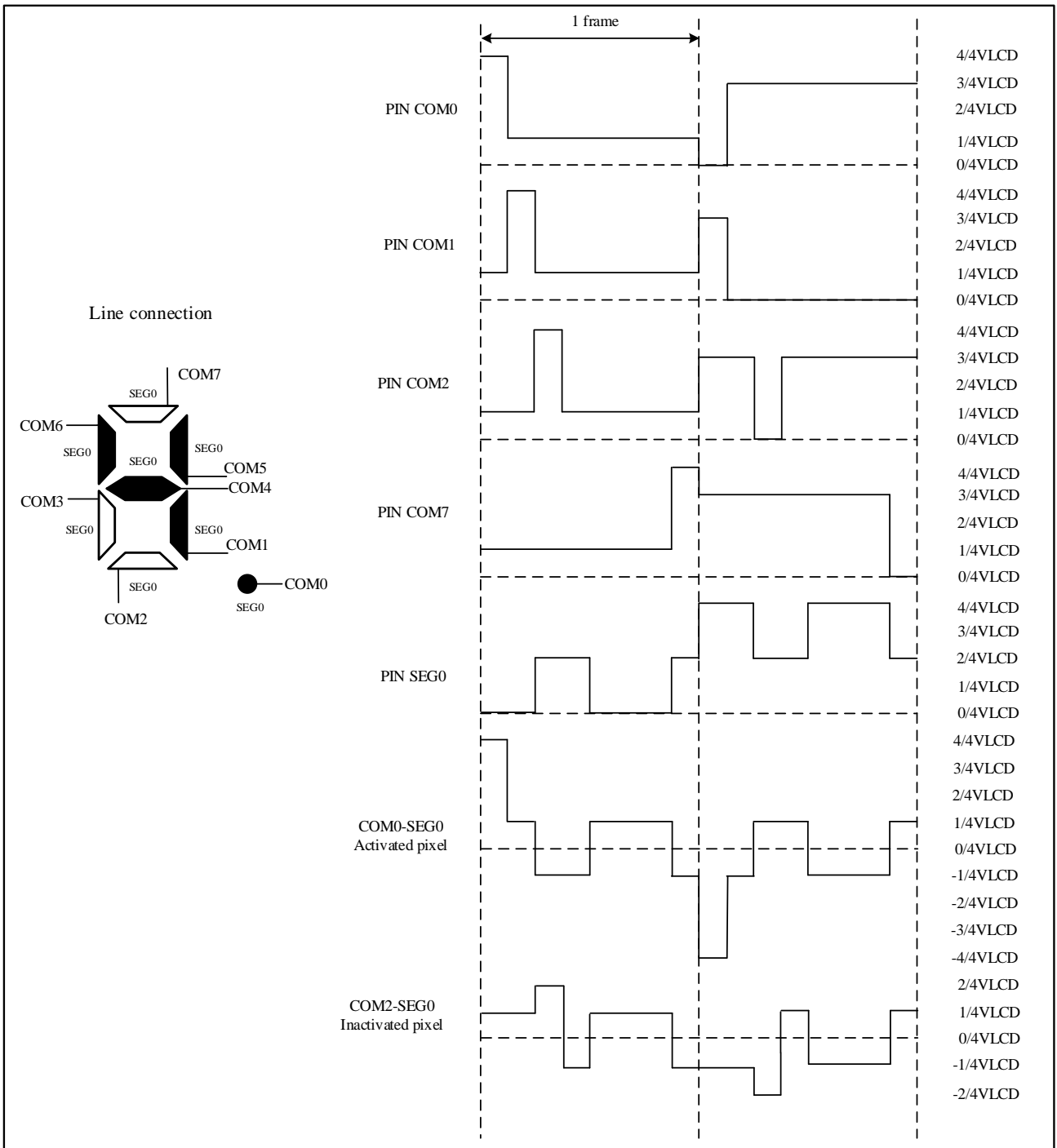
图 22-7 1/8 占空比, 1/4 偏置
