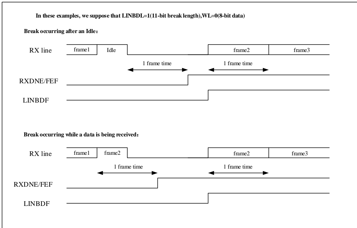
图 24-21 LIN 模式下的断开检测与帧错误的检测
