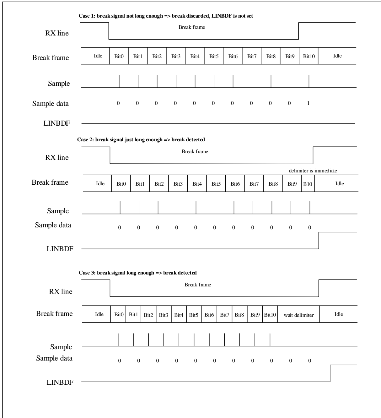
图 24-20 LIN 模式下的断开检测（11 位断开帧长度-设置了 LINBDL 位）
