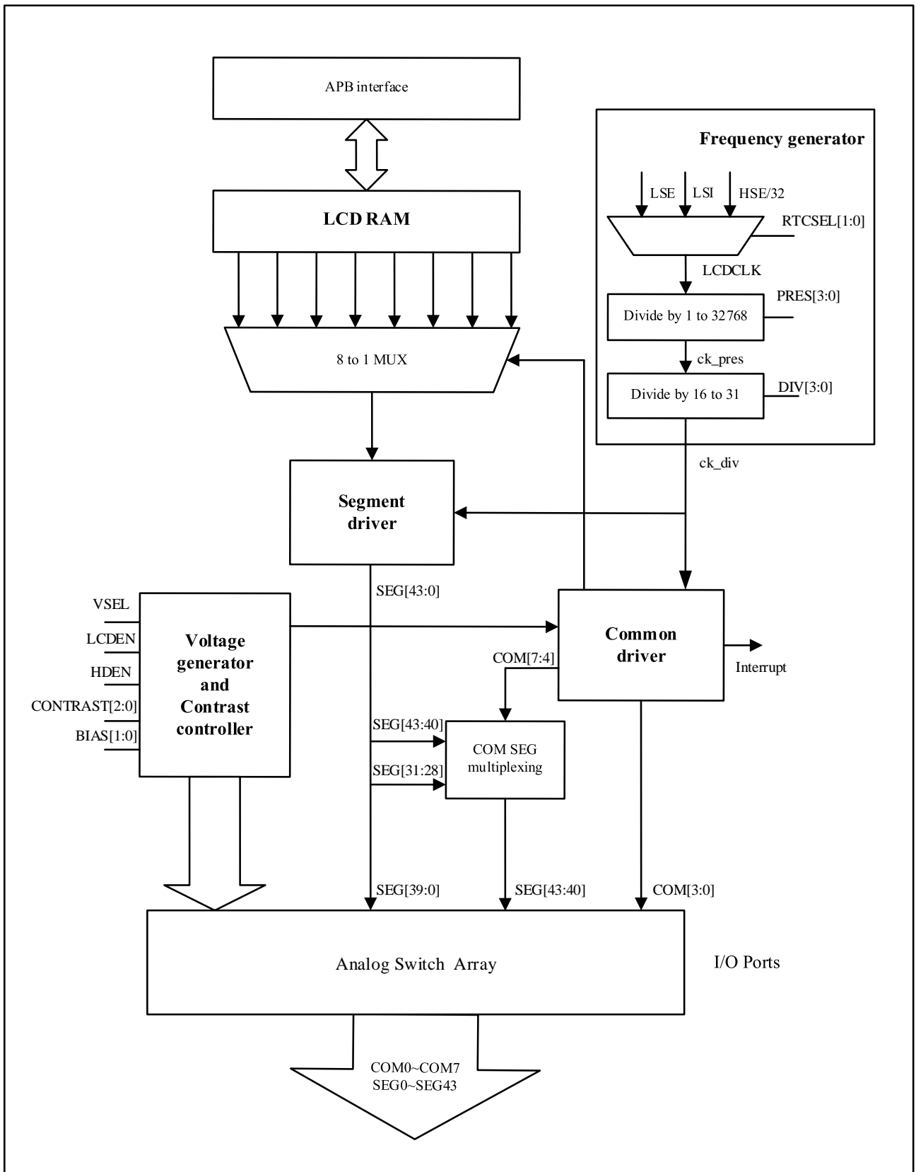
图 22-1 LCD 控制器框图
