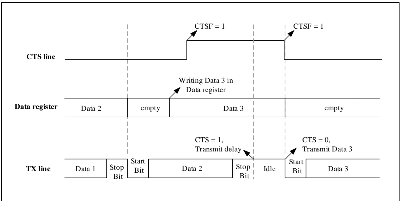
图 24-11 CTS 流控制
