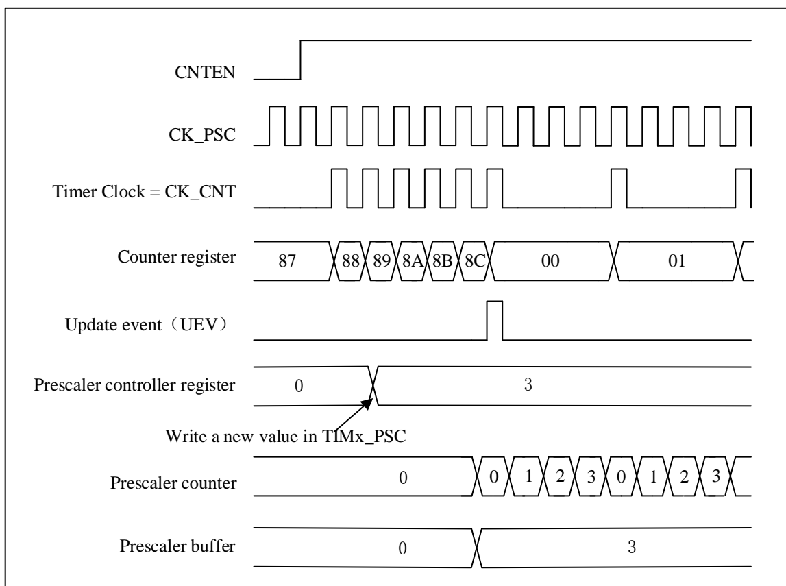
图 12-2 预分频器分频从 1 到 4 的计数器时序图
