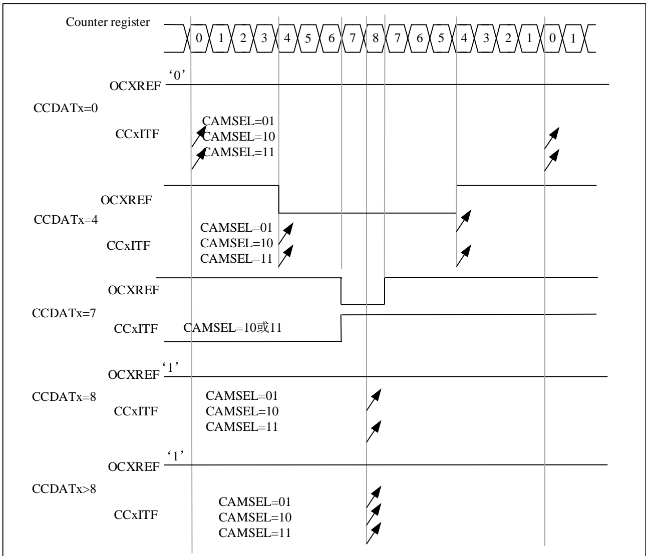
图 10-22 中央对齐的 PWM 波形(AR=8)
