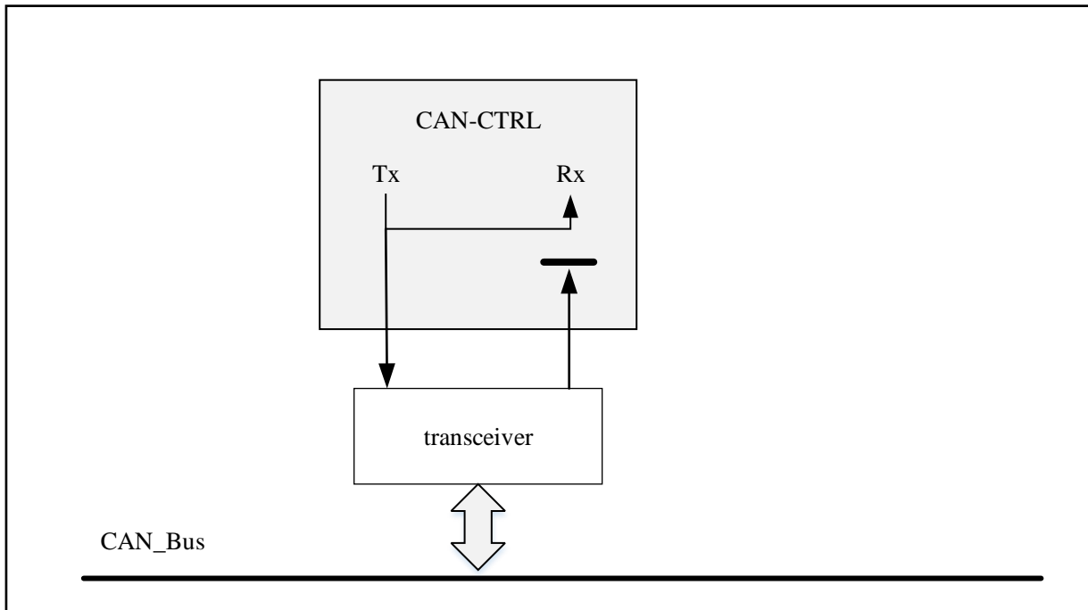
图 27-4 回环模式
