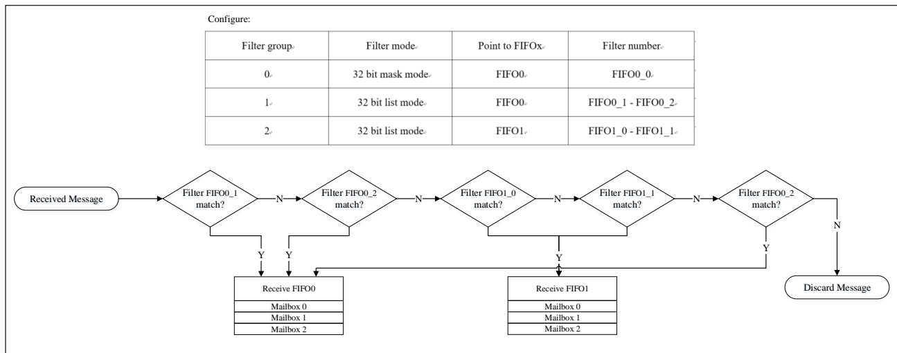
图 27-10 过滤机制示例
