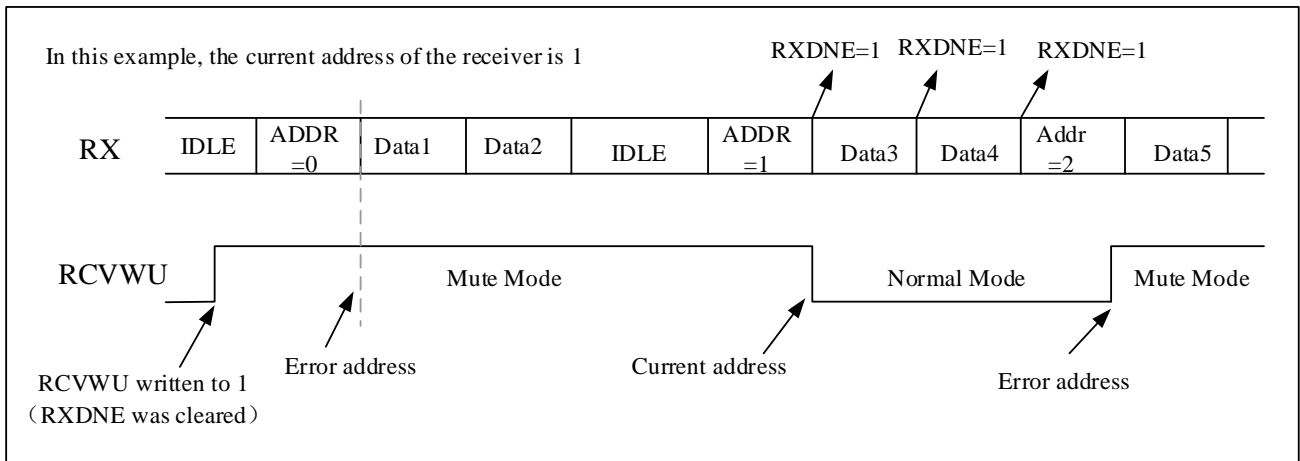
图 24-13 静默模式下的地址标识检测
