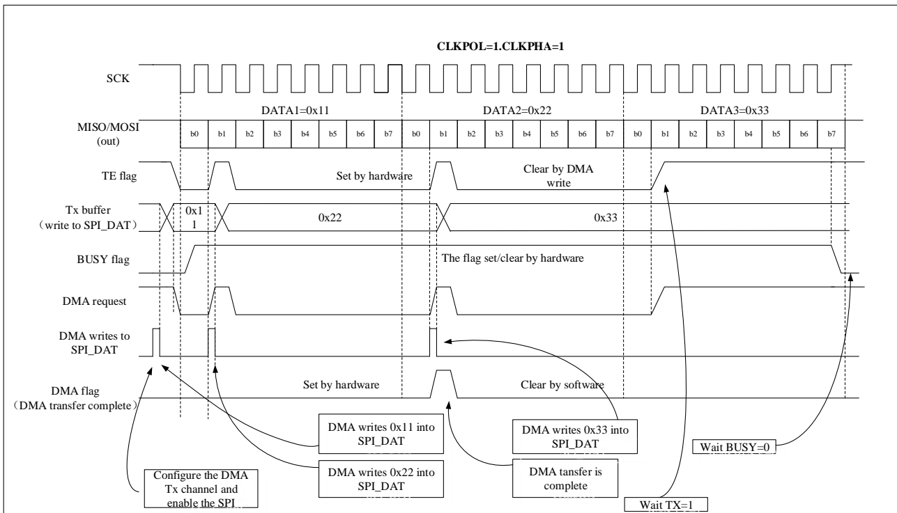
图 26-11 使用 DMA 发送
