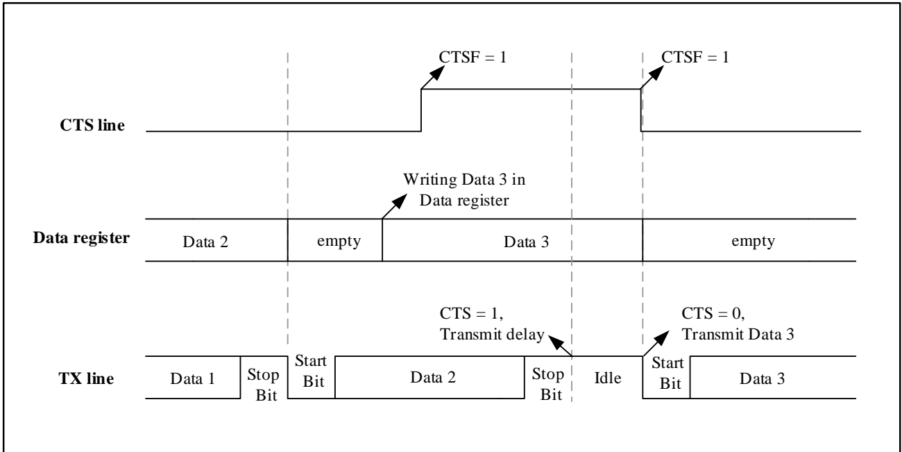
图 25-9 CTS 流控制
