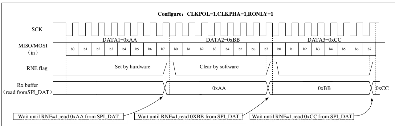
图 26-7 只接收模式 (BIDIRMODE = 0 并且 ROONLY = 1) 下连续传输时, RNE 变化示意图
