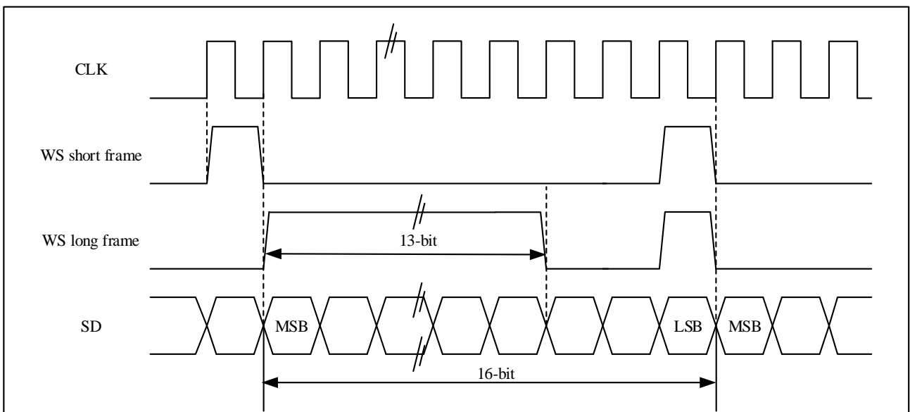
图 26-23 PCM 标准波形（16 位）
