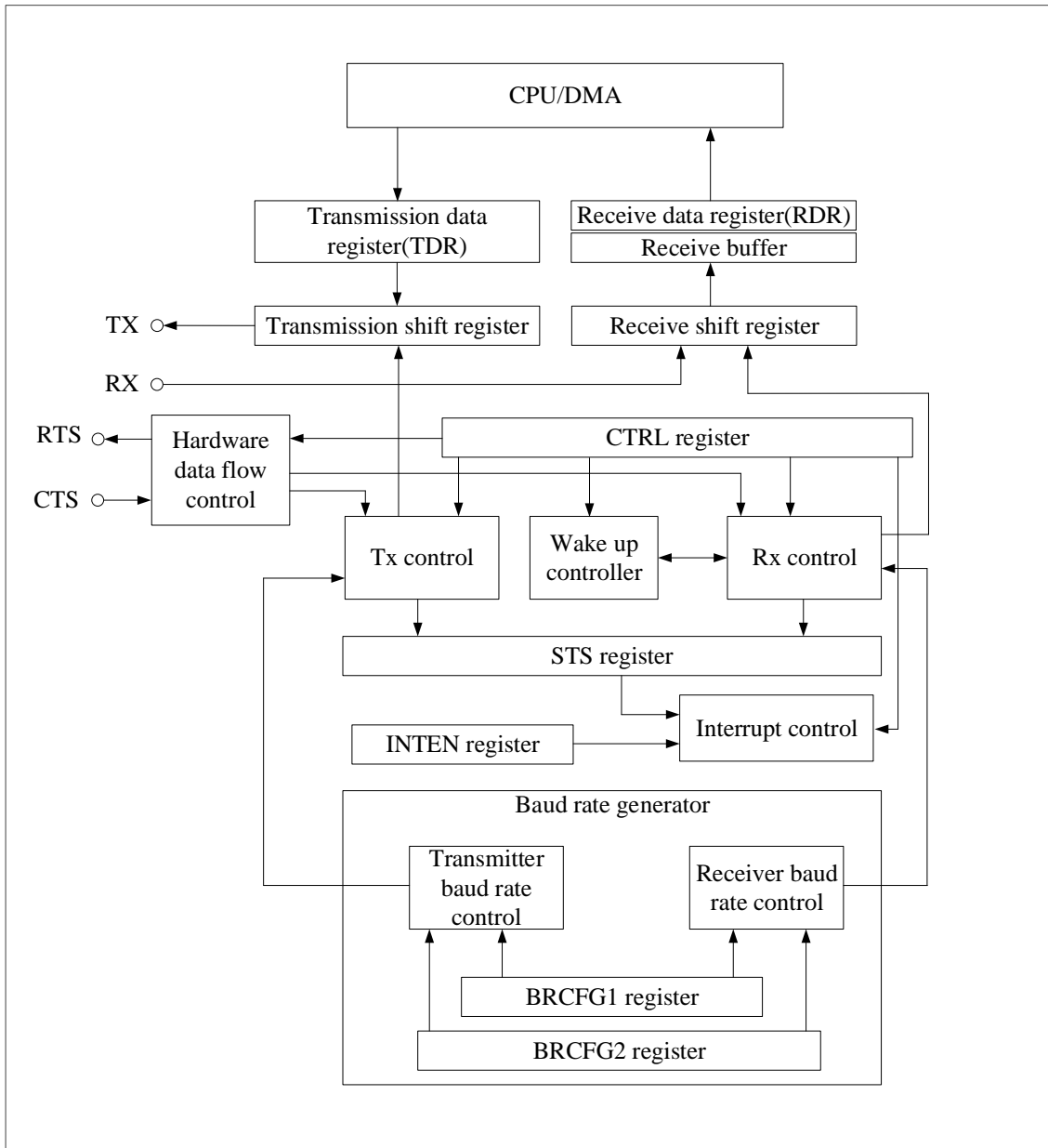
图 25-1 LPUART 框图
