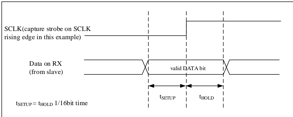
图 24-17 RX 数据采样/保持时间
