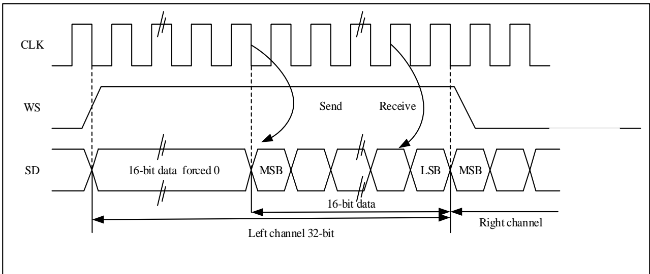
图 26-22 LSB 对齐 16 位数据扩展到 32 位包帧，CLKPOL = 0
