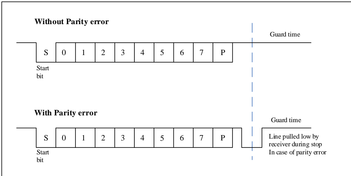
图 24-22 ISO7816-3 异步协议
