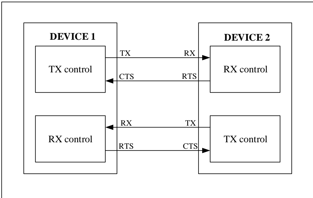
图 24-9 两个 USART 间的硬件流控制
