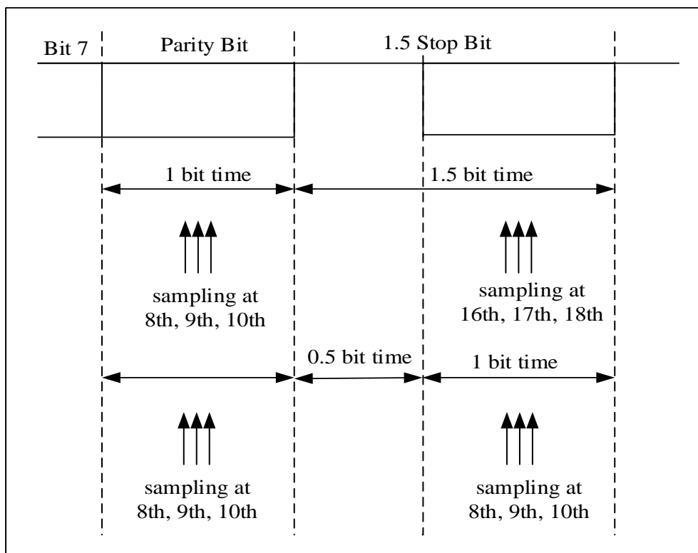
图 24-23 使用 1.5 停止位检测奇偶检验错误
