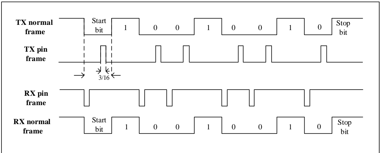
图 24-19 IrDA 数据调制(3/16)-正常模式
