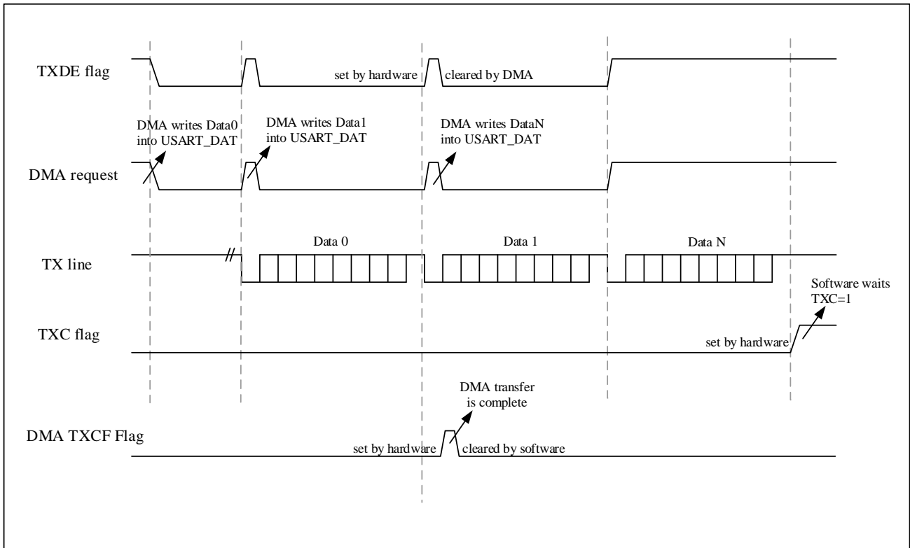
图 24-7 DMA 发送
