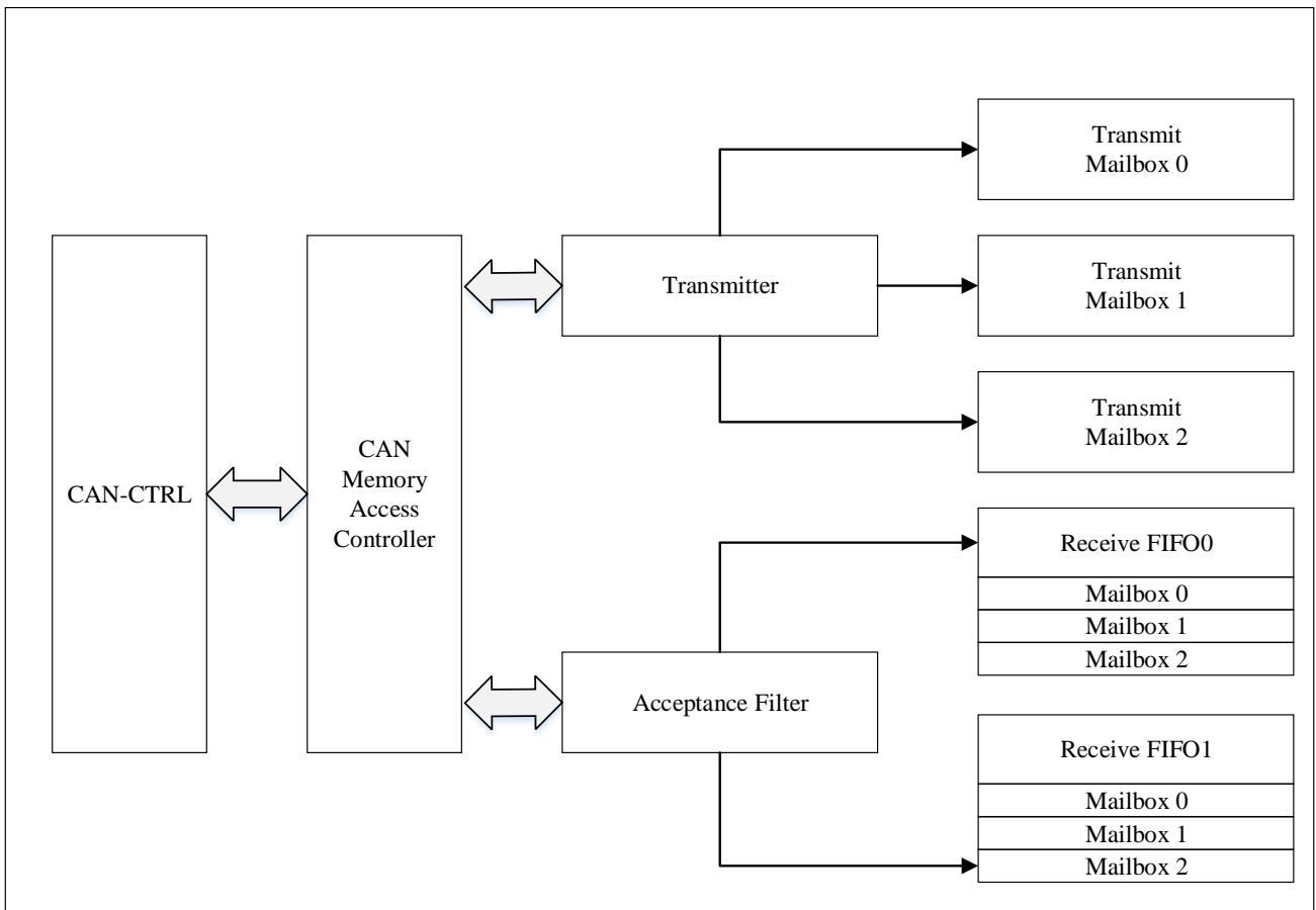
图 27-3 单 CAN 框图
