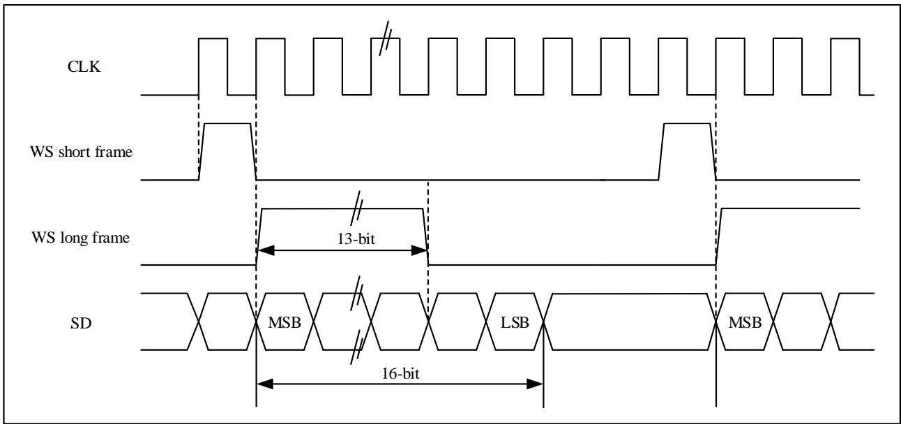
图 26-24 PCM 标准波形（16 位扩展到 32 位包帧）
