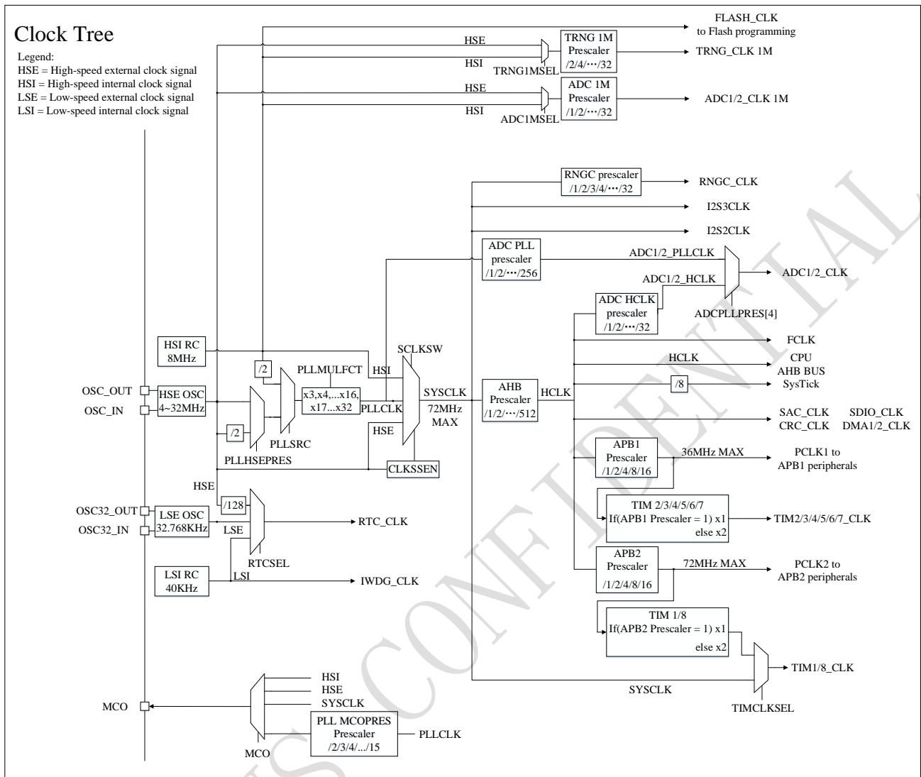
图 2-2 时钟树
