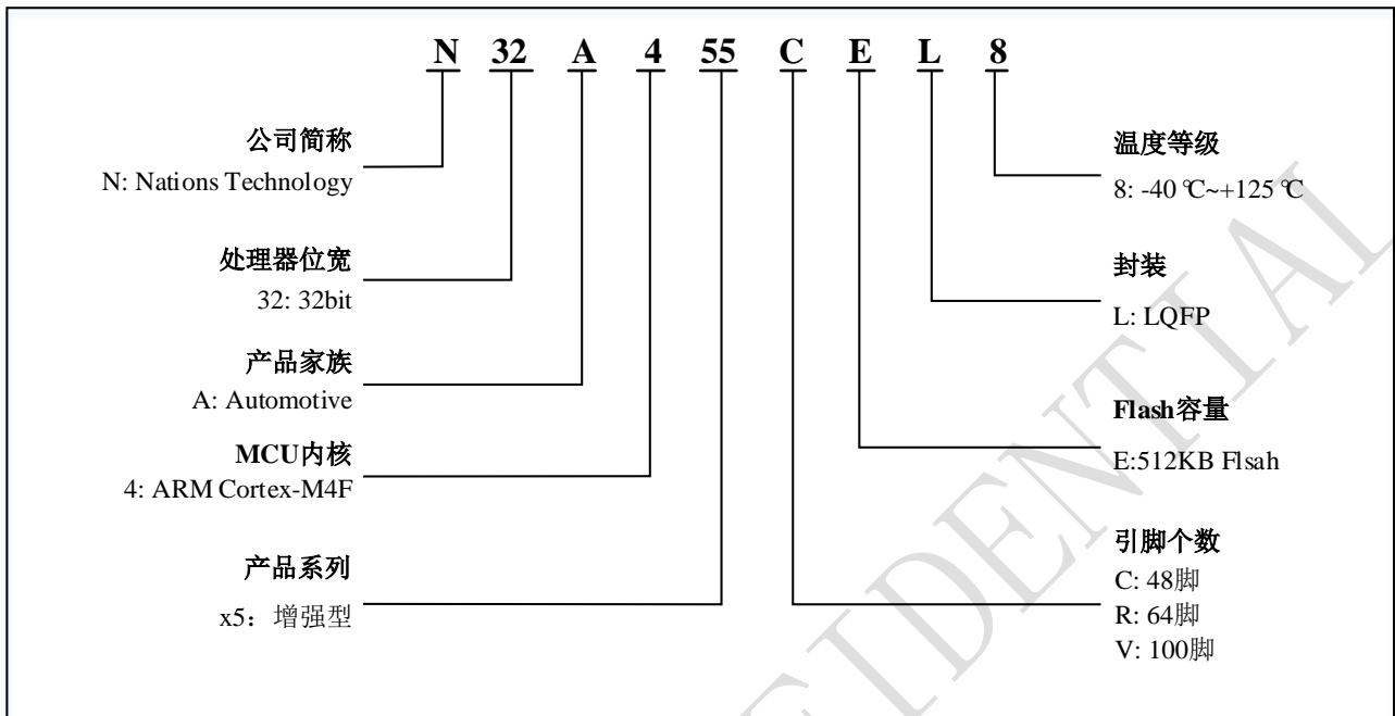
图 1-2 N32A455xxL8系列订货代码信息图示
