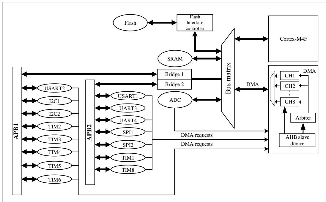
图 7-1 DMA 框图
