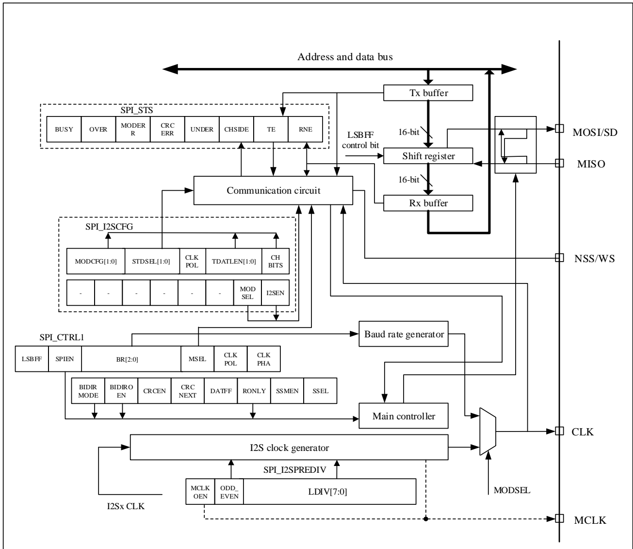
图 19-13 I 2 S 框图
