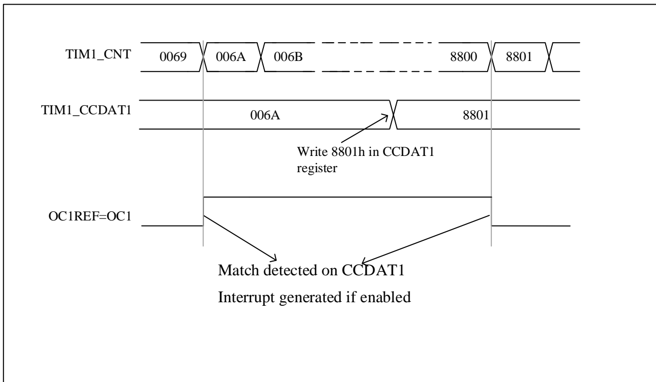
图 10-18 输出比较模式，开启 OC1
