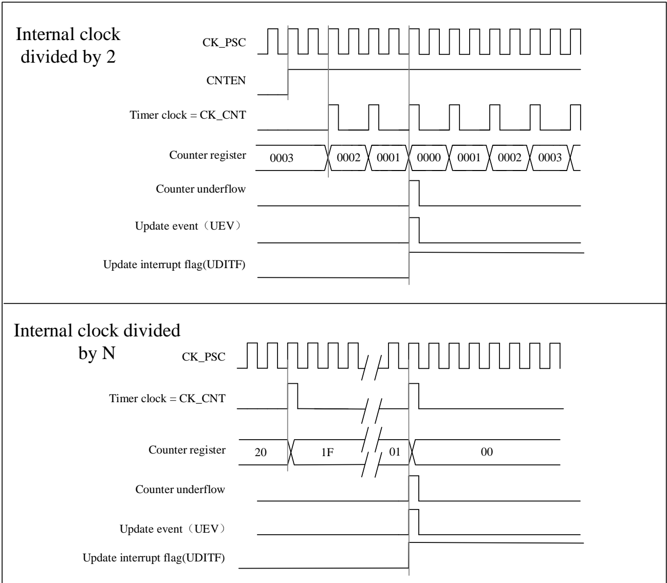
图 9-7 内部时钟分频因子 = 2/N，中央对齐时序图
