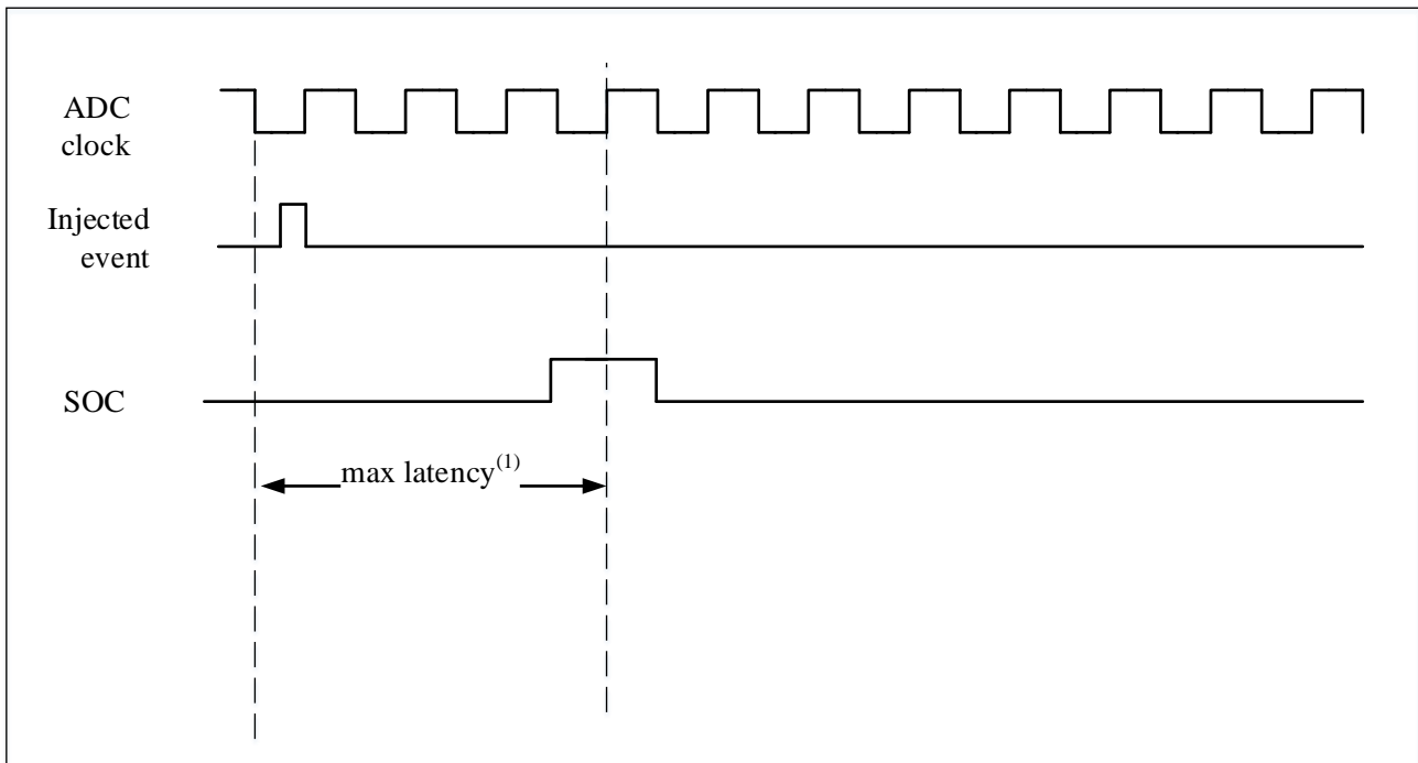
图 15-5 注入转换延时
