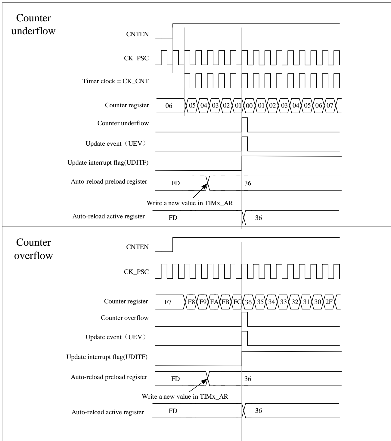
图 9-8 包含计数器上溢和下溢的中央对齐时序图(ARPEN=1)
