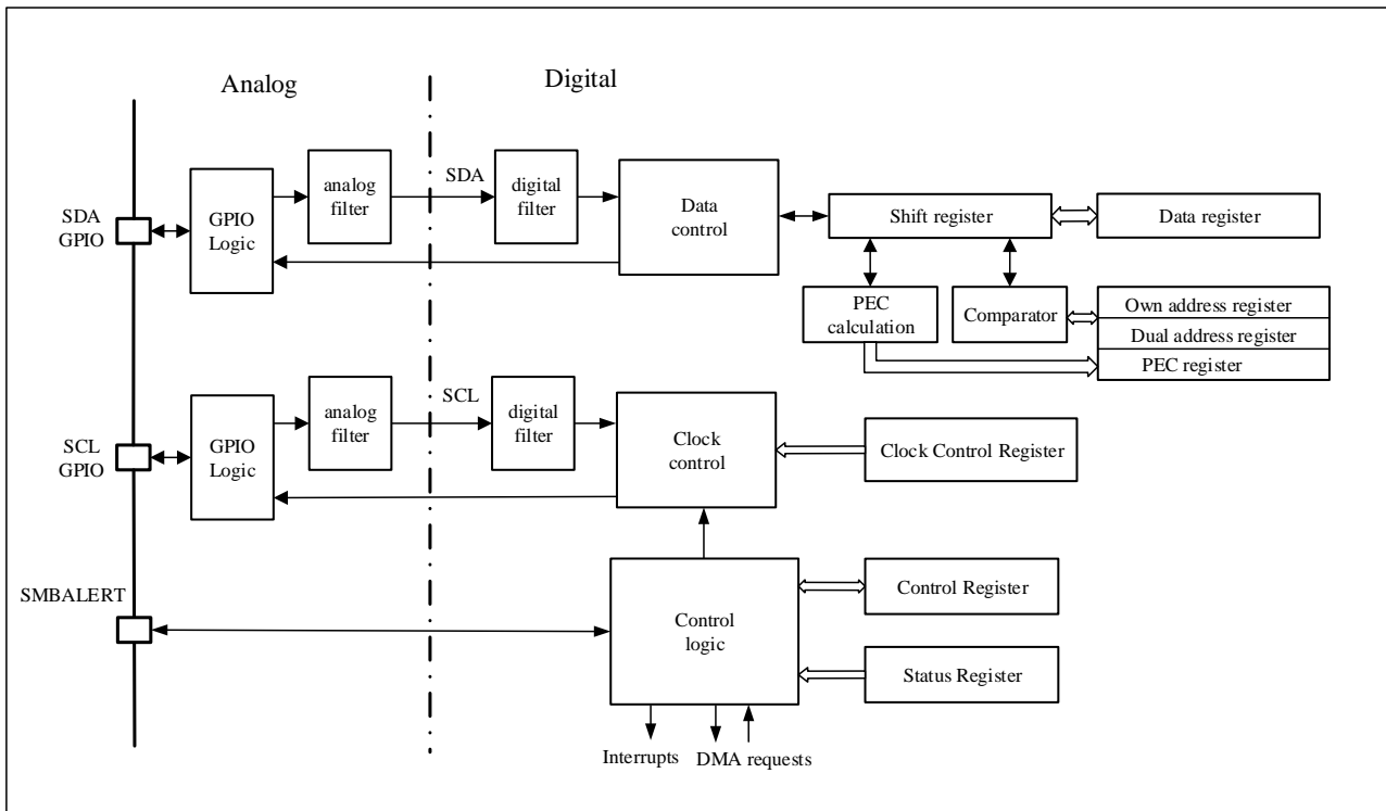
图 17-1 I 2 C 功能框图
