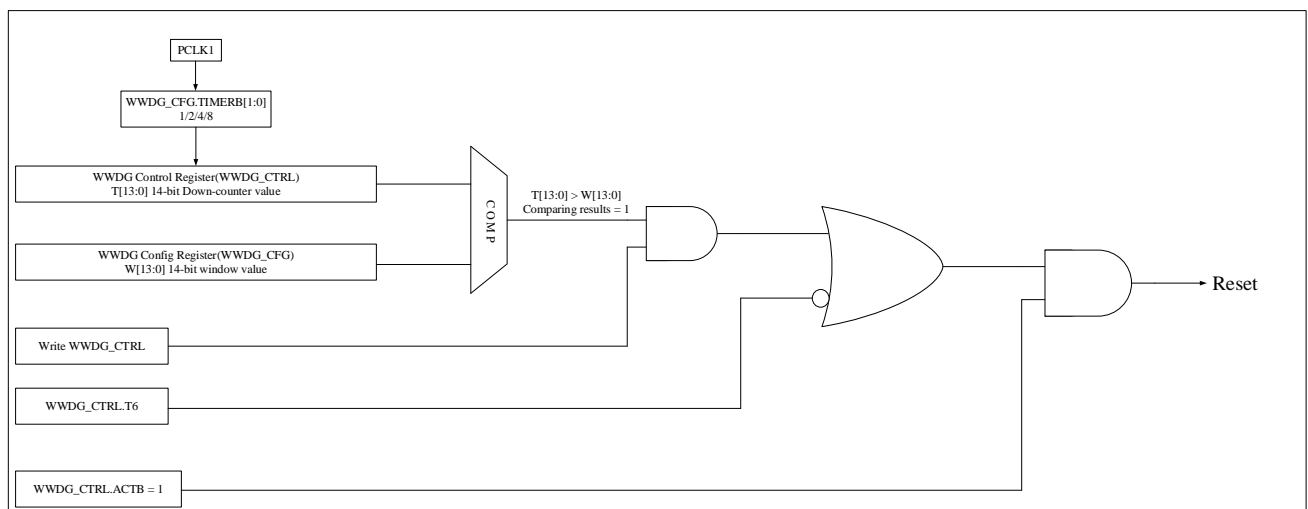
图 14-1 窗口看门狗功能框图
