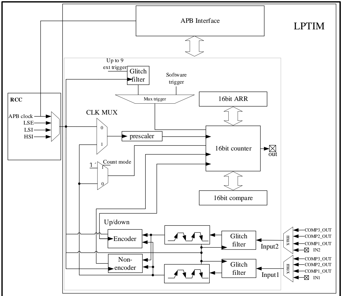
图 12-1 LPTIM 主框图
