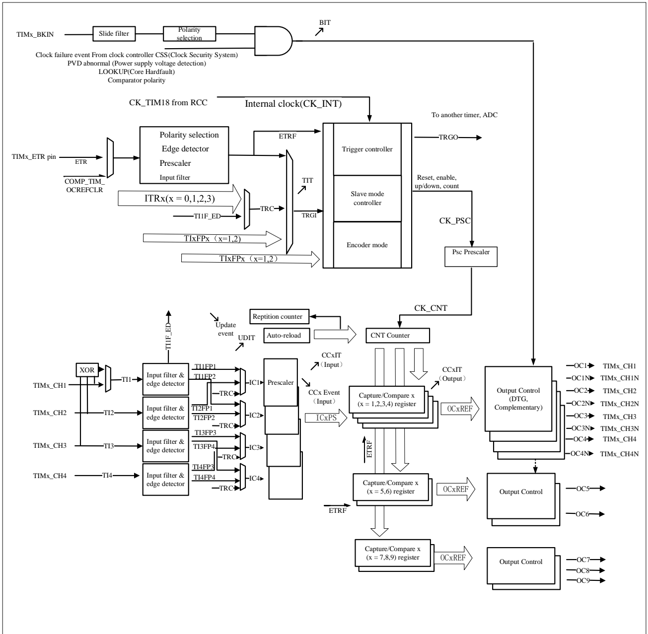
图 9-1 TIM1 框图
