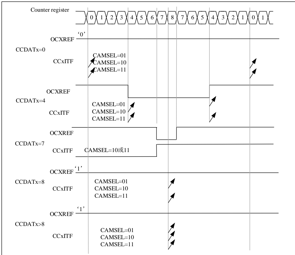
图 9-27 中央对齐的 PWM 波形 (AR=8)
