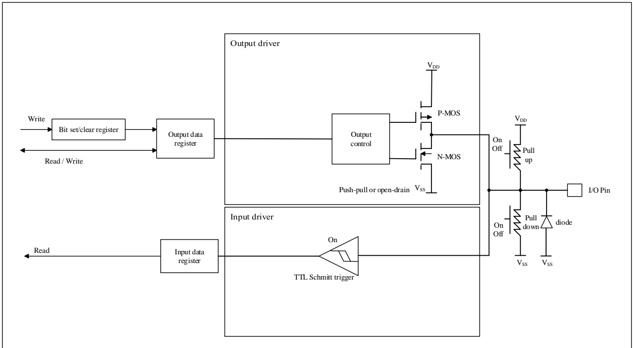
图 5-4 输出模式
