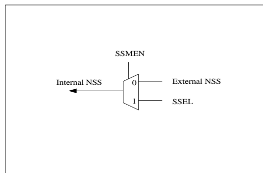
图 19-2 硬件/软件的从选择管理
