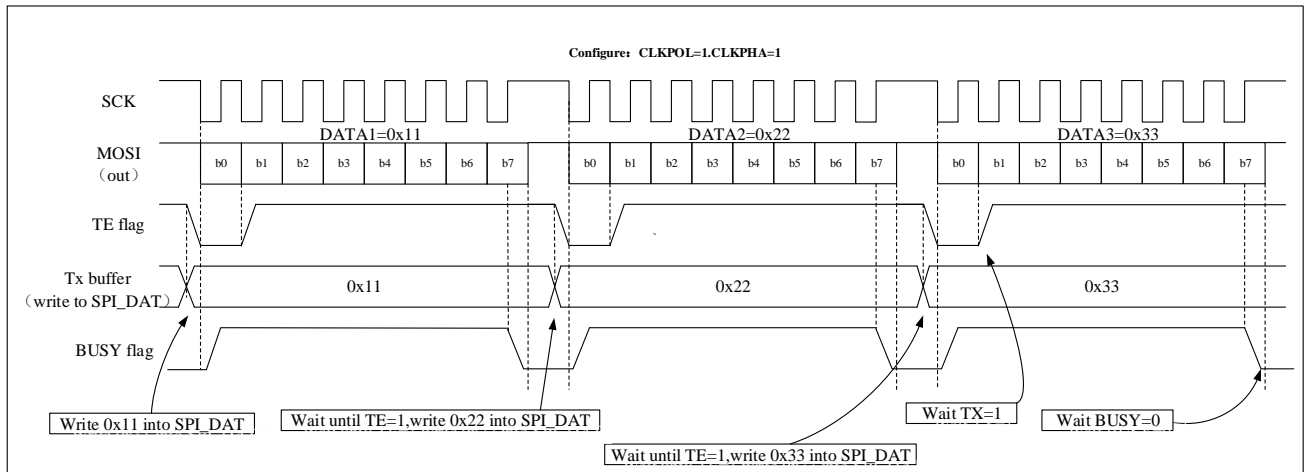
图 19-10 BIDIRMODE=0, RONLY=0 非连续传输发送时，SPI_STS.TE/BUSY 变化示意图
