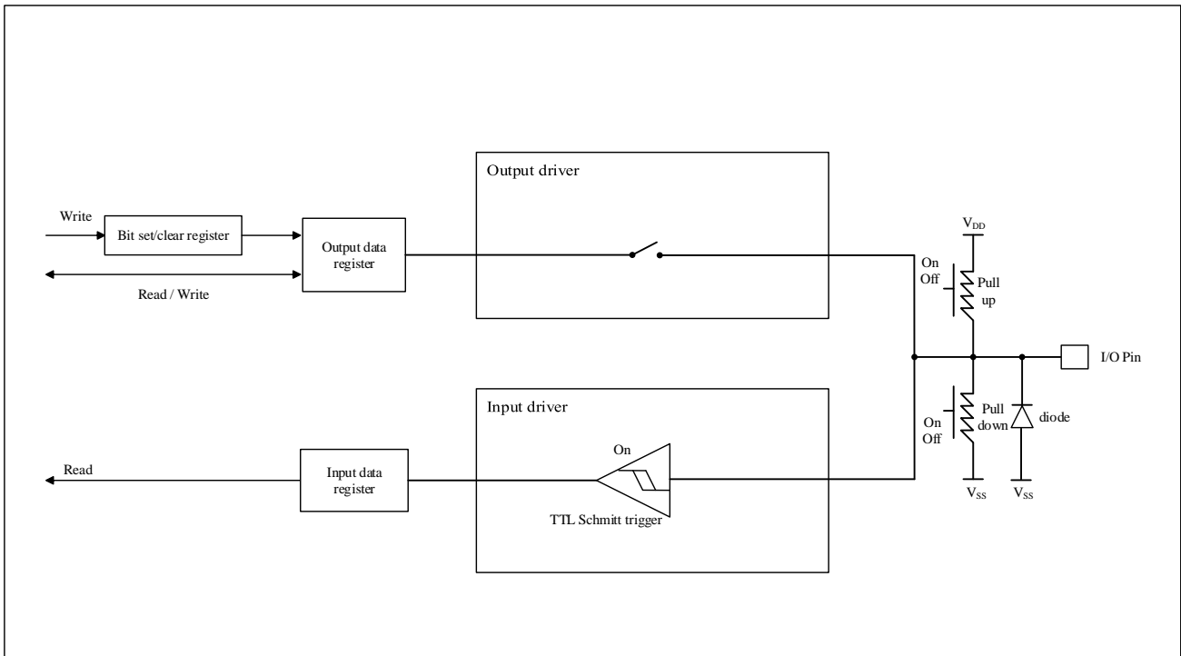
图 5-3 浮空输入/上拉/下拉配置模式
