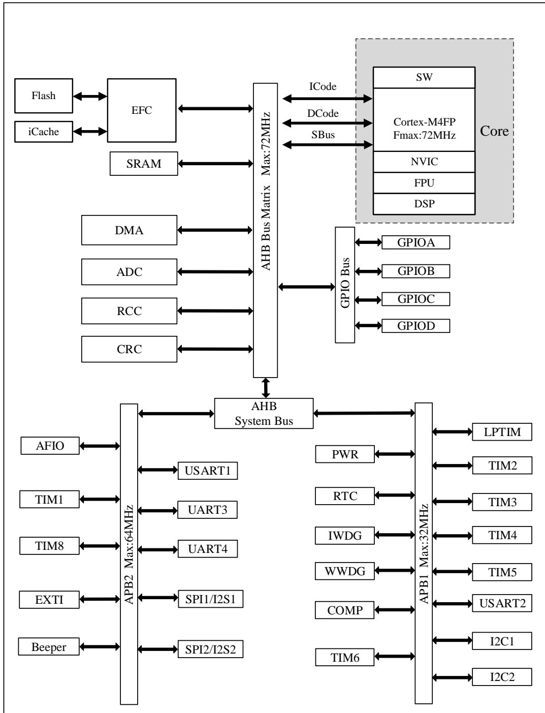
图 2-1 总线架构图
