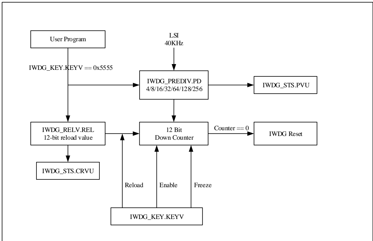
图 13-1 独立看门狗功能框图
