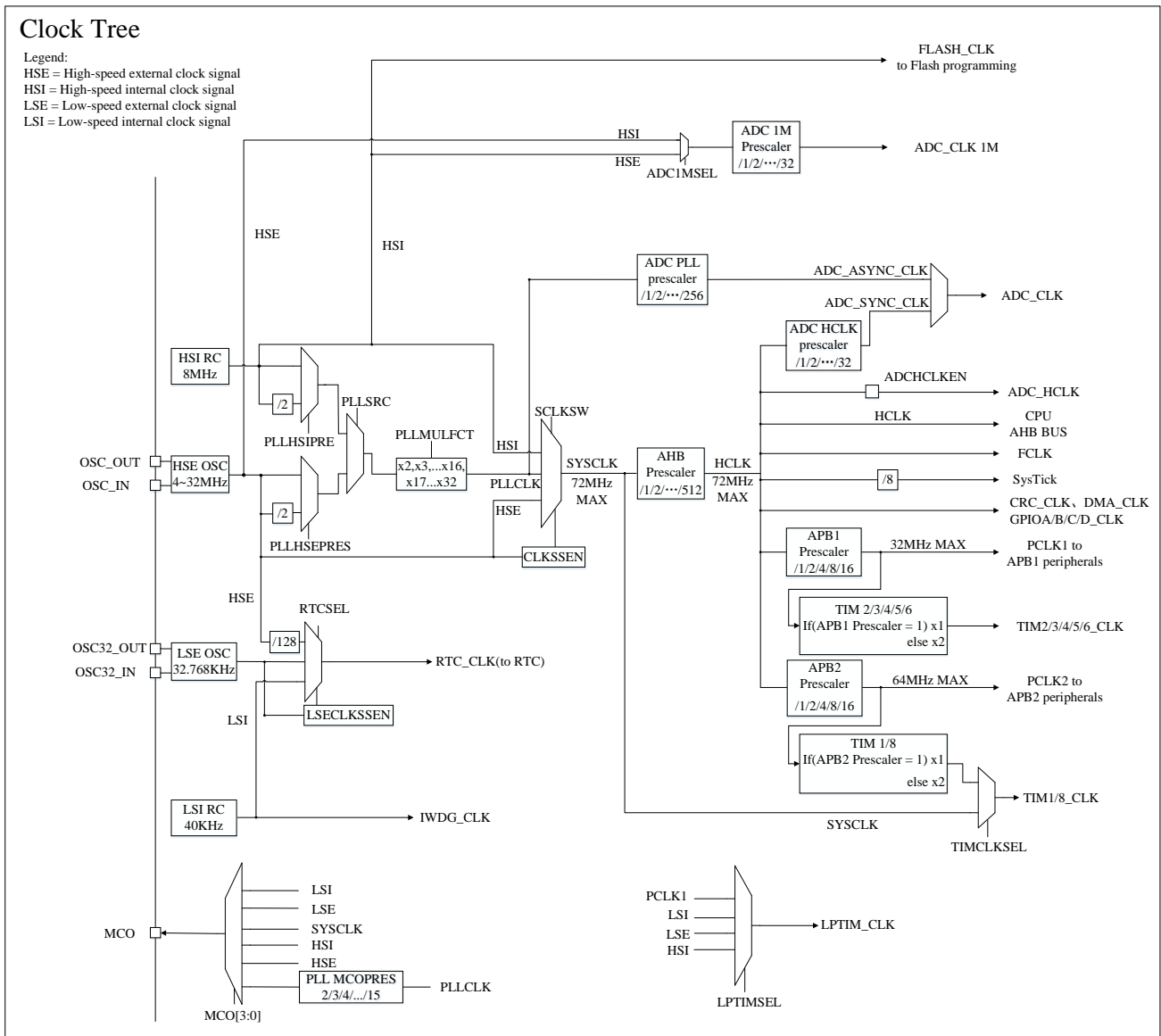
图 4-2 时钟树
