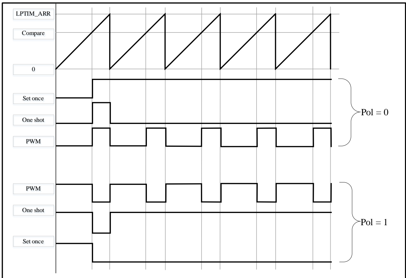
图 12-6 波形发生器
