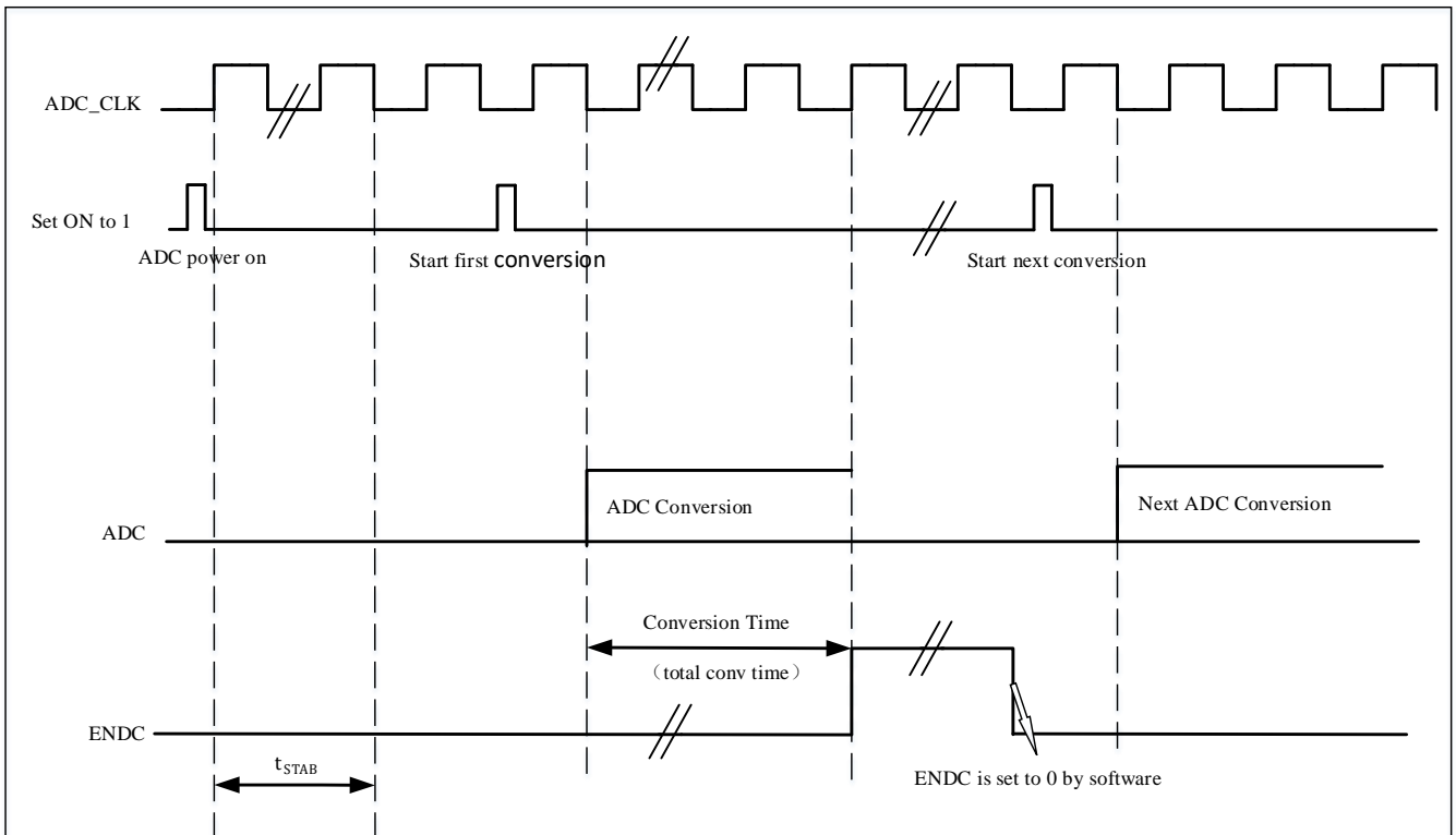
图 15-4 时序图
