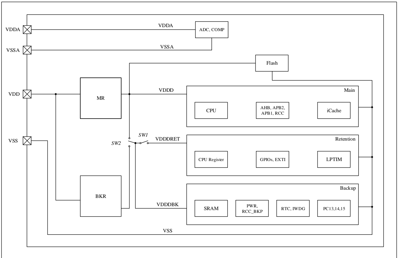
图 3-1 电源框图
