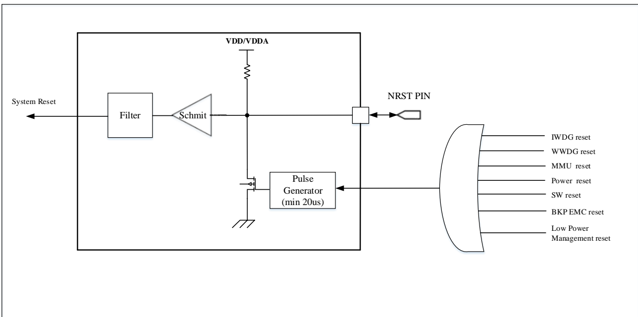
图 4-1 复位电路
