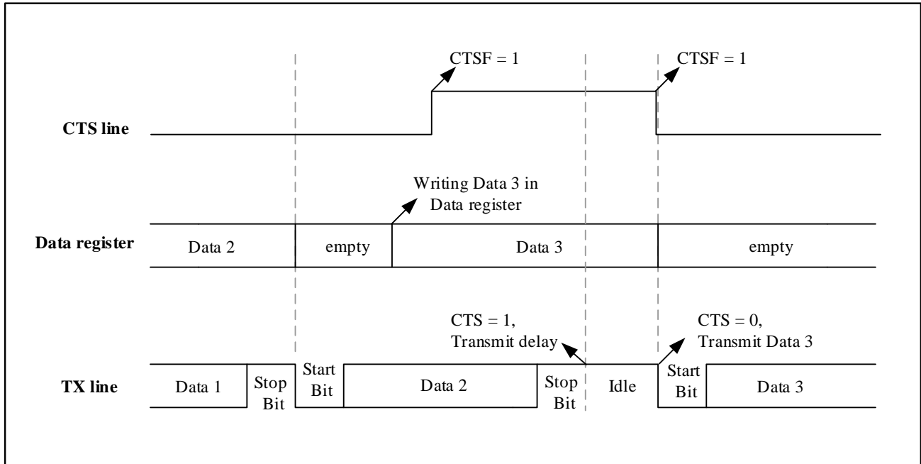
图 18-11 CTS 流控制
