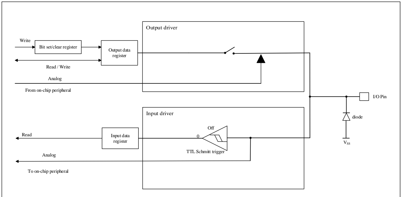
图 5-5 高阻抗模拟输入配置
