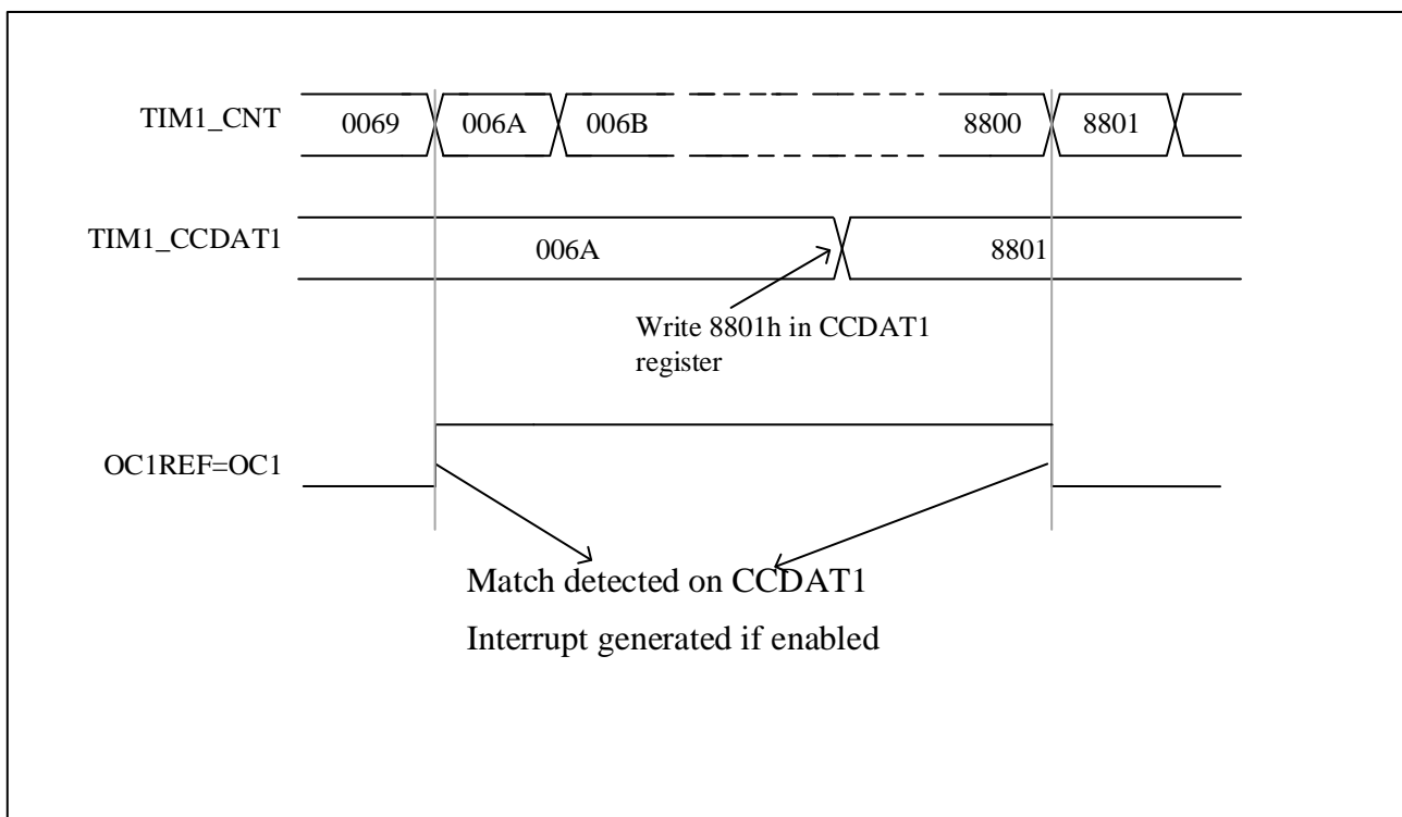
图 9-26 输出比较模式，开启 OC1
