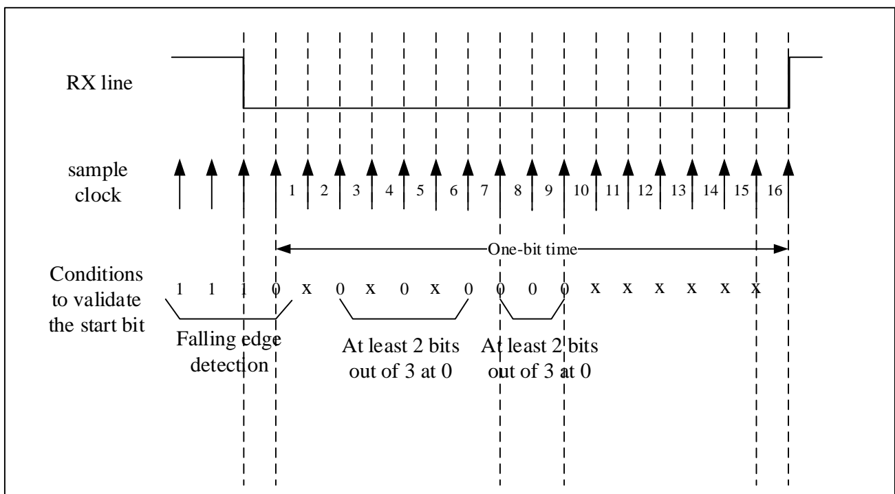
图 18-6 起始位检测
