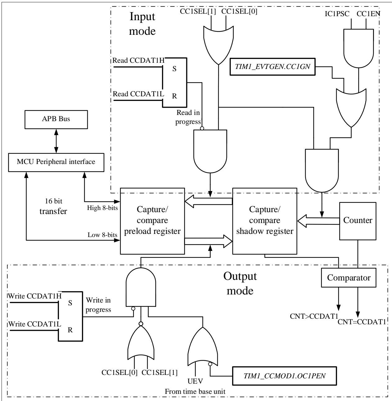
图 9-23 通道 x 的输出部分 (TIM1 的 x=1,2,3,4; TIM8 的 x=1,2,3。以通道 1 为例子)
