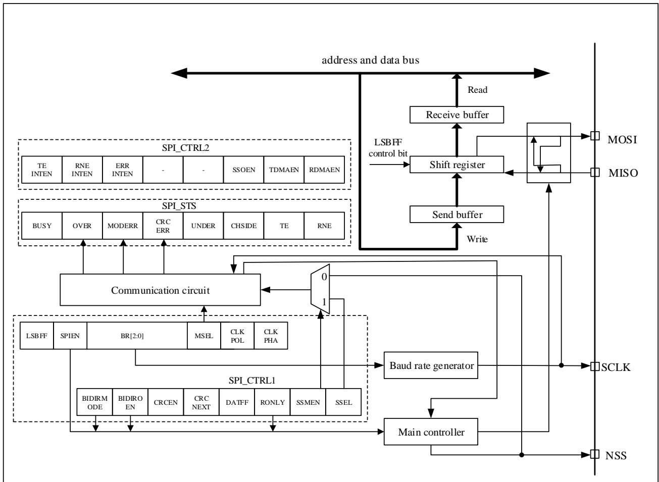
图 19-1 SPI 框图
