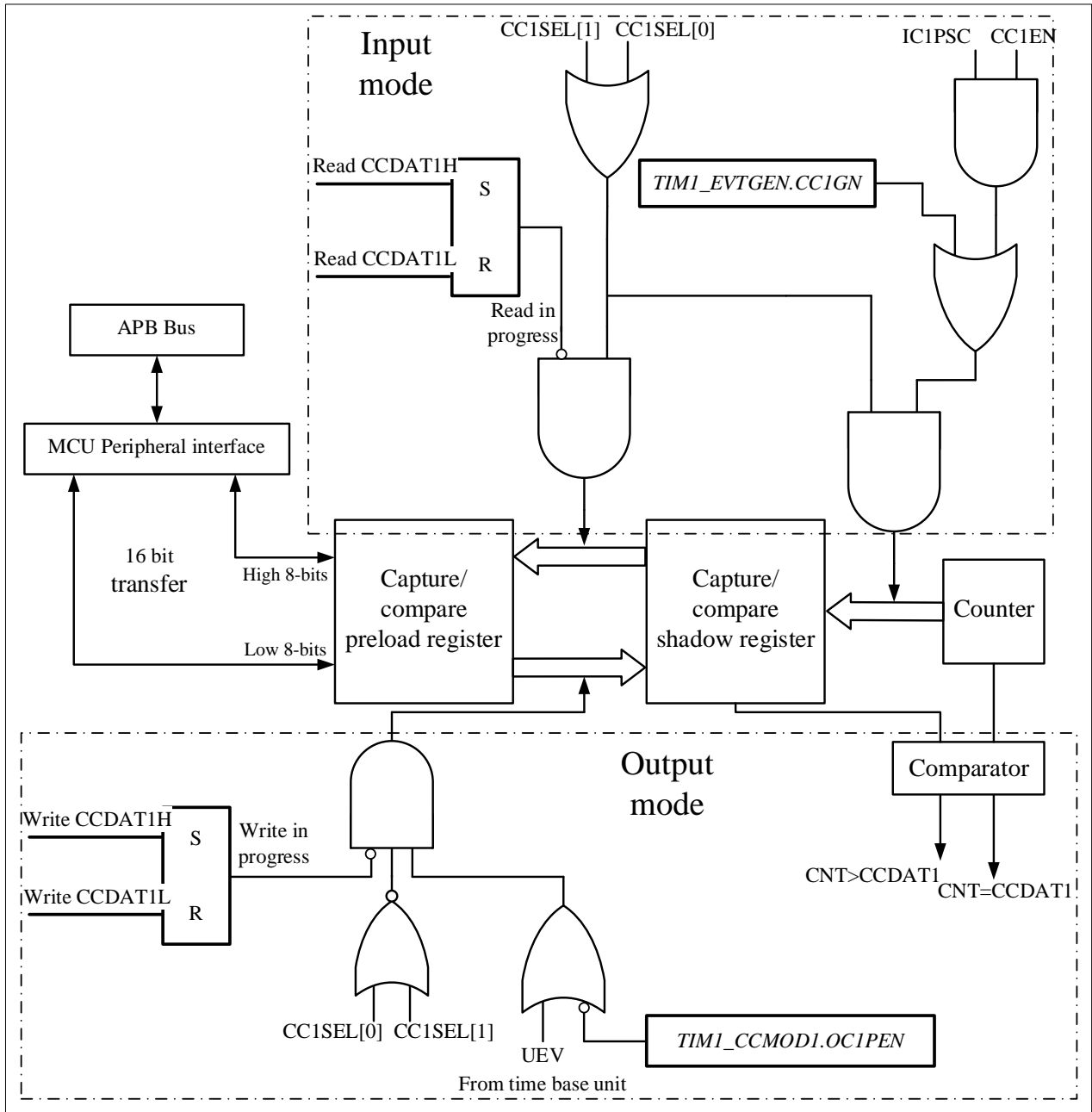
图 10-14 捕获/比较通道 1 主电路
