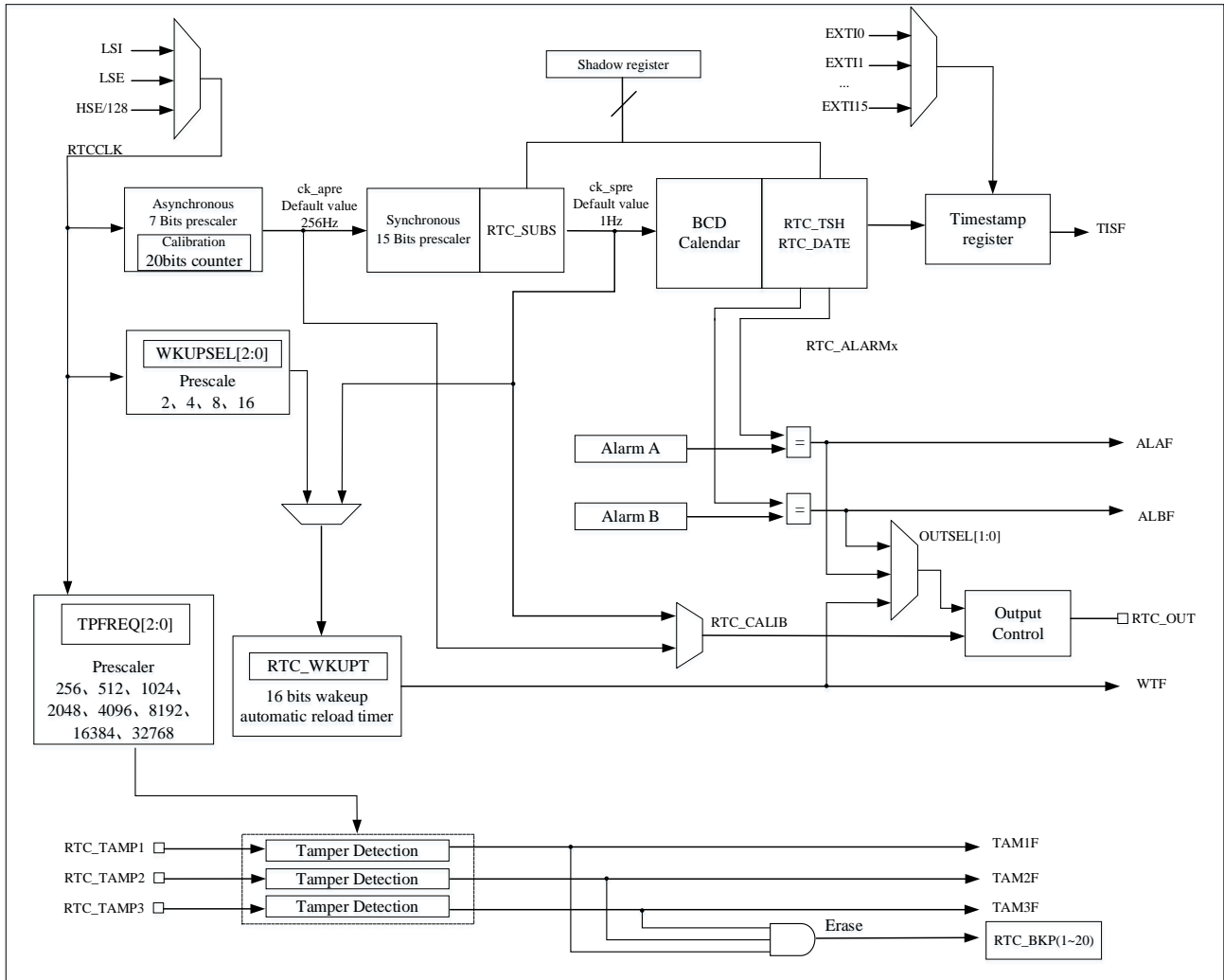
图 20-1 RTC 功能框图
