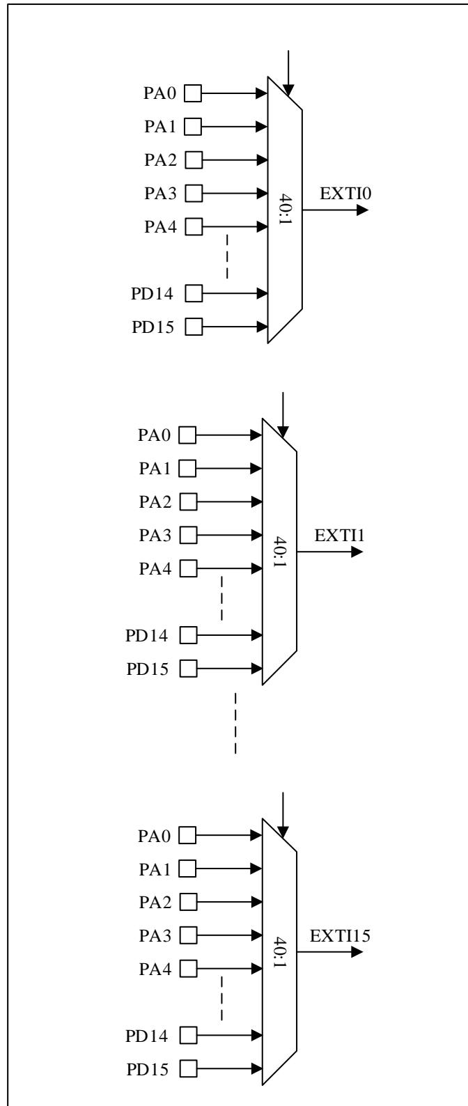
图 6-2 外部中断 GPIO 映射
