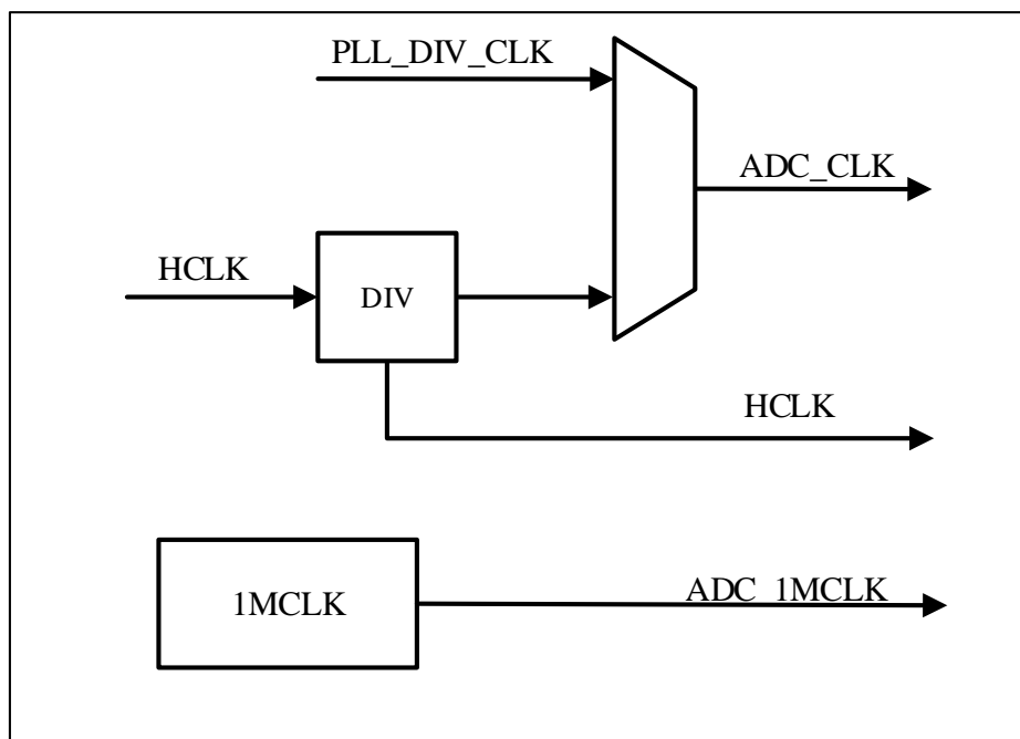
图 15-2 ADC 时钟
