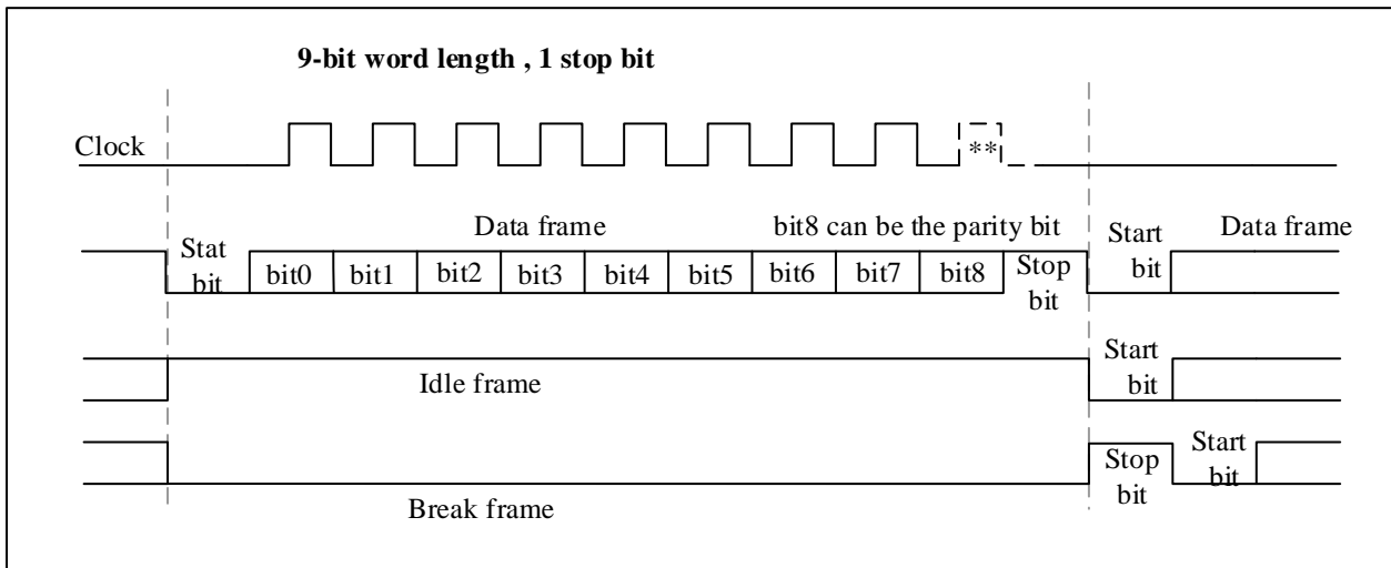
图 18-3 字长=9 设置
