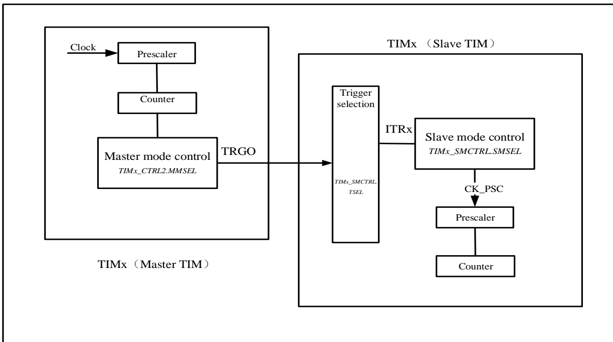
图 10-27 主/从定时器的例子
